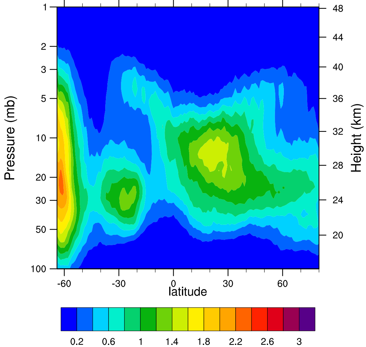
HIRDLSv6 2005d229 ClONO2_Ascending (ppbv)
