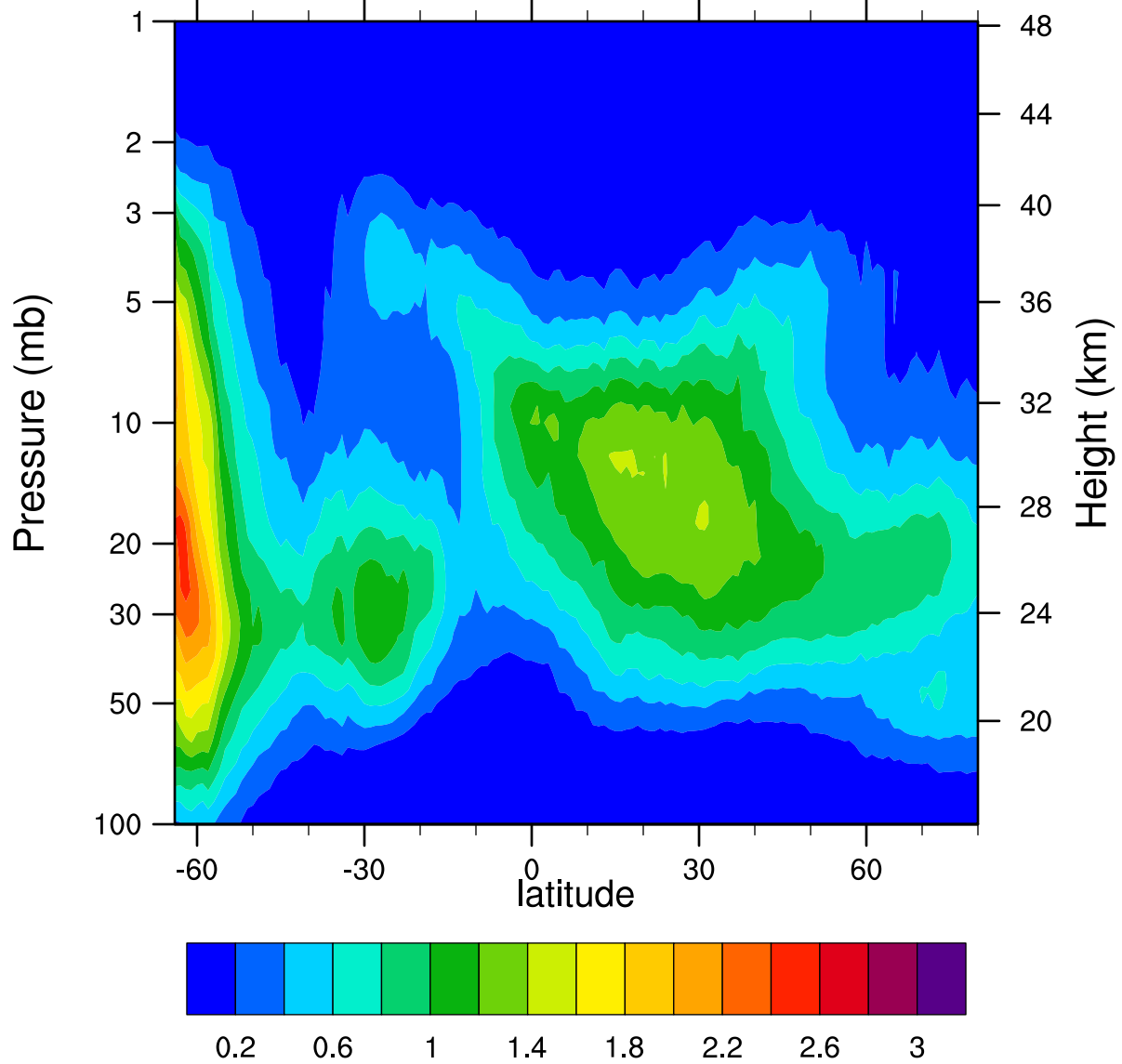
HIRDLSv6 2005d217 ClONO2_Ascending (ppbv)
