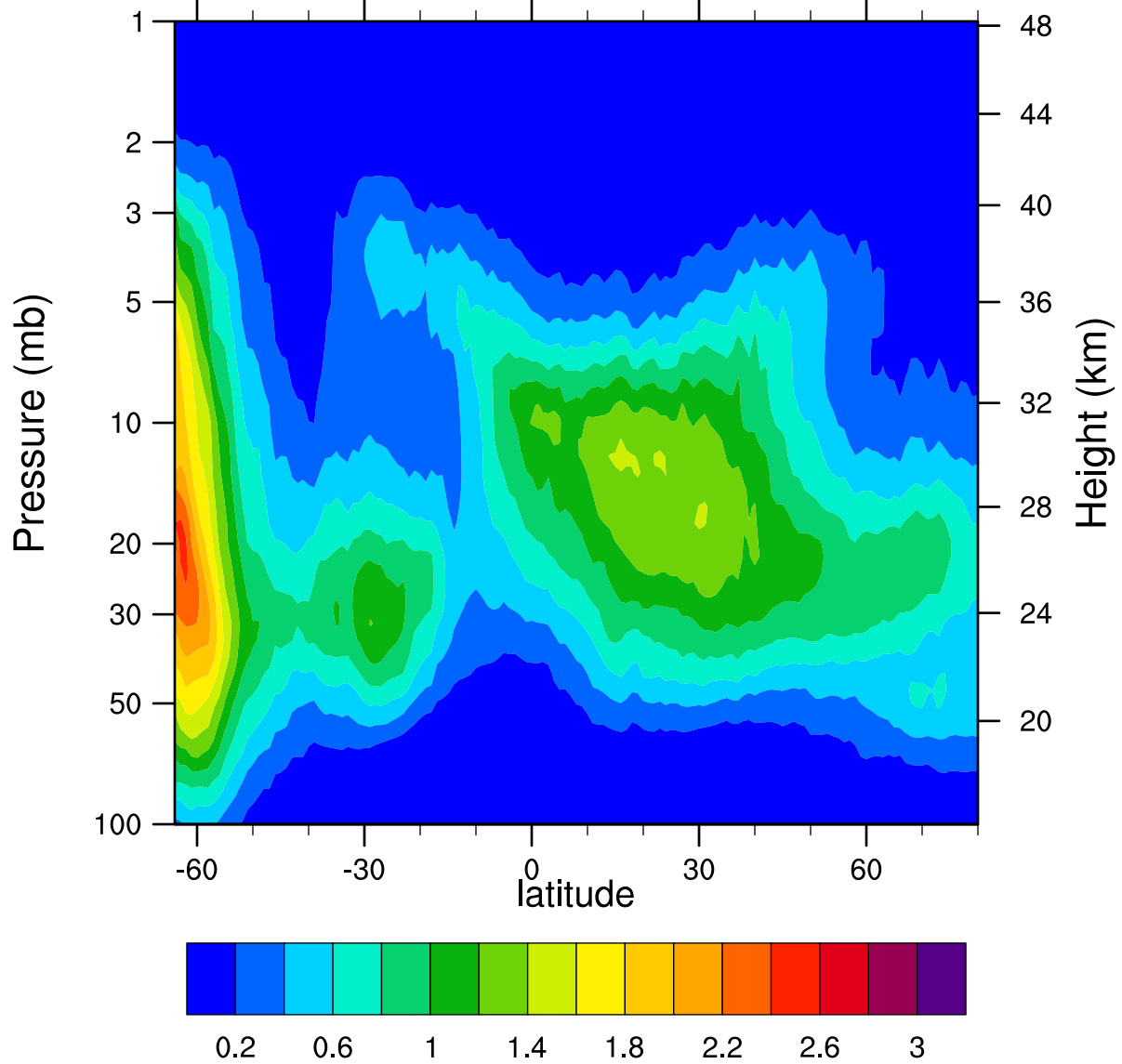
HIRDLSv6 2005d216 ClONO2_Ascending (ppbv)
