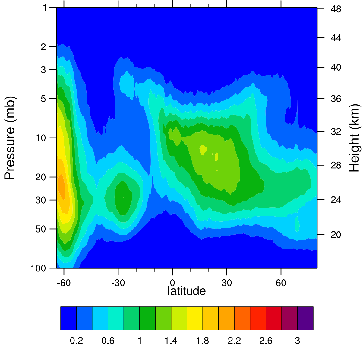
HIRDLSv6 2005d211 ClONO2_Ascending (ppbv)
