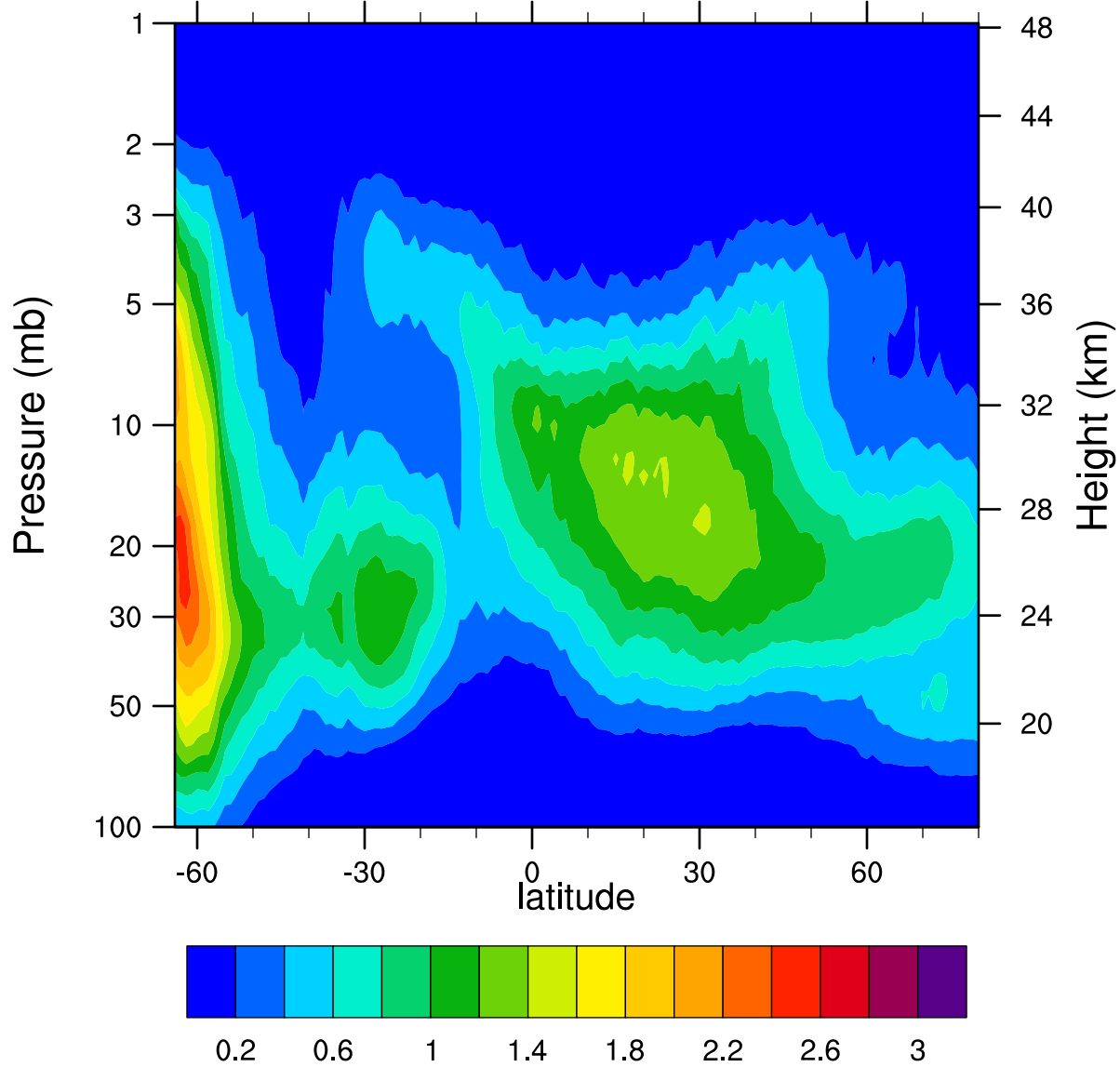
HIRDLSv6 2005d218 ClONO2_Ascending (ppbv)
