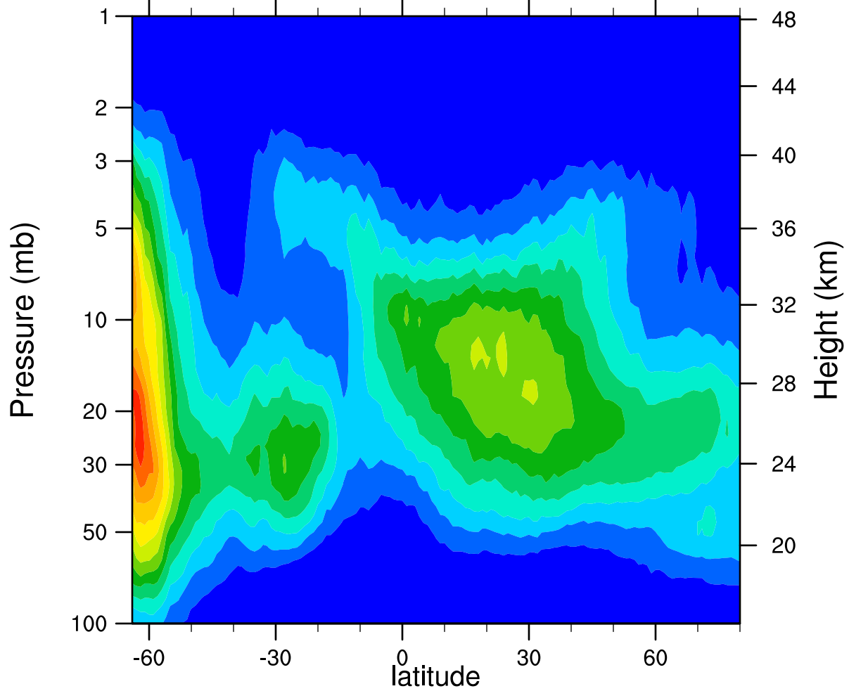
HIRDLSv6 2005d219 ClONO2_Ascending (ppbv)
