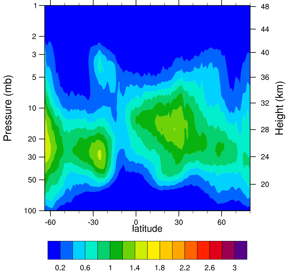
HIRDLSv6 2005d284 ClONO2_Ascending (ppbv)
