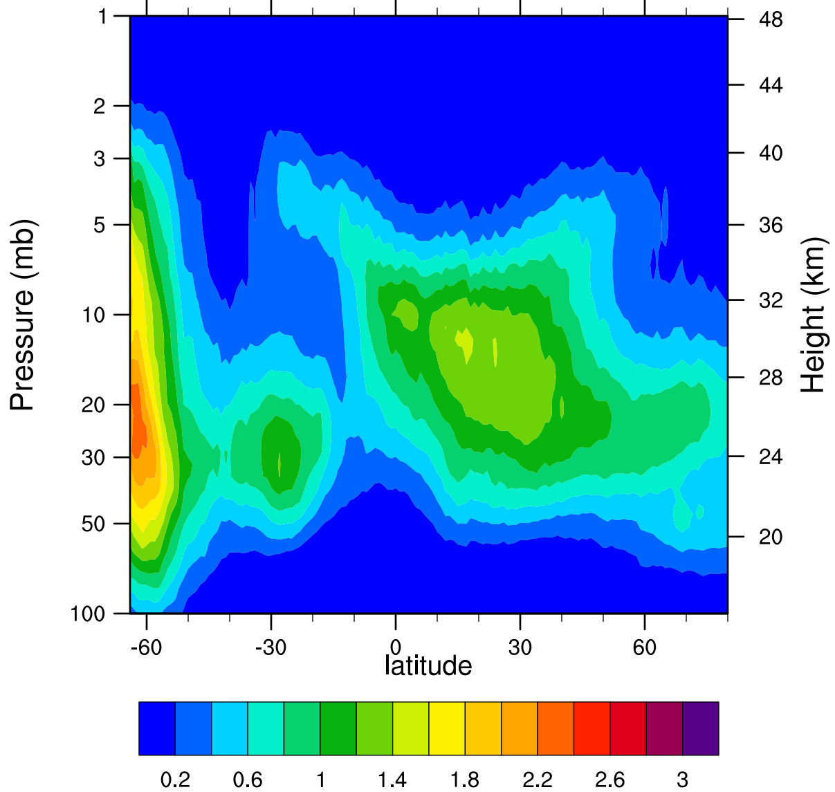
HIRDLSv6 2005d214 ClONO2_Ascending (ppbv)
