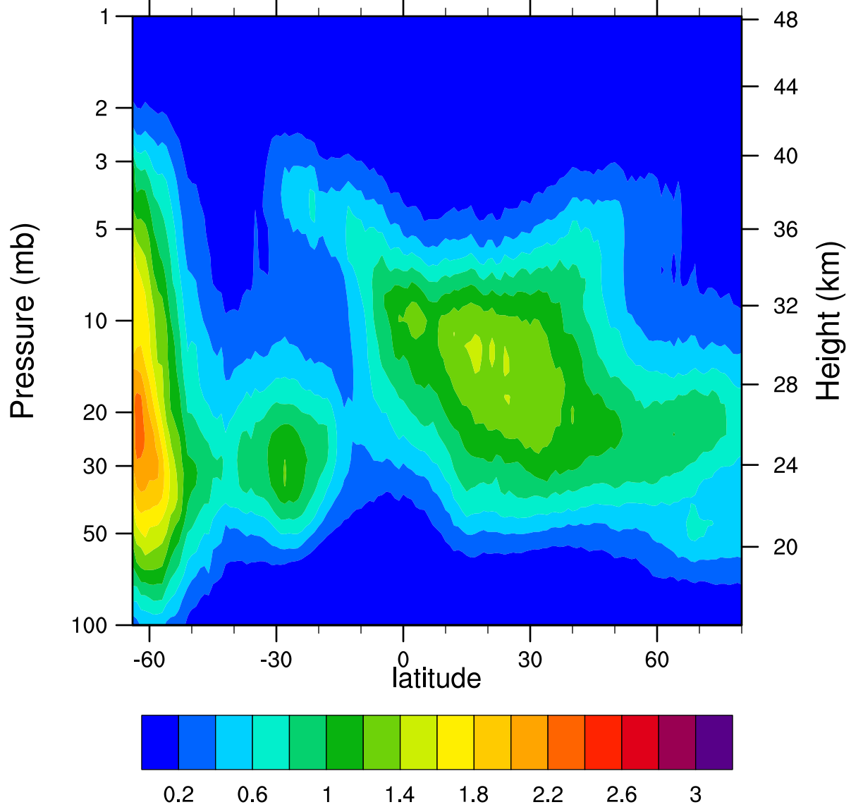
HIRDLSv6 2005d213 ClONO2_Ascending (ppbv)
