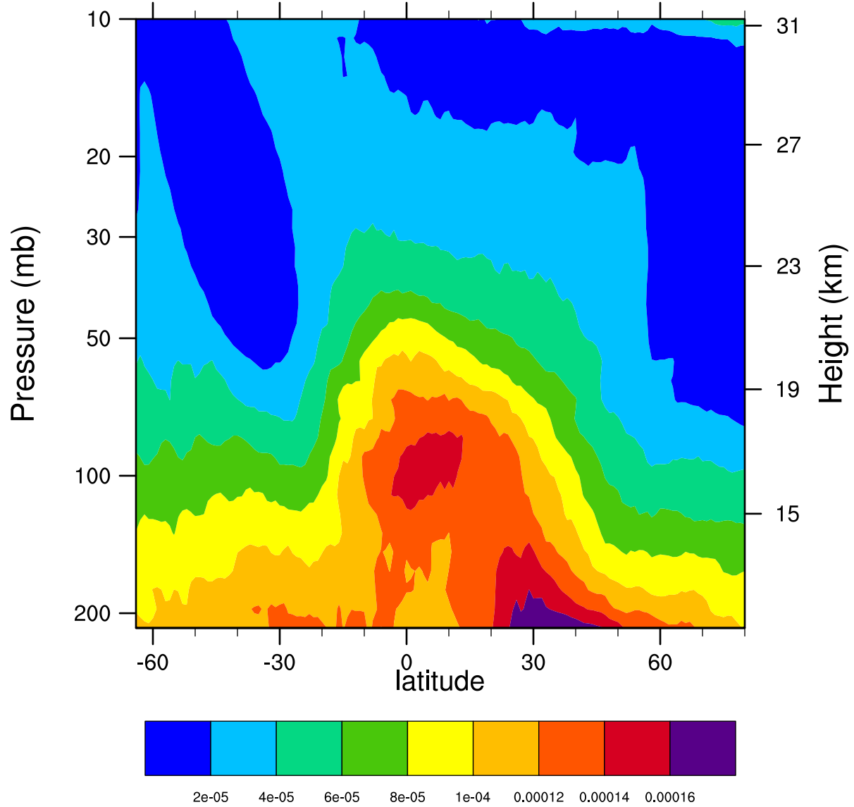
2005d160 12.1MicronExtinction_Combined (km -1 )
