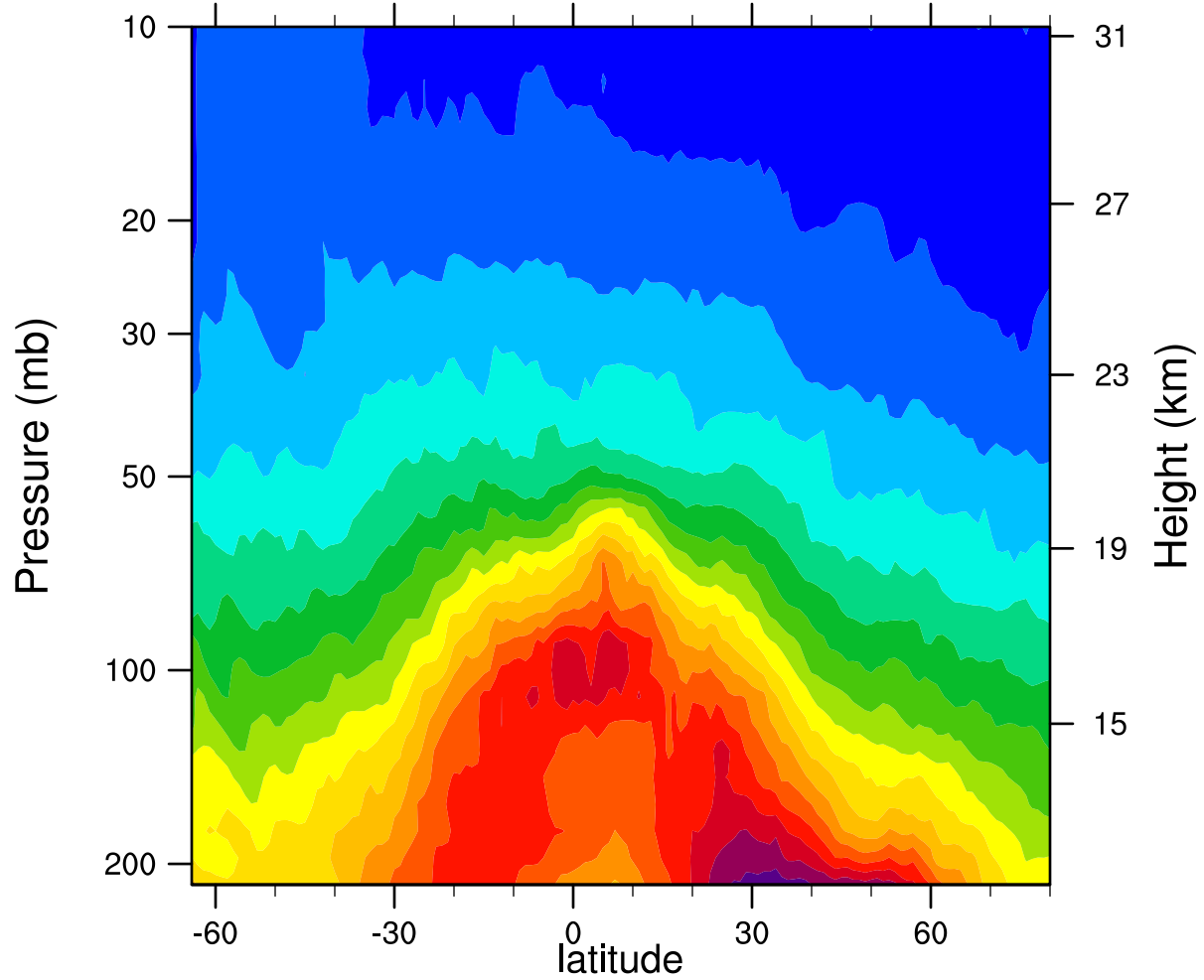
2006d160 12.1MicronExtinction_Combined (km -1 )
