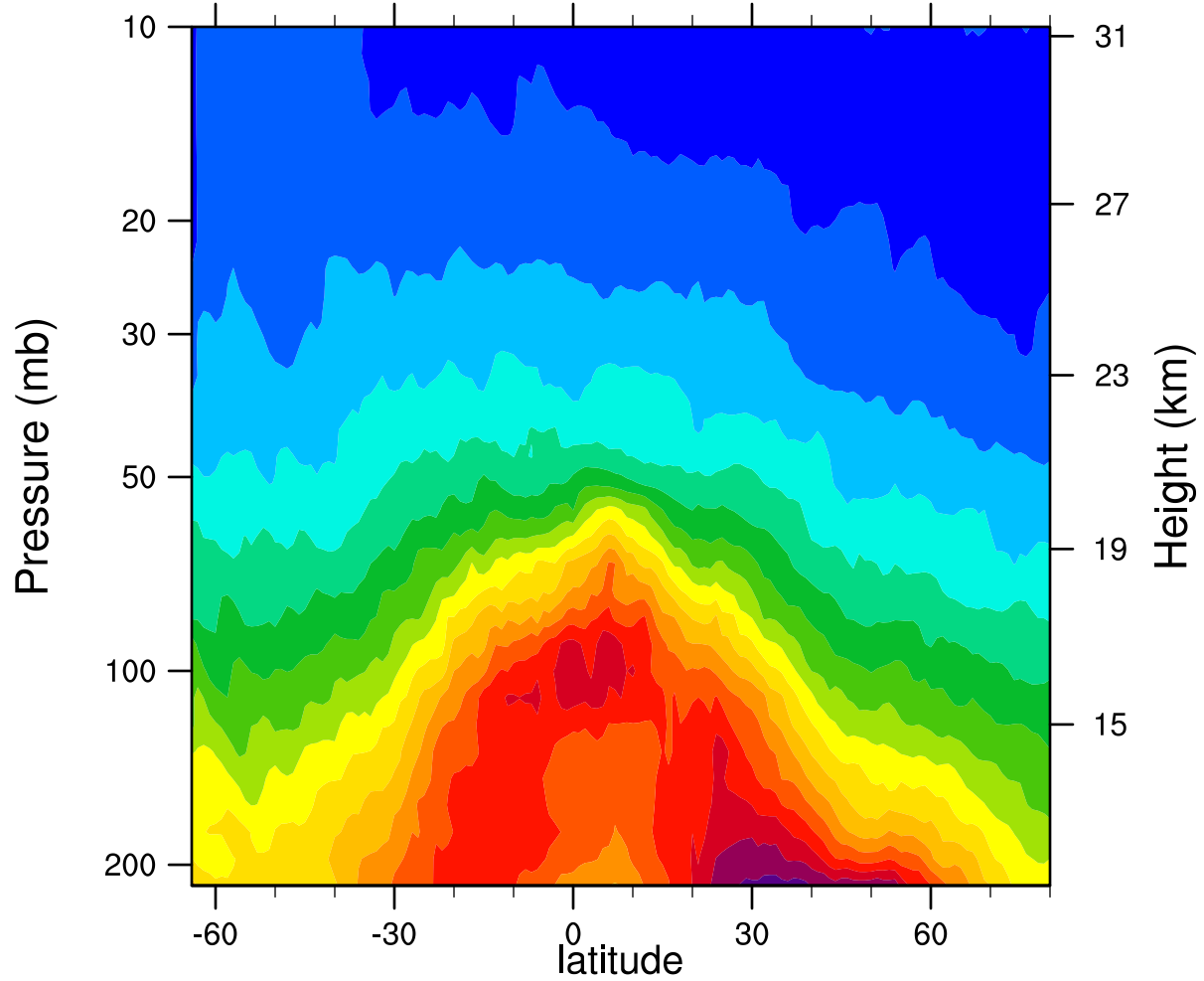
2006d161 12.1MicronExtinction_Combined (km -1 )
