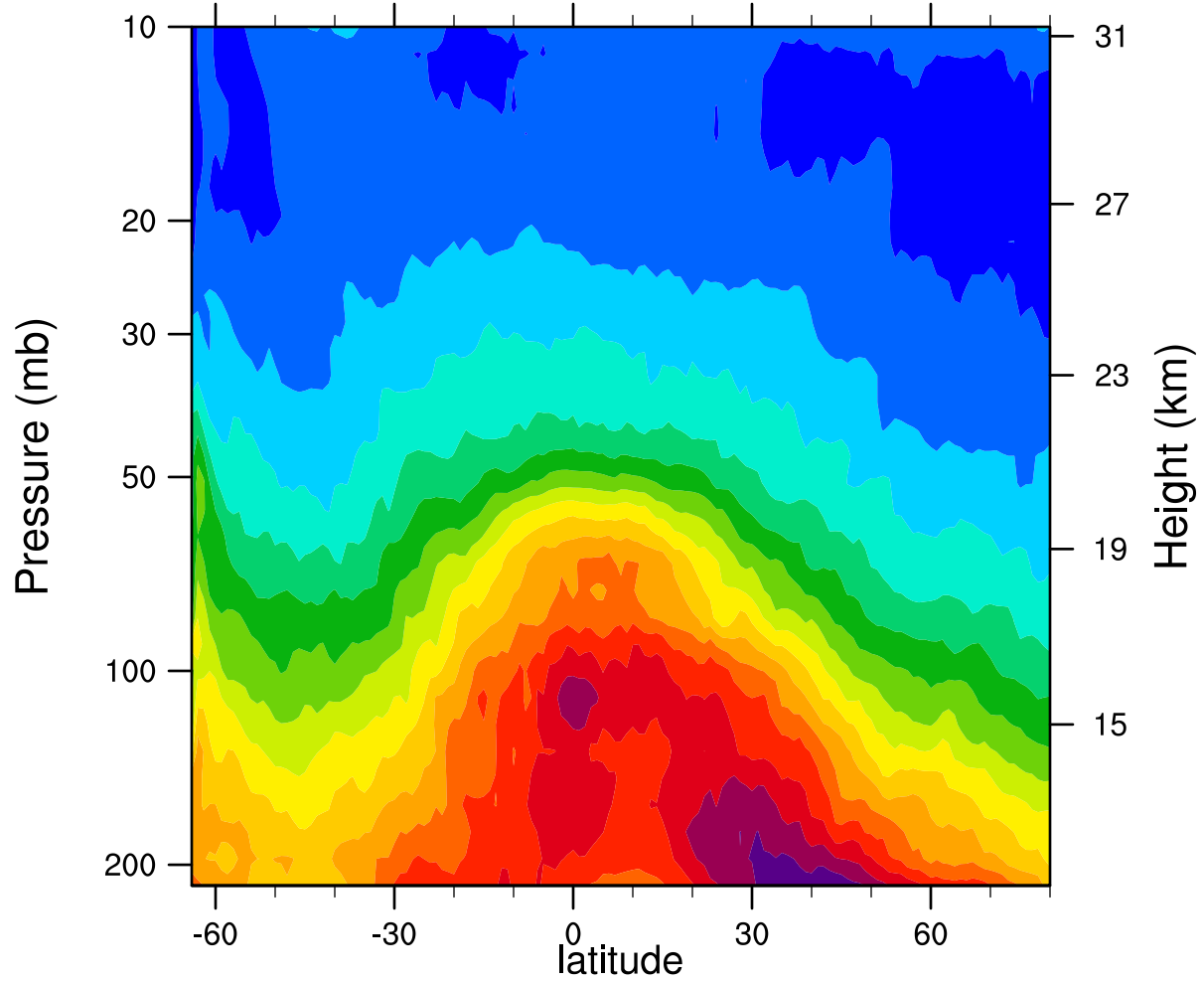
2006d228 12.1MicronExtinction_Combined (km -1 )
