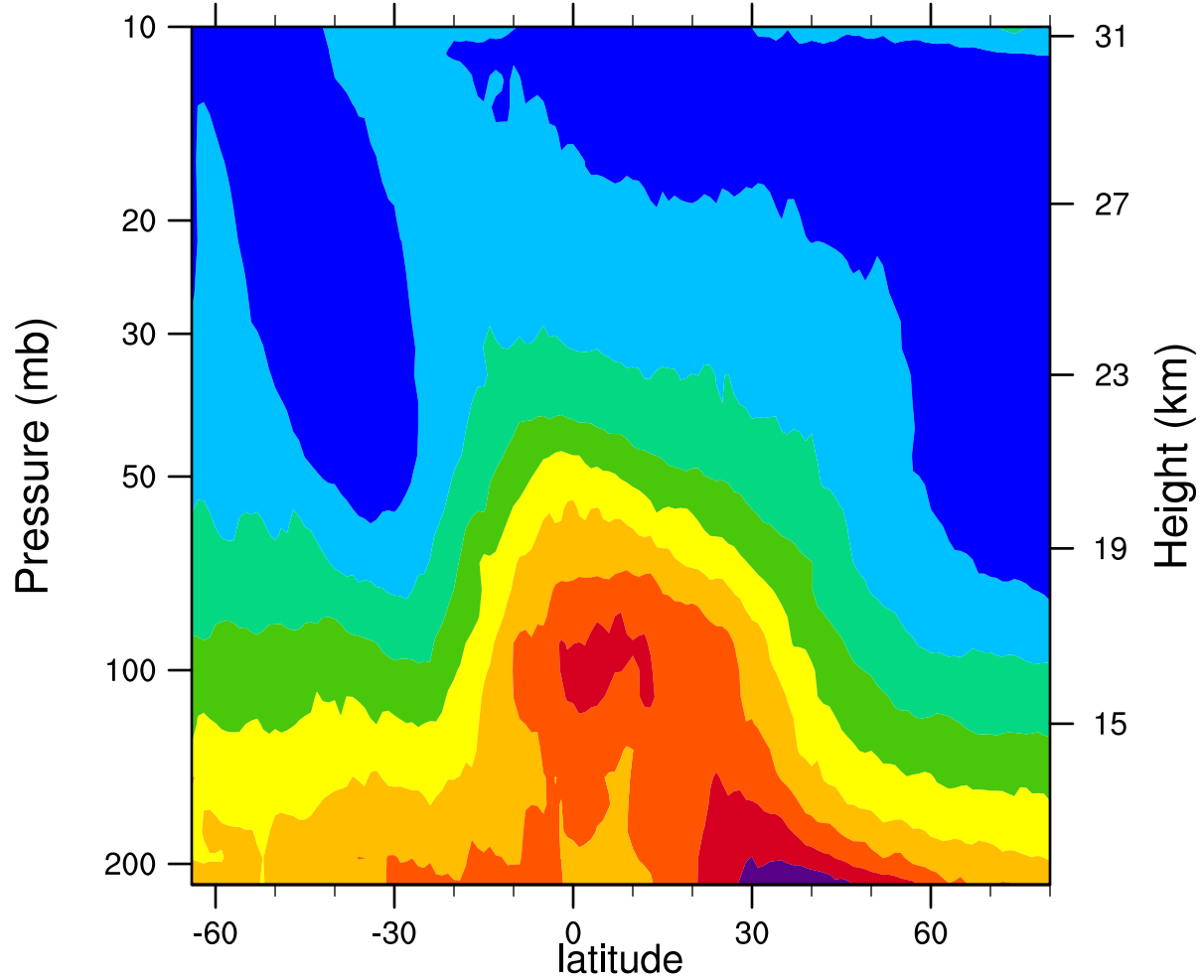
2005d166 12.1MicronExtinction_Combined (km -1 )
