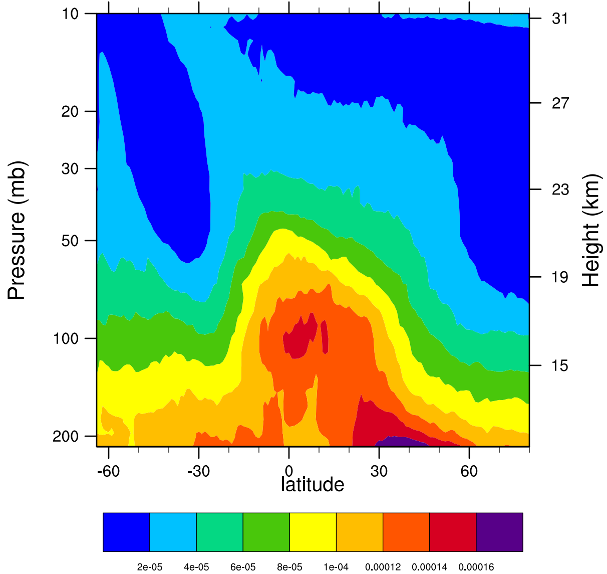
2005d167 12.1MicronExtinction_Combined (km -1 )
