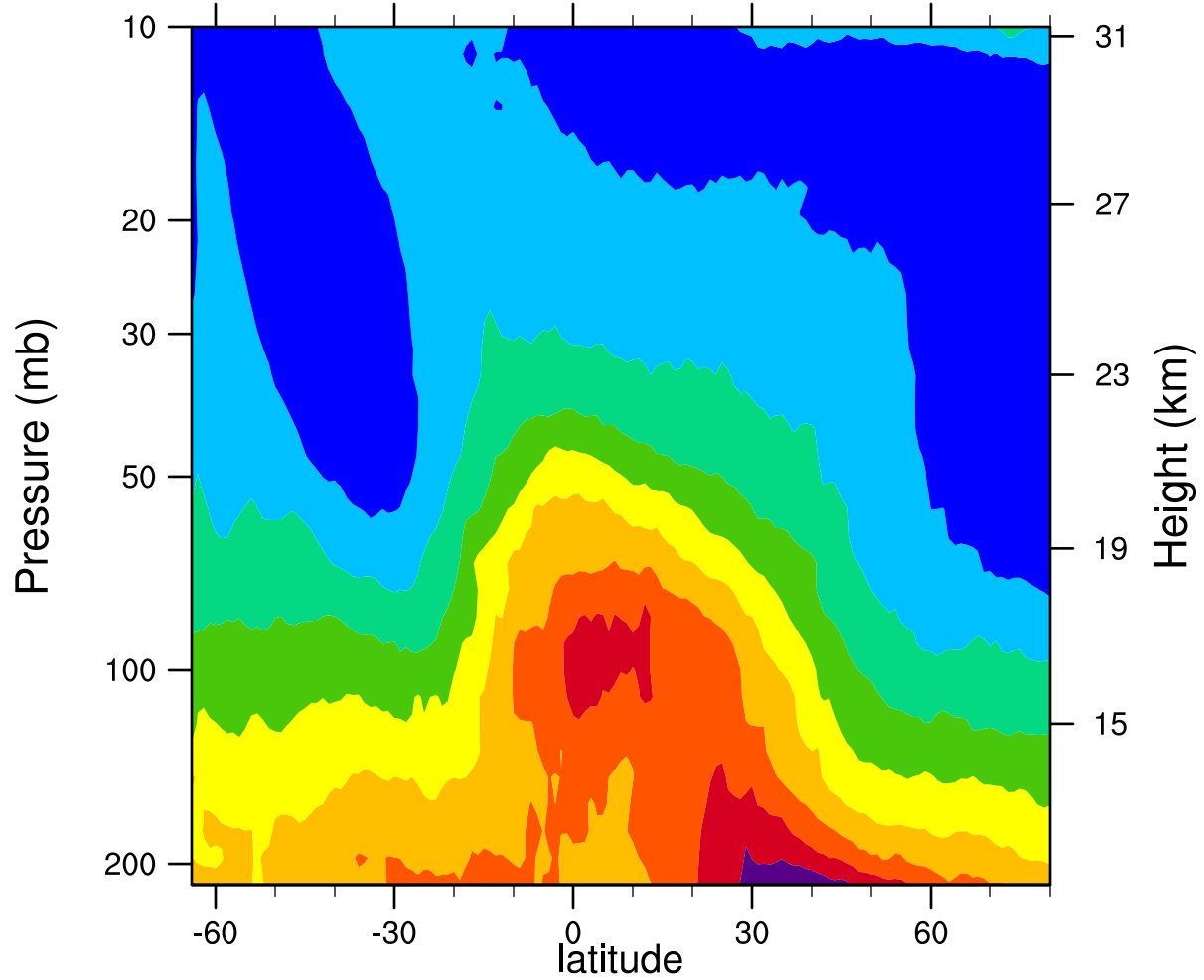
2005d164 12.1MicronExtinction_Combined (km -1 )
