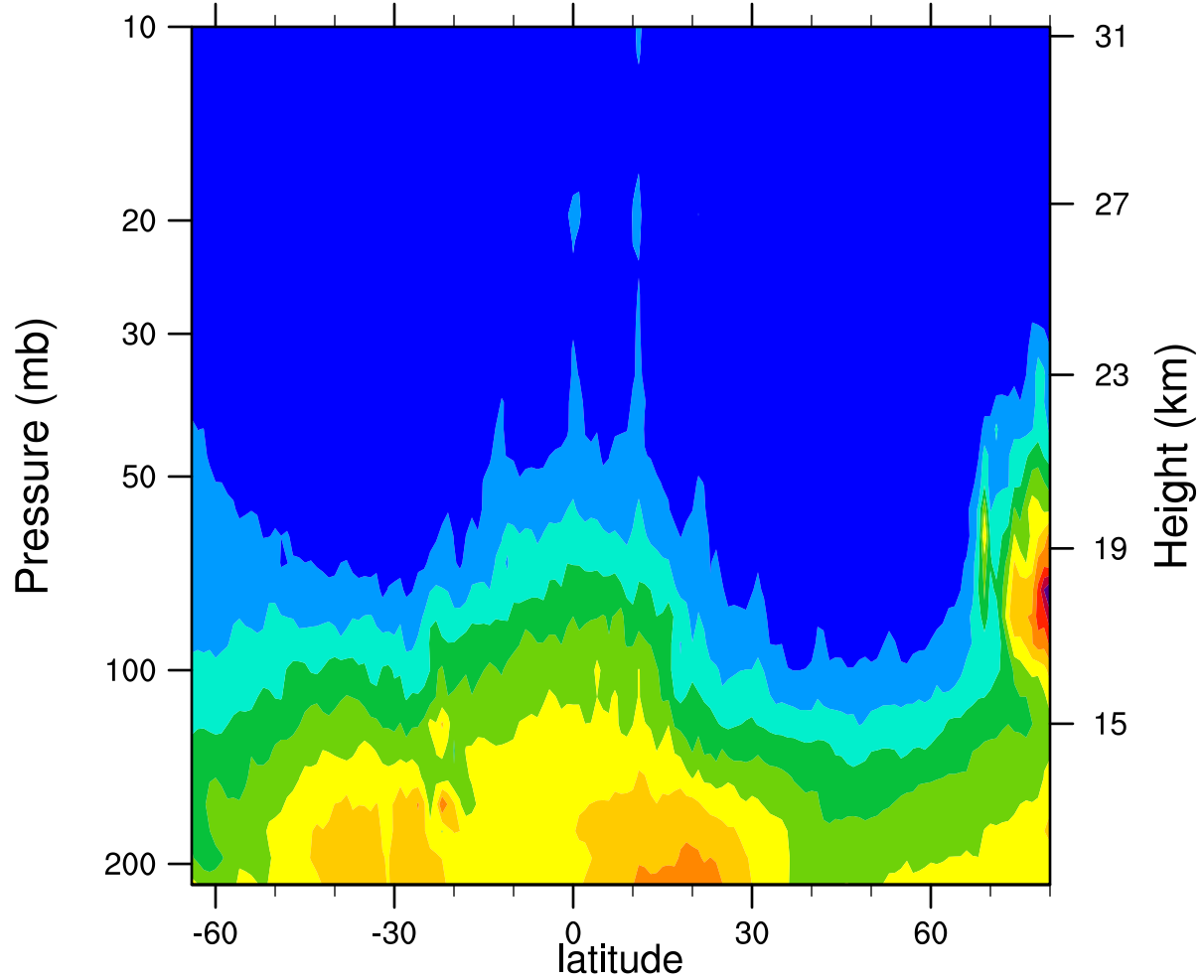
2005d025 12.1MicronExtinction_Combined (km -1 )
