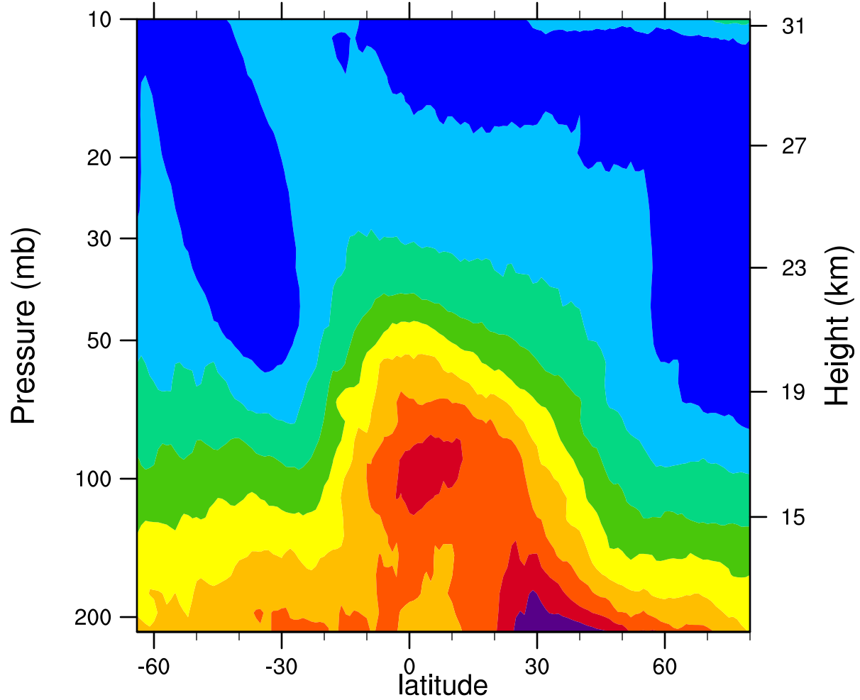
2005d161 12.1MicronExtinction_Combined (km -1 )
