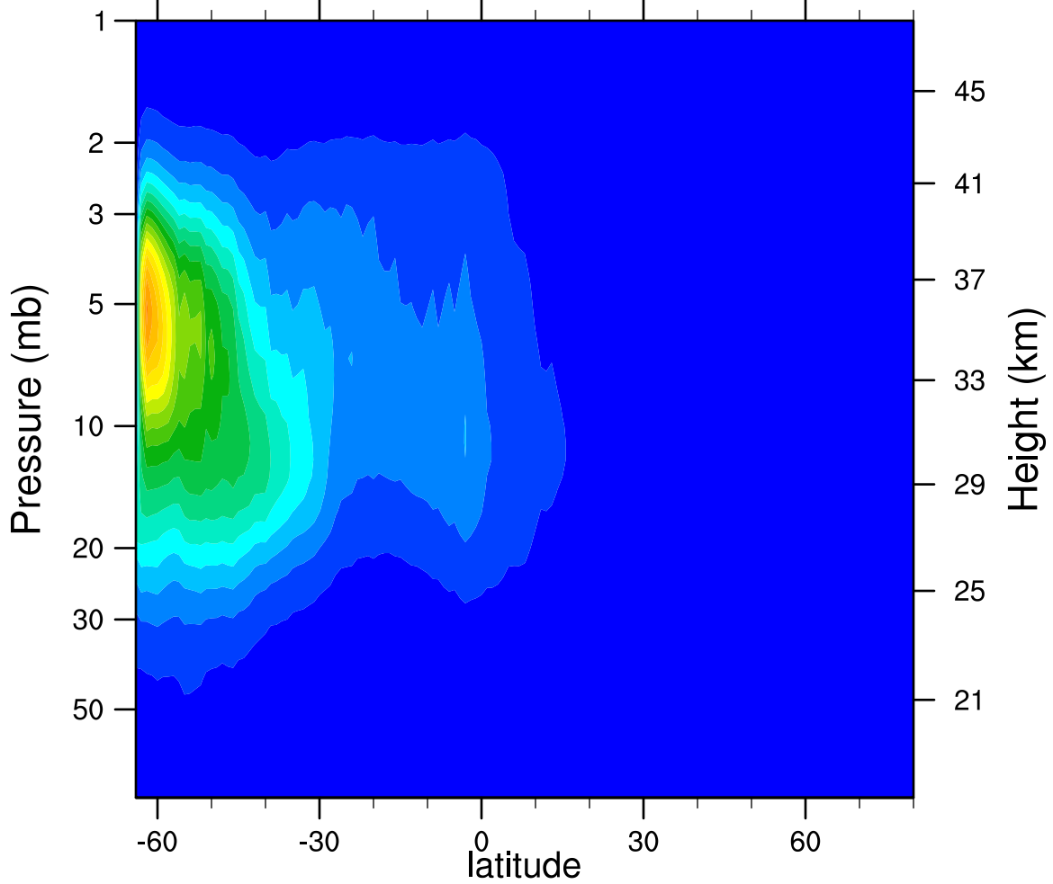
2006d156 N2O5_Ascending (ppbv)
