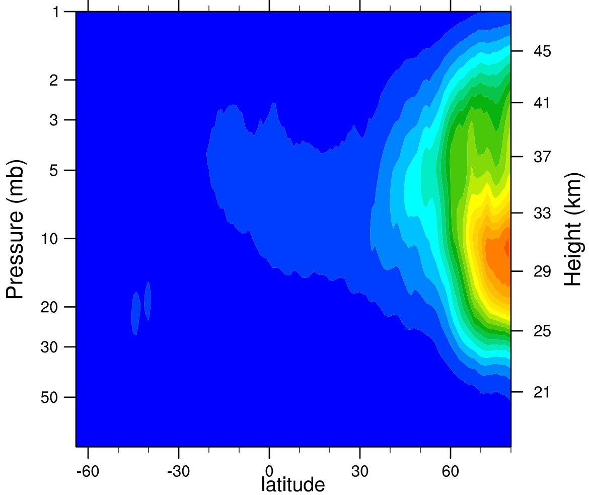
2005d313 N2O5_Ascending (ppbv)
