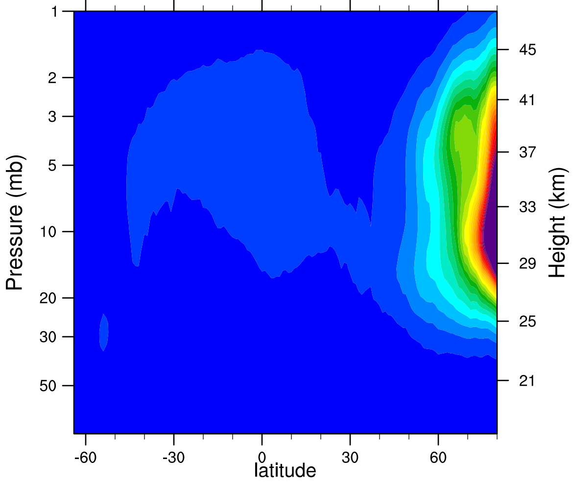
2006d042 N2O5_Ascending (ppbv)
