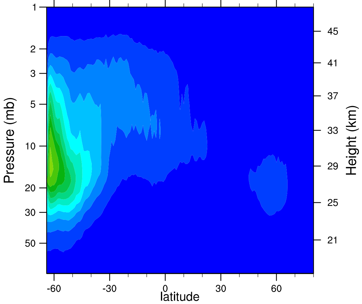
2006d112 N2O5_Ascending (ppbv)
