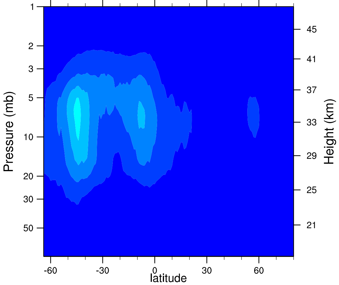
2006d211 N2O5_Ascending (ppbv)
