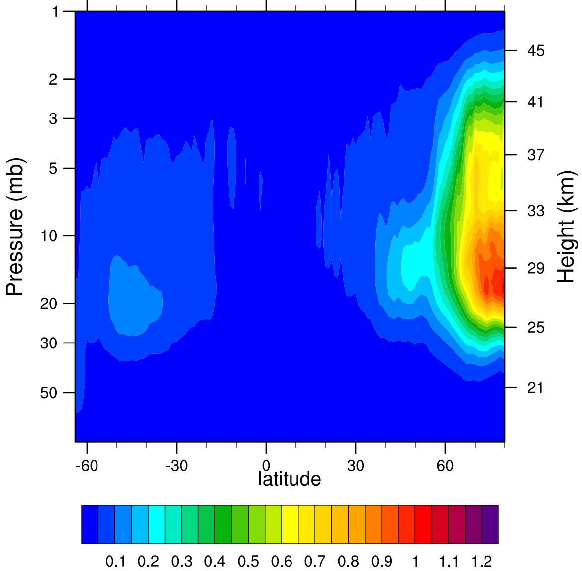
2006d315 N2O5_Ascending (ppbv)
