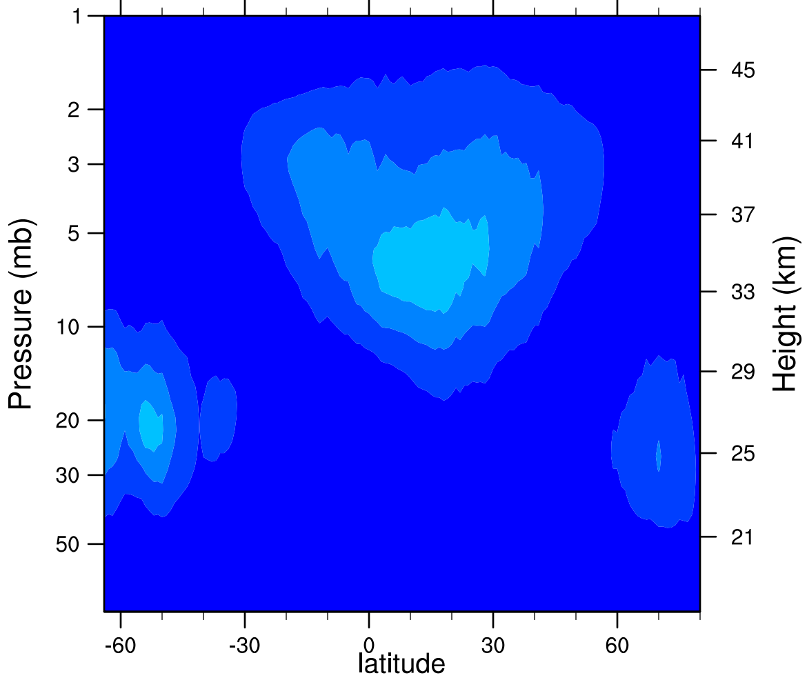
2005d256 N2O5_Ascending (ppbv)
