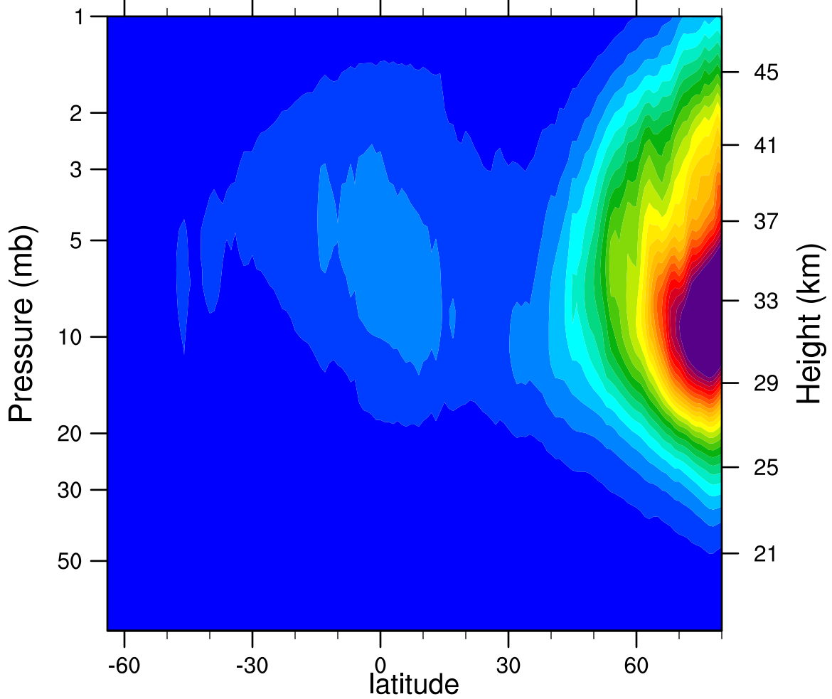
2006d009 N2O5_Ascending (ppbv)
