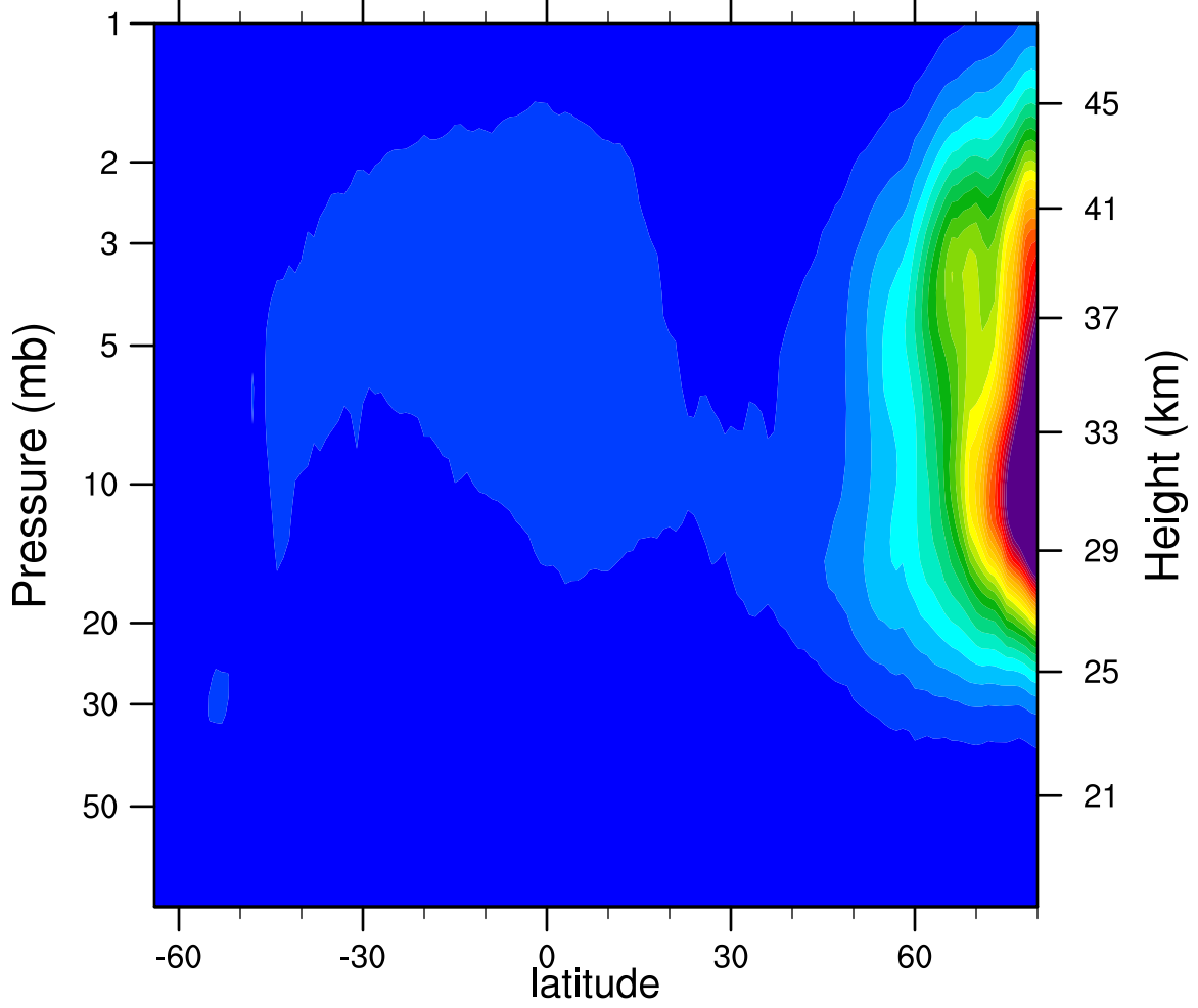
2006d041 N2O5_Ascending (ppbv)
