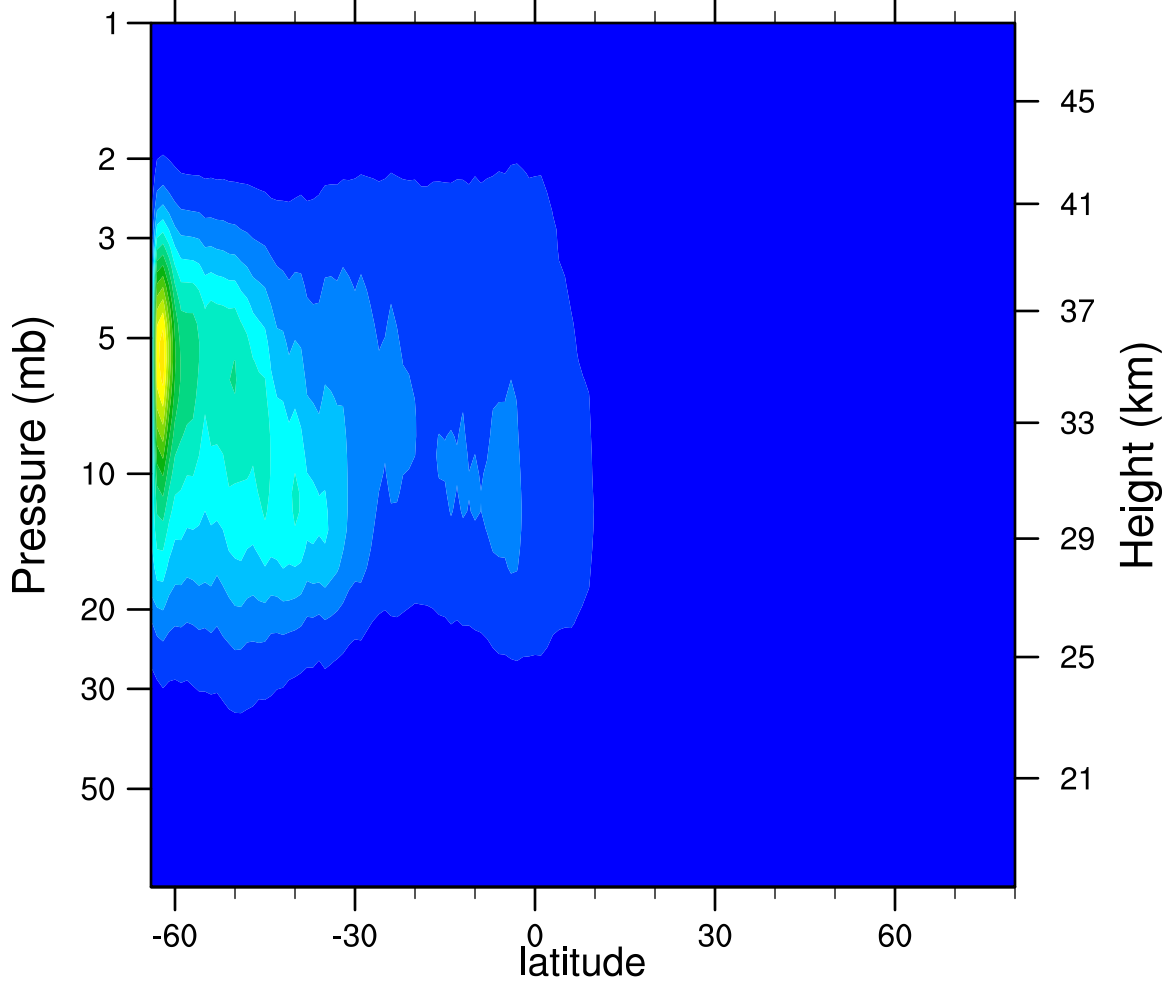
2006d174 N2O5_Ascending (ppbv)
