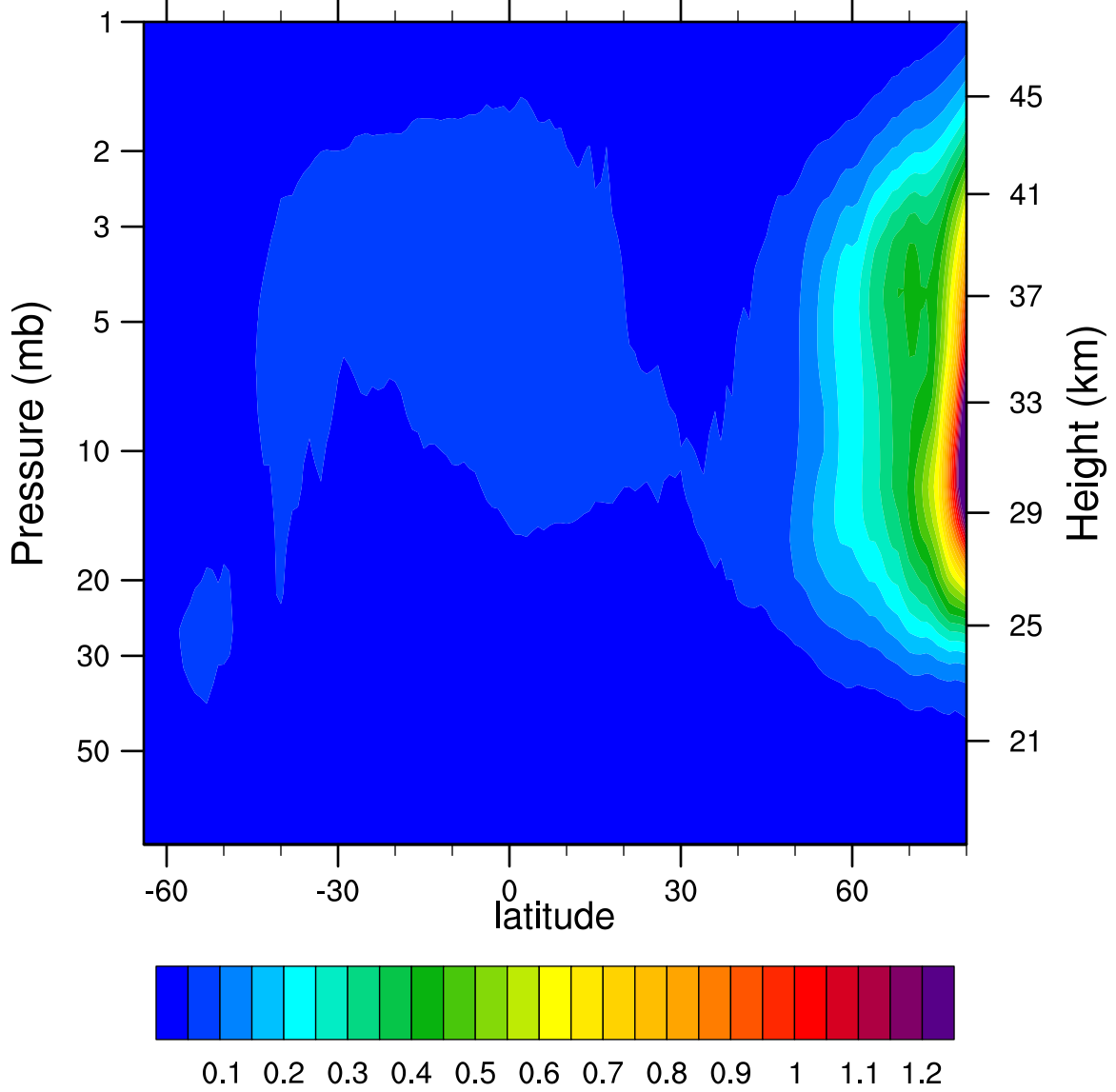
2006d047 N2O5_Ascending (ppbv)
