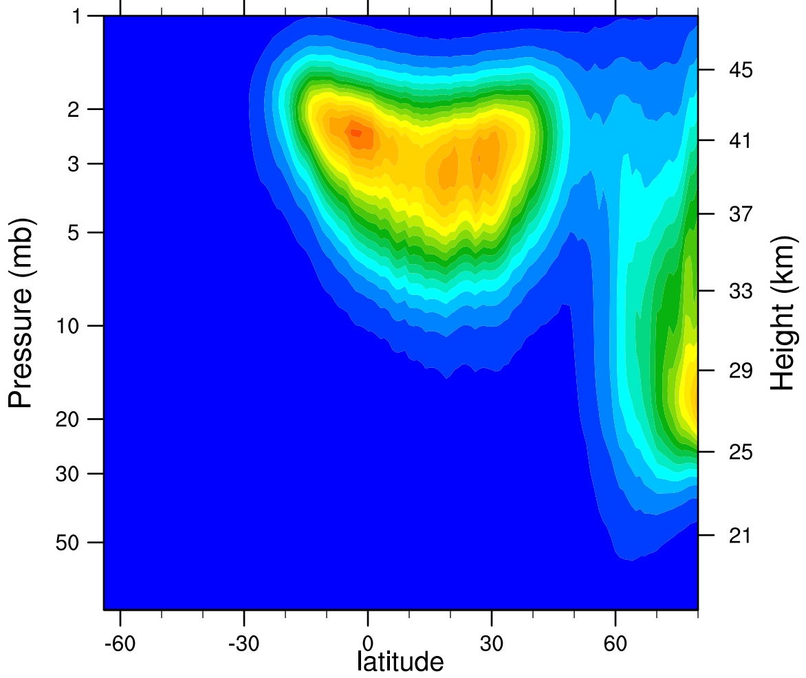
2005d037 N2O5_Ascending (ppbv)
