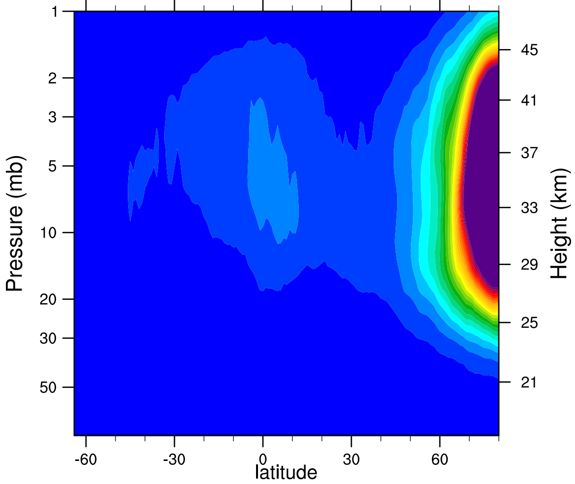
2006d028 N2O5_Ascending (ppbv)
