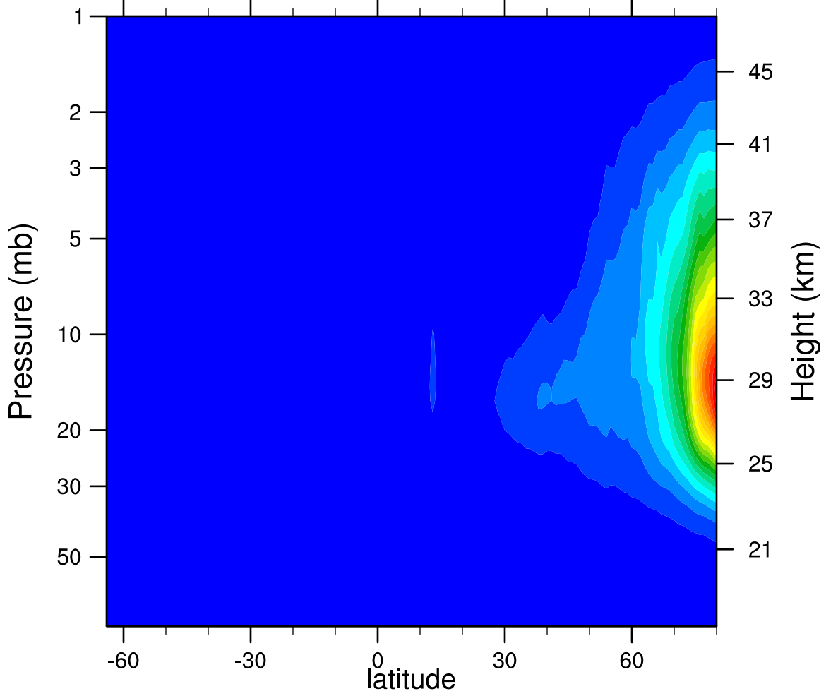
2006d293 N2O5_Ascending (ppbv)
