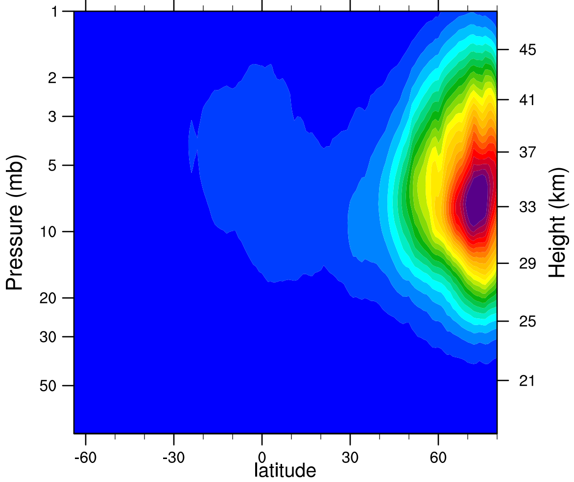
2005d349 N2O5_Ascending (ppbv)
