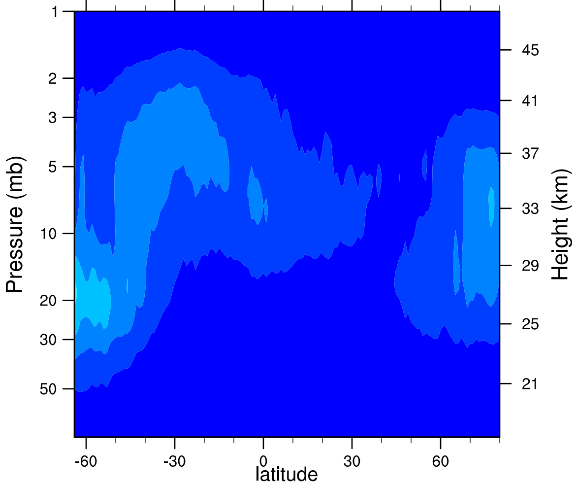
2006d086 N2O5_Ascending (ppbv)
