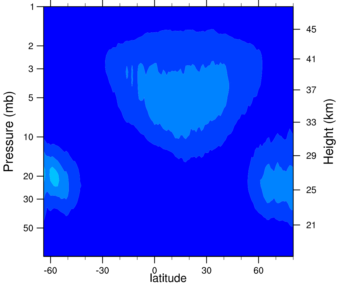
2005d270 N2O5_Ascending (ppbv)
