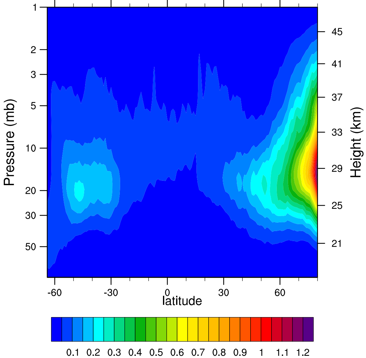
2007d290 N2O5_Ascending (ppbv)
