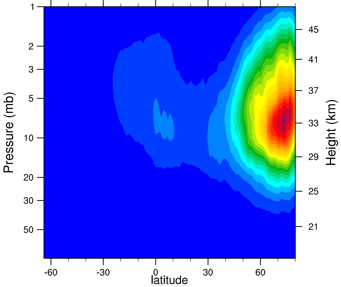
2005d360 N2O5_Ascending (ppbv)
