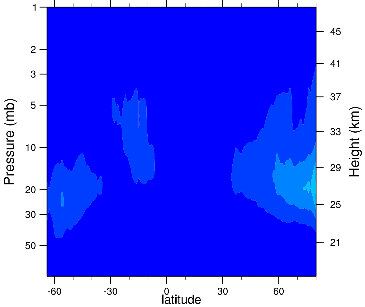
2006d273 N2O5_Ascending (ppbv)
