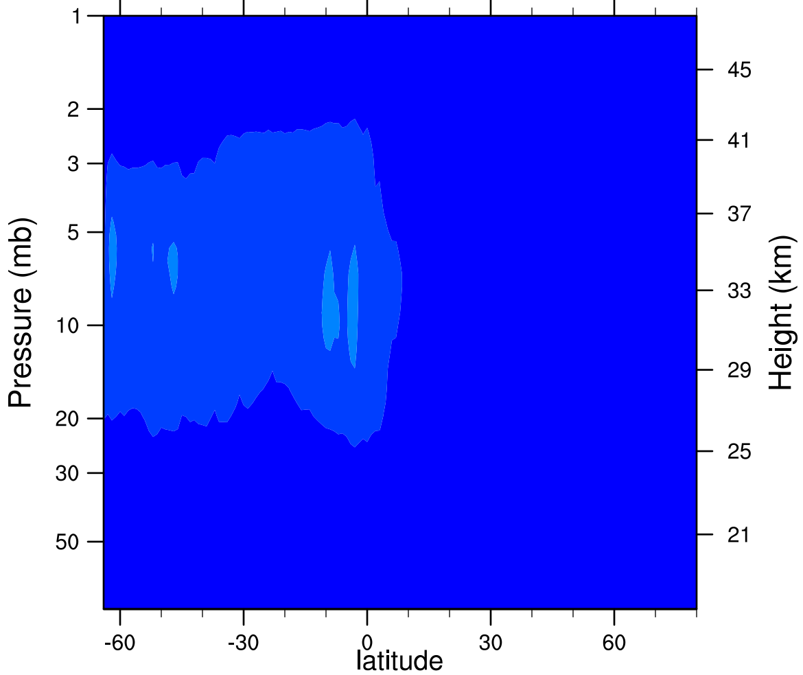
2006d181 N2O5_Ascending (ppbv)
