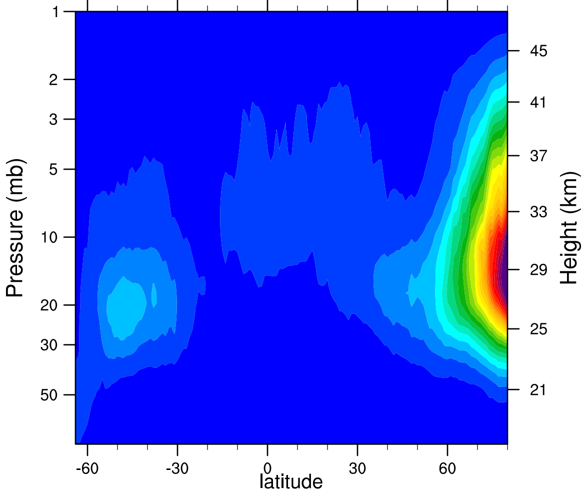
2007d298 N2O5_Ascending (ppbv)
