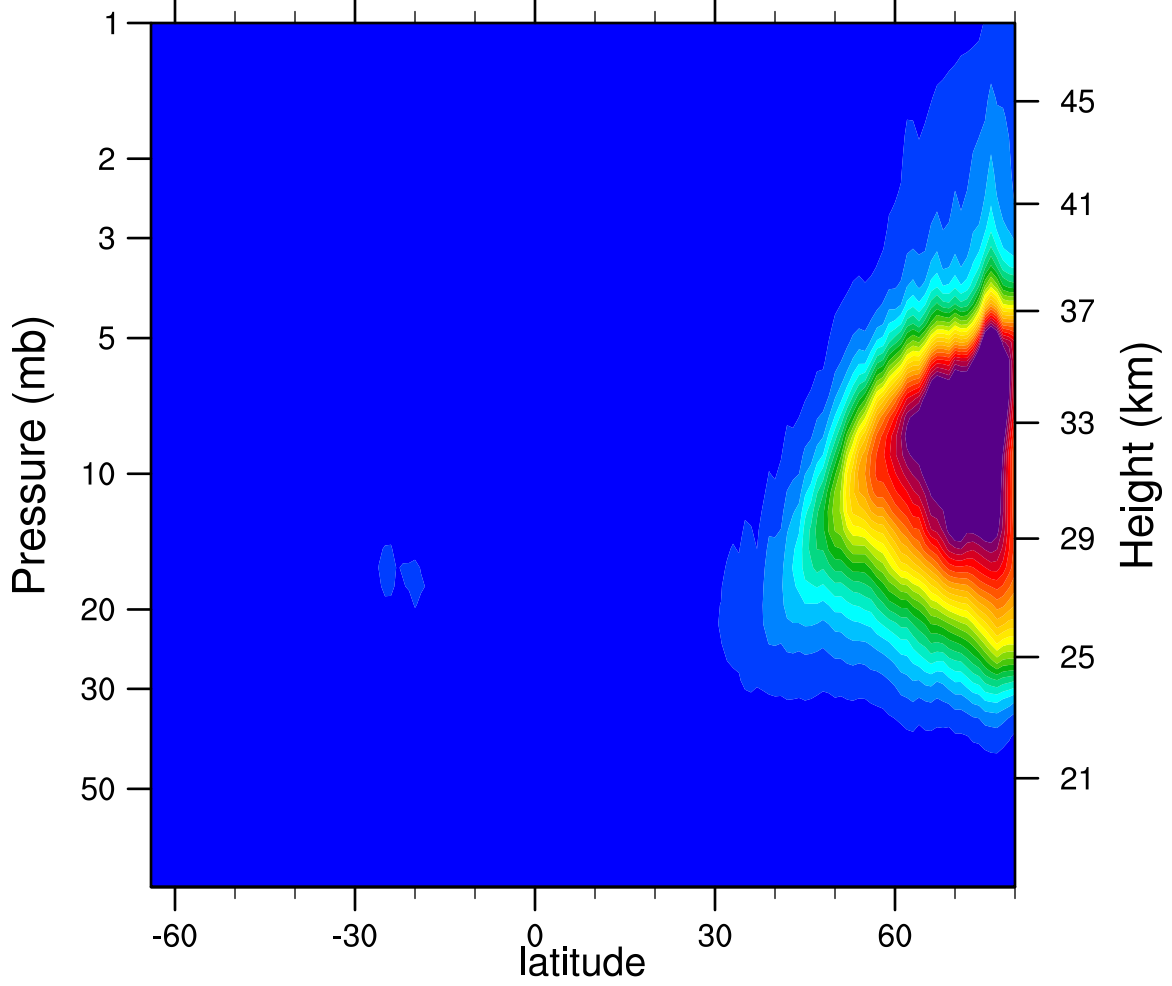
2006d360 N2O5_Ascending (ppbv)
