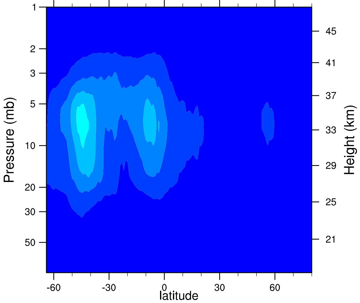
2006d209 N2O5_Ascending (ppbv)
