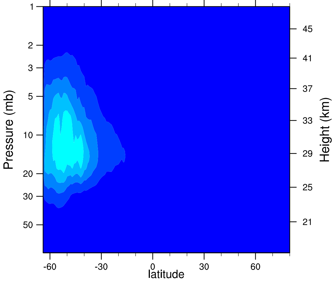
2007d200 N2O5_Ascending (ppbv)
