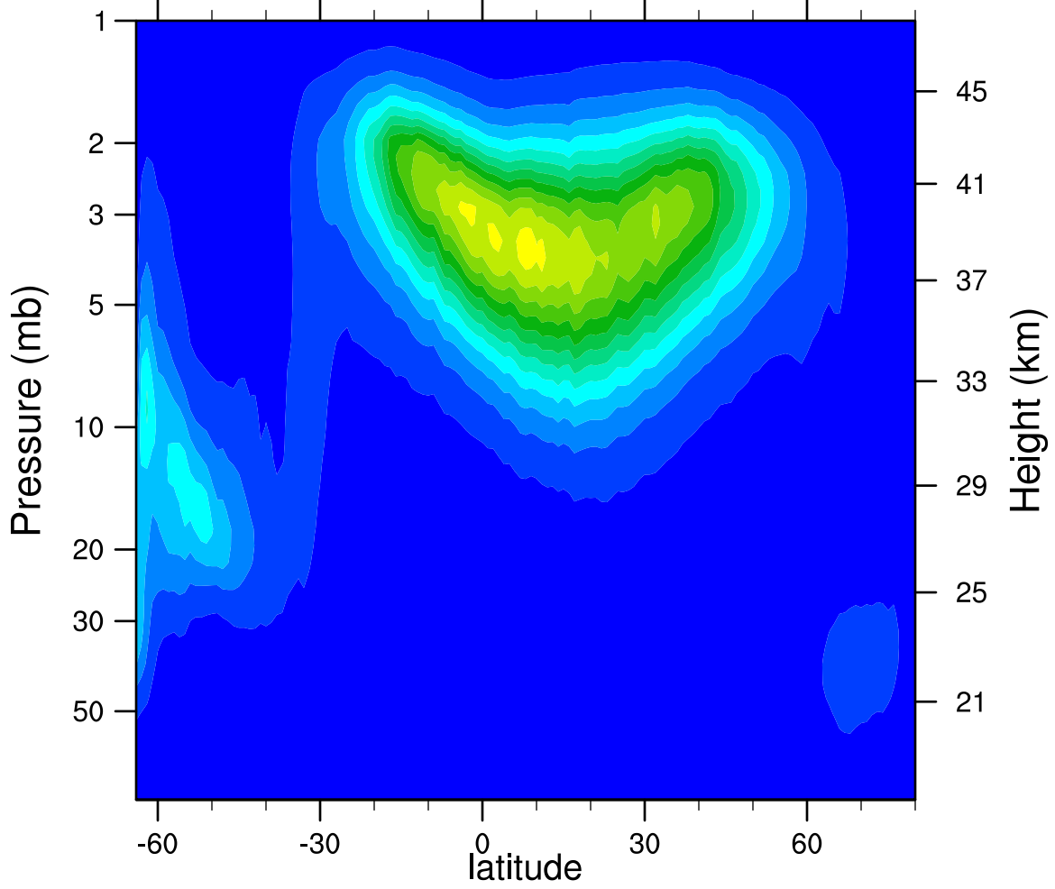
2005d098 N2O5_Ascending (ppbv)
