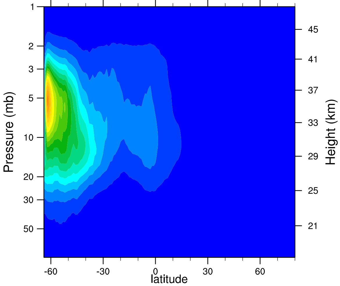
2006d149 N2O5_Ascending (ppbv)
