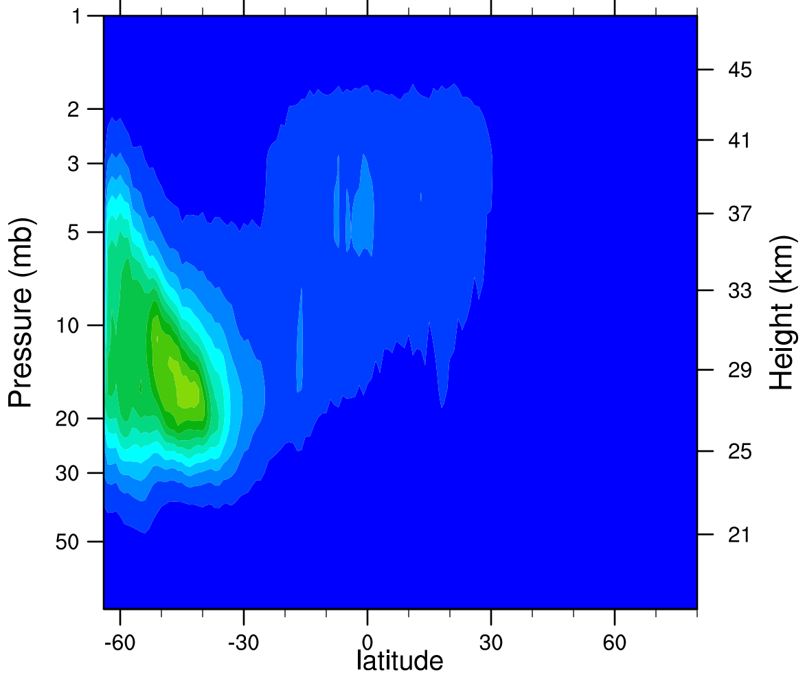
2007d214 N2O5_Ascending (ppbv)
