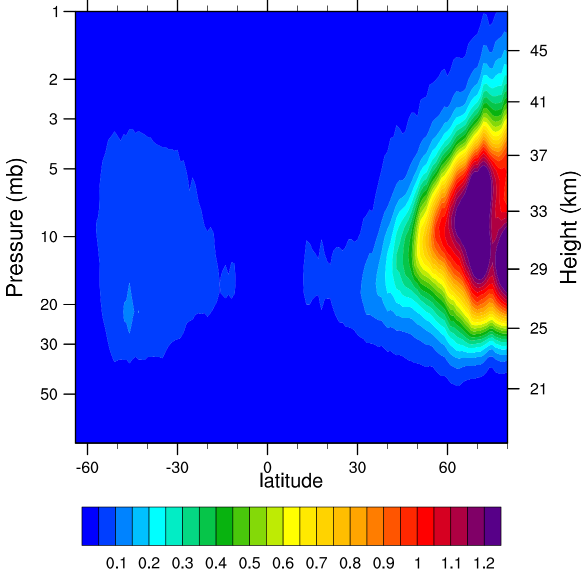
2006d353 N2O5_Ascending (ppbv)
