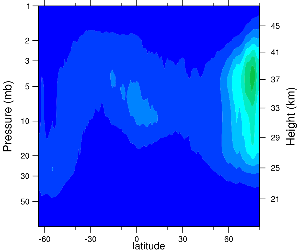
2006d066 N2O5_Ascending (ppbv)
