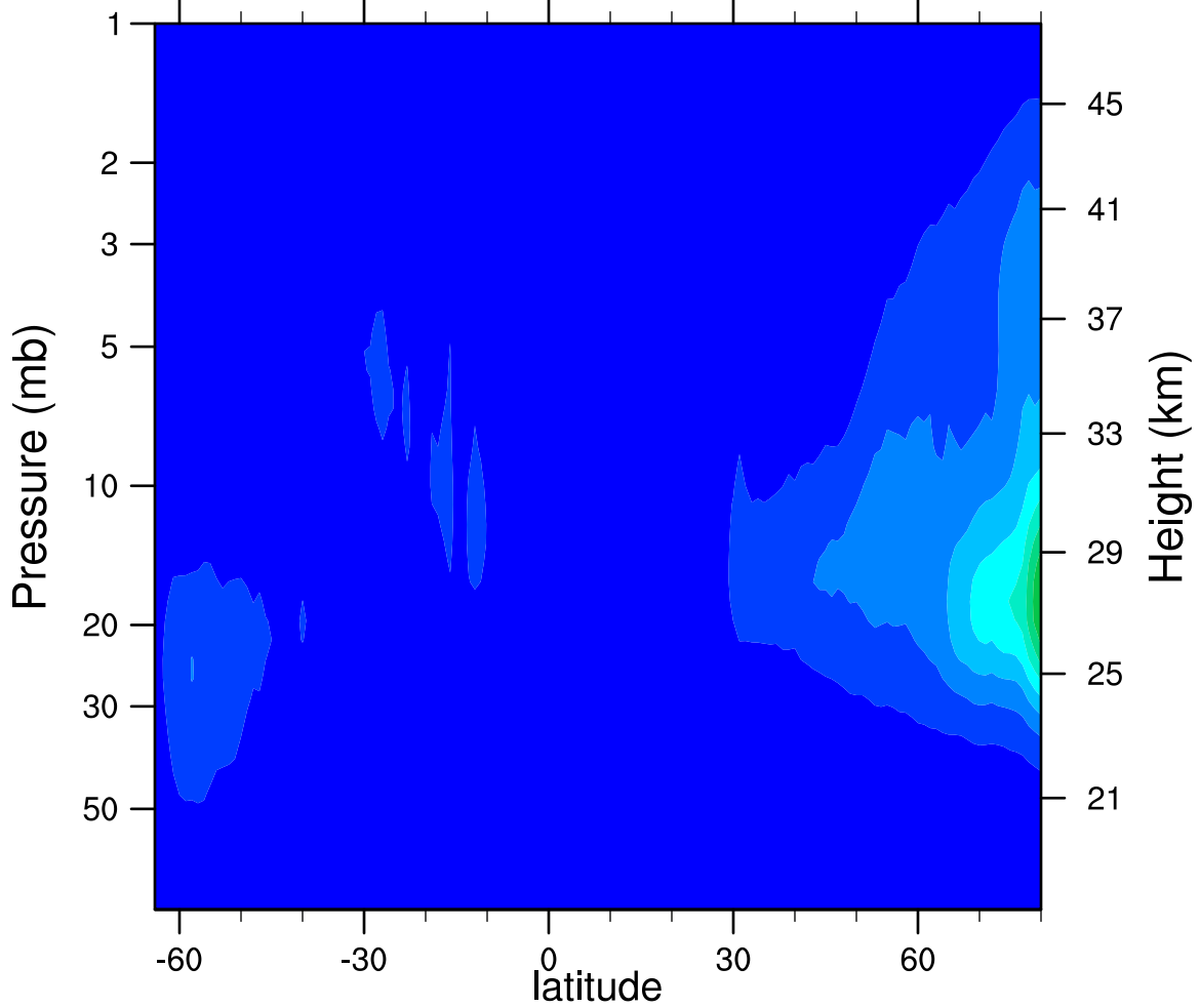
2006d283 N2O5_Ascending (ppbv)
