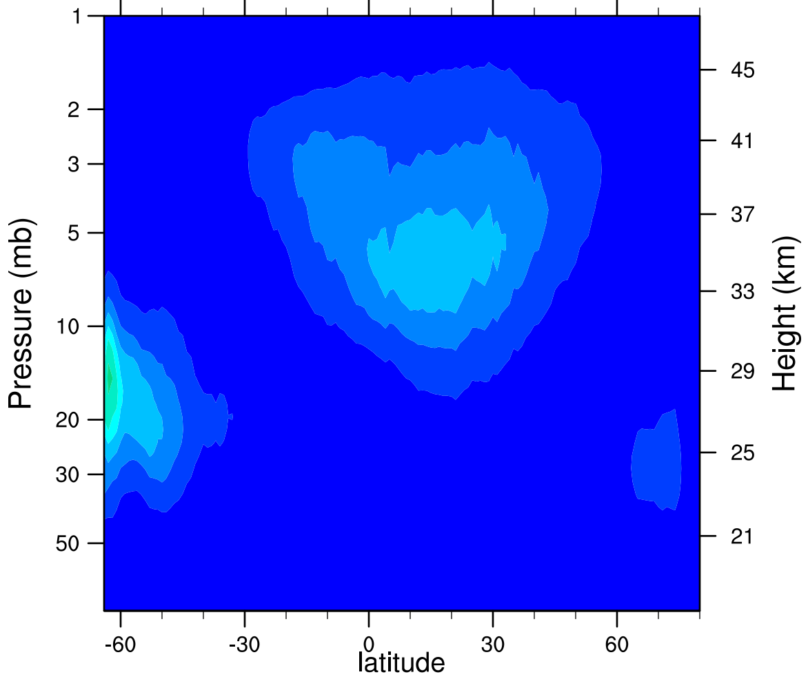
2005d250 N2O5_Ascending (ppbv)
