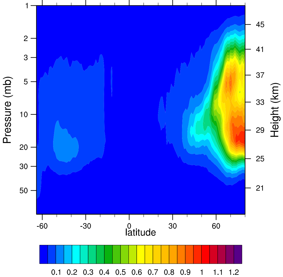
2006d314 N2O5_Ascending (ppbv)
