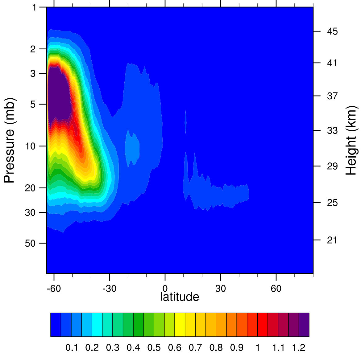
2007d160 N2O5_Ascending (ppbv)
