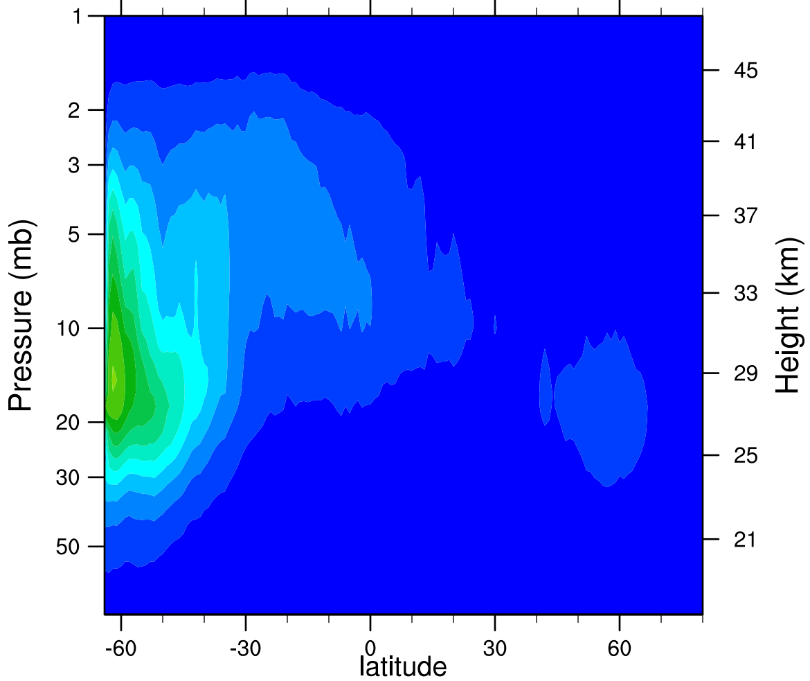
2006d110 N2O5_Ascending (ppbv)
