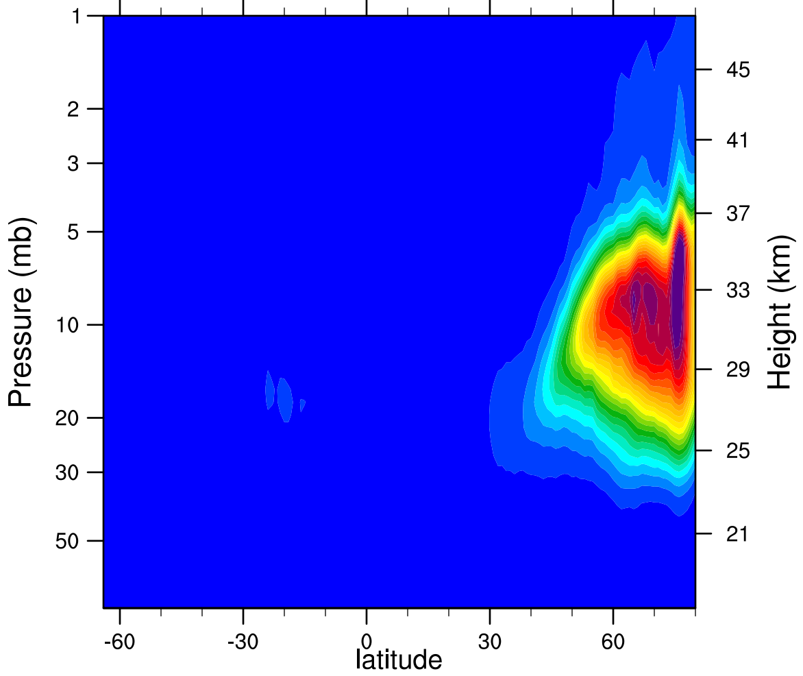
2006d362 N2O5_Ascending (ppbv)
