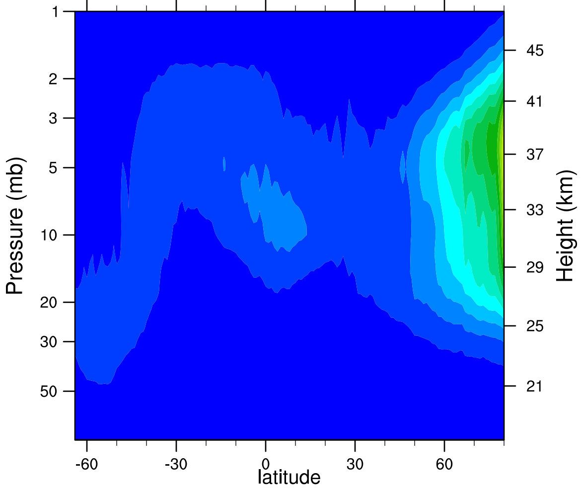
2006d060 N2O5_Ascending (ppbv)
