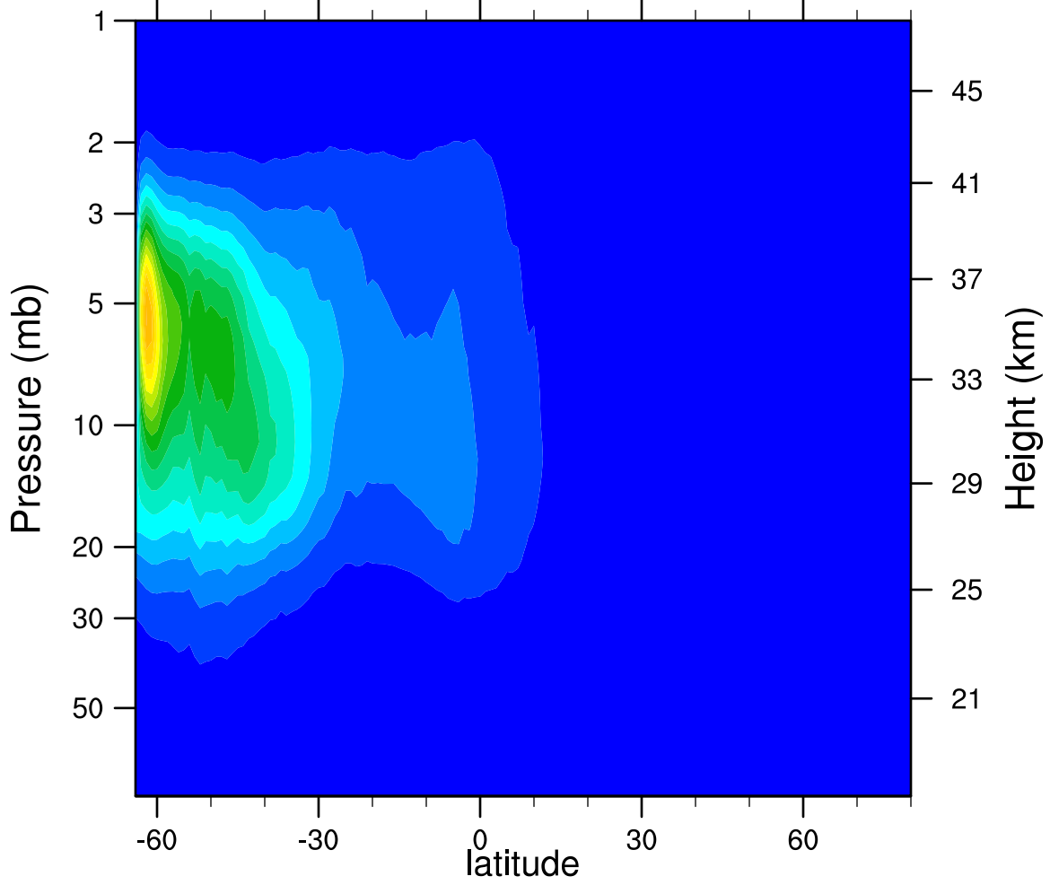
2006d170 N2O5_Ascending (ppbv)
