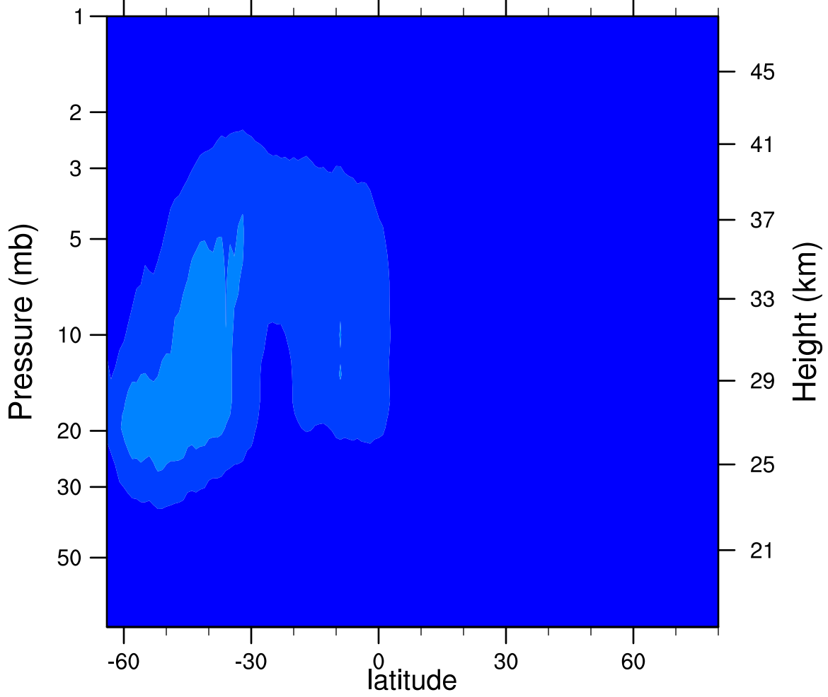
2006d231 N2O5_Ascending (ppbv)
