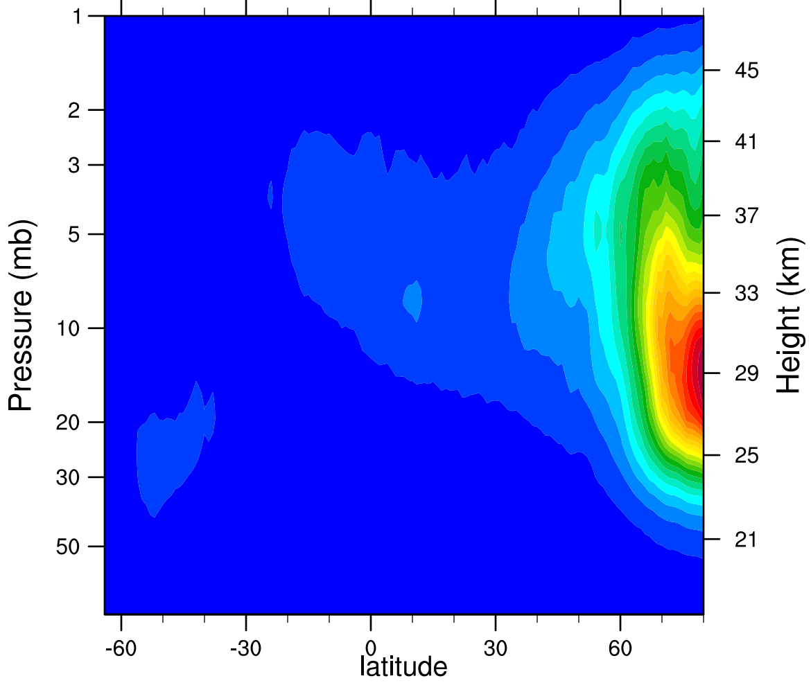
2005d305 N2O5_Ascending (ppbv)
