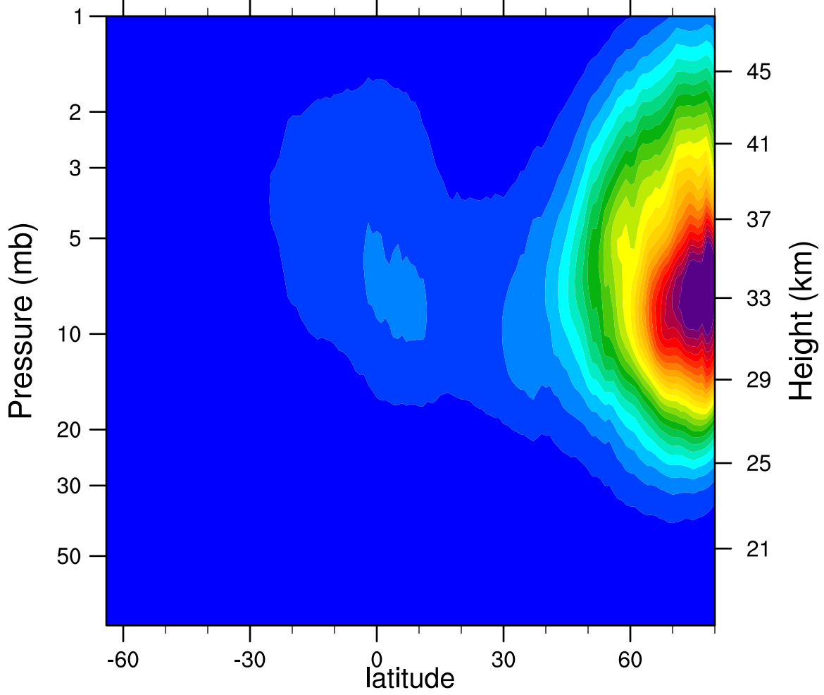
2005d363 N2O5_Ascending (ppbv)
