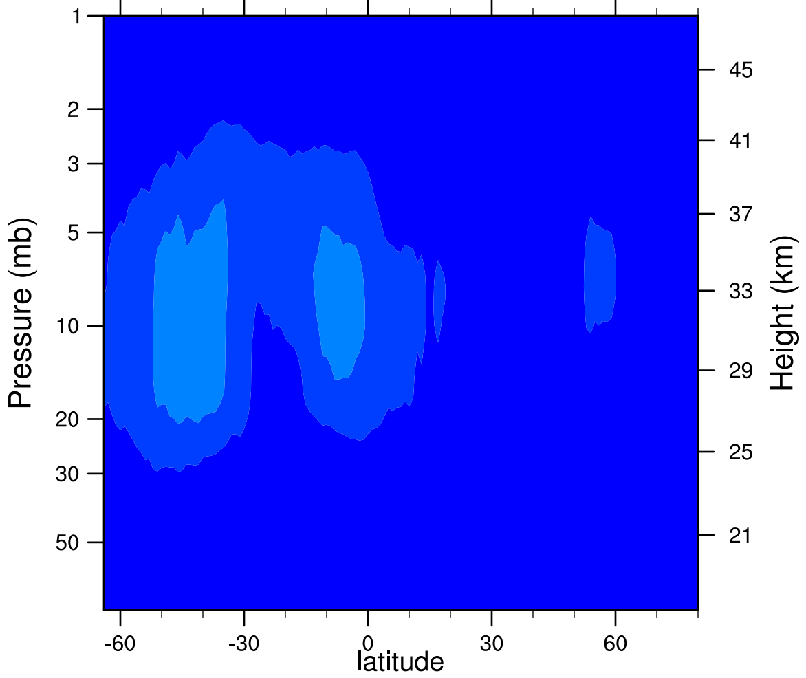
2006d217 N2O5_Ascending (ppbv)
