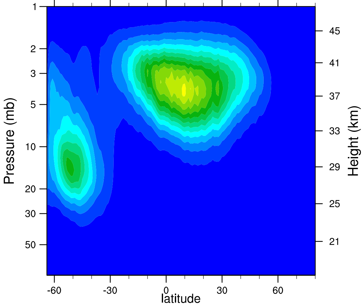
2005d150 N2O5_Ascending (ppbv)
