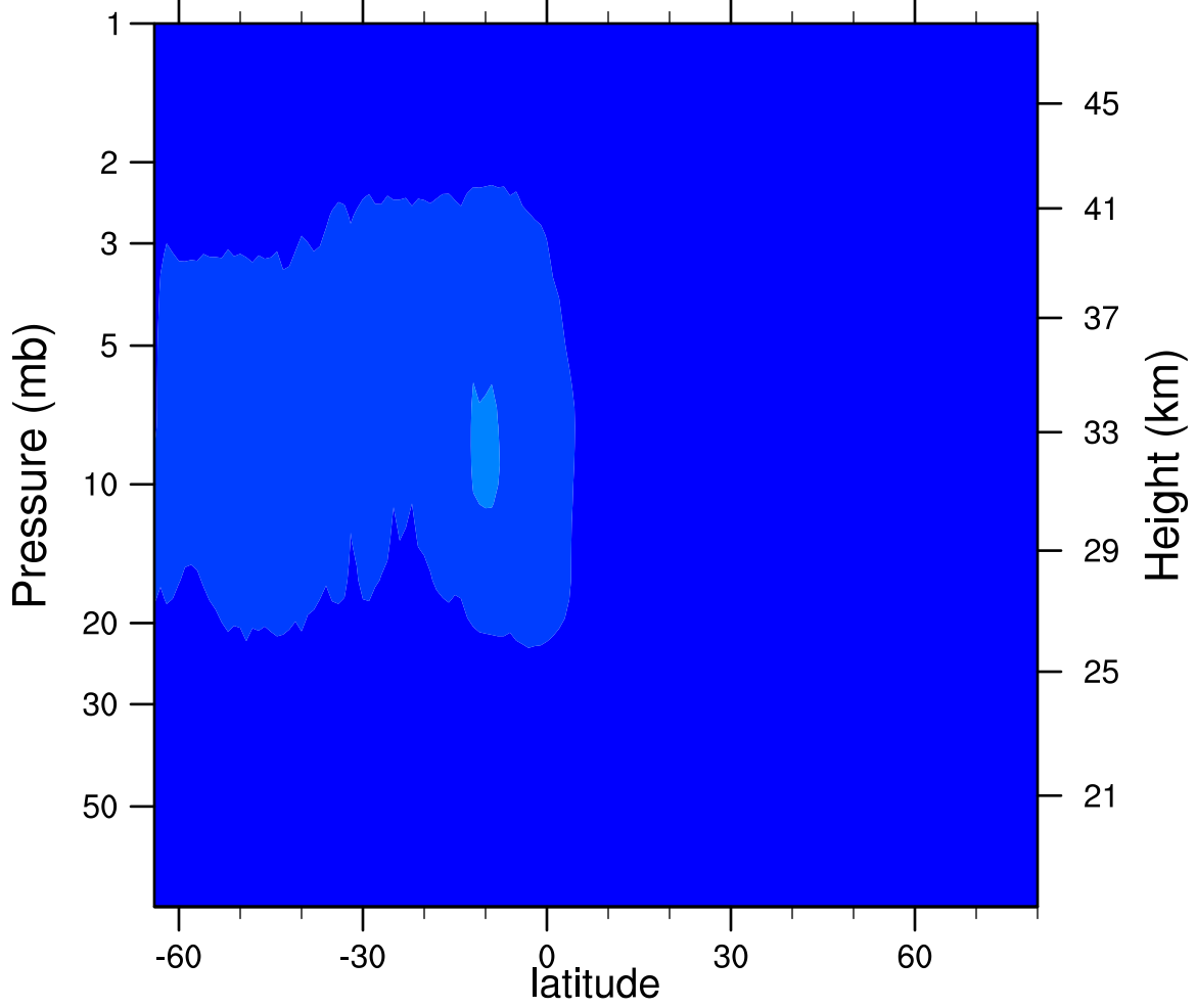
2006d184 N2O5_Ascending (ppbv)
