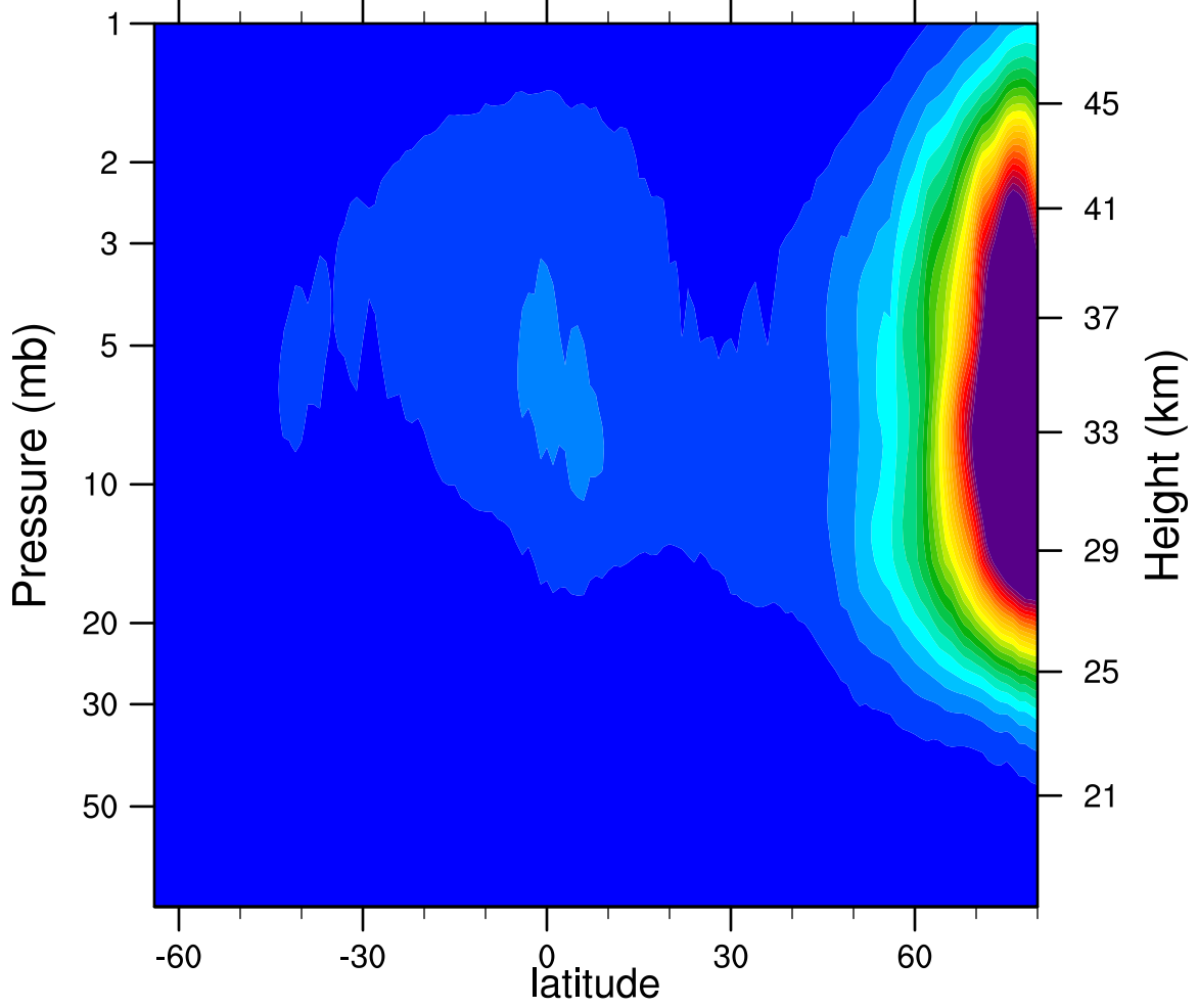
2006d031 N2O5_Ascending (ppbv)
