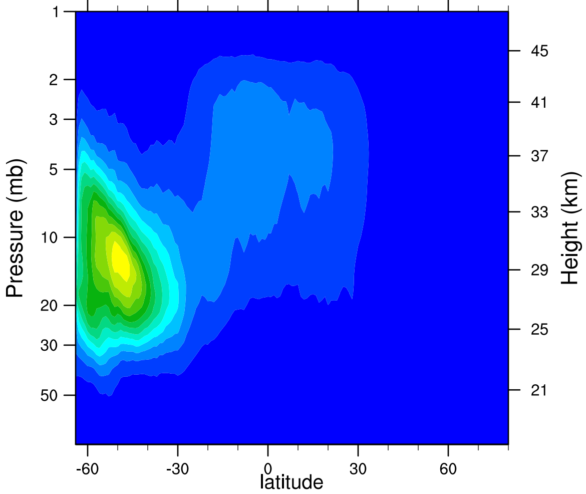
2007d223 N2O5_Ascending (ppbv)
