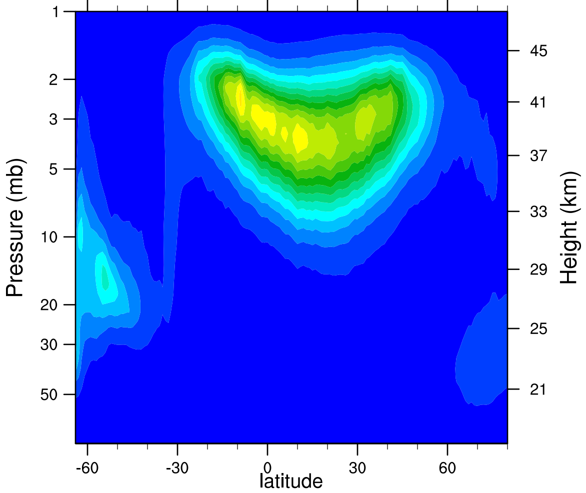
2005d092 N2O5_Ascending (ppbv)
