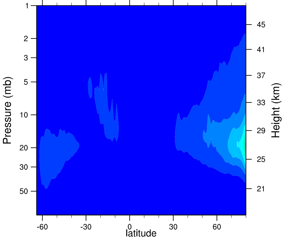
2006d277 N2O5_Ascending (ppbv)
