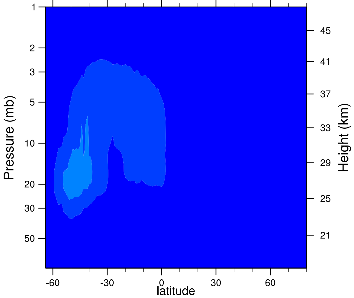
2006d238 N2O5_Ascending (ppbv)
