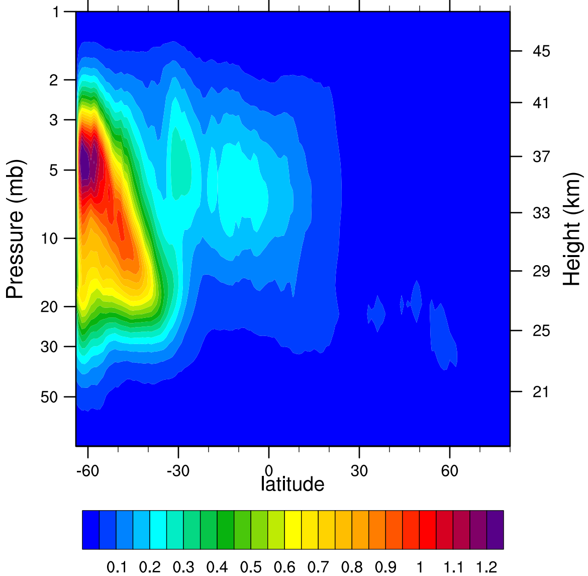
2007d137 N2O5_Ascending (ppbv)
