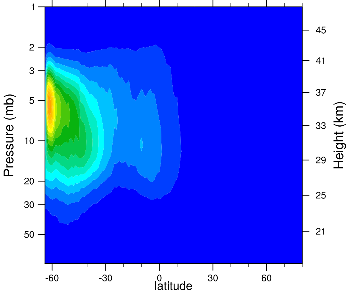
2006d167 N2O5_Ascending (ppbv)
