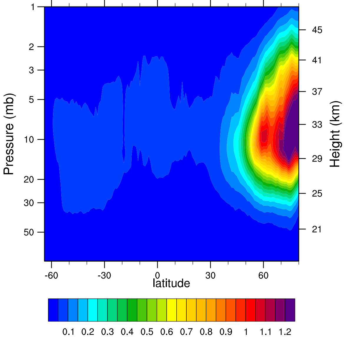
2007d358 N2O5_Ascending (ppbv)
