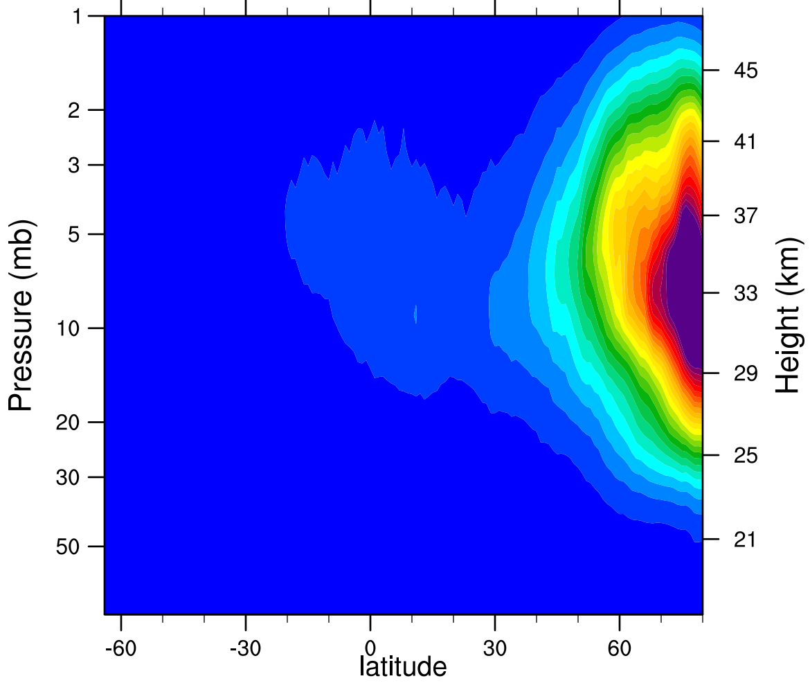
2005d331 N2O5_Ascending (ppbv)
