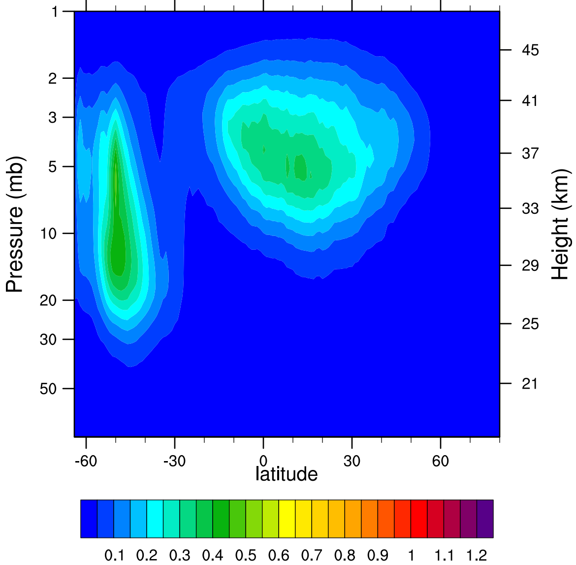
2005d183 N2O5_Ascending (ppbv)
