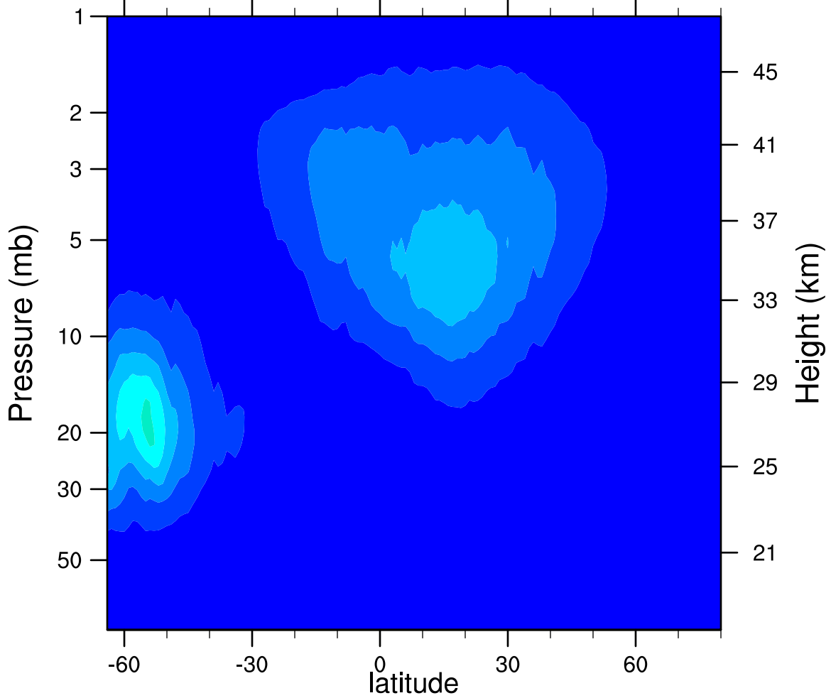
2005d242 N2O5_Ascending (ppbv)
