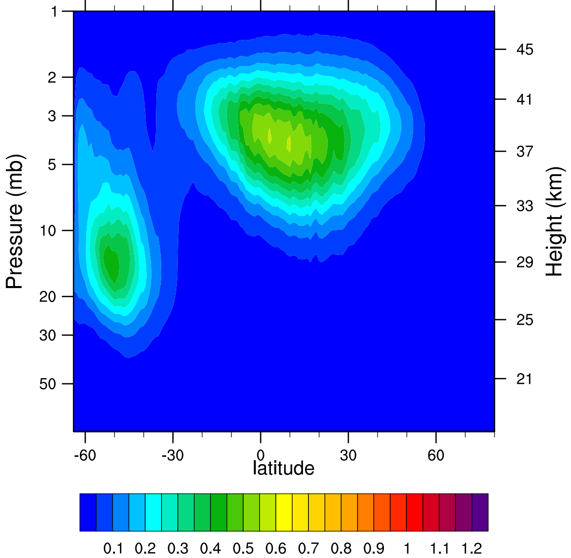
2005d152 N2O5_Ascending (ppbv)
