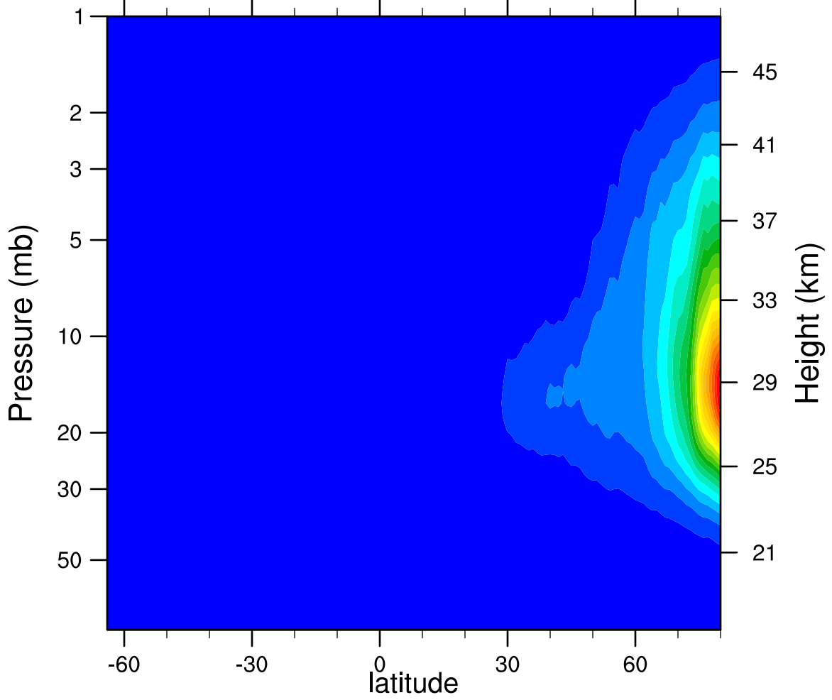
2006d292 N2O5_Ascending (ppbv)
