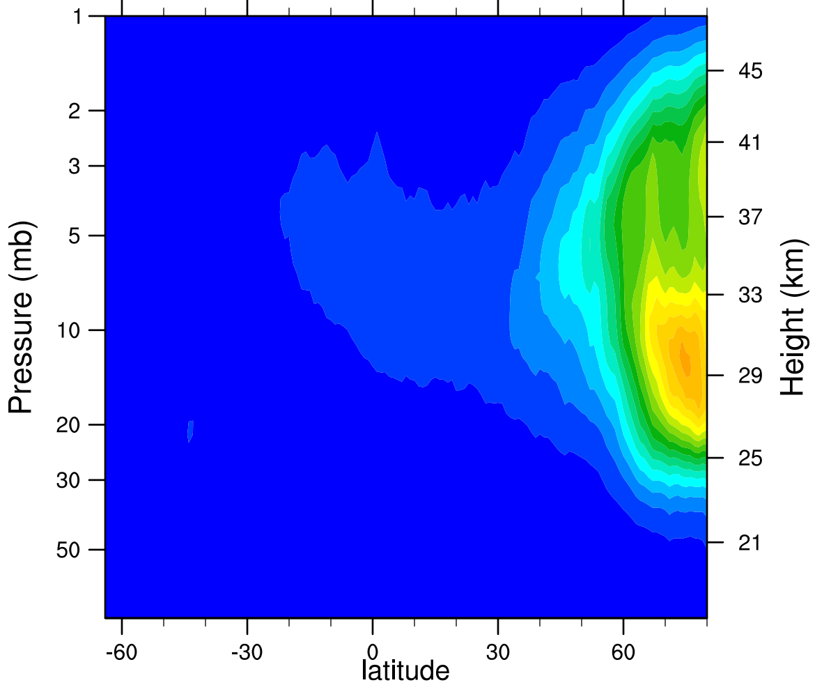
2005d315 N2O5_Ascending (ppbv)
