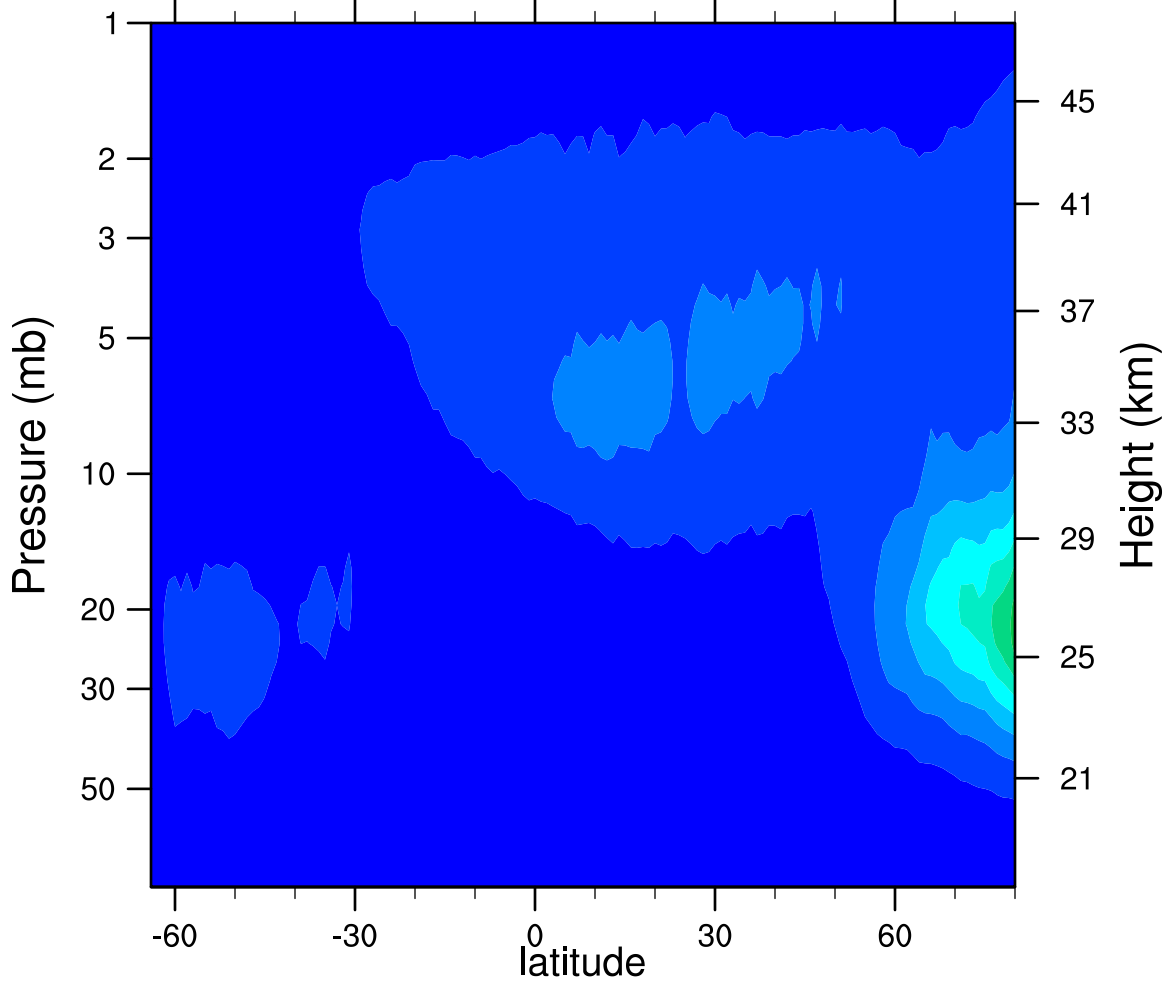
2005d281 N2O5_Ascending (ppbv)
