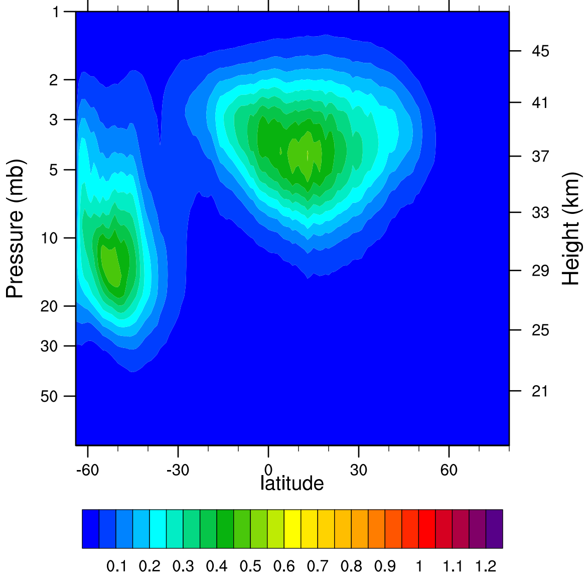
2005d157 N2O5_Ascending (ppbv)
