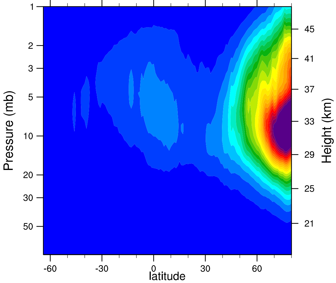
2006d008 N2O5_Ascending (ppbv)
