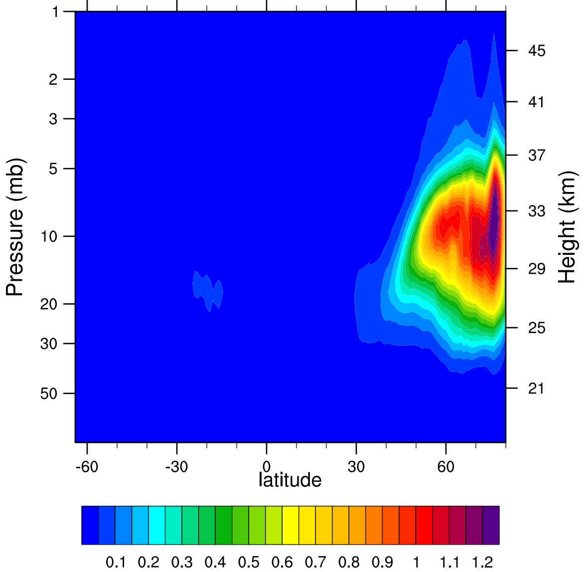
2006d364 N2O5_Ascending (ppbv)
