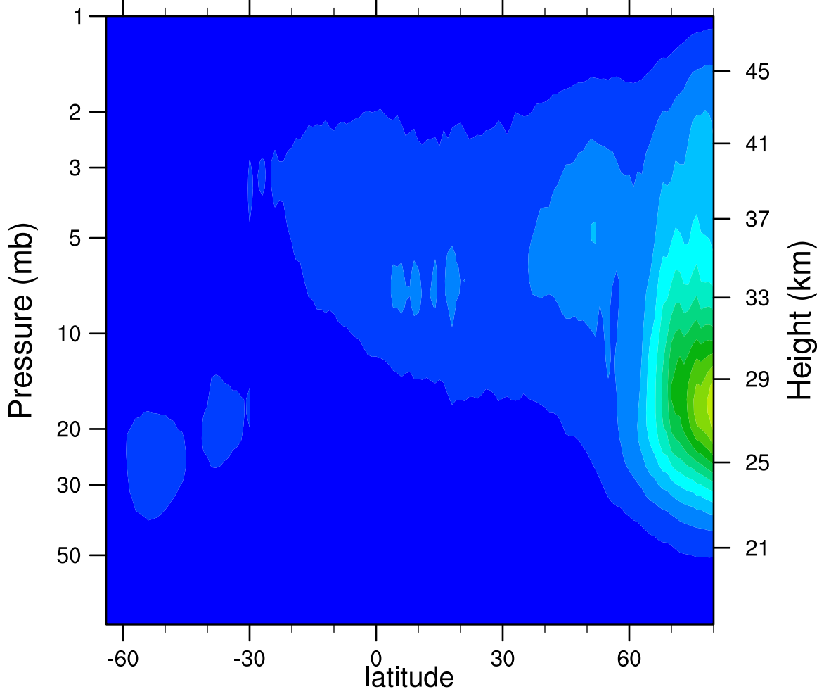
2005d291 N2O5_Ascending (ppbv)
