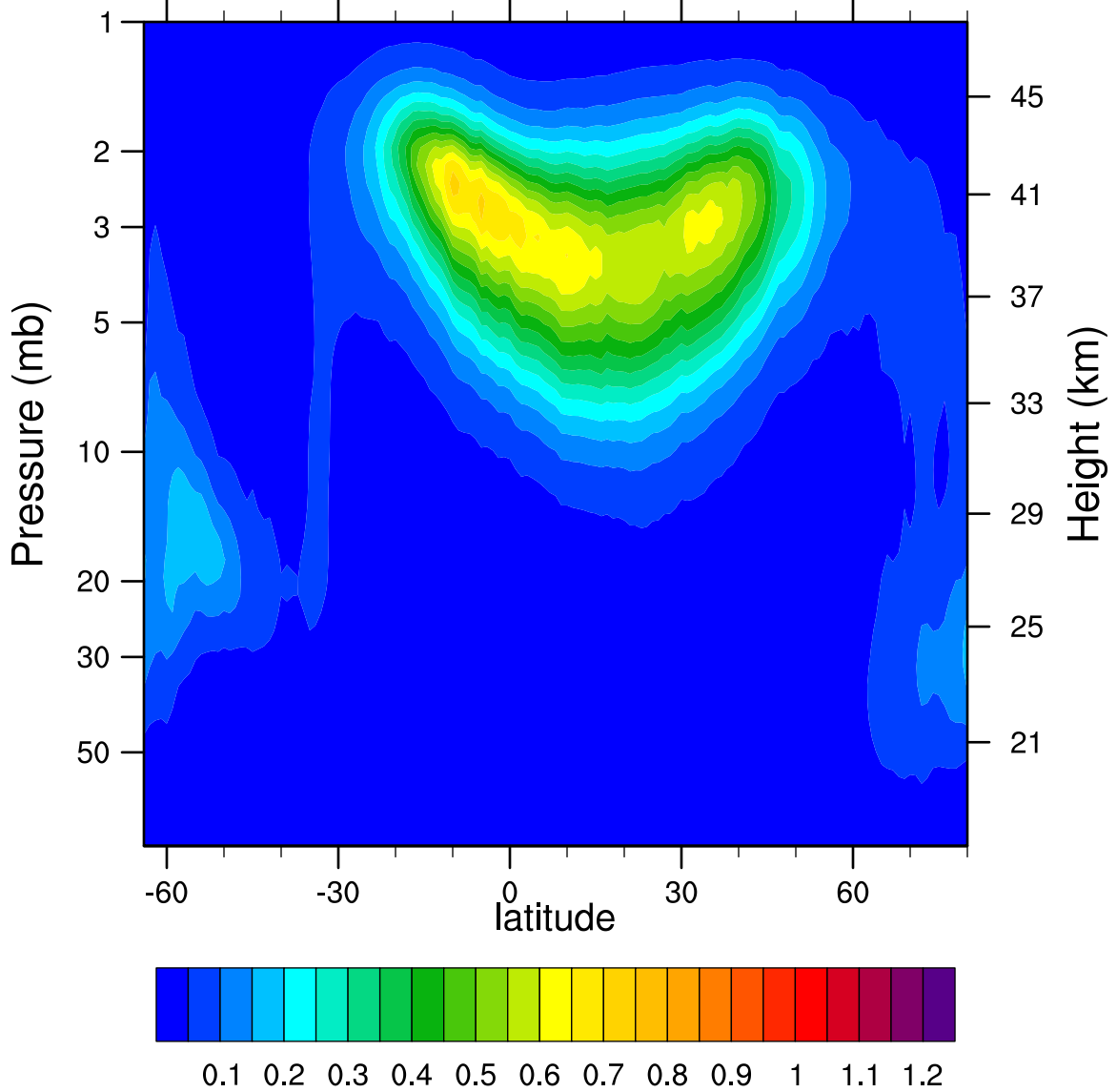
2005d085 N2O5_Ascending (ppbv)
