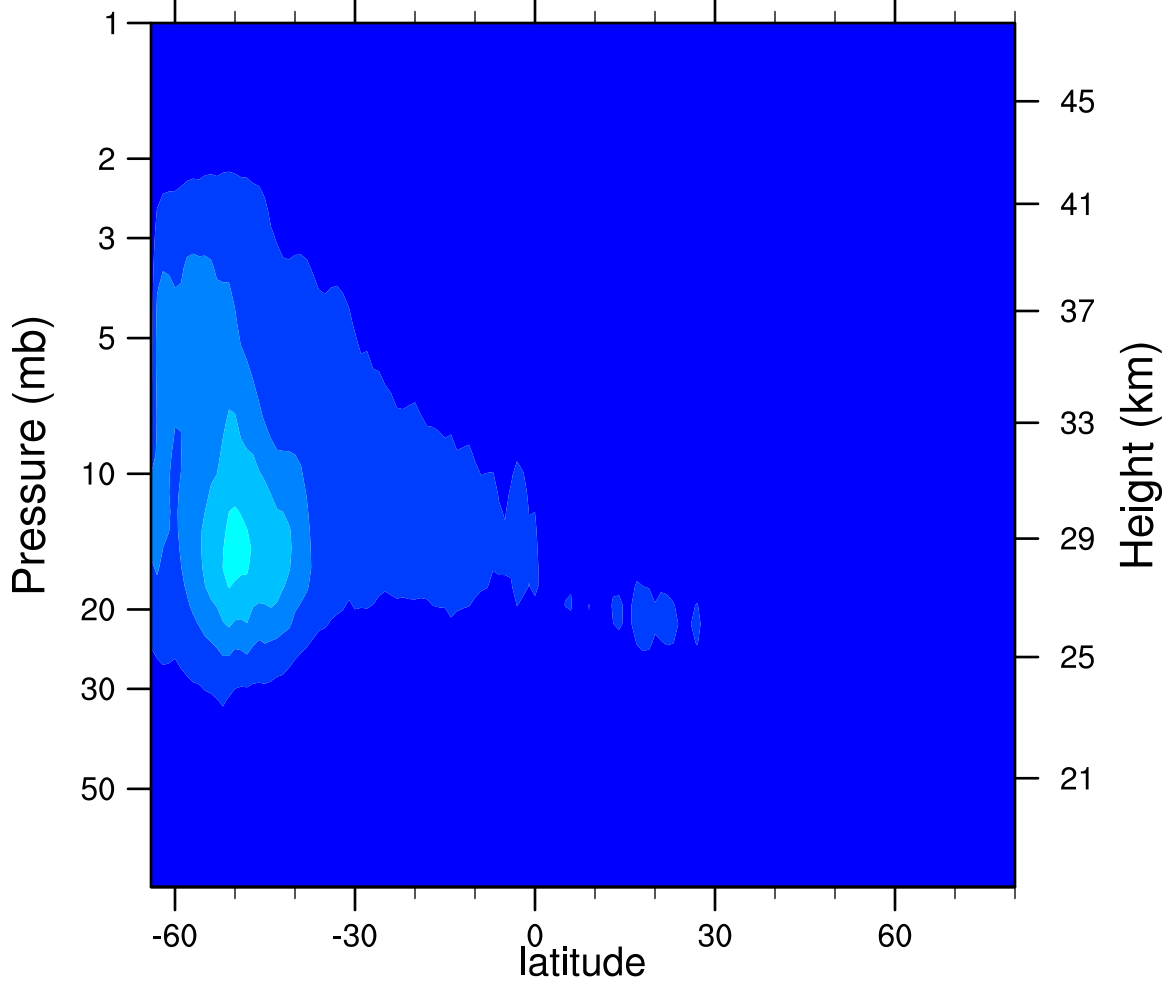
2007d184 N2O5_Ascending (ppbv)
