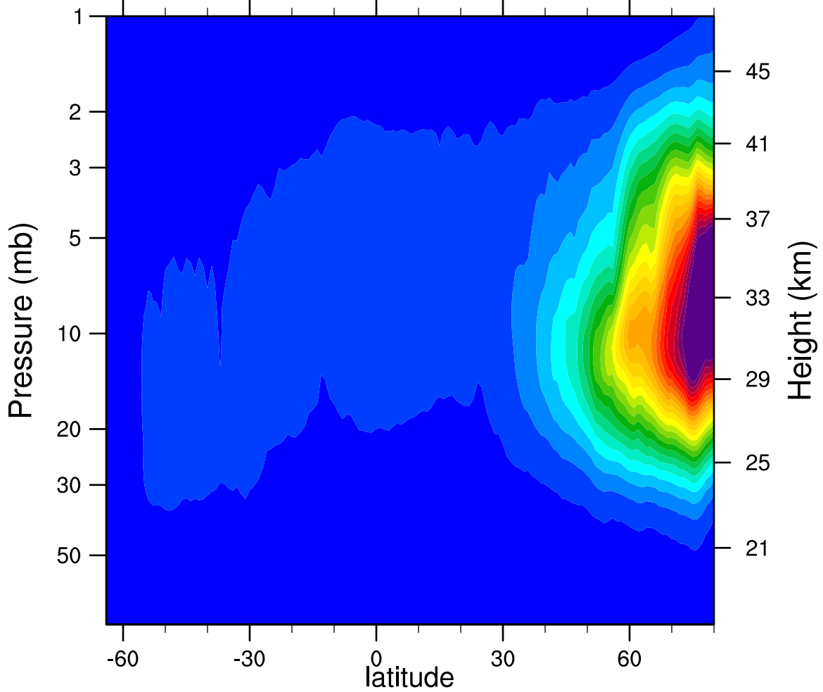
2007d350 N2O5_Ascending (ppbv)
