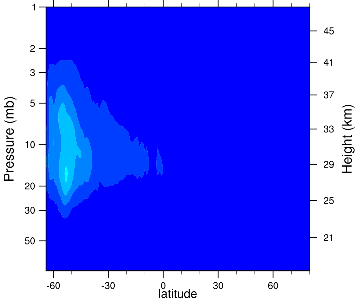
2007d193 N2O5_Ascending (ppbv)
