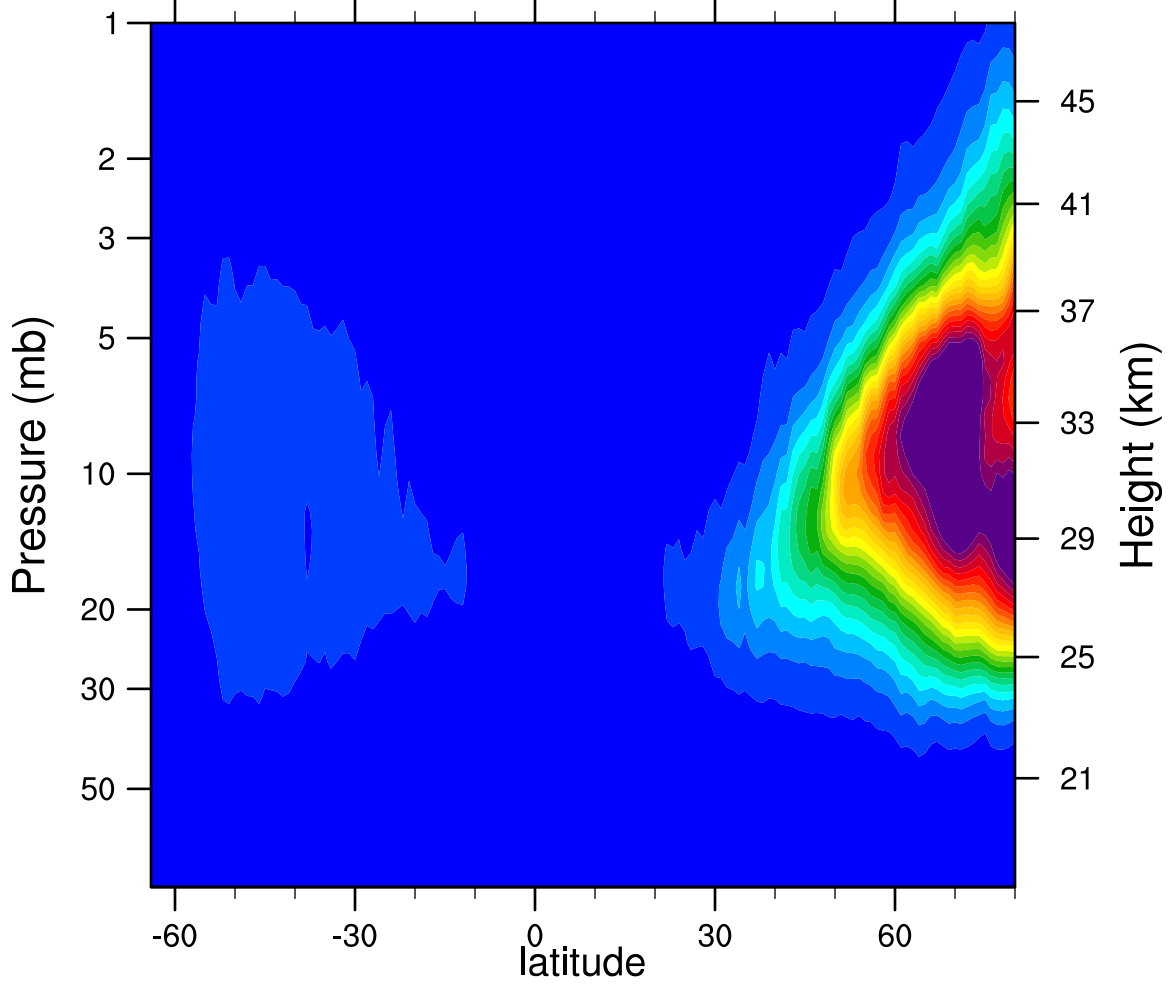
2006d356 N2O5_Ascending (ppbv)
