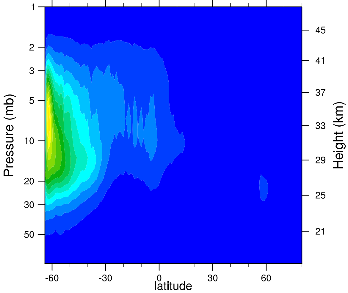
2006d126 N2O5_Ascending (ppbv)
