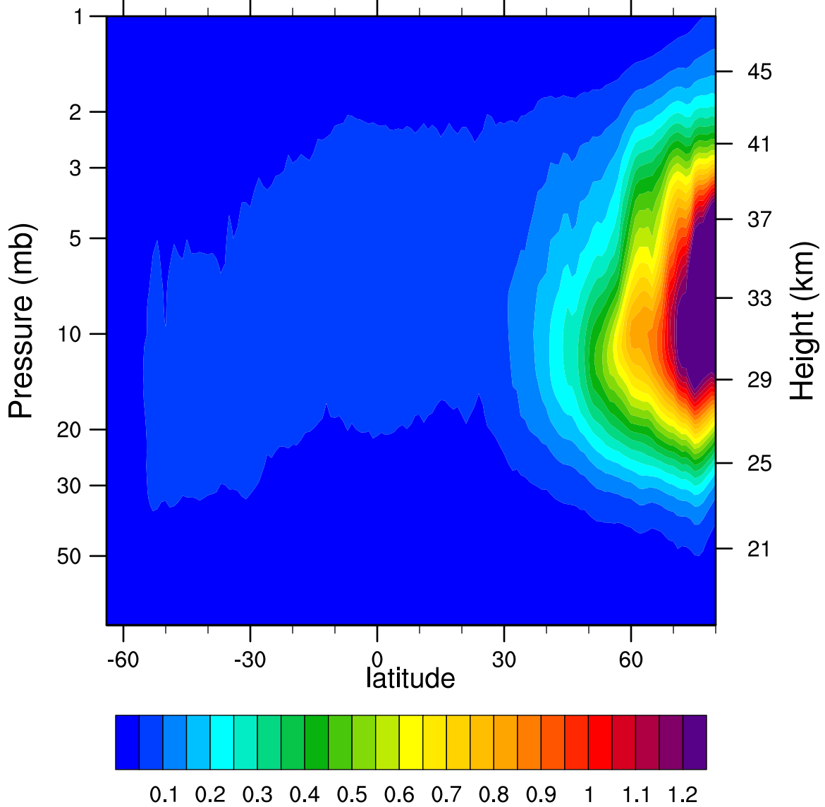
2007d348 N2O5_Ascending (ppbv)
