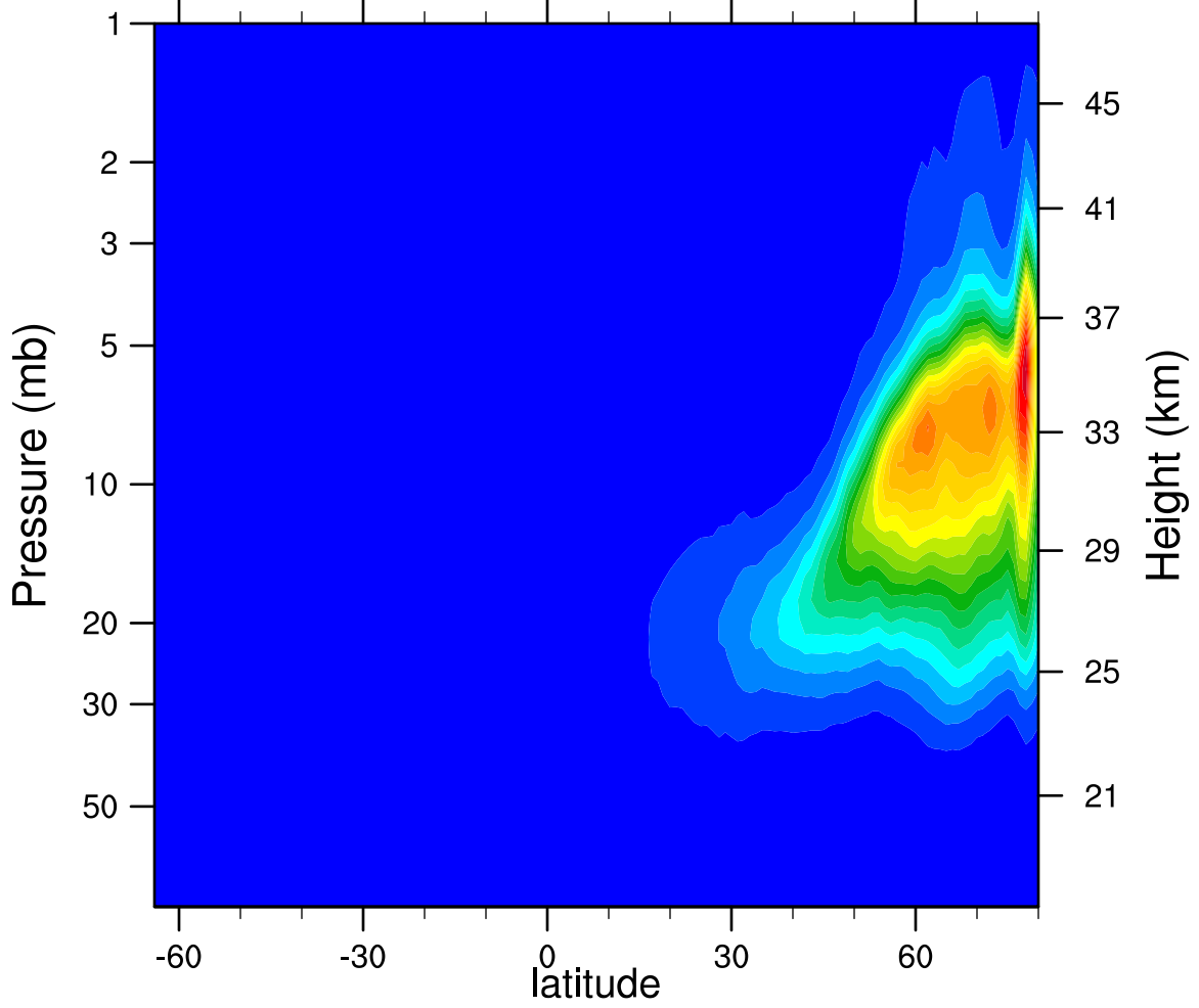
2007d021 N2O5_Ascending (ppbv)
