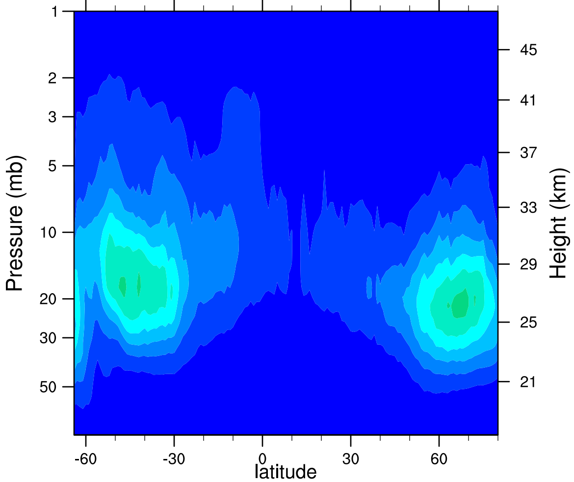
2007d262 N2O5_Ascending (ppbv)
