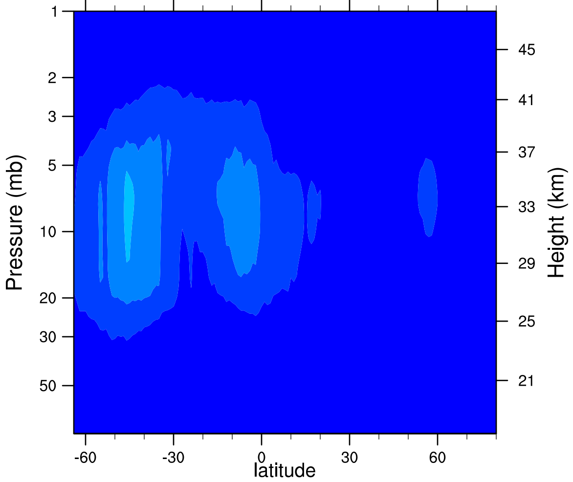
2006d215 N2O5_Ascending (ppbv)
