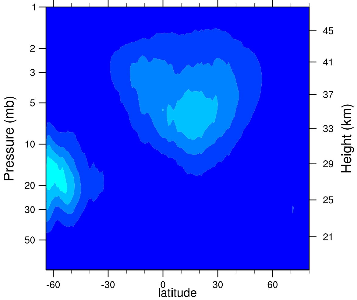
2005d247 N2O5_Ascending (ppbv)
