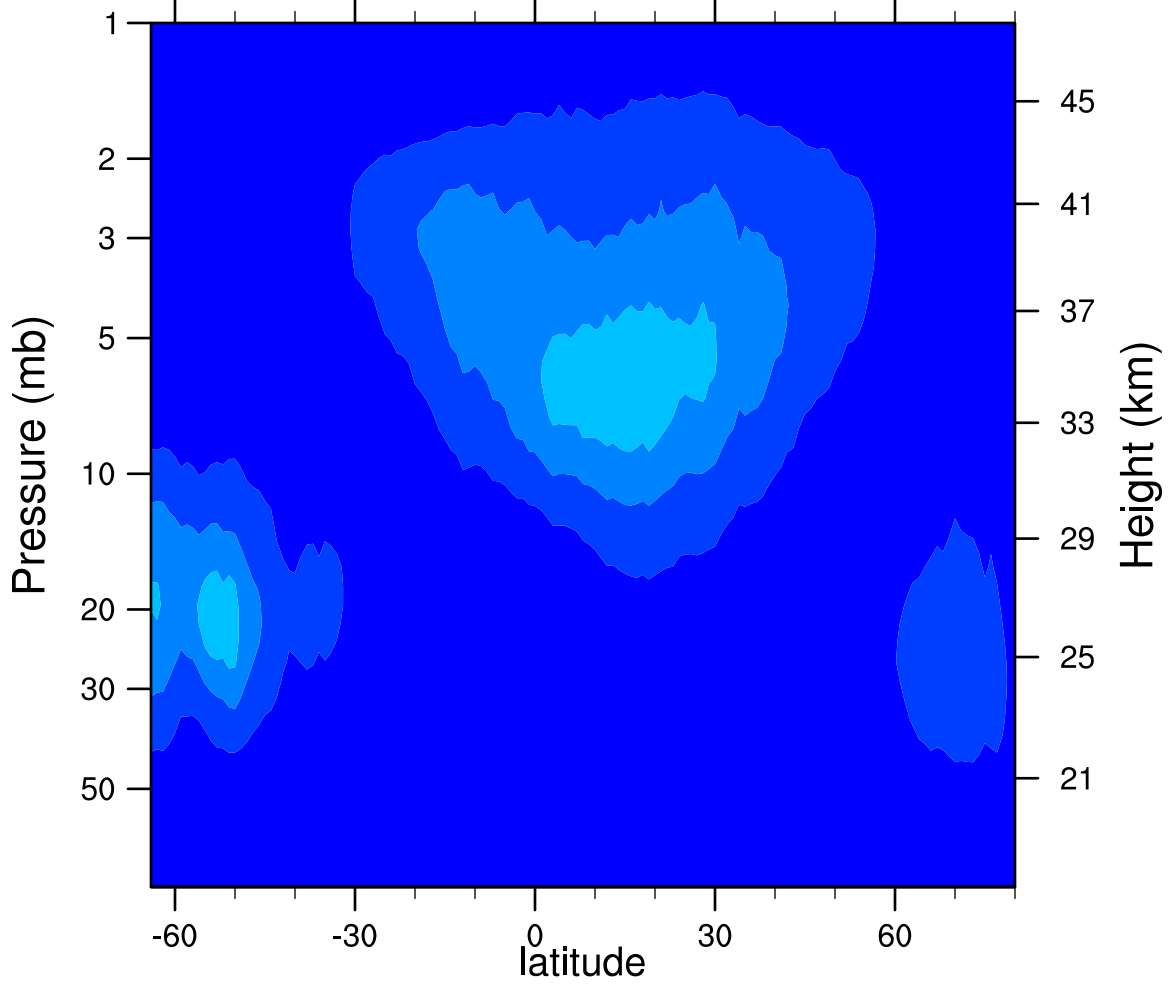
2005d255 N2O5_Ascending (ppbv)
