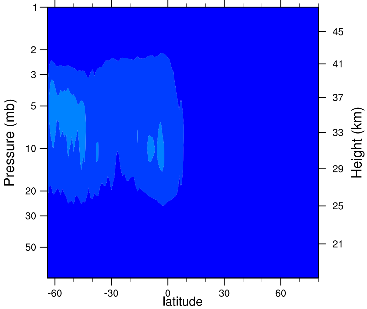
2006d177 N2O5_Ascending (ppbv)
