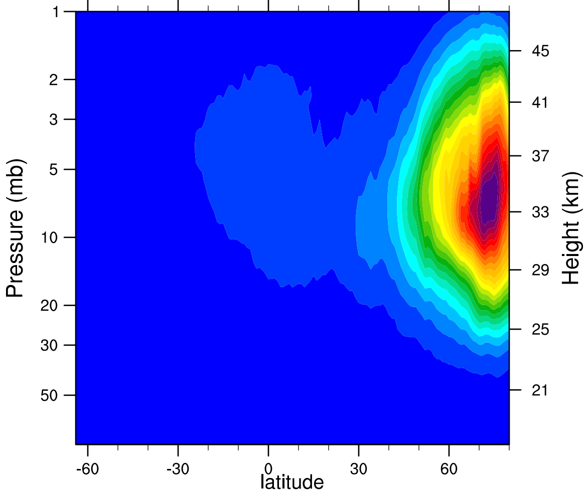
2005d345 N2O5_Ascending (ppbv)
