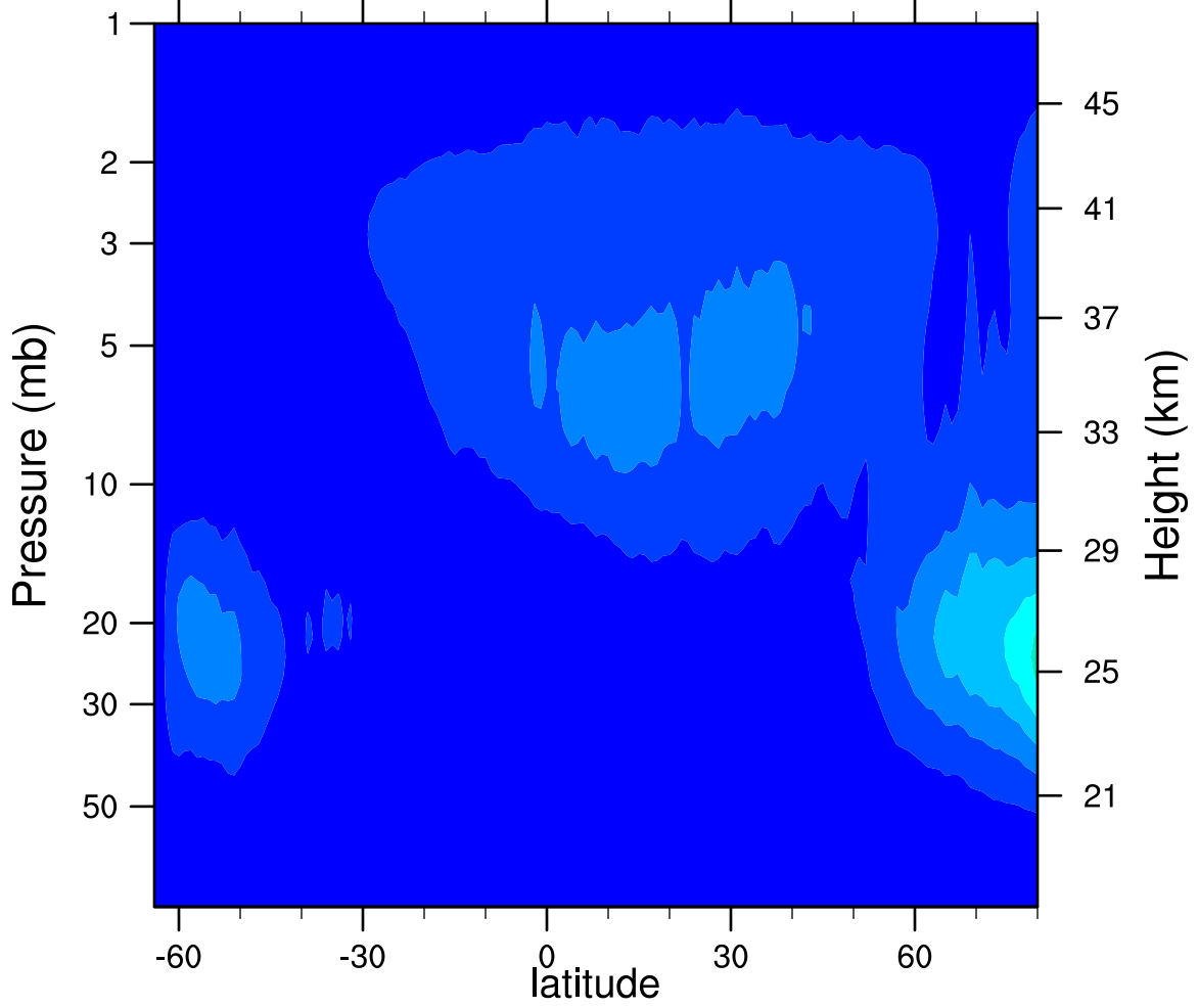
2005d276 N2O5_Ascending (ppbv)
