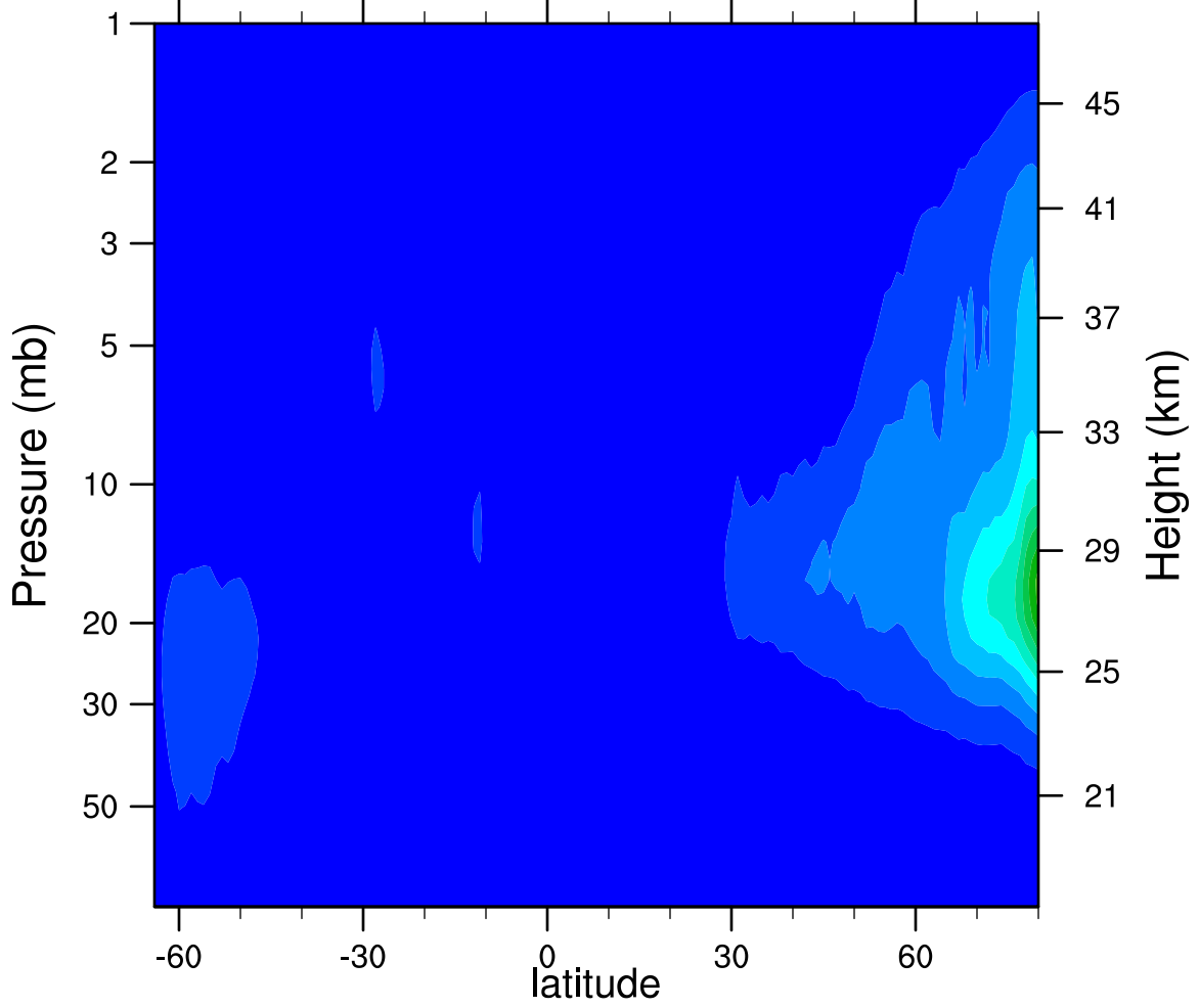
2006d285 N2O5_Ascending (ppbv)
