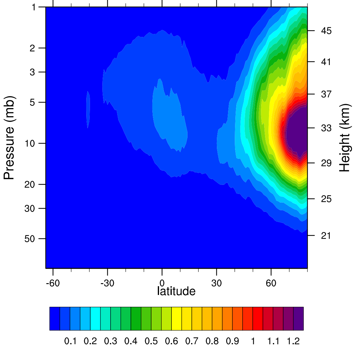
2006d005 N2O5_Ascending (ppbv)
