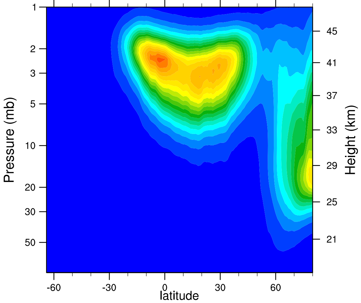
2005d040 N2O5_Ascending (ppbv)
