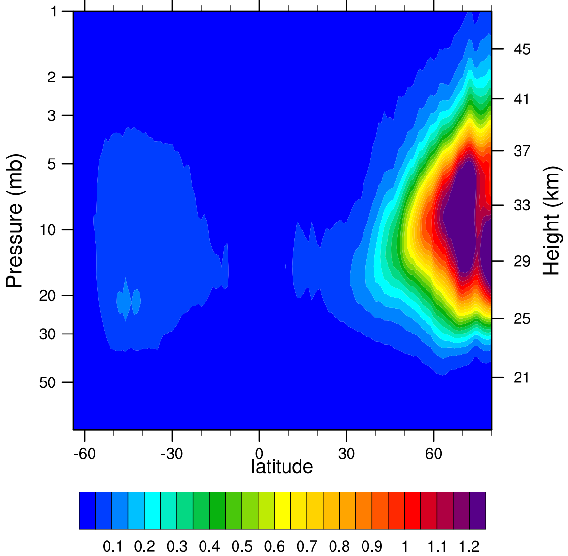
2006d352 N2O5_Ascending (ppbv)
