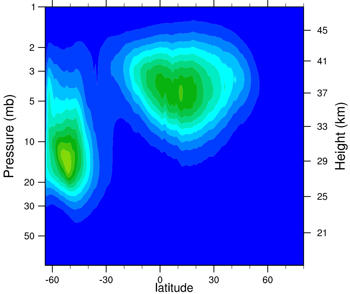
2005d160 N2O5_Ascending (ppbv)
