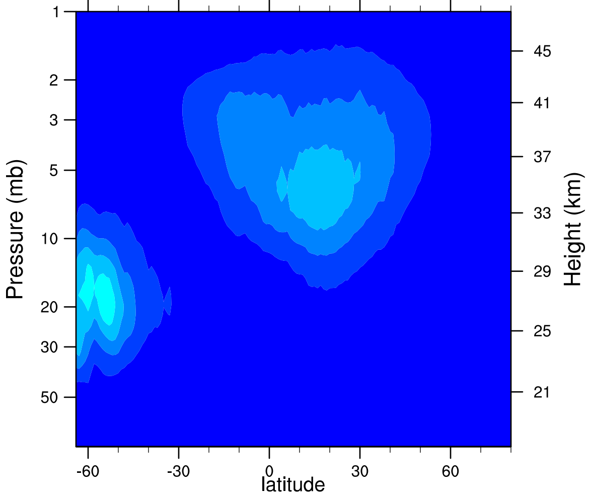
2005d244 N2O5_Ascending (ppbv)
