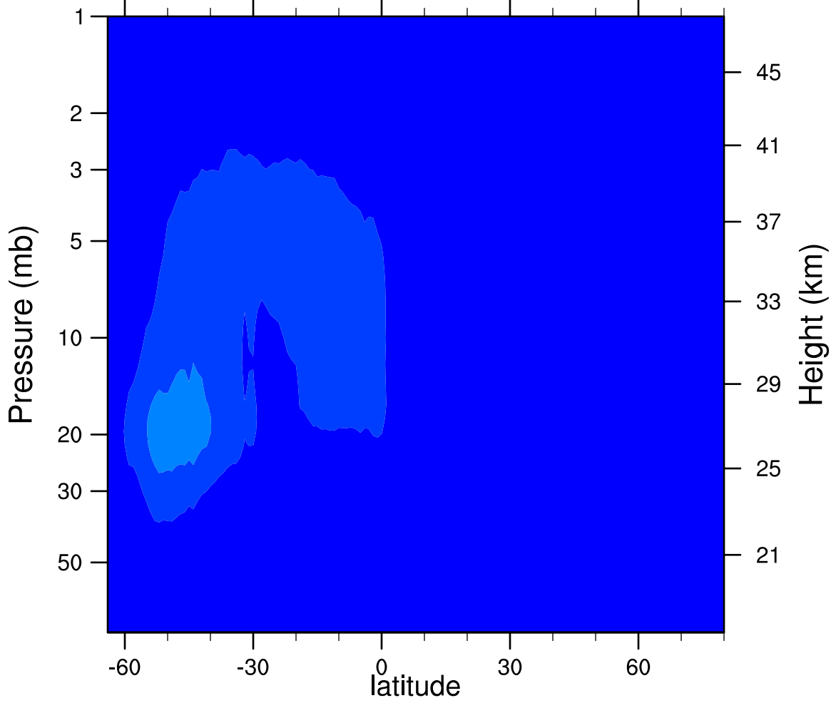
2006d246 N2O5_Ascending (ppbv)
