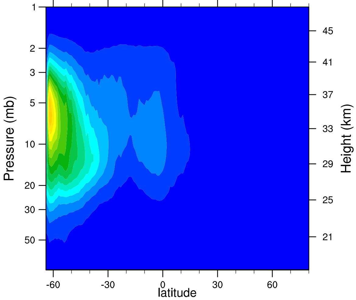
2006d144 N2O5_Ascending (ppbv)
