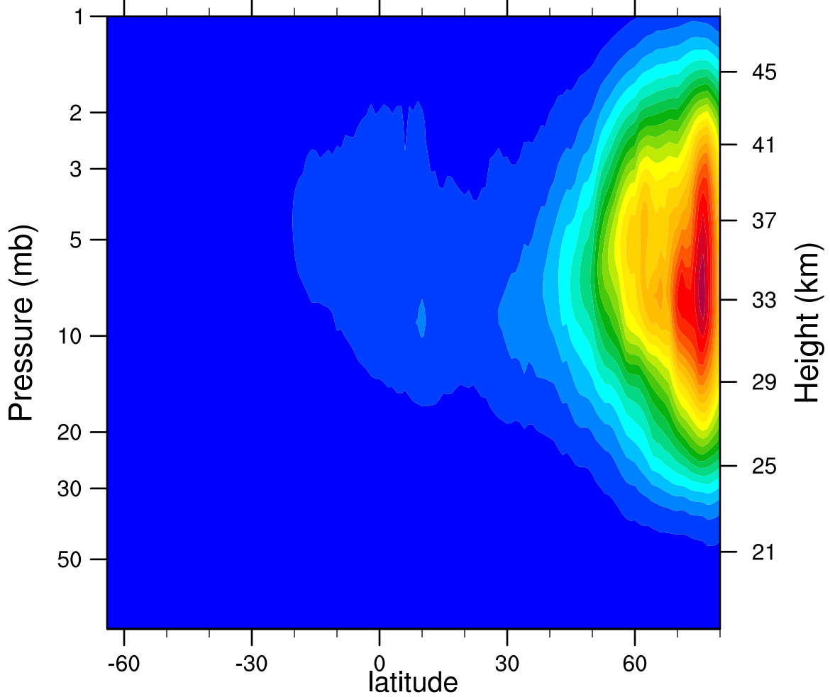
2005d335 N2O5_Ascending (ppbv)
