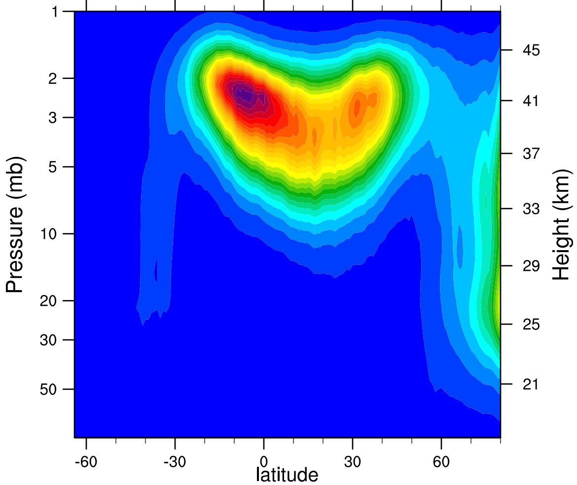
2005d056 N2O5_Ascending (ppbv)
