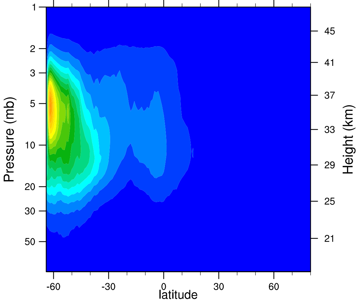
2006d148 N2O5_Ascending (ppbv)
