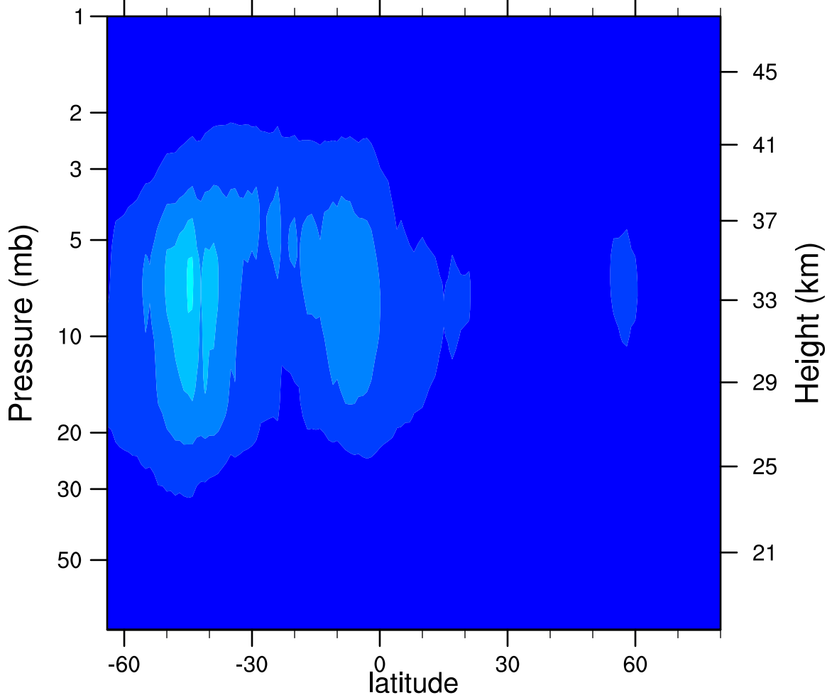
2006d213 N2O5_Ascending (ppbv)
