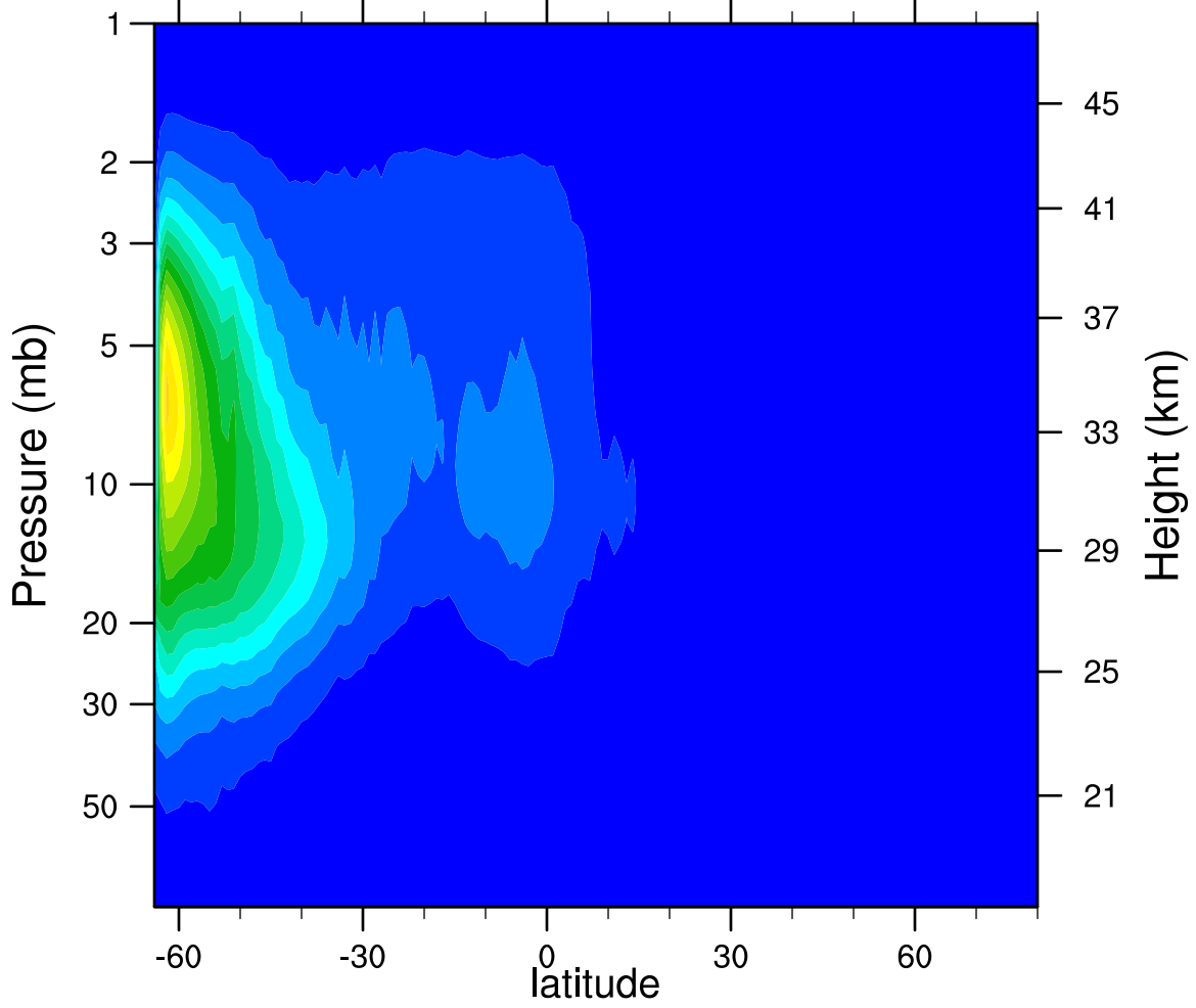
2006d140 N2O5_Ascending (ppbv)
