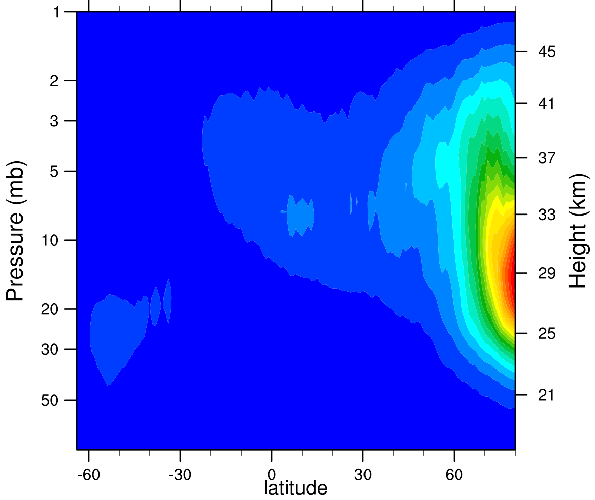
2005d300 N2O5_Ascending (ppbv)
