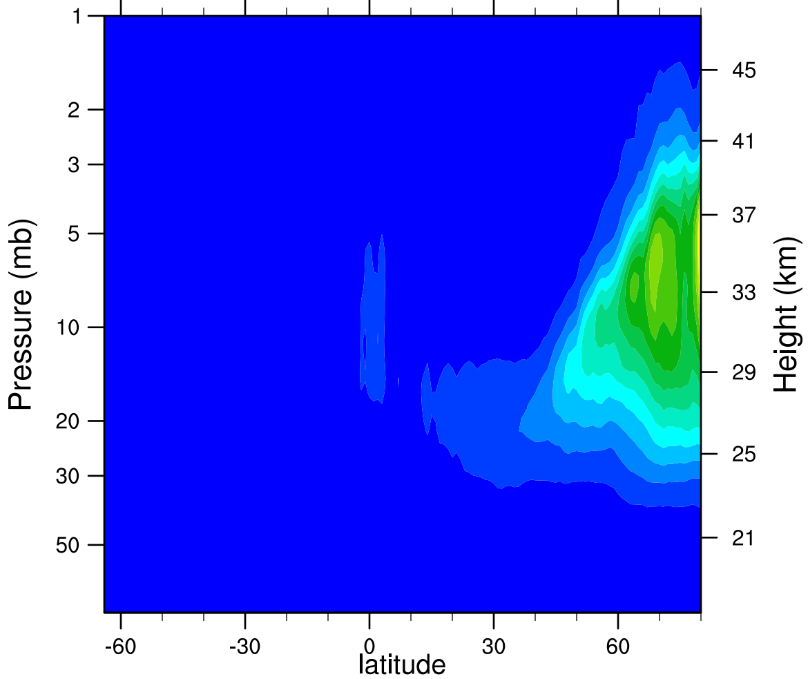
2007d043 N2O5_Ascending (ppbv)
