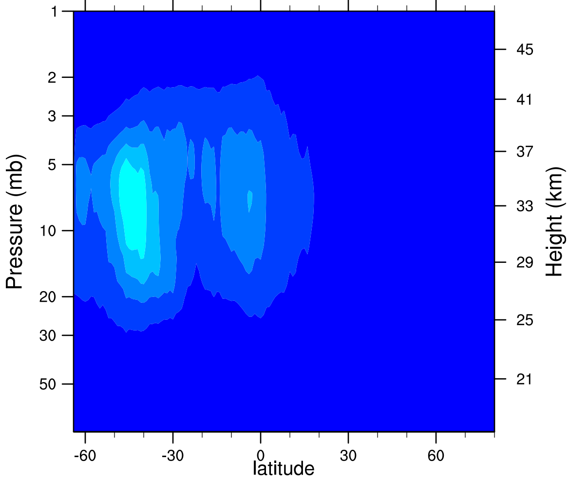
2006d194 N2O5_Ascending (ppbv)
