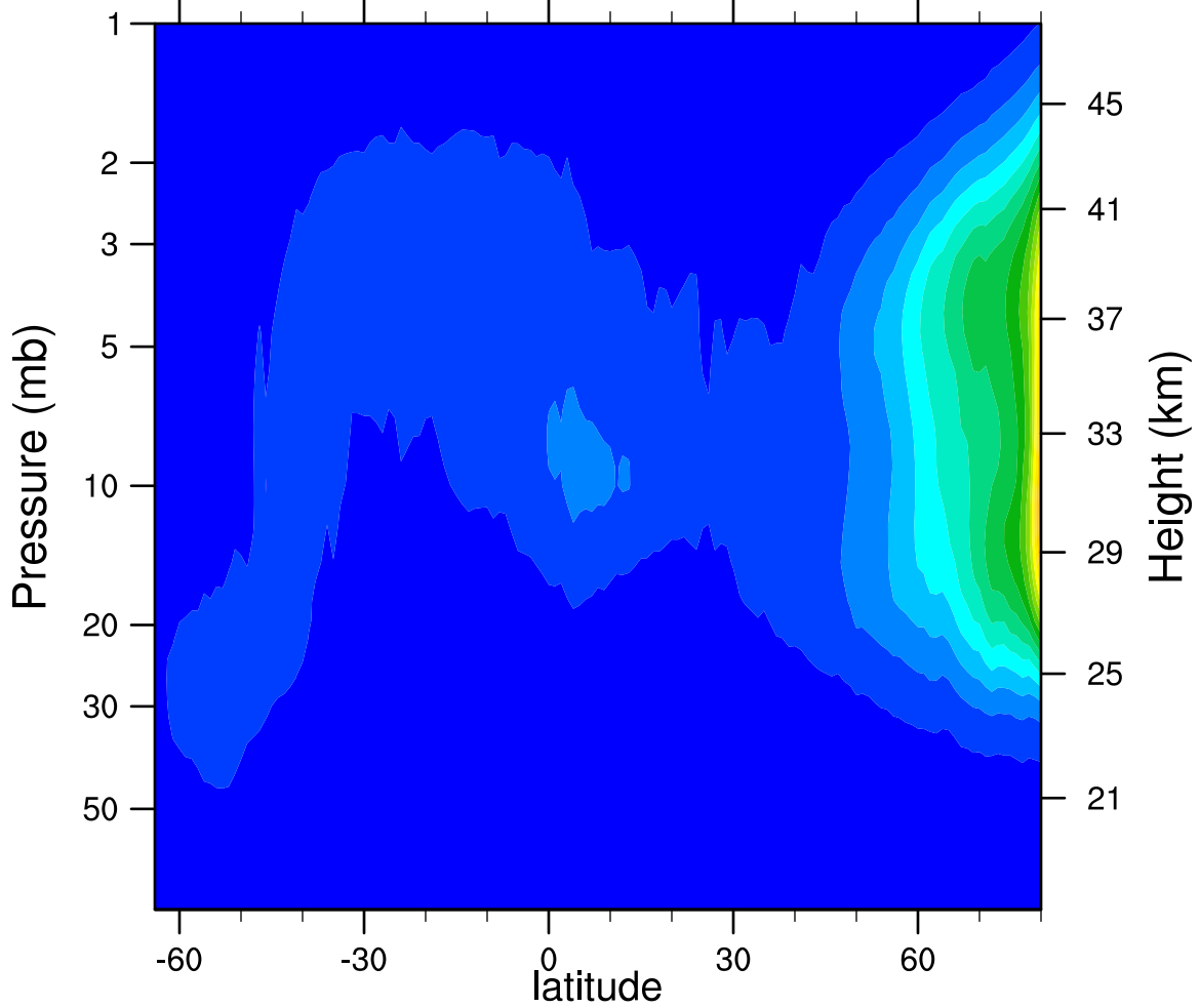
2006d055 N2O5_Ascending (ppbv)
