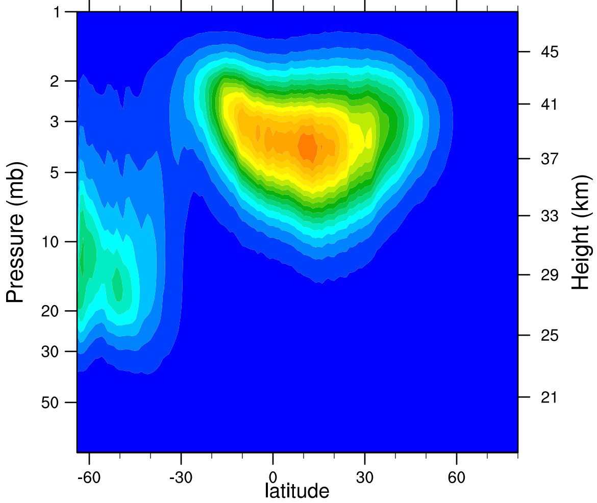
2005d122 N2O5_Ascending (ppbv)
