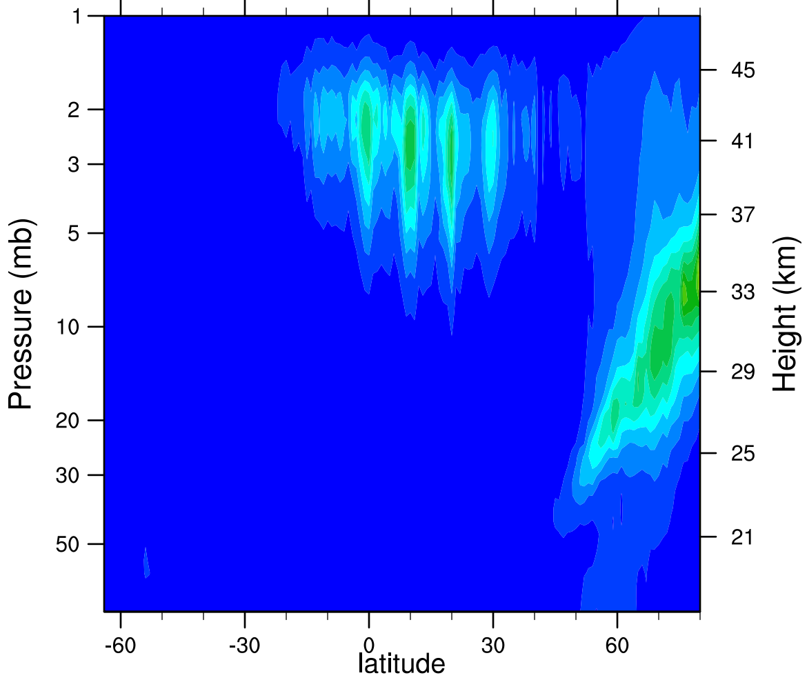
2005d024 N2O5_Ascending (ppbv)
