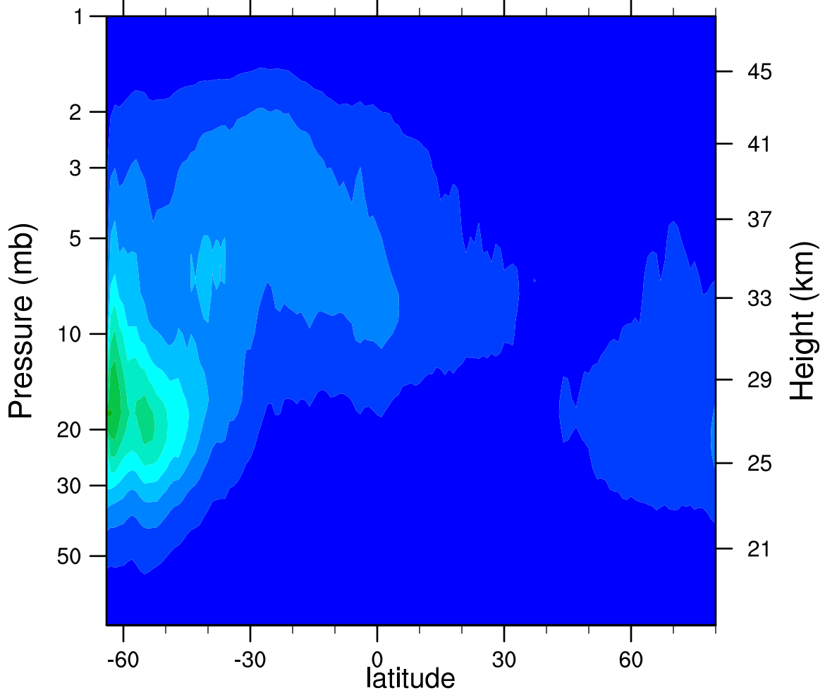
2006d098 N2O5_Ascending (ppbv)
