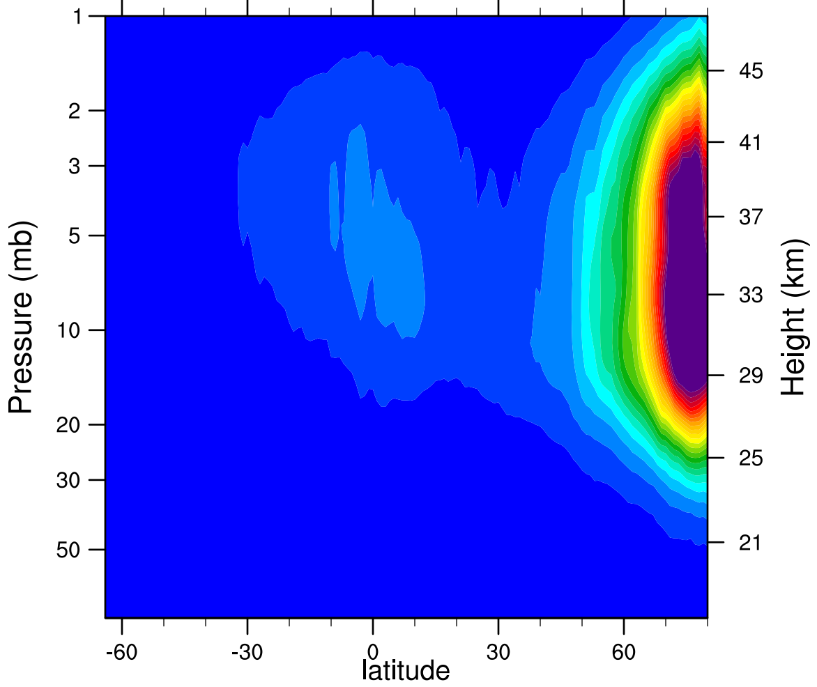
2006d020 N2O5_Ascending (ppbv)
