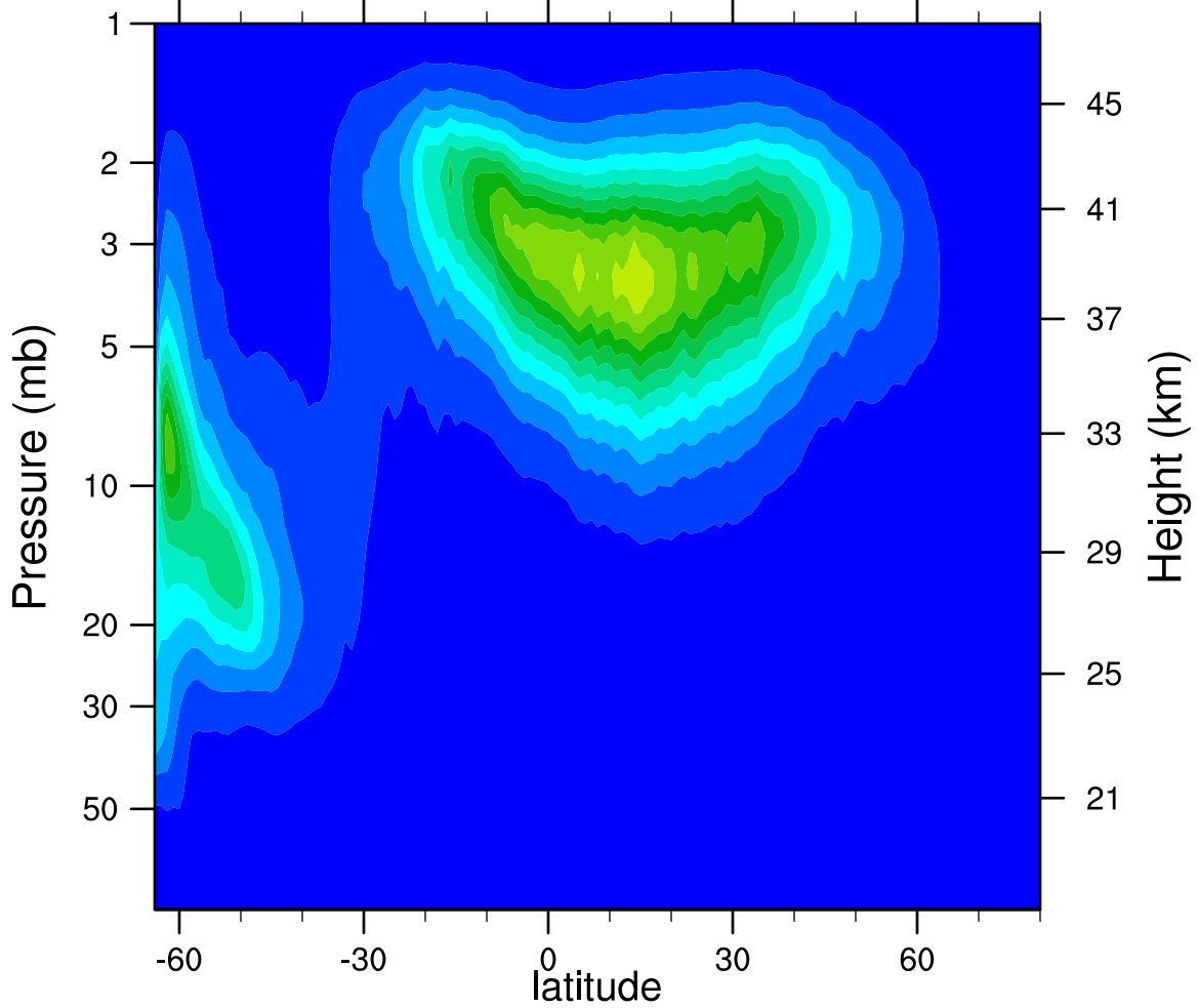
2005d111 N2O5_Ascending (ppbv)
