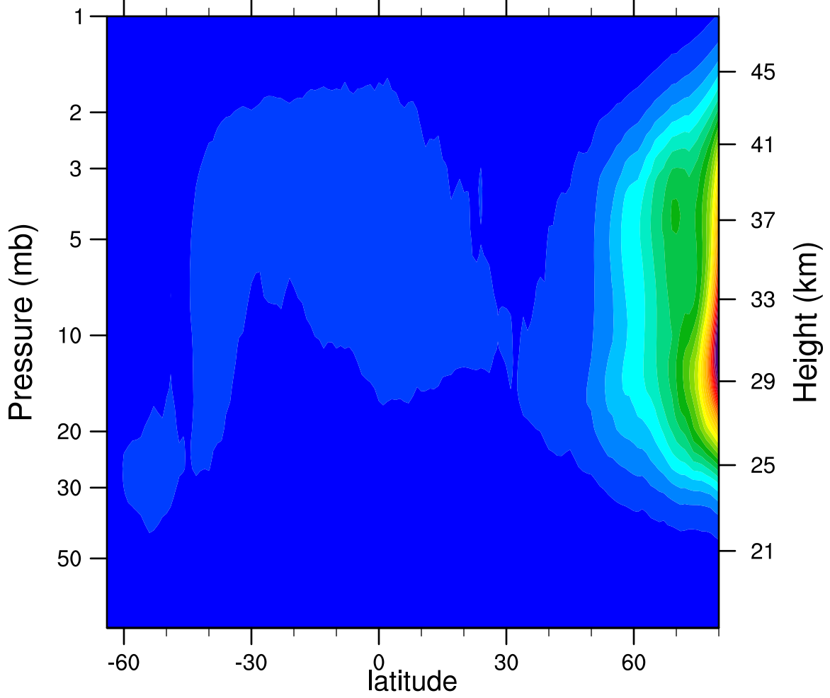
2006d050 N2O5_Ascending (ppbv)
