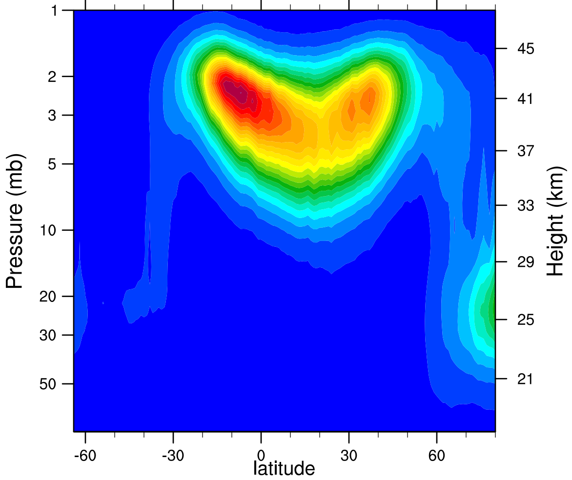
2005d064 N2O5_Ascending (ppbv)
