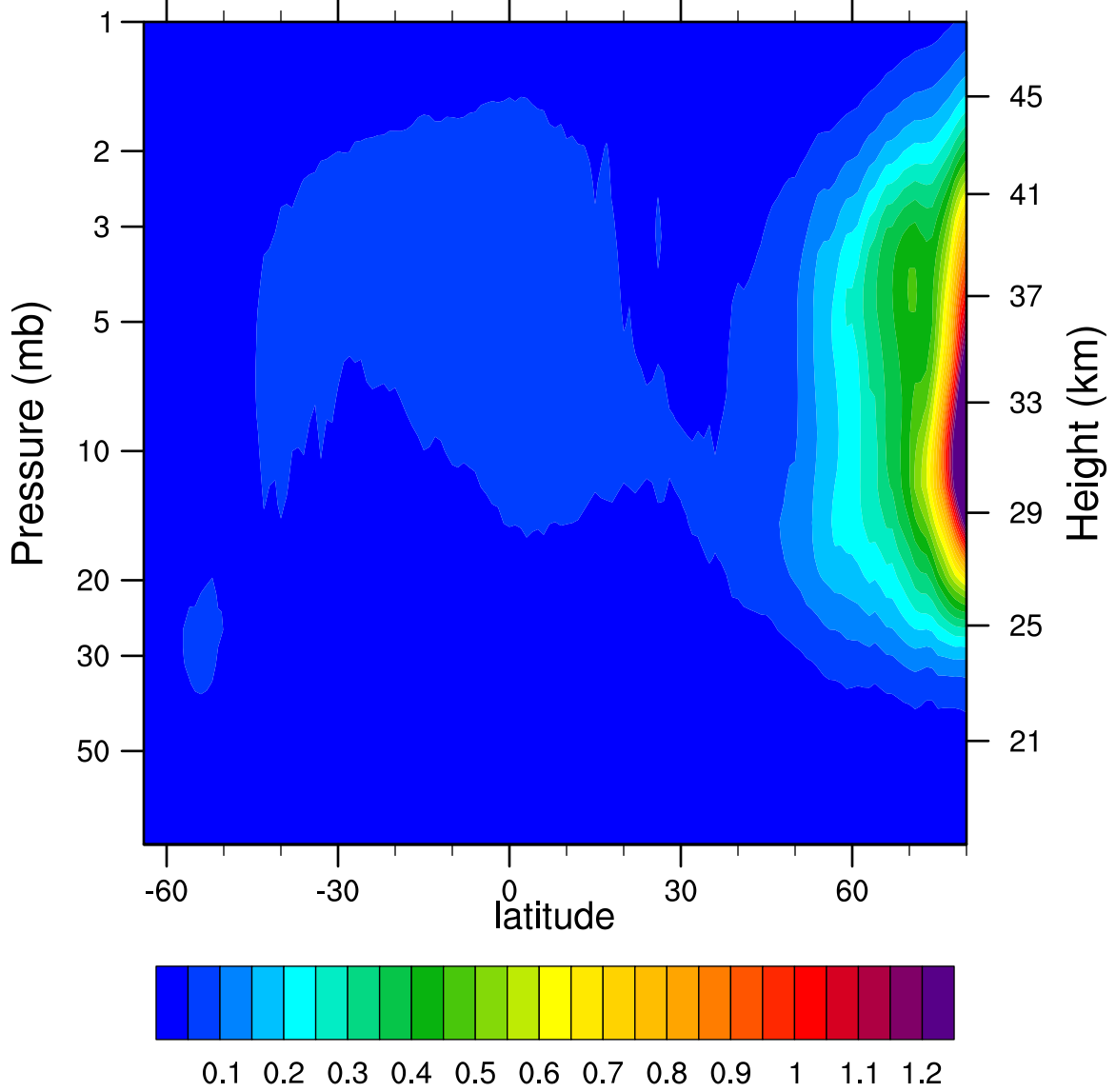
2006d045 N2O5_Ascending (ppbv)
