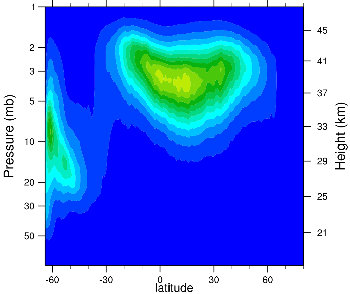
2005d108 N2O5_Ascending (ppbv)
