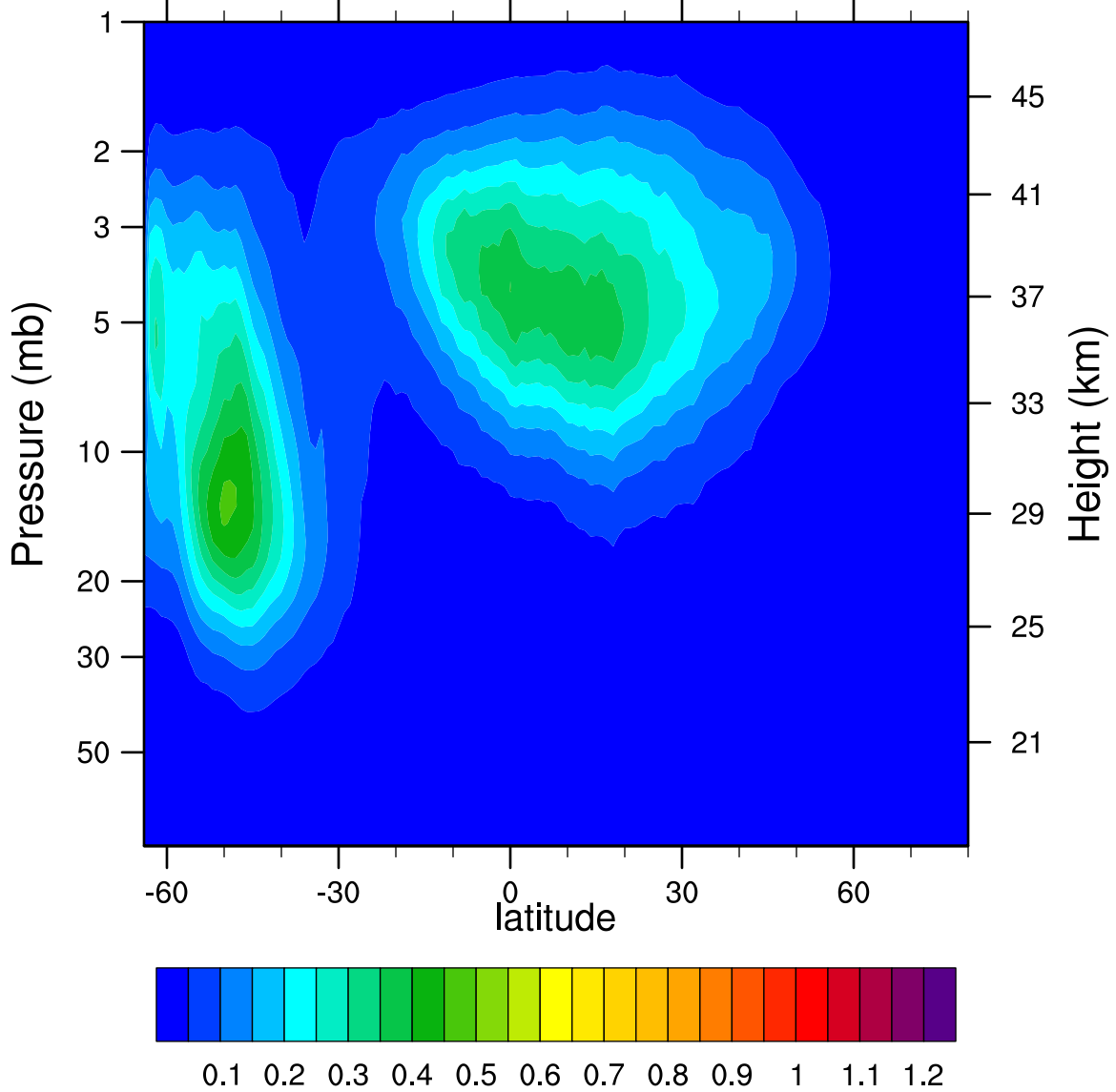
2005d177 N2O5_Ascending (ppbv)
