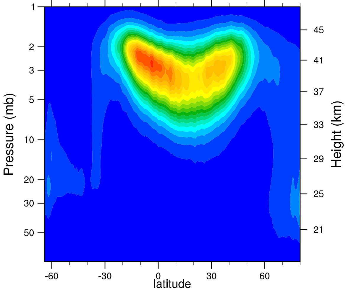
2005d074 N2O5_Ascending (ppbv)
