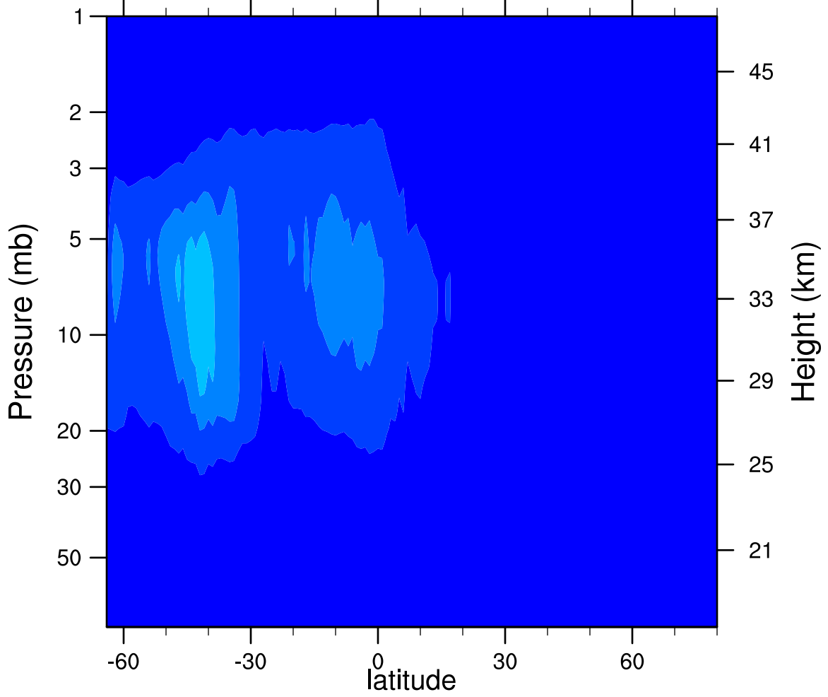
2006d190 N2O5_Ascending (ppbv)
