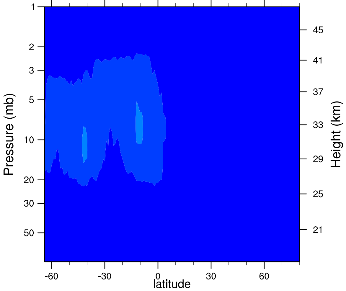
2006d187 N2O5_Ascending (ppbv)
