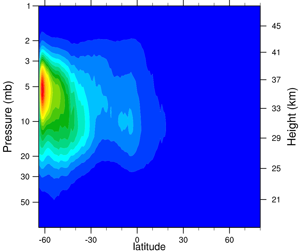
2006d160 N2O5_Ascending (ppbv)
