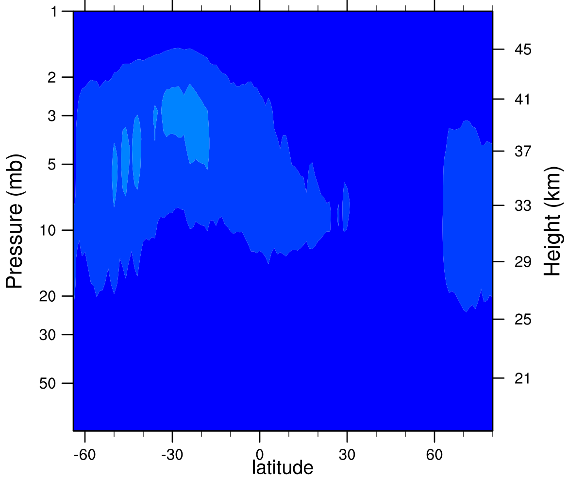
2006d091 N2O5_Ascending (ppbv)
