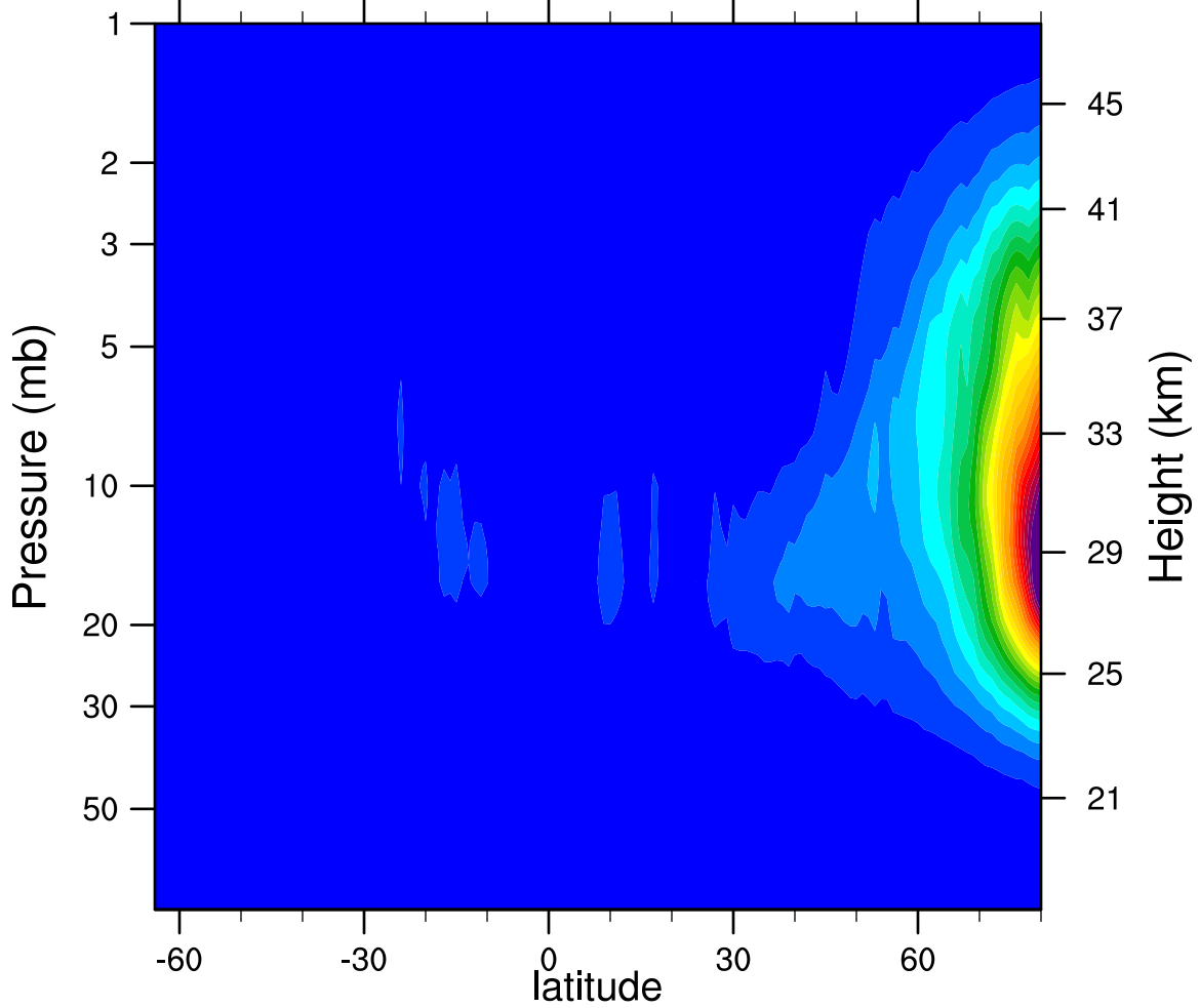
2006d297 N2O5_Ascending (ppbv)
