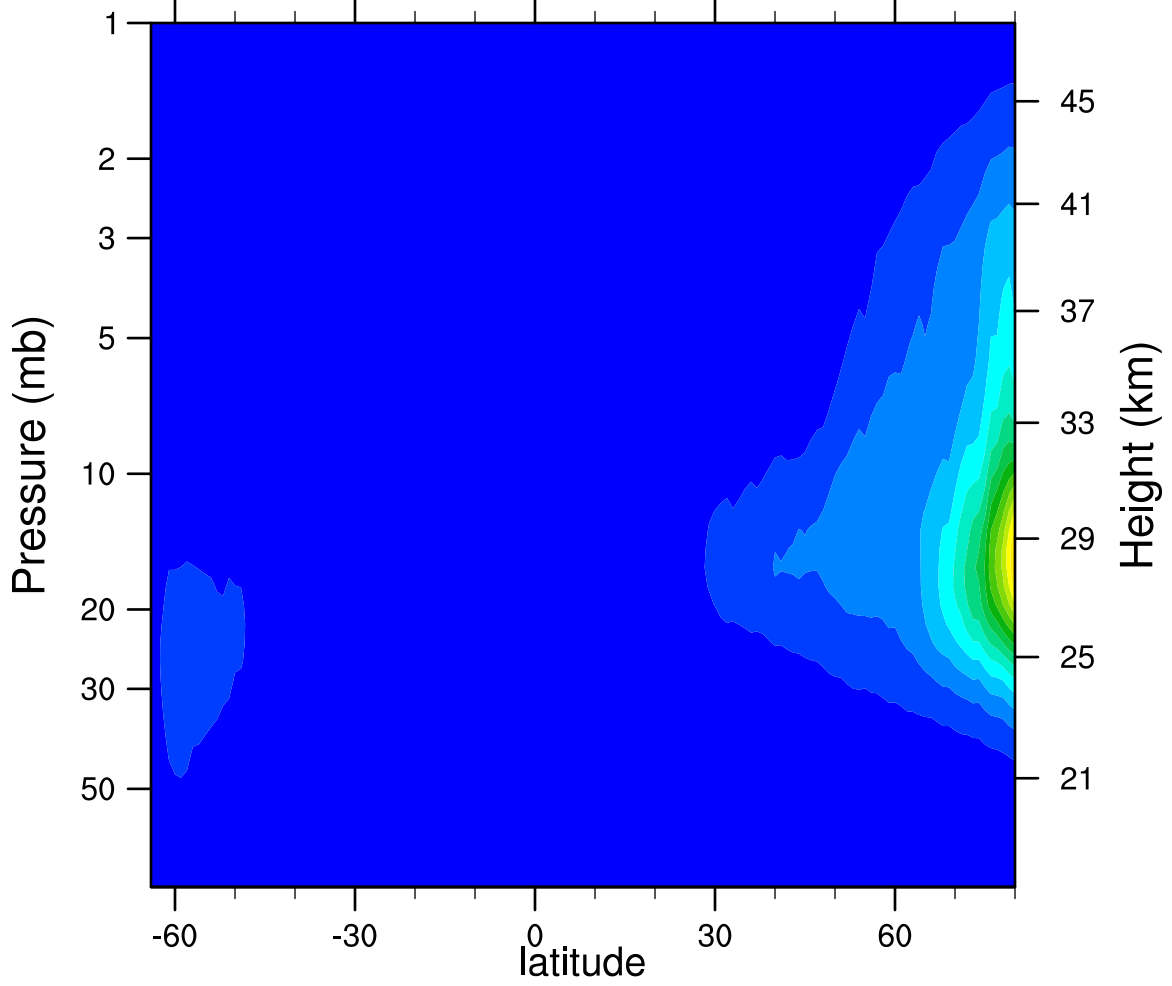
2006d288 N2O5_Ascending (ppbv)
