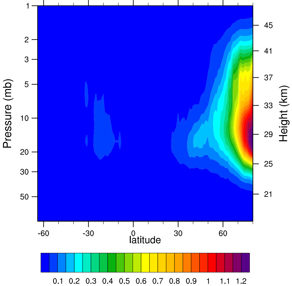
2006d306 N2O5_Ascending (ppbv)
