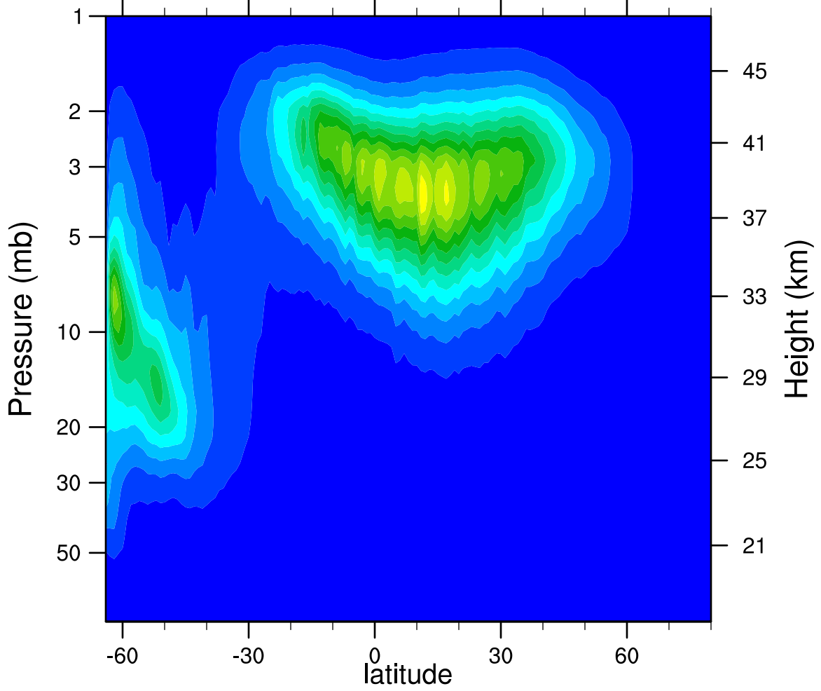
2005d115 N2O5_Ascending (ppbv)
