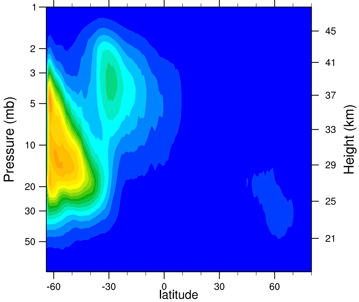
2007d118 N2O5_Ascending (ppbv)
