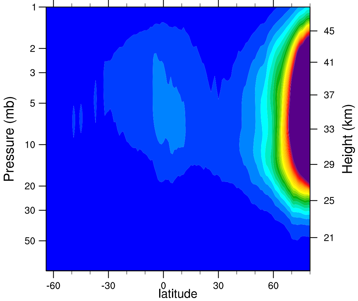
2006d025 N2O5_Ascending (ppbv)
