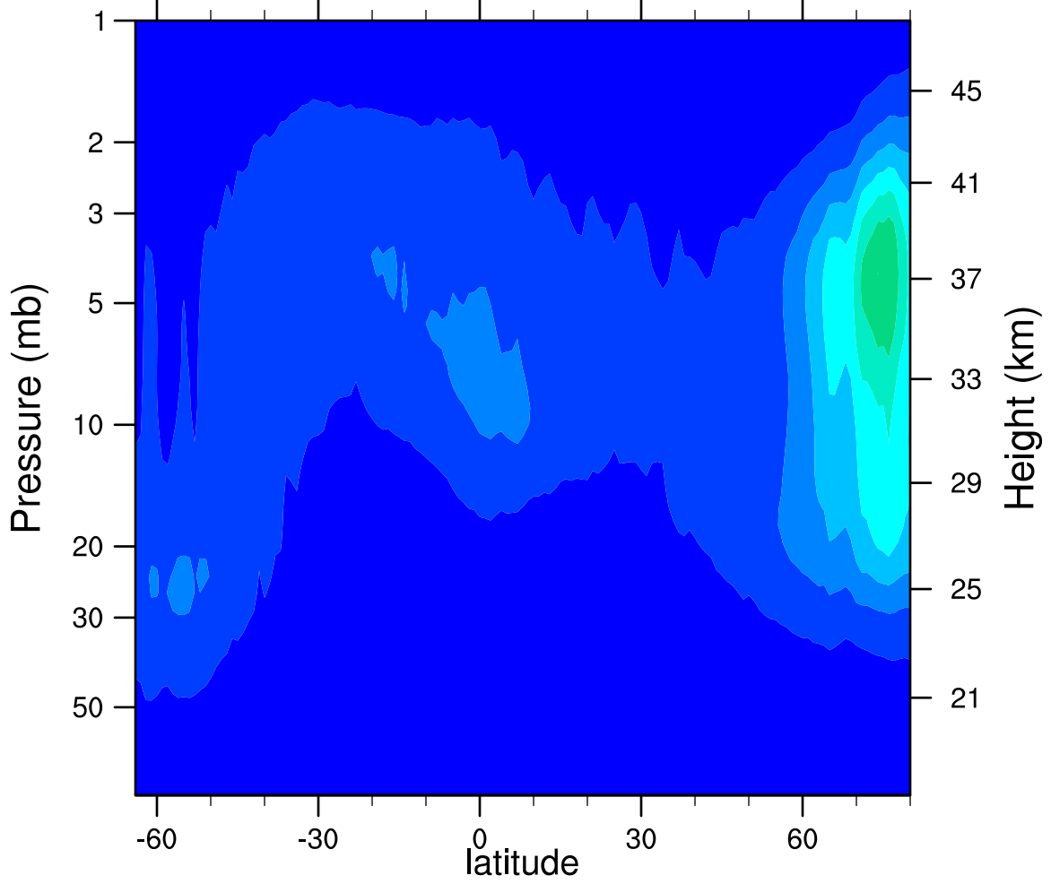
2006d068 N2O5_Ascending (ppbv)
