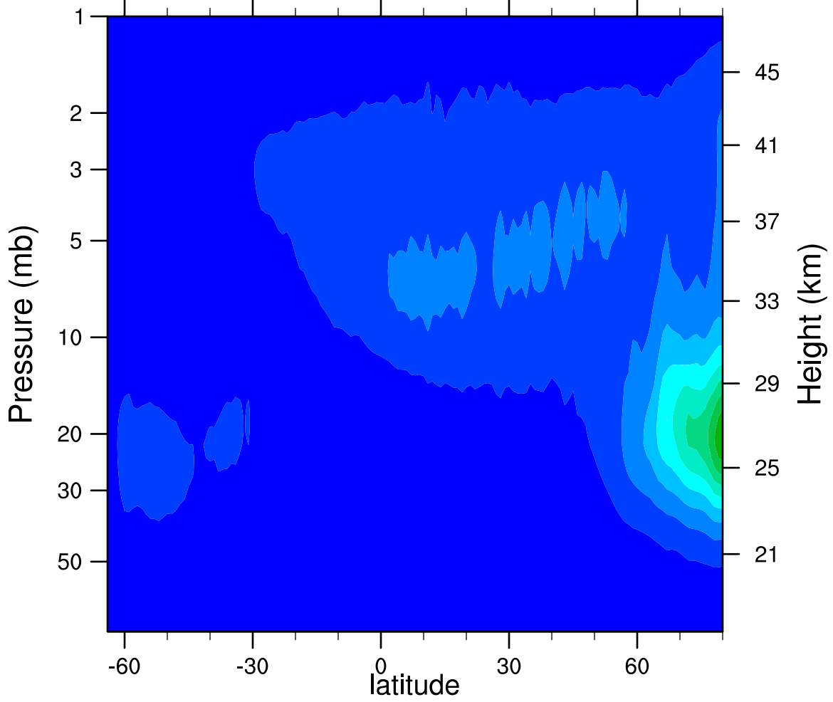
2005d284 N2O5_Ascending (ppbv)
