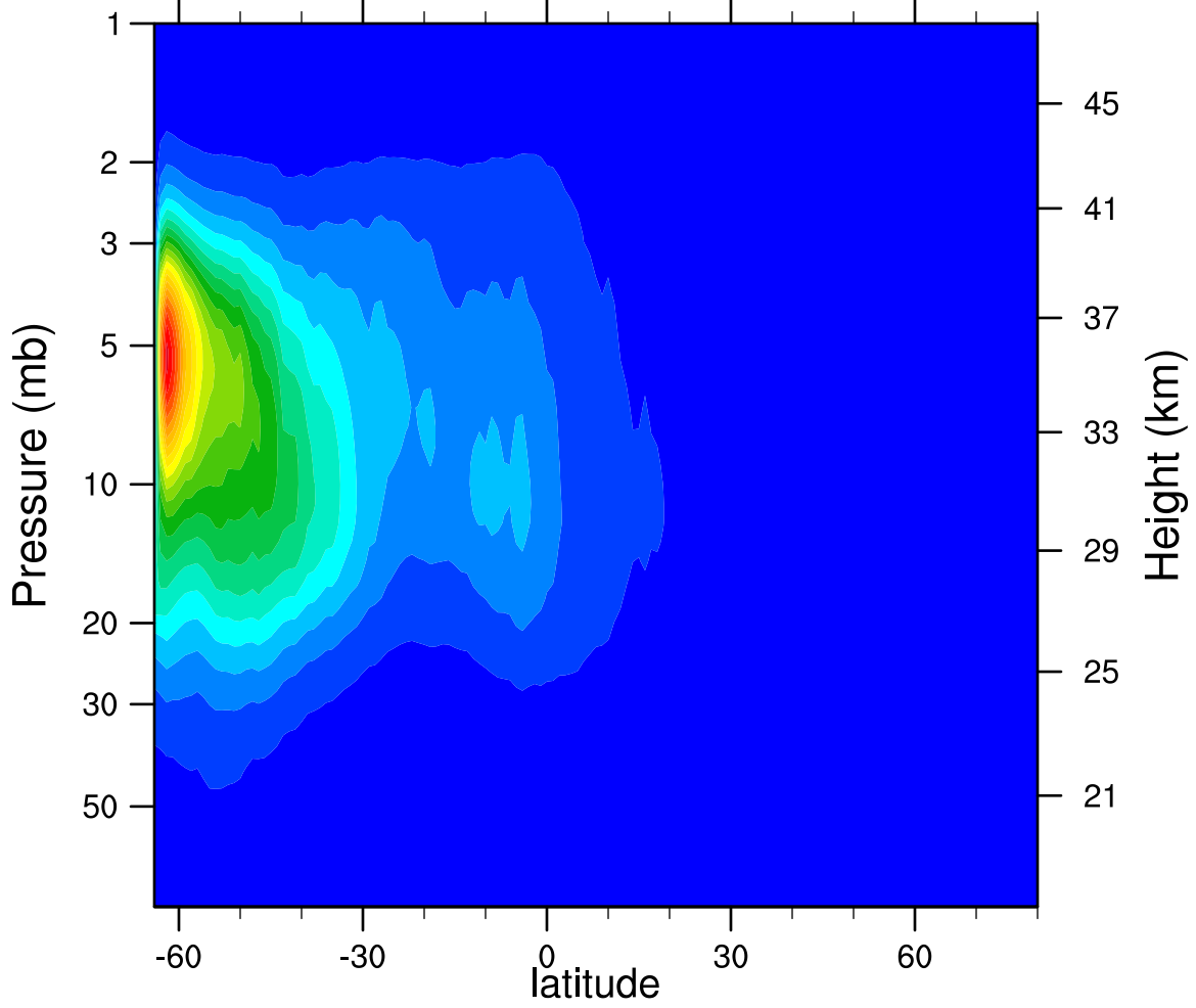
2006d162 N2O5_Ascending (ppbv)
