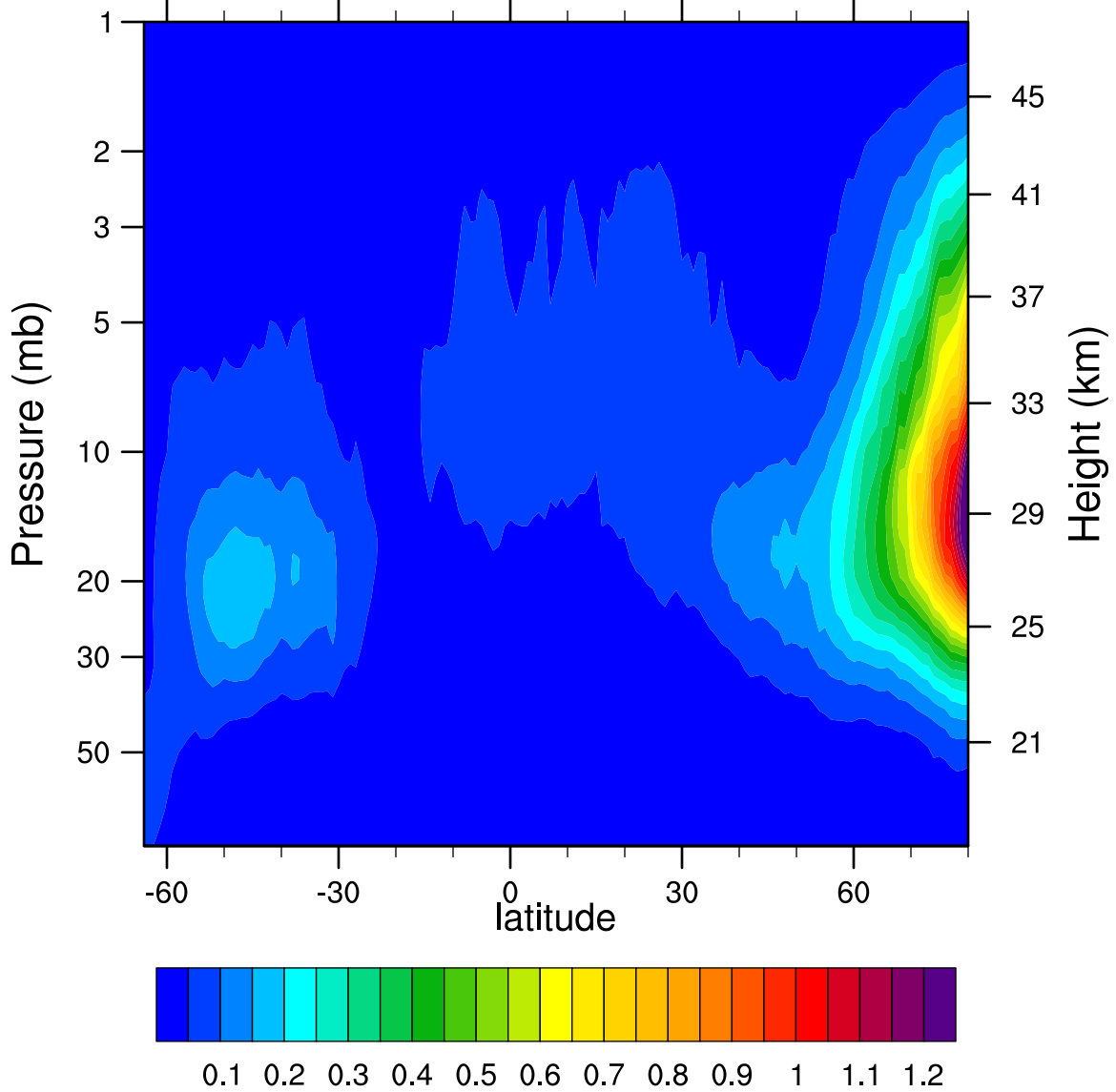
2007d297 N2O5_Ascending (ppbv)
