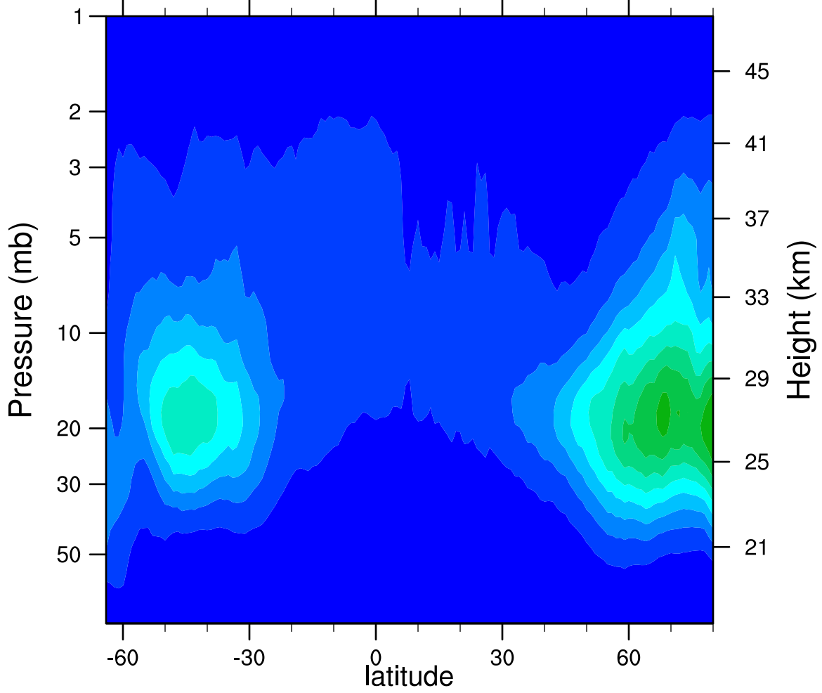
2007d273 N2O5_Ascending (ppbv)
