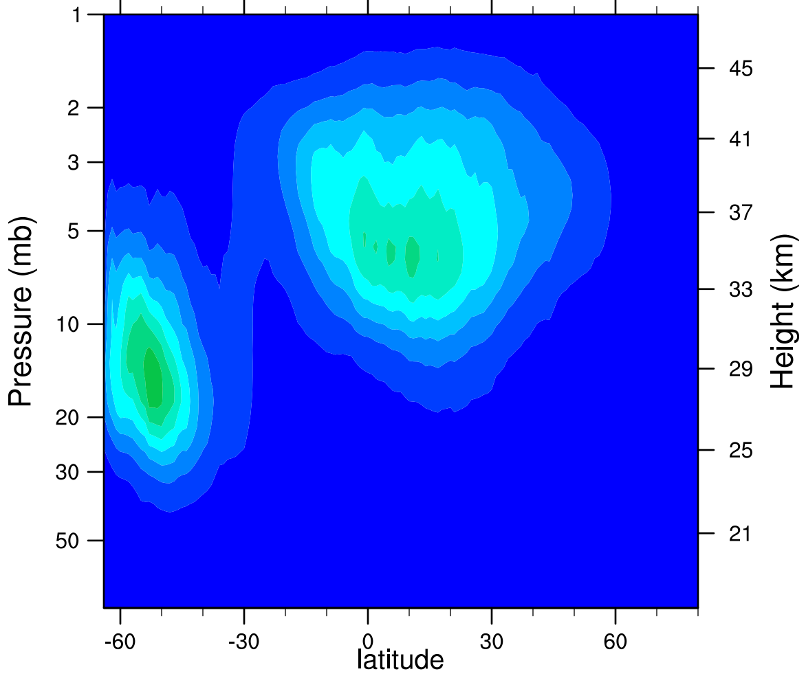
2005d216 N2O5_Ascending (ppbv)
