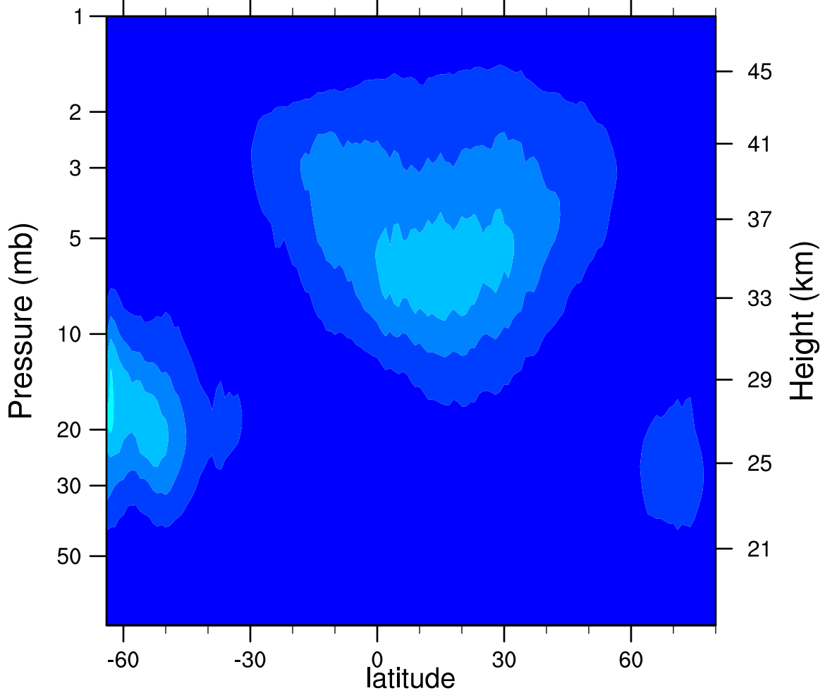
2005d252 N2O5_Ascending (ppbv)
