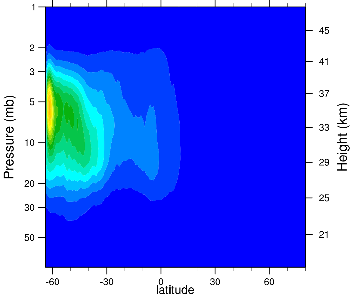
2006d171 N2O5_Ascending (ppbv)
