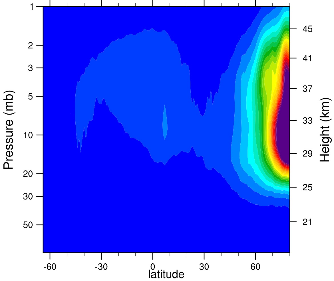
2006d037 N2O5_Ascending (ppbv)
