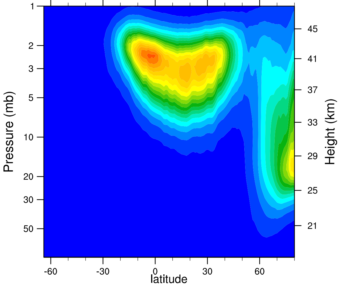
2005d041 N2O5_Ascending (ppbv)
