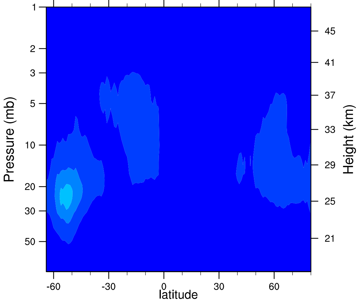
2006d264 N2O5_Ascending (ppbv)
