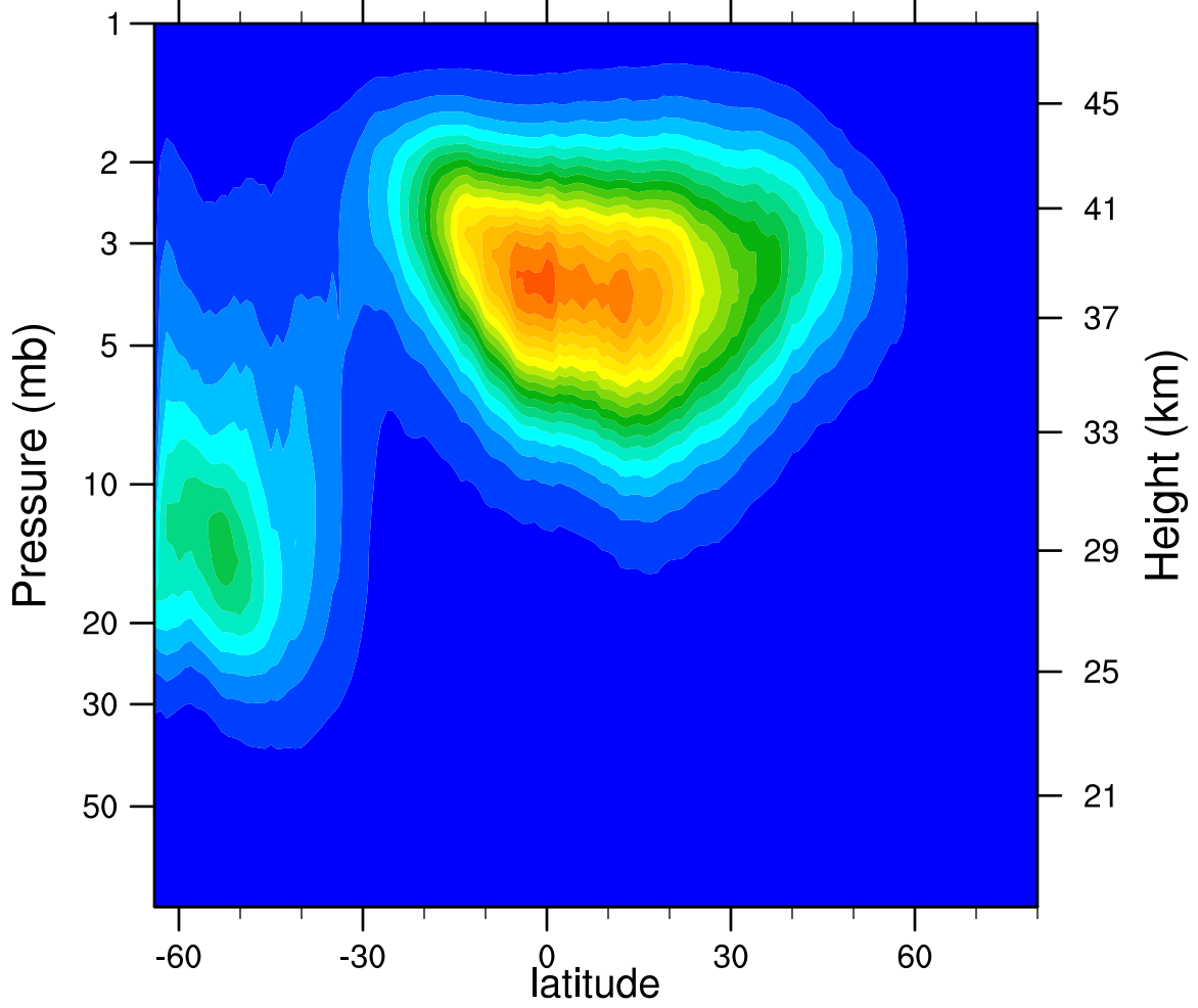
2005d131 N2O5_Ascending (ppbv)
