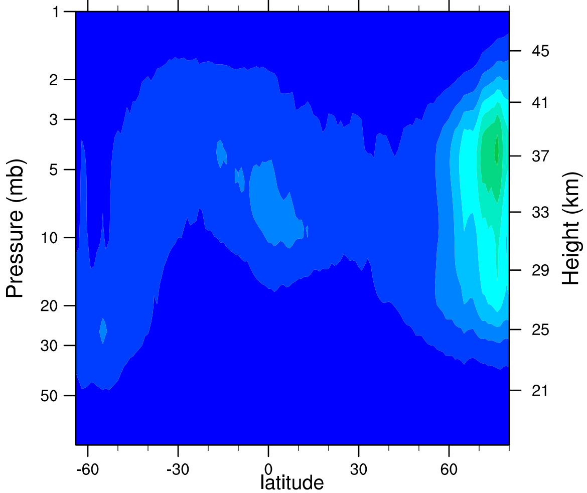
2006d067 N2O5_Ascending (ppbv)
