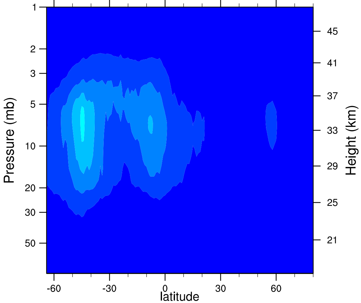
2006d212 N2O5_Ascending (ppbv)
