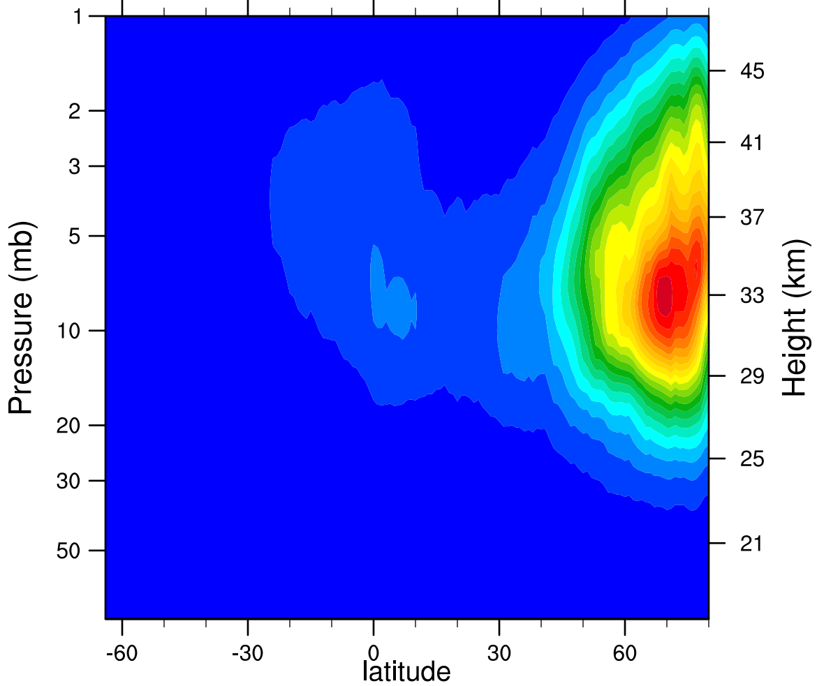
2005d358 N2O5_Ascending (ppbv)
