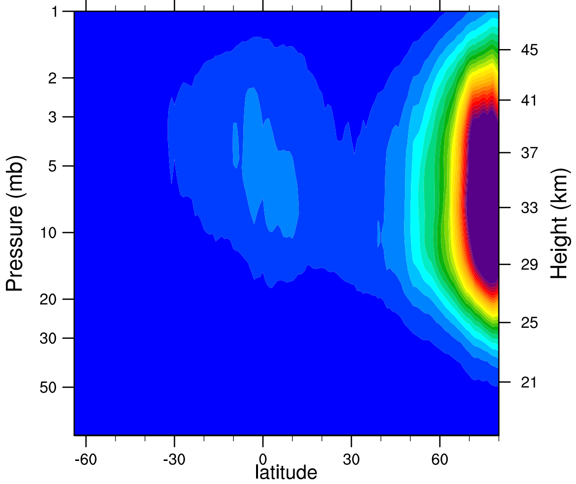
2006d021 N2O5_Ascending (ppbv)
