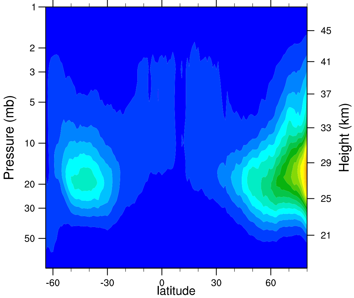
2007d280 N2O5_Ascending (ppbv)
