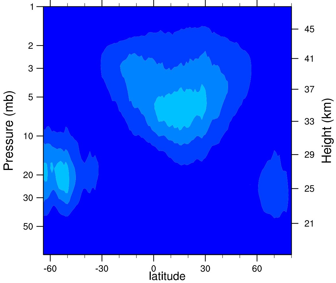
2005d254 N2O5_Ascending (ppbv)
