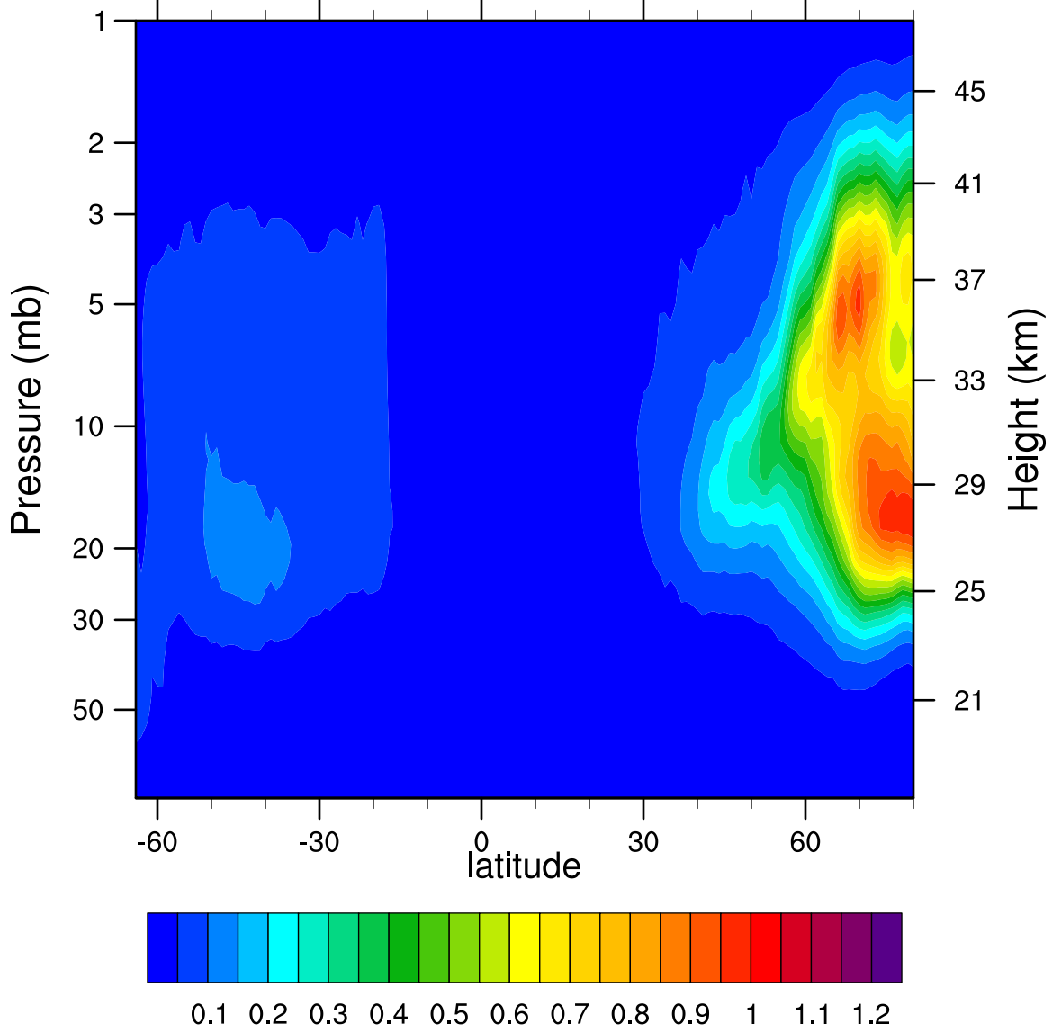
2006d313 N2O5_Ascending (ppbv)
