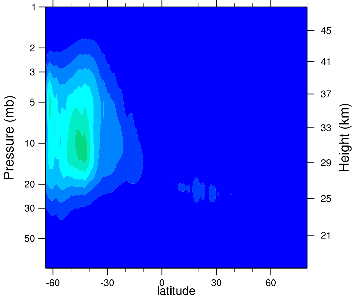
2007d170 N2O5_Ascending (ppbv)
