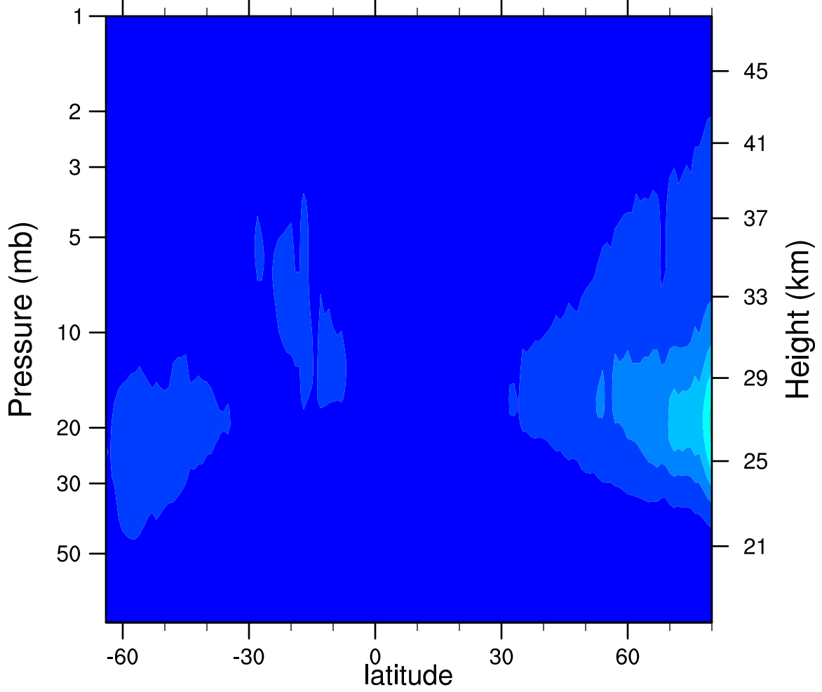
2006d275 N2O5_Ascending (ppbv)
