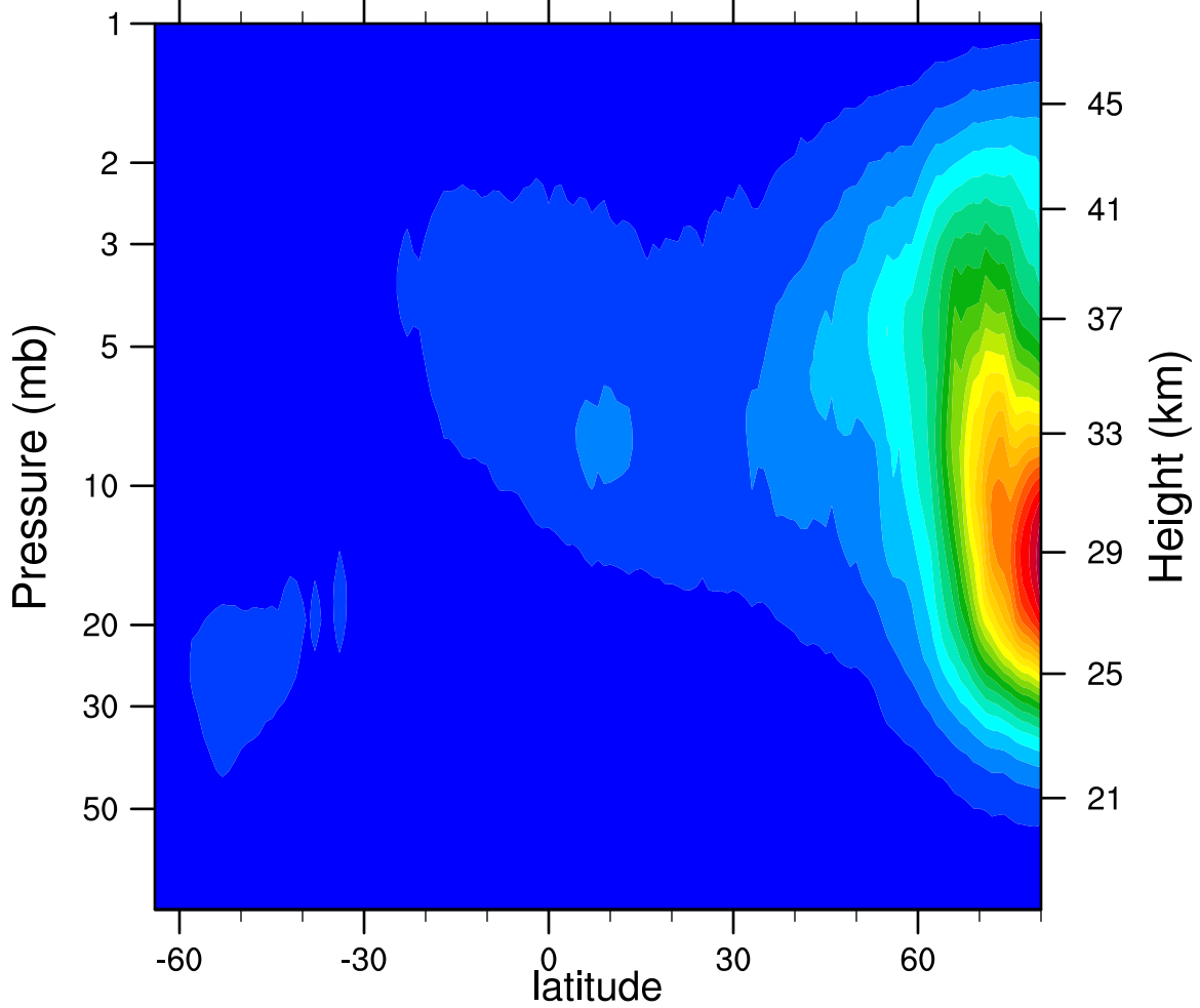
2005d302 N2O5_Ascending (ppbv)
