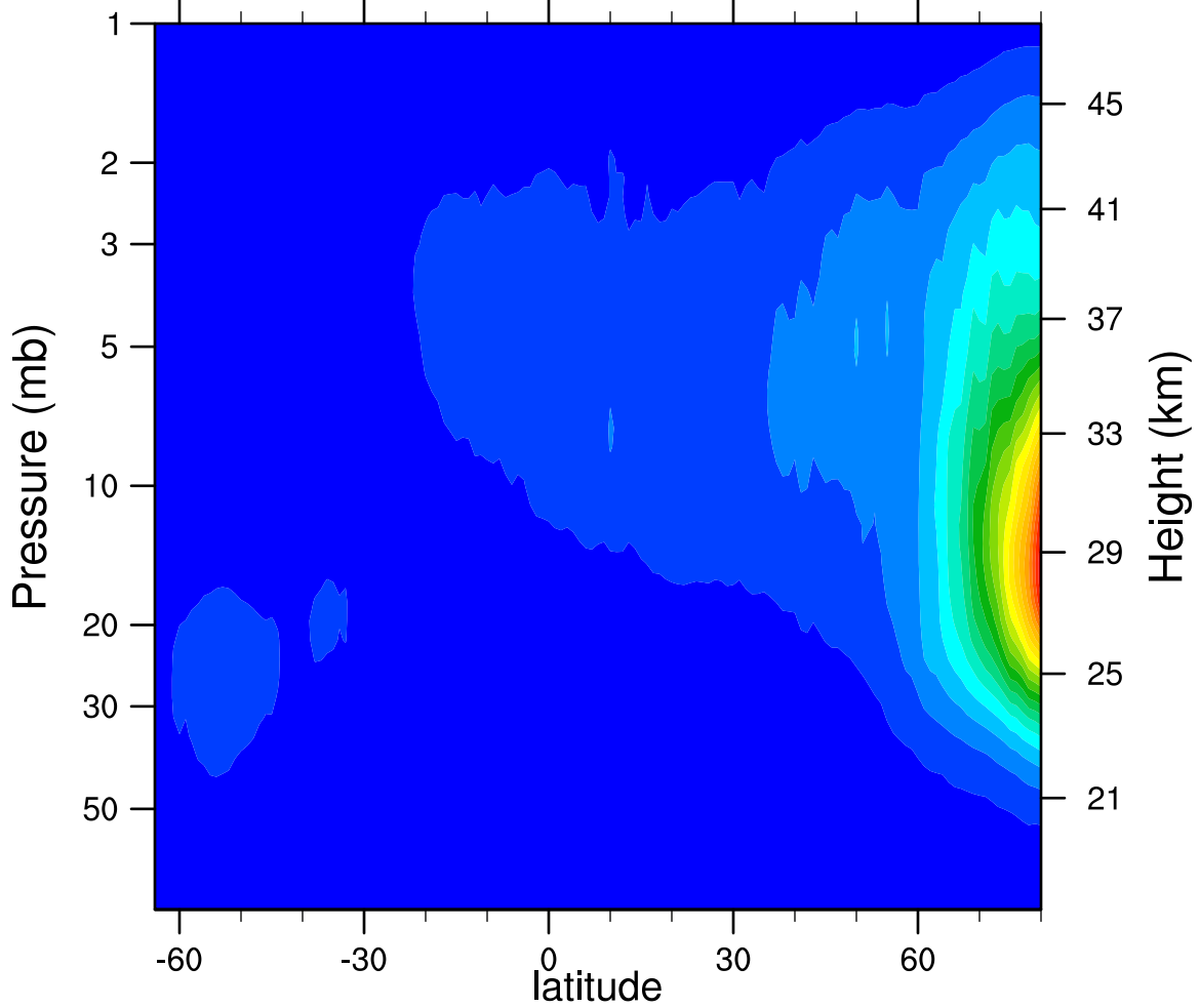
2005d297 N2O5_Ascending (ppbv)
