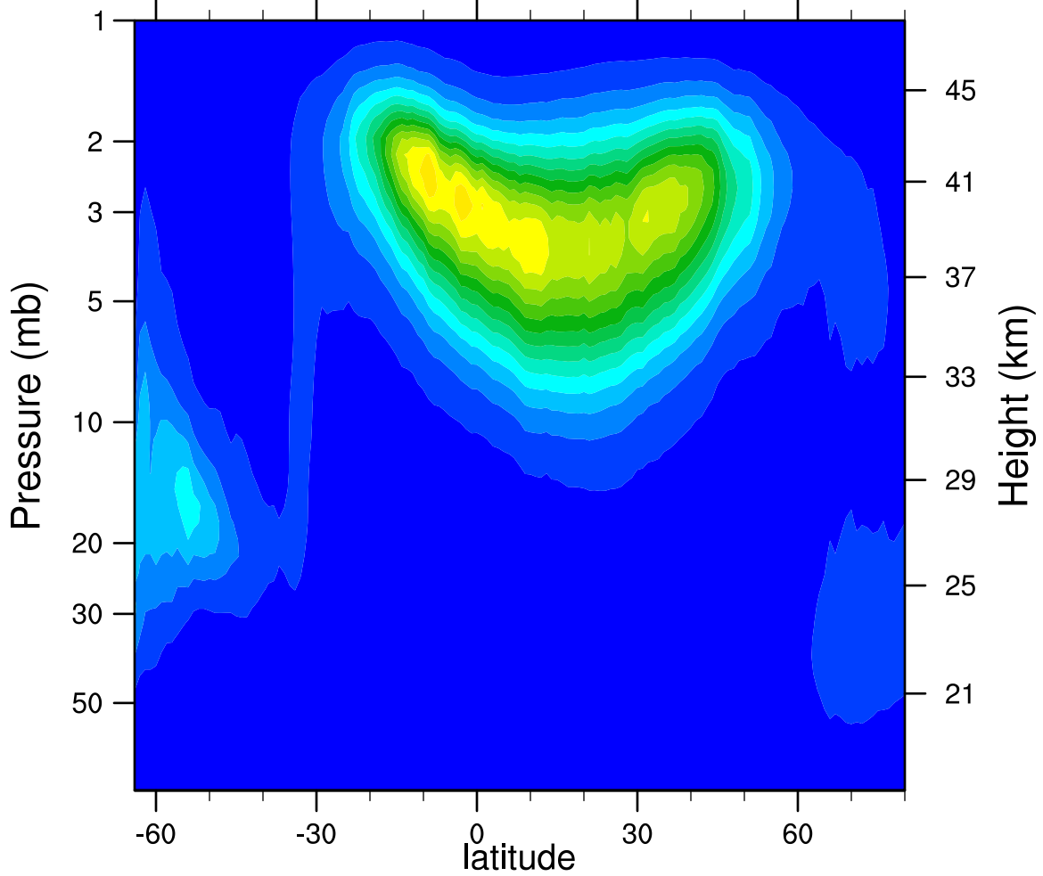
2005d088 N2O5_Ascending (ppbv)
