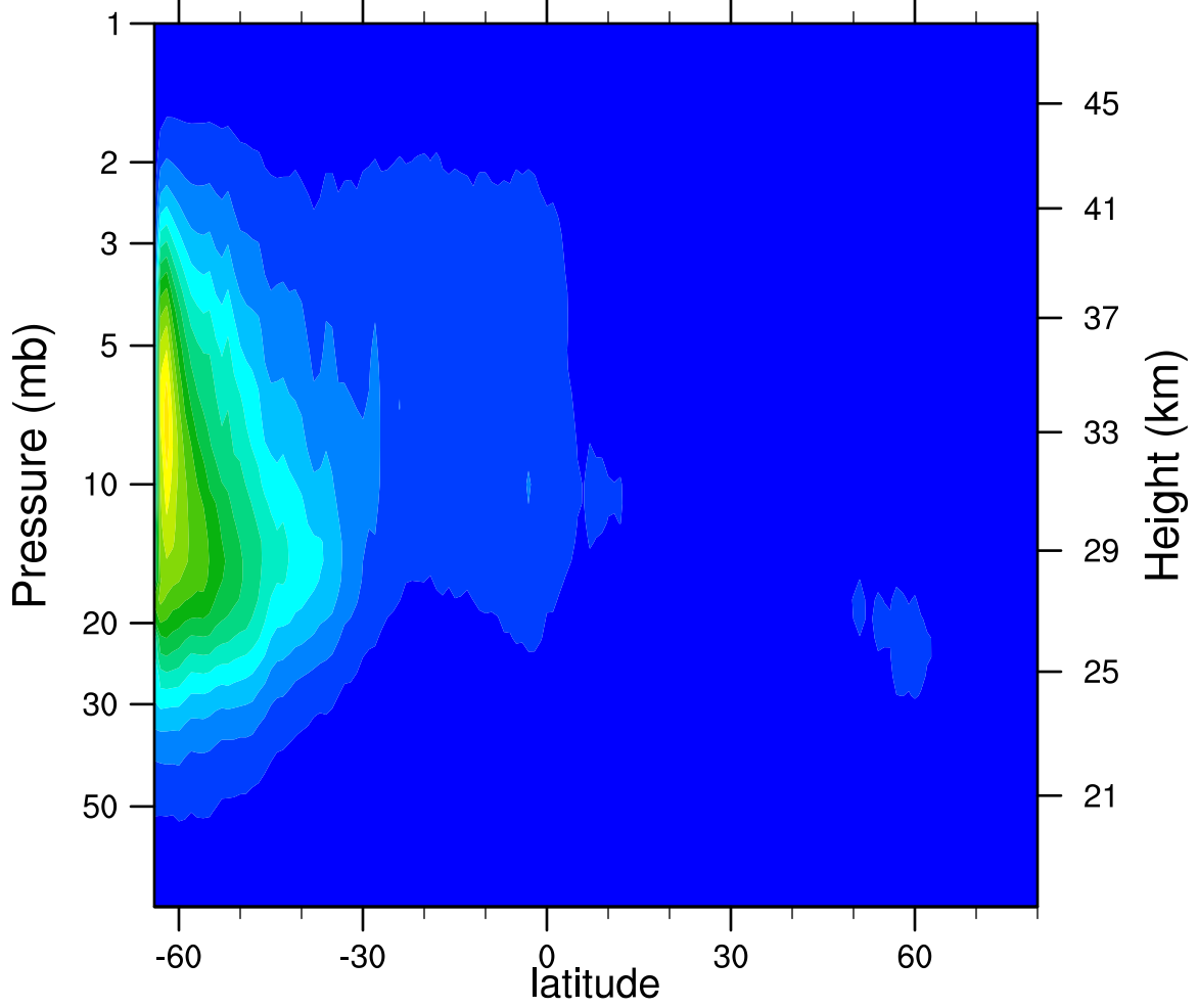
2006d124 N2O5_Ascending (ppbv)
