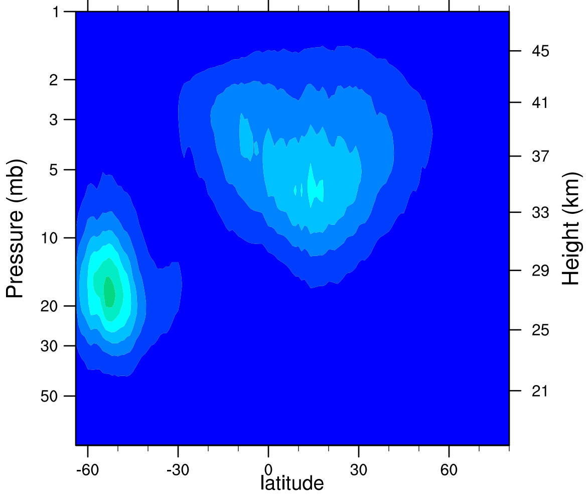
2005d232 N2O5_Ascending (ppbv)
