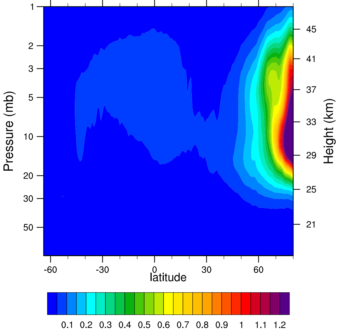
2006d040 N2O5_Ascending (ppbv)
