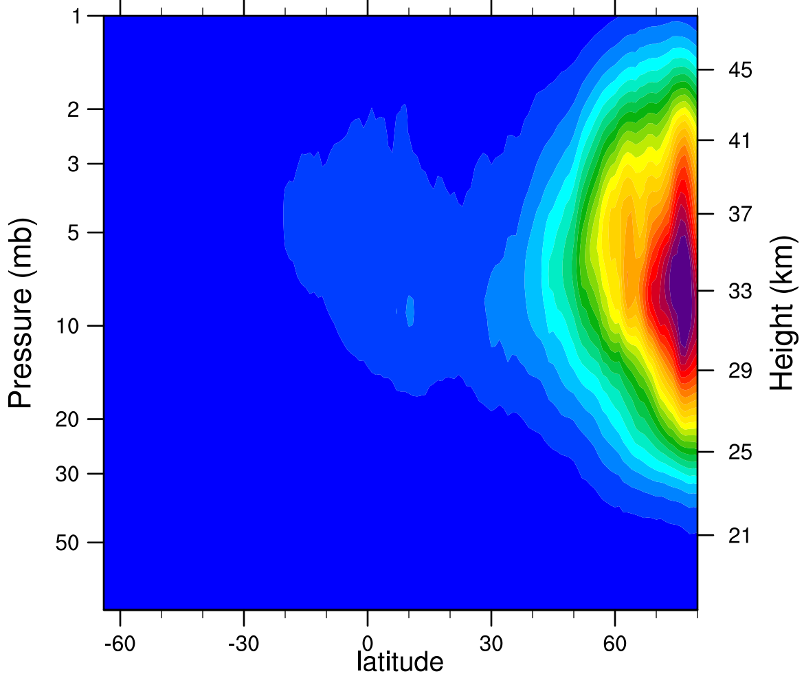
2005d333 N2O5_Ascending (ppbv)
