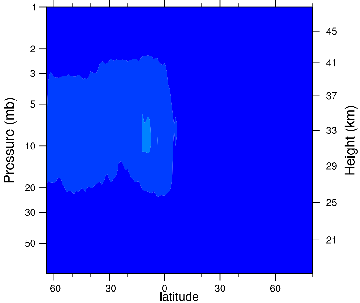
2006d183 N2O5_Ascending (ppbv)
