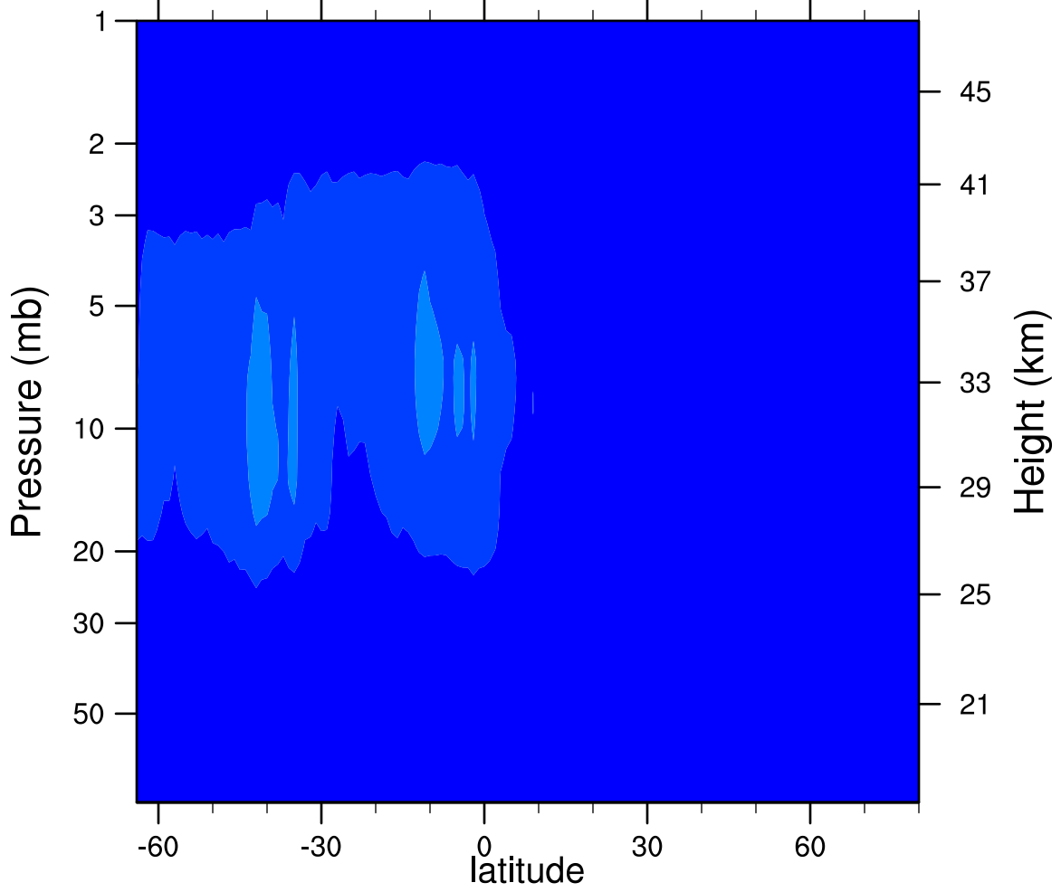
2006d188 N2O5_Ascending (ppbv)
