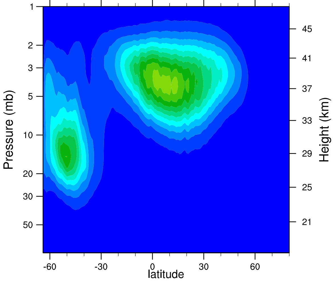
2005d153 N2O5_Ascending (ppbv)
