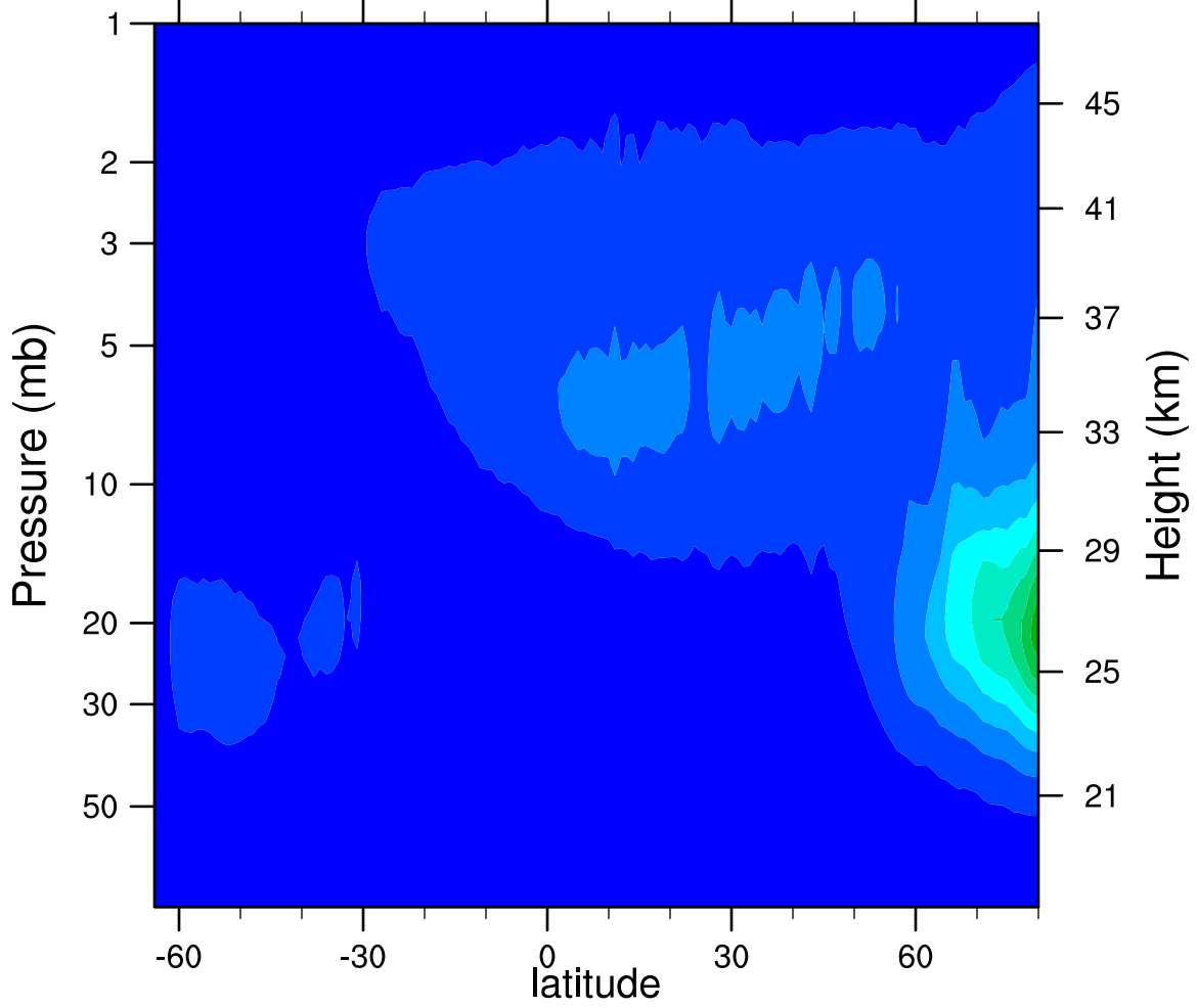
2005d283 N2O5_Ascending (ppbv)
