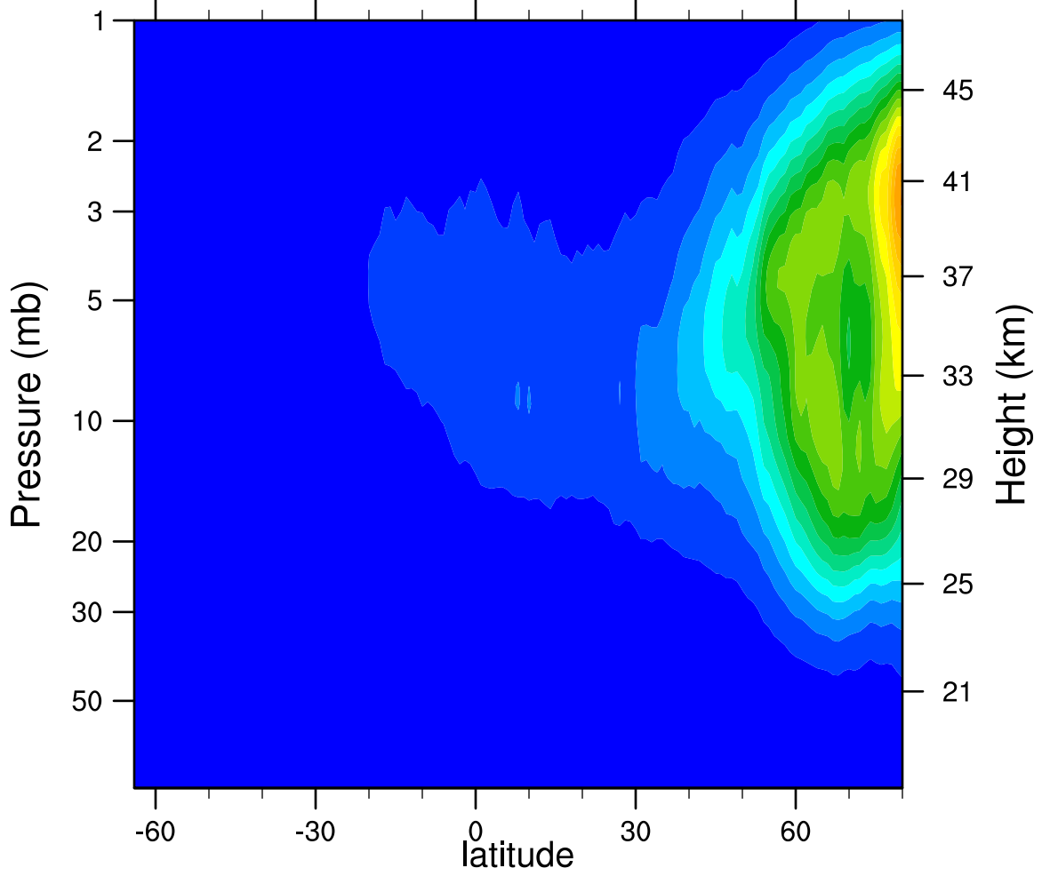
2005d321 N2O5_Ascending (ppbv)
