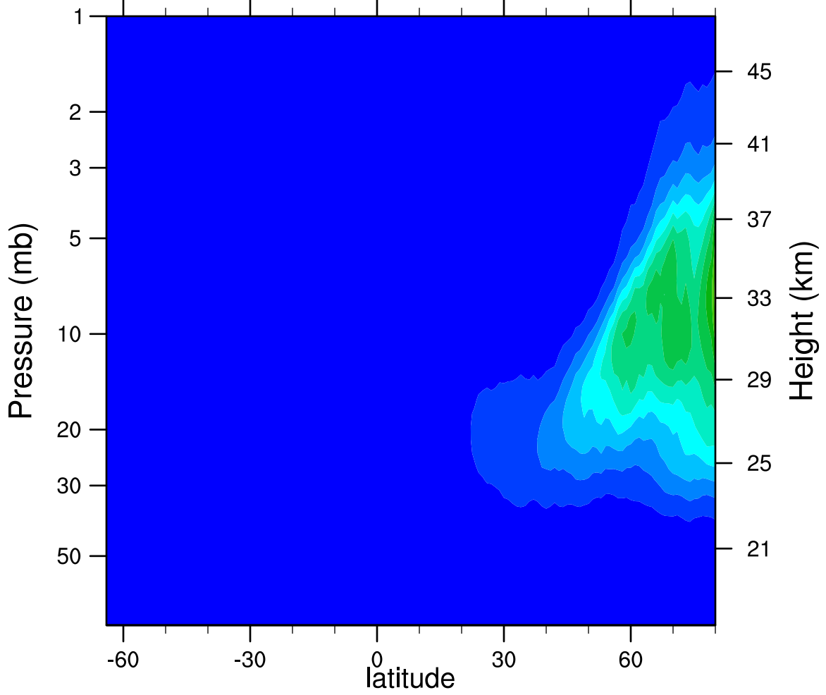
2007d050 N2O5_Ascending (ppbv)
