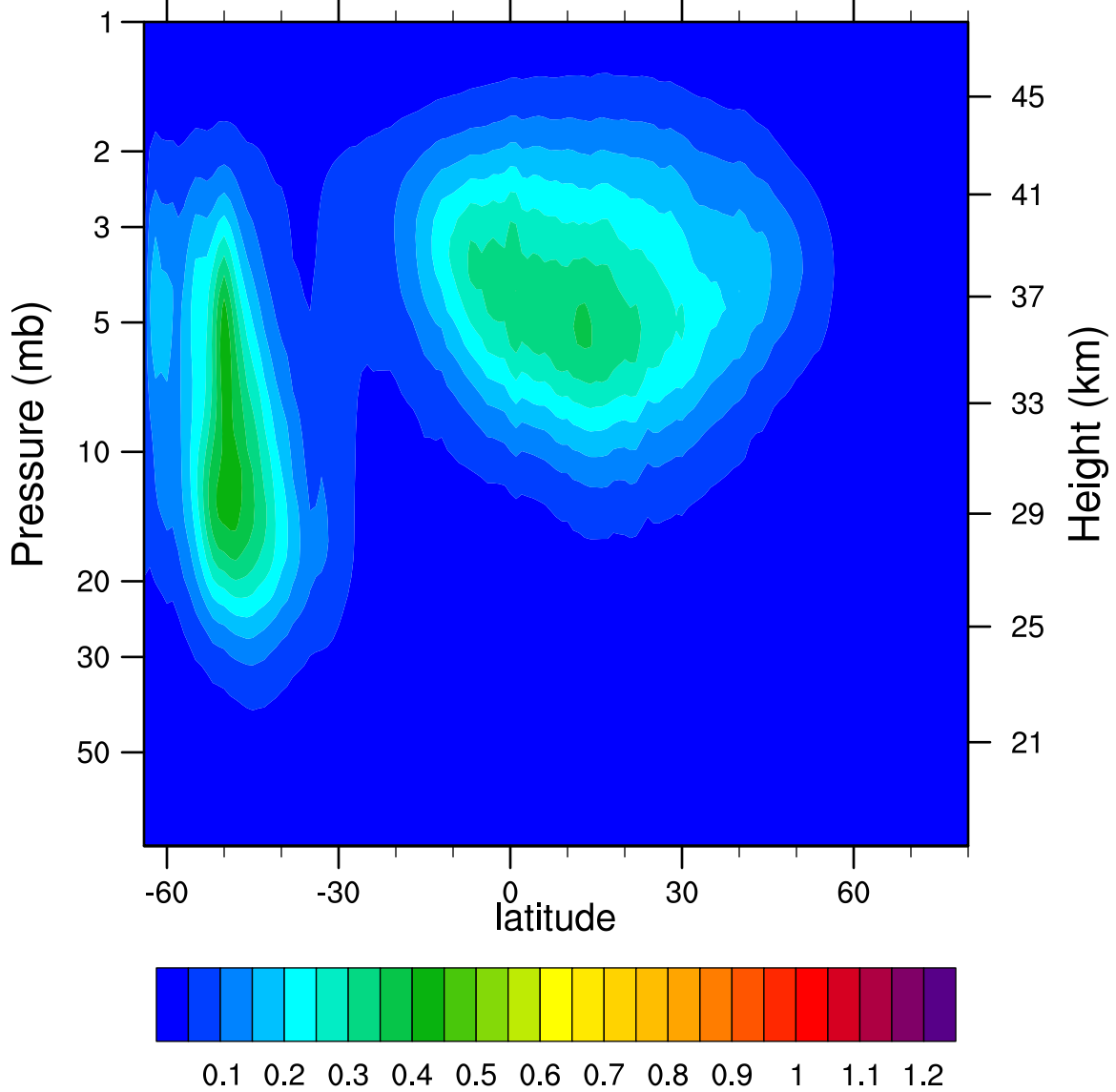
2005d184 N2O5_Ascending (ppbv)
