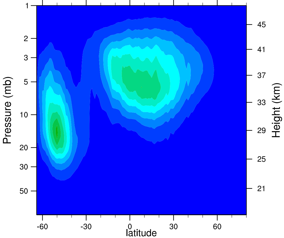
2005d204 N2O5_Ascending (ppbv)
