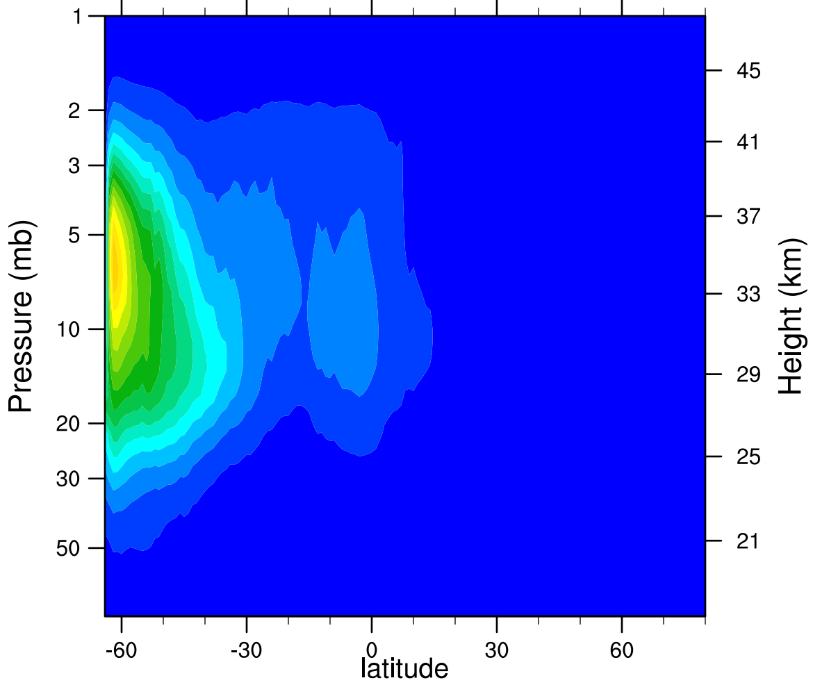
2006d142 N2O5_Ascending (ppbv)
