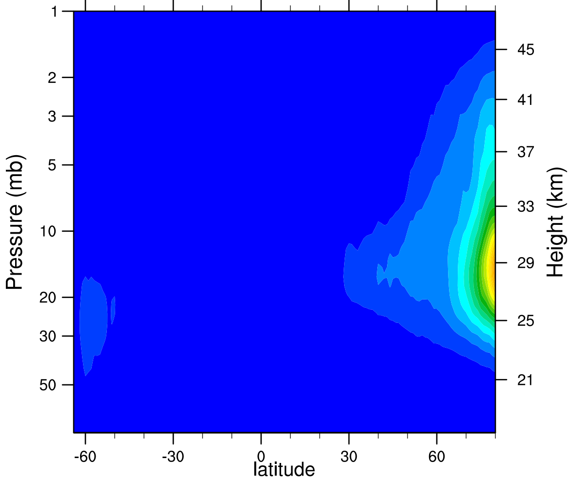
2006d289 N2O5_Ascending (ppbv)
