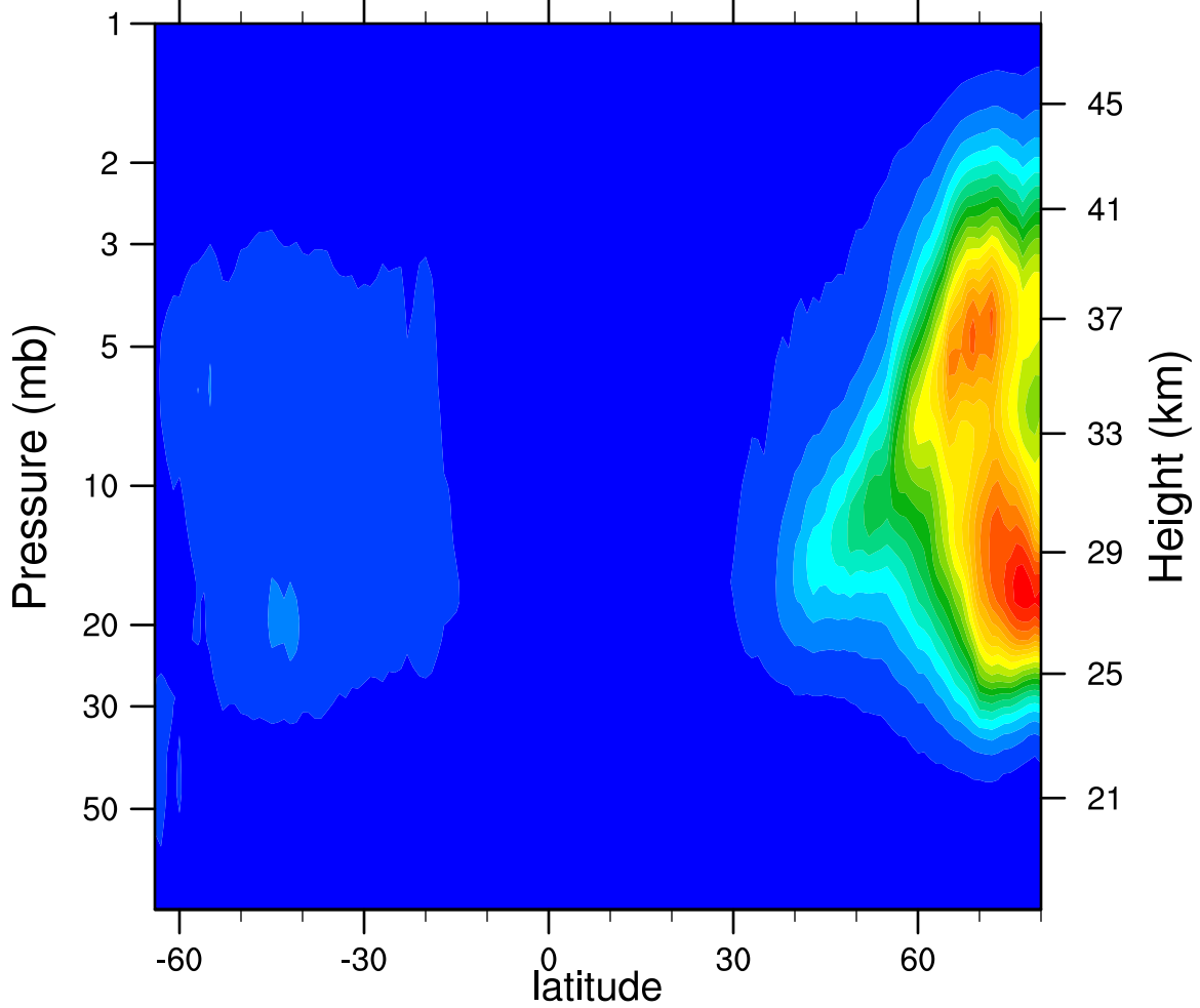
2006d311 N2O5_Ascending (ppbv)
