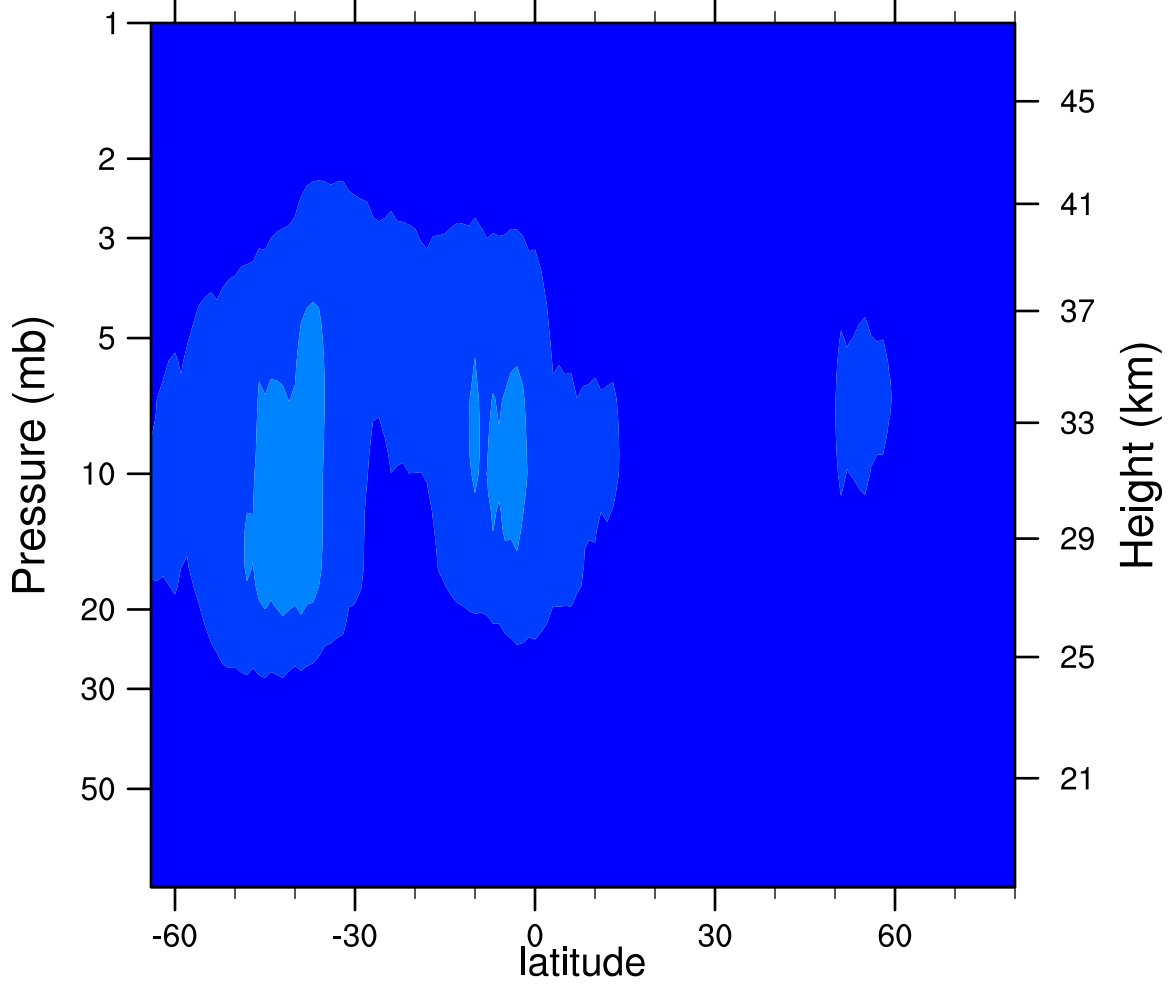
2006d220 N2O5_Ascending (ppbv)
