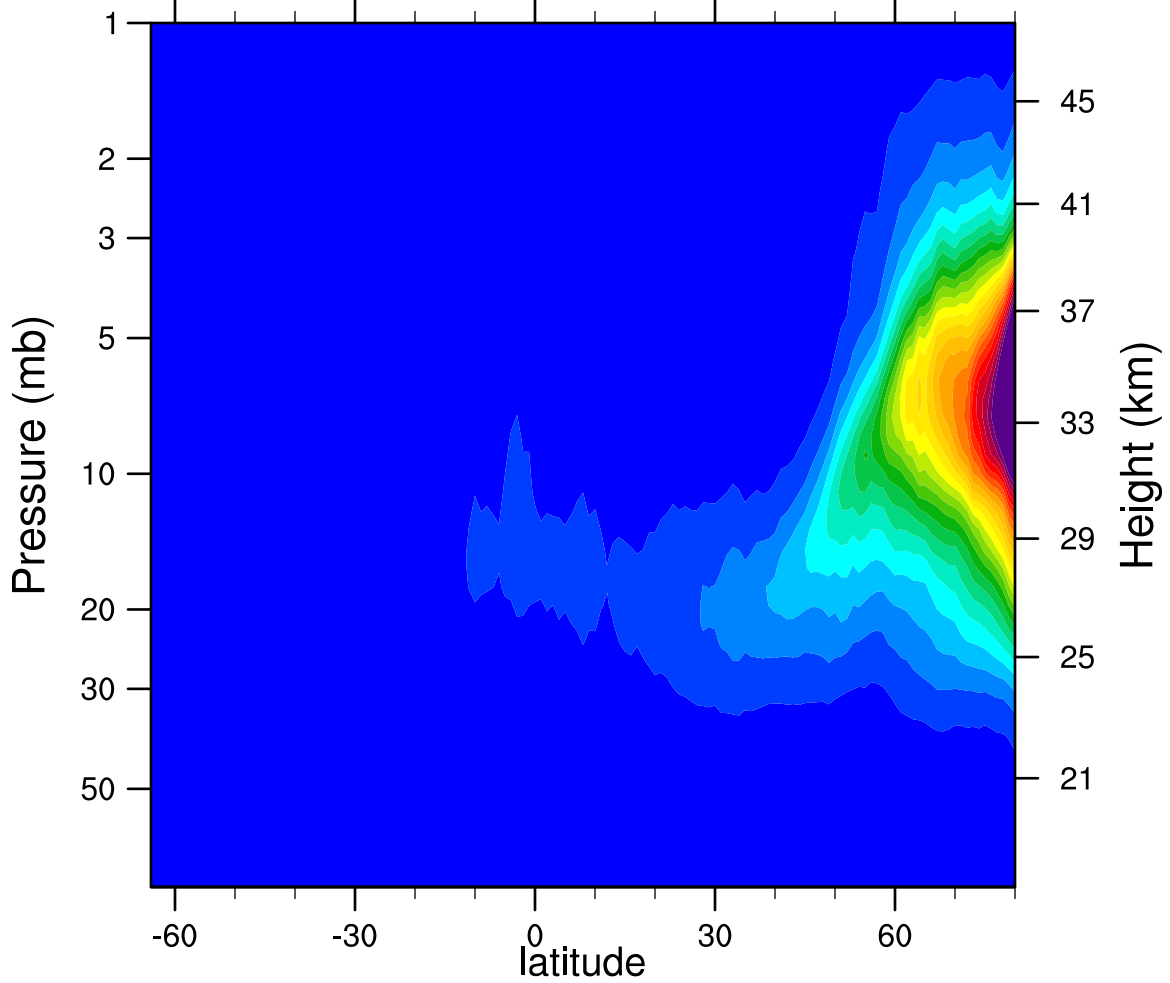
2007d036 N2O5_Ascending (ppbv)
