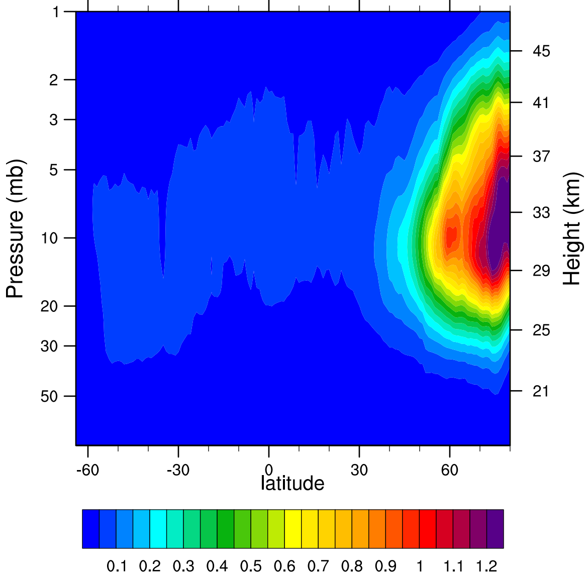
2007d356 N2O5_Ascending (ppbv)
