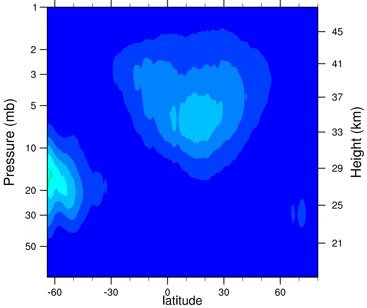
2005d248 N2O5_Ascending (ppbv)
