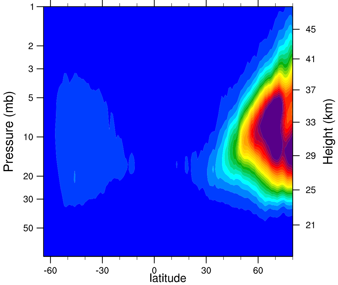
2006d355 N2O5_Ascending (ppbv)
