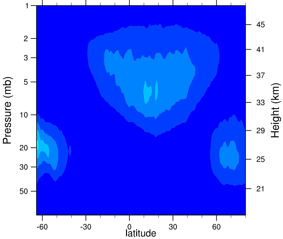
2005d267 N2O5_Ascending (ppbv)
