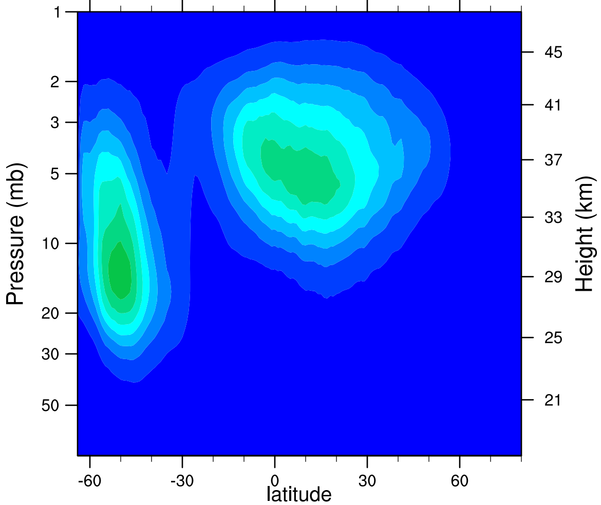
2005d194 N2O5_Ascending (ppbv)
