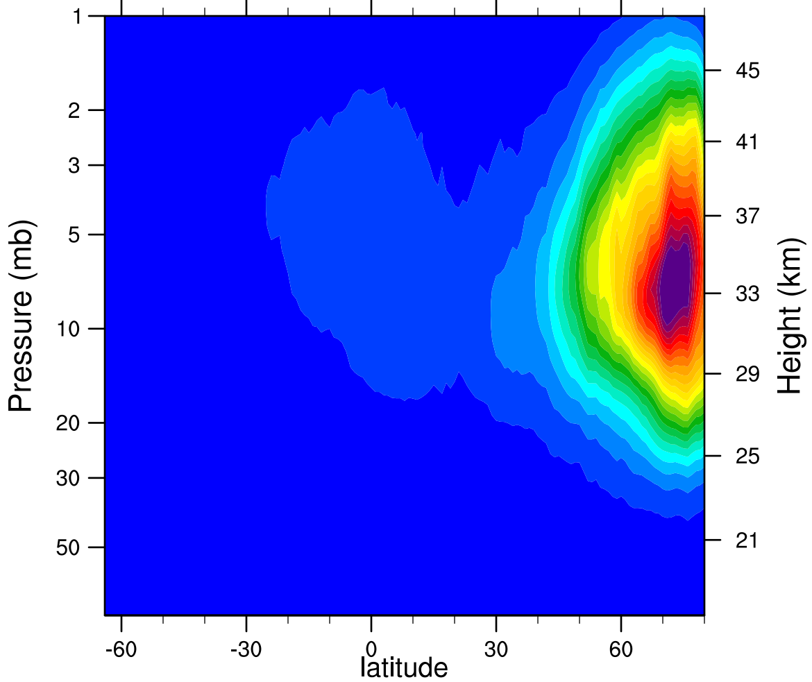
2005d347 N2O5_Ascending (ppbv)
