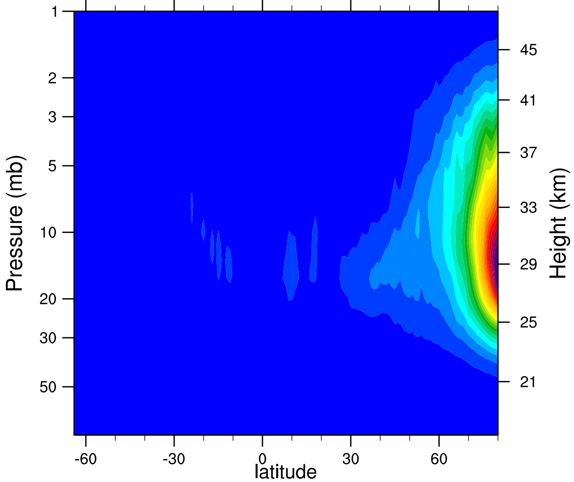
2006d296 N2O5_Ascending (ppbv)
