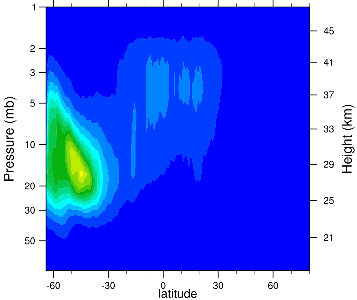
2007d215 N2O5_Ascending (ppbv)
