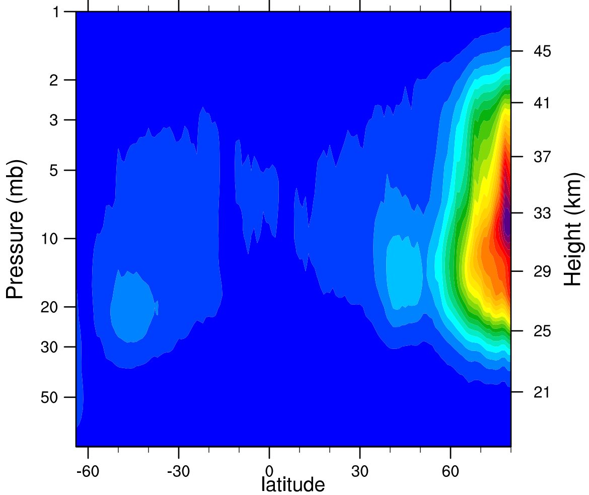
2006d319 N2O5_Ascending (ppbv)
