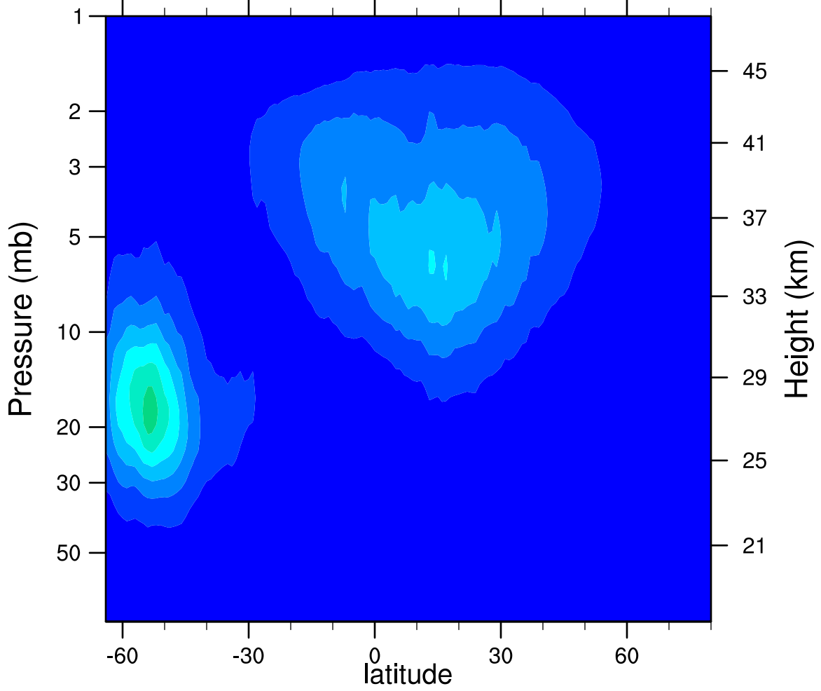
2005d234 N2O5_Ascending (ppbv)
