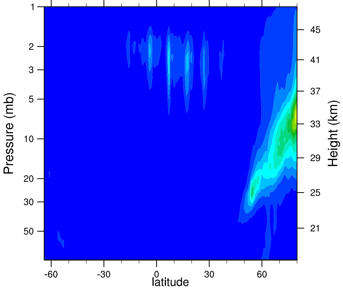
2005d022 N2O5_Ascending (ppbv)
