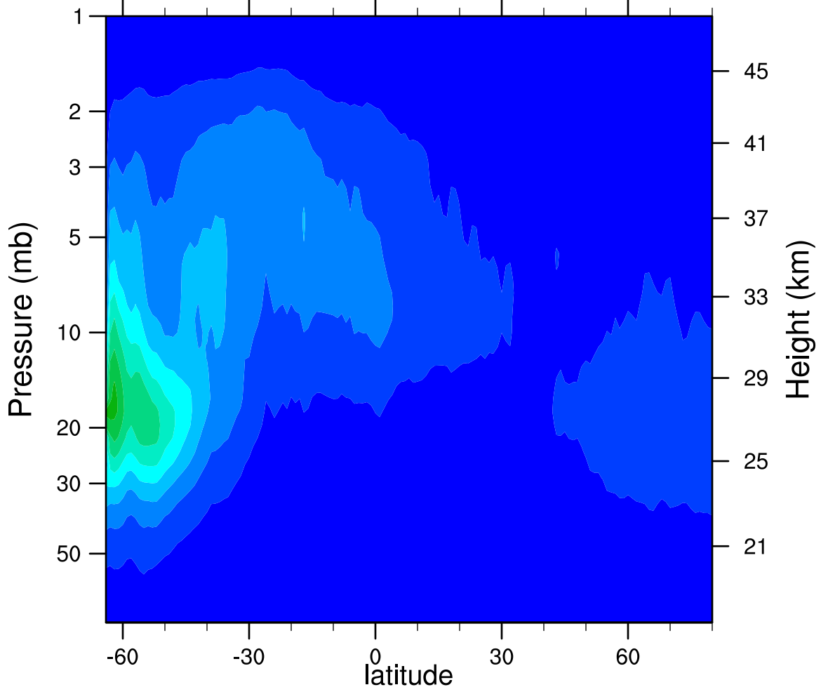
2006d100 N2O5_Ascending (ppbv)
