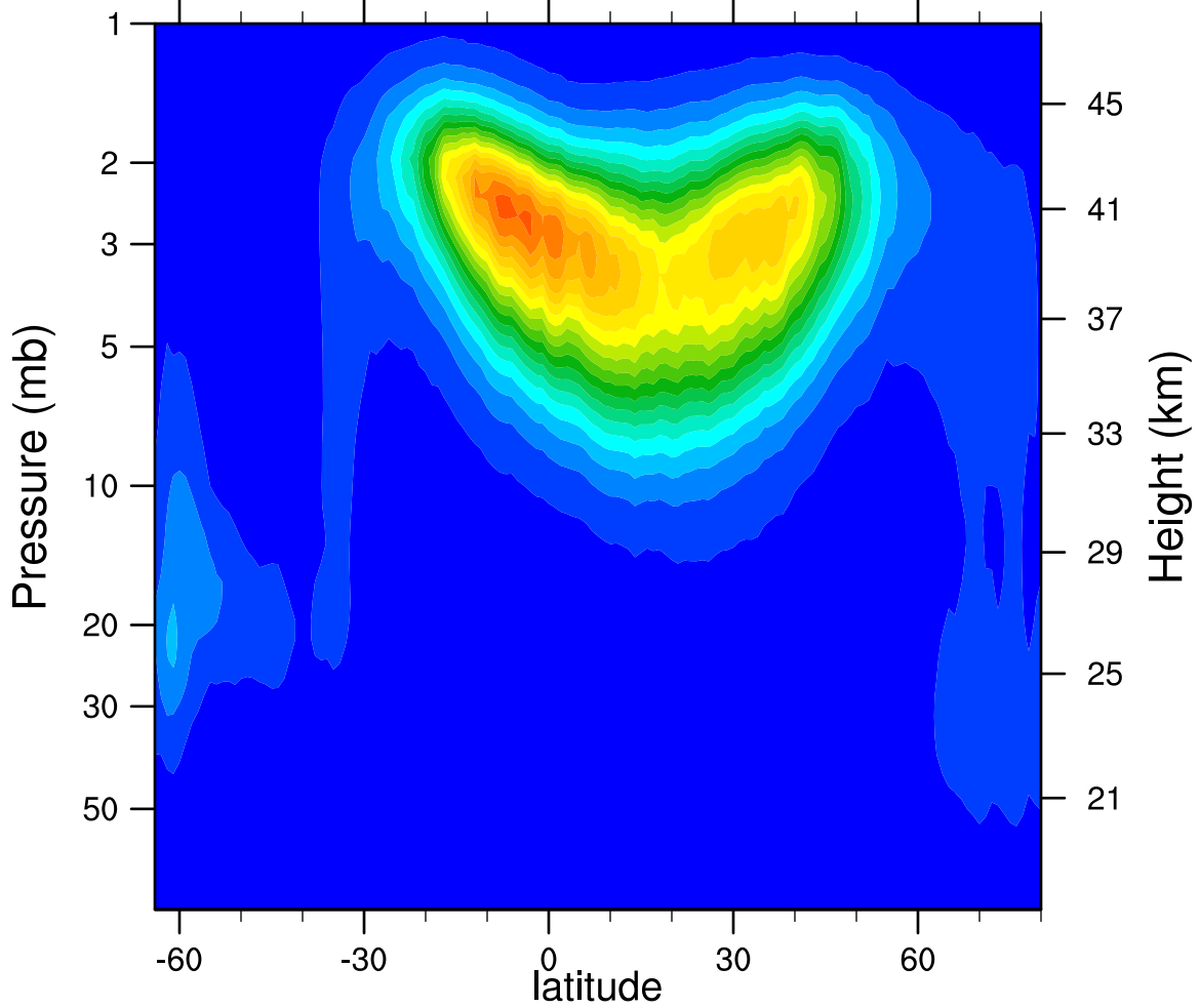
2005d077 N2O5_Ascending (ppbv)
