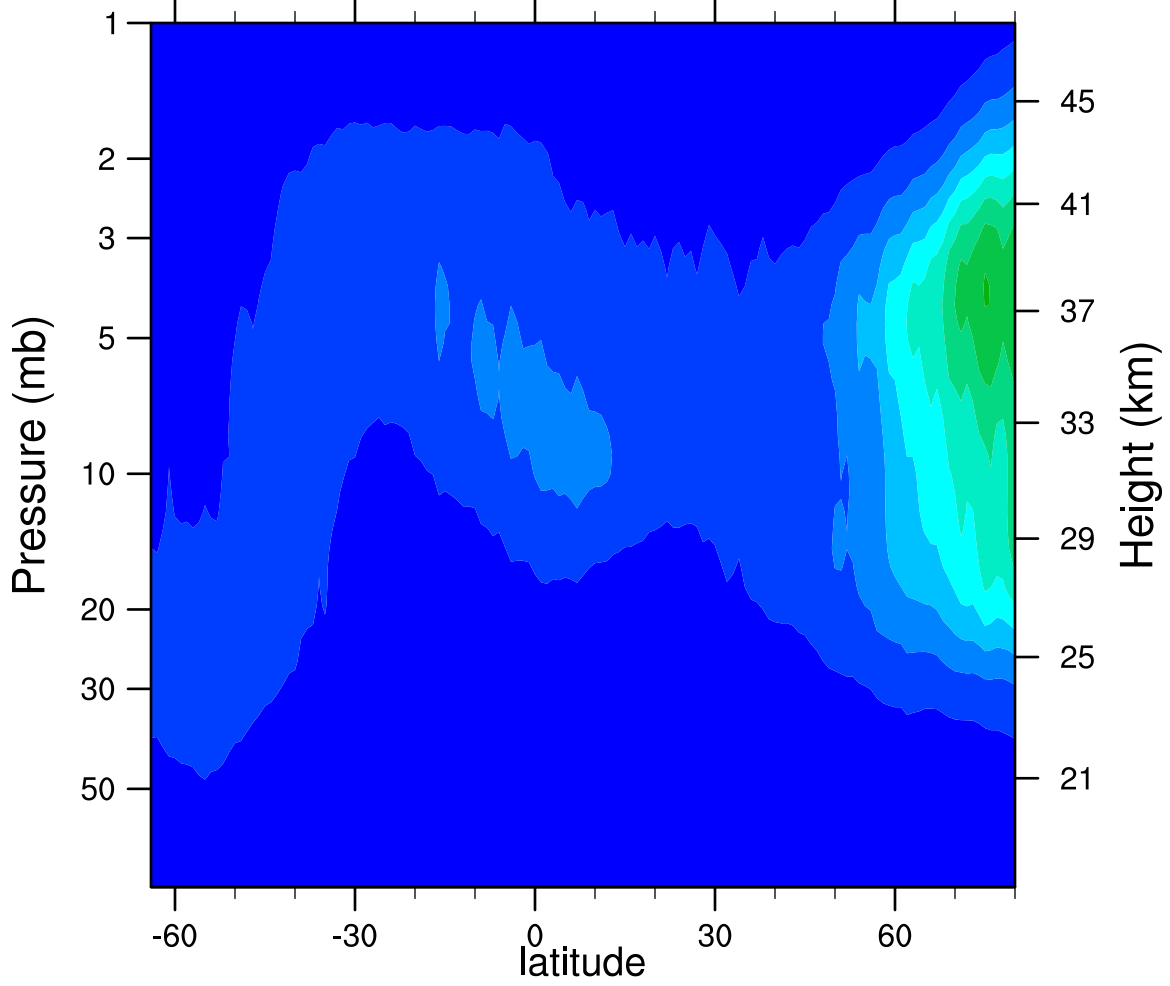
2006d063 N2O5_Ascending (ppbv)
