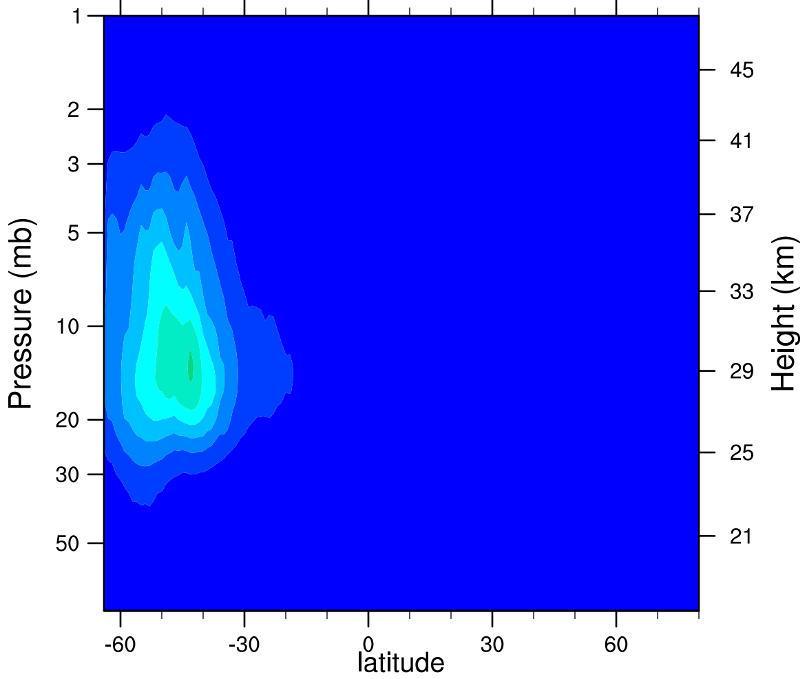
2007d205 N2O5_Ascending (ppbv)
