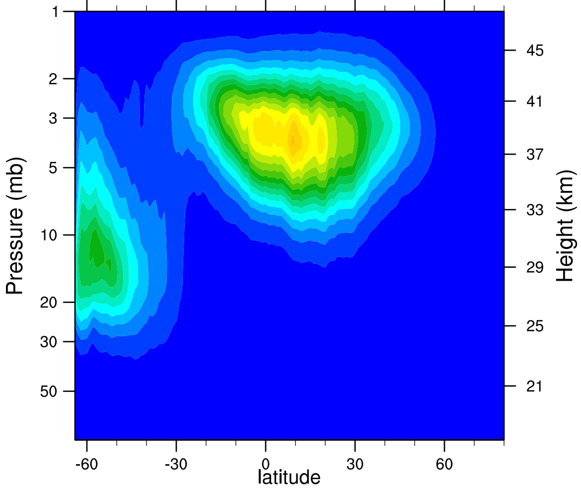
2005d143 N2O5_Ascending (ppbv)
