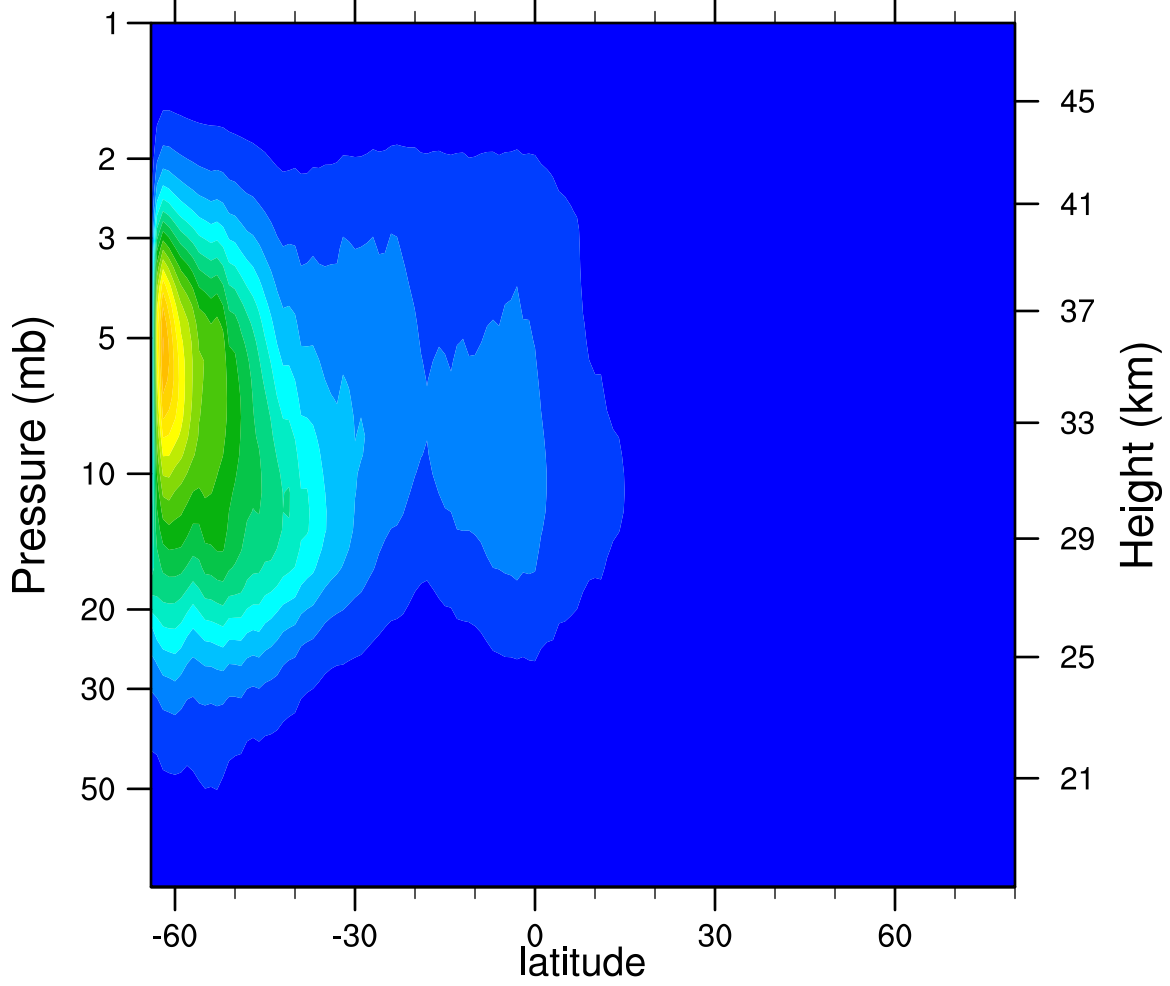
2006d146 N2O5_Ascending (ppbv)
