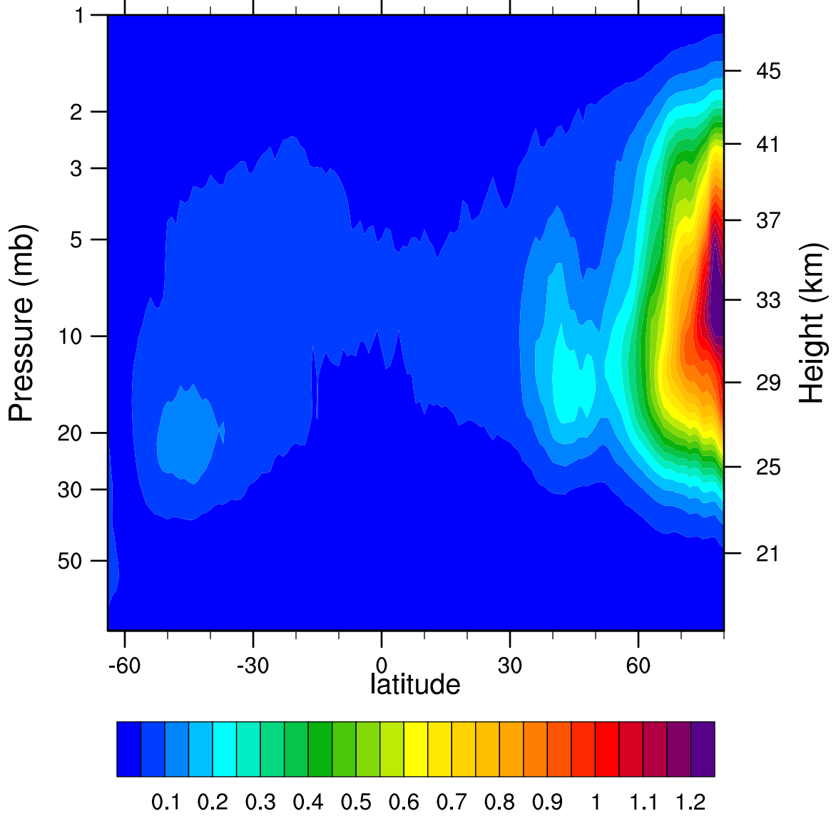
2006d321 N2O5_Ascending (ppbv)
