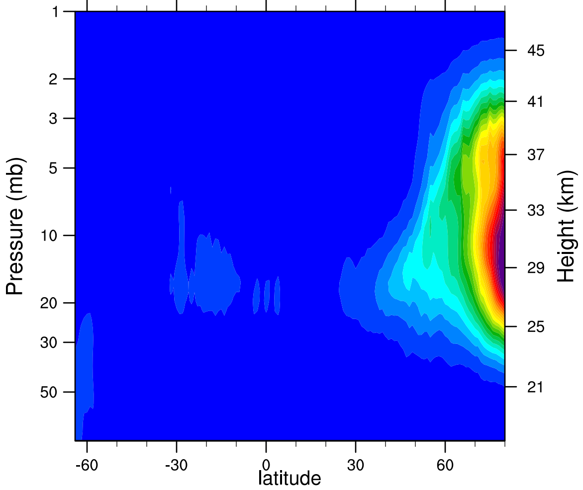
2006d301 N2O5_Ascending (ppbv)
