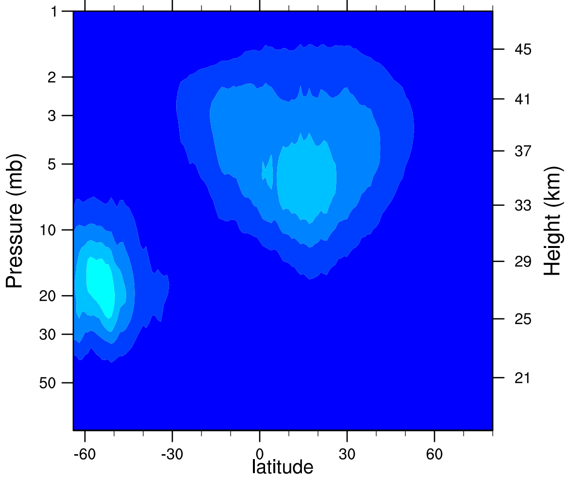
2005d240 N2O5_Ascending (ppbv)
