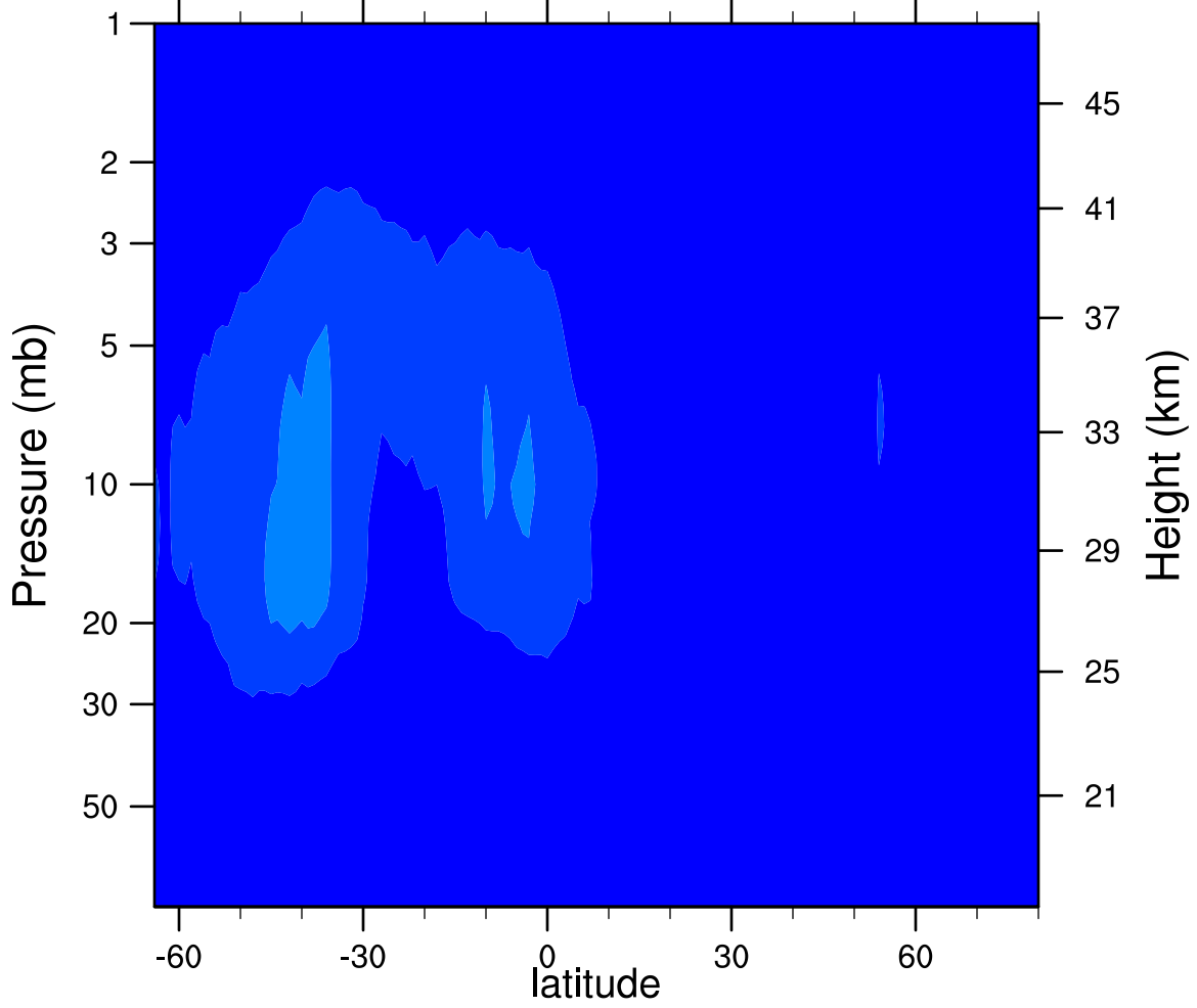
2006d223 N2O5_Ascending (ppbv)
