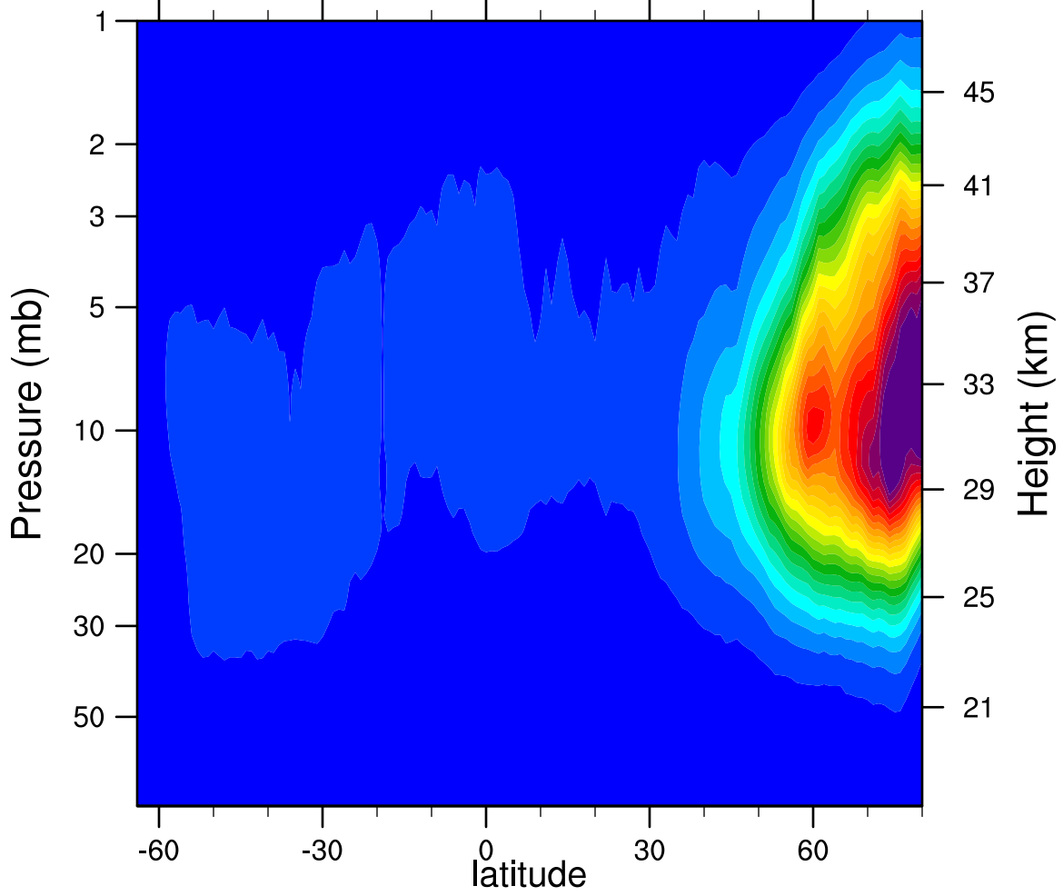
2007d357 N2O5_Ascending (ppbv)
