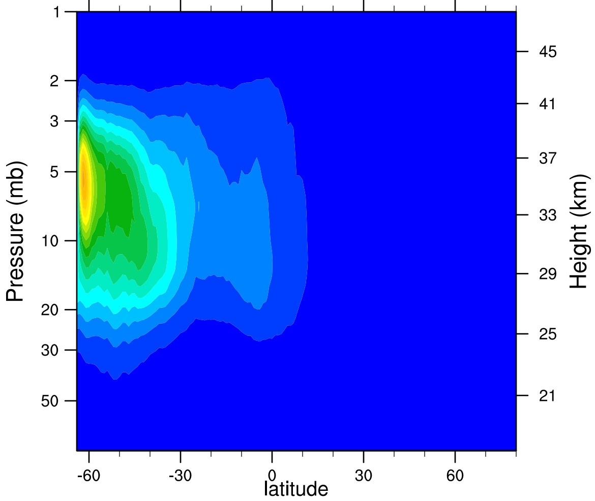
2006d169 N2O5_Ascending (ppbv)
