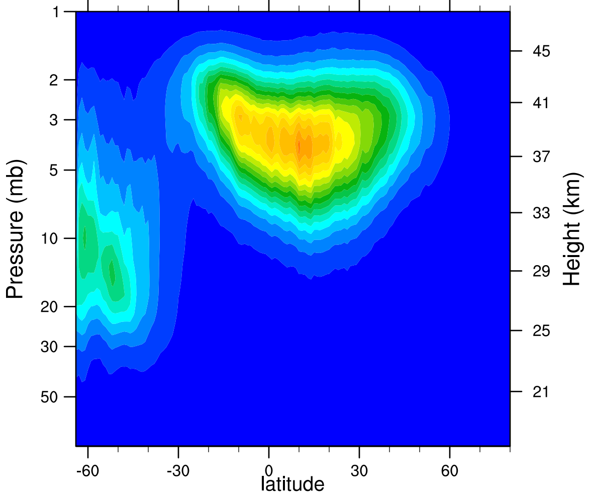
2005d119 N2O5_Ascending (ppbv)
