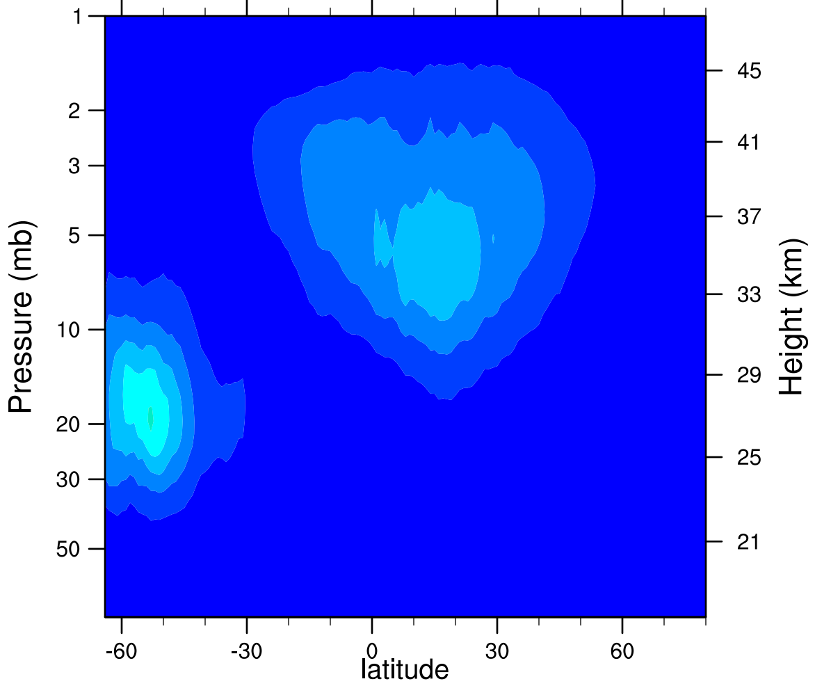
2005d238 N2O5_Ascending (ppbv)
