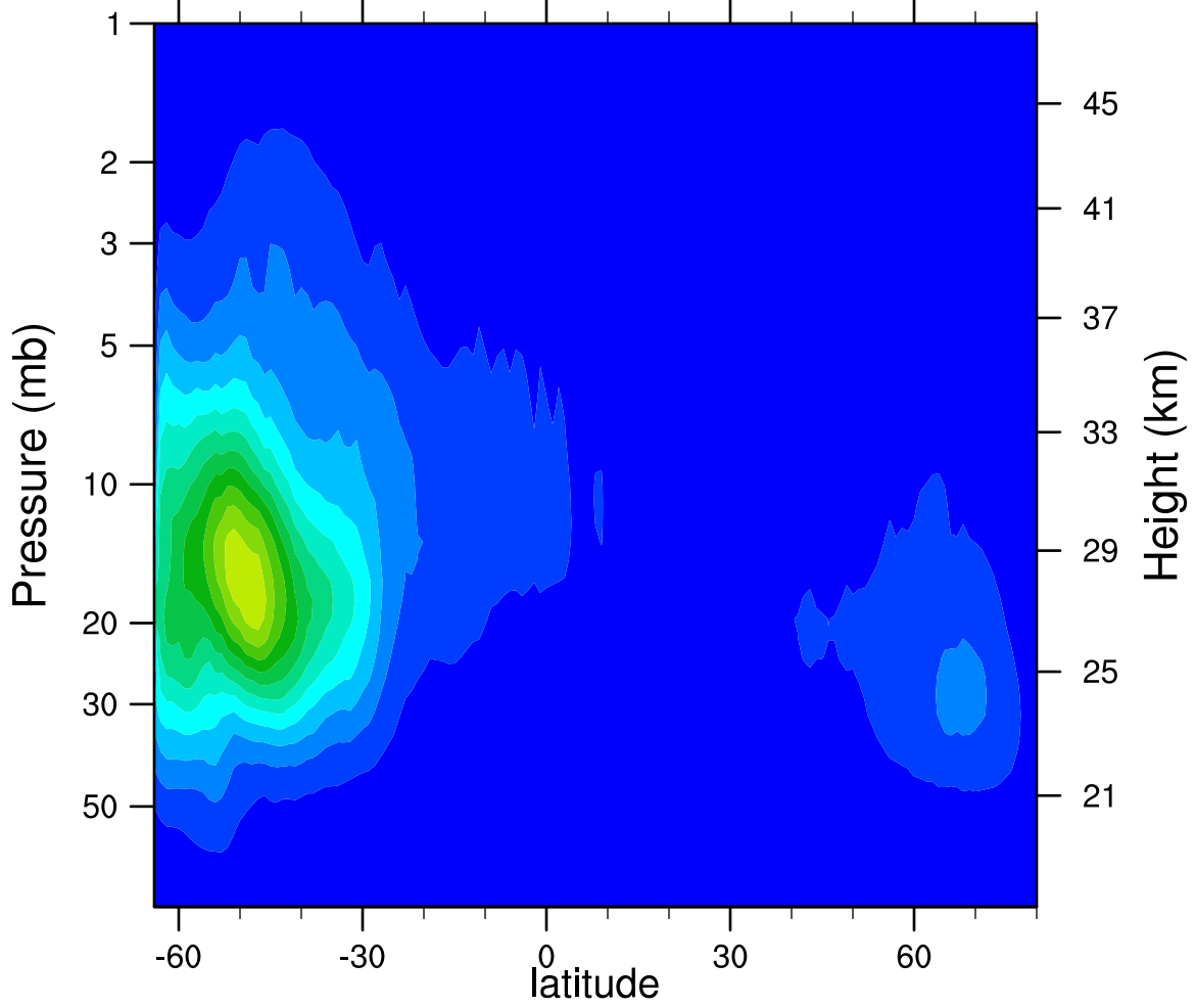
2007d239 N2O5_Ascending (ppbv)
