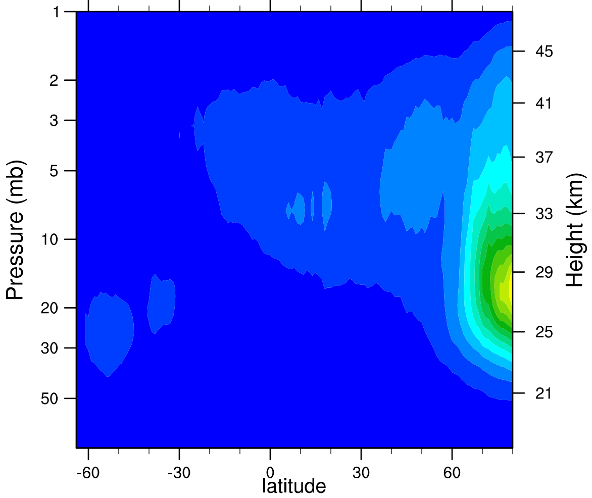
2005d292 N2O5_Ascending (ppbv)
