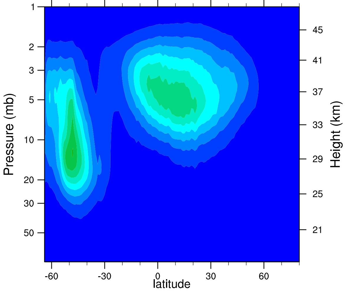
2005d187 N2O5_Ascending (ppbv)
