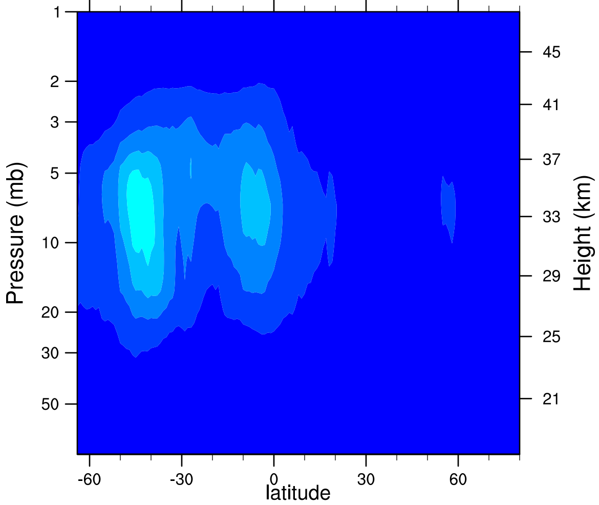
2006d205 N2O5_Ascending (ppbv)
