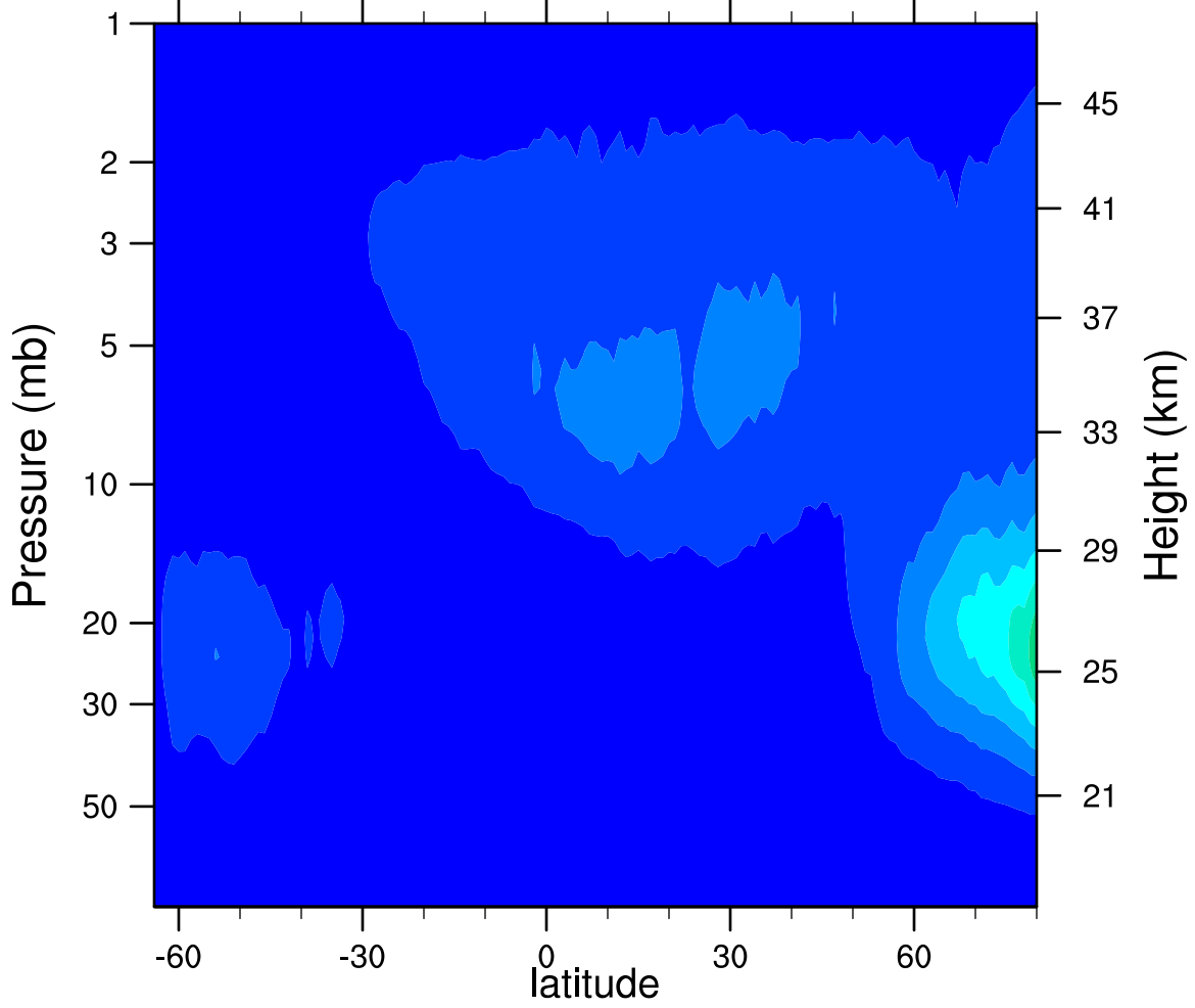
2005d279 N2O5_Ascending (ppbv)
