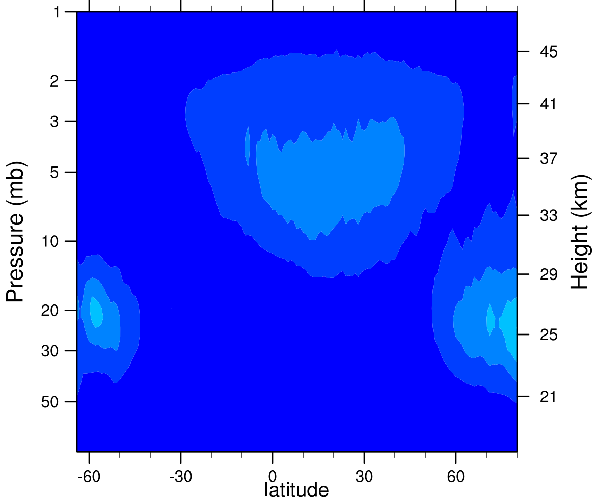
2005d273 N2O5_Ascending (ppbv)
