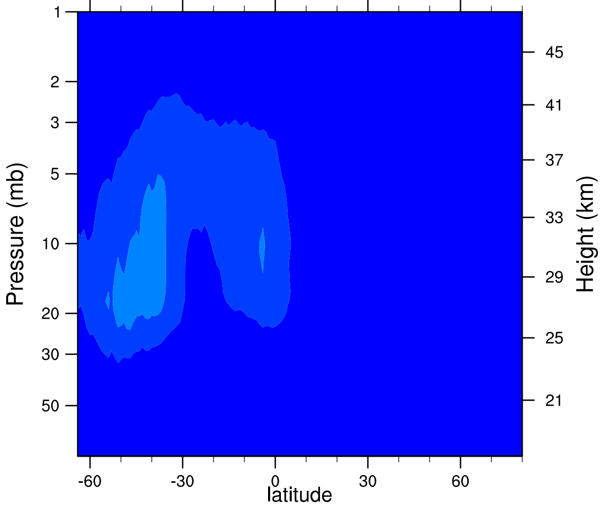
2006d226 N2O5_Ascending (ppbv)
