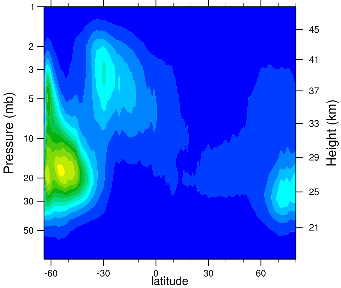
2007d093 N2O5_Ascending (ppbv)
