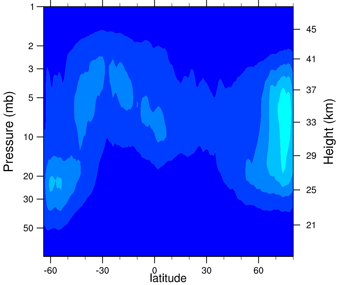
2006d076 N2O5_Ascending (ppbv)
