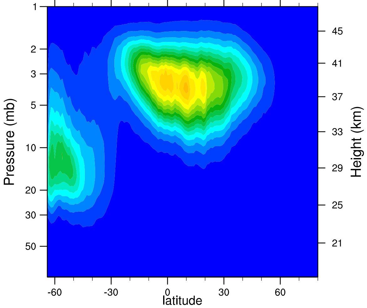
2005d141 N2O5_Ascending (ppbv)
