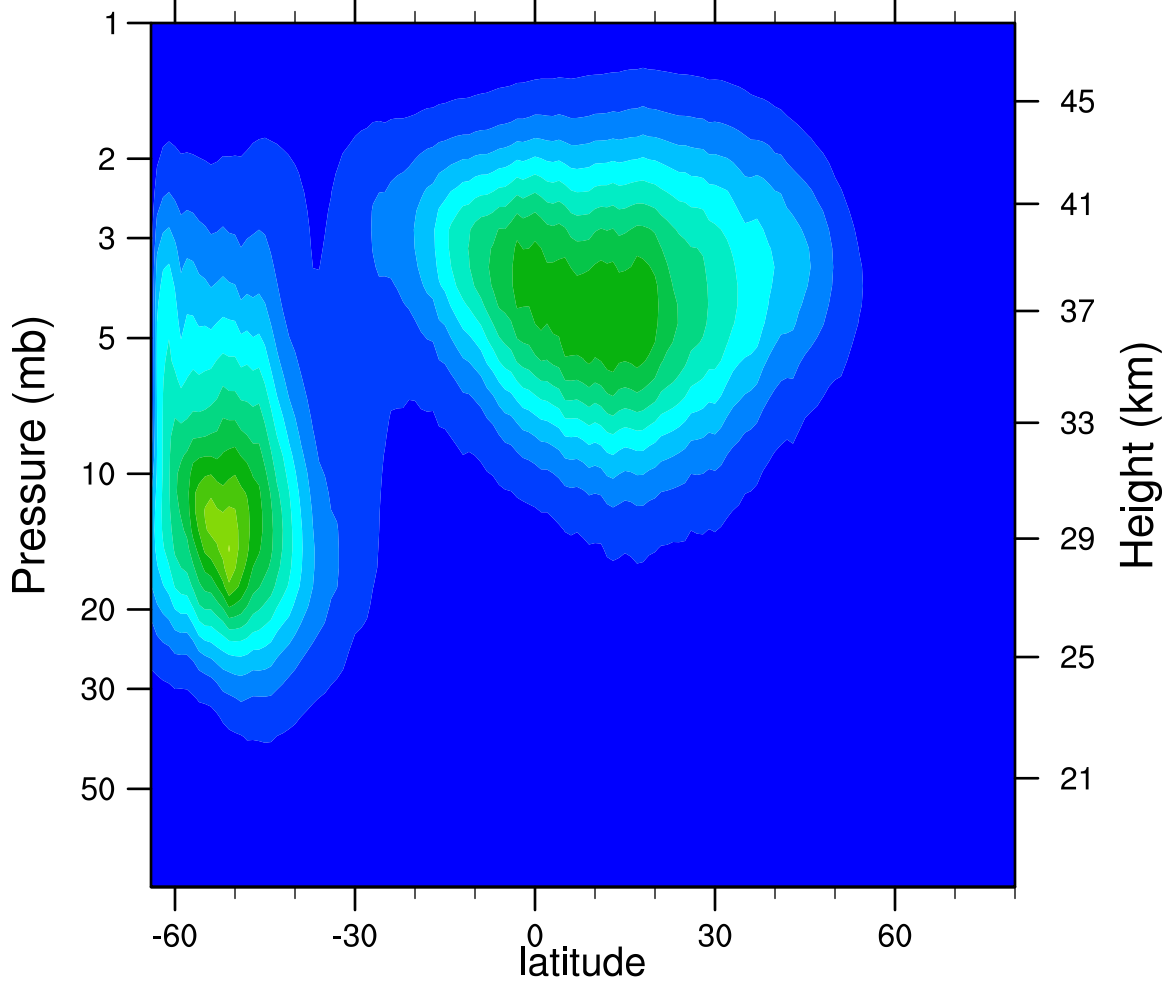
2005d163 N2O5_Ascending (ppbv)
