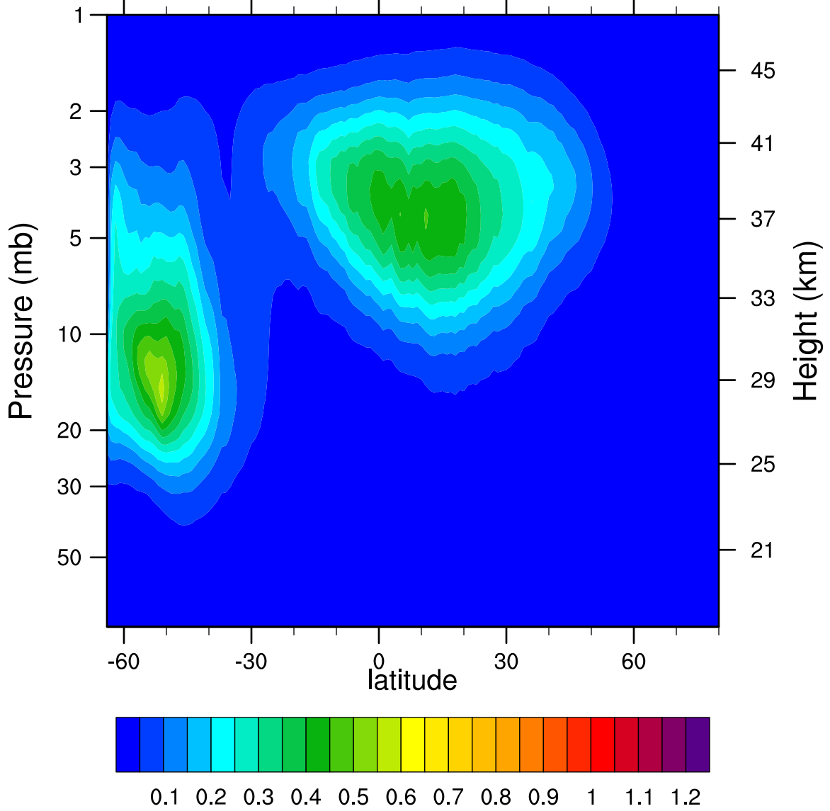
2005d161 N2O5_Ascending (ppbv)
