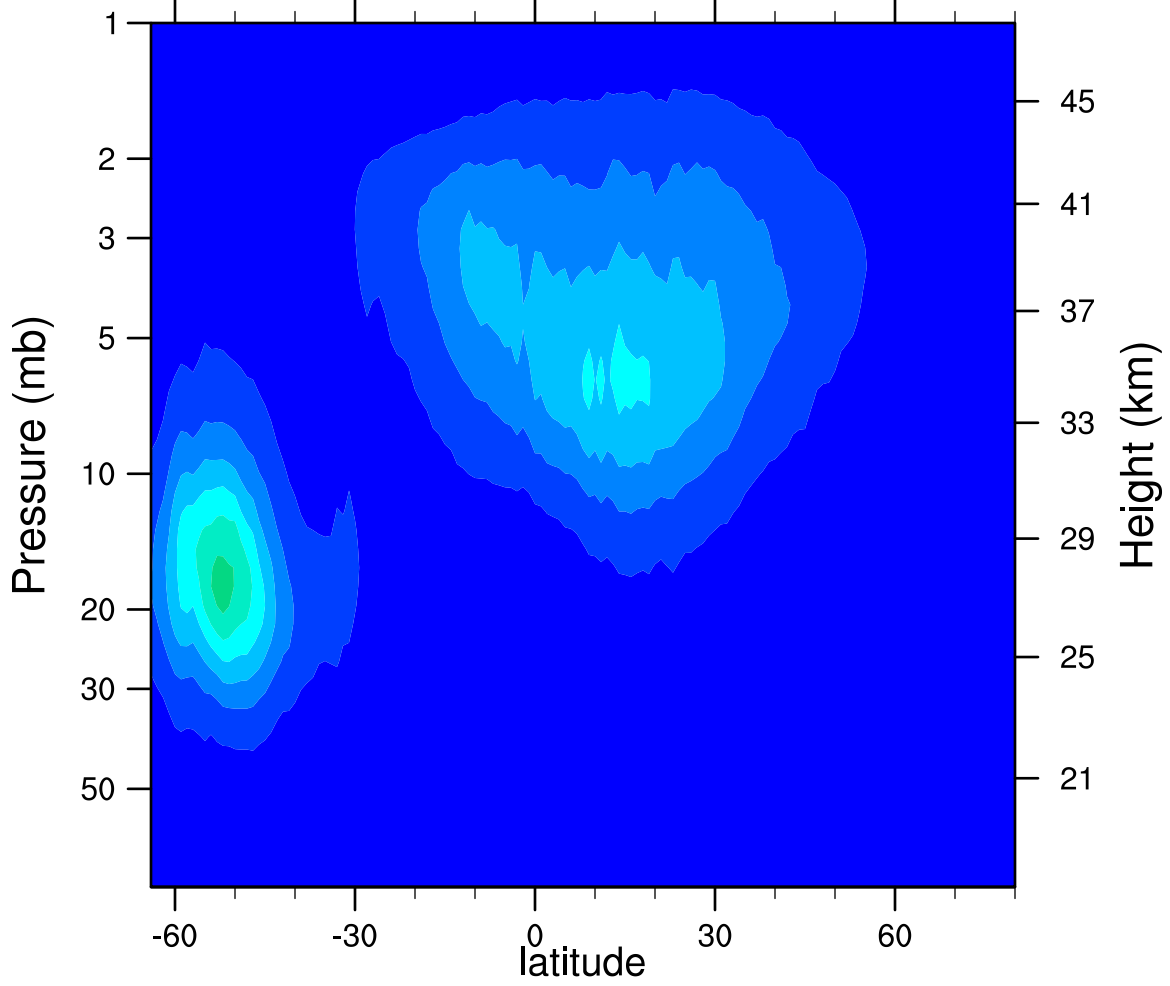
2005d231 N2O5_Ascending (ppbv)
