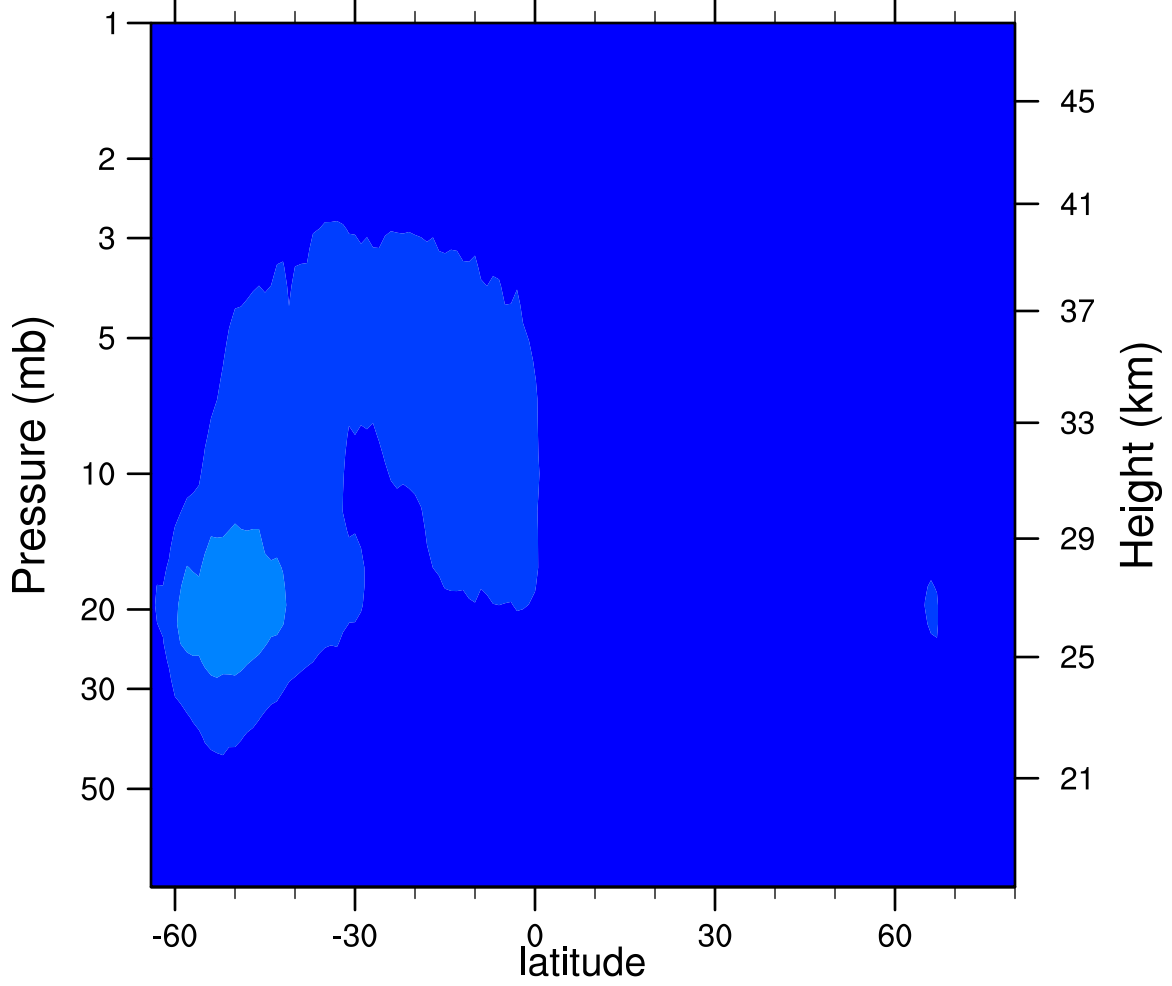
2006d251 N2O5_Ascending (ppbv)
