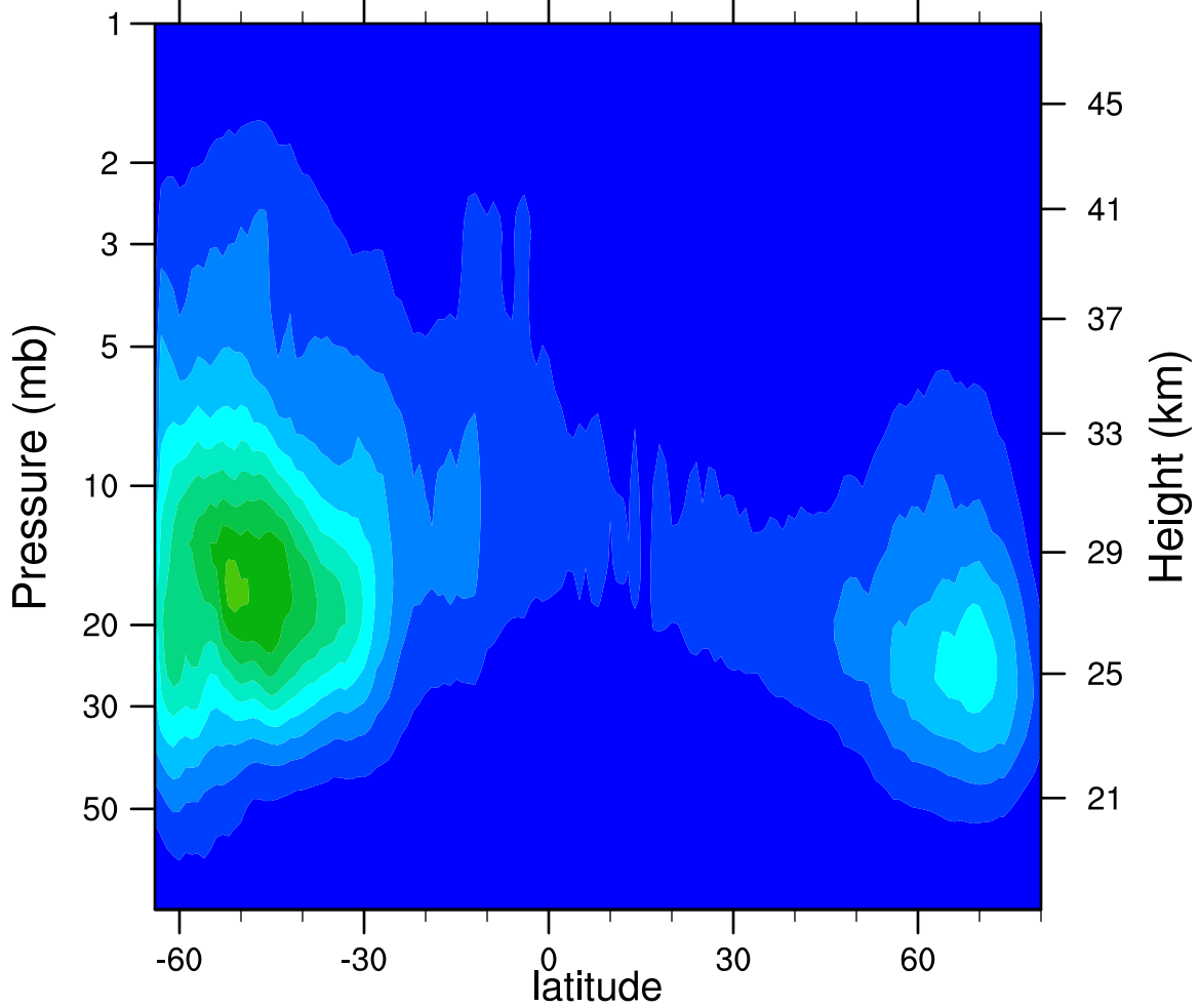
2007d250 N2O5_Ascending (ppbv)
