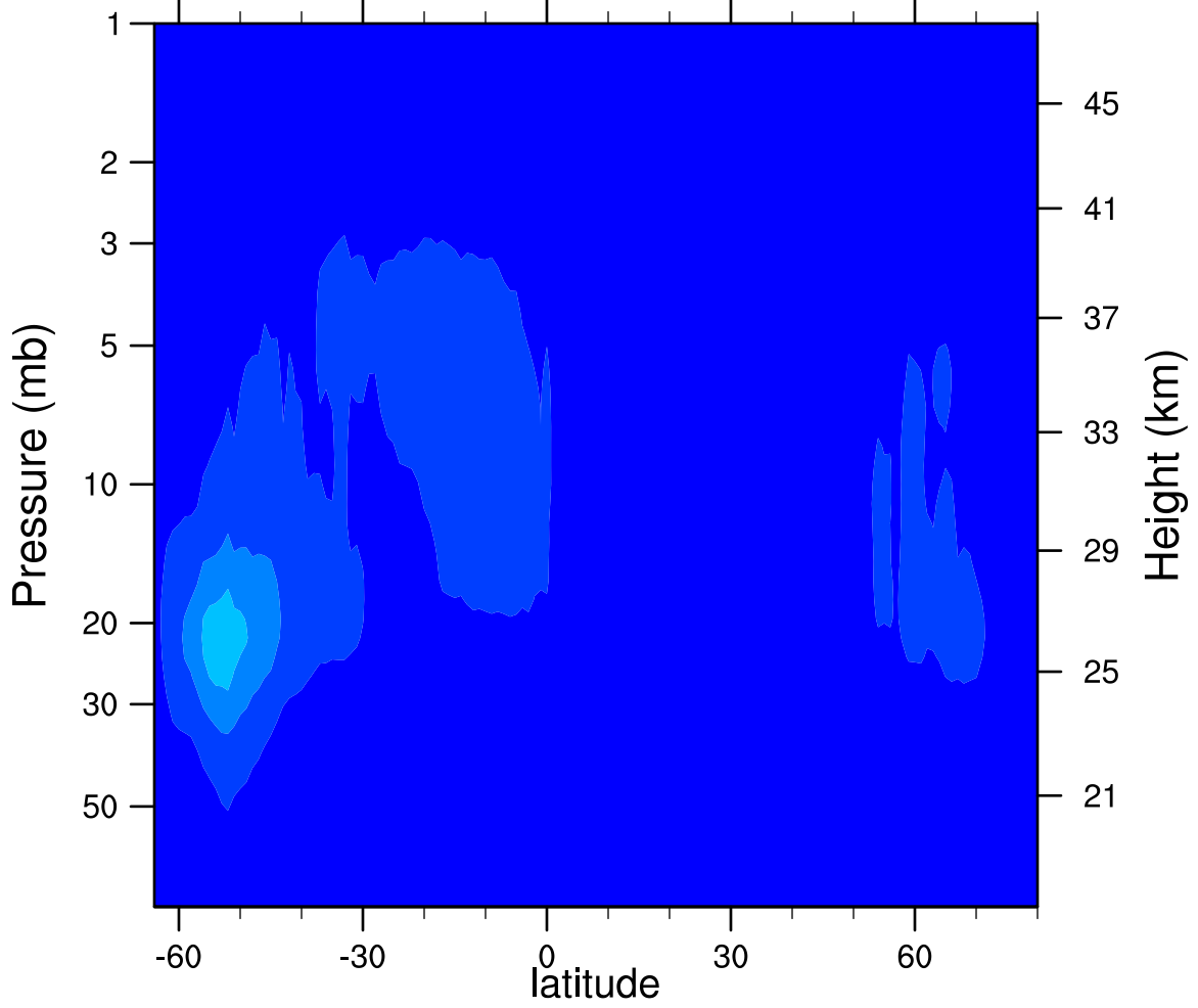
2006d257 N2O5_Ascending (ppbv)
