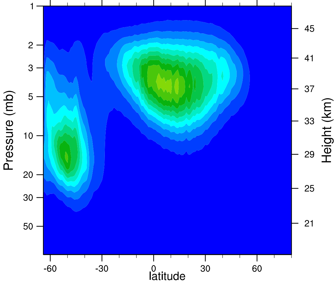
2005d154 N2O5_Ascending (ppbv)
