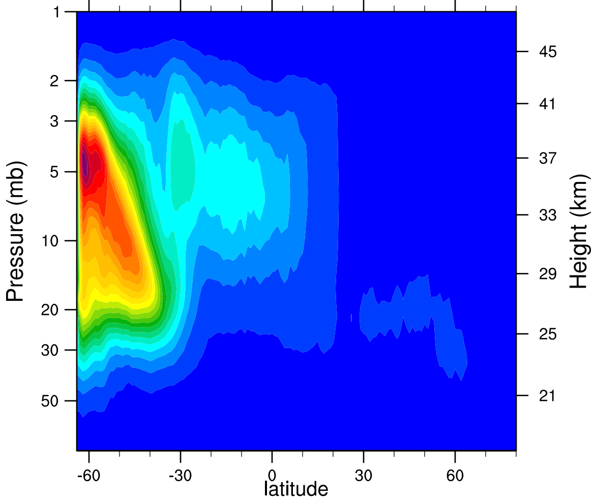
2007d134 N2O5_Ascending (ppbv)
