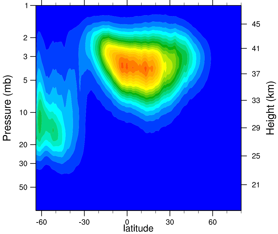
2005d127 N2O5_Ascending (ppbv)
