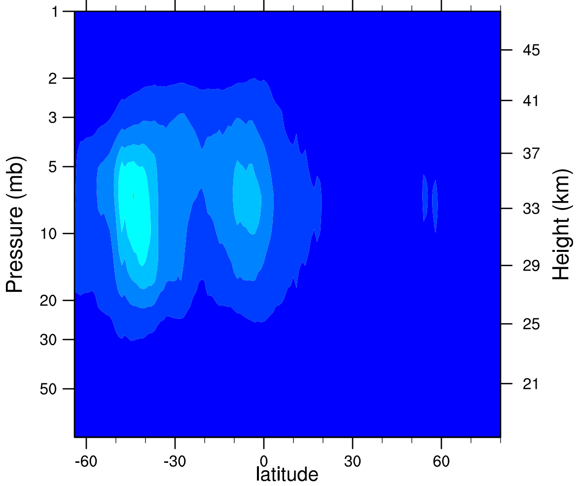
2006d202 N2O5_Ascending (ppbv)
