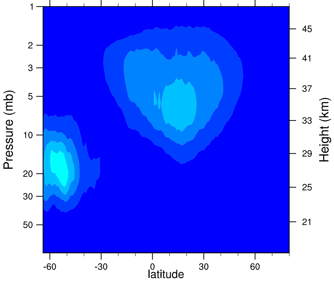
2005d239 N2O5_Ascending (ppbv)
