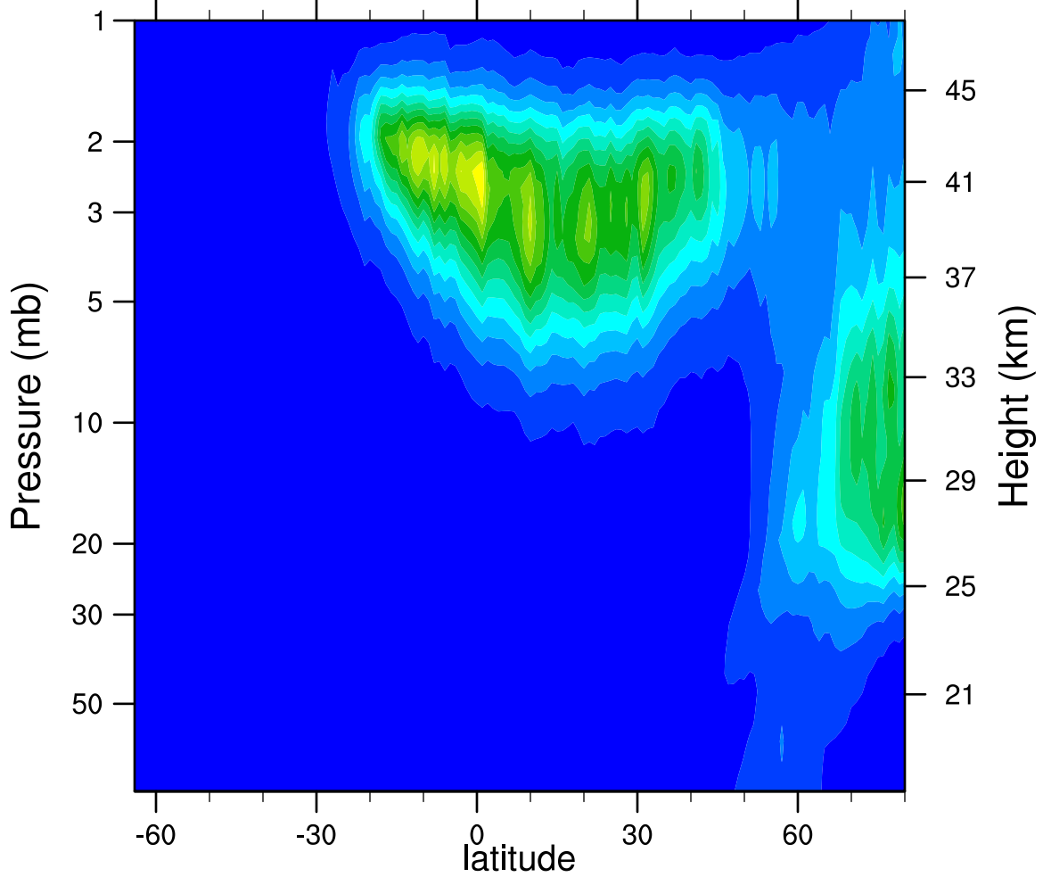
2005d026 N2O5_Ascending (ppbv)
