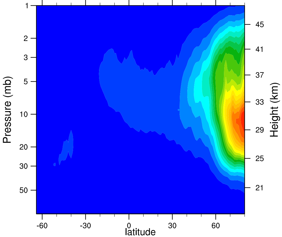
2005d312 N2O5_Ascending (ppbv)
