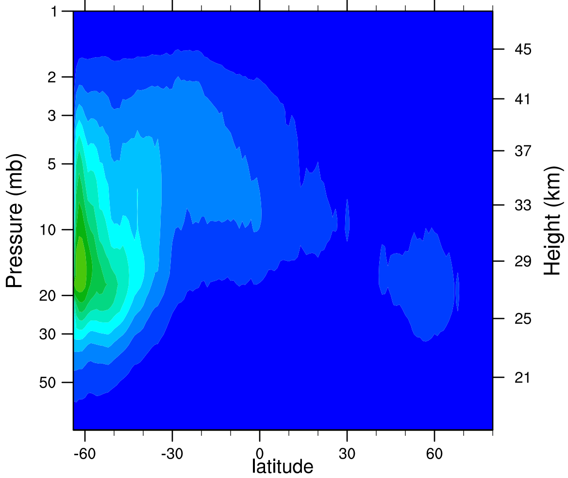
2006d109 N2O5_Ascending (ppbv)
