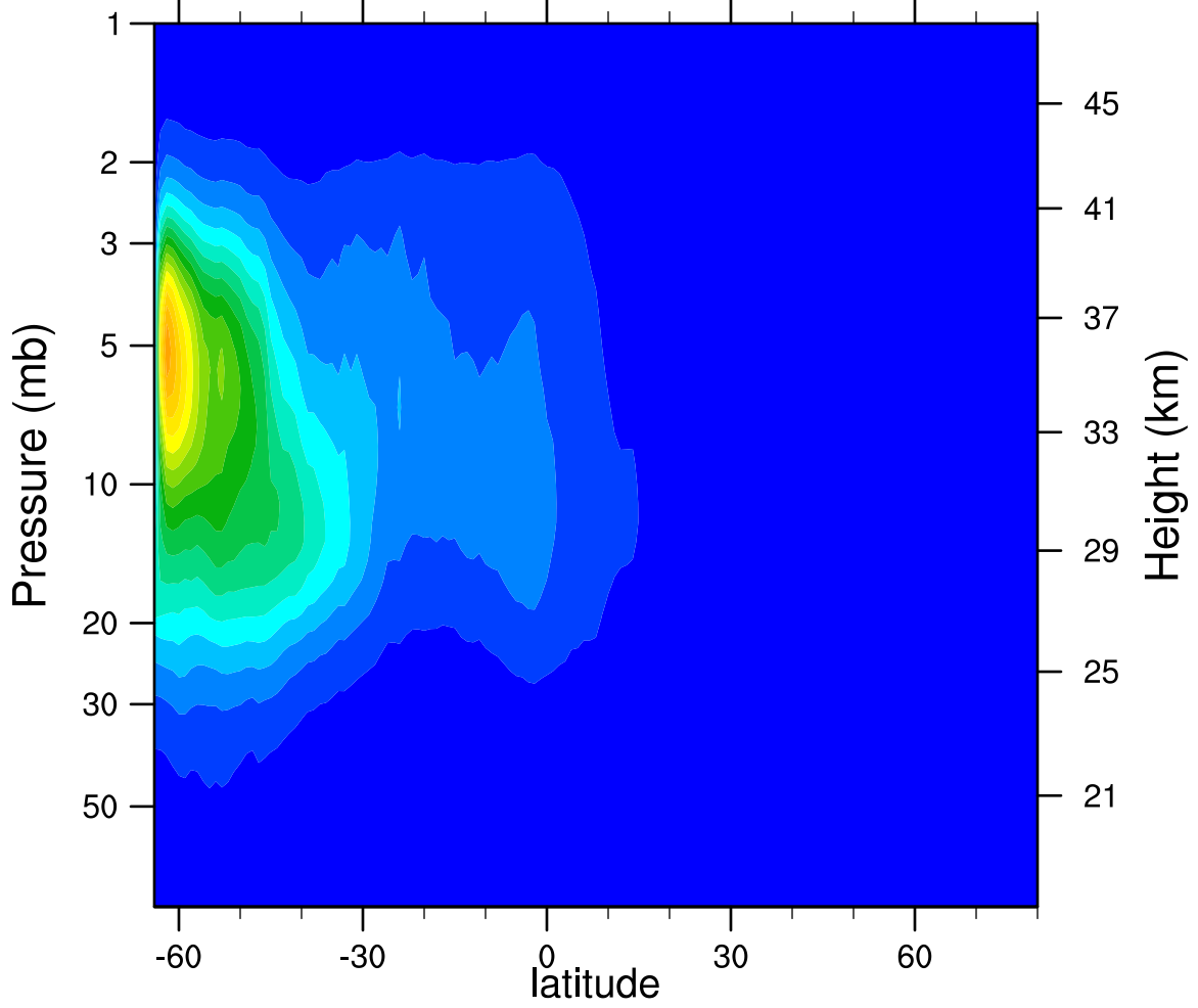
2006d154 N2O5_Ascending (ppbv)
