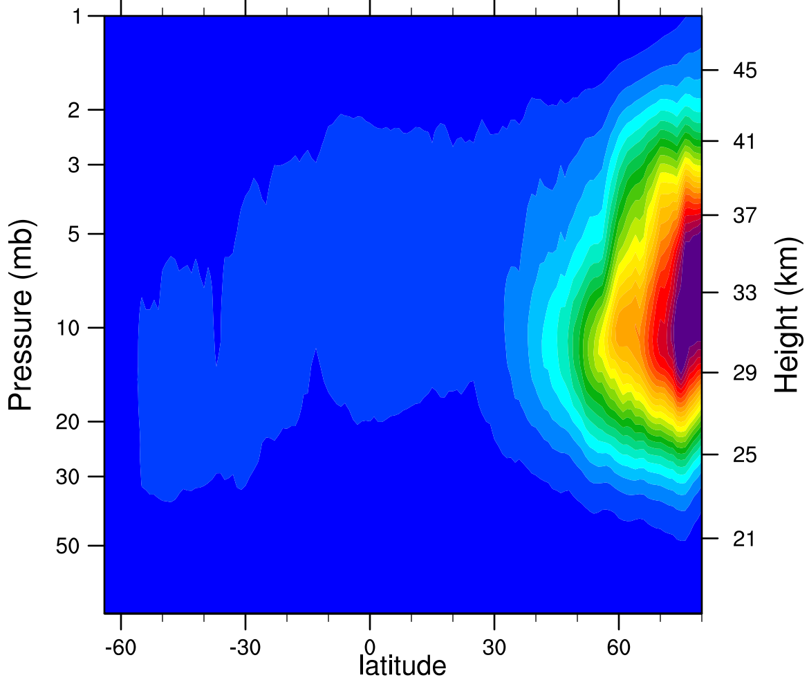
2007d351 N2O5_Ascending (ppbv)
