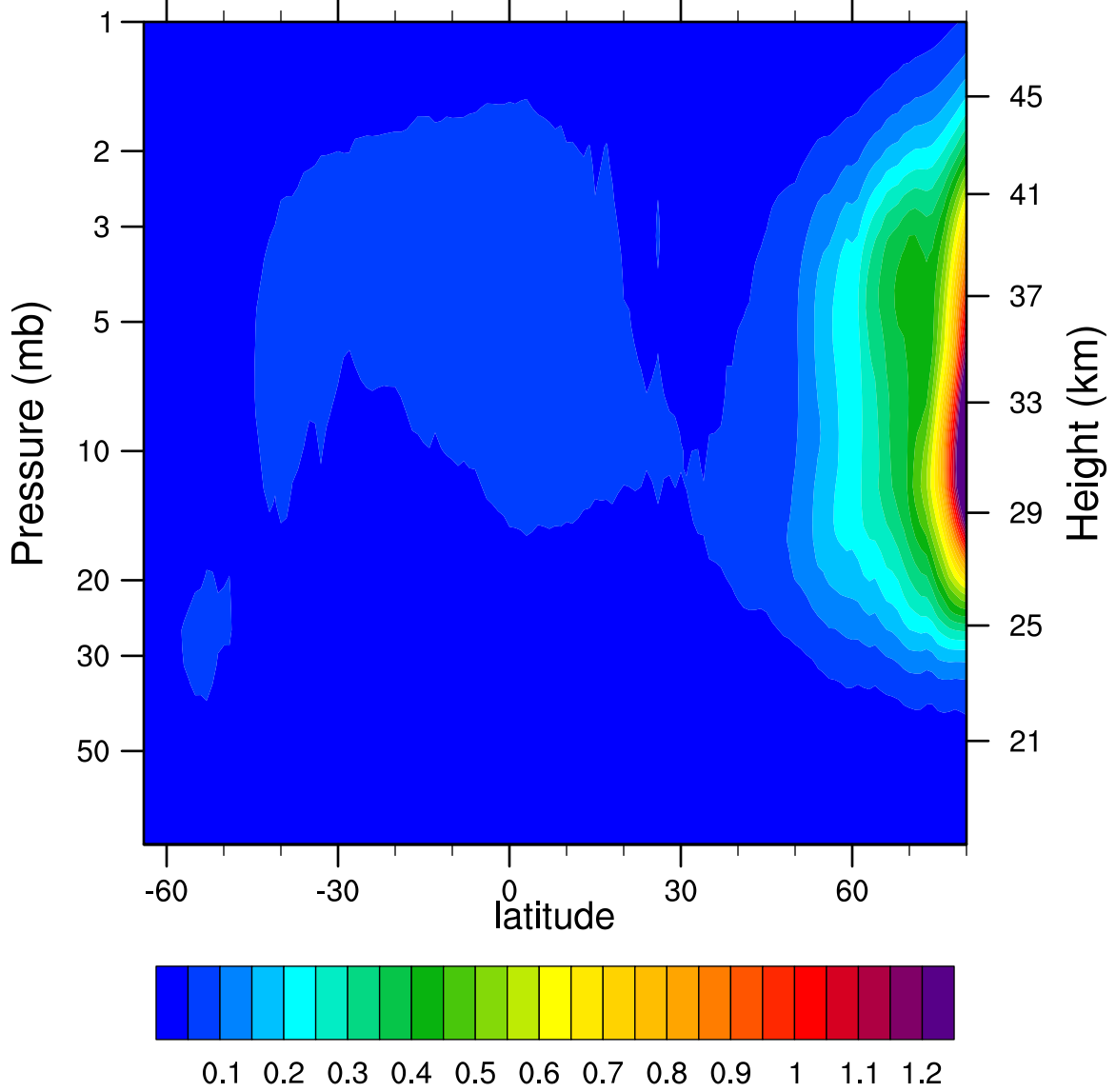
2006d046 N2O5_Ascending (ppbv)
