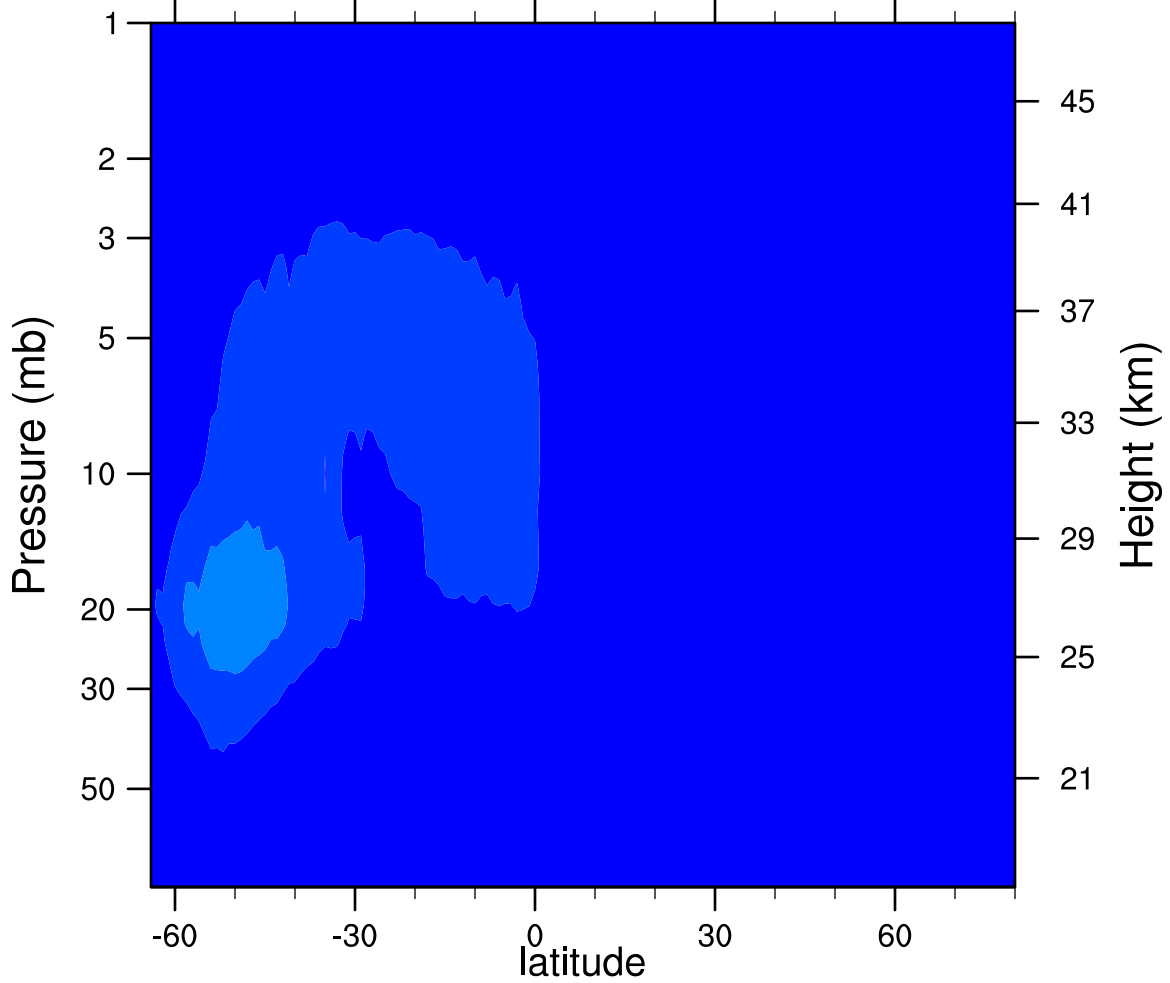
2006d250 N2O5_Ascending (ppbv)
