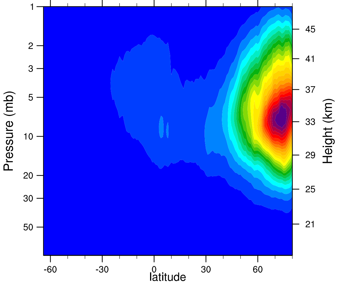
2005d354 N2O5_Ascending (ppbv)
