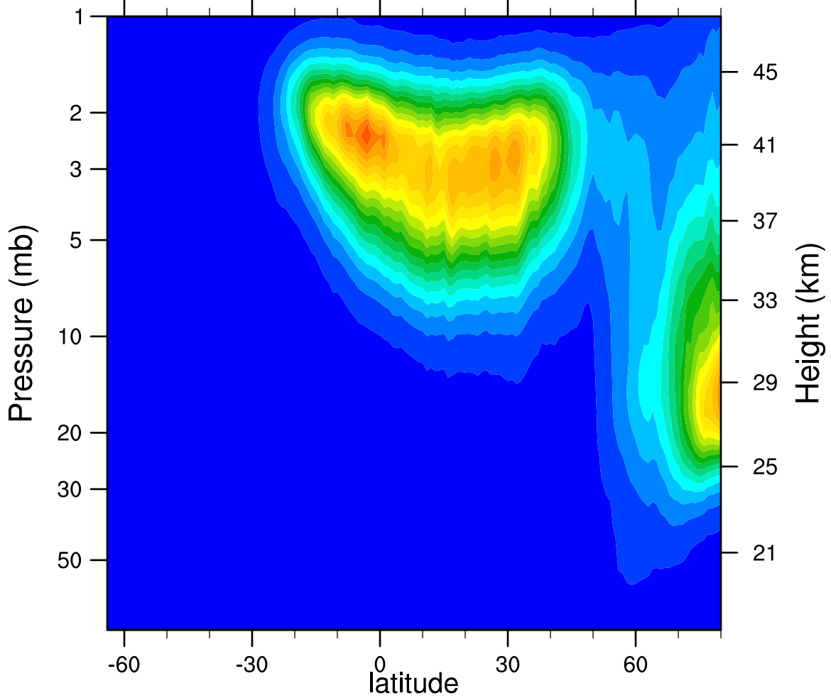
2005d030 N2O5_Ascending (ppbv)
