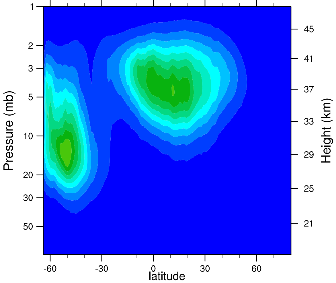
2005d166 N2O5_Ascending (ppbv)
