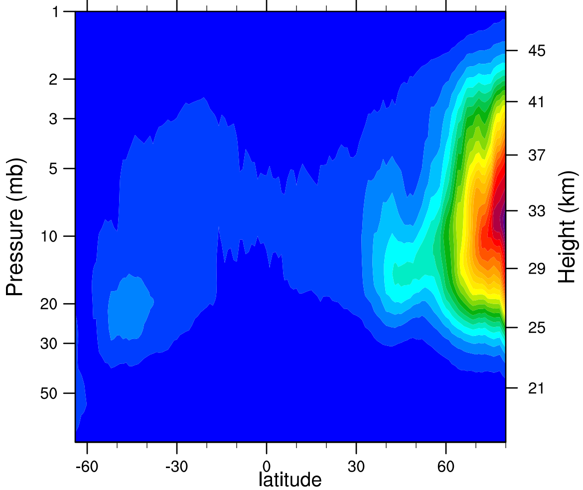
2006d323 N2O5_Ascending (ppbv)
