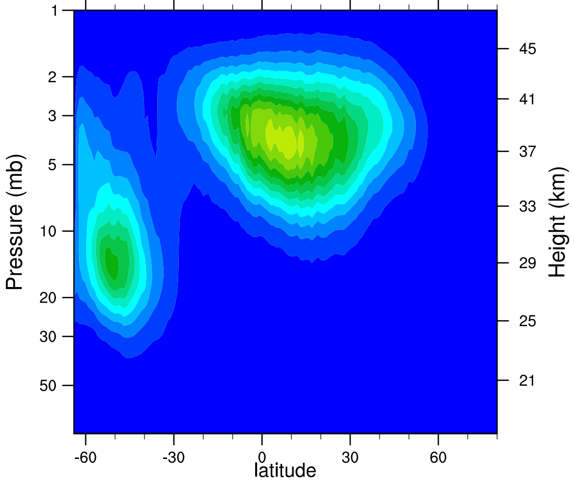
2005d151 N2O5_Ascending (ppbv)
