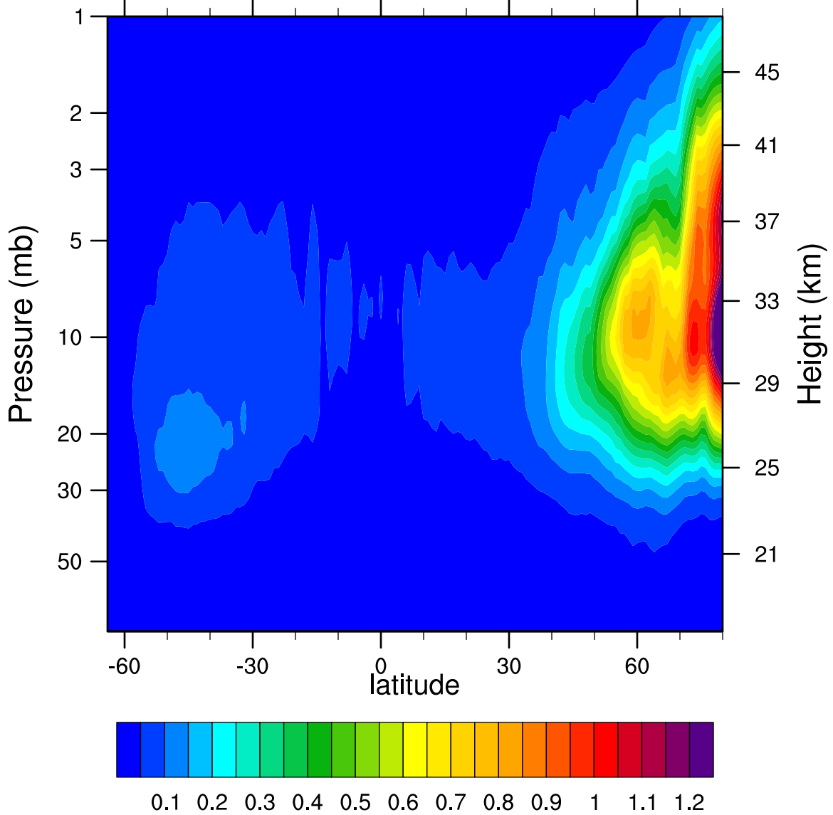
2006d341 N2O5_Ascending (ppbv)
