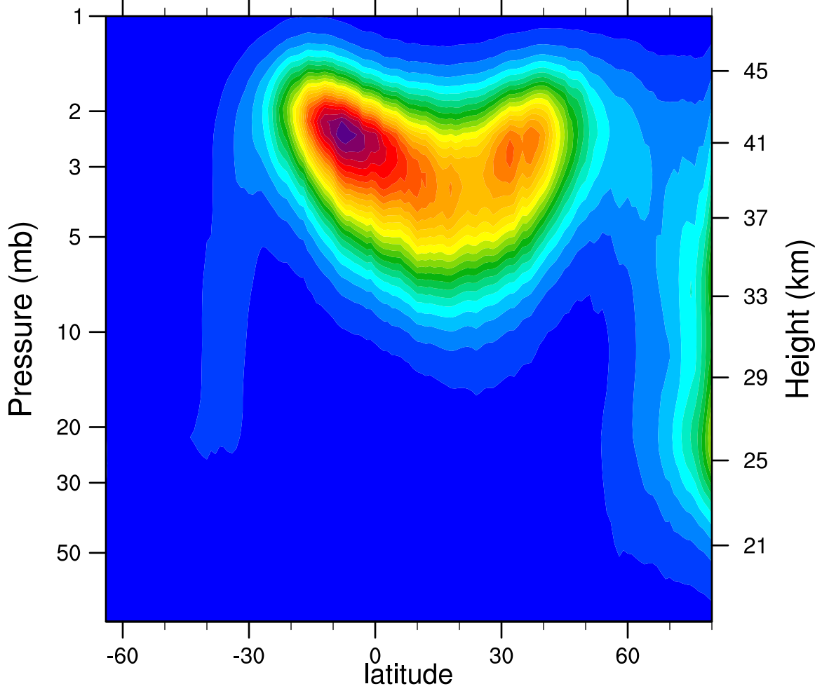
2005d058 N2O5_Ascending (ppbv)
