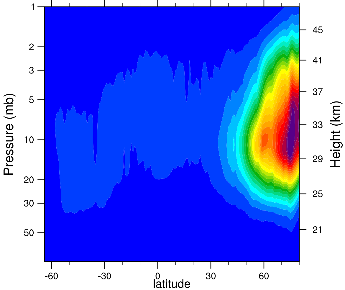
2007d355 N2O5_Ascending (ppbv)
