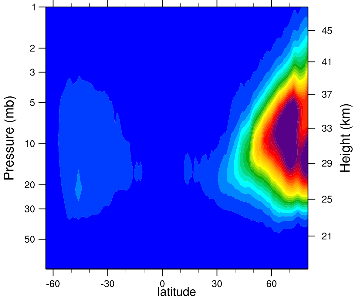
2006d354 N2O5_Ascending (ppbv)
