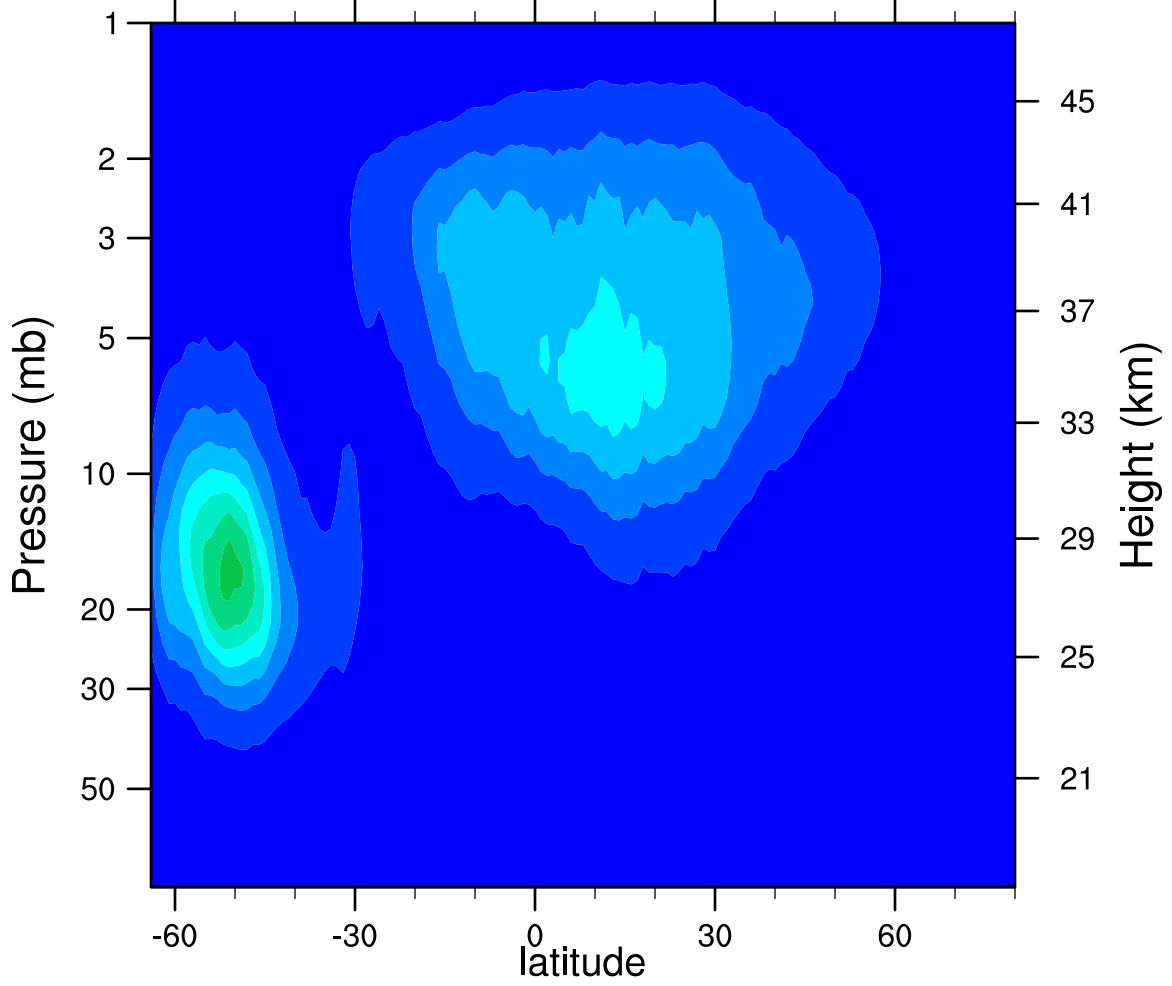
2005d227 N2O5_Ascending (ppbv)
