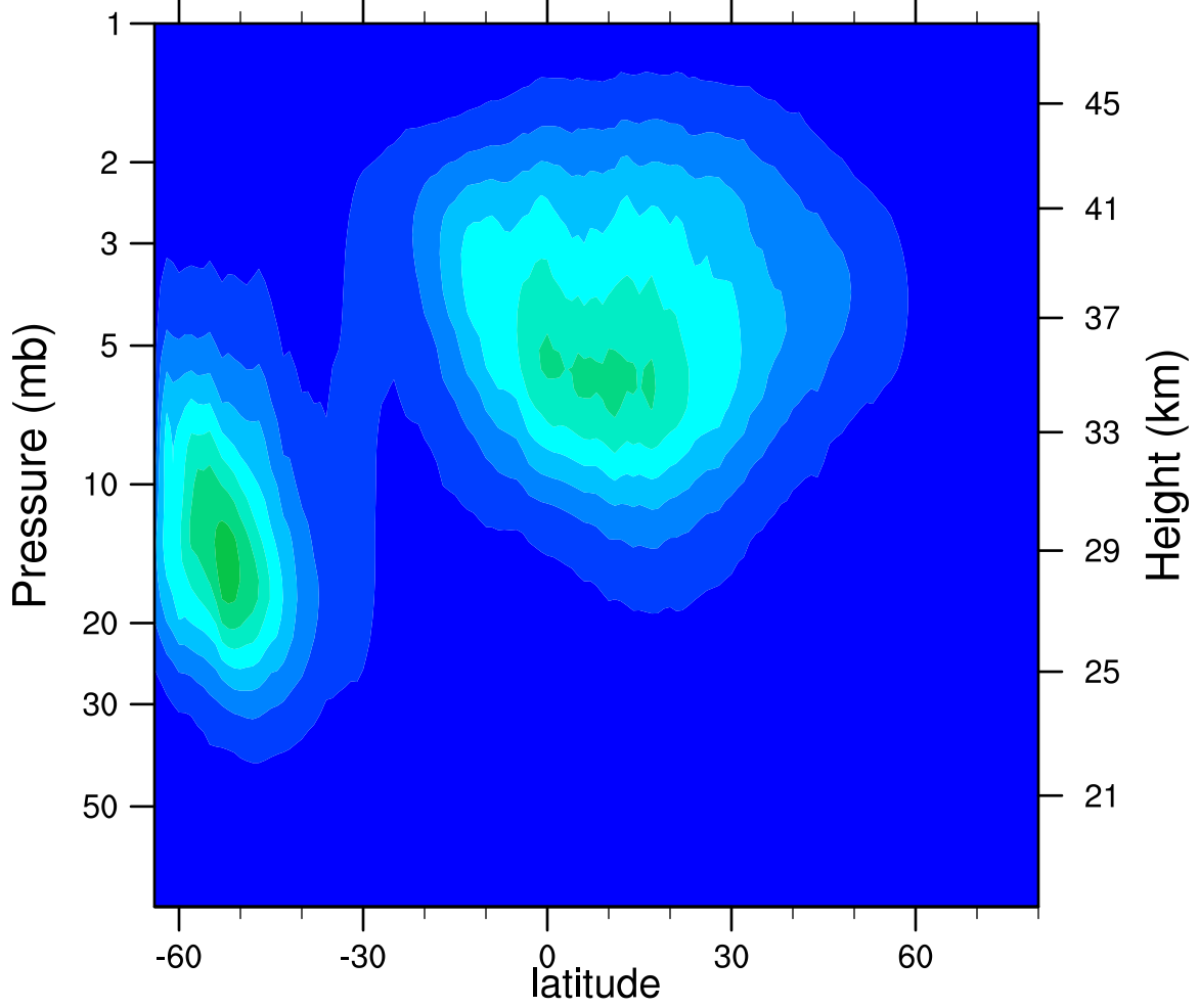
2005d215 N2O5_Ascending (ppbv)
