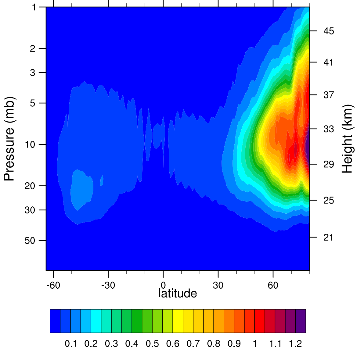
2006d344 N2O5_Ascending (ppbv)
