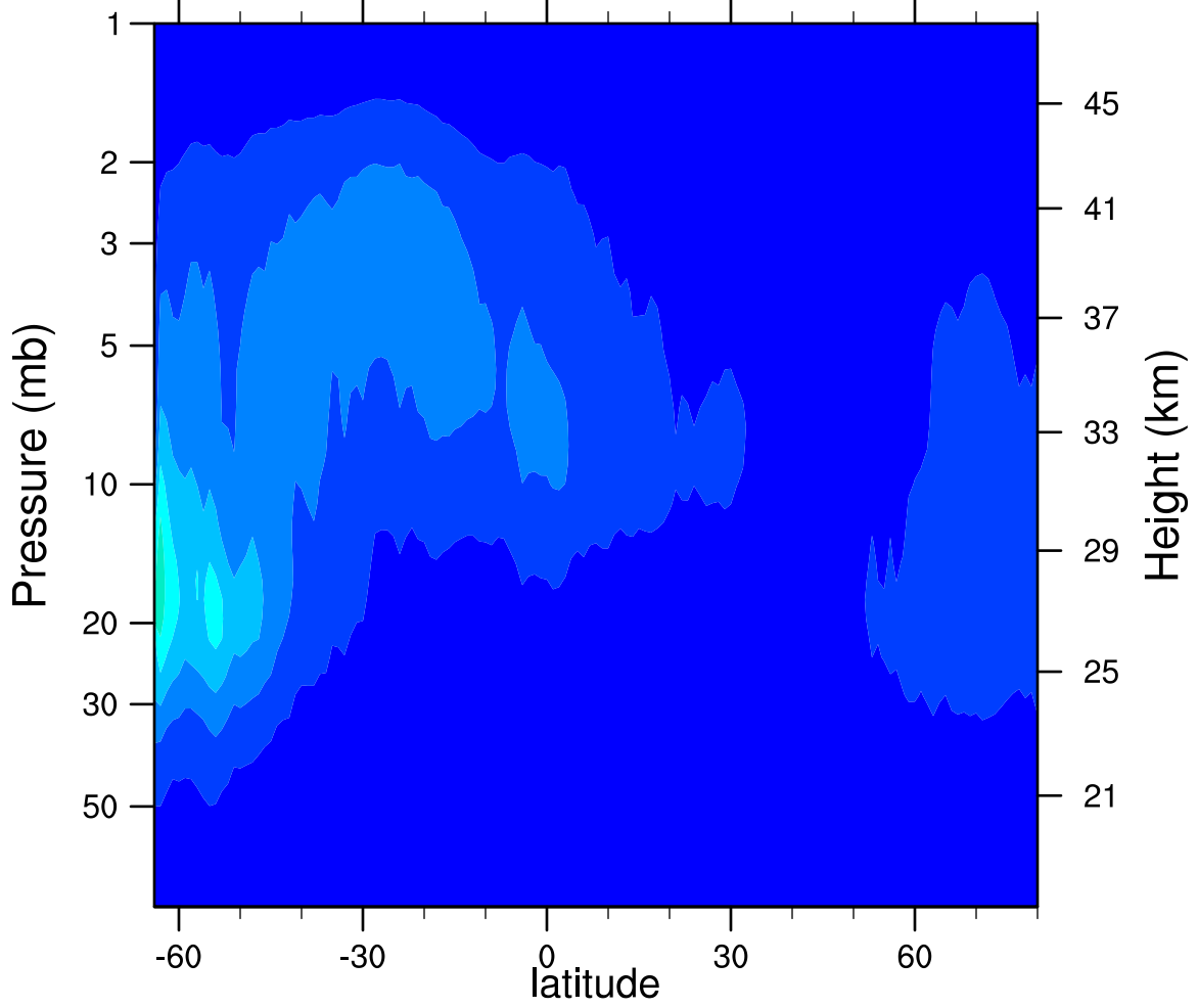
2006d095 N2O5_Ascending (ppbv)
