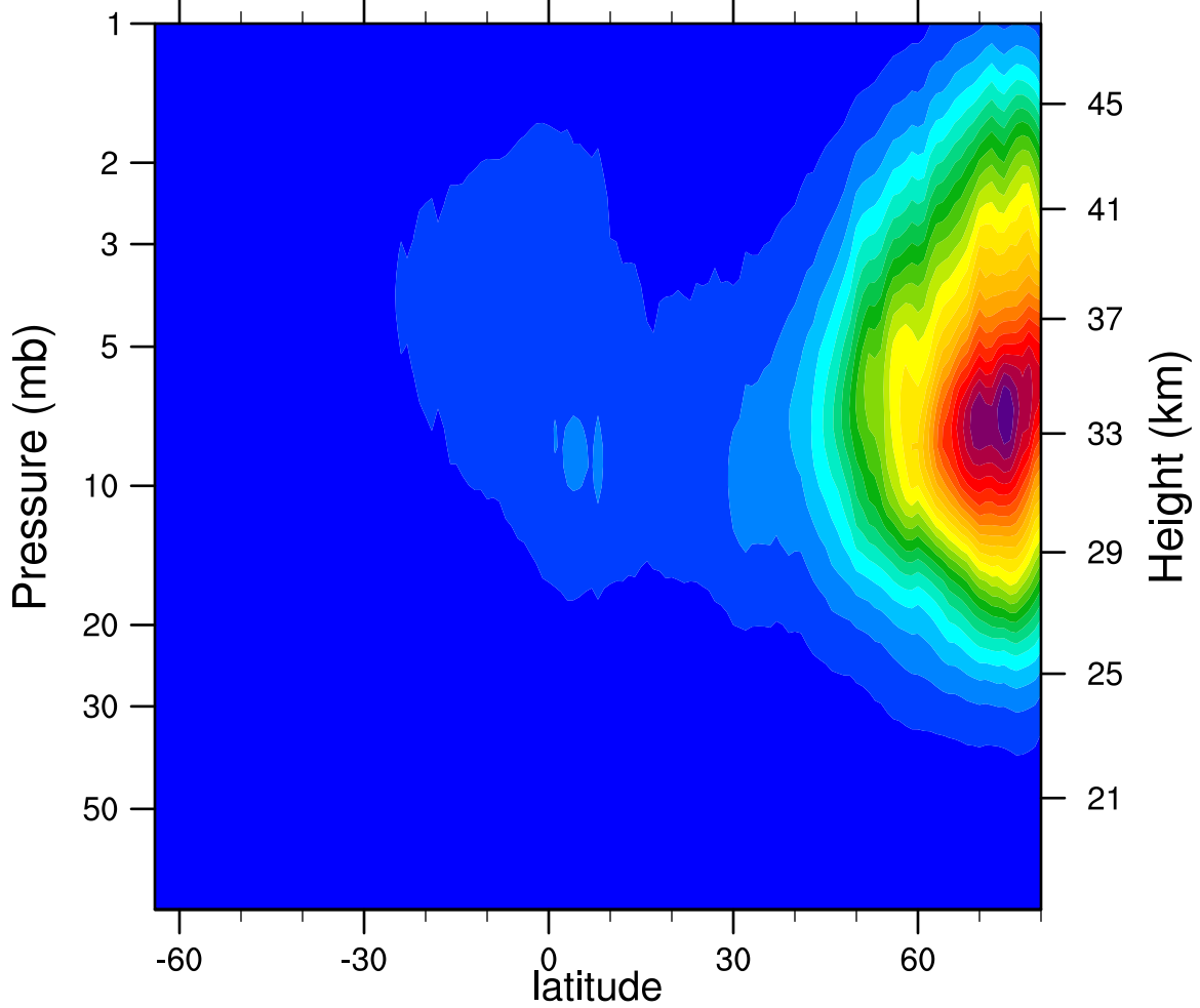
2005d355 N2O5_Ascending (ppbv)
