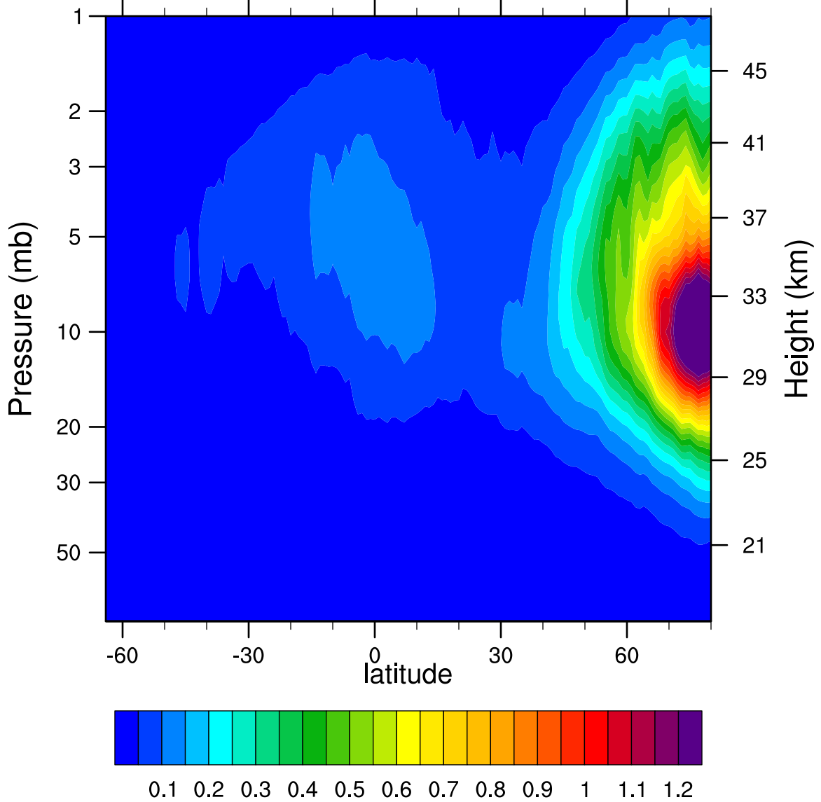
2006d011 N2O5_Ascending (ppbv)
