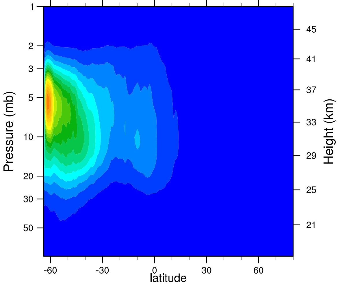
2006d166 N2O5_Ascending (ppbv)
