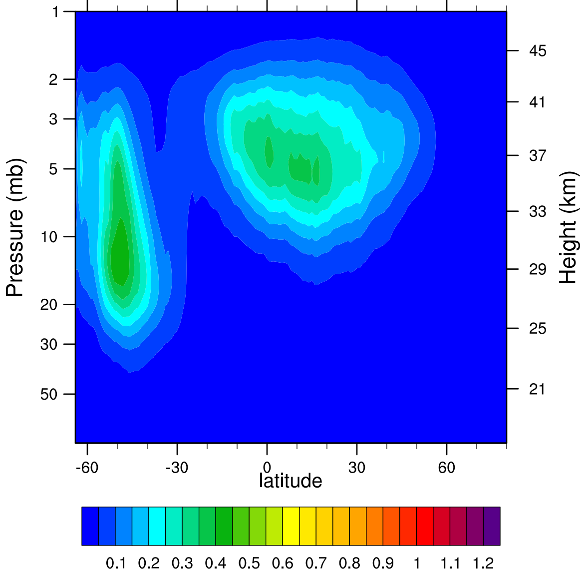
2005d181 N2O5_Ascending (ppbv)
