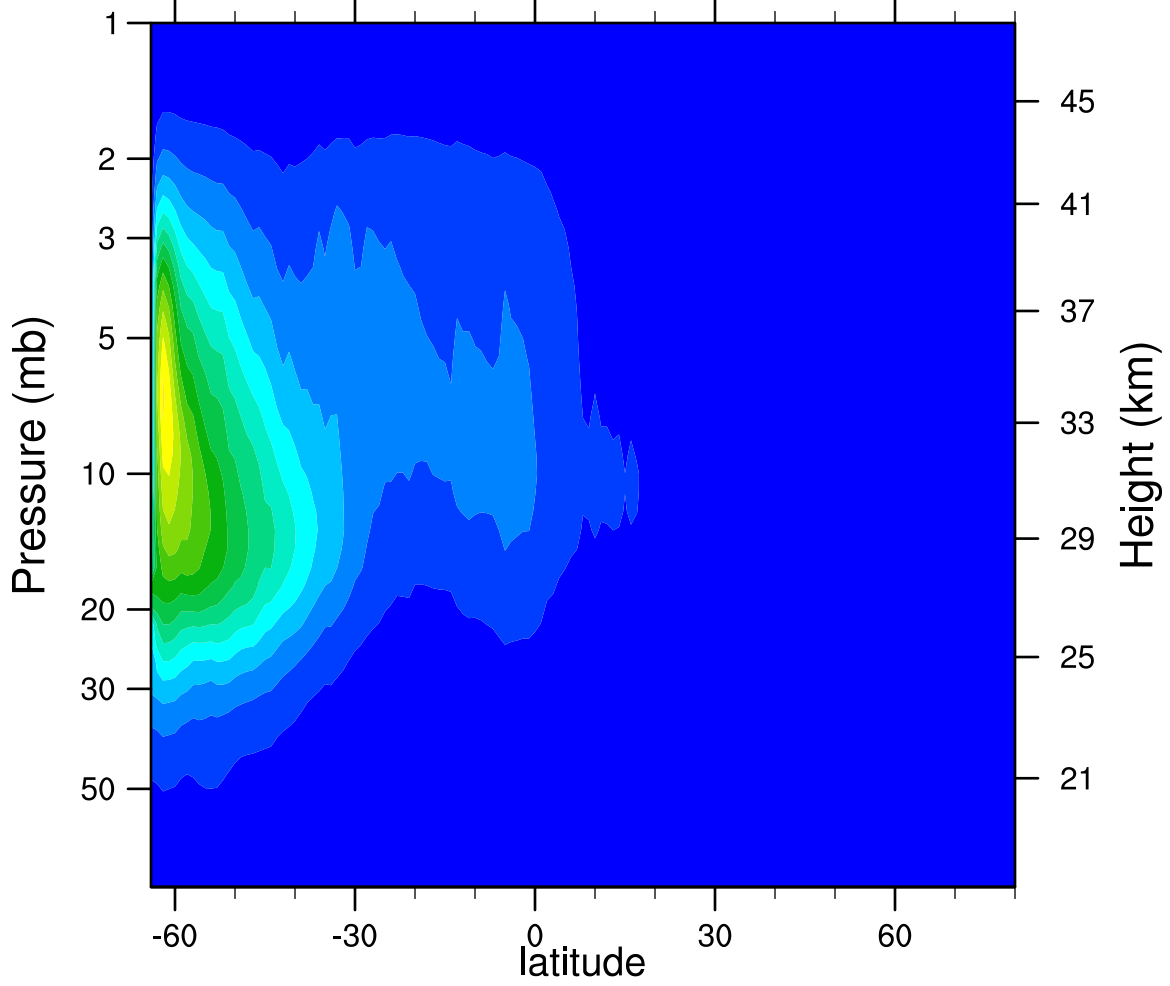
2006d133 N2O5_Ascending (ppbv)
