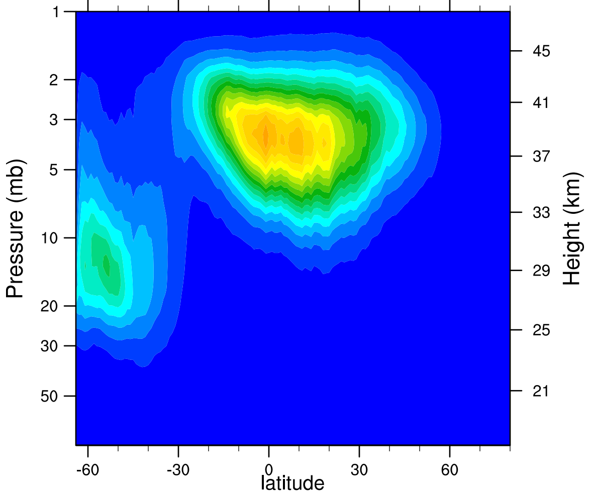
2005d139 N2O5_Ascending (ppbv)
