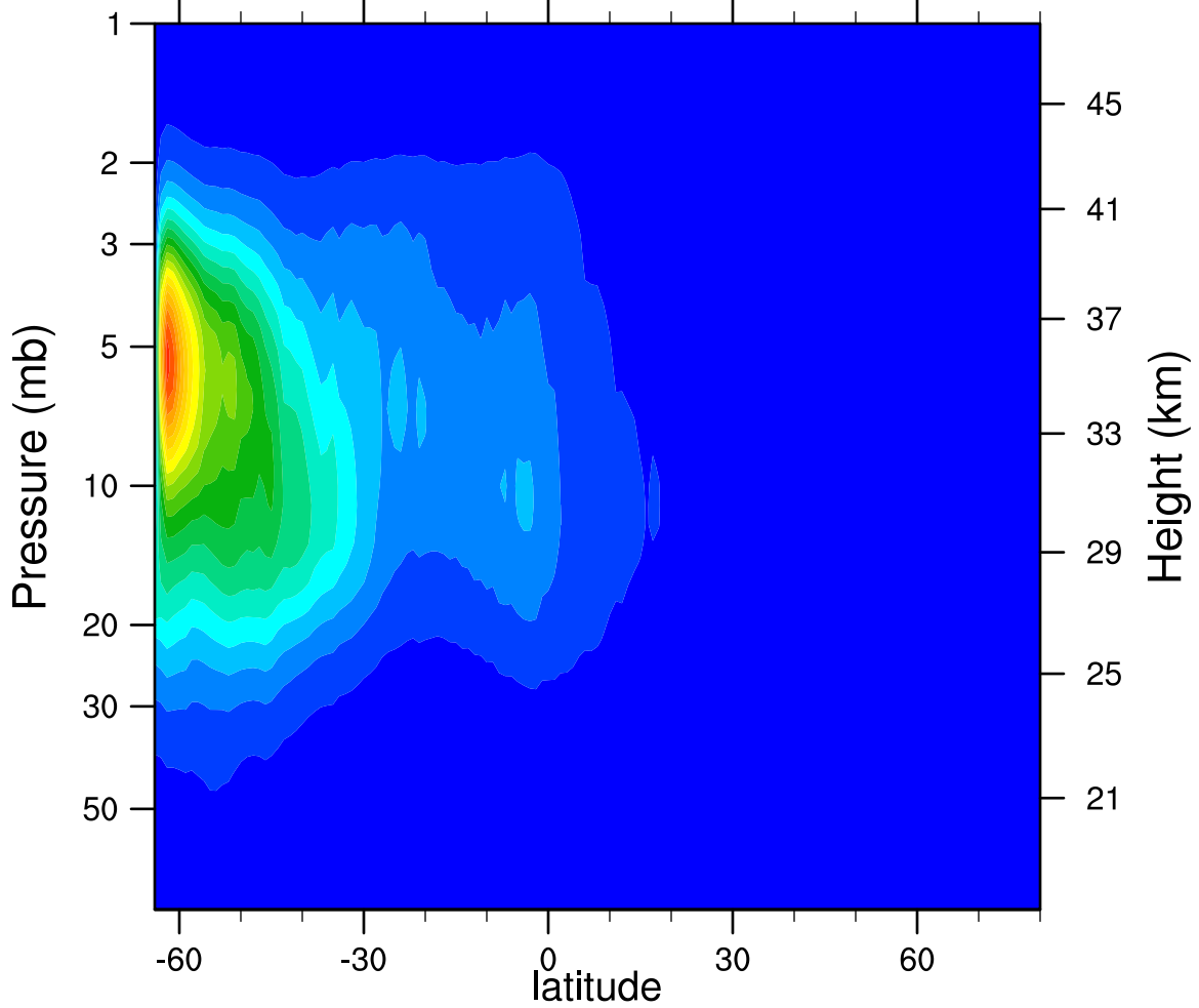
2006d158 N2O5_Ascending (ppbv)
