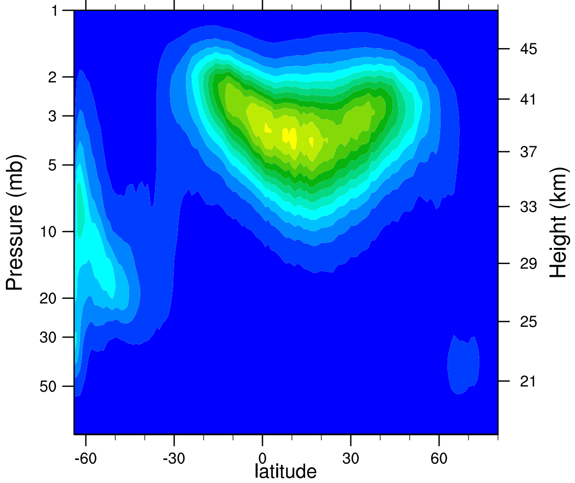
2005d101 N2O5_Ascending (ppbv)
