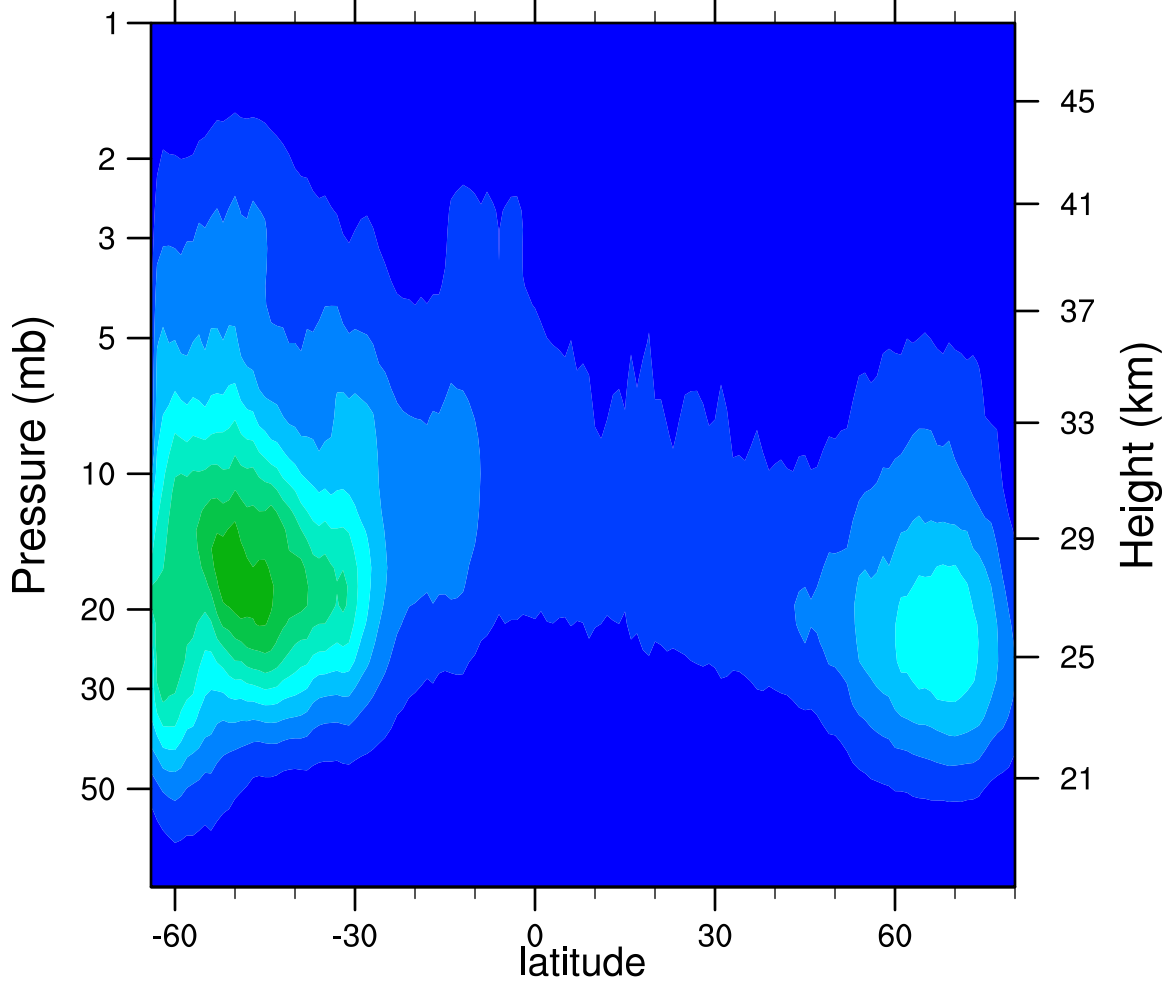
2007d253 N2O5_Ascending (ppbv)
