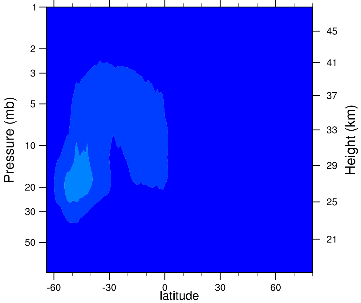
2006d241 N2O5_Ascending (ppbv)
