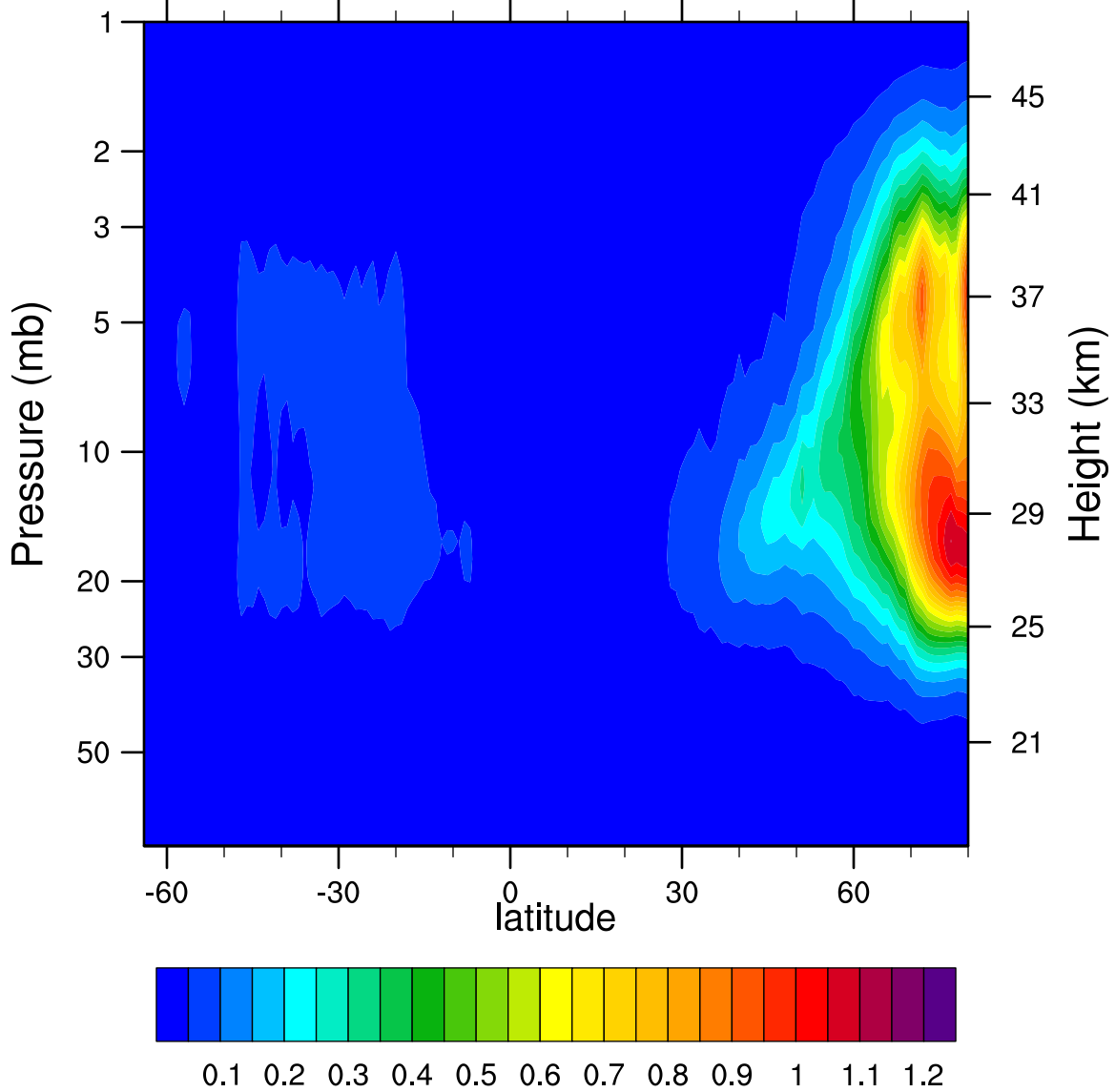
2006d309 N2O5_Ascending (ppbv)
