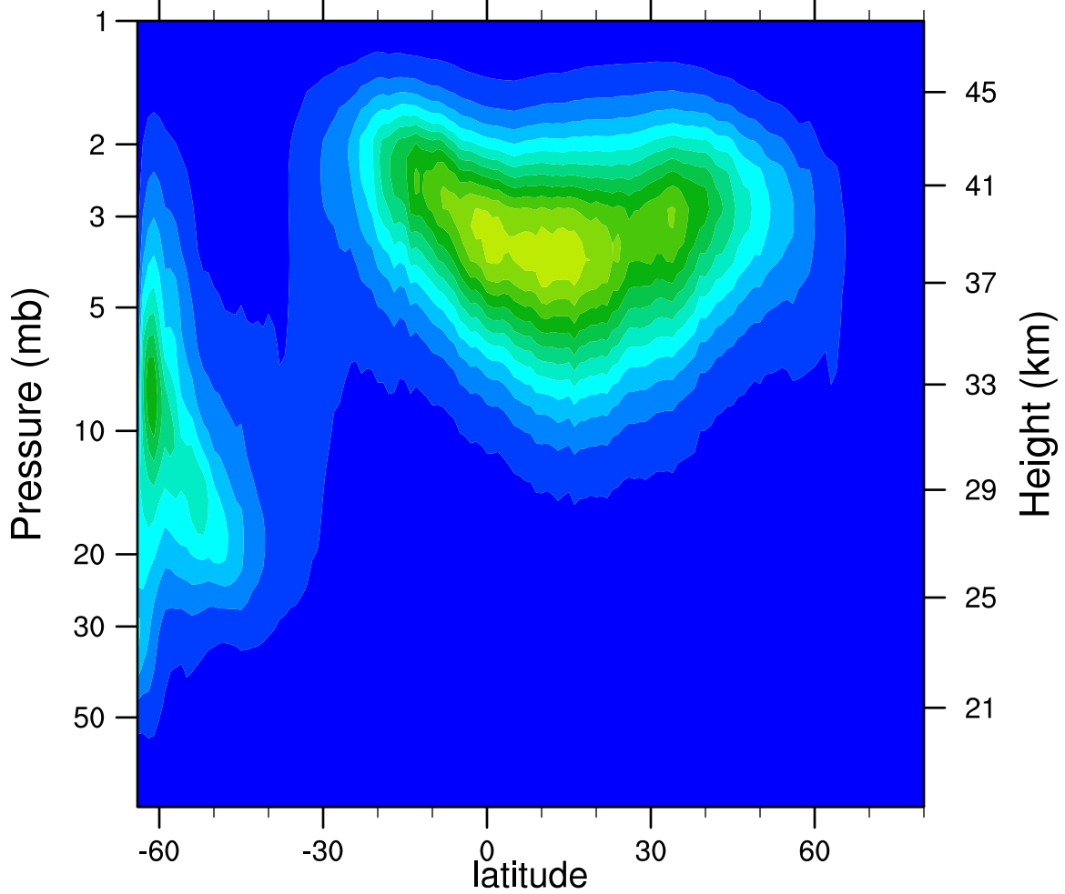
2005d107 N2O5_Ascending (ppbv)
