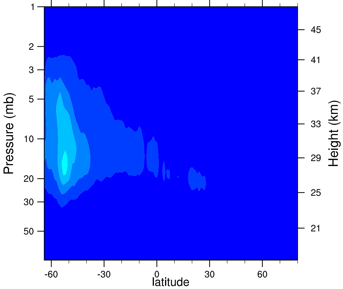
2007d190 N2O5_Ascending (ppbv)
