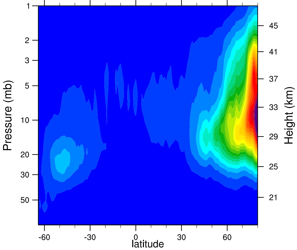
2006d333 N2O5_Ascending (ppbv)
