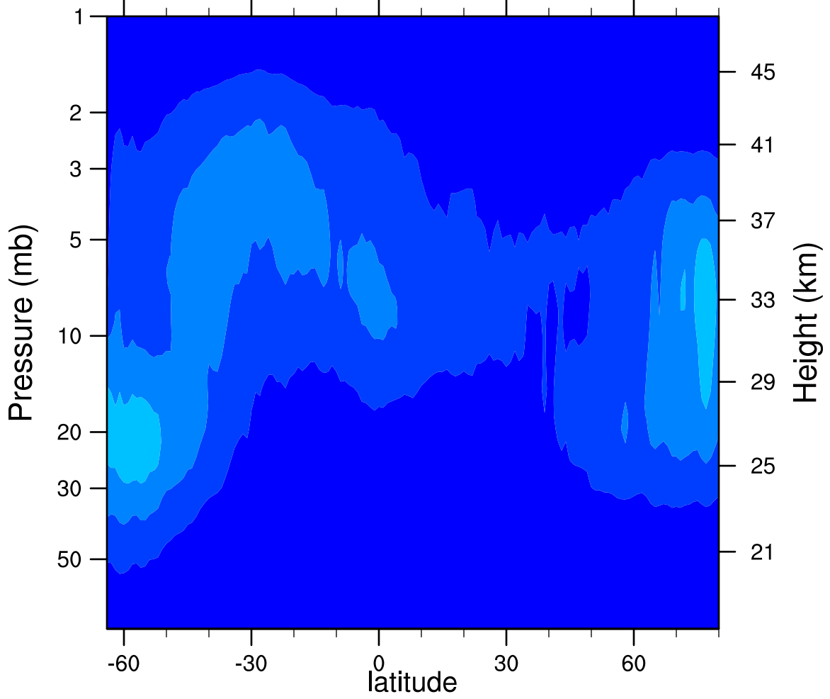
2006d084 N2O5_Ascending (ppbv)
