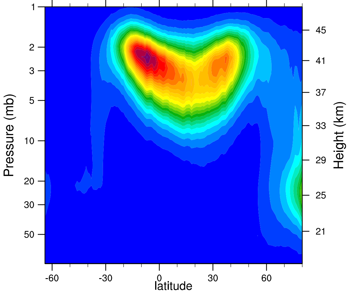
2005d062 N2O5_Ascending (ppbv)
