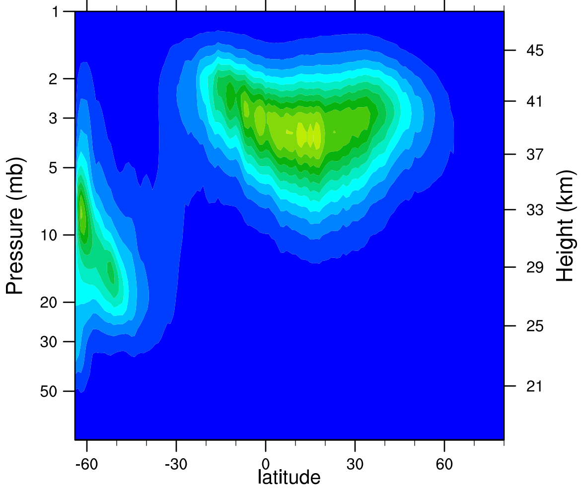
2005d113 N2O5_Ascending (ppbv)
