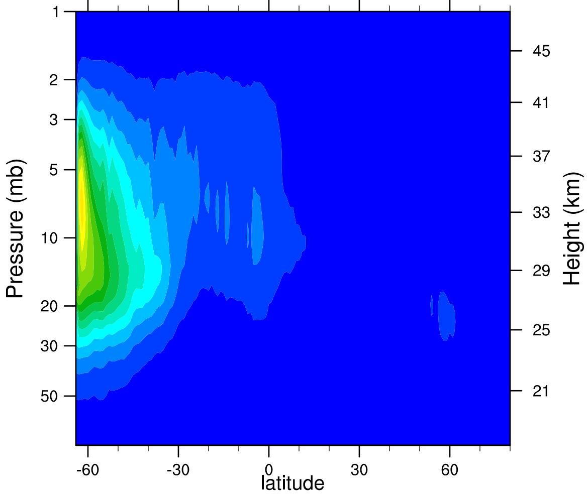
2006d125 N2O5_Ascending (ppbv)
