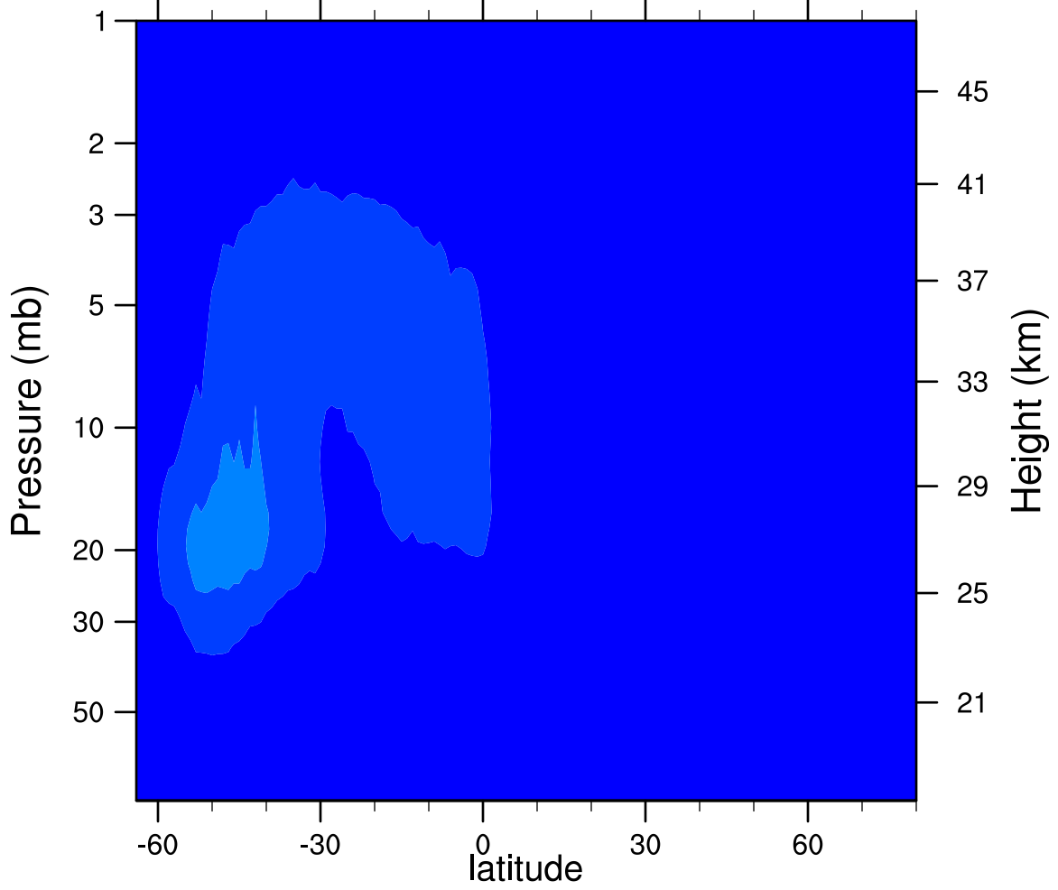
2006d242 N2O5_Ascending (ppbv)
