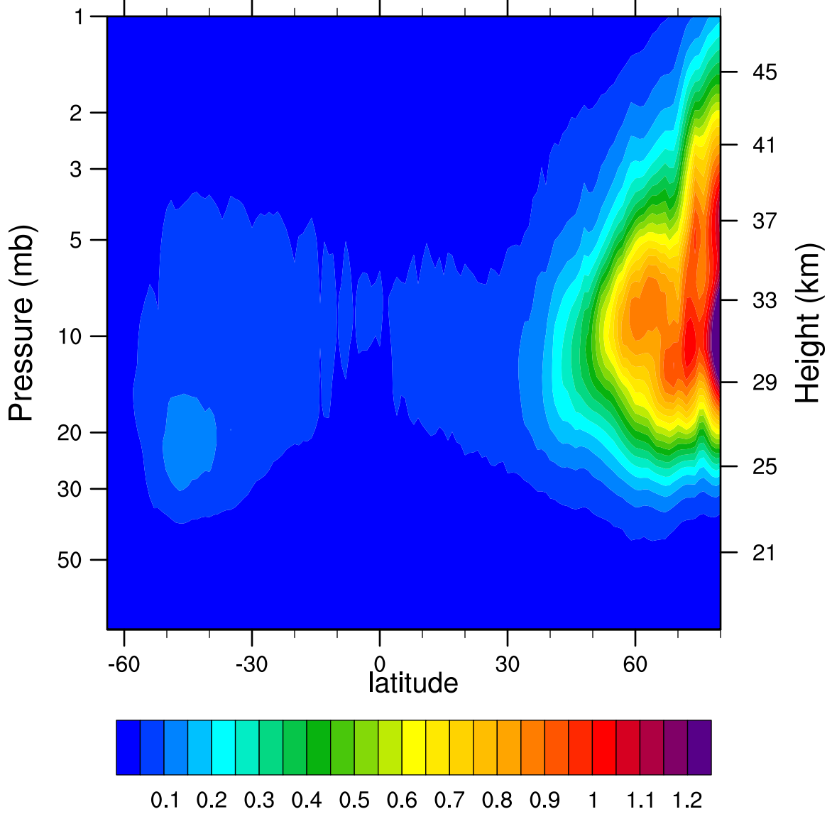
2006d343 N2O5_Ascending (ppbv)
