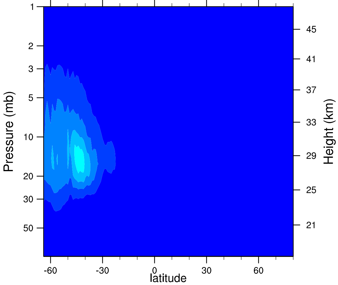
2007d210 N2O5_Ascending (ppbv)
