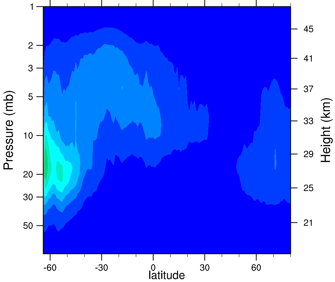
2006d096 N2O5_Ascending (ppbv)
