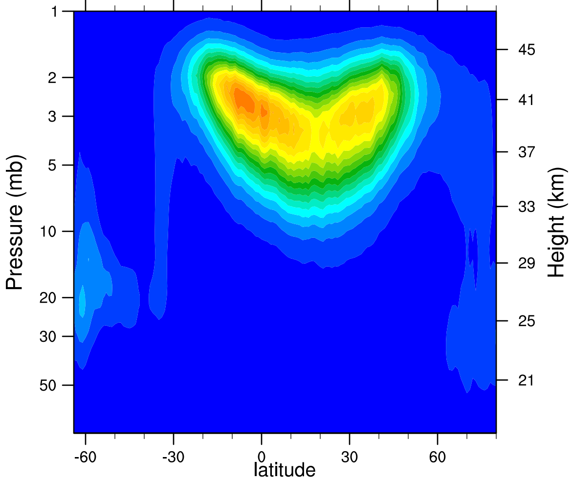
2005d078 N2O5_Ascending (ppbv)
