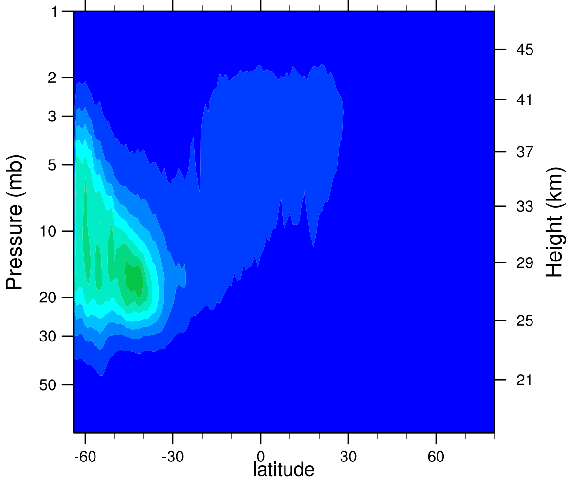
2007d213 N2O5_Ascending (ppbv)
