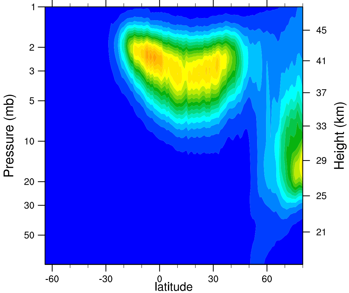
2005d028 N2O5_Ascending (ppbv)
