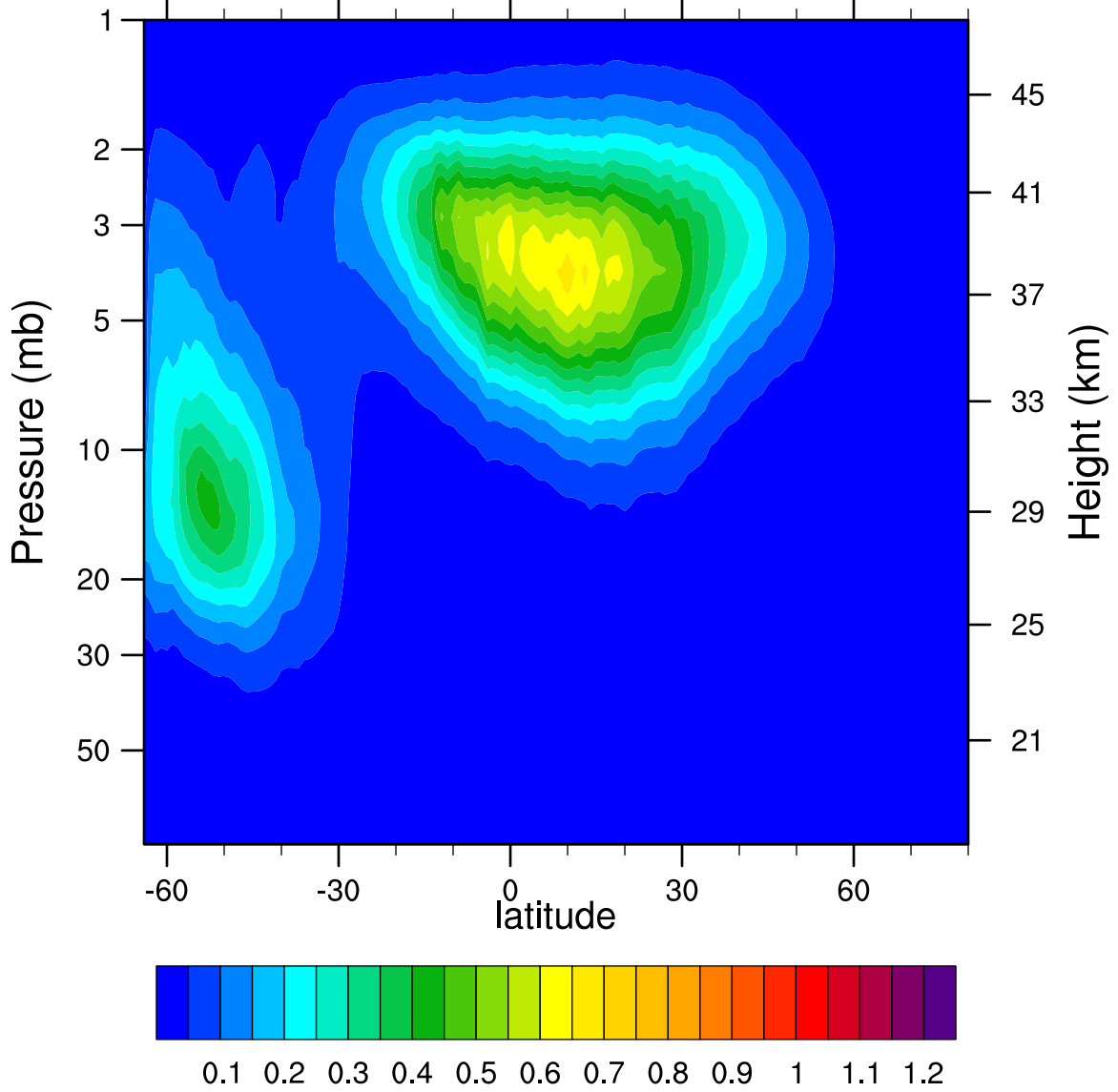
2005d147 N2O5_Ascending (ppbv)
