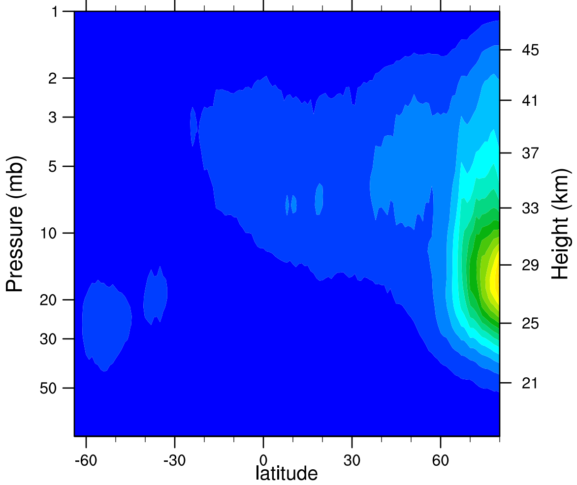
2005d293 N2O5_Ascending (ppbv)
