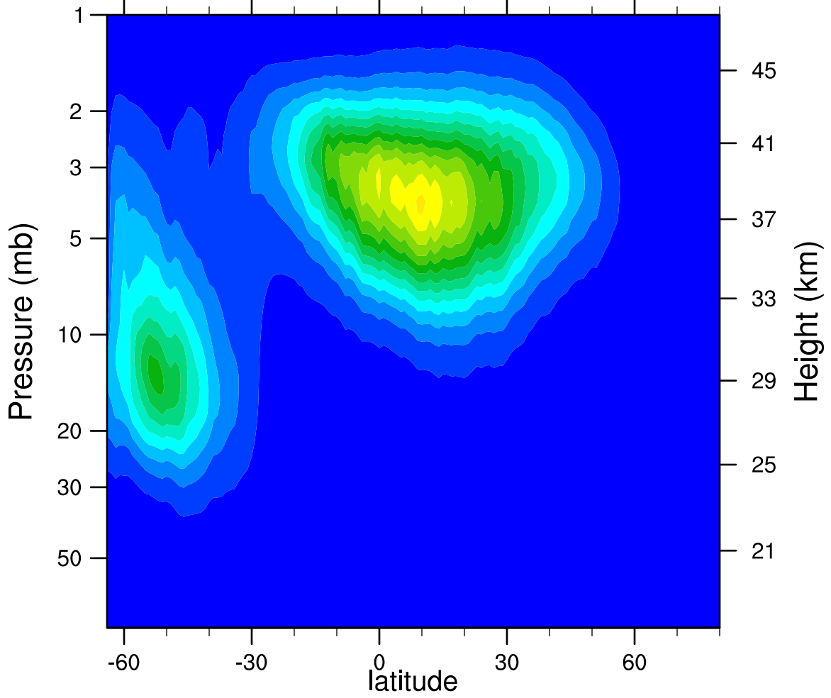
2005d148 N2O5_Ascending (ppbv)
