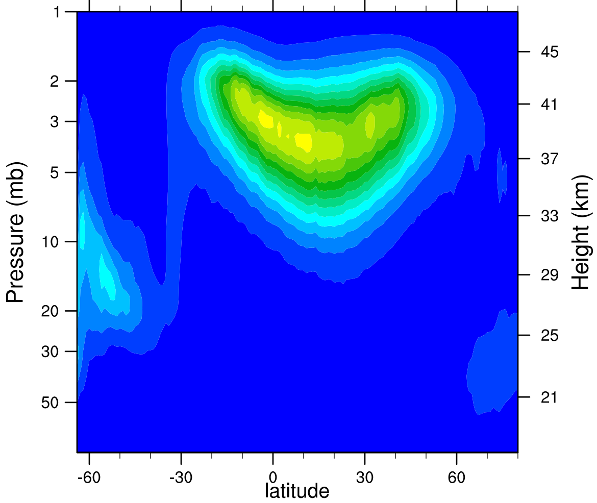
2005d095 N2O5_Ascending (ppbv)
