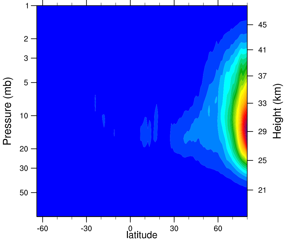
2006d295 N2O5_Ascending (ppbv)
