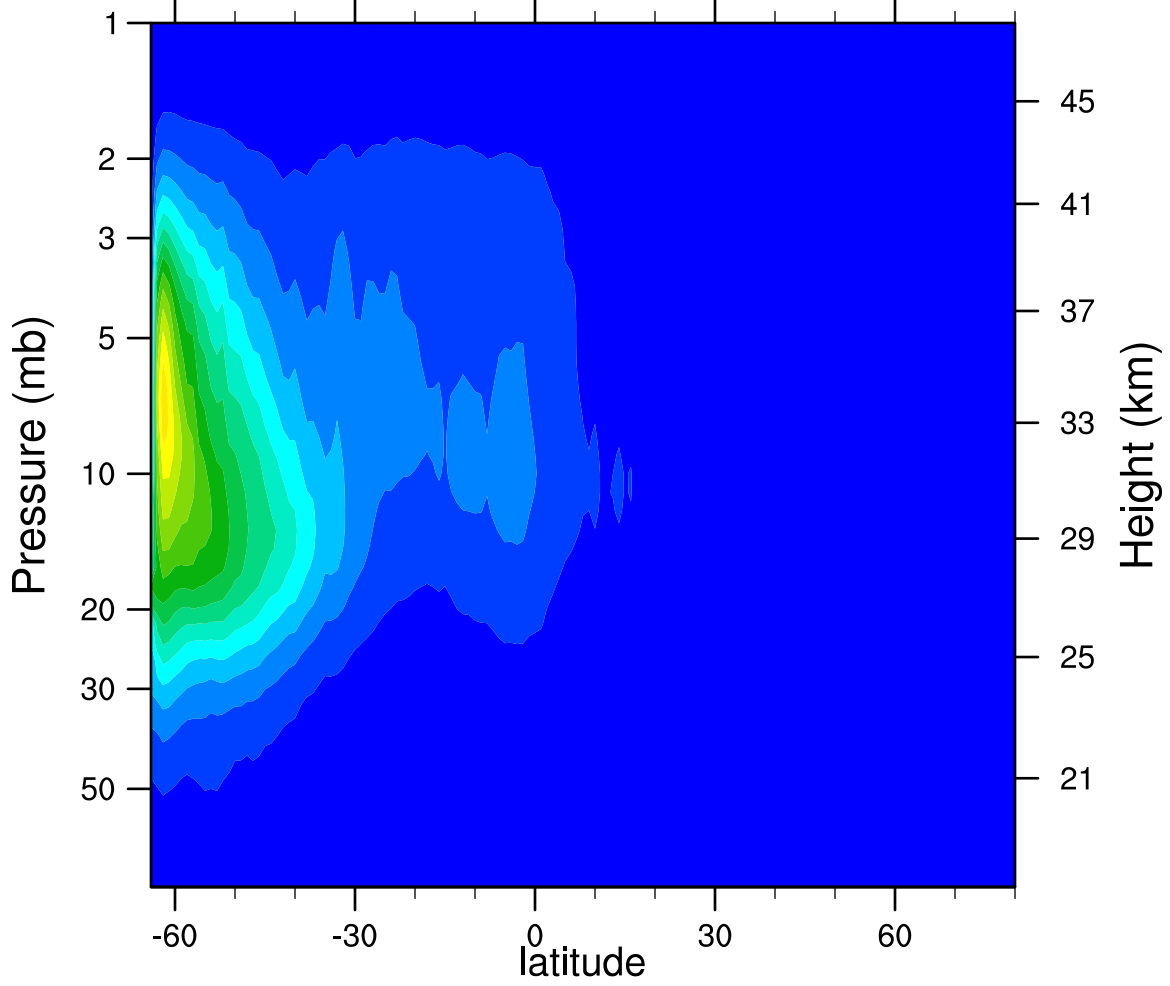
2006d135 N2O5_Ascending (ppbv)
