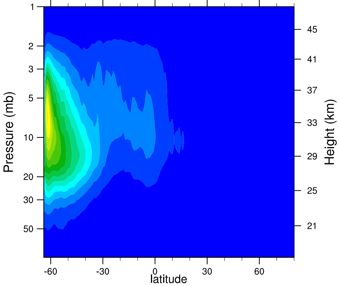
2006d134 N2O5_Ascending (ppbv)
