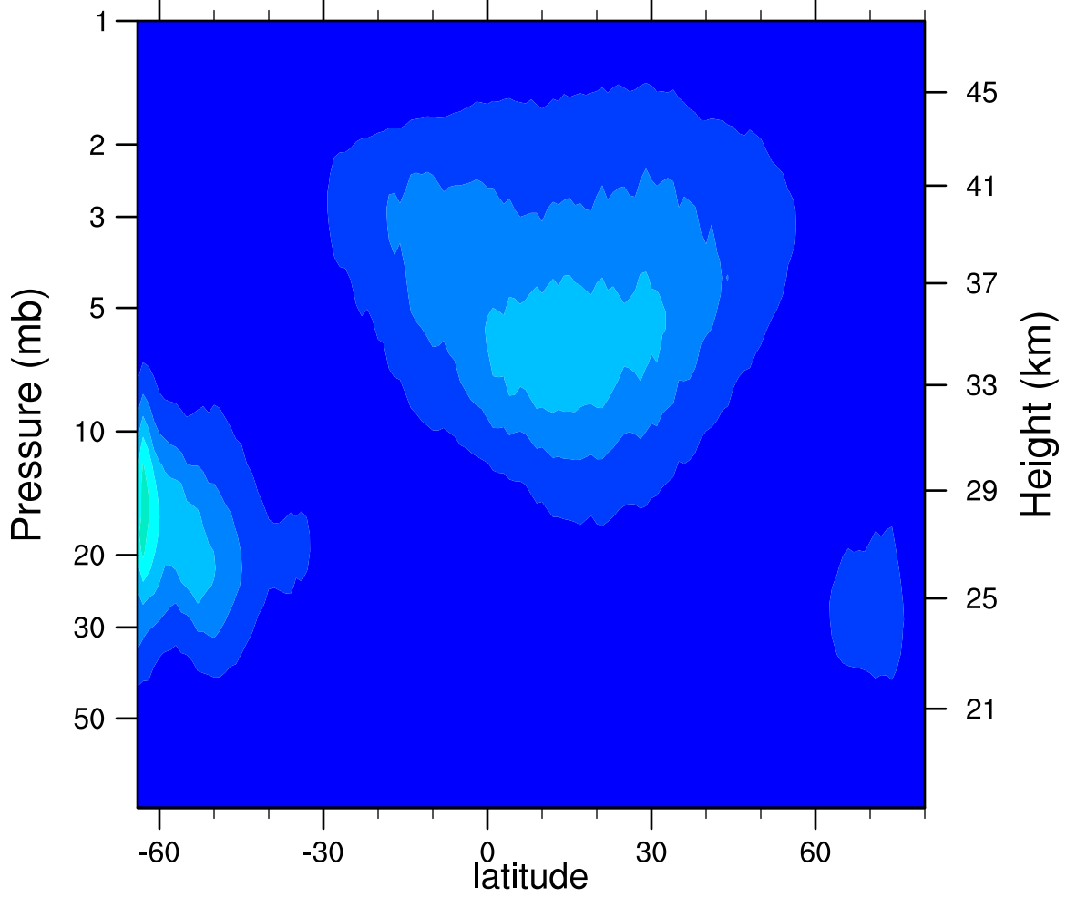
2005d251 N2O5_Ascending (ppbv)
