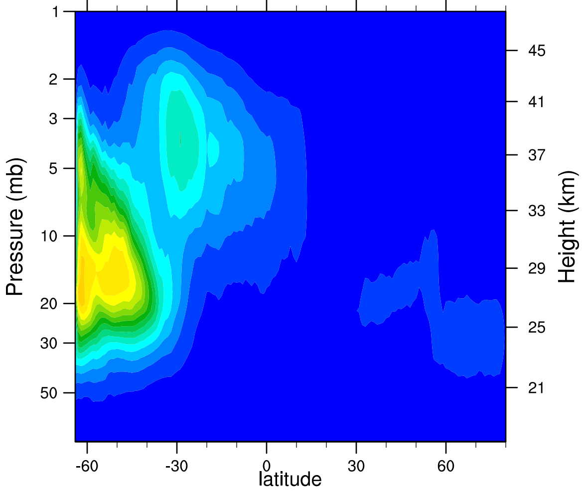
2007d110 N2O5_Ascending (ppbv)
