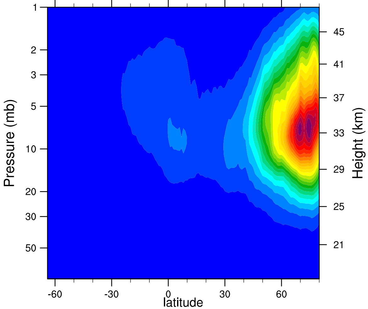
2005d356 N2O5_Ascending (ppbv)
