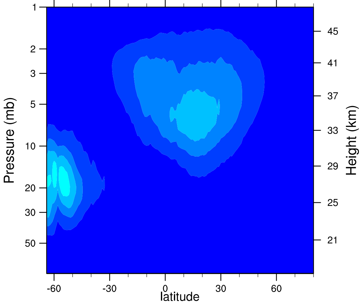
2005d245 N2O5_Ascending (ppbv)
