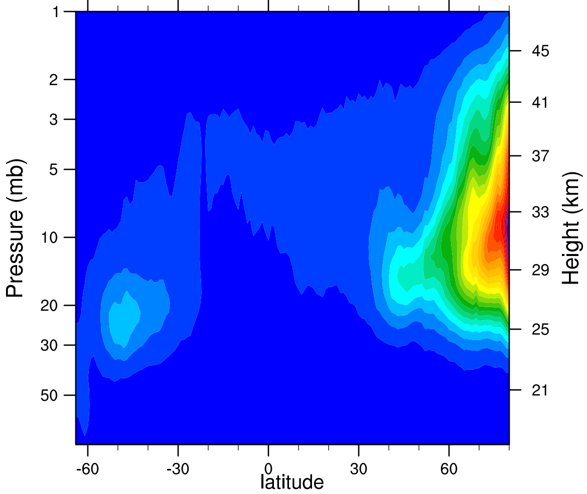
2006d329 N2O5_Ascending (ppbv)
