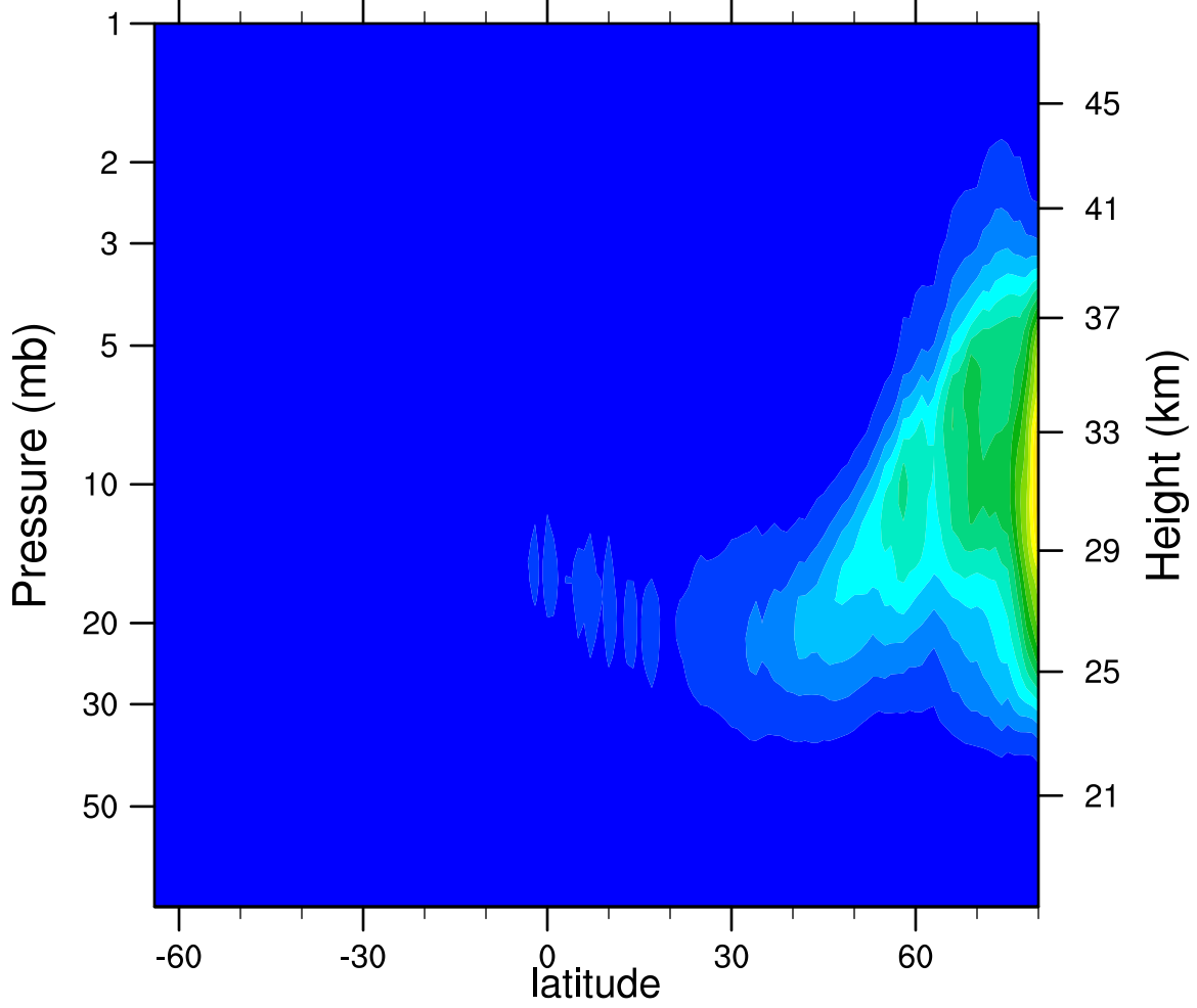
2007d052 N2O5_Ascending (ppbv)
