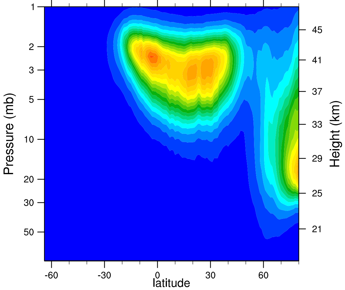
2005d035 N2O5_Ascending (ppbv)
