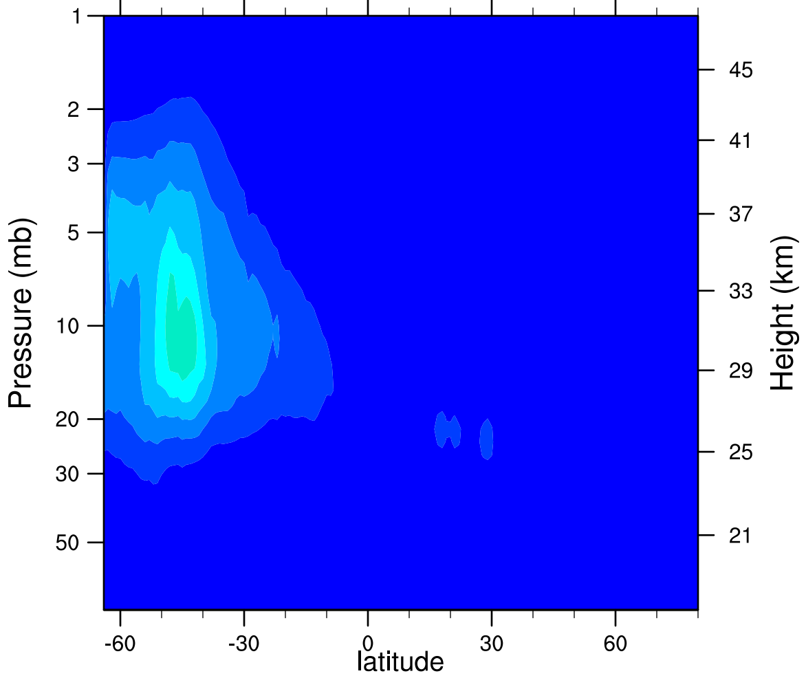
2007d176 N2O5_Ascending (ppbv)
