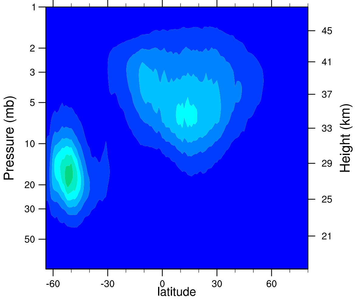
2005d230 N2O5_Ascending (ppbv)
