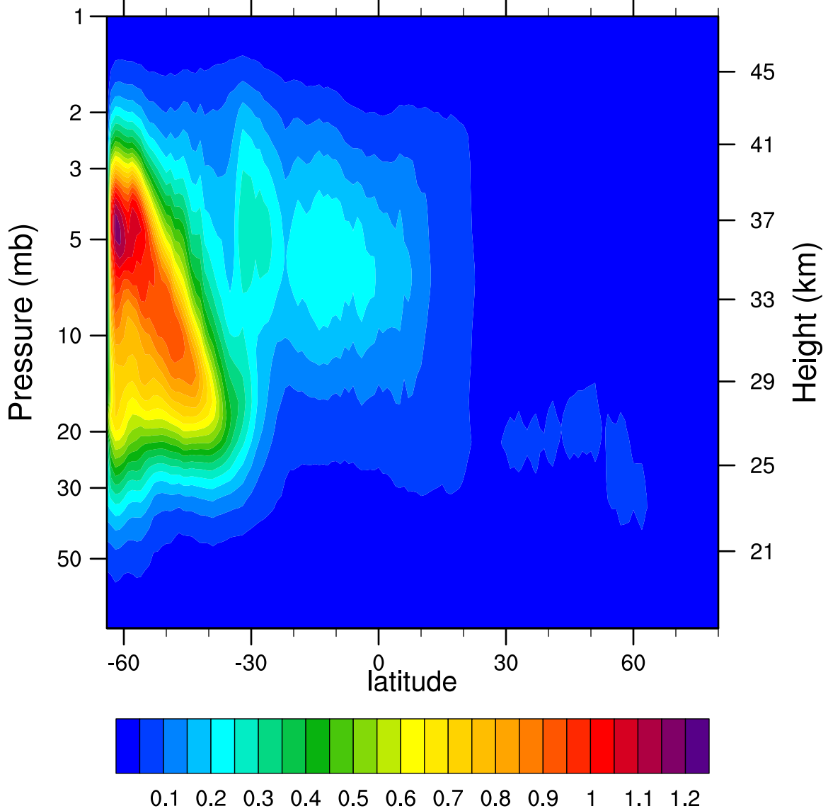
2007d135 N2O5_Ascending (ppbv)
