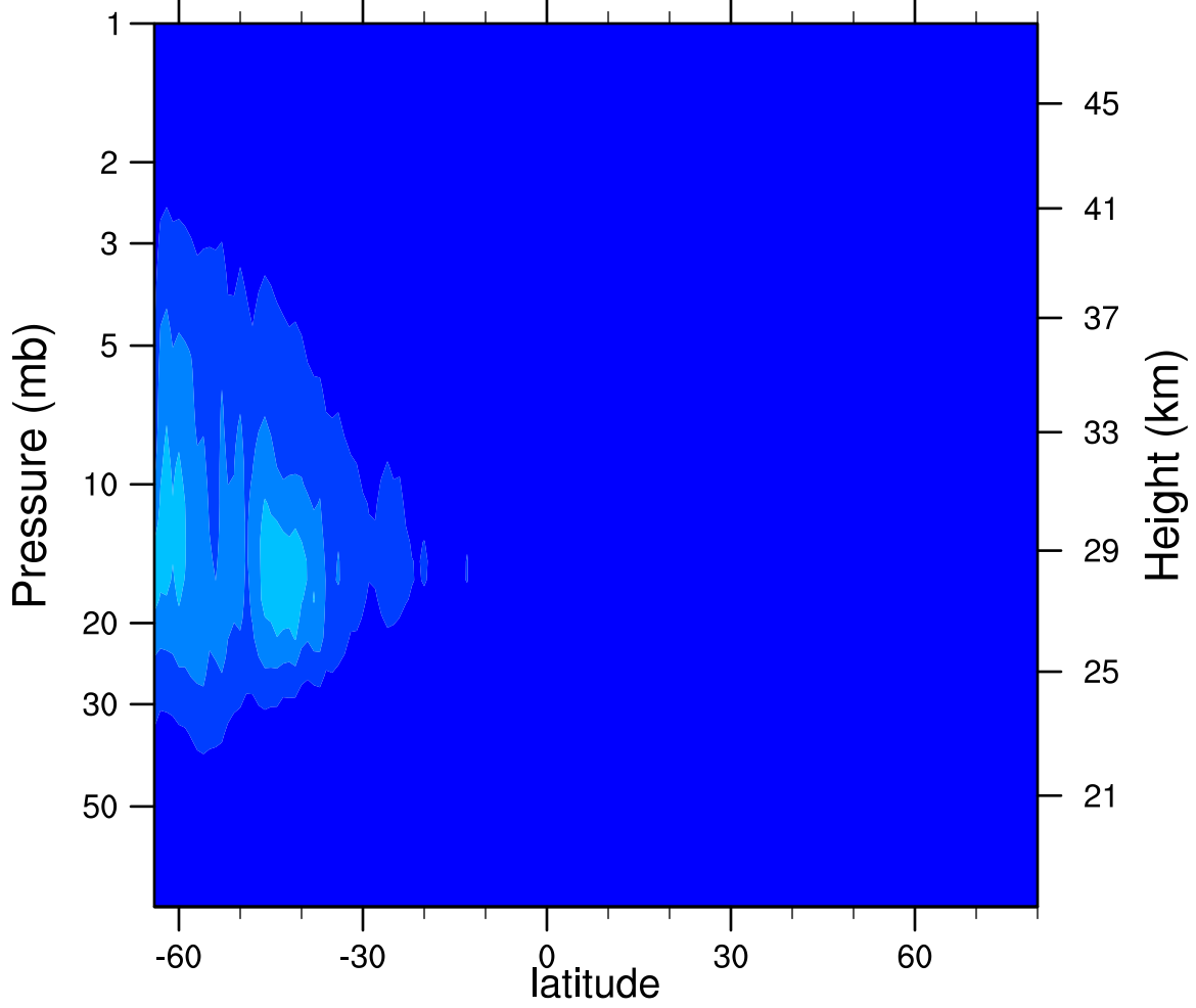
2007d211 N2O5_Ascending (ppbv)
