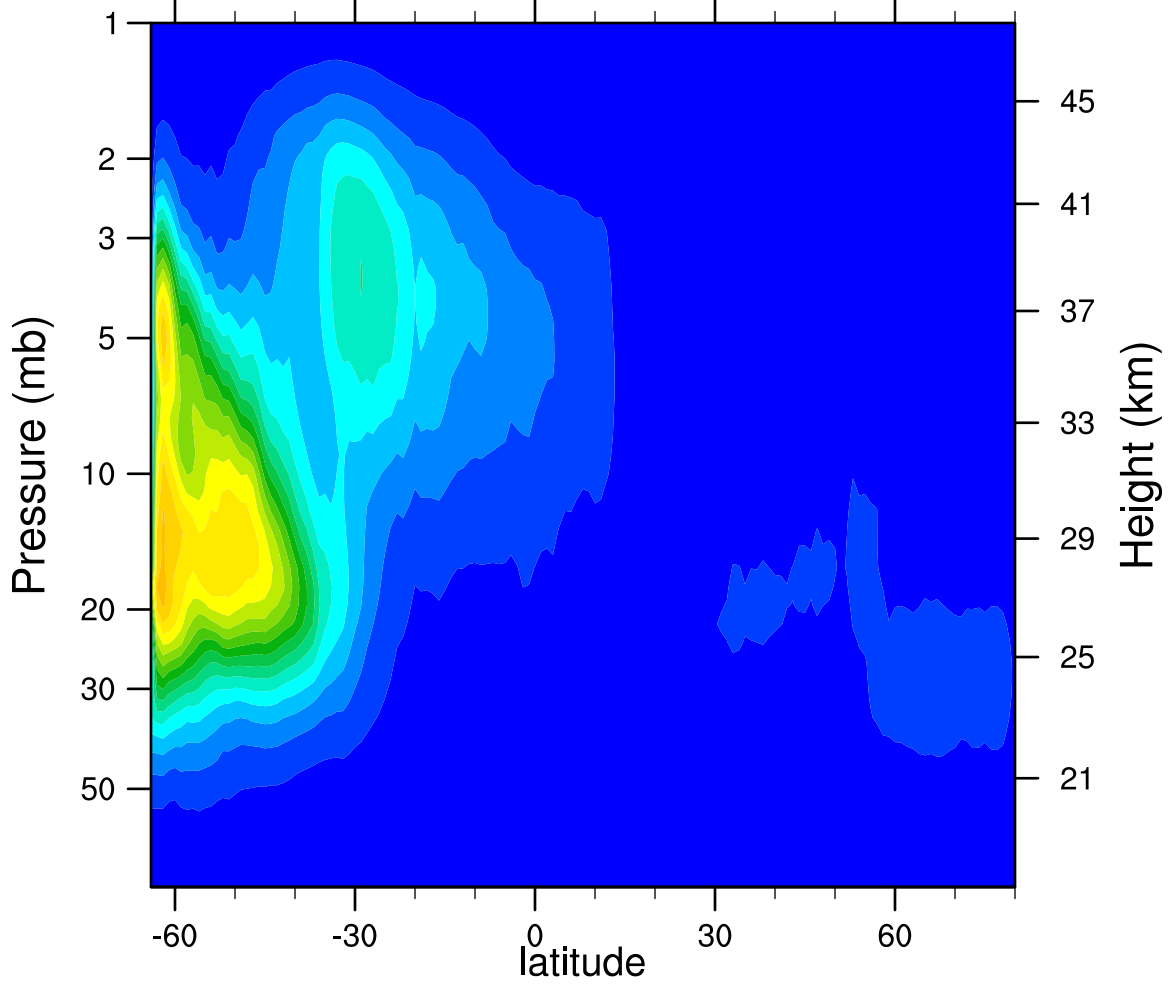
2007d111 N2O5_Ascending (ppbv)
