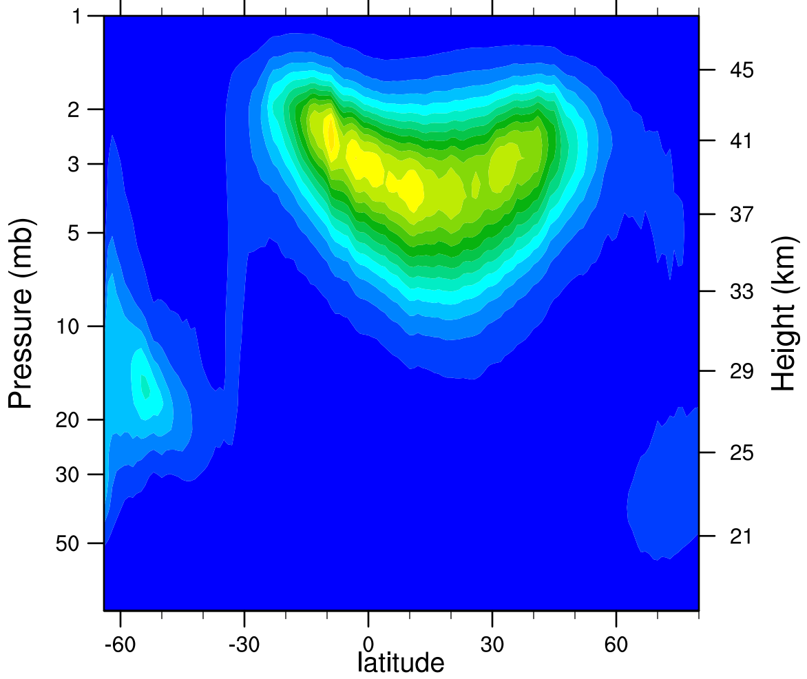
2005d091 N2O5_Ascending (ppbv)
