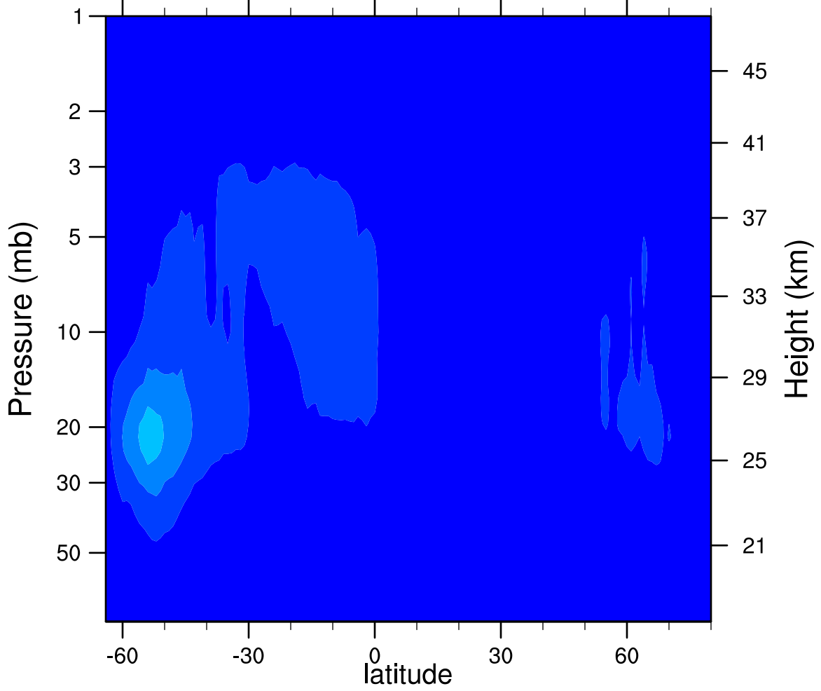
2006d255 N2O5_Ascending (ppbv)
