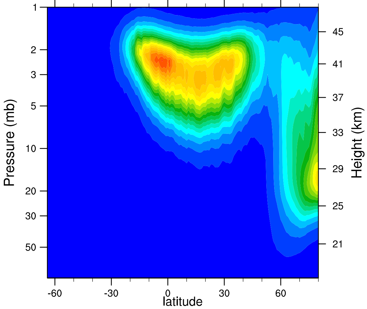
2005d043 N2O5_Ascending (ppbv)
