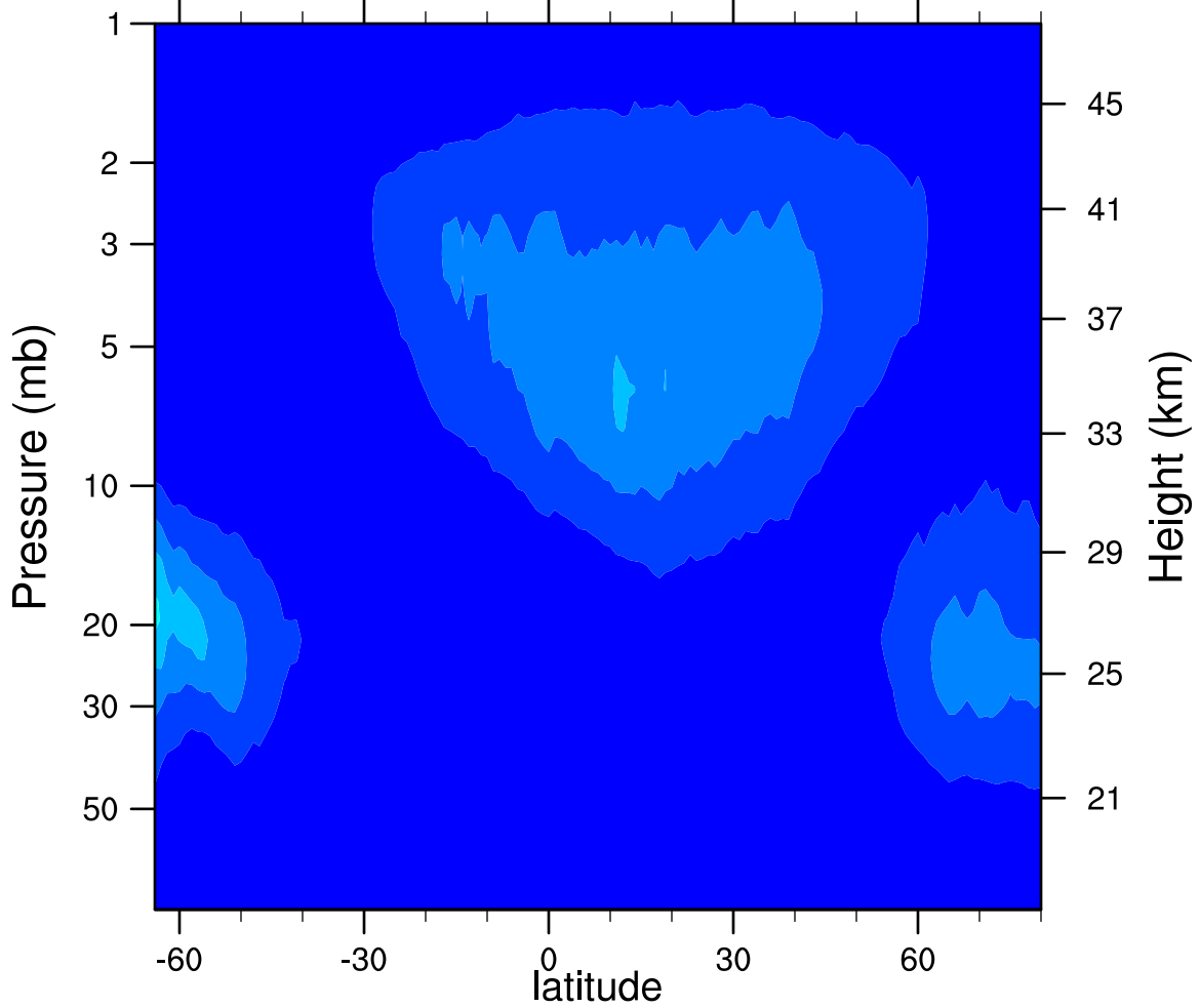
2005d268 N2O5_Ascending (ppbv)
