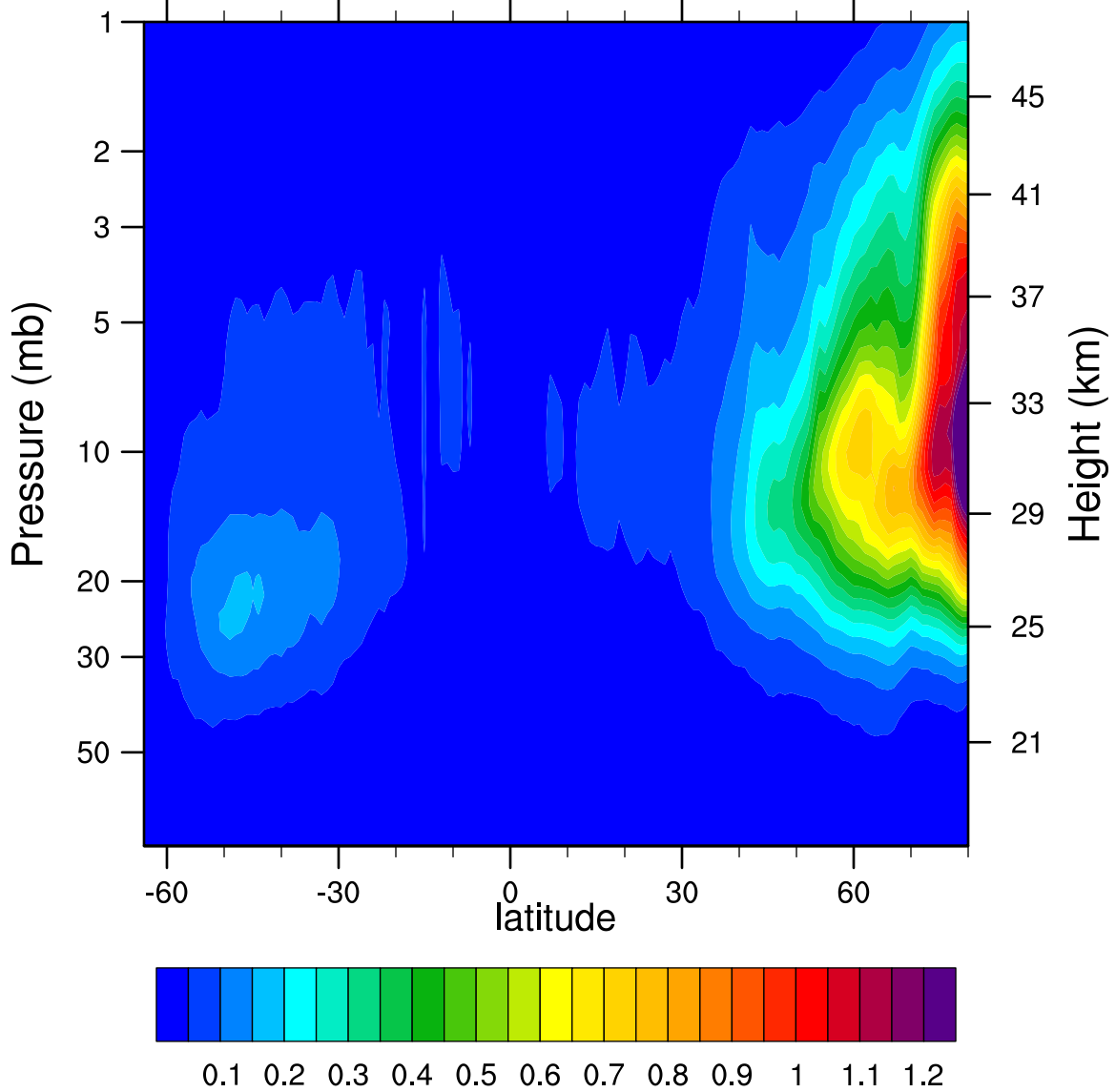
2006d336 N2O5_Ascending (ppbv)
