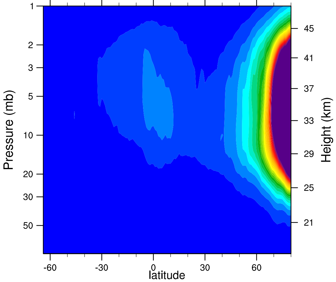
2006d023 N2O5_Ascending (ppbv)
