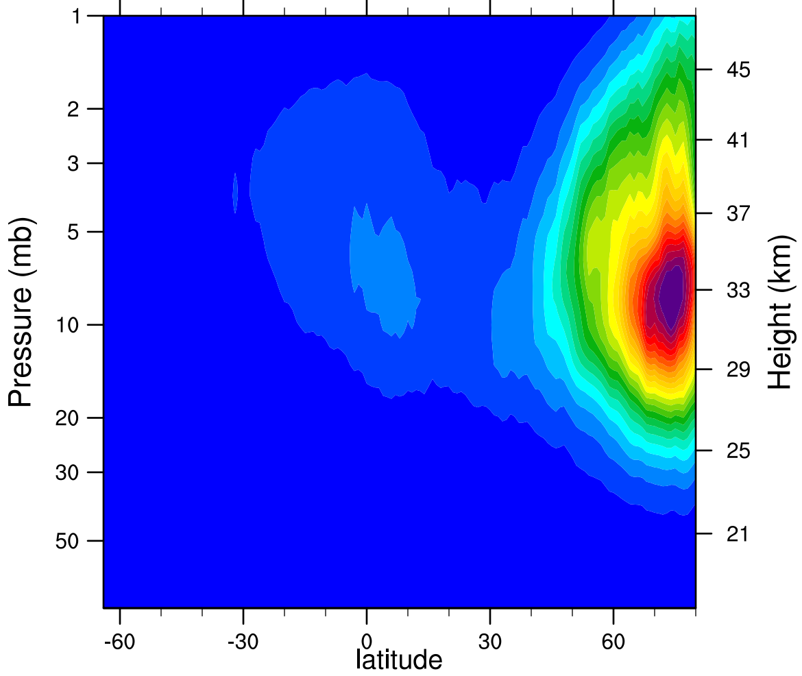
2006d002 N2O5_Ascending (ppbv)
