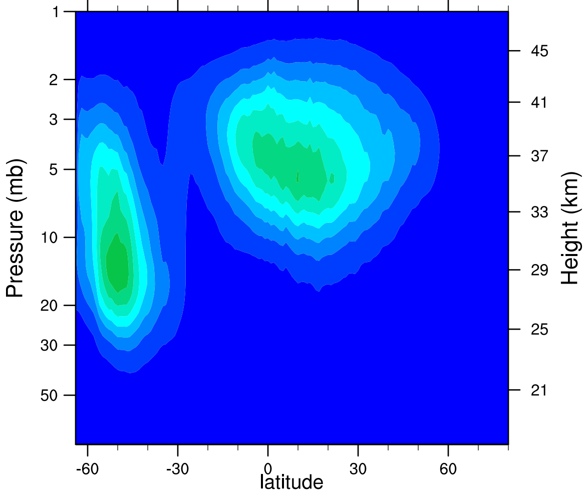
2005d193 N2O5_Ascending (ppbv)
