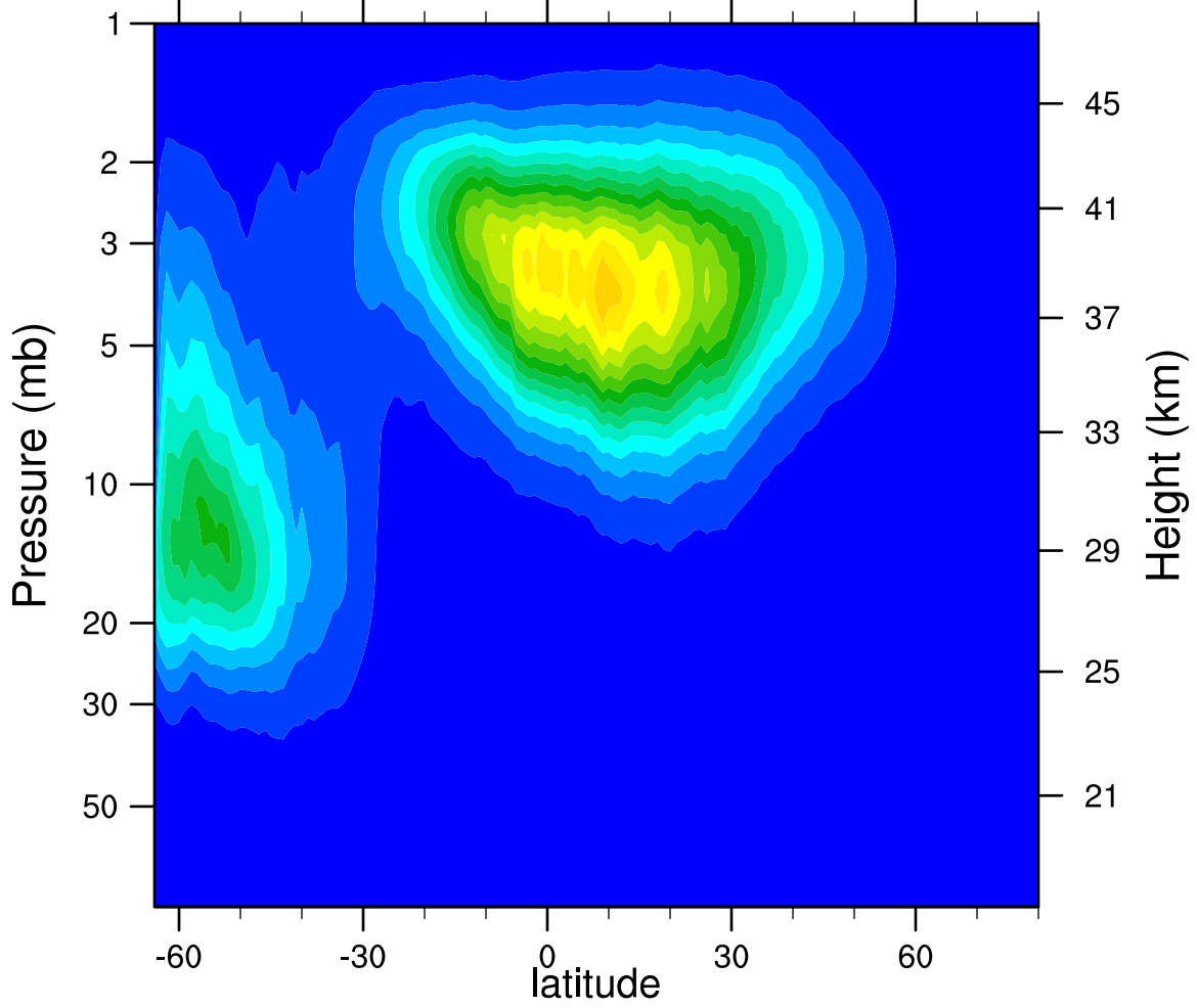
2005d144 N2O5_Ascending (ppbv)
