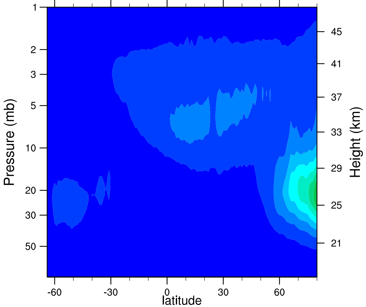
2005d282 N2O5_Ascending (ppbv)
