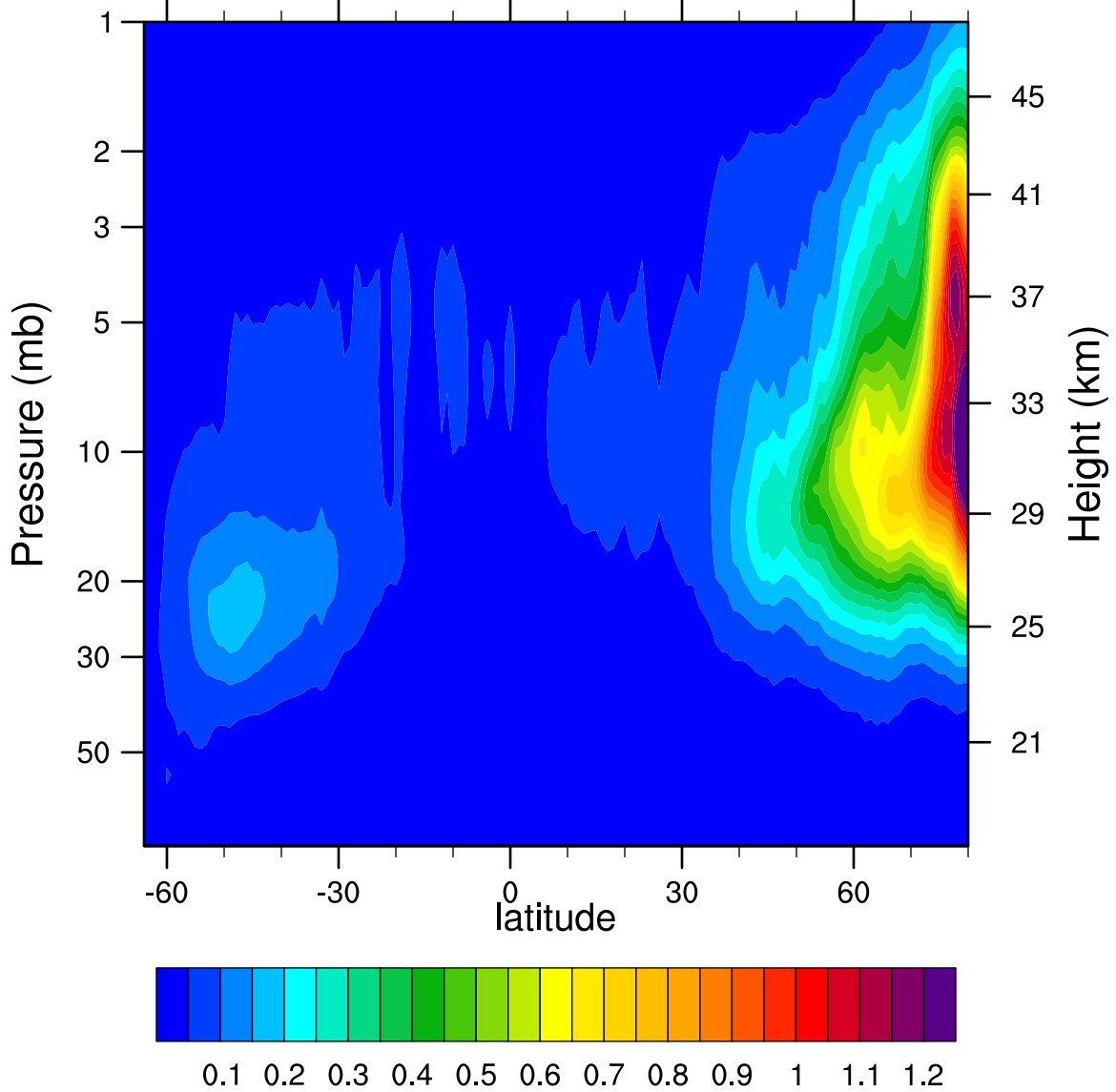
2006d334 N2O5_Ascending (ppbv)
