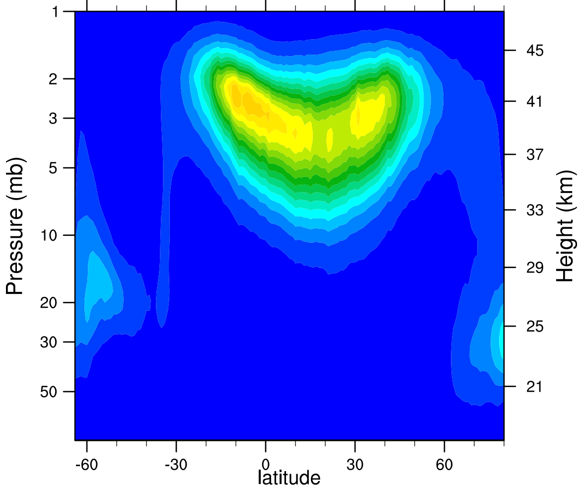
2005d083 N2O5_Ascending (ppbv)
