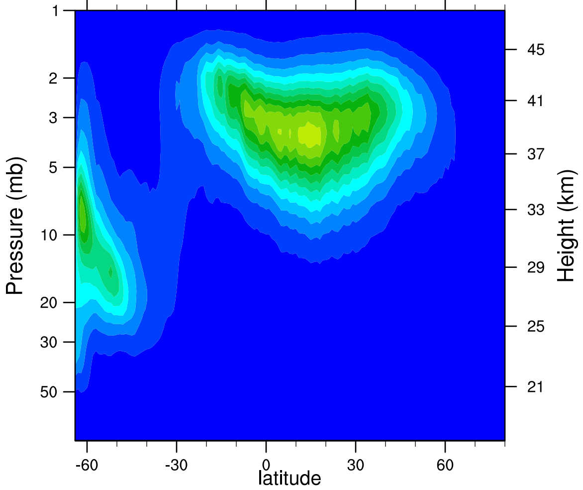
2005d112 N2O5_Ascending (ppbv)
