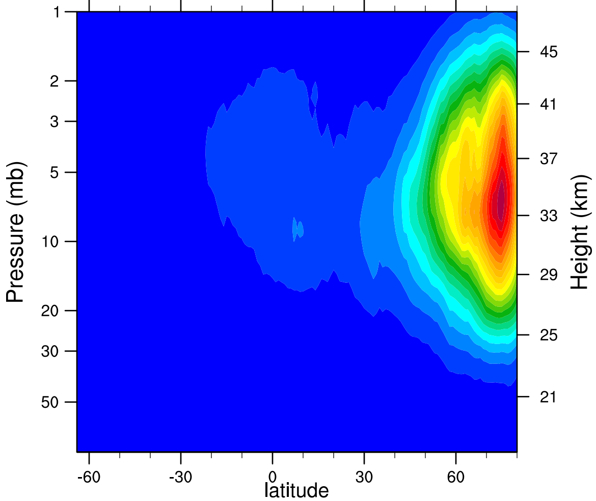
2005d340 N2O5_Ascending (ppbv)
