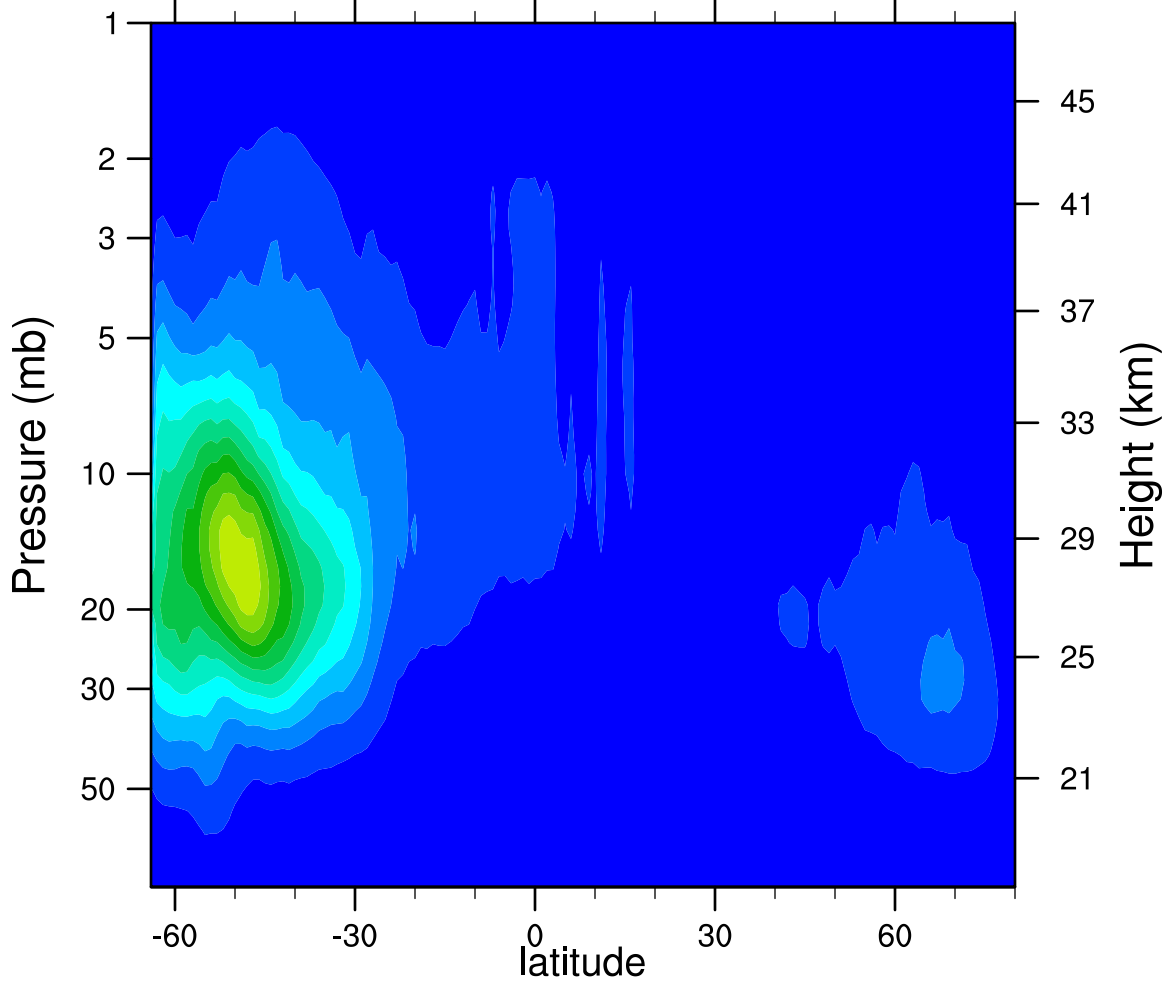
2007d238 N2O5_Ascending (ppbv)
