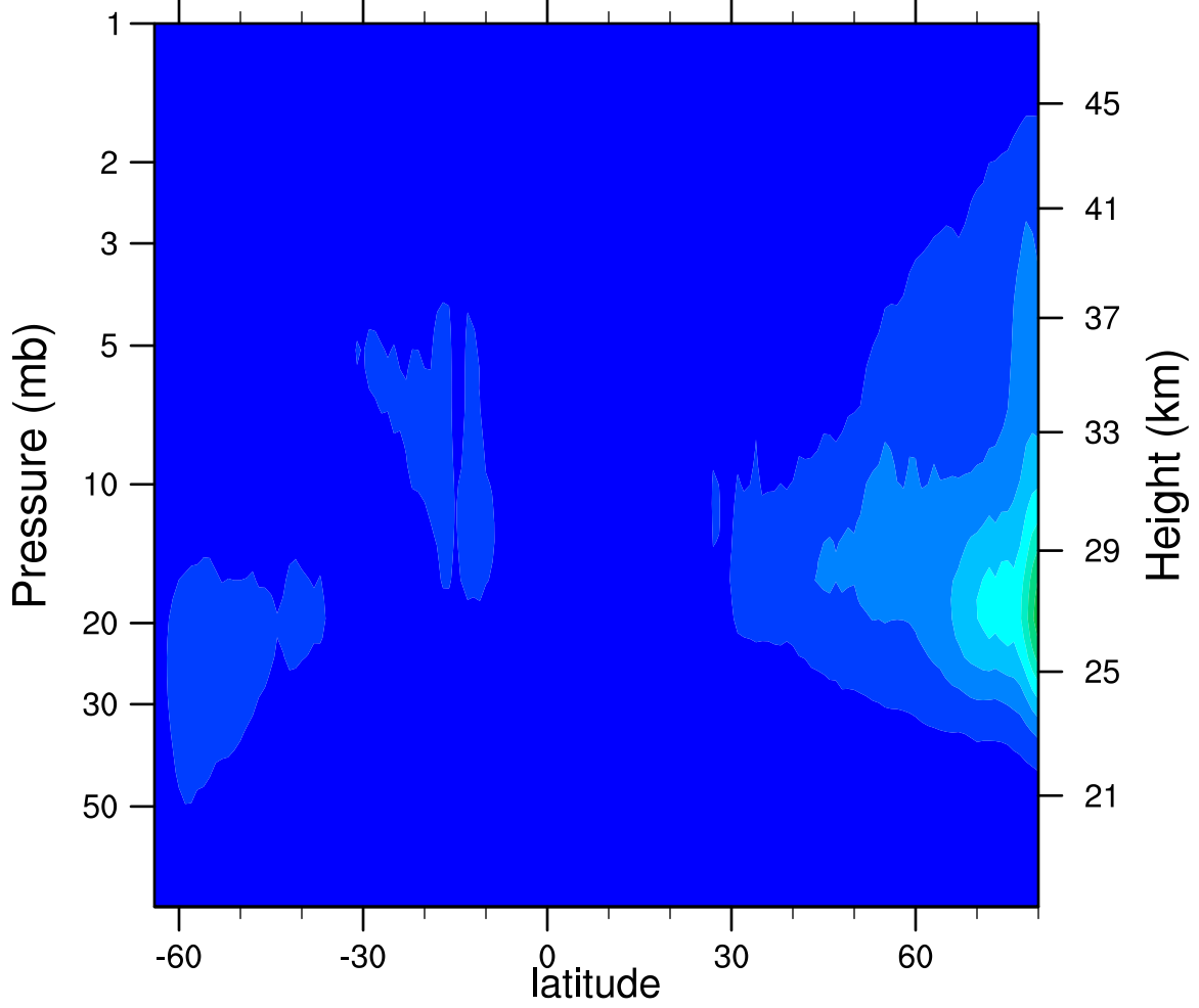
2006d280 N2O5_Ascending (ppbv)
