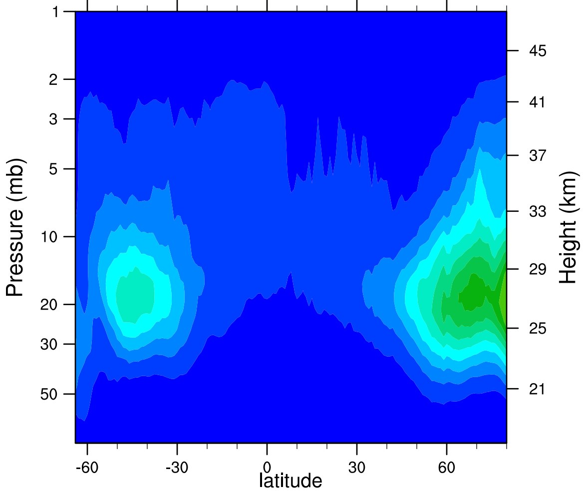
2007d274 N2O5_Ascending (ppbv)
