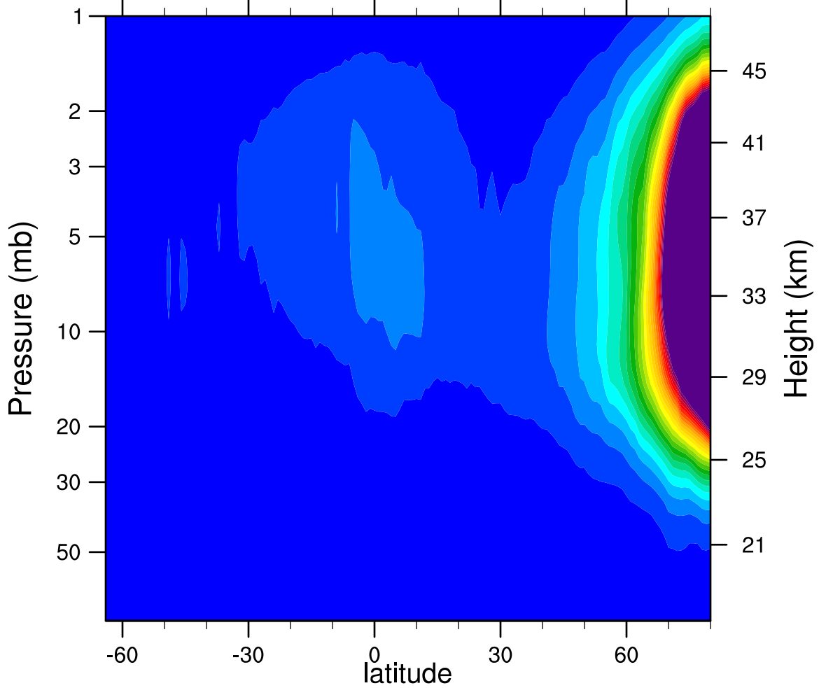
2006d024 N2O5_Ascending (ppbv)
