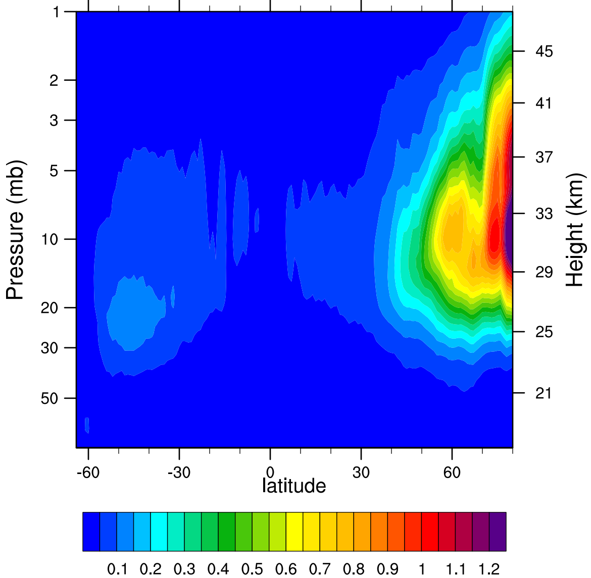
2006d340 N2O5_Ascending (ppbv)
