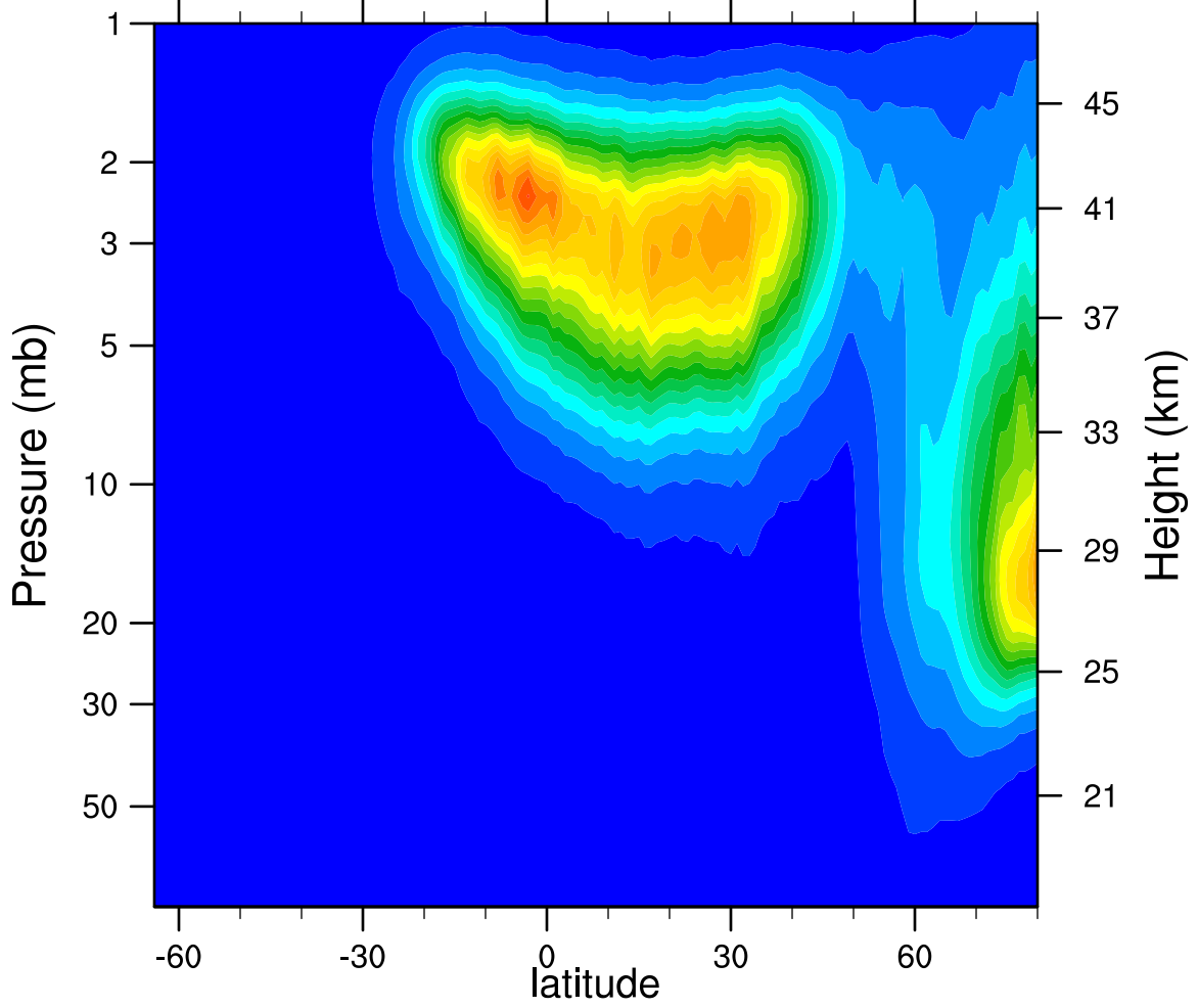
2005d031 N2O5_Ascending (ppbv)
