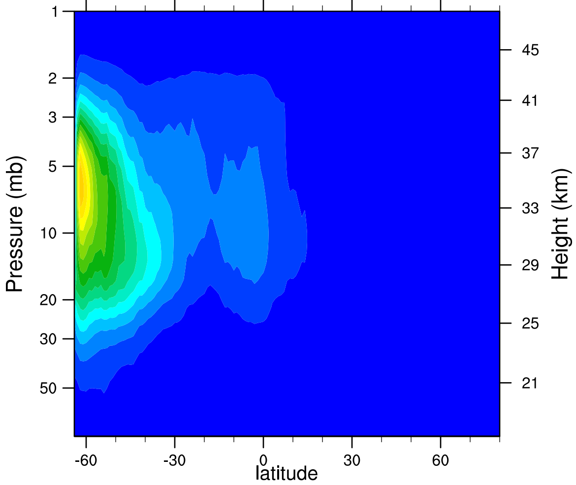
2006d143 N2O5_Ascending (ppbv)
