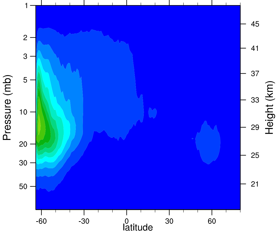
2006d114 N2O5_Ascending (ppbv)
