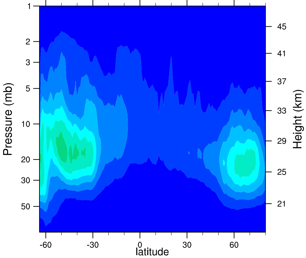
2007d259 N2O5_Ascending (ppbv)
