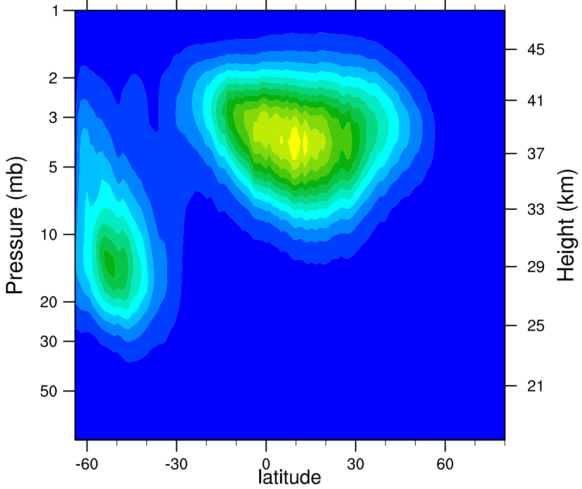
2005d149 N2O5_Ascending (ppbv)
