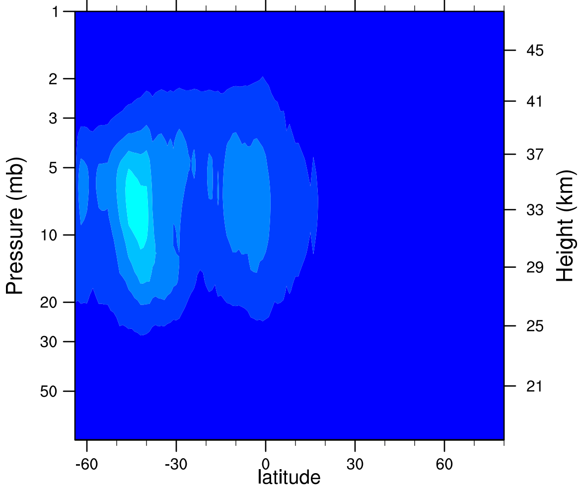
2006d192 N2O5_Ascending (ppbv)
