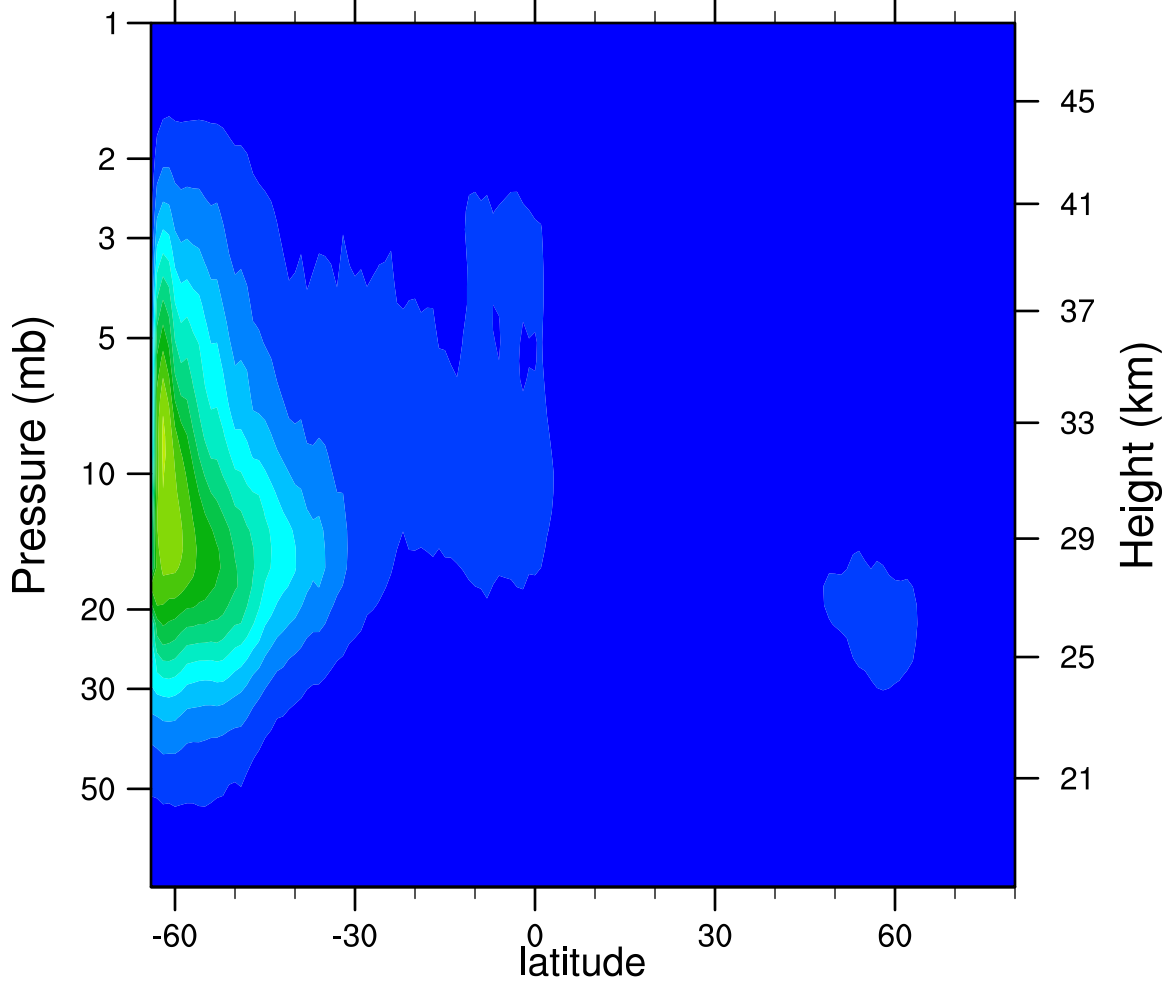
2006d120 N2O5_Ascending (ppbv)
