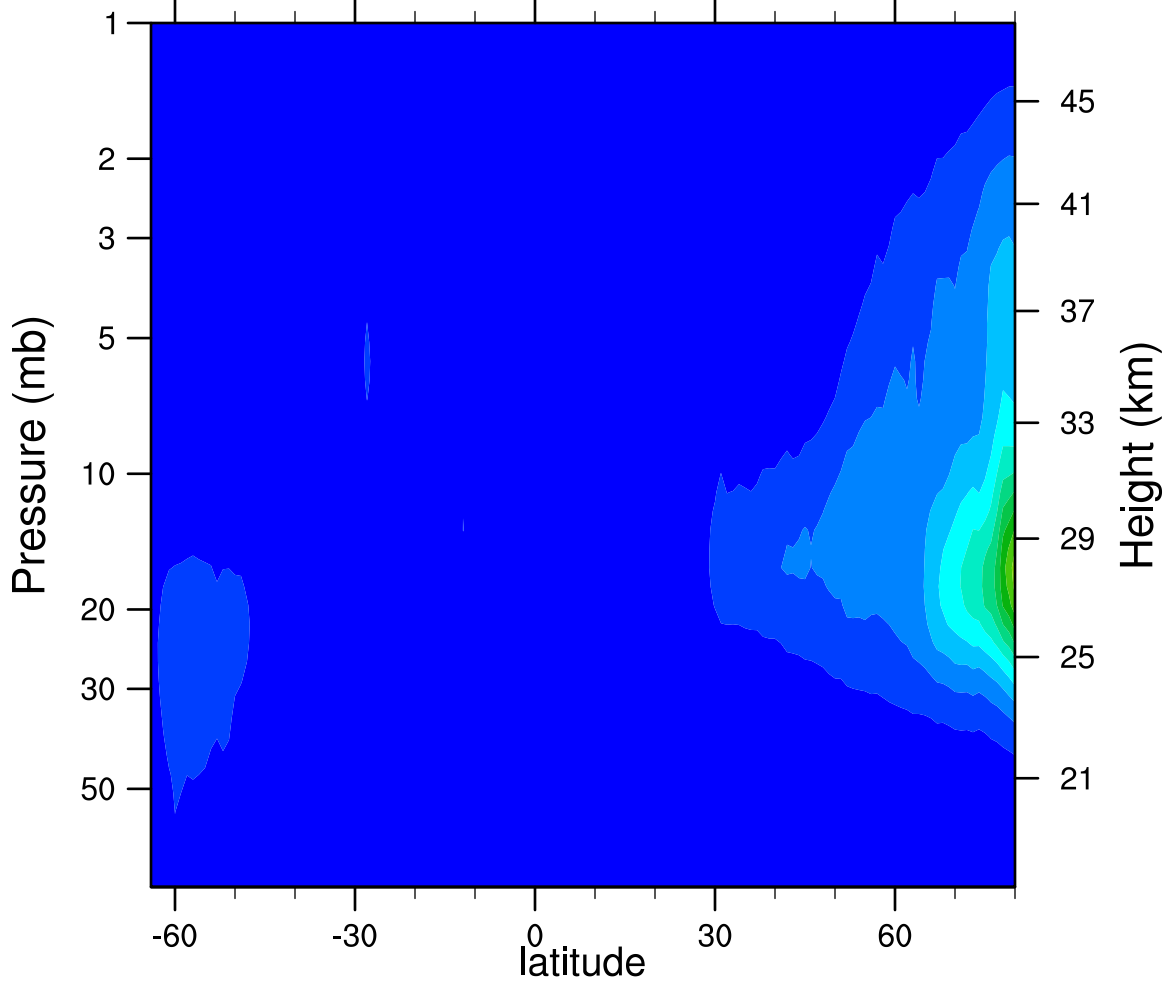
2006d286 N2O5_Ascending (ppbv)
