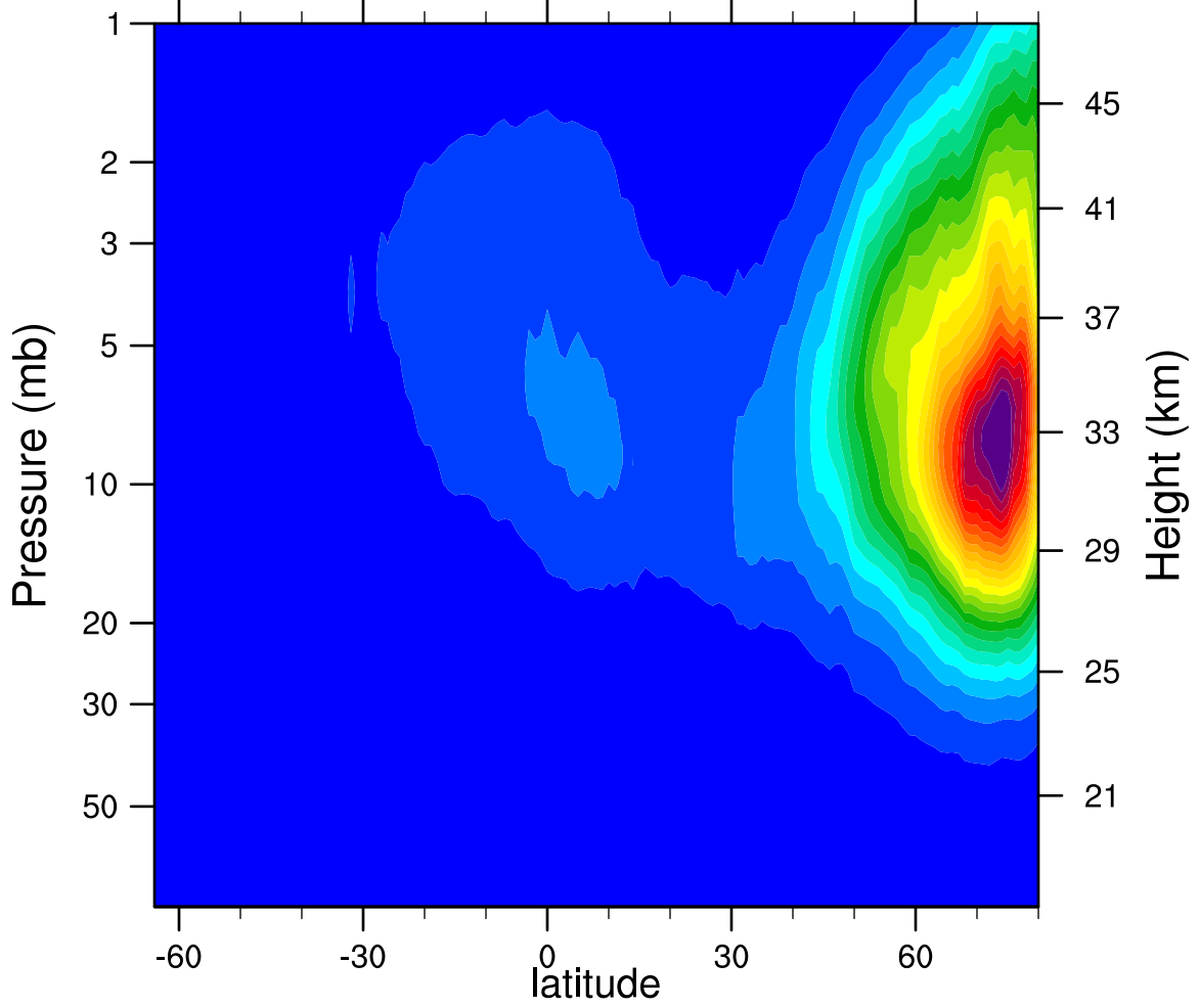
2006d001 N2O5_Ascending (ppbv)
