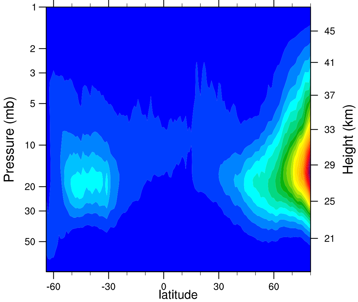
2007d288 N2O5_Ascending (ppbv)
