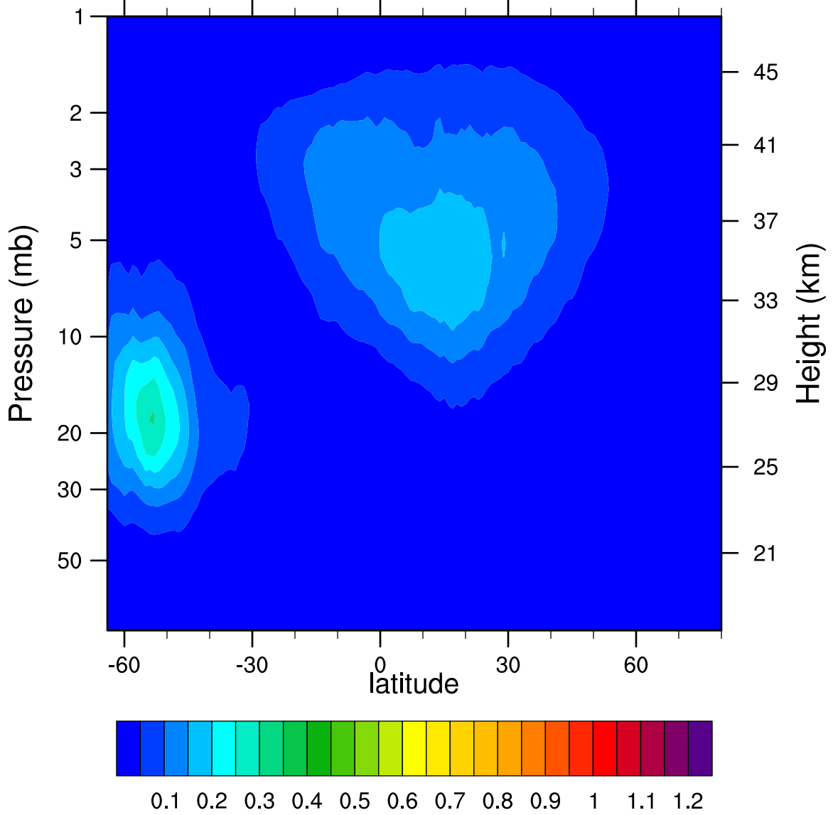
2005d236 N2O5_Ascending (ppbv)
