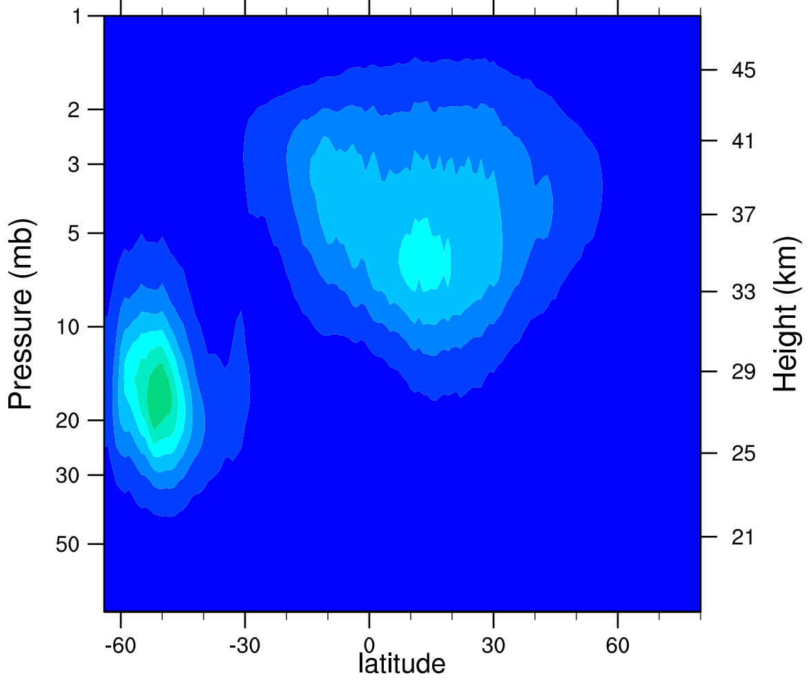
2005d229 N2O5_Ascending (ppbv)
