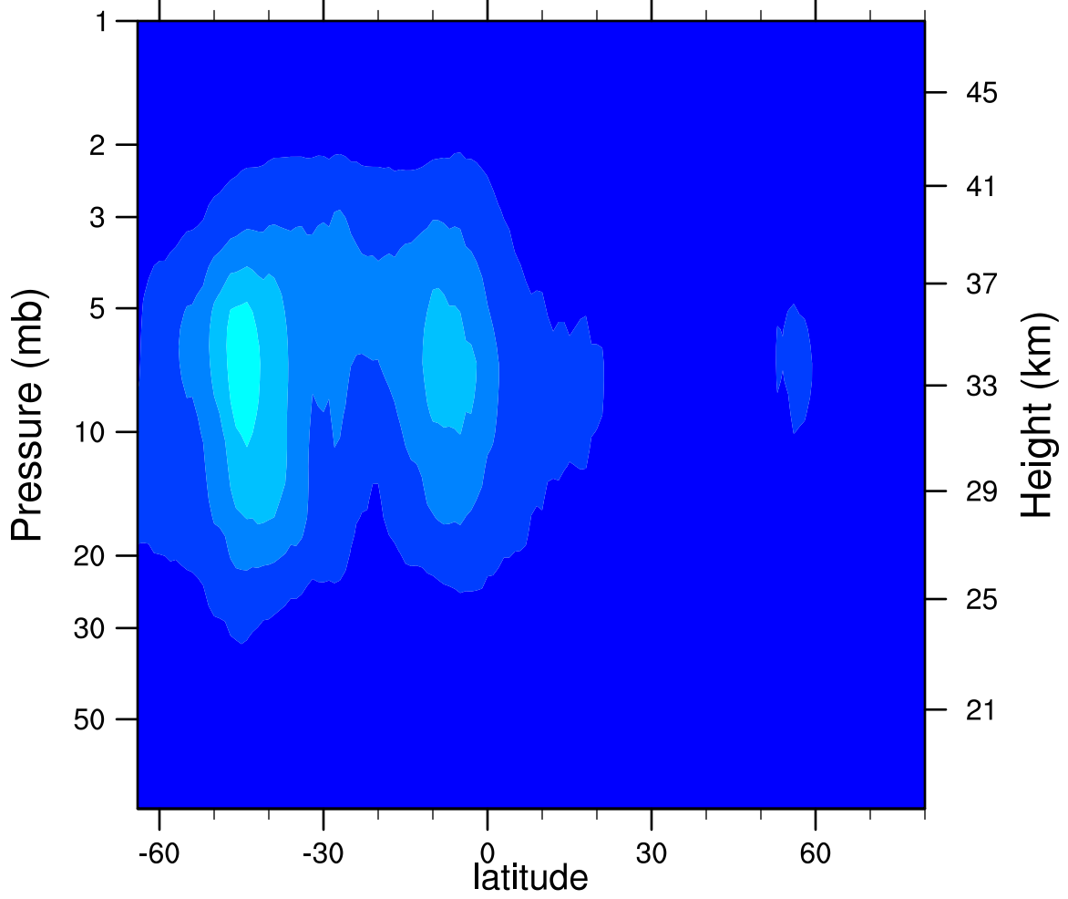
2006d208 N2O5_Ascending (ppbv)
