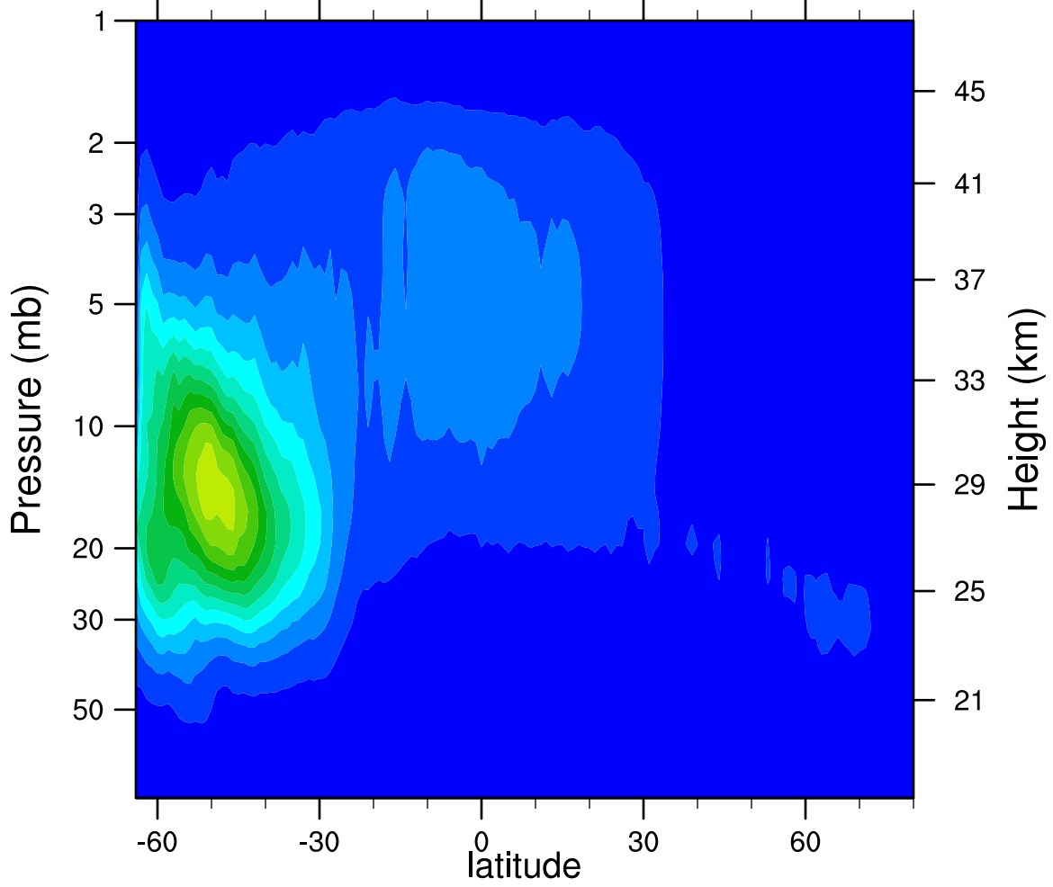
2007d231 N2O5_Ascending (ppbv)
