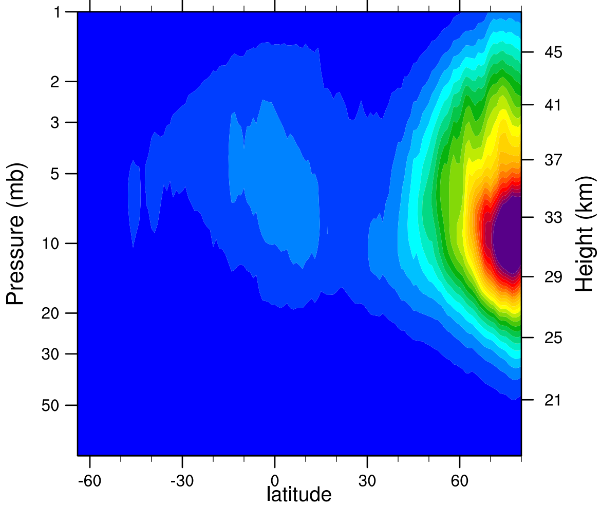
2006d010 N2O5_Ascending (ppbv)
