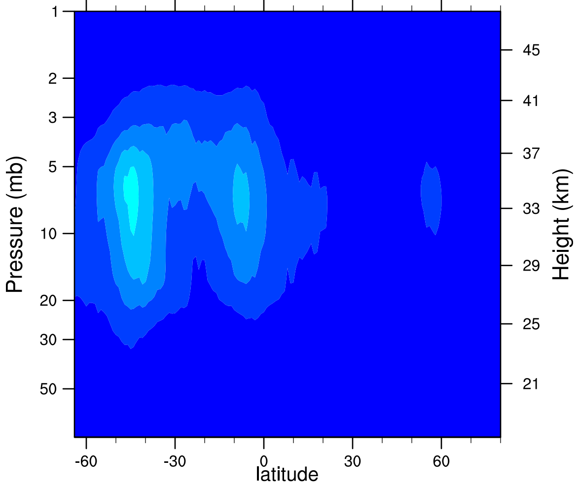
2006d210 N2O5_Ascending (ppbv)
