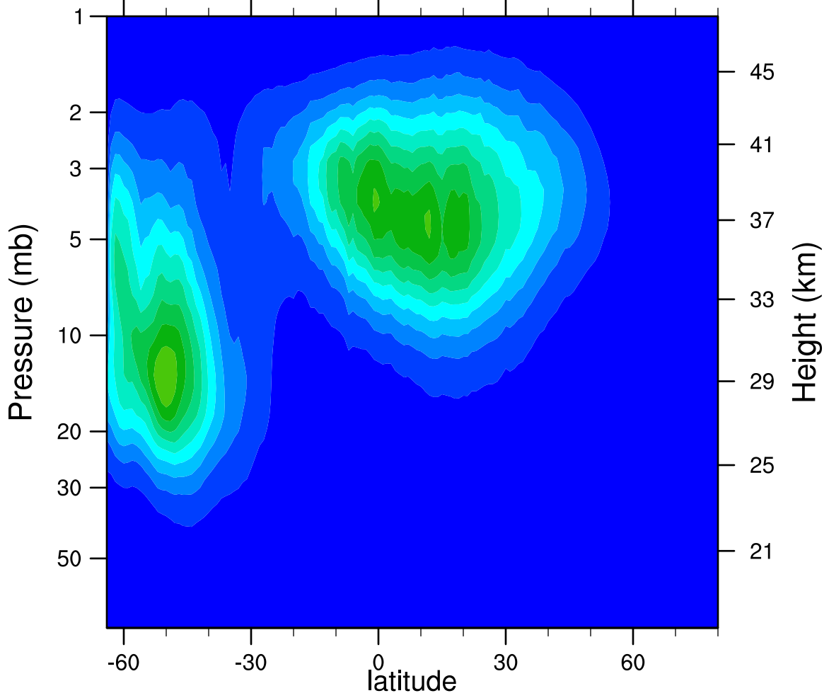
2005d168 N2O5_Ascending (ppbv)
