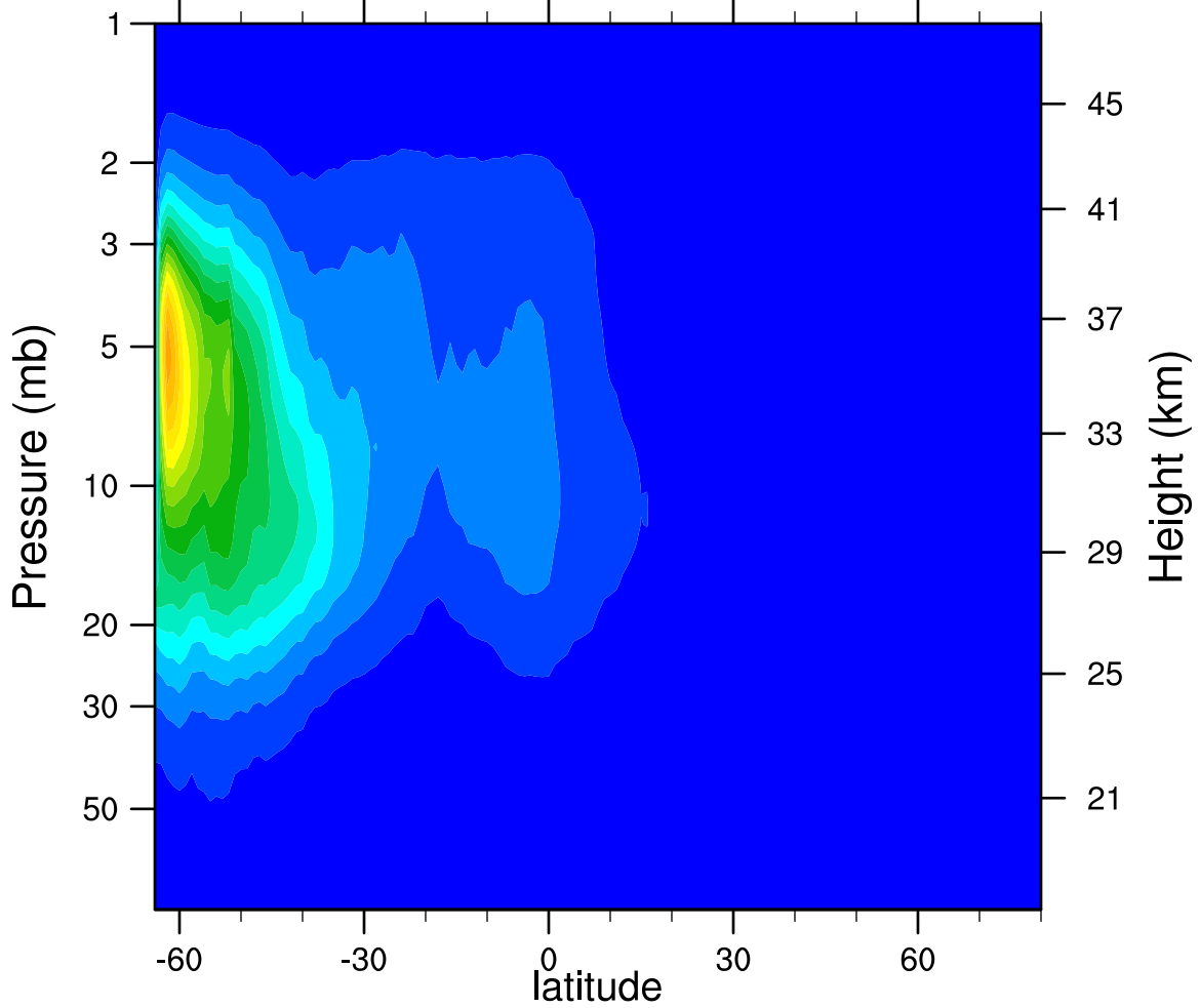
2006d147 N2O5_Ascending (ppbv)
