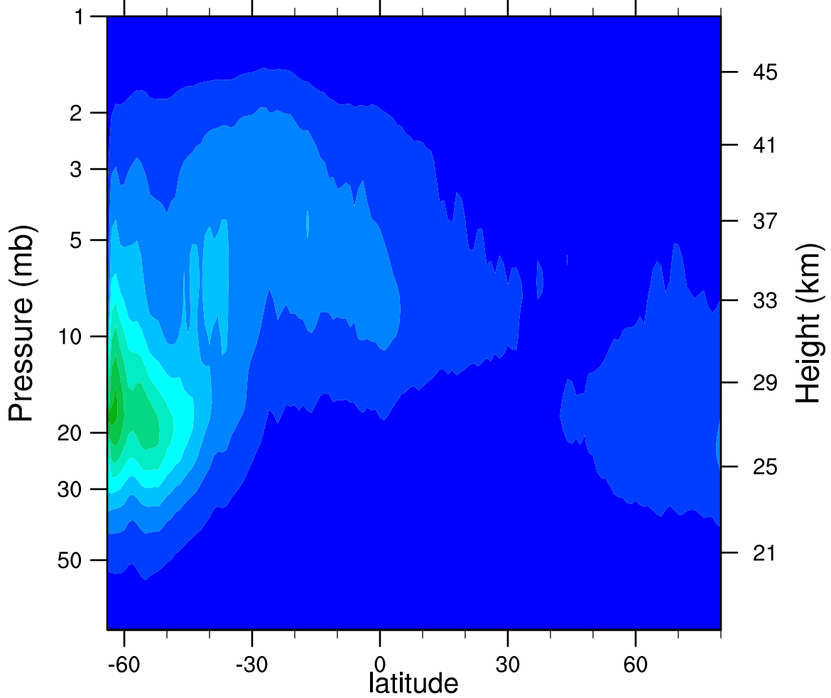
2006d099 N2O5_Ascending (ppbv)
