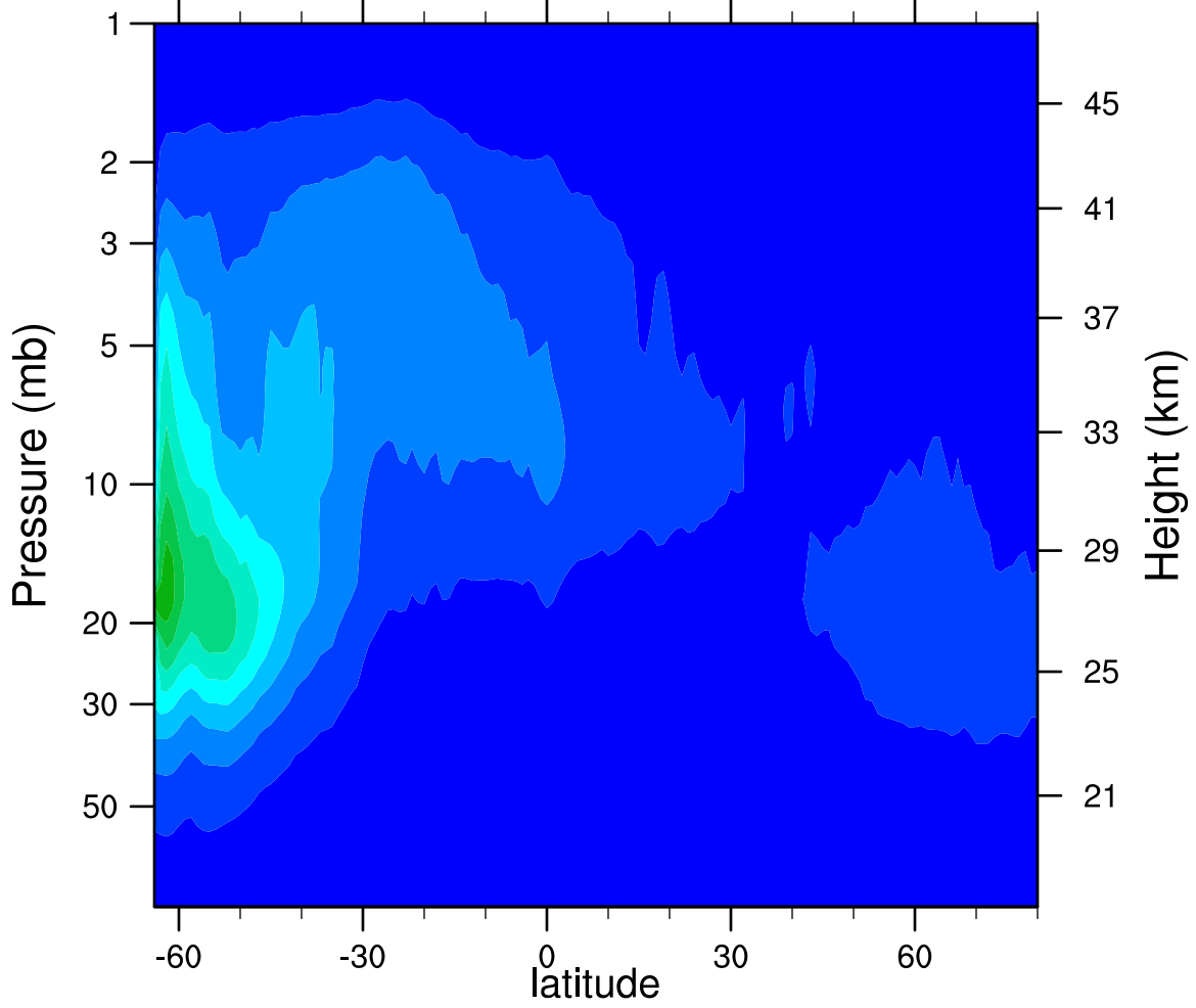
2006d103 N2O5_Ascending (ppbv)
