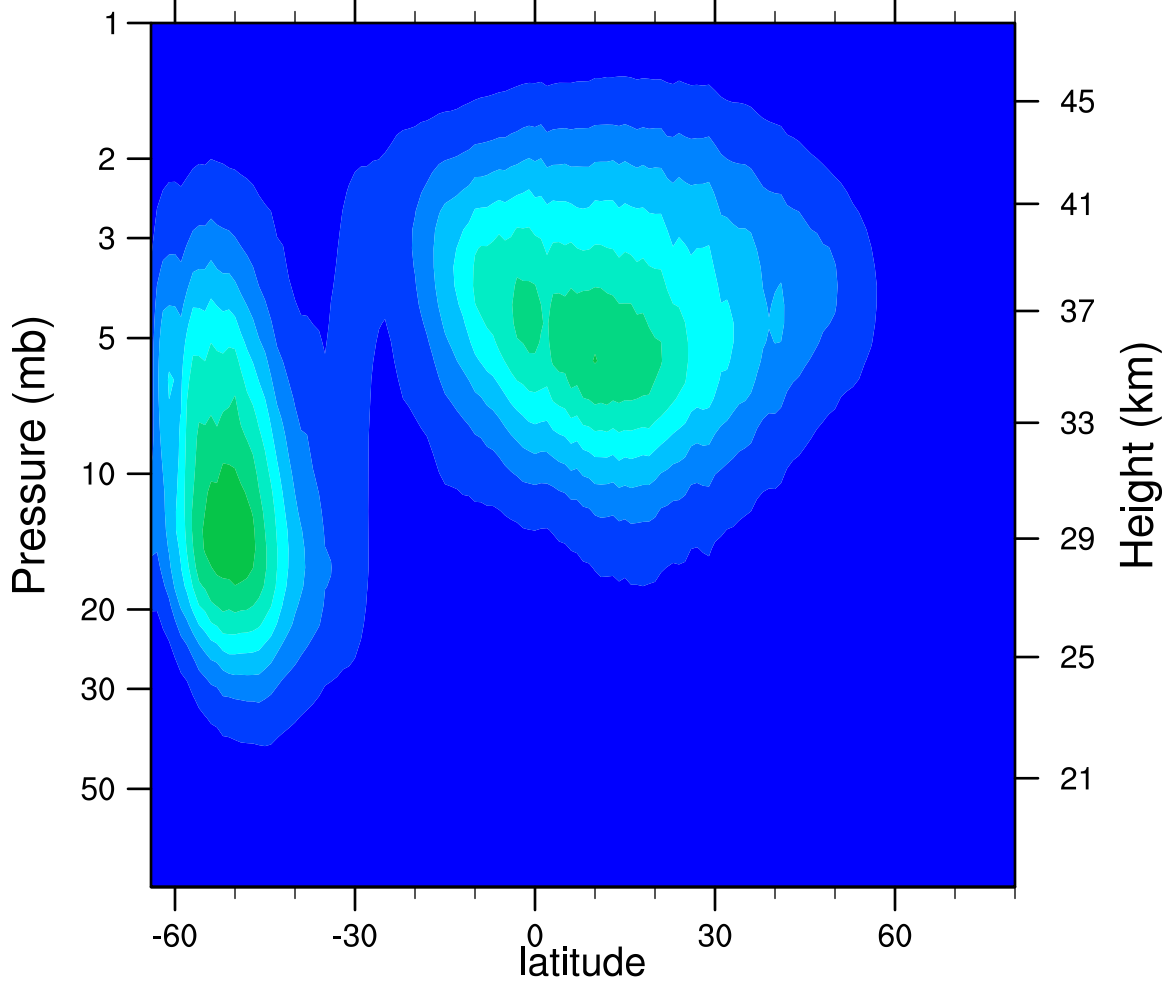
2005d196 N2O5_Ascending (ppbv)
