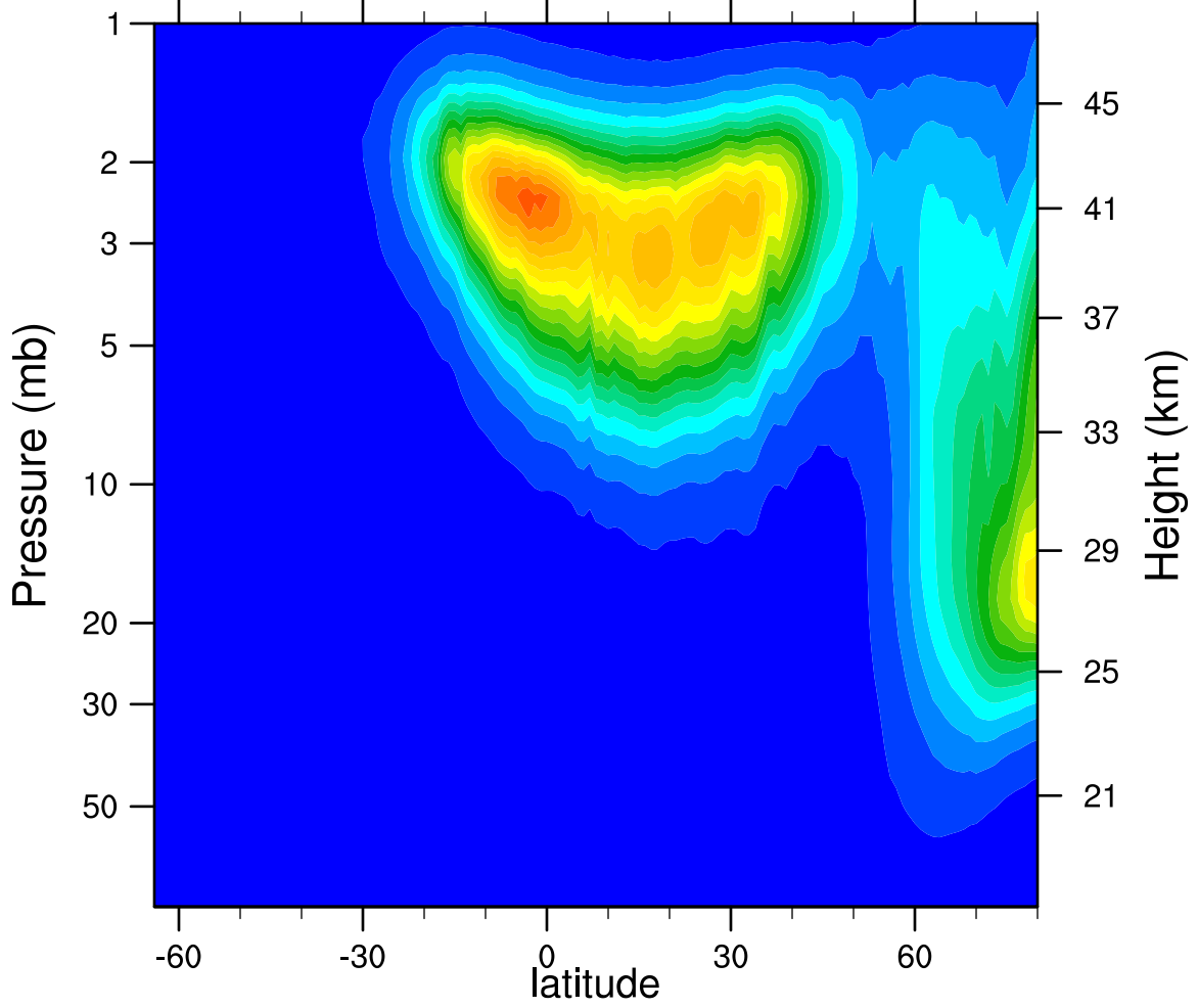
2005d042 N2O5_Ascending (ppbv)
