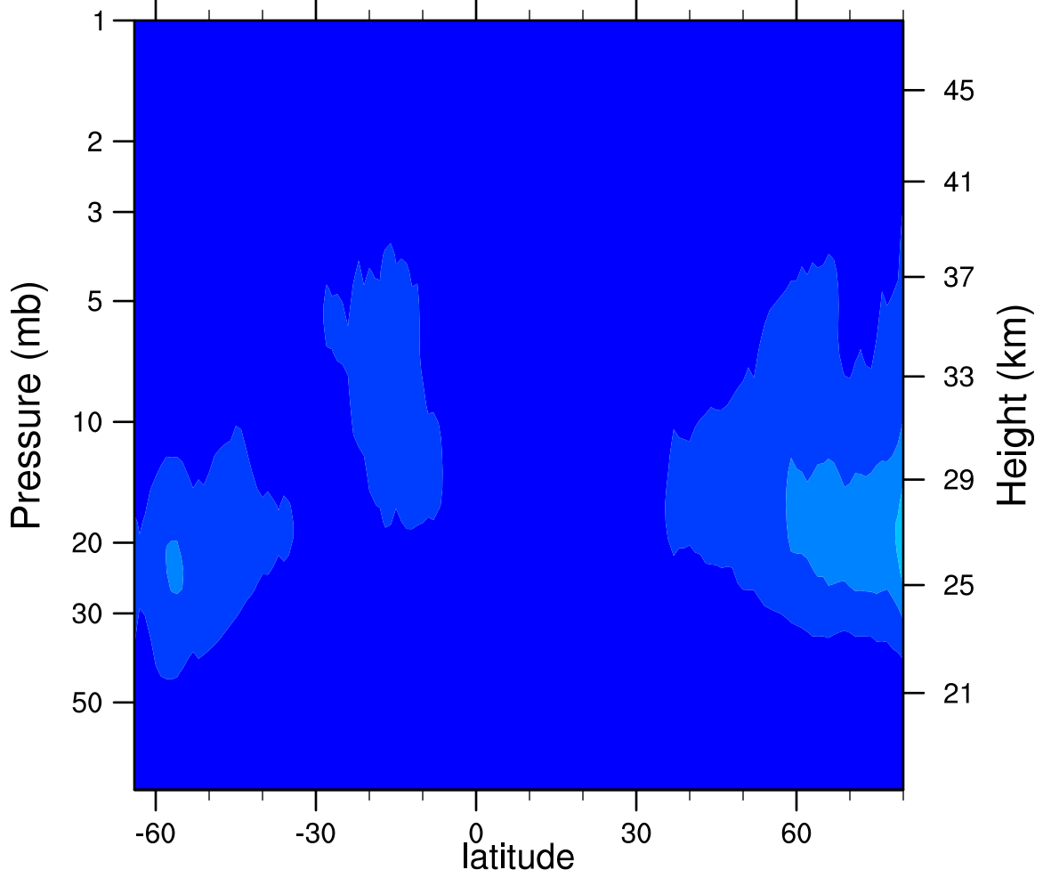
2006d272 N2O5_Ascending (ppbv)
