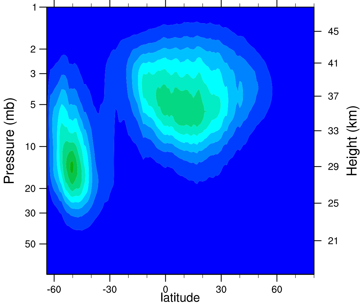
2005d203 N2O5_Ascending (ppbv)
