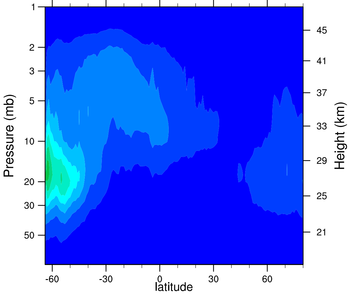
2006d097 N2O5_Ascending (ppbv)
