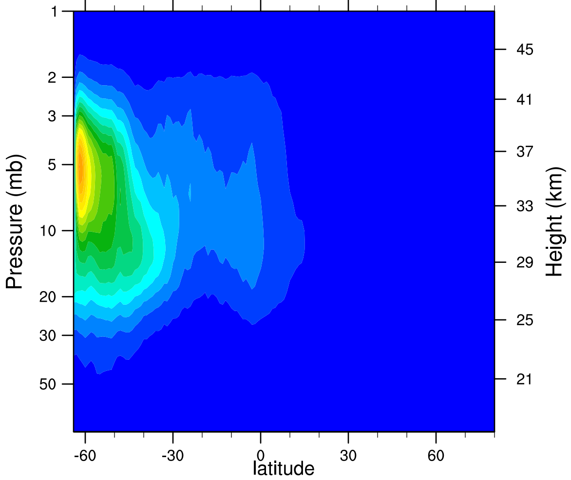
2006d152 N2O5_Ascending (ppbv)
