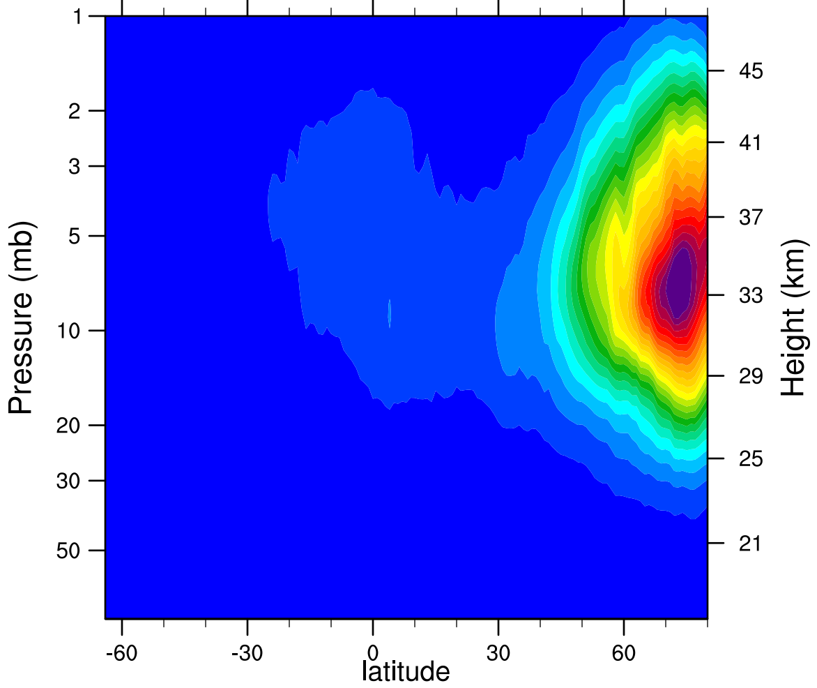
2005d351 N2O5_Ascending (ppbv)
