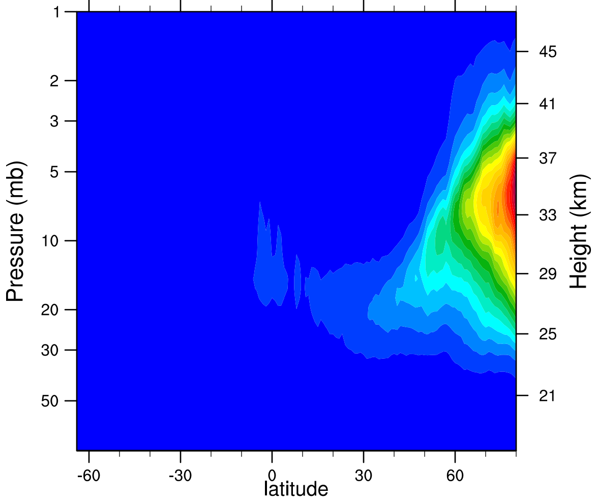
2007d039 N2O5_Ascending (ppbv)
