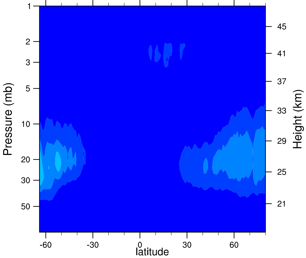
2007d077 N2O5_Ascending (ppbv)
