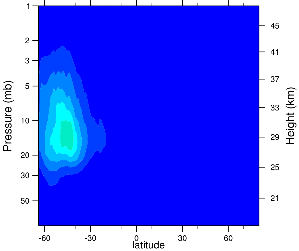
2007d206 N2O5_Ascending (ppbv)
