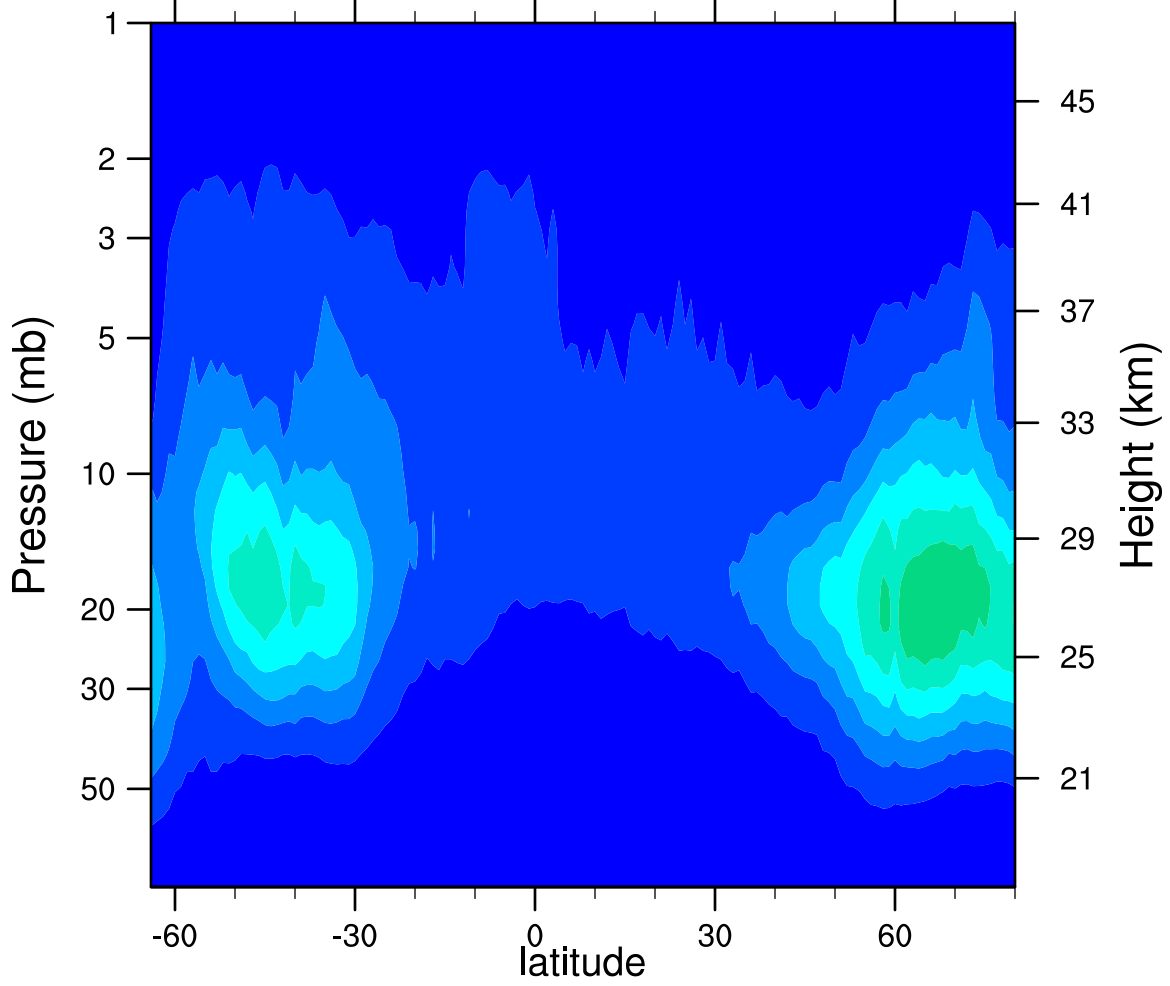
2007d268 N2O5_Ascending (ppbv)
