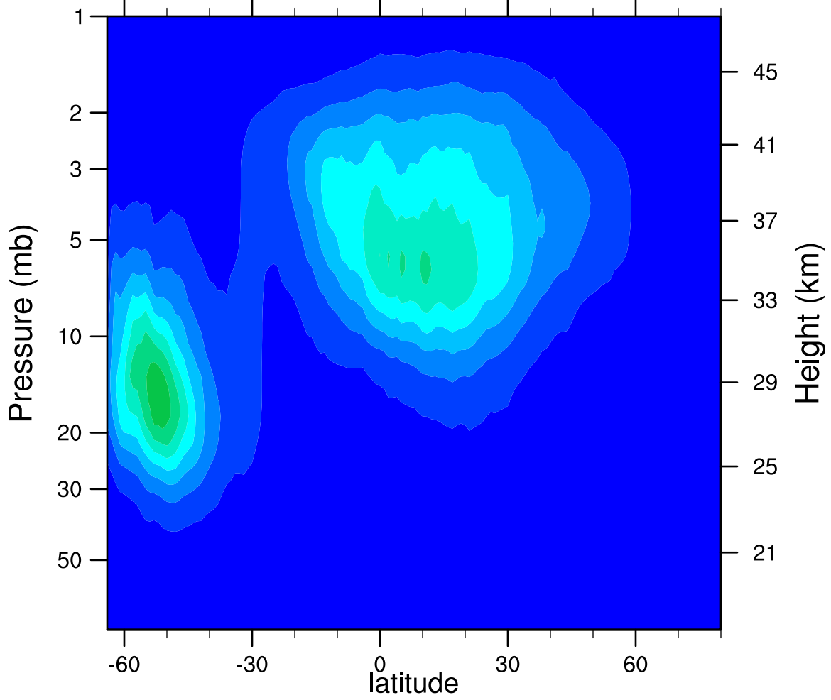
2005d217 N2O5_Ascending (ppbv)
