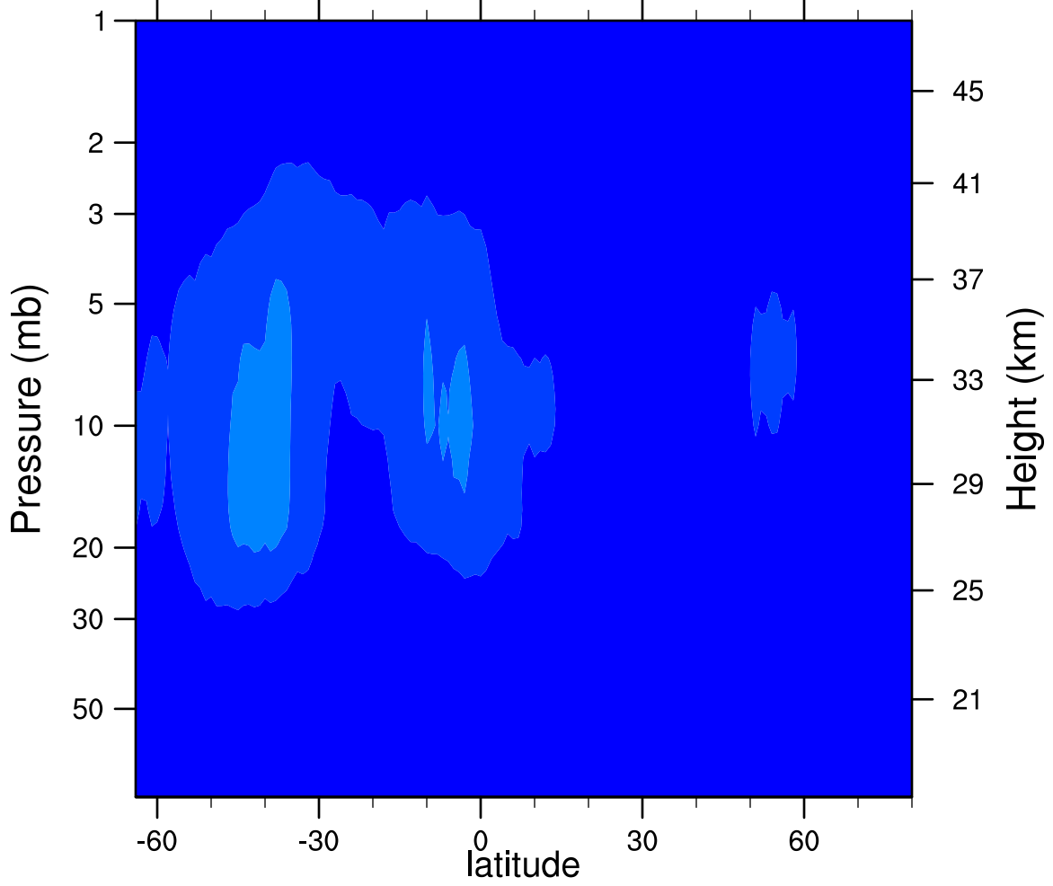
2006d221 N2O5_Ascending (ppbv)
