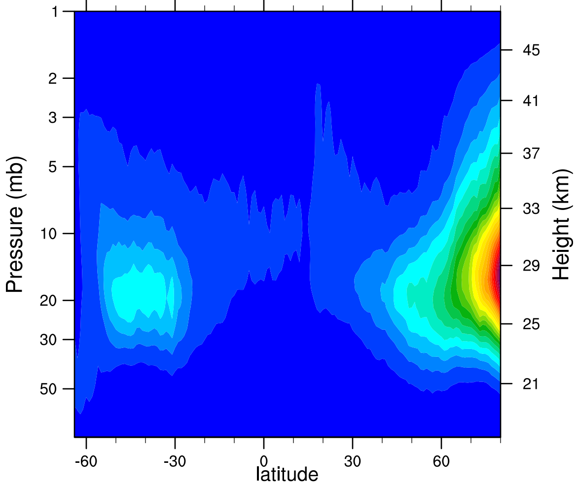
2007d287 N2O5_Ascending (ppbv)
