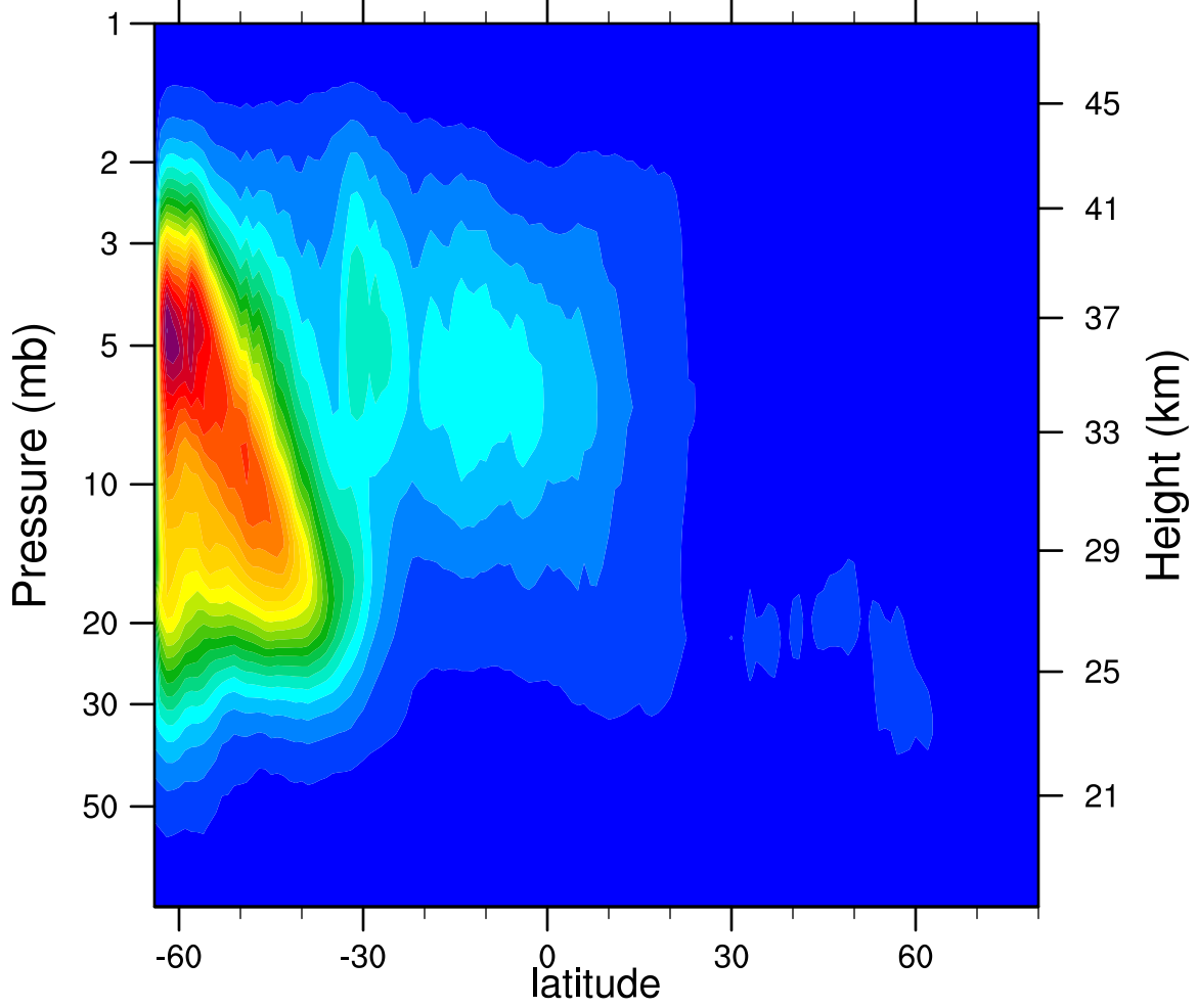
2007d136 N2O5_Ascending (ppbv)
