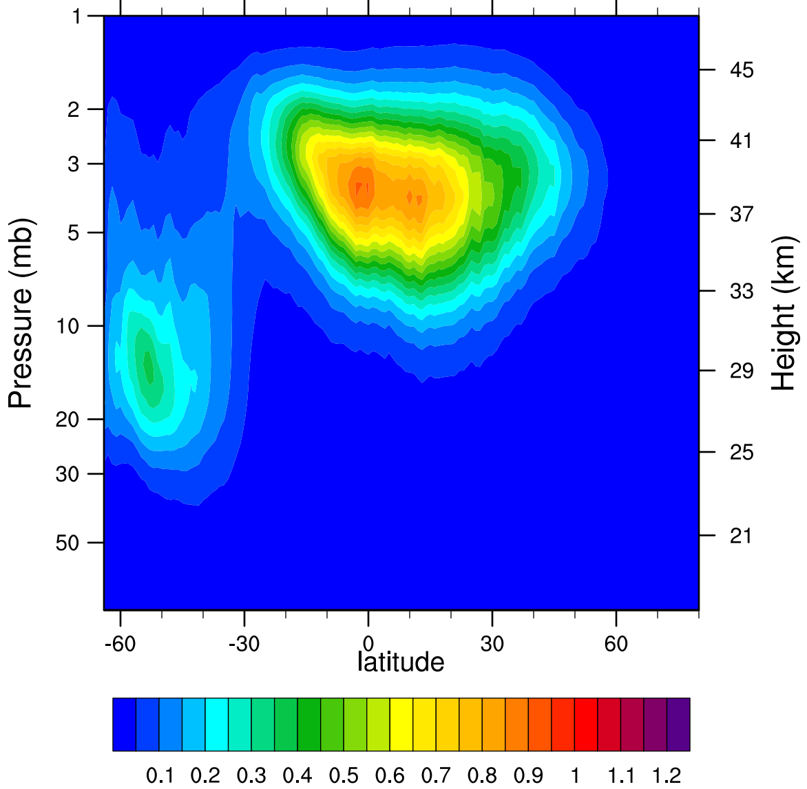
2005d135 N2O5_Ascending (ppbv)
