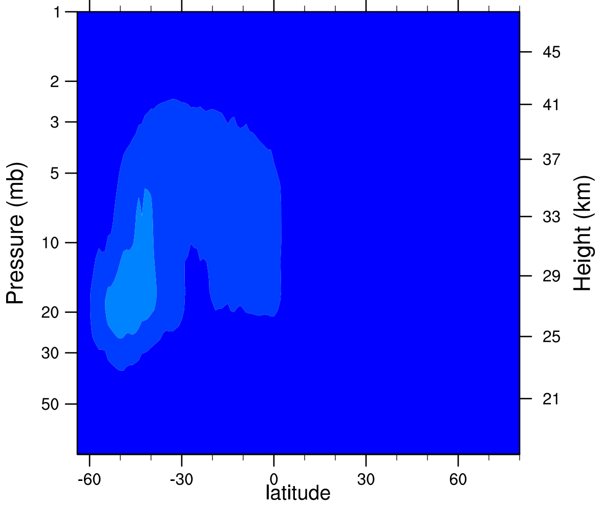
2006d237 N2O5_Ascending (ppbv)
