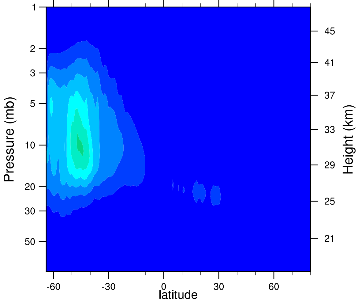
2007d173 N2O5_Ascending (ppbv)
