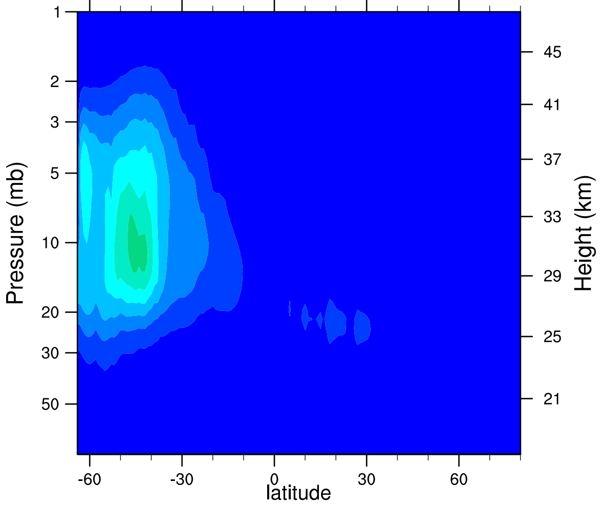
2007d171 N2O5_Ascending (ppbv)
