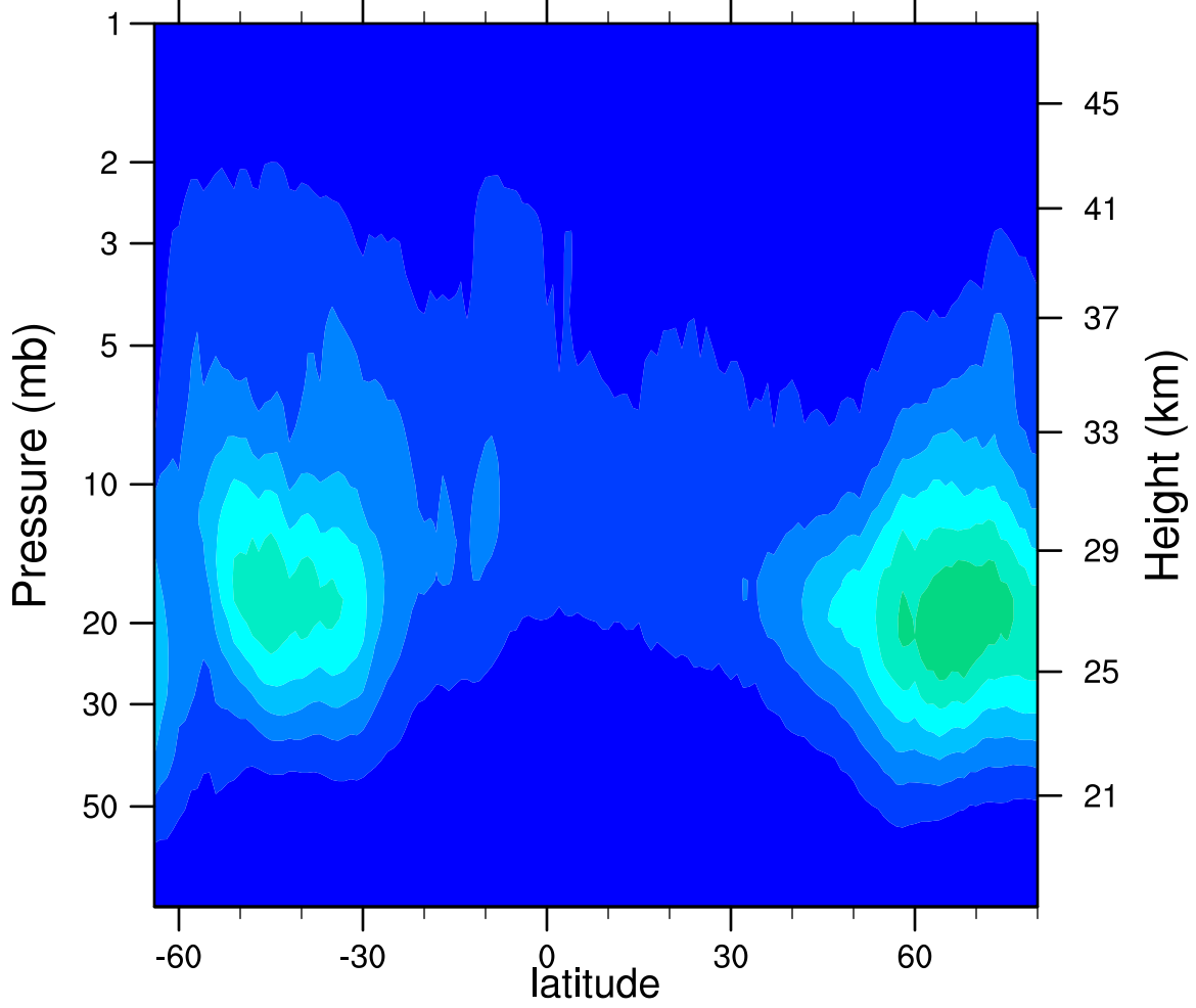
2007d267 N2O5_Ascending (ppbv)
