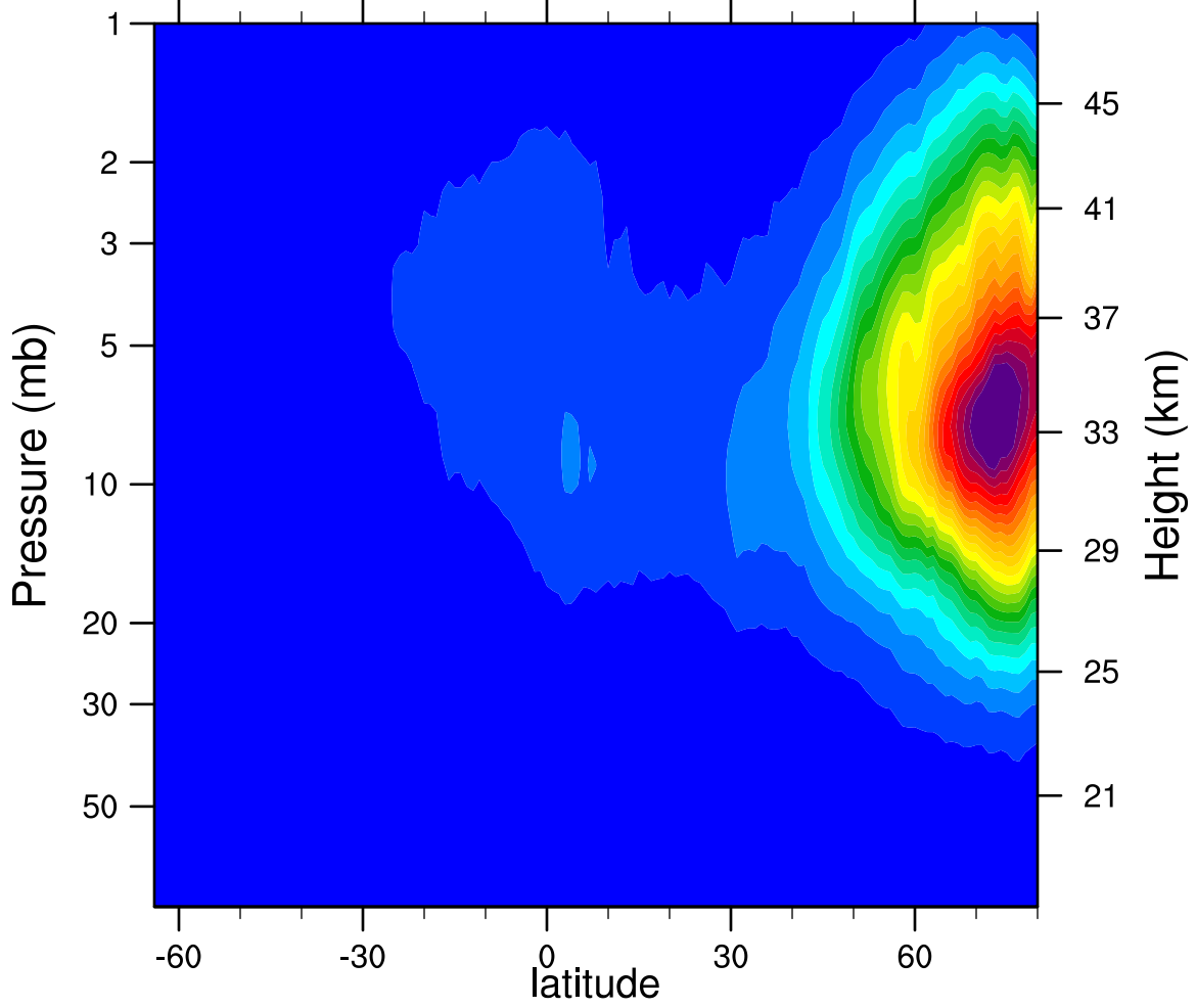
2005d352 N2O5_Ascending (ppbv)
