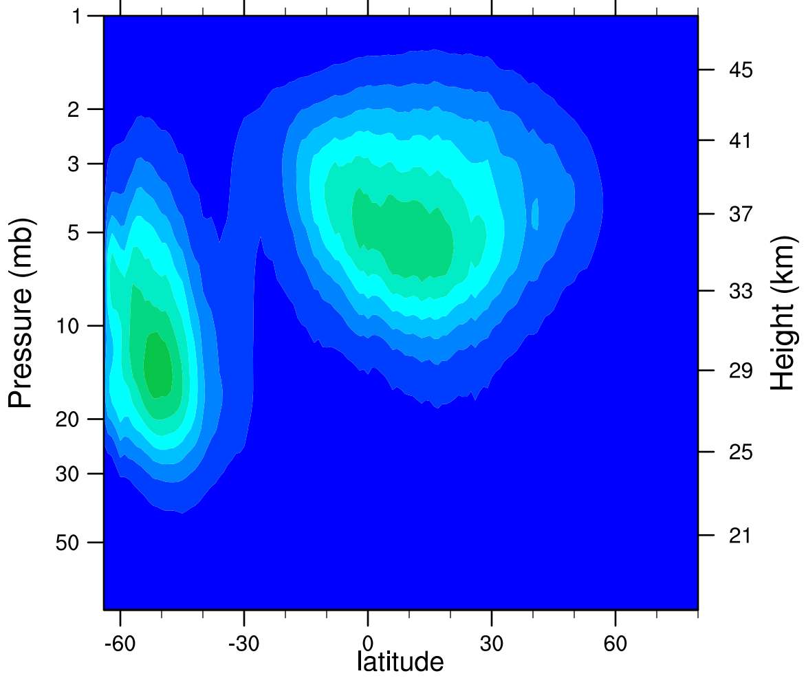
2005d200 N2O5_Ascending (ppbv)
