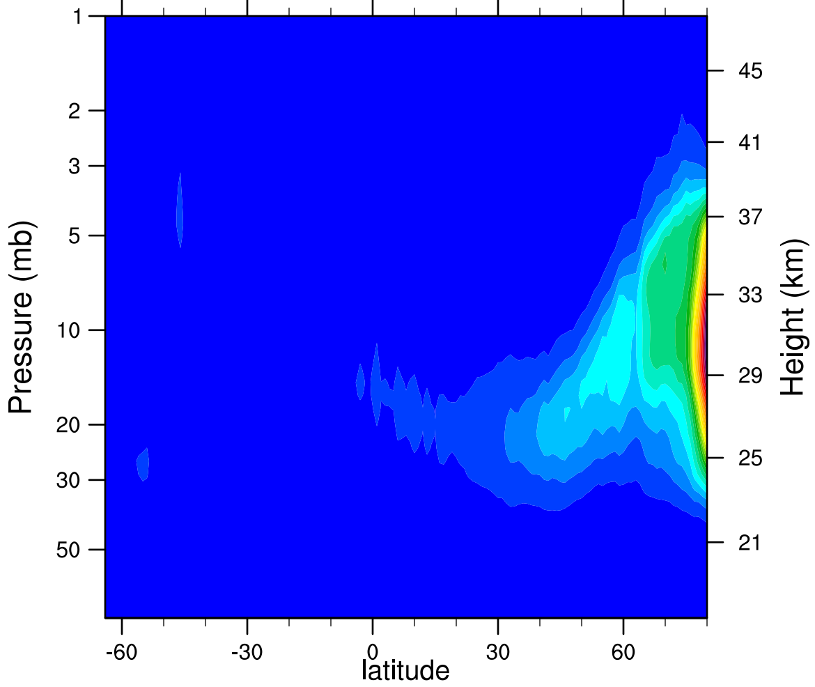
2007d054 N2O5_Ascending (ppbv)
