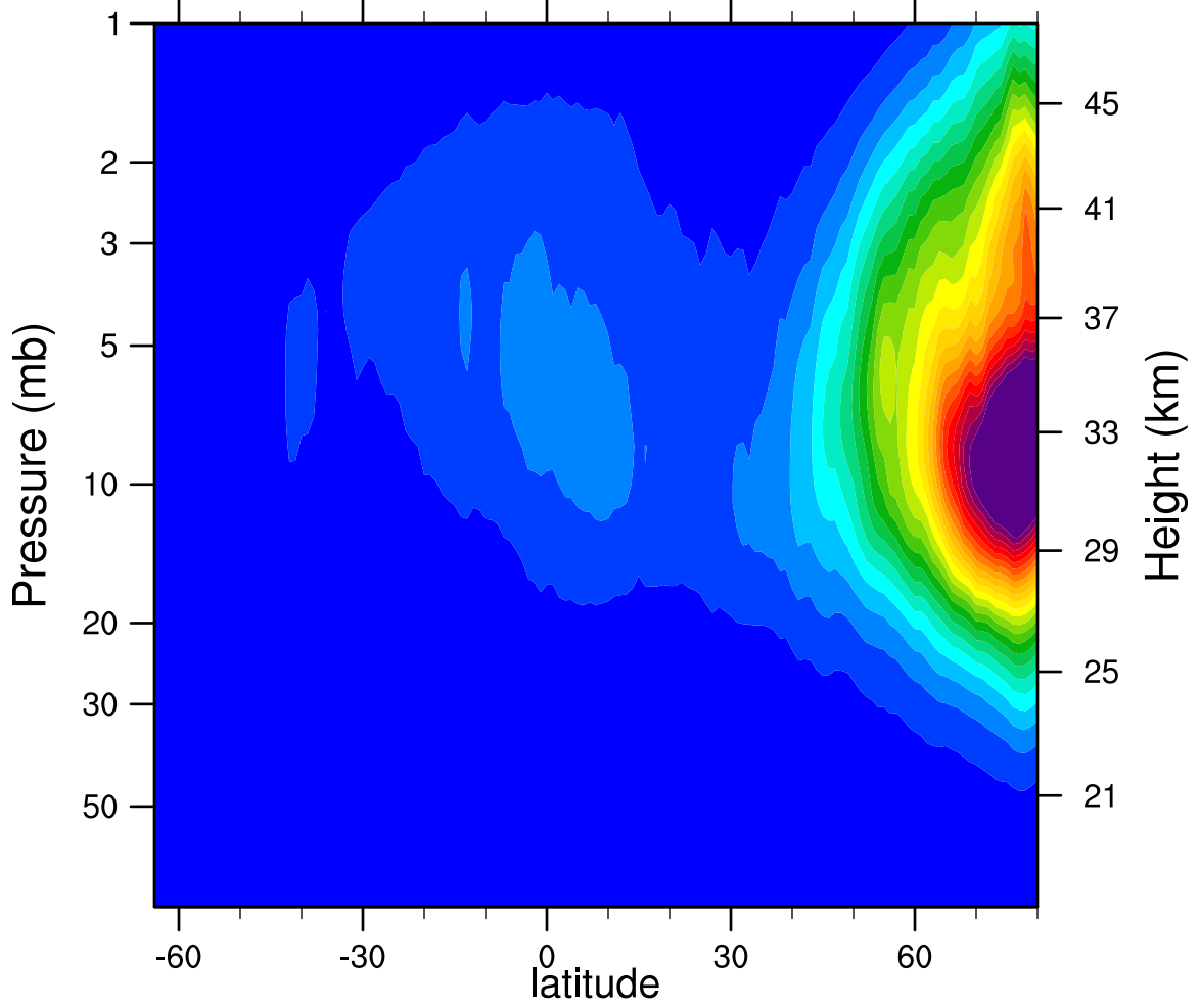
2006d007 N2O5_Ascending (ppbv)
