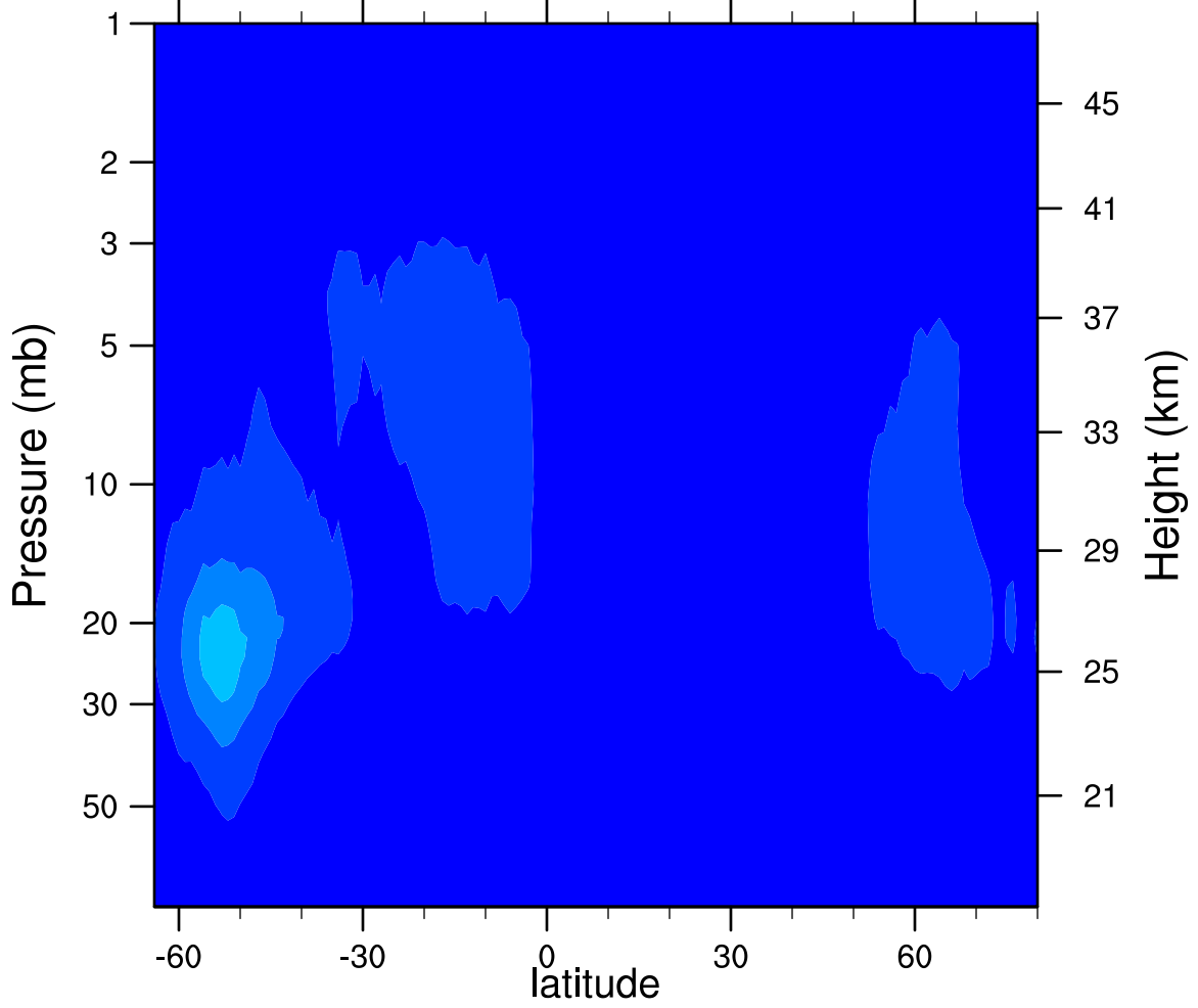
2006d261 N2O5_Ascending (ppbv)
