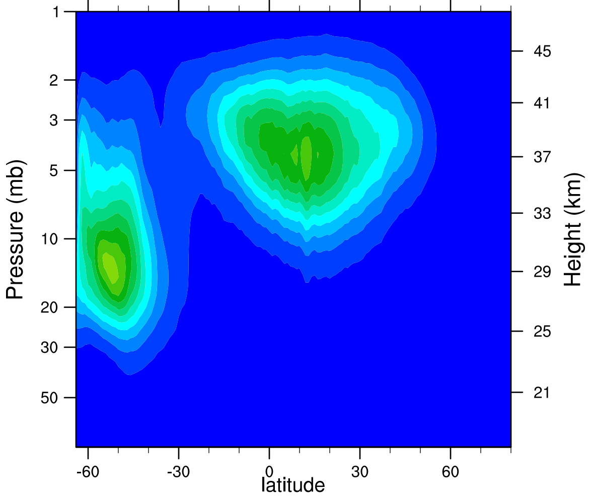
2005d159 N2O5_Ascending (ppbv)
