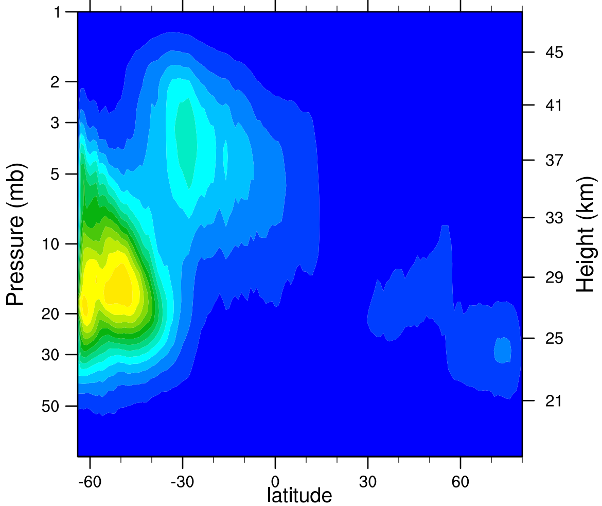
2007d107 N2O5_Ascending (ppbv)
