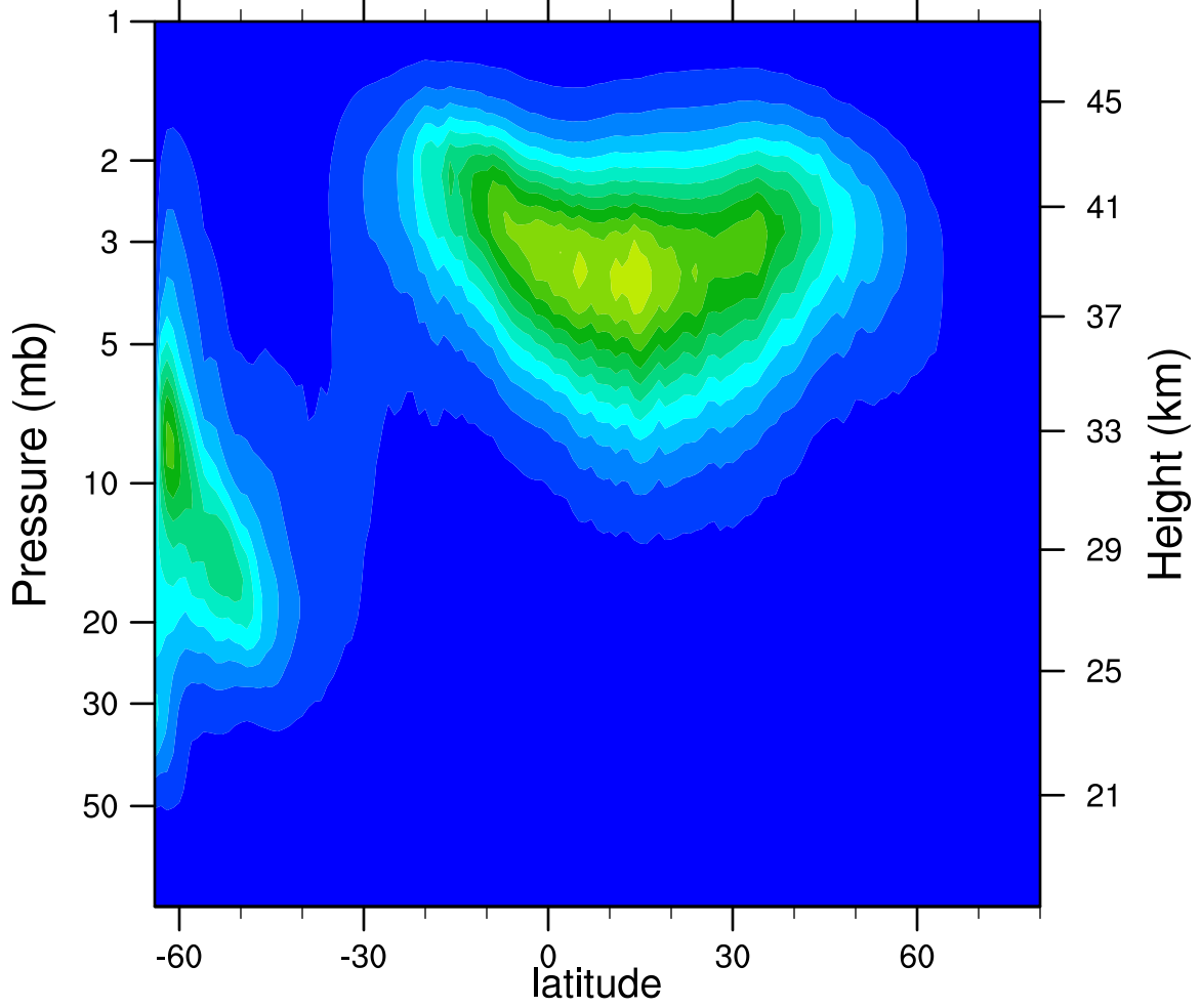
2005d110 N2O5_Ascending (ppbv)
