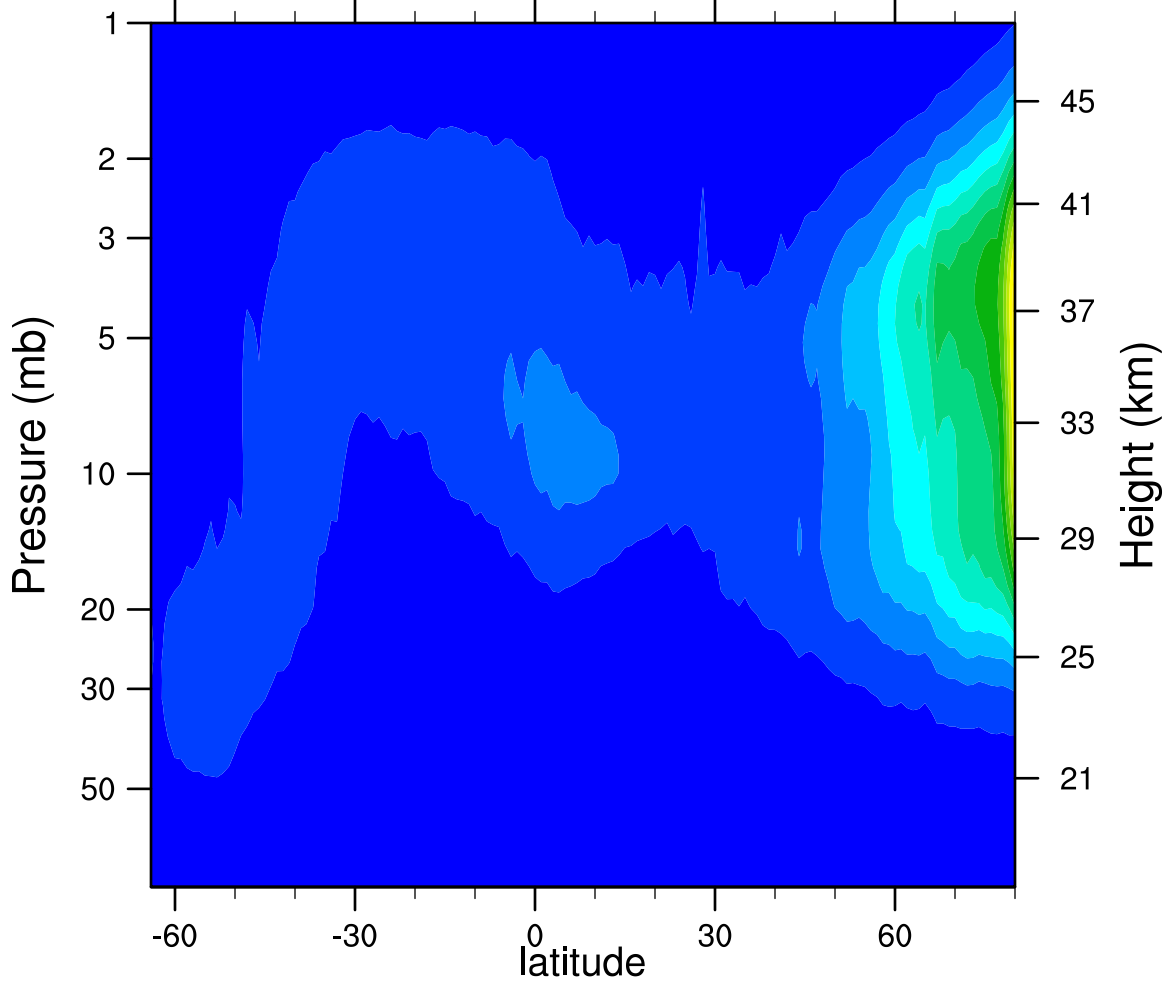
2006d058 N2O5_Ascending (ppbv)
