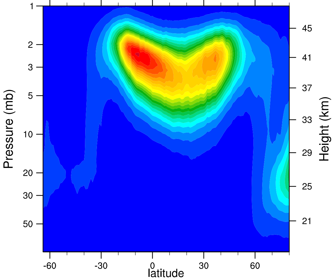
2005d067 N2O5_Ascending (ppbv)
