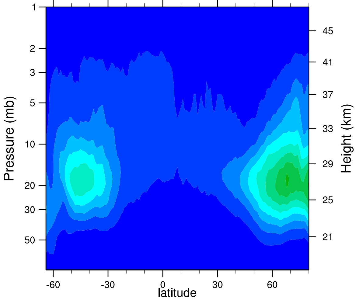
2007d272 N2O5_Ascending (ppbv)
