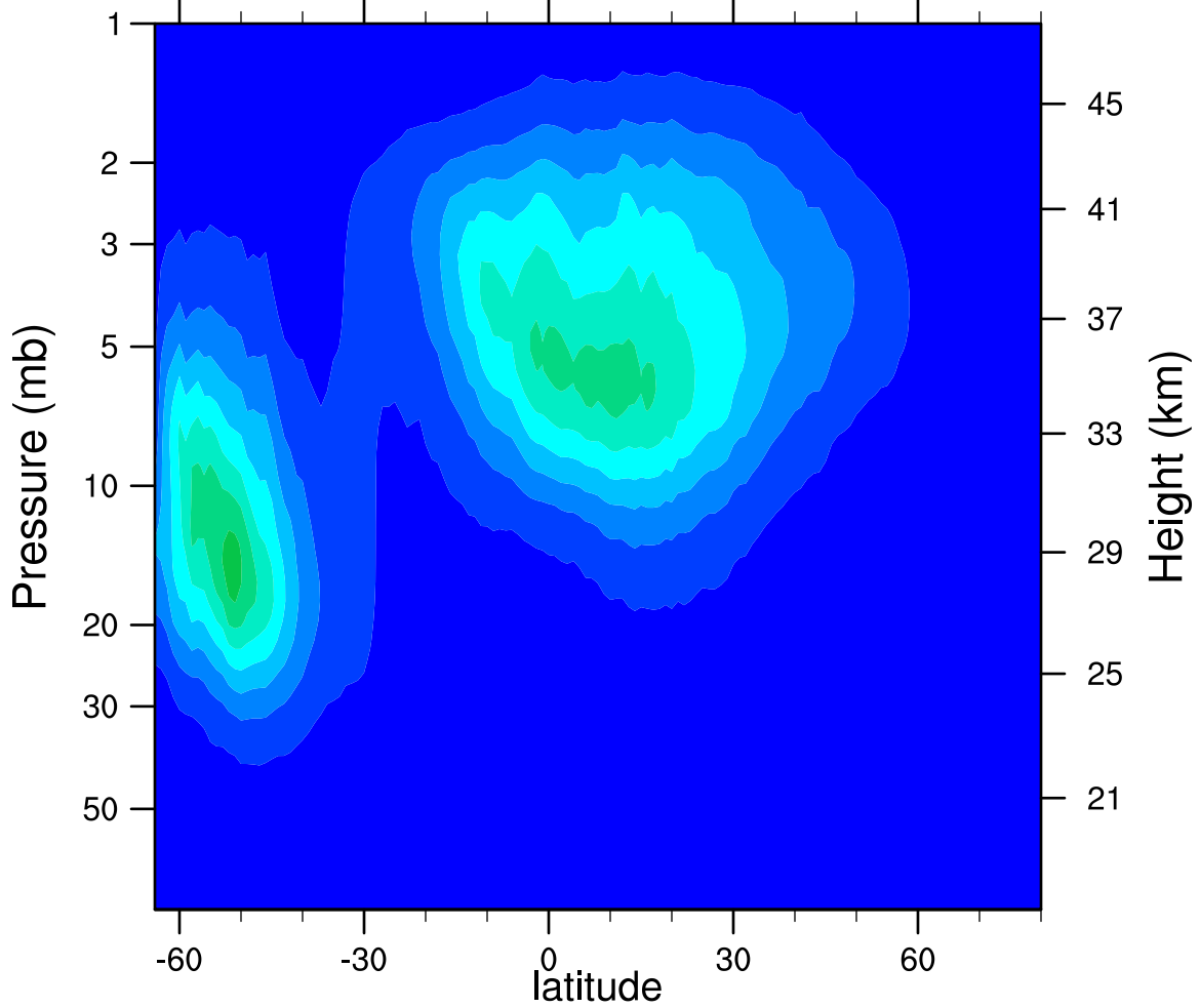
2005d213 N2O5_Ascending (ppbv)
