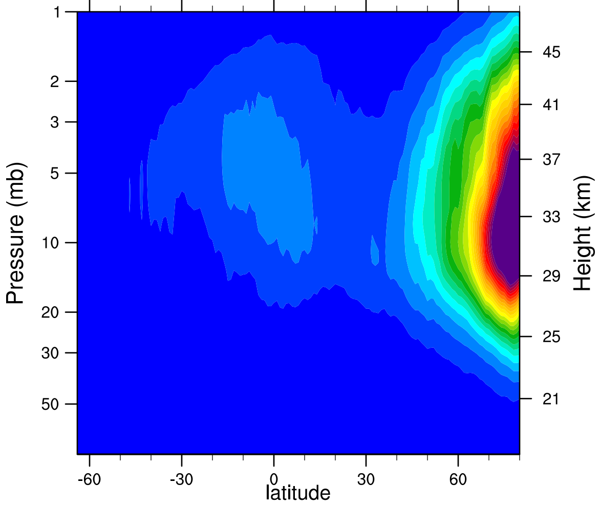
2006d014 N2O5_Ascending (ppbv)
