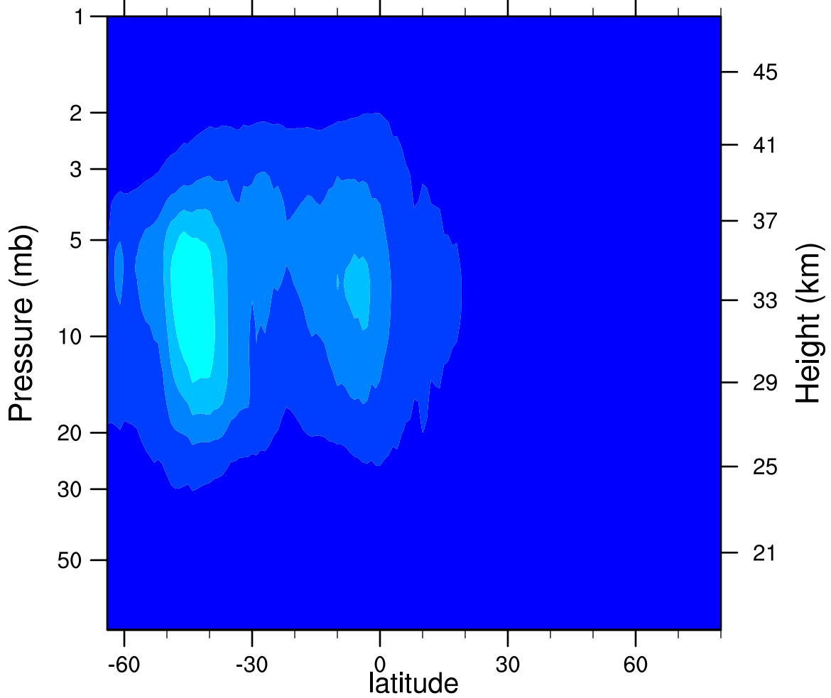
2006d198 N2O5_Ascending (ppbv)
