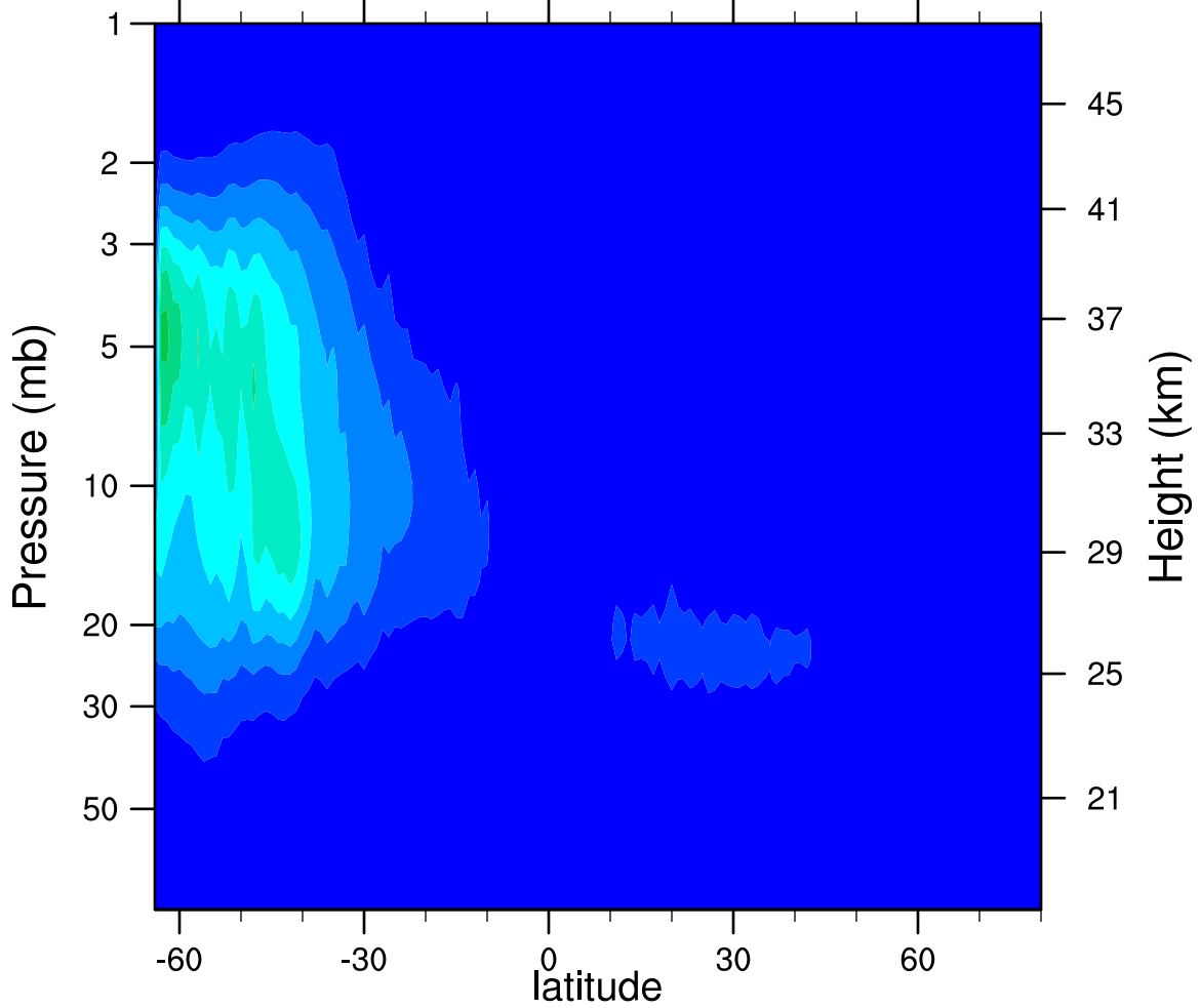
2007d165 N2O5_Ascending (ppbv)
