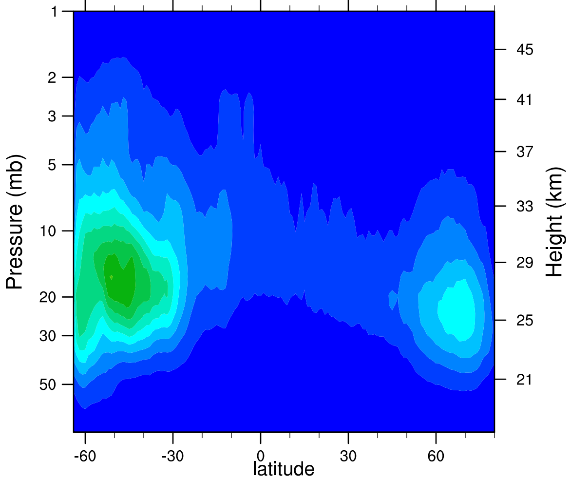
2007d252 N2O5_Ascending (ppbv)
