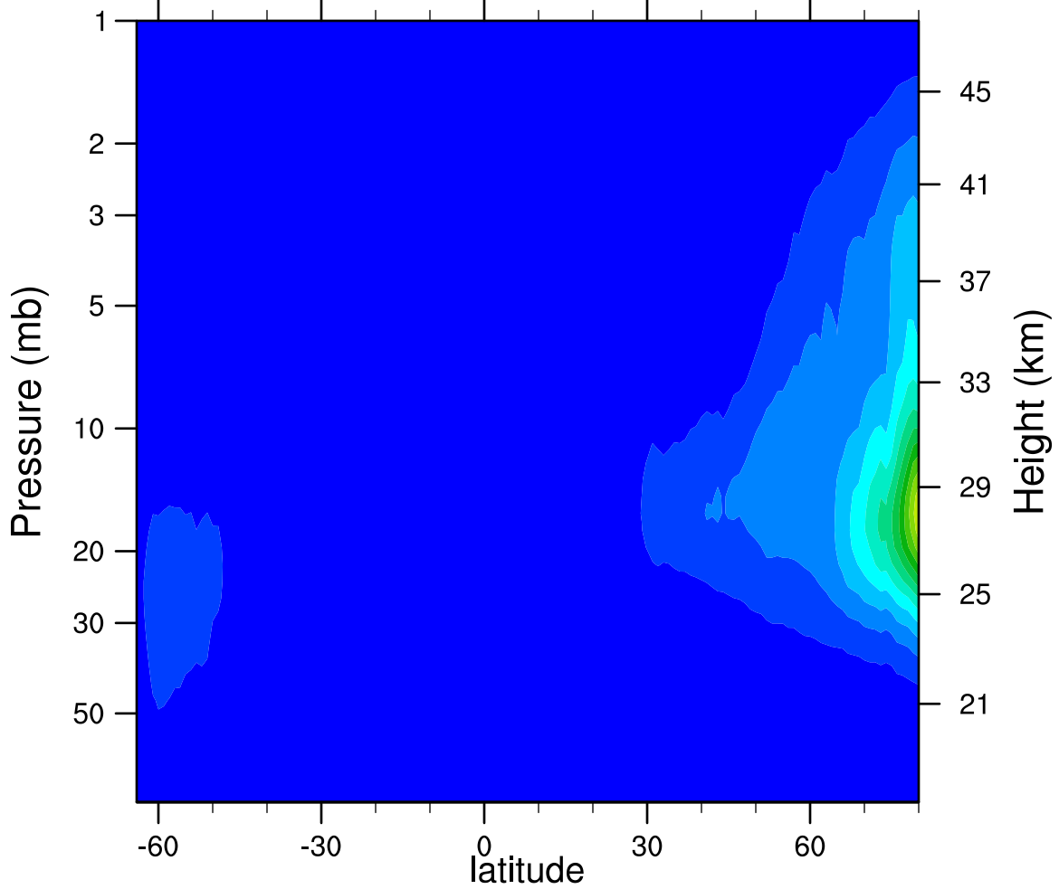
2006d287 N2O5_Ascending (ppbv)
