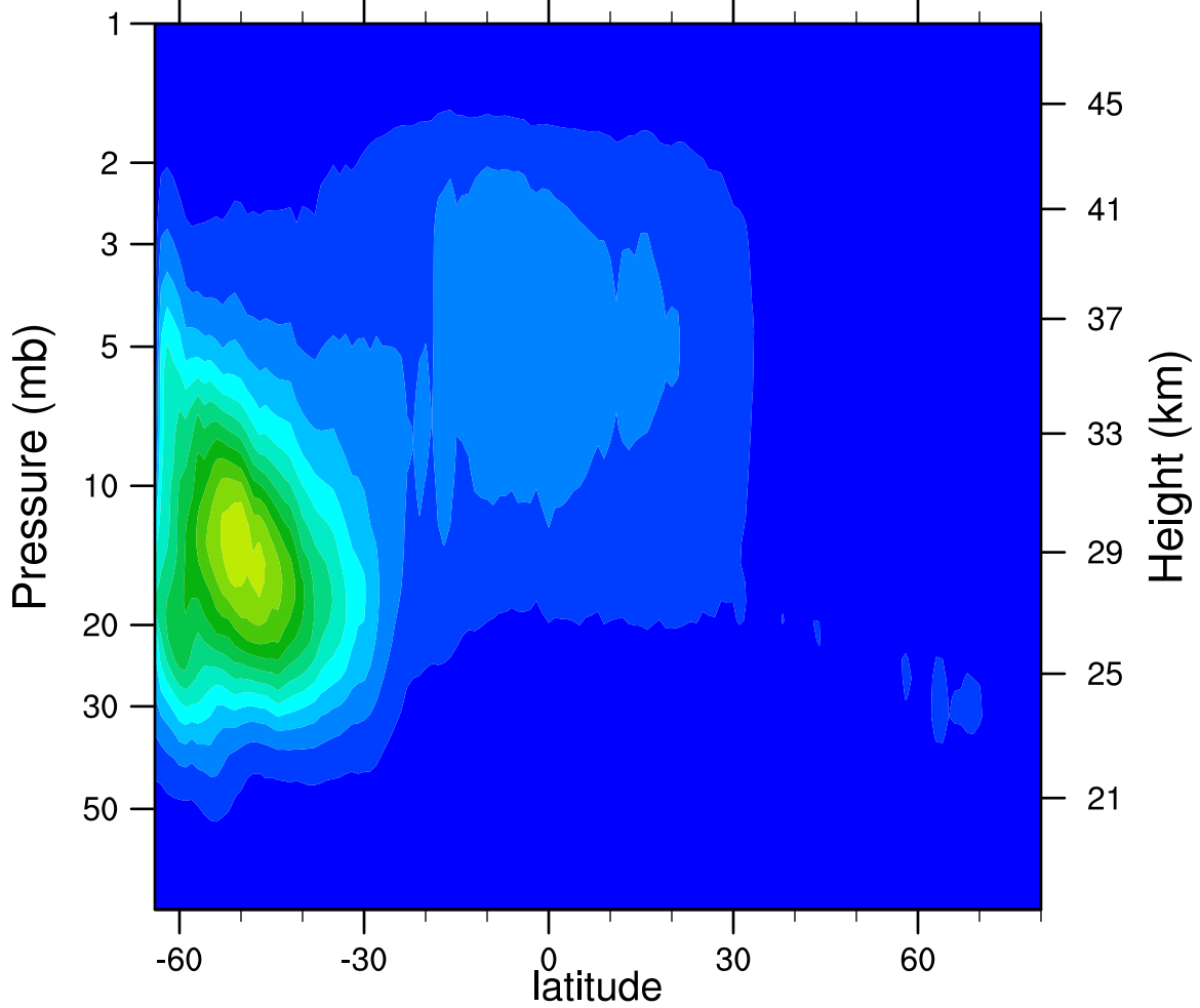
2007d230 N2O5_Ascending (ppbv)
