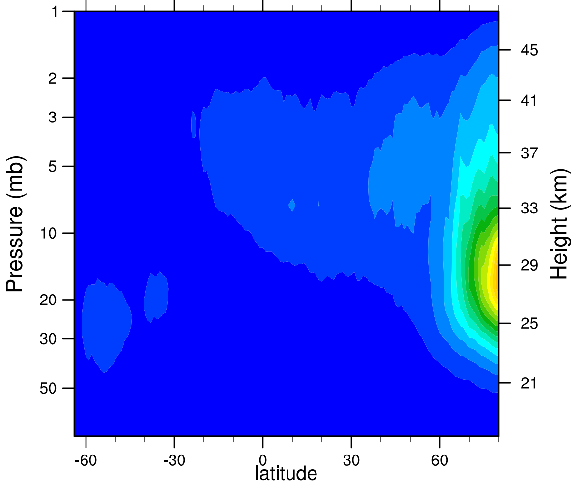
2005d294 N2O5_Ascending (ppbv)
