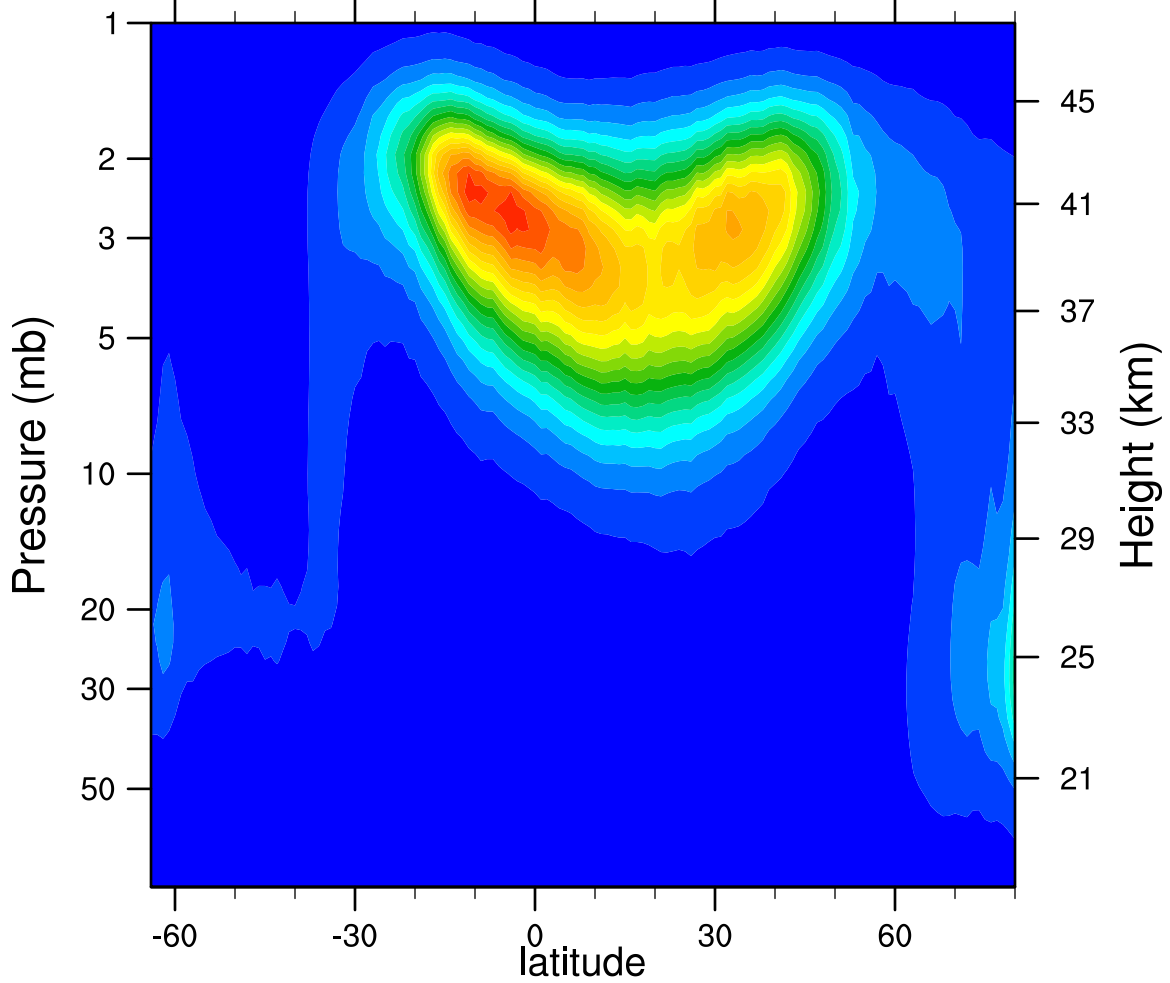
2005d072 N2O5_Ascending (ppbv)
