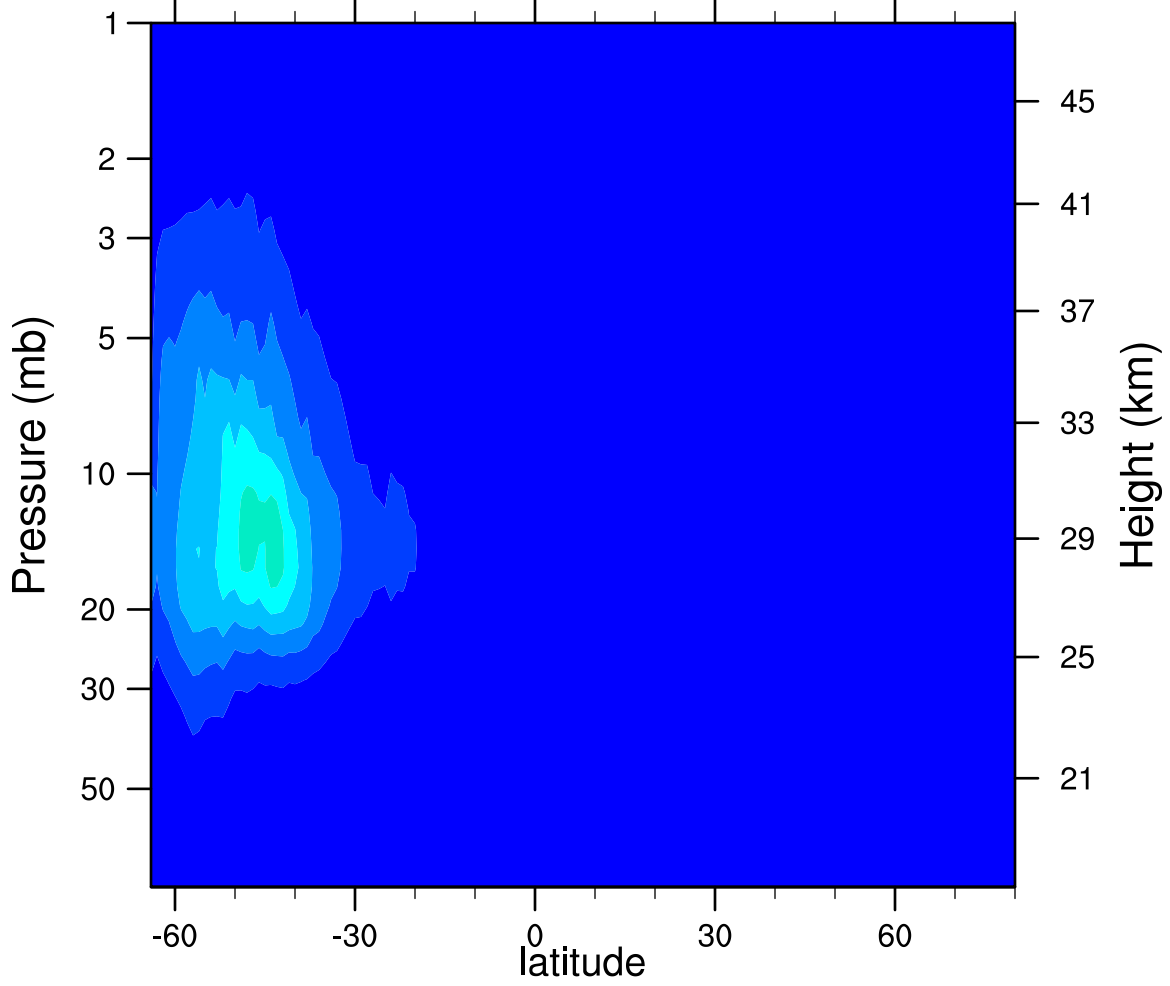
2007d207 N2O5_Ascending (ppbv)
