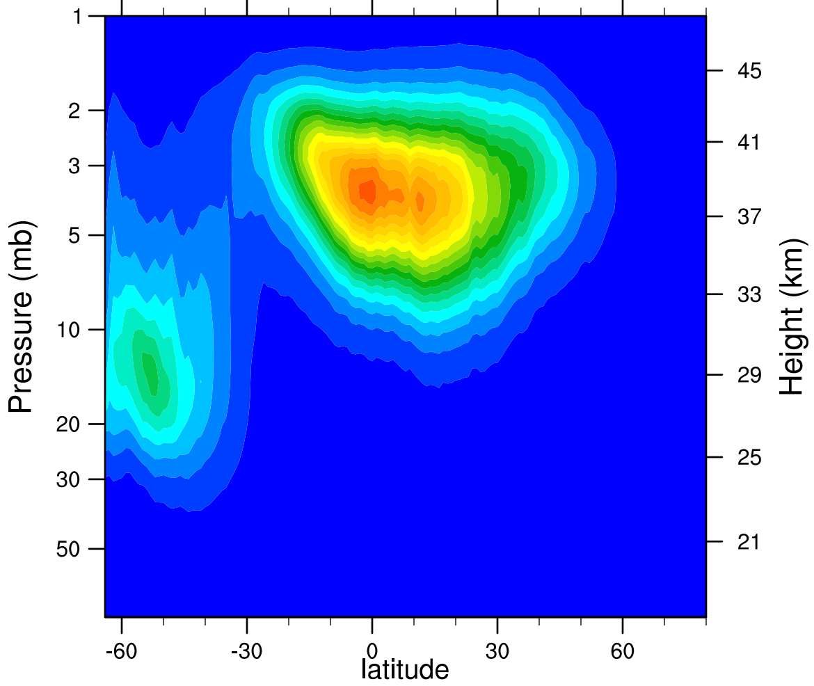
2005d133 N2O5_Ascending (ppbv)
