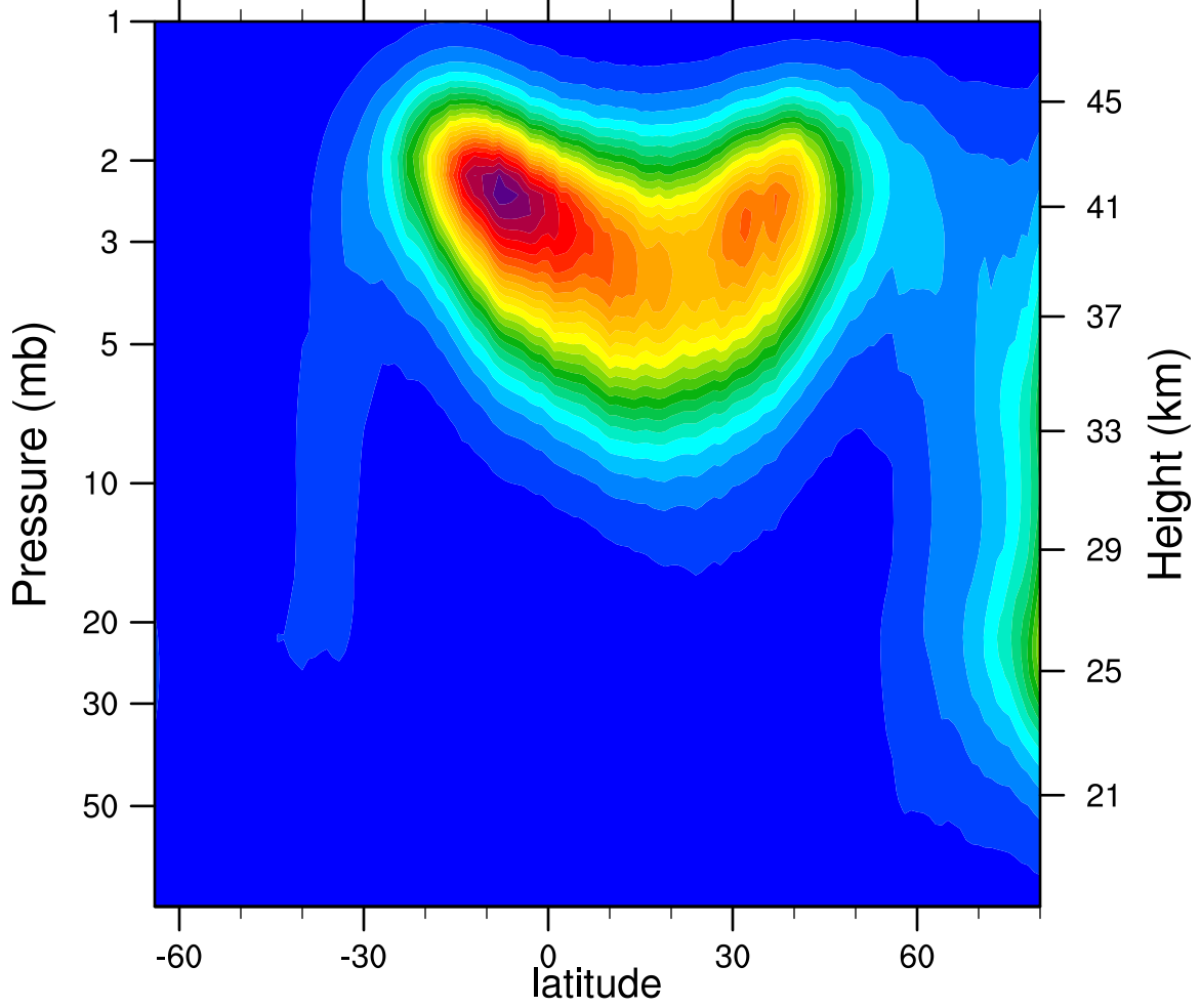
2005d059 N2O5_Ascending (ppbv)
