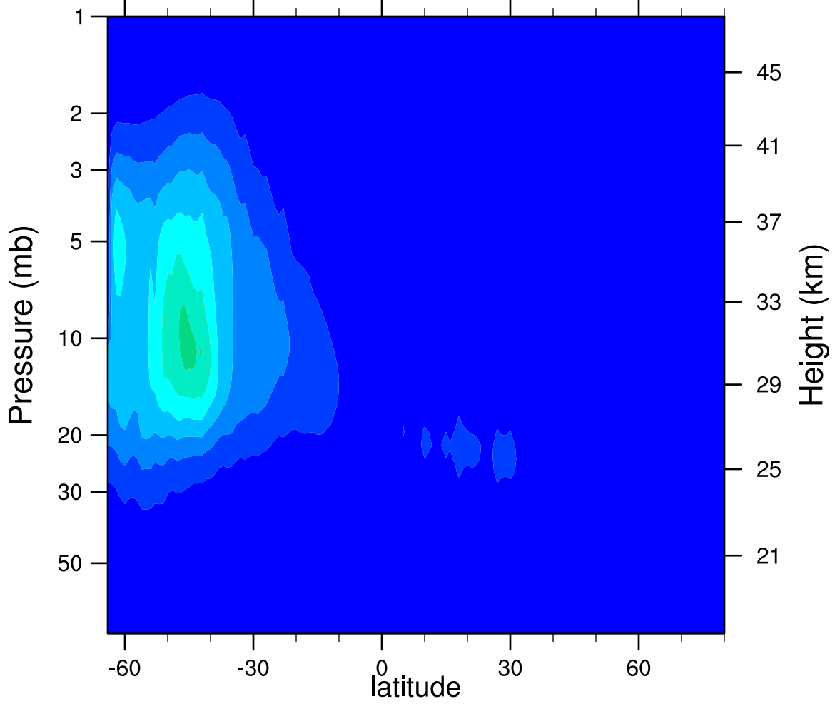
2007d172 N2O5_Ascending (ppbv)
