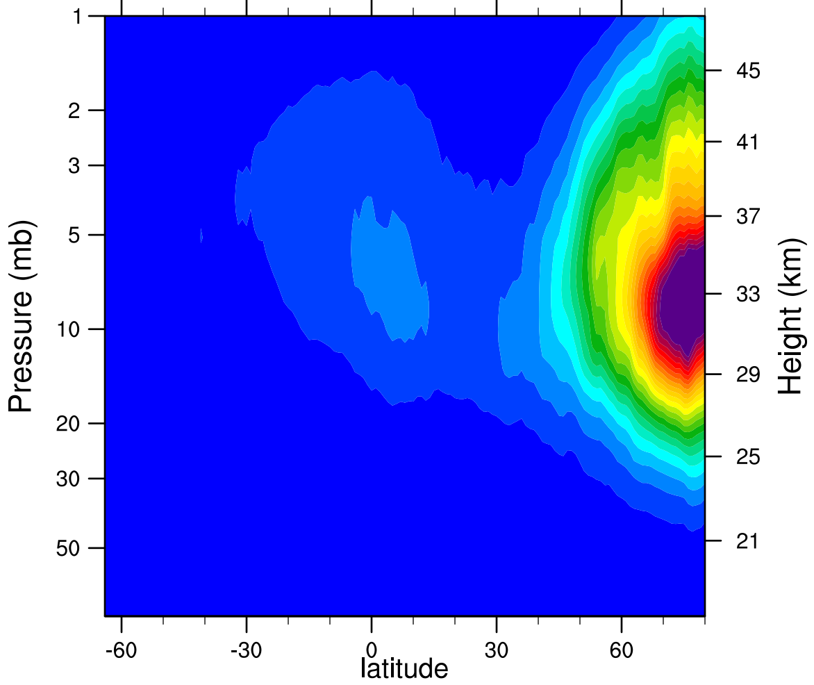
2006d004 N2O5_Ascending (ppbv)
