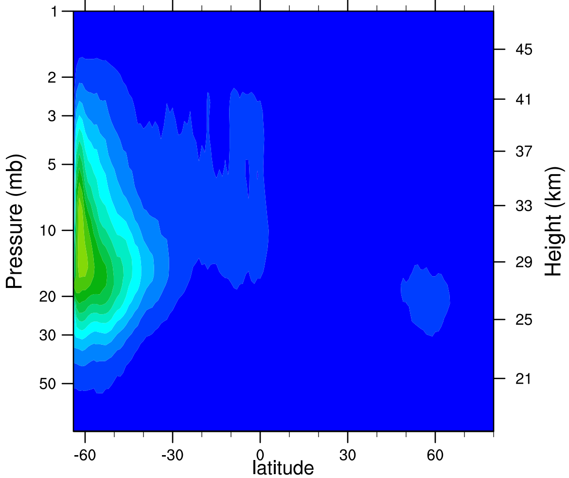
2006d118 N2O5_Ascending (ppbv)
