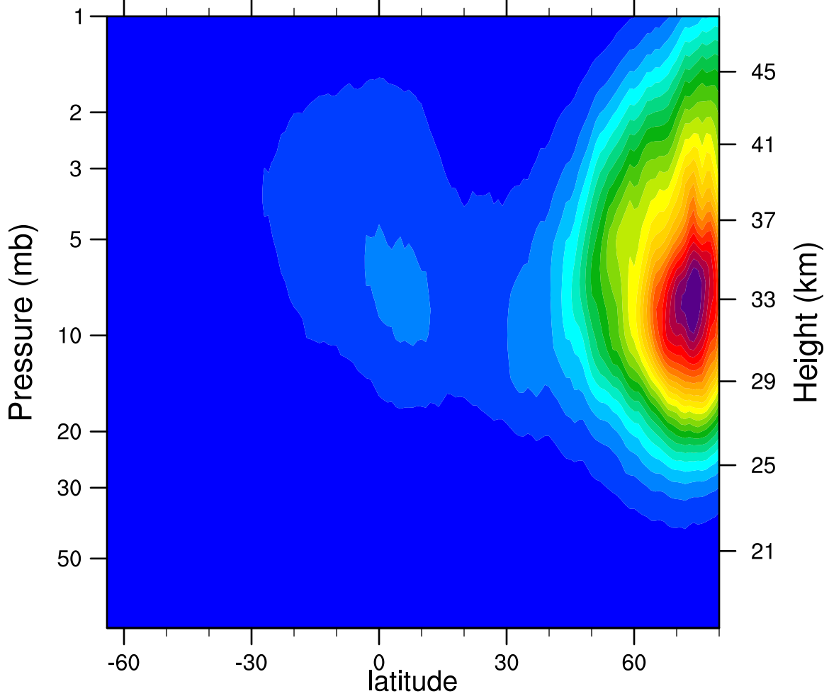
2005d365 N2O5_Ascending (ppbv)
