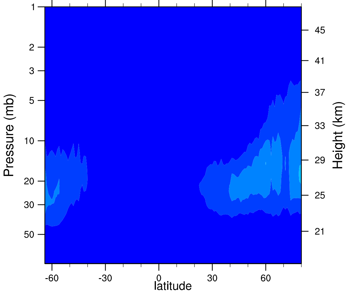
2007d075 N2O5_Ascending (ppbv)
