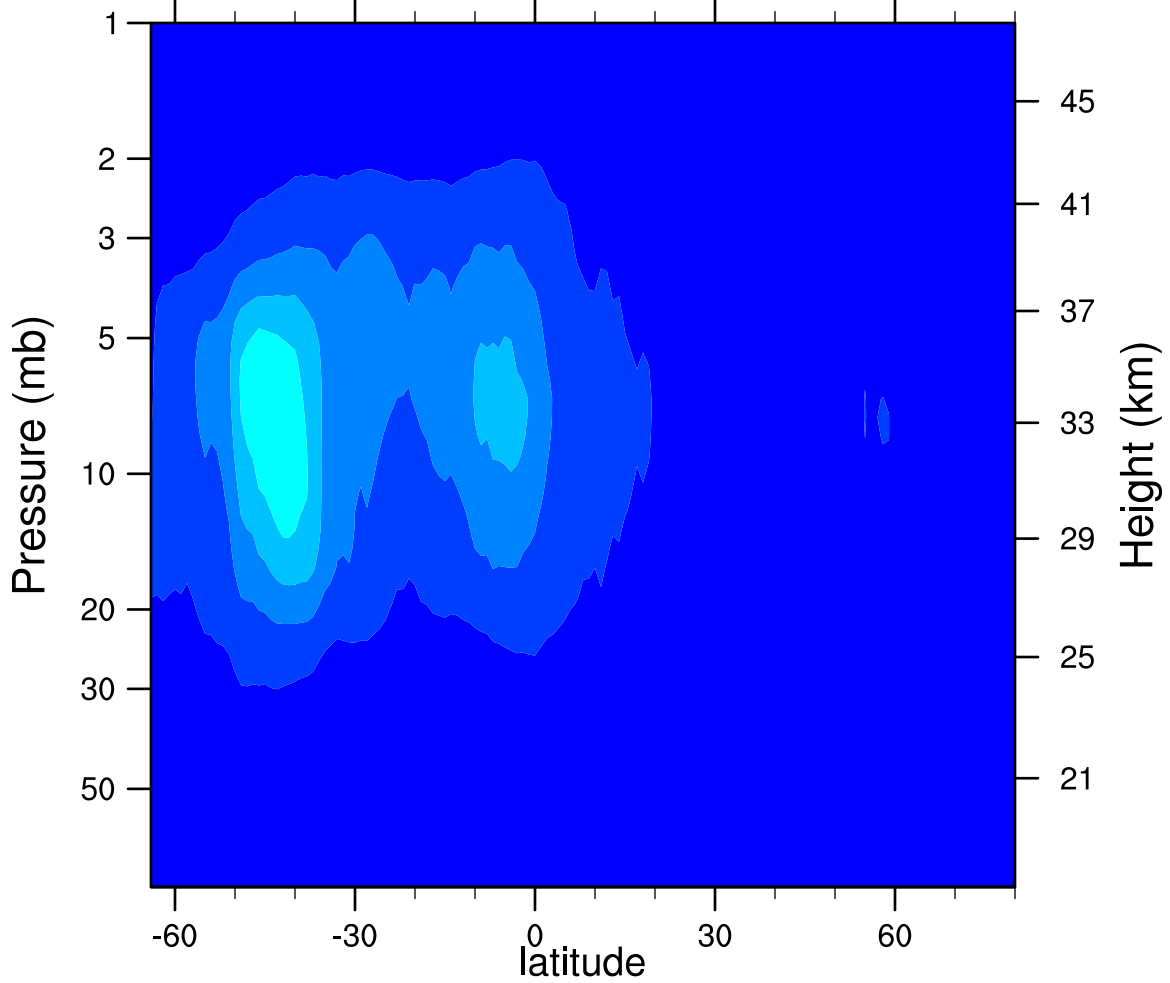
2006d200 N2O5_Ascending (ppbv)
