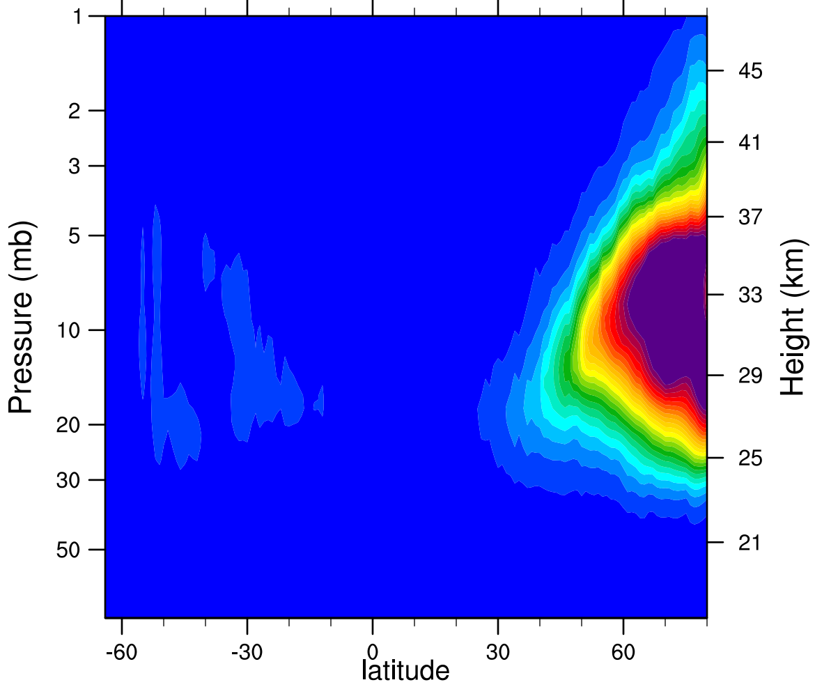
2006d357 N2O5_Ascending (ppbv)
