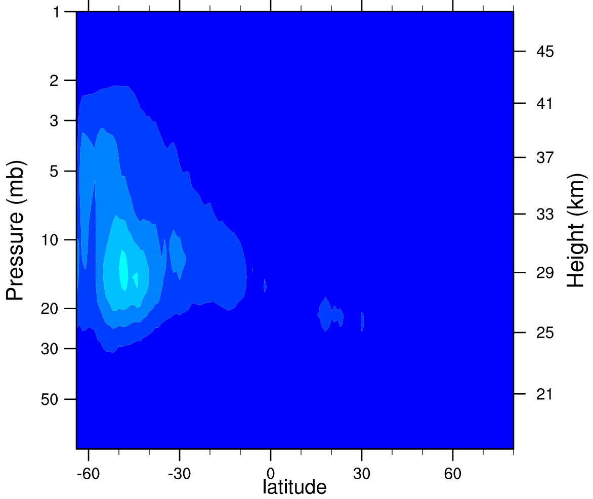
2007d182 N2O5_Ascending (ppbv)
