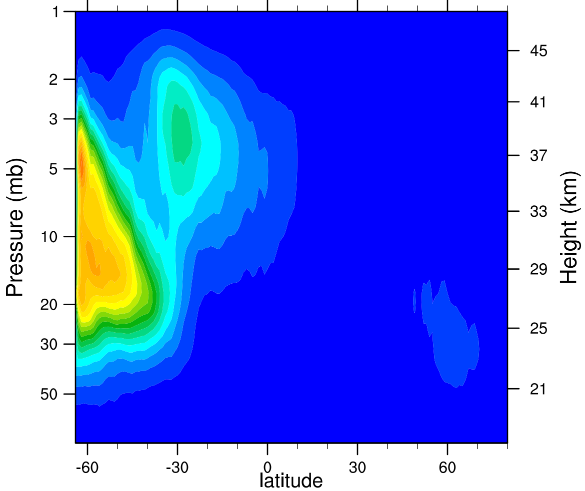
2007d117 N2O5_Ascending (ppbv)
