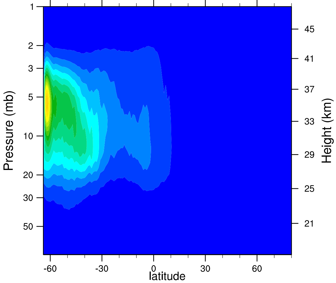
2006d172 N2O5_Ascending (ppbv)
