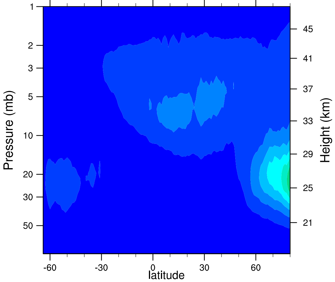
2005d280 N2O5_Ascending (ppbv)
