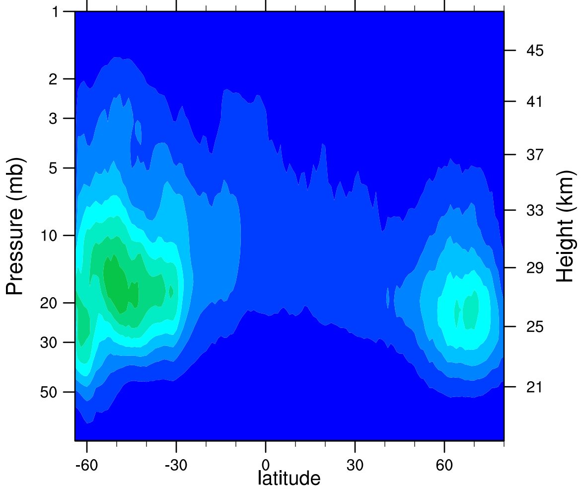
2007d256 N2O5_Ascending (ppbv)
