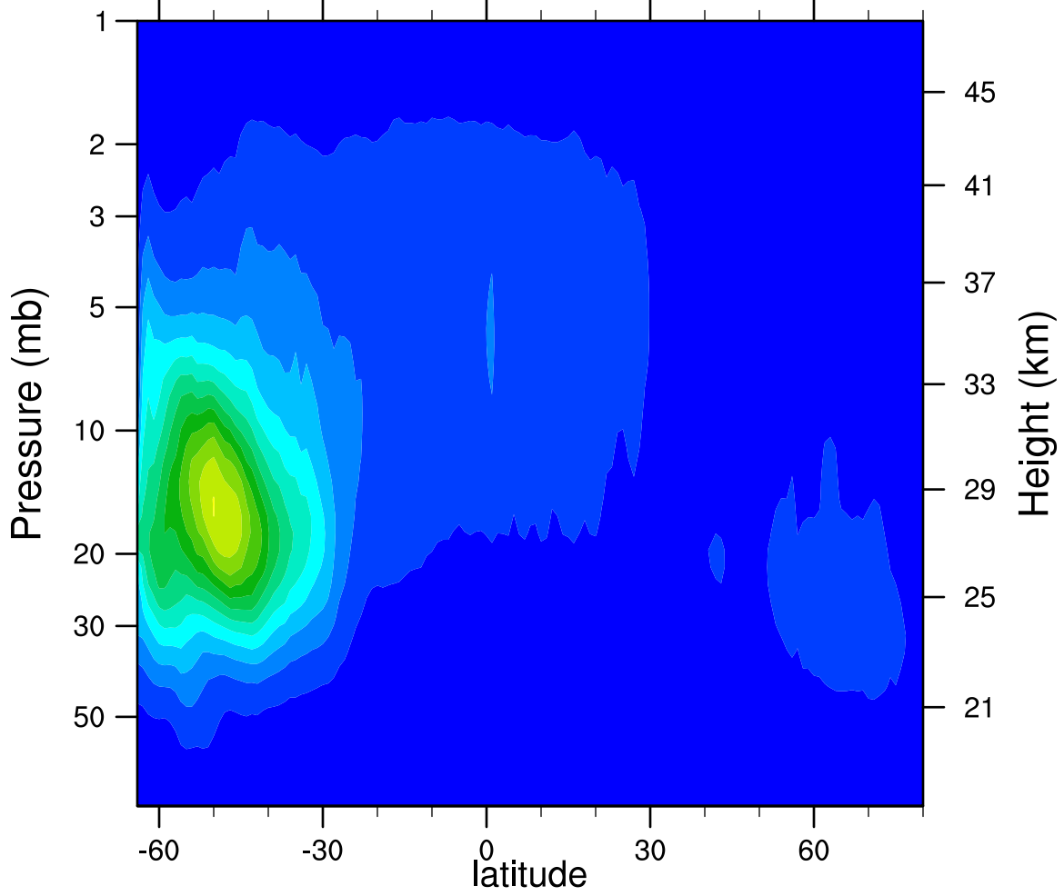
2007d235 N2O5_Ascending (ppbv)
