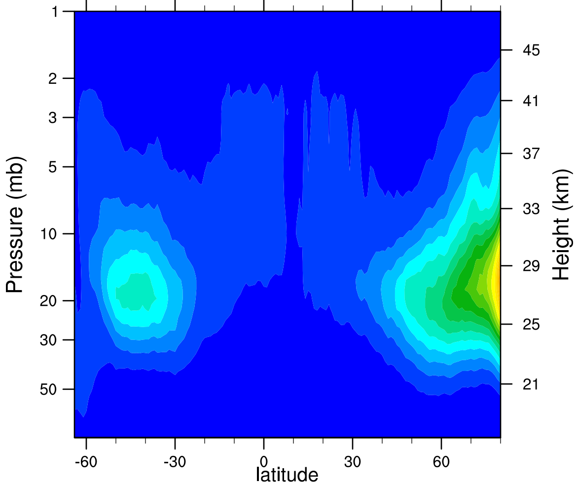
2007d279 N2O5_Ascending (ppbv)
