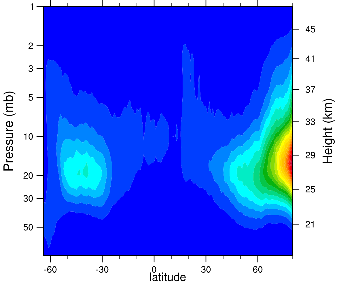
2007d285 N2O5_Ascending (ppbv)
