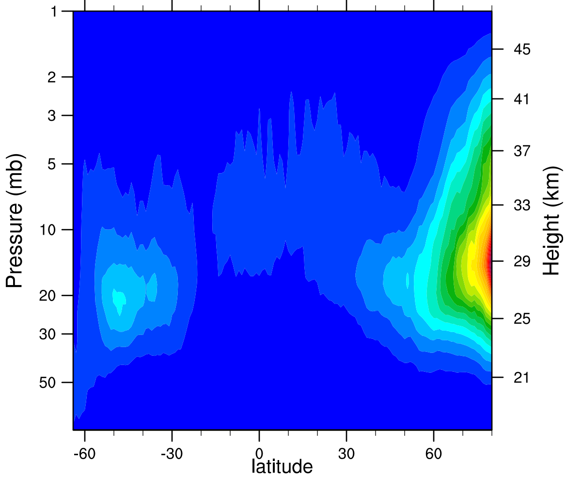
2007d293 N2O5_Ascending (ppbv)
