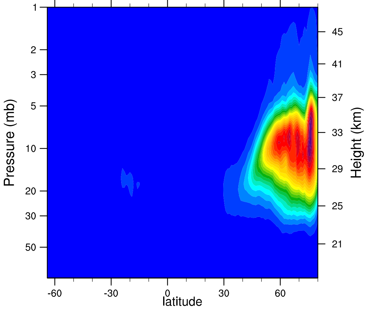
2006d363 N2O5_Ascending (ppbv)
