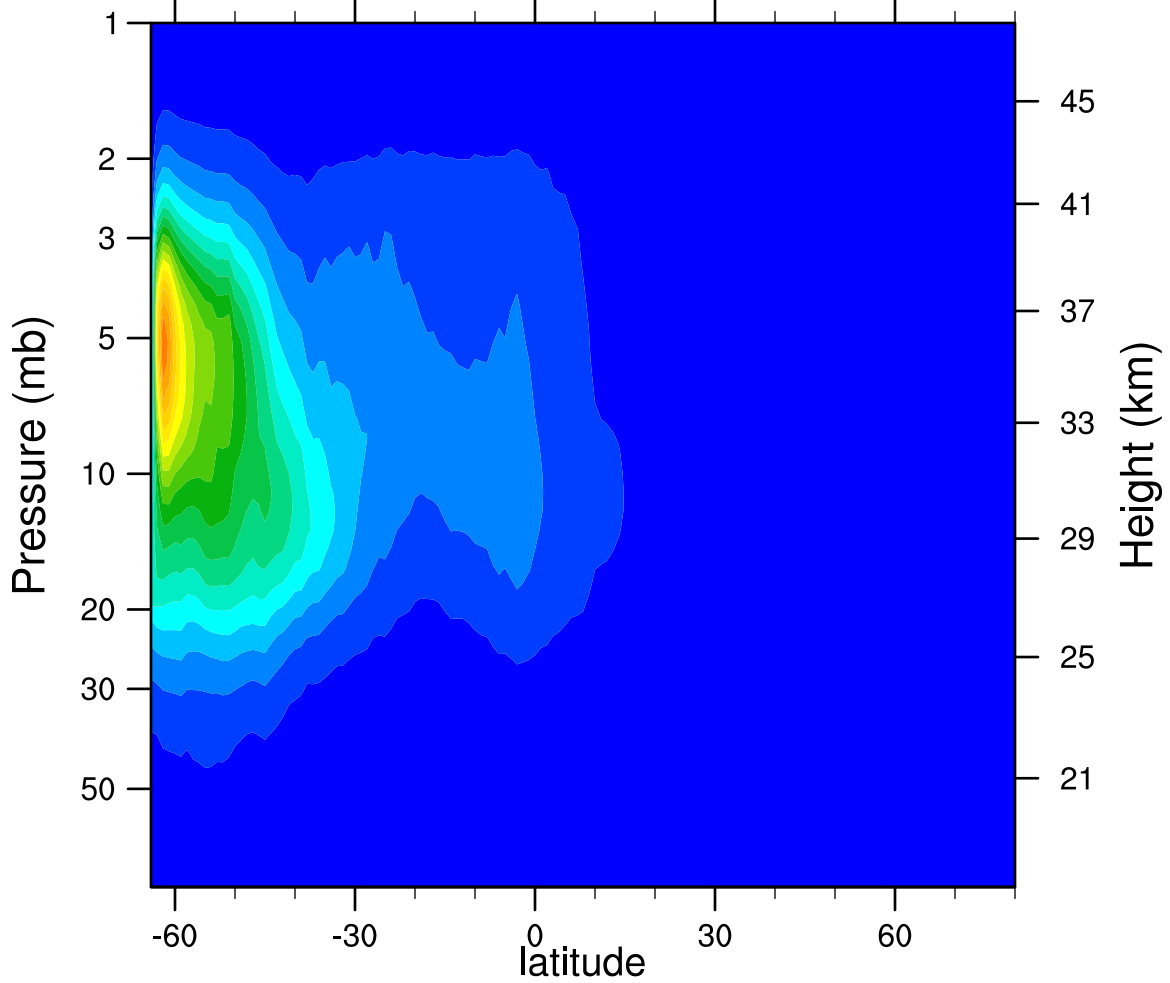
2006d150 N2O5_Ascending (ppbv)
