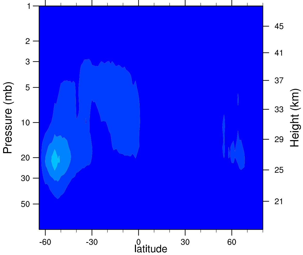
2006d254 N2O5_Ascending (ppbv)
