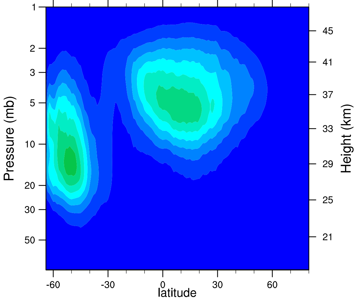
2005d199 N2O5_Ascending (ppbv)
