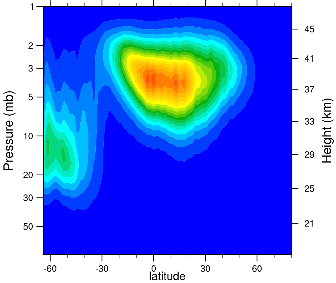
2005d128 N2O5_Ascending (ppbv)
