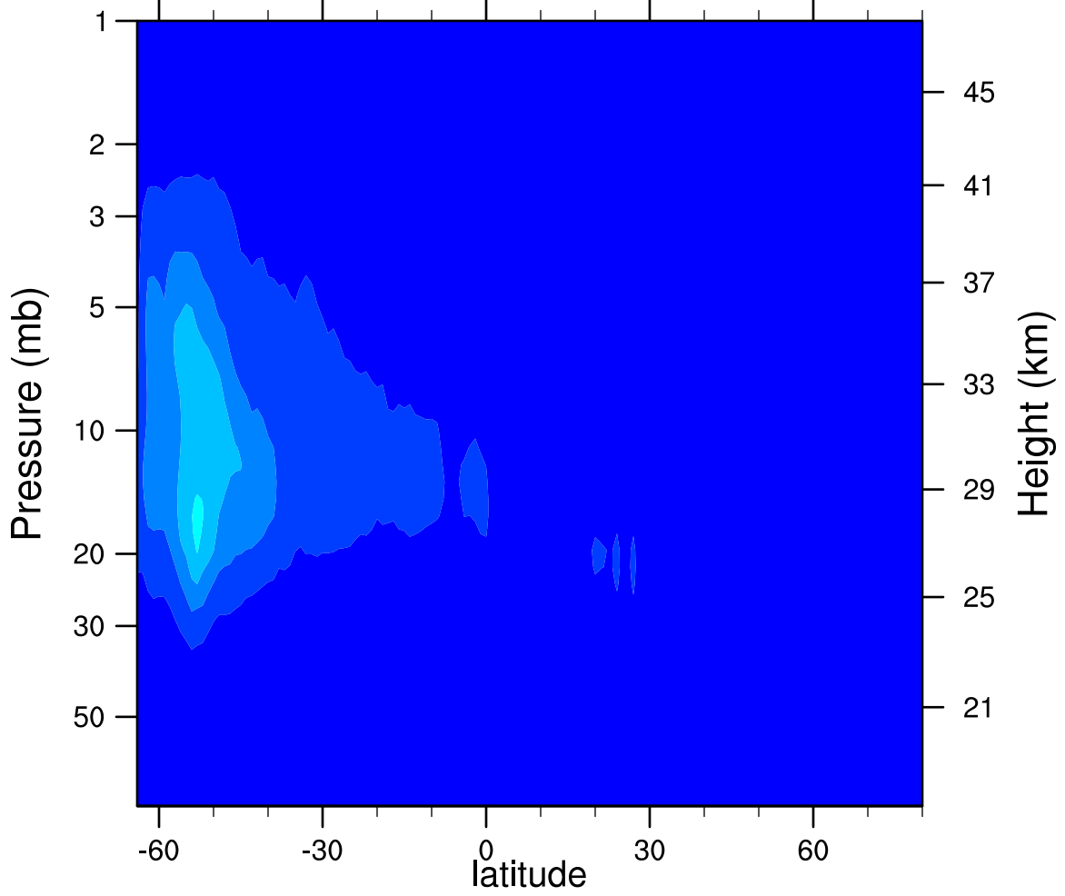
2007d192 N2O5_Ascending (ppbv)
