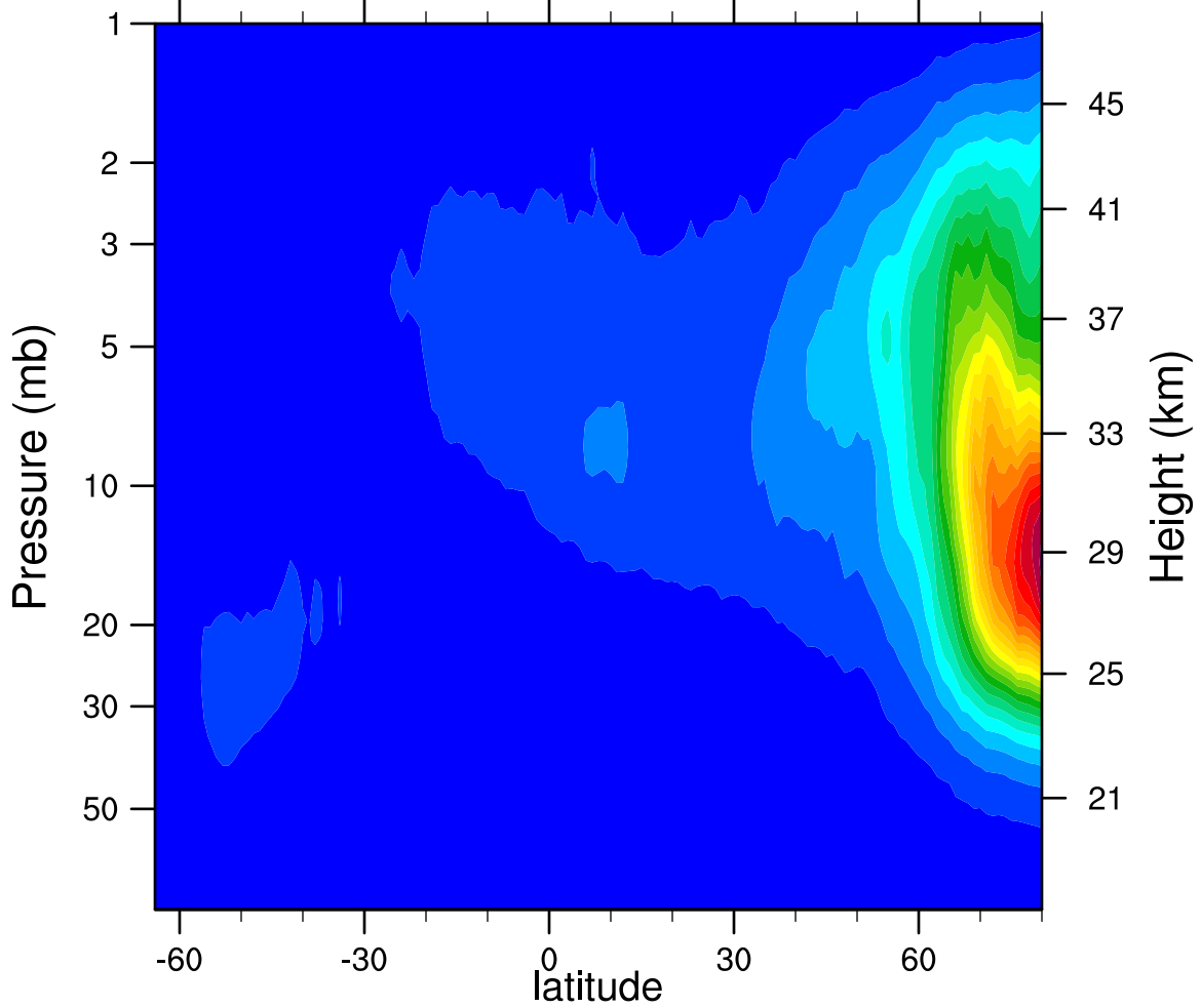
2005d304 N2O5_Ascending (ppbv)
