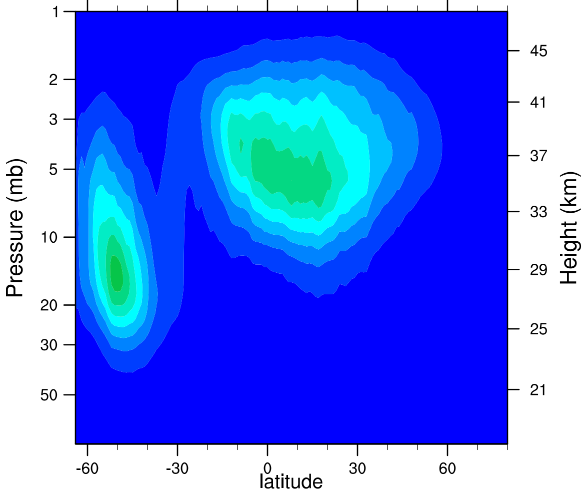
2005d207 N2O5_Ascending (ppbv)
