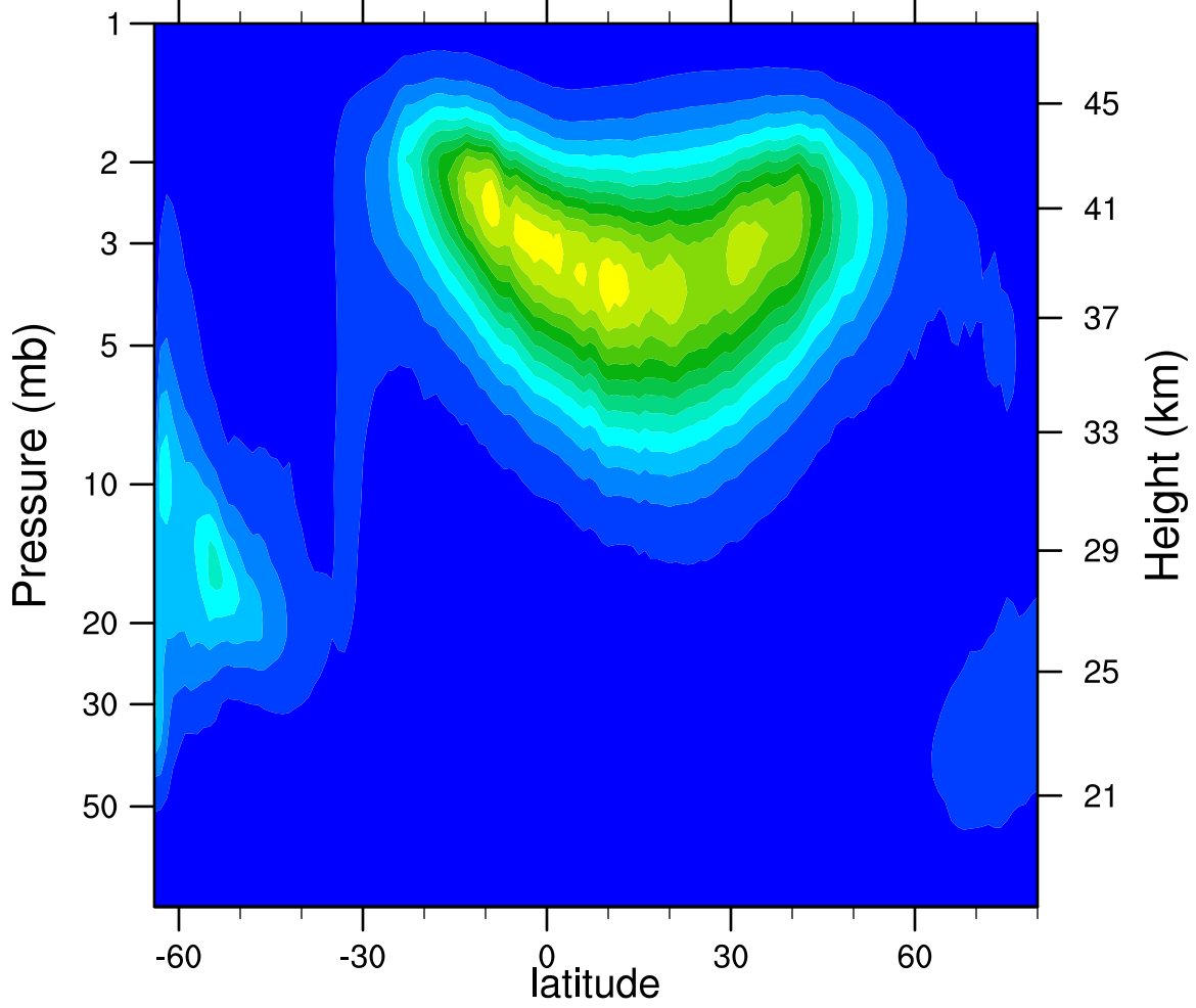
2005d093 N2O5_Ascending (ppbv)
