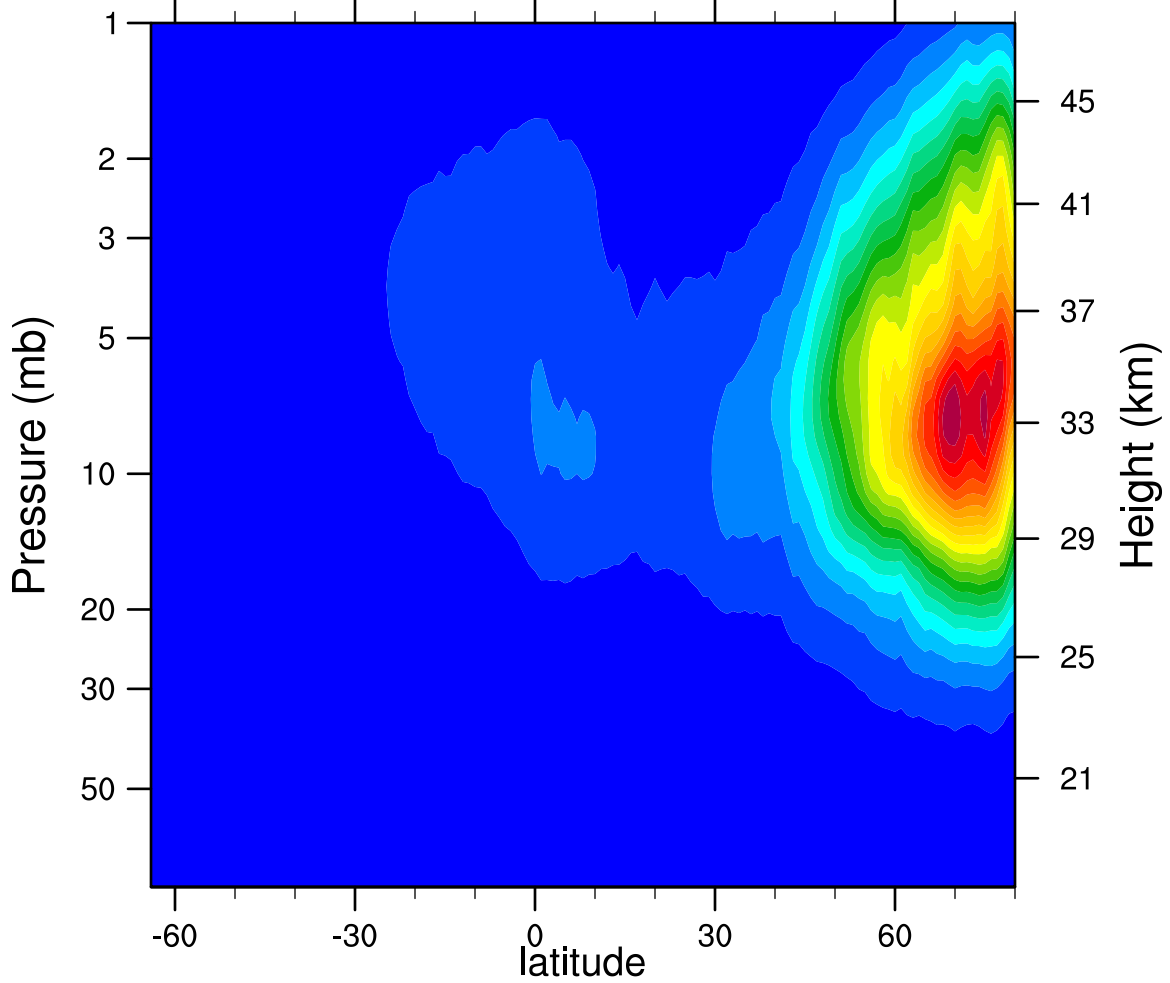
2005d357 N2O5_Ascending (ppbv)
