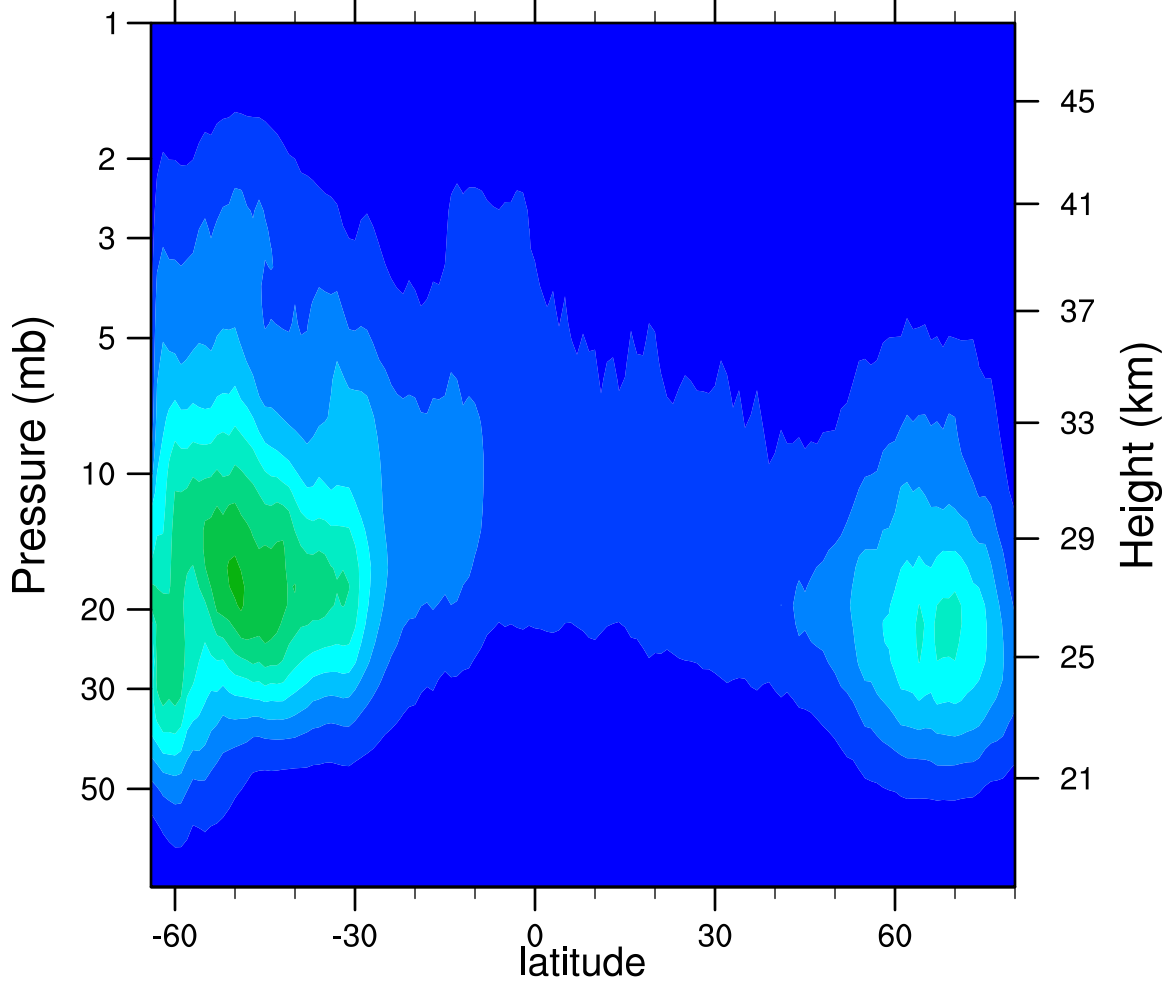
2007d255 N2O5_Ascending (ppbv)
