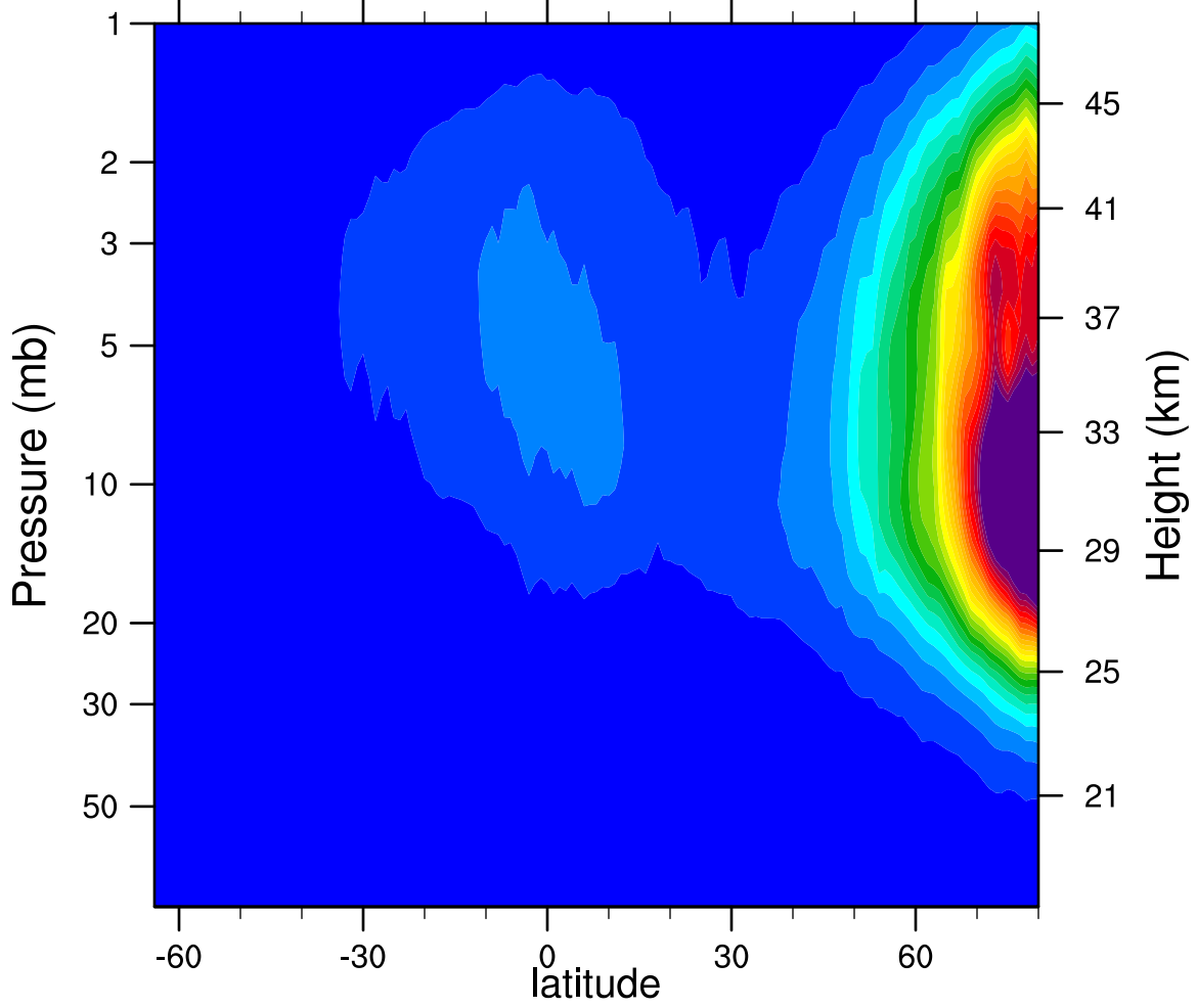
2006d018 N2O5_Ascending (ppbv)
