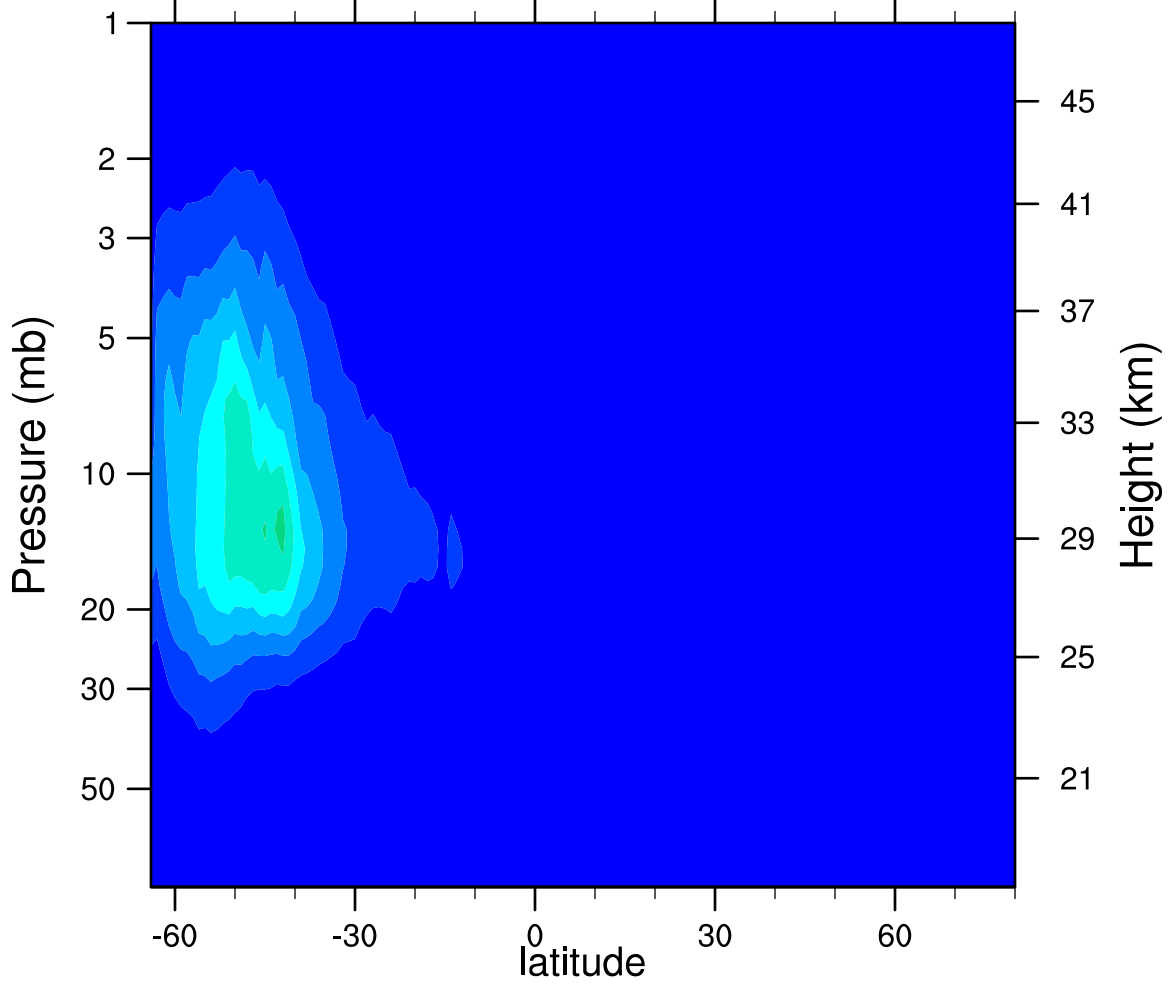
2007d202 N2O5_Ascending (ppbv)
