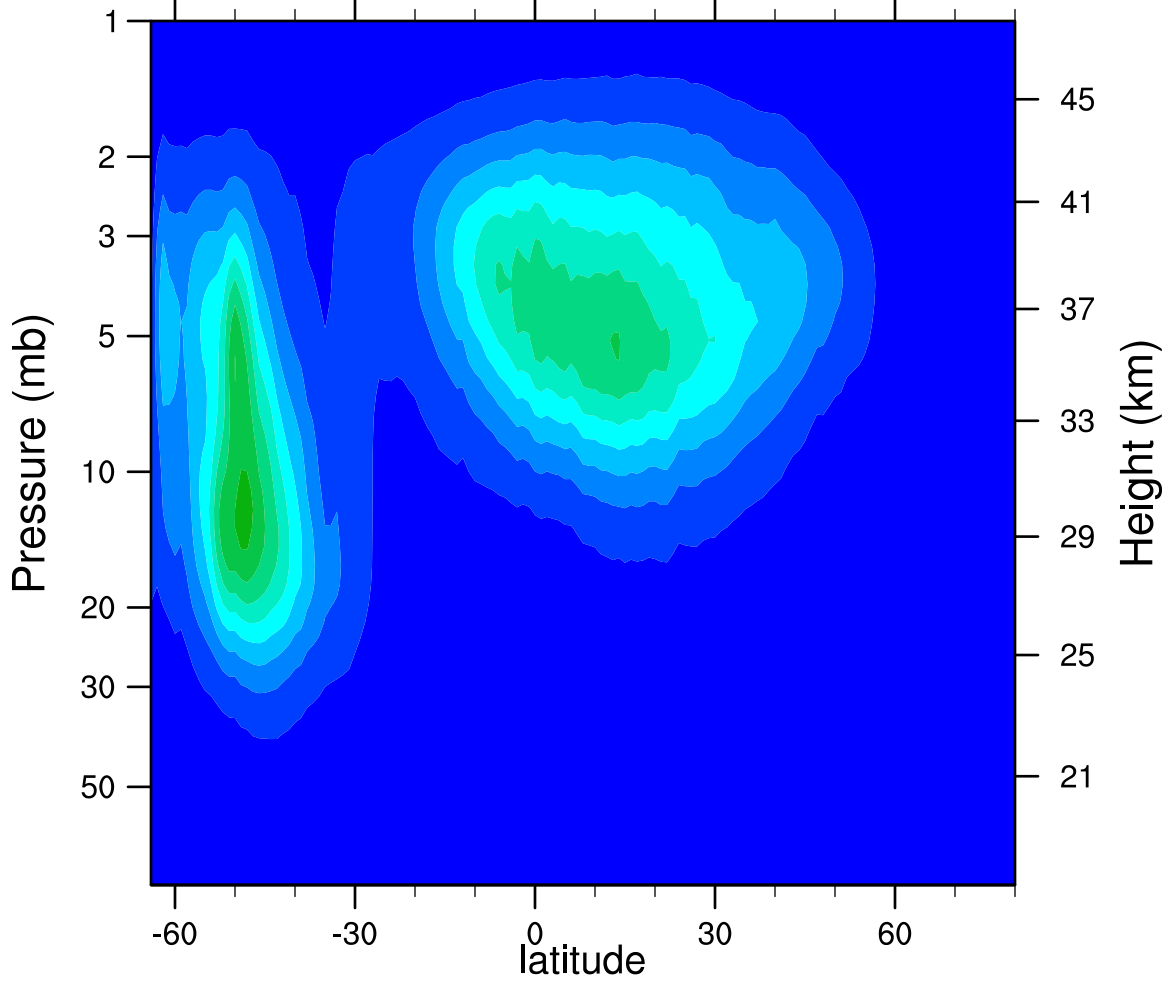
2005d185 N2O5_Ascending (ppbv)
