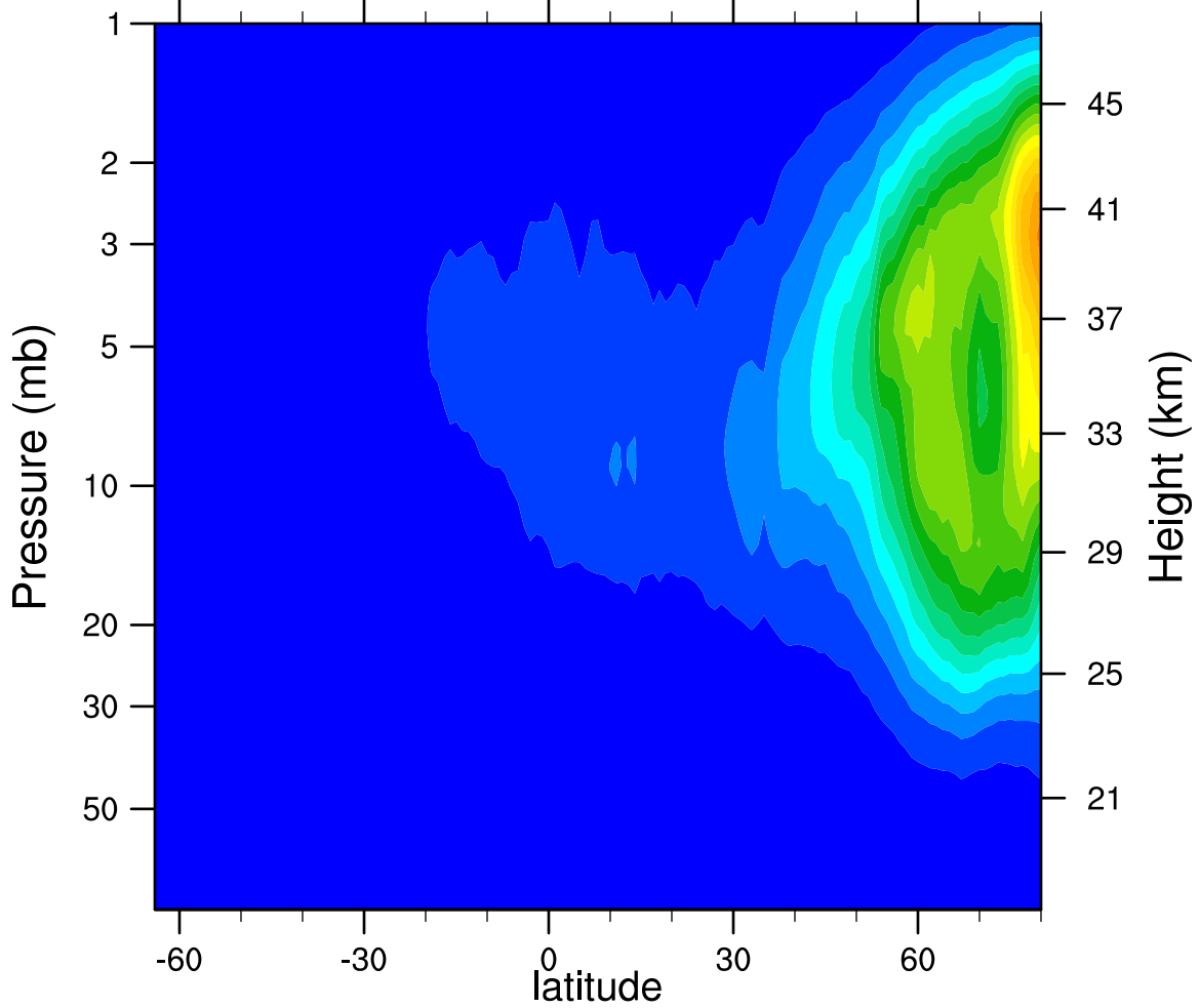
2005d323 N2O5_Ascending (ppbv)
