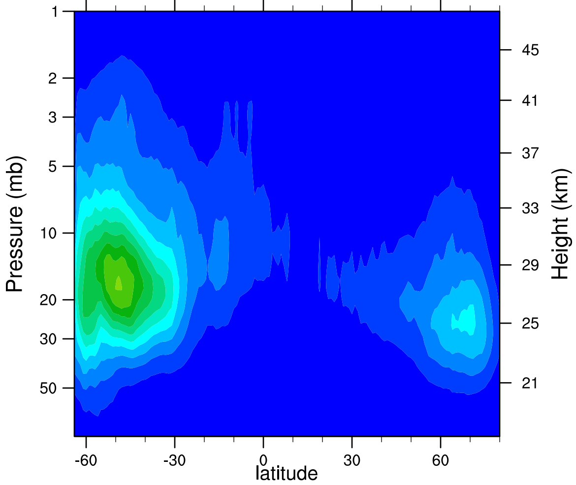
2007d248 N2O5_Ascending (ppbv)
