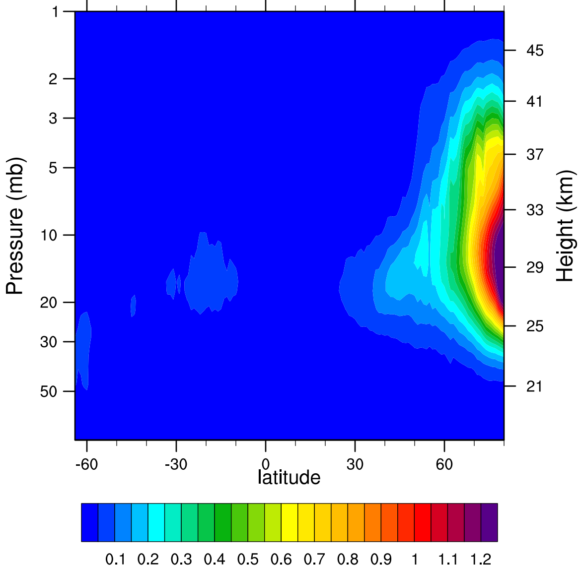
2006d304 N2O5_Ascending (ppbv)
