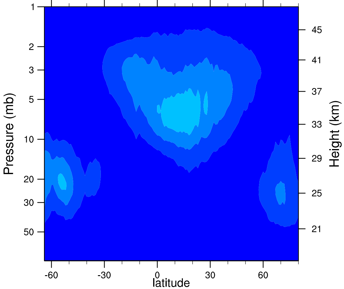
2005d258 N2O5_Ascending (ppbv)
