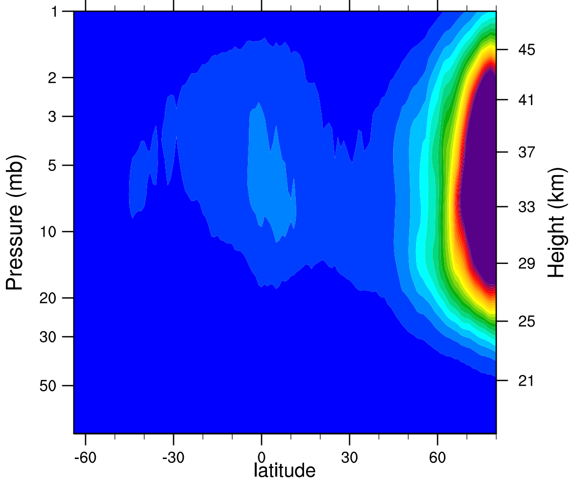
2006d029 N2O5_Ascending (ppbv)
