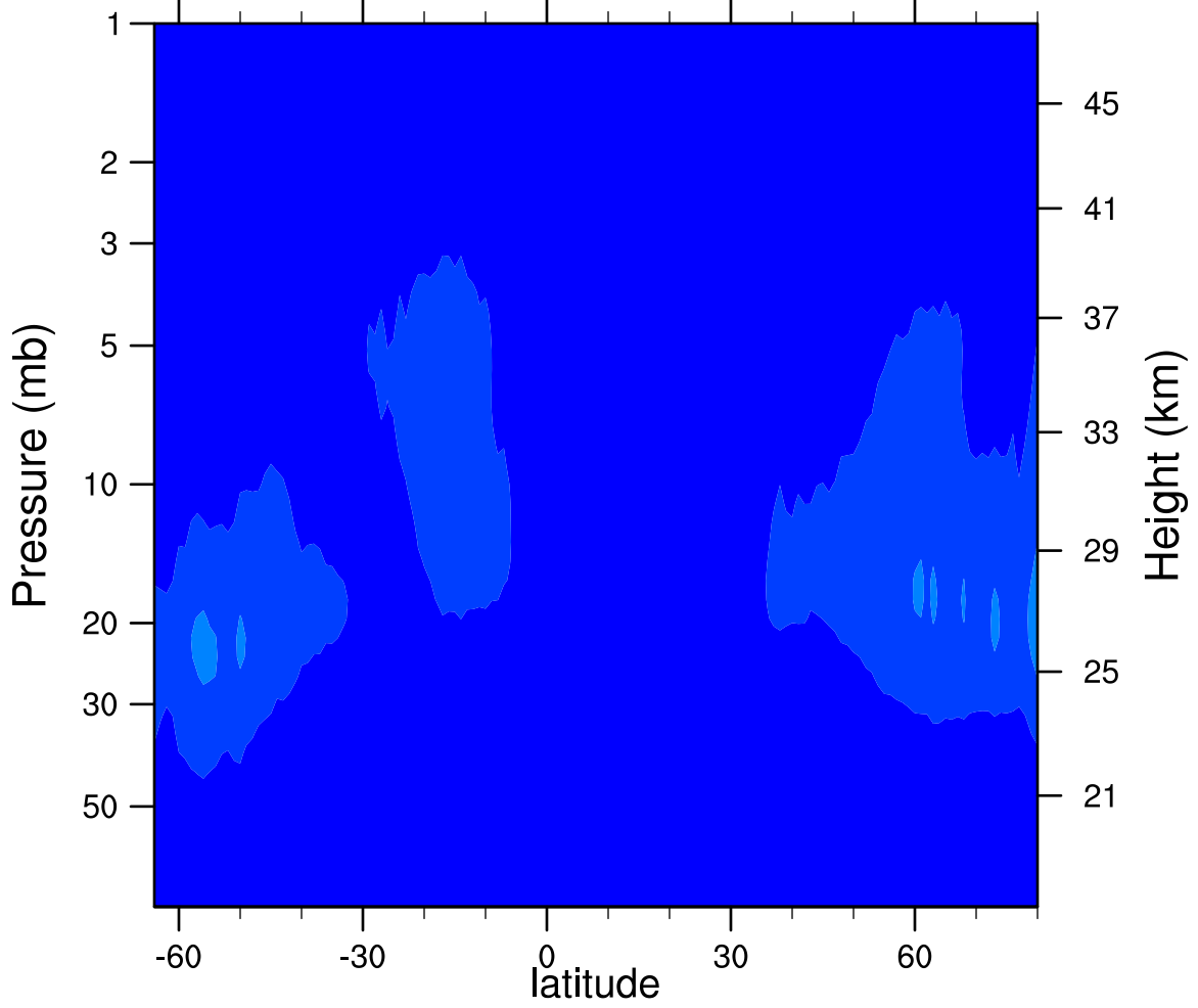
2006d269 N2O5_Ascending (ppbv)
