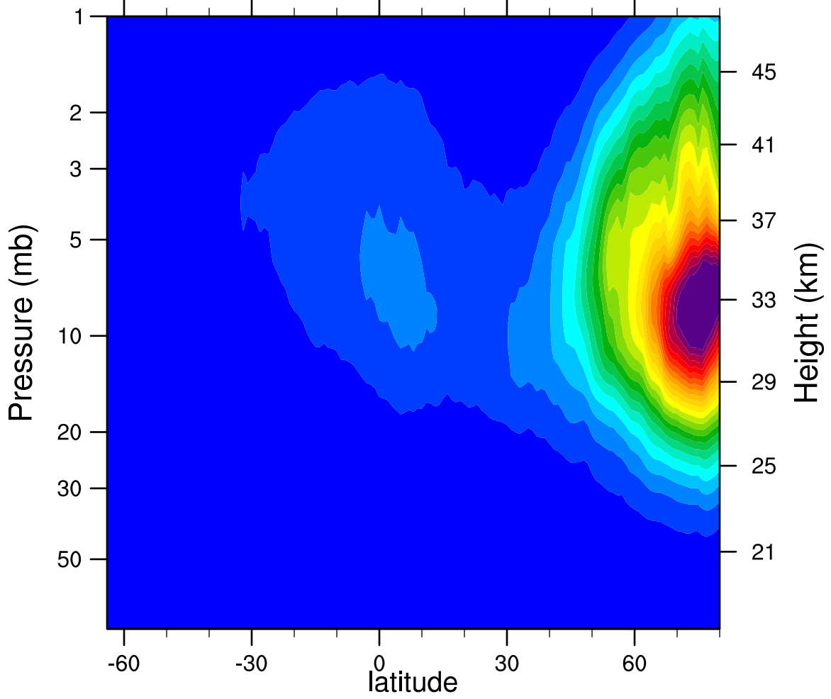
2006d003 N2O5_Ascending (ppbv)
