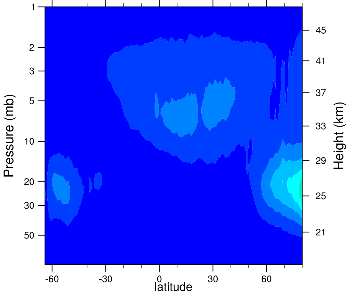
2005d277 N2O5_Ascending (ppbv)
