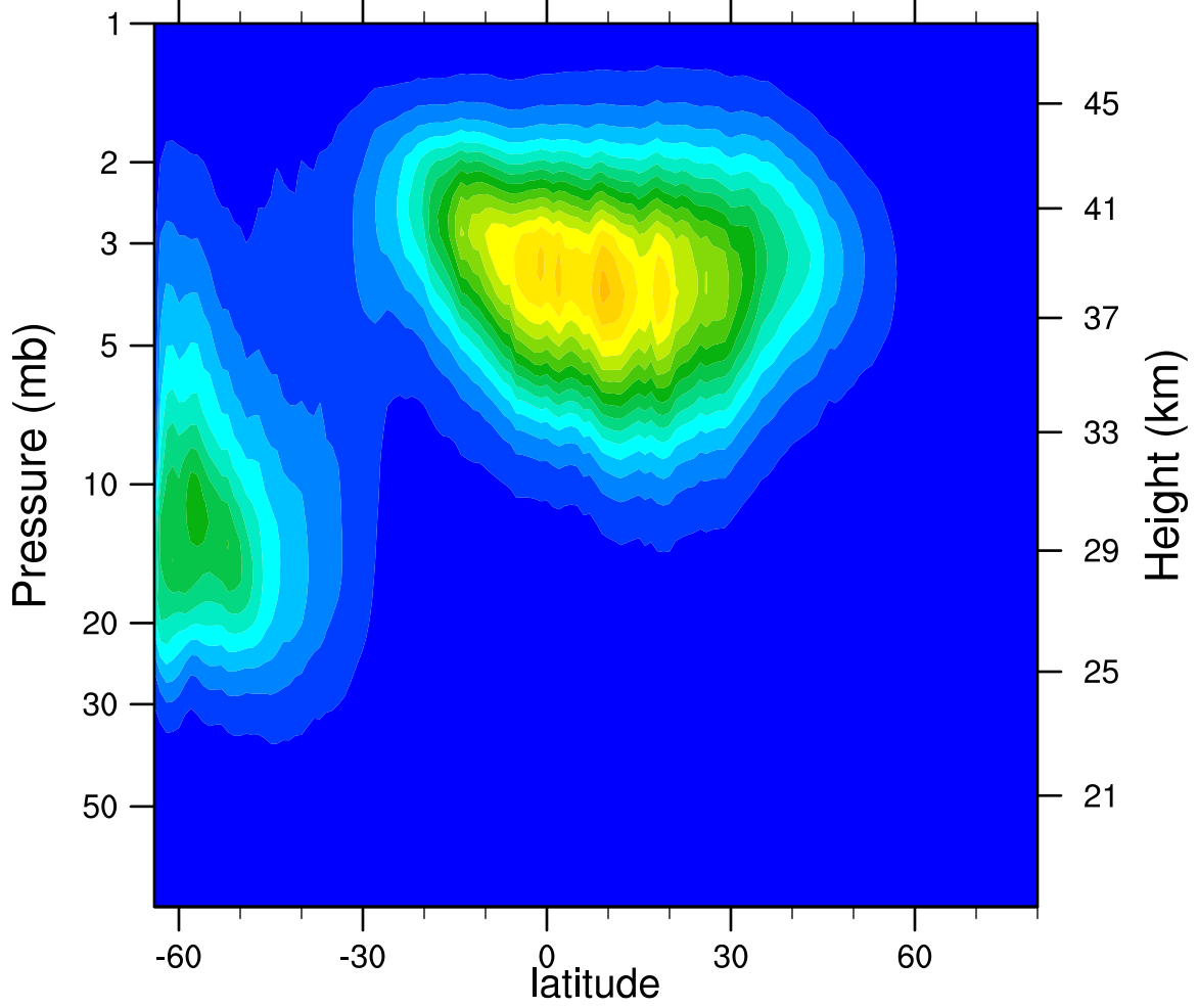
2005d142 N2O5_Ascending (ppbv)
