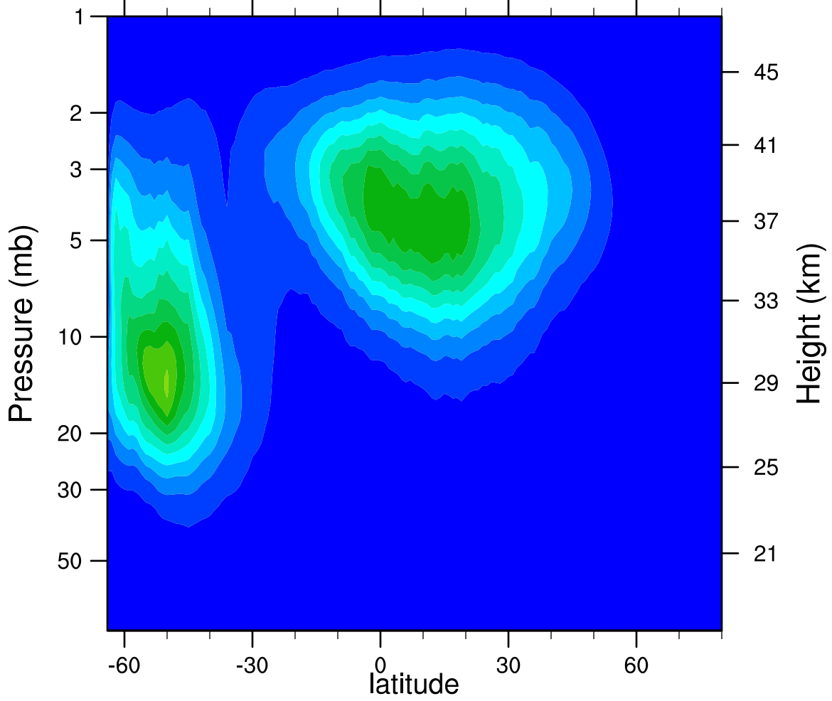
2005d165 N2O5_Ascending (ppbv)
