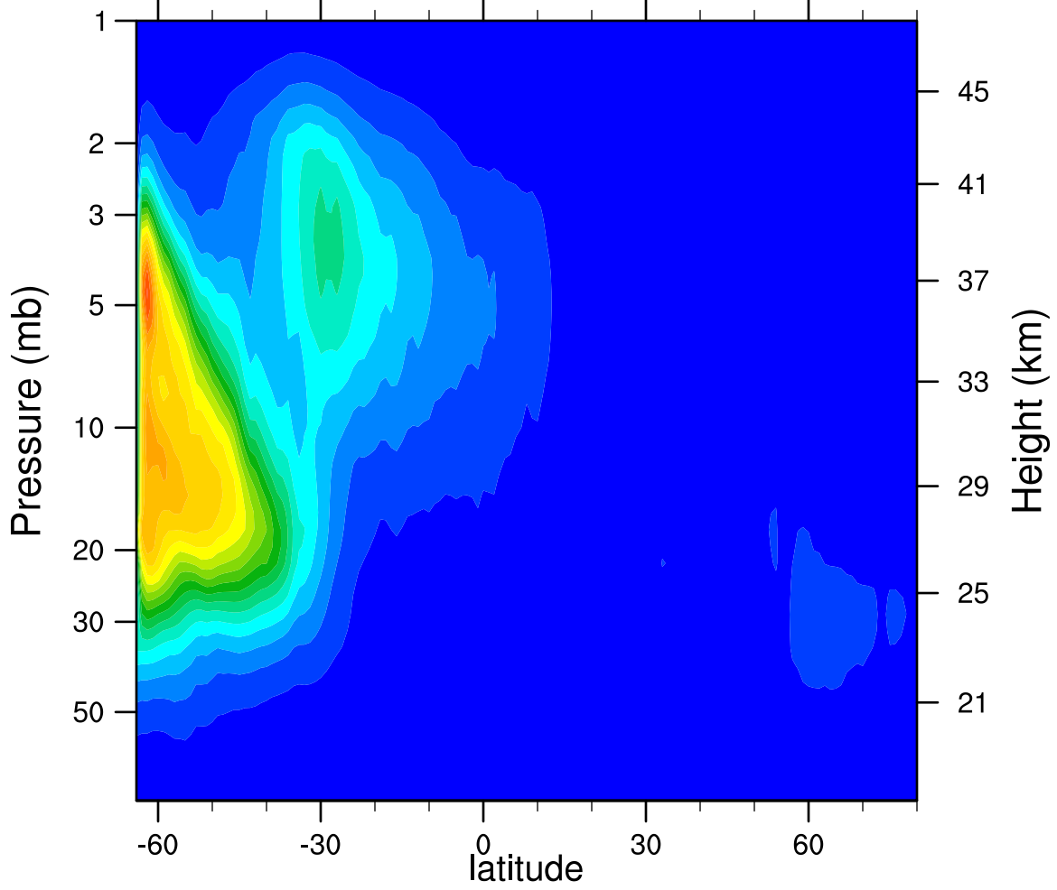
2007d115 N2O5_Ascending (ppbv)
