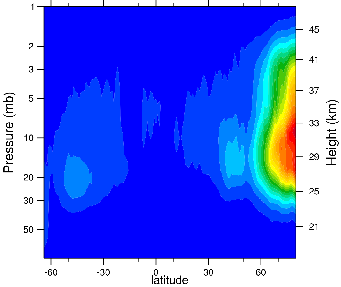
2006d318 N2O5_Ascending (ppbv)
