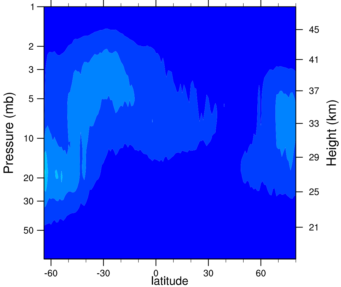
2006d087 N2O5_Ascending (ppbv)
