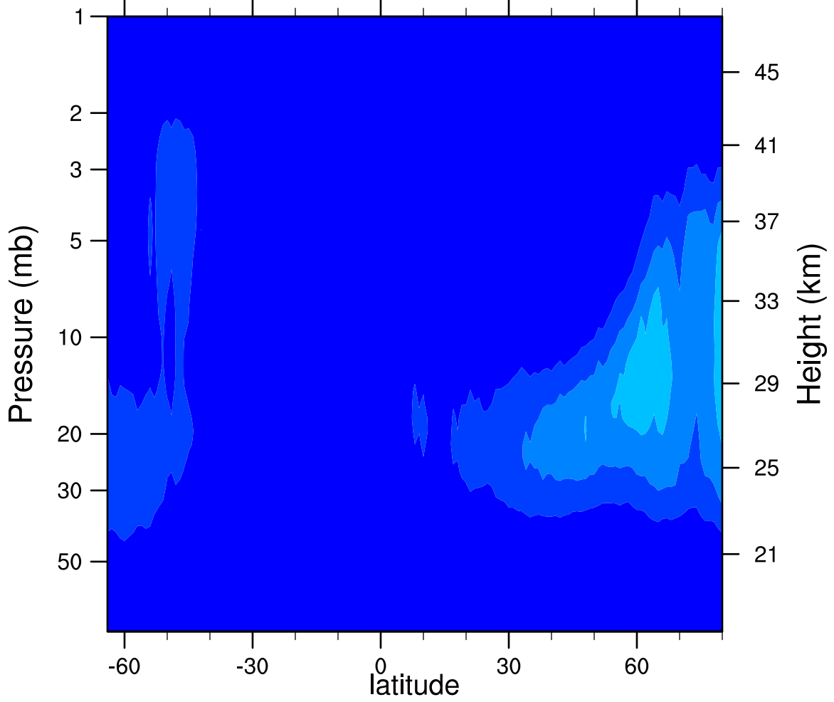
2007d073 N2O5_Ascending (ppbv)
