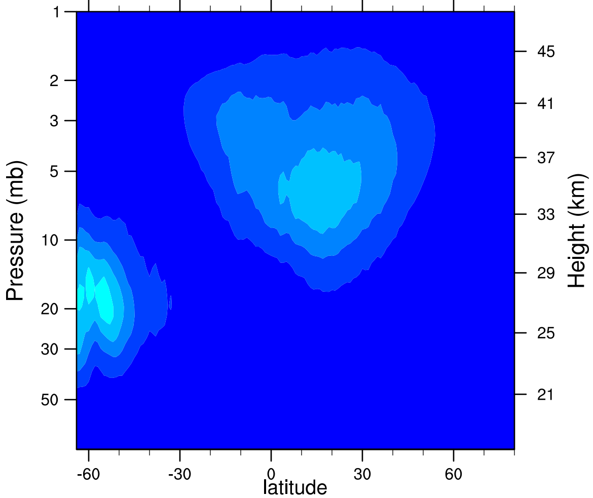
2005d246 N2O5_Ascending (ppbv)
