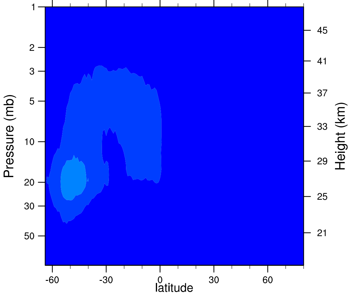
2006d249 N2O5_Ascending (ppbv)
