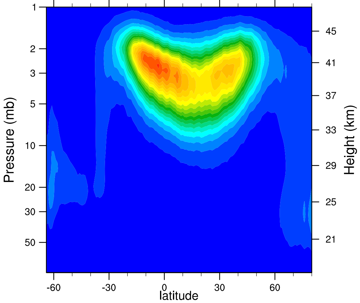
2005d075 N2O5_Ascending (ppbv)
