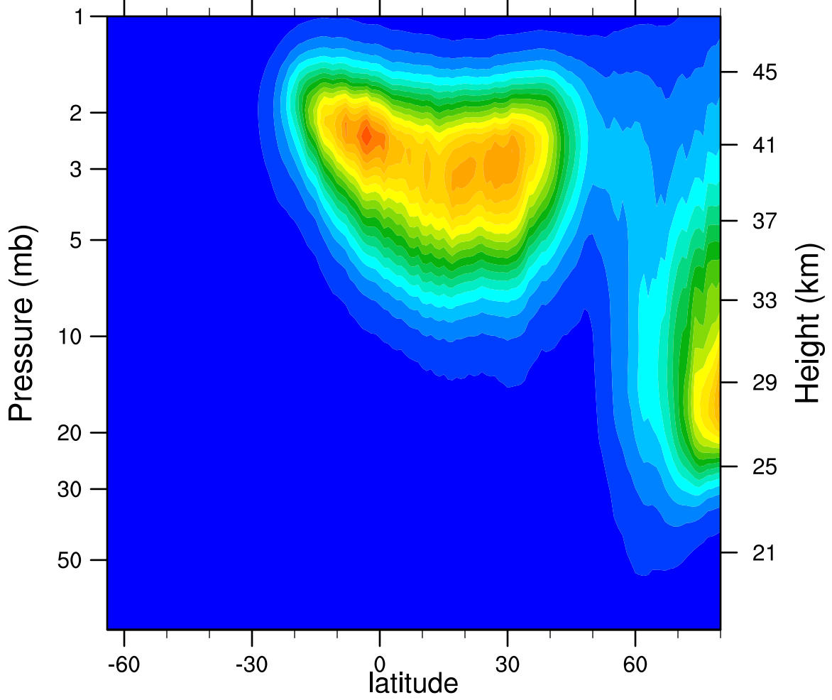
2005d032 N2O5_Ascending (ppbv)
