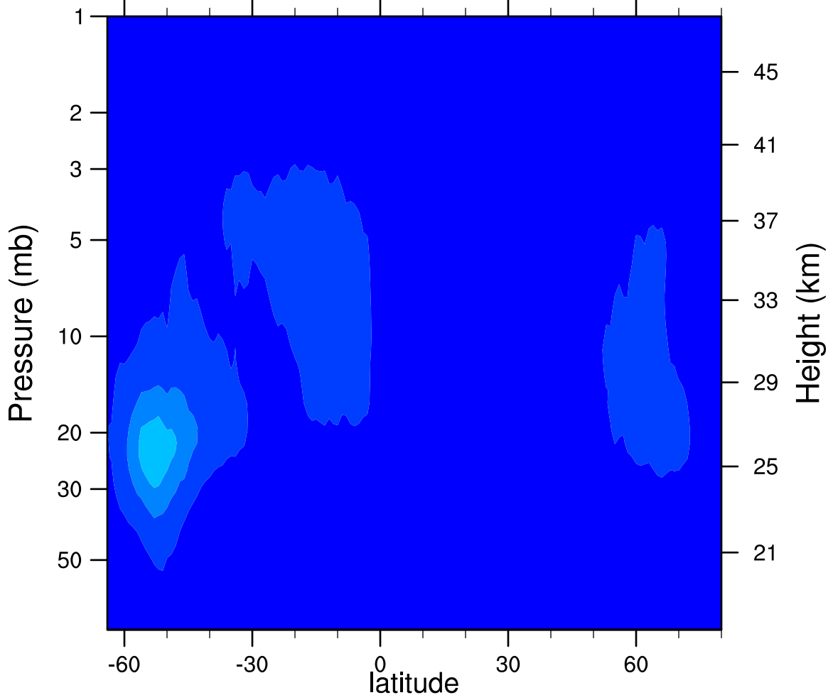
2006d260 N2O5_Ascending (ppbv)
