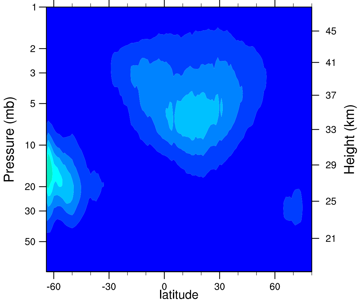
2005d249 N2O5_Ascending (ppbv)
