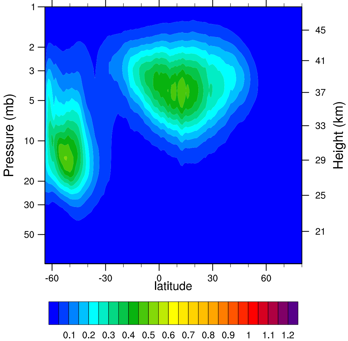
2005d158 N2O5_Ascending (ppbv)
