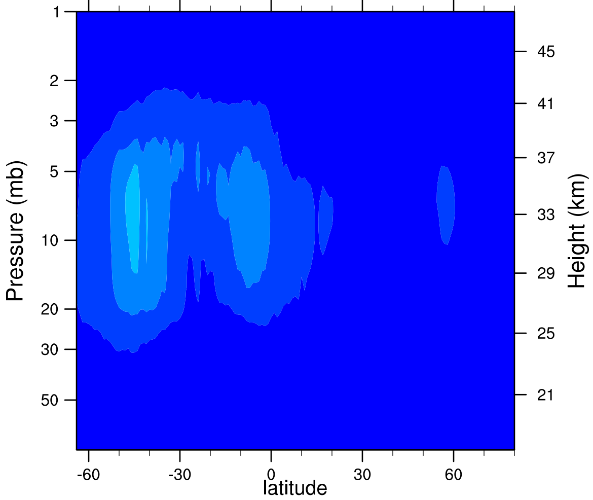
2006d214 N2O5_Ascending (ppbv)
