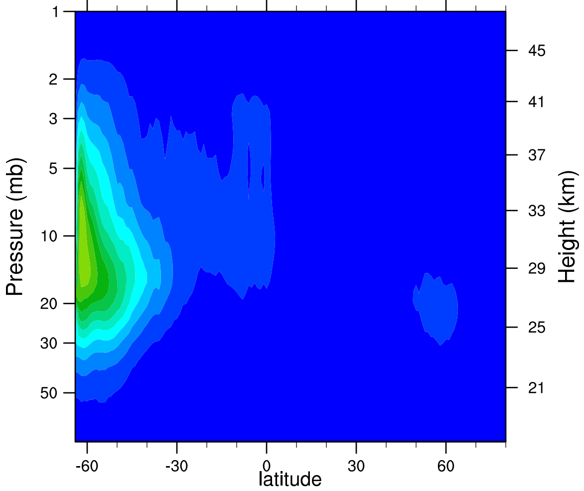
2006d119 N2O5_Ascending (ppbv)
