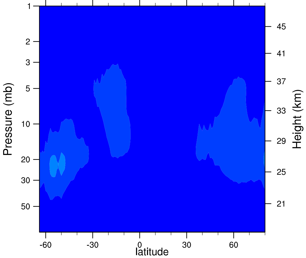
2006d268 N2O5_Ascending (ppbv)
