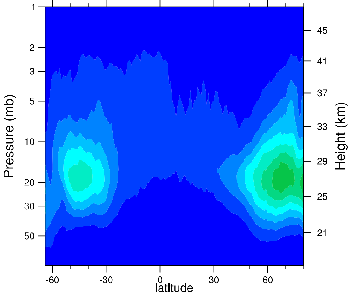
2007d271 N2O5_Ascending (ppbv)
