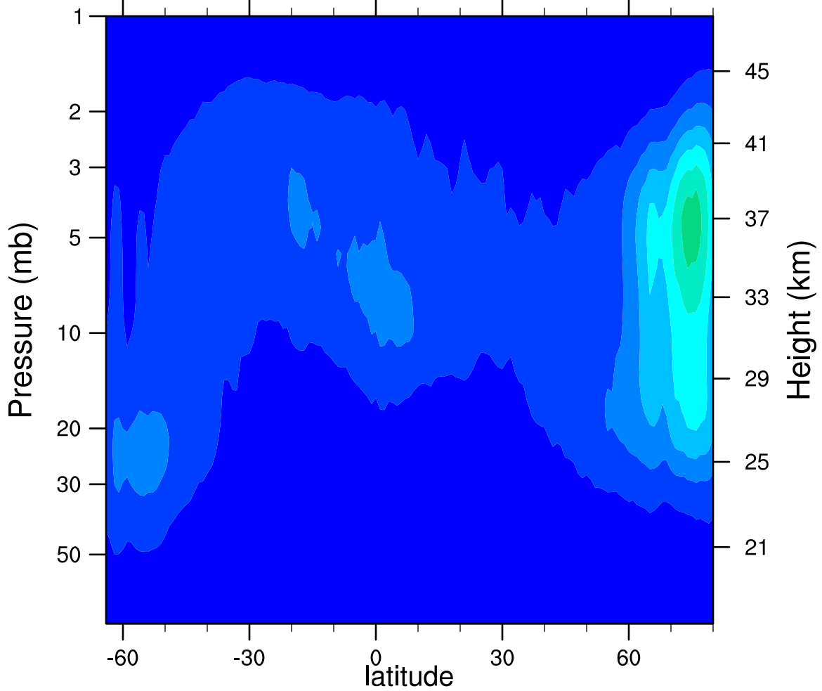
2006d070 N2O5_Ascending (ppbv)
