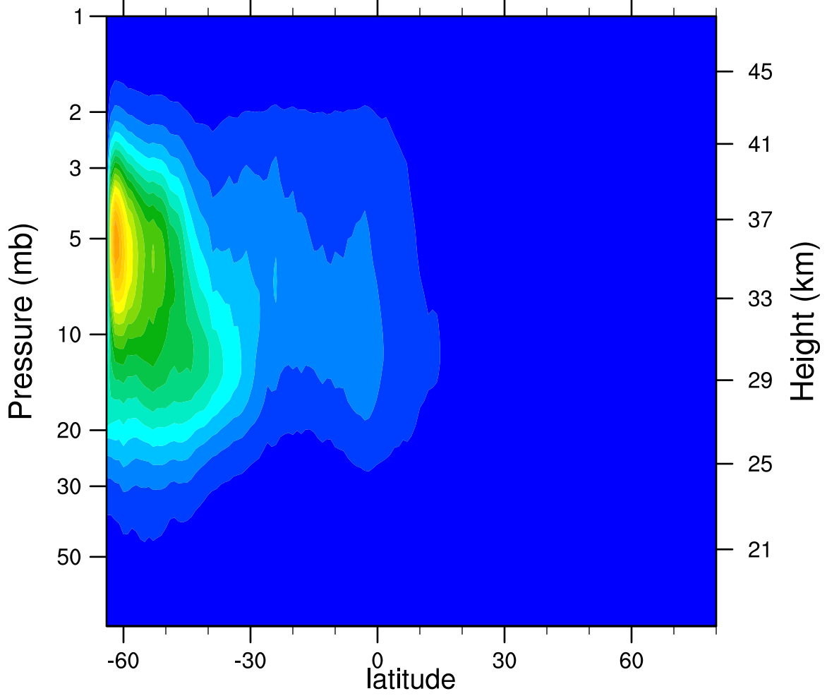
2006d153 N2O5_Ascending (ppbv)
