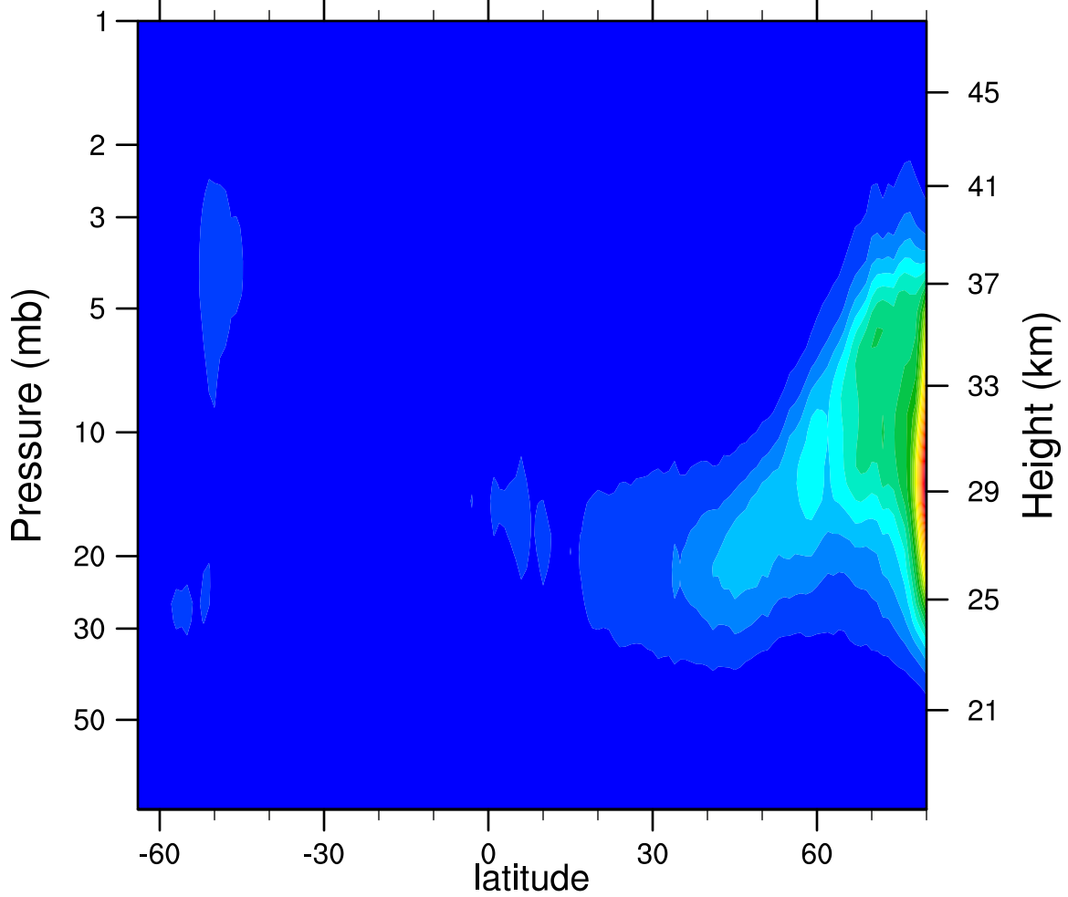
2007d058 N2O5_Ascending (ppbv)
