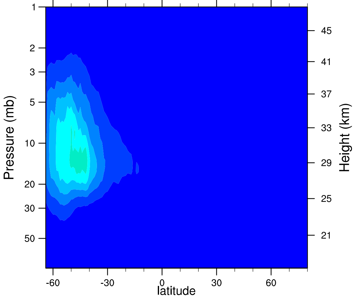
2007d201 N2O5_Ascending (ppbv)
