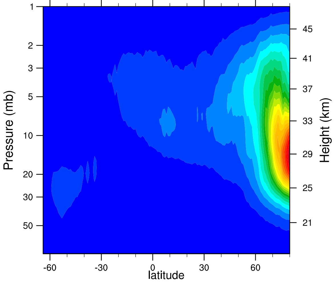
2005d301 N2O5_Ascending (ppbv)
