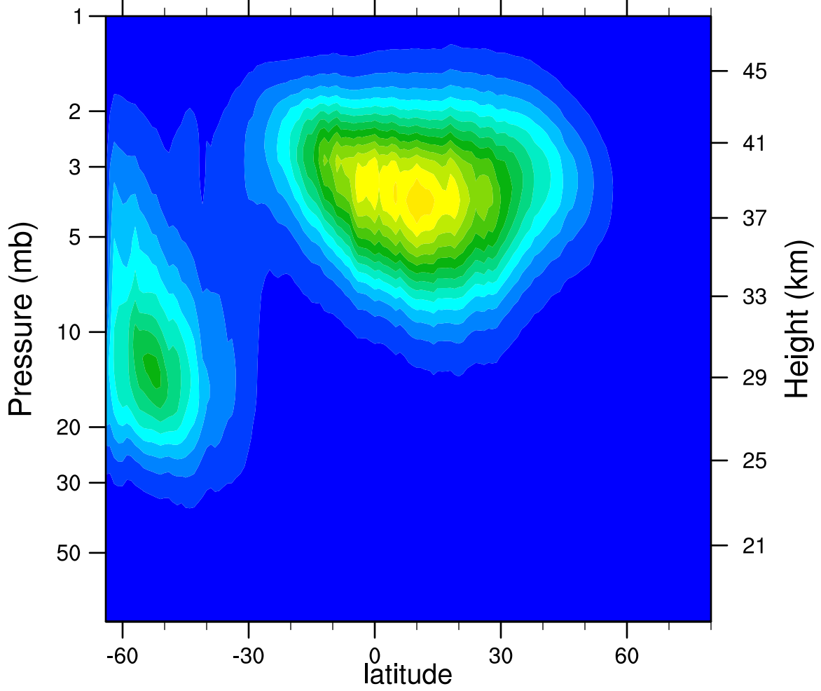
2005d146 N2O5_Ascending (ppbv)
