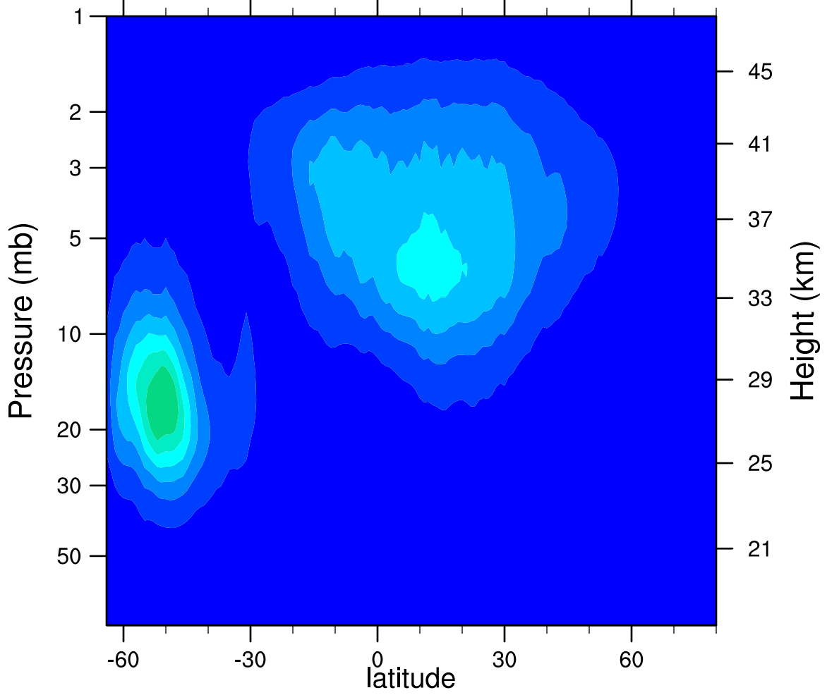
2005d228 N2O5_Ascending (ppbv)
