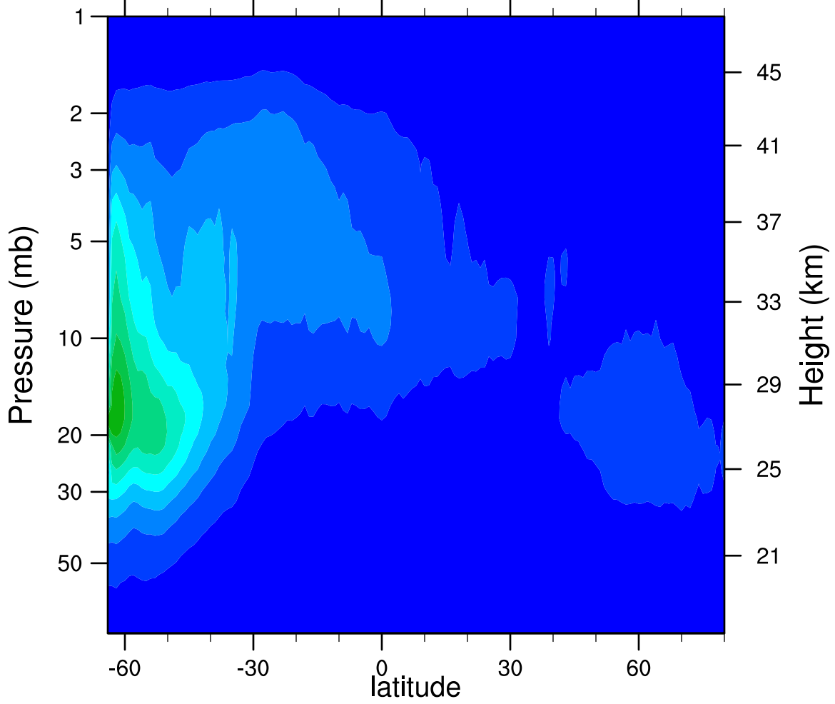
2006d105 N2O5_Ascending (ppbv)
