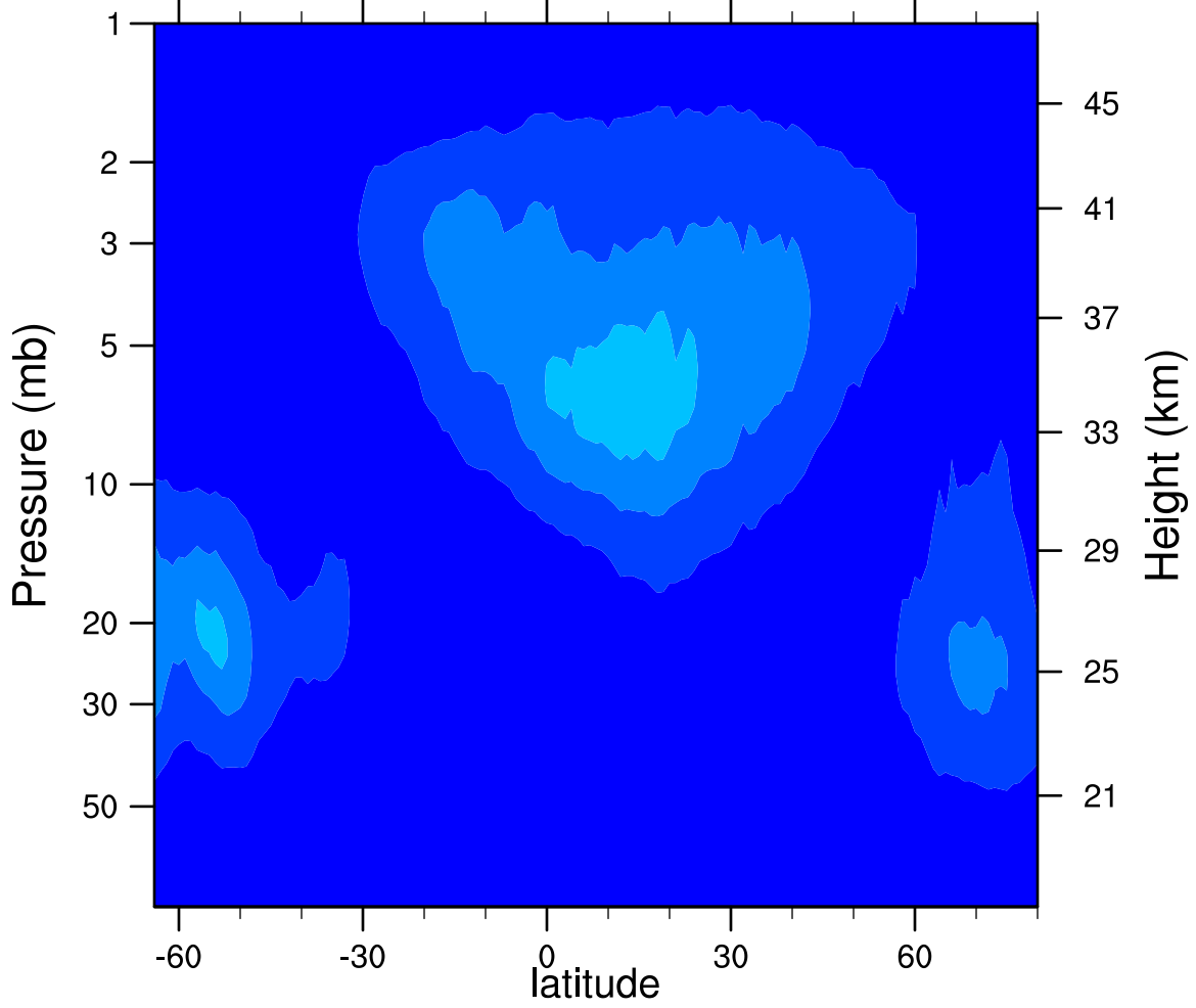
2005d260 N2O5_Ascending (ppbv)
