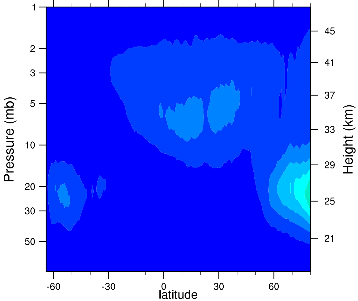
2005d278 N2O5_Ascending (ppbv)
