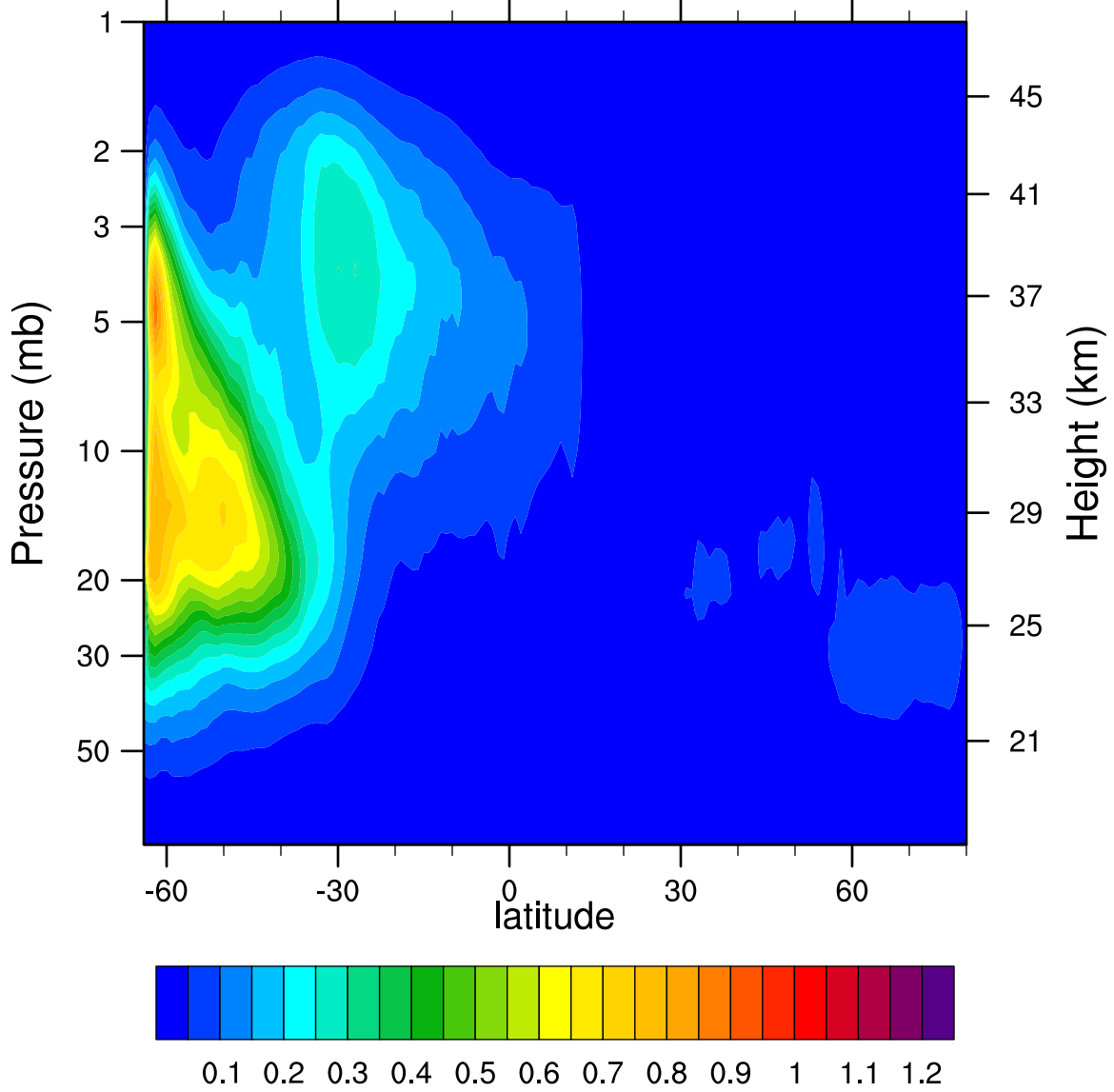
2007d112 N2O5_Ascending (ppbv)
