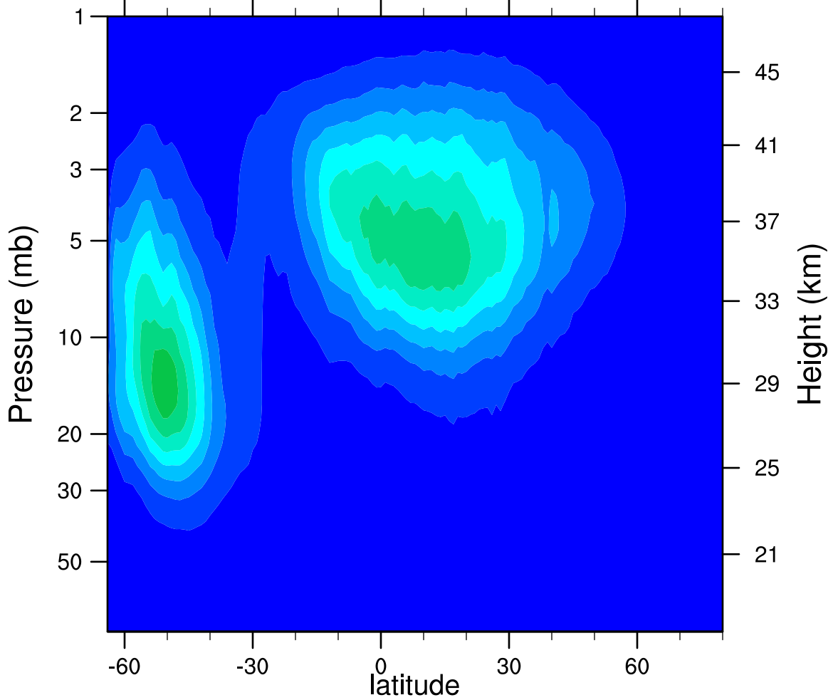
2005d202 N2O5_Ascending (ppbv)
