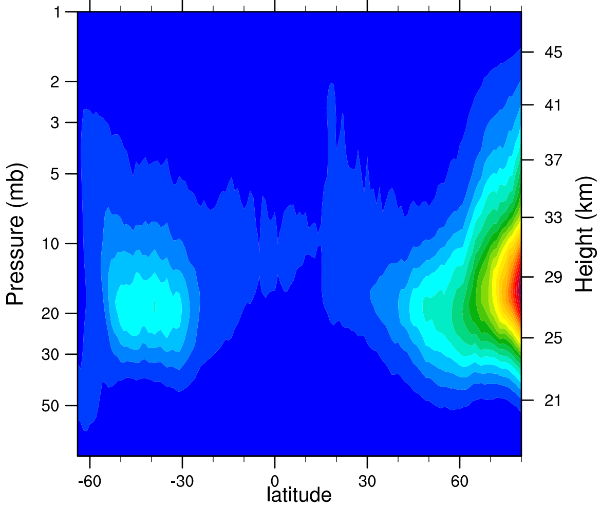
2007d286 N2O5_Ascending (ppbv)
