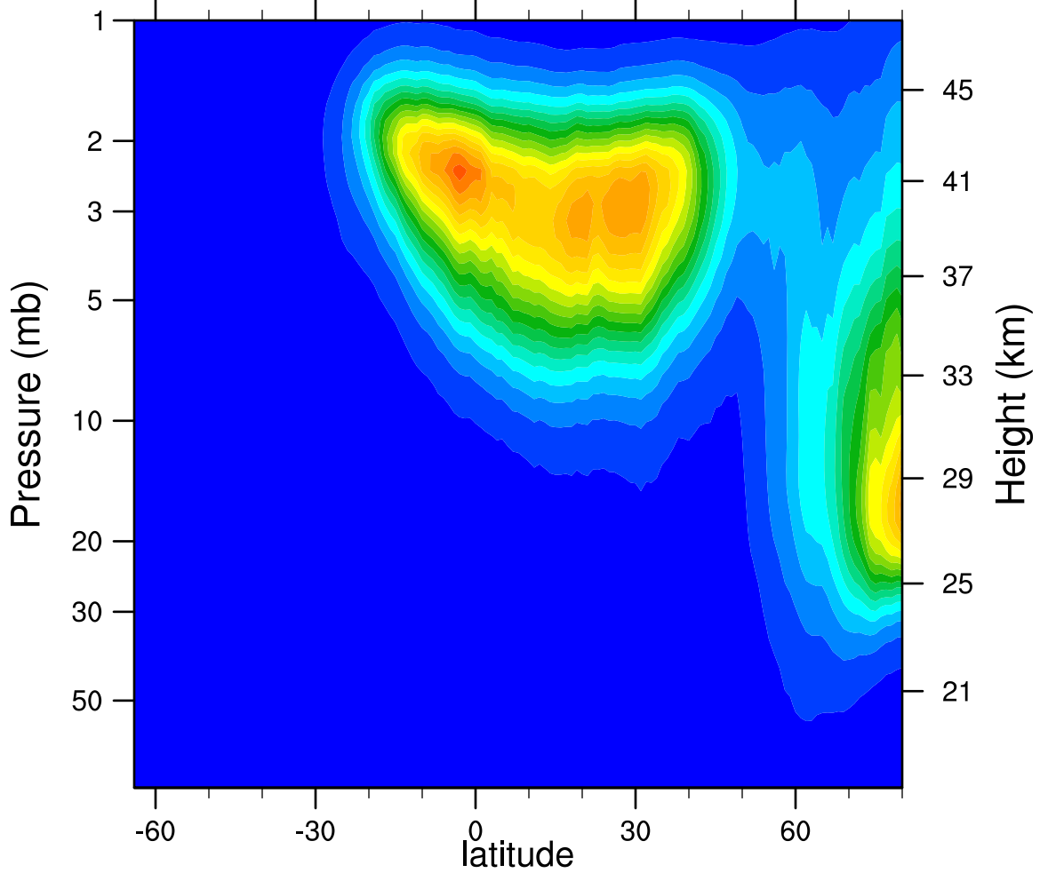
2005d033 N2O5_Ascending (ppbv)
