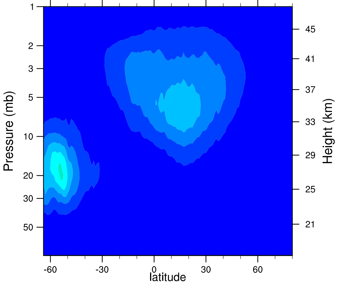
2005d241 N2O5_Ascending (ppbv)
