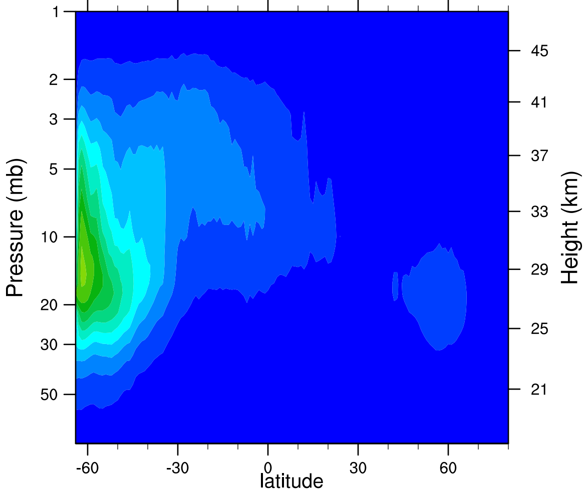
2006d111 N2O5_Ascending (ppbv)
