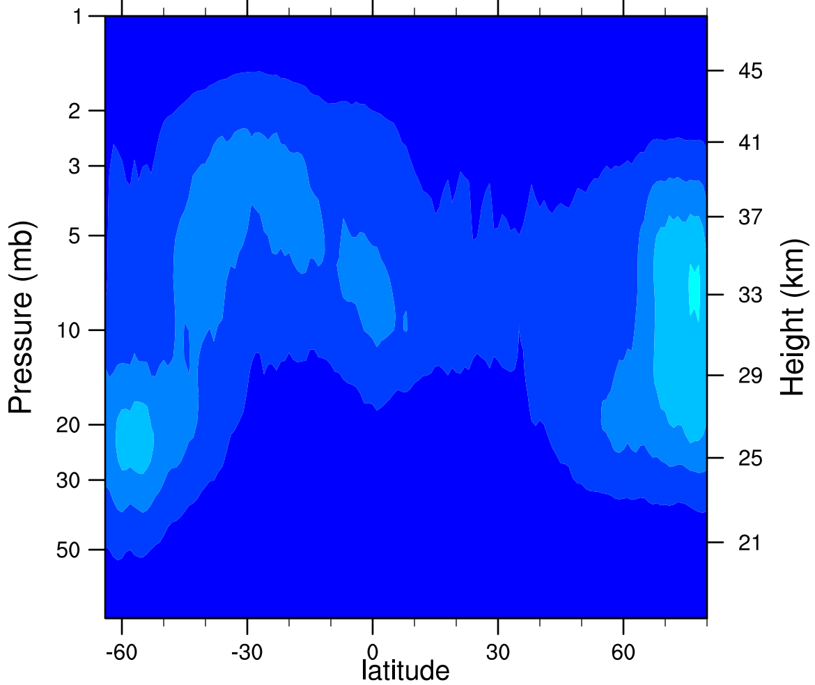
2006d080 N2O5_Ascending (ppbv)
