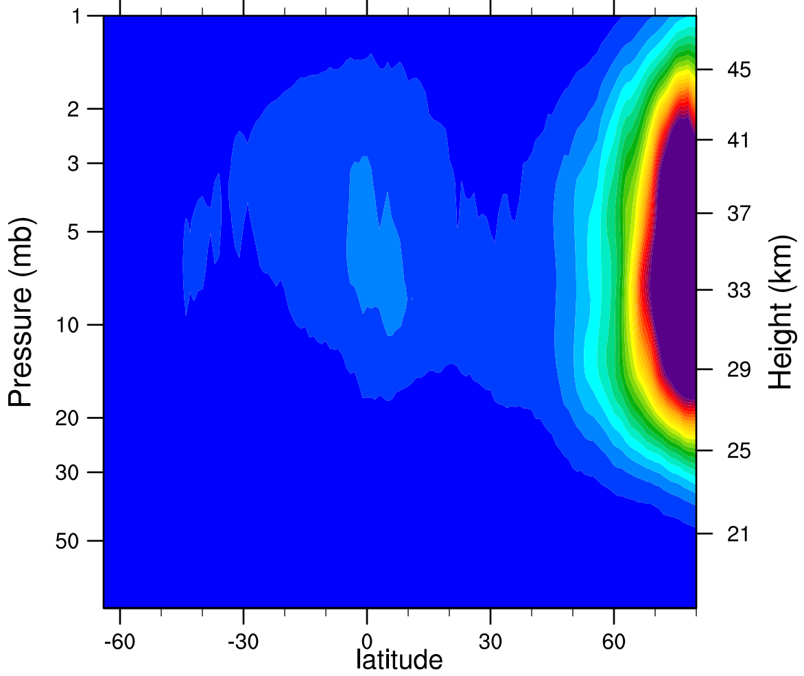
2006d030 N2O5_Ascending (ppbv)
