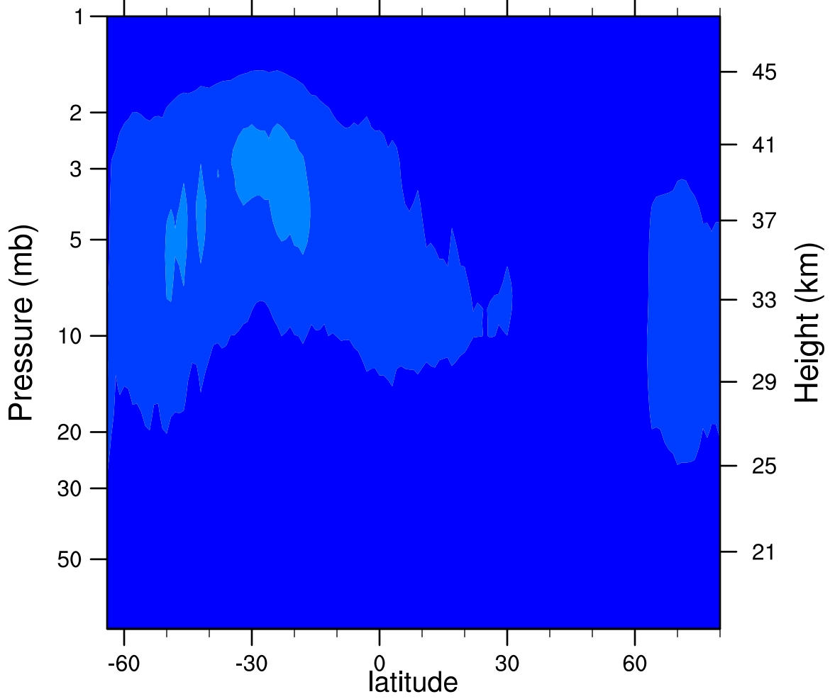
2006d092 N2O5_Ascending (ppbv)
