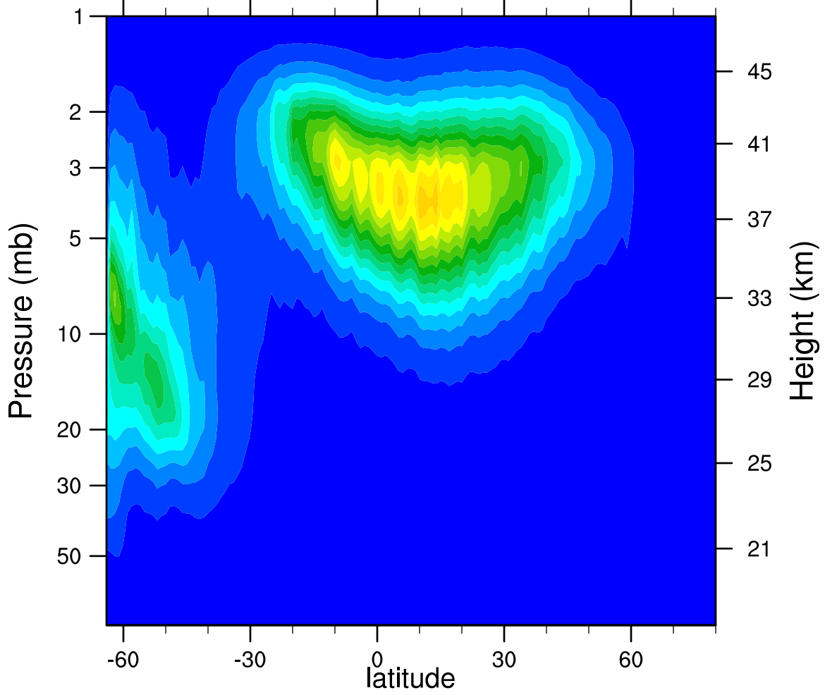
2005d117 N2O5_Ascending (ppbv)
