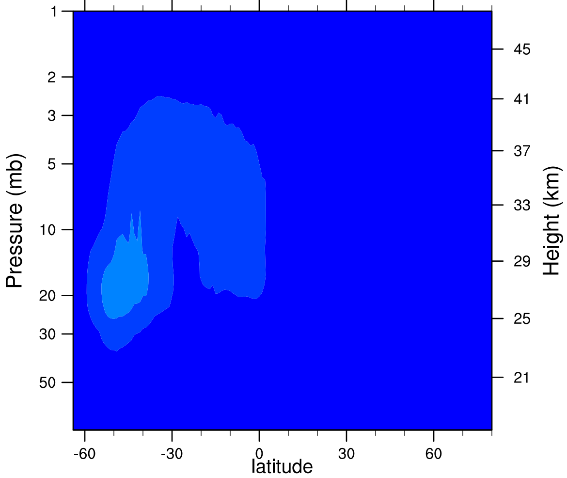
2006d239 N2O5_Ascending (ppbv)
