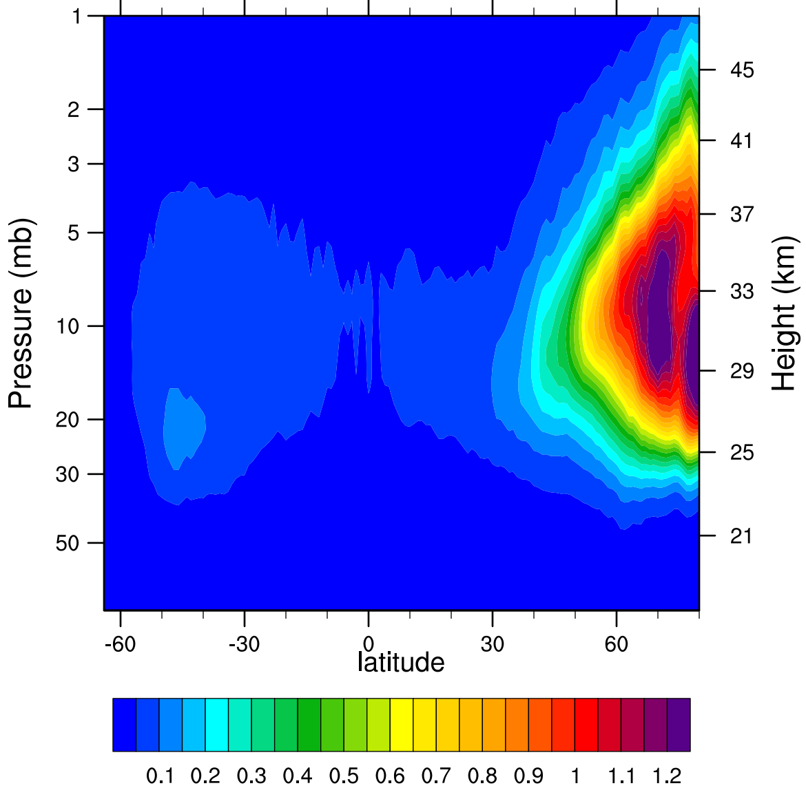
2006d347 N2O5_Ascending (ppbv)
