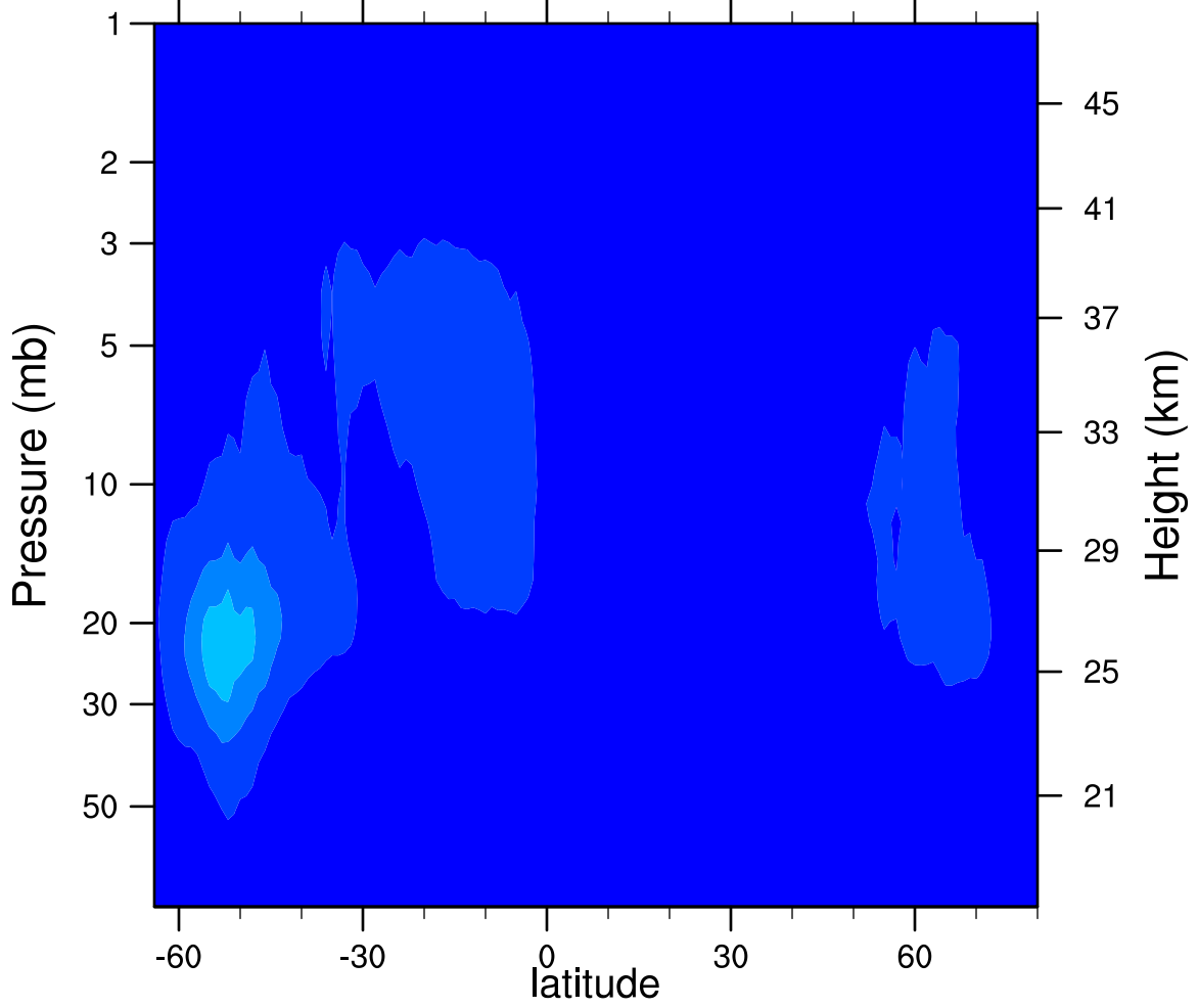
2006d259 N2O5_Ascending (ppbv)
