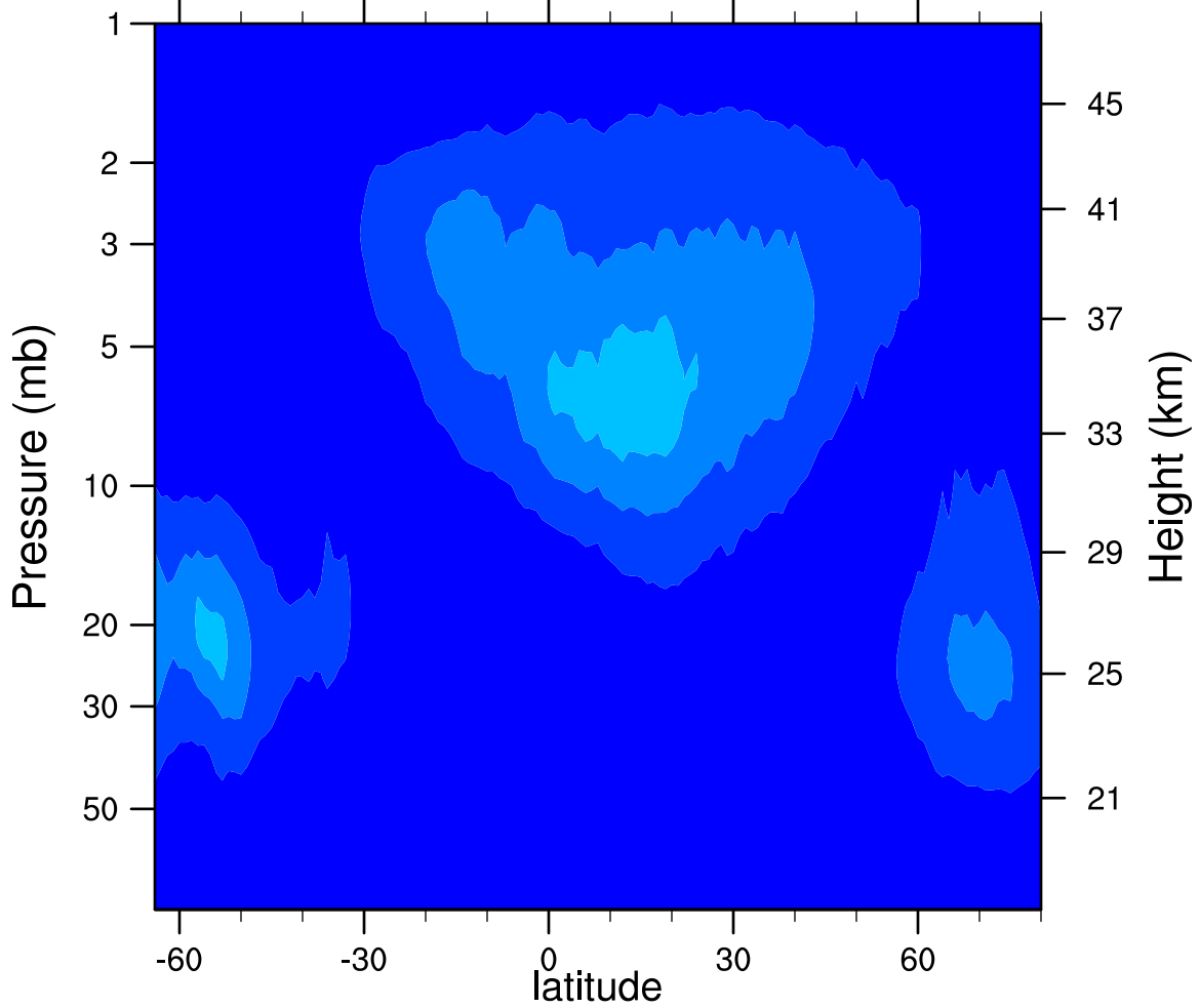
2005d261 N2O5_Ascending (ppbv)
