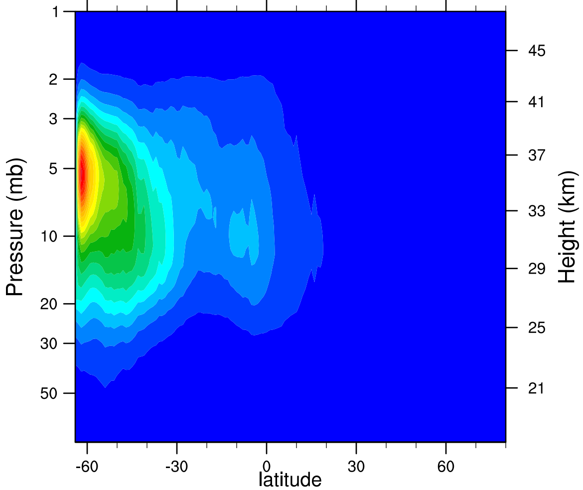
2006d161 N2O5_Ascending (ppbv)
