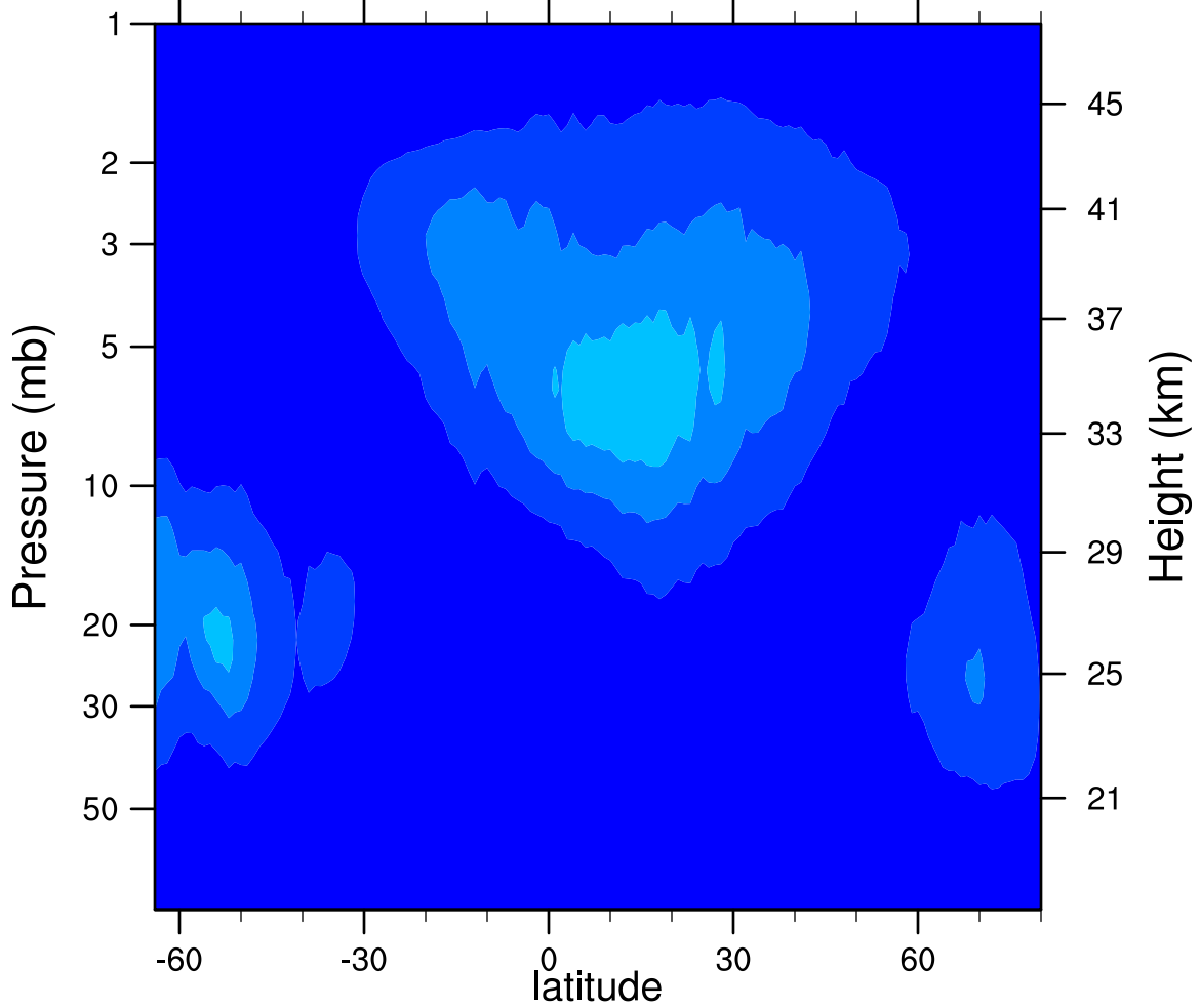
2005d257 N2O5_Ascending (ppbv)
