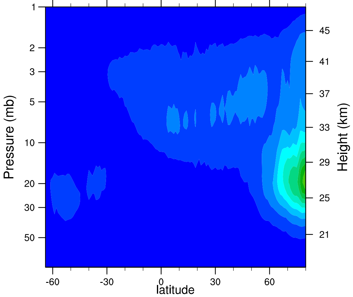
2005d287 N2O5_Ascending (ppbv)
