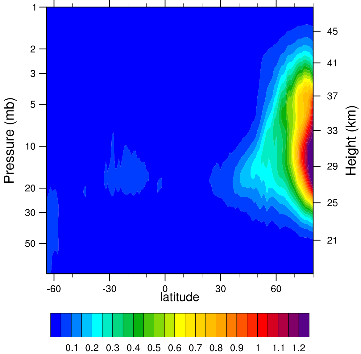
2006d302 N2O5_Ascending (ppbv)
