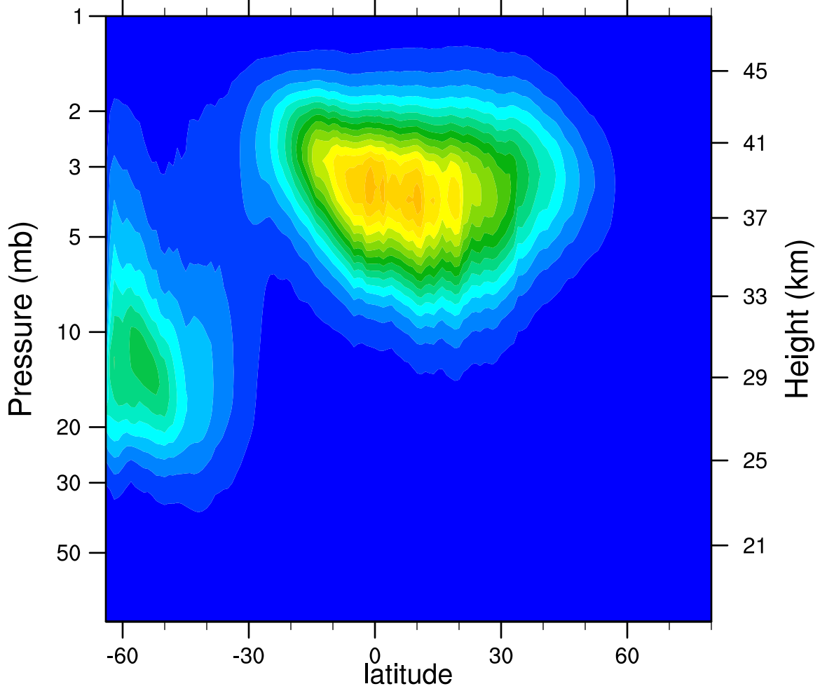
2005d140 N2O5_Ascending (ppbv)
