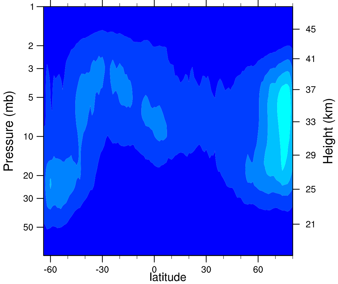
2006d075 N2O5_Ascending (ppbv)
