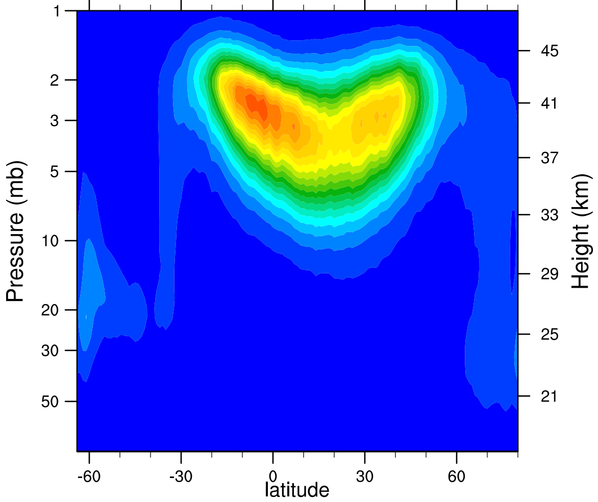
2005d076 N2O5_Ascending (ppbv)
