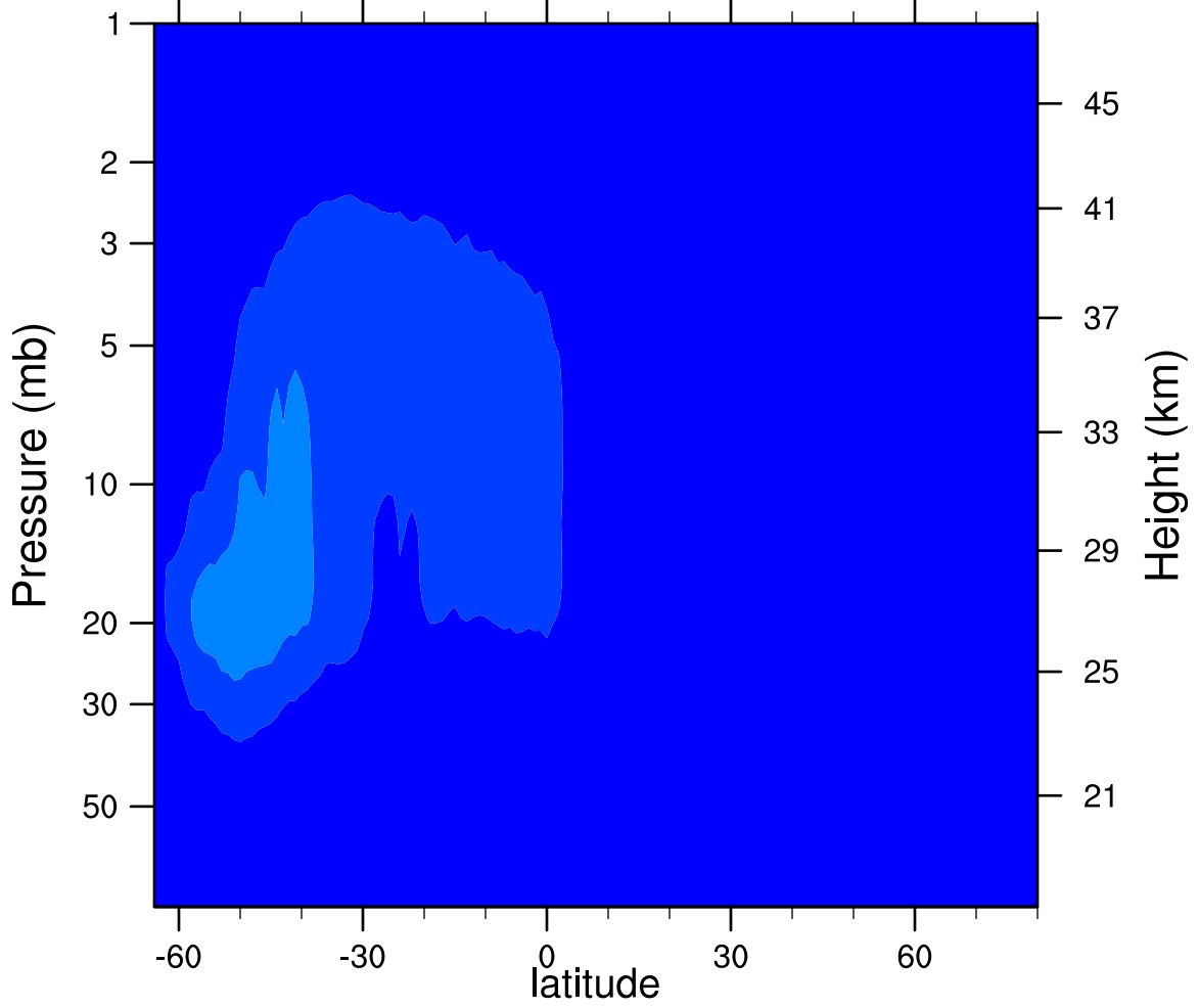
2006d236 N2O5_Ascending (ppbv)
