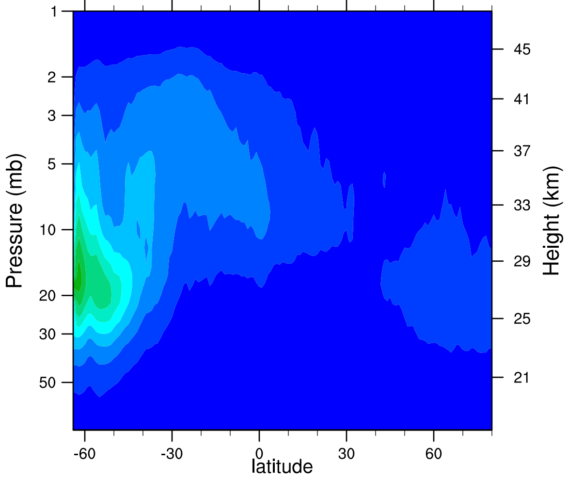
2006d101 N2O5_Ascending (ppbv)
