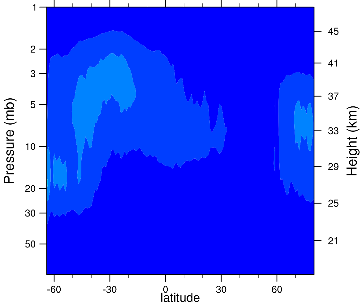
2006d088 N2O5_Ascending (ppbv)
