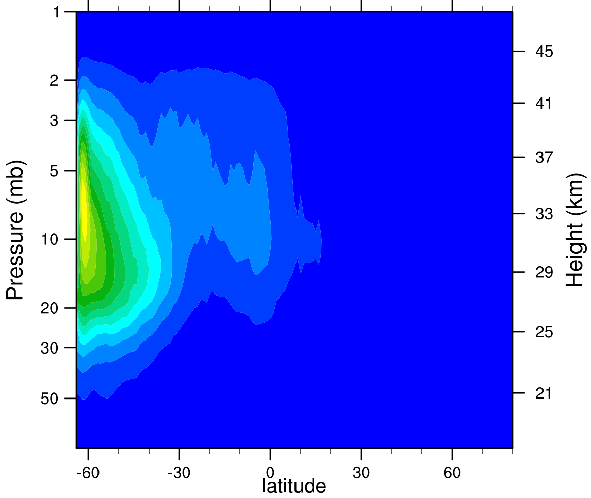
2006d132 N2O5_Ascending (ppbv)
