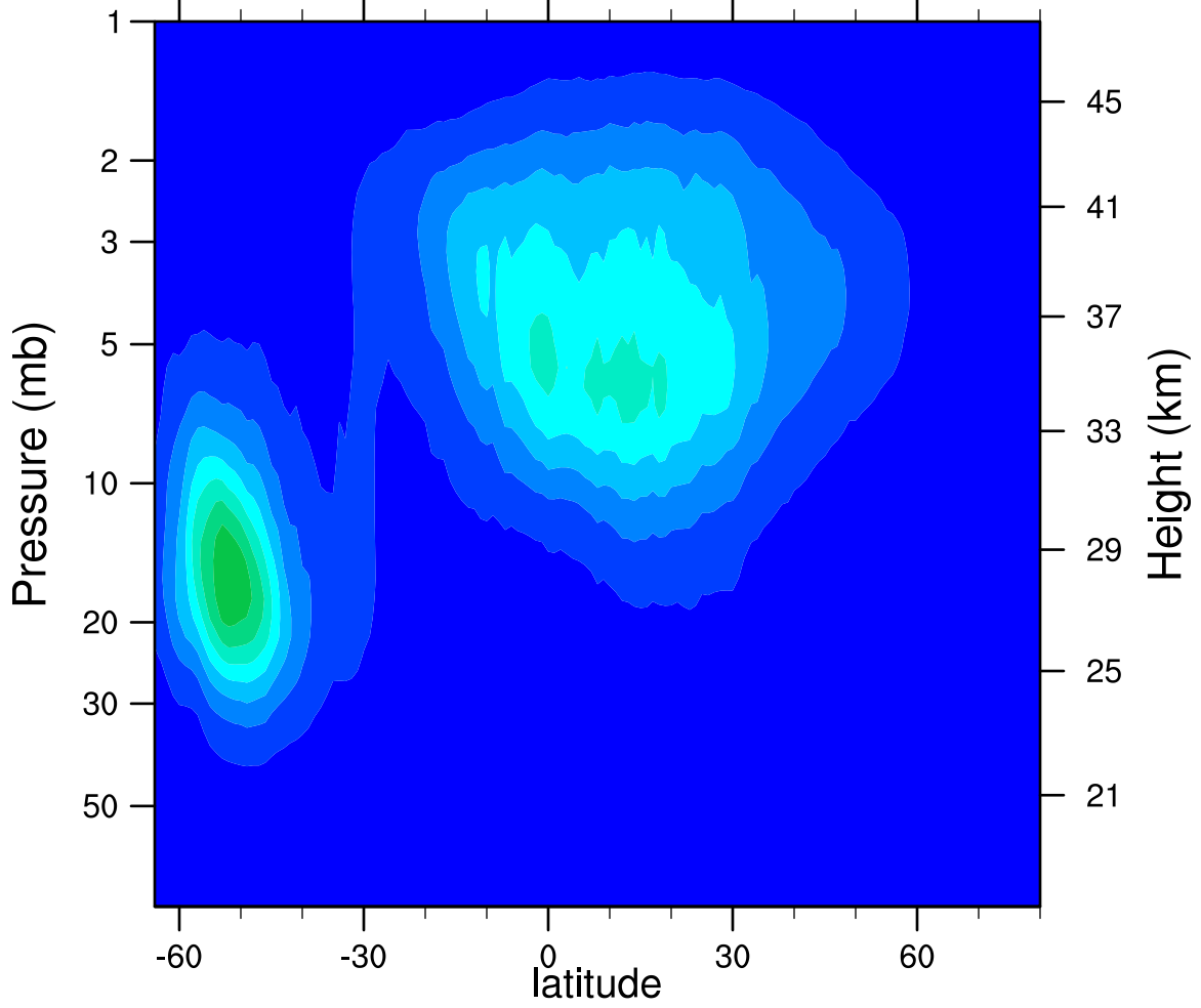
2005d221 N2O5_Ascending (ppbv)
