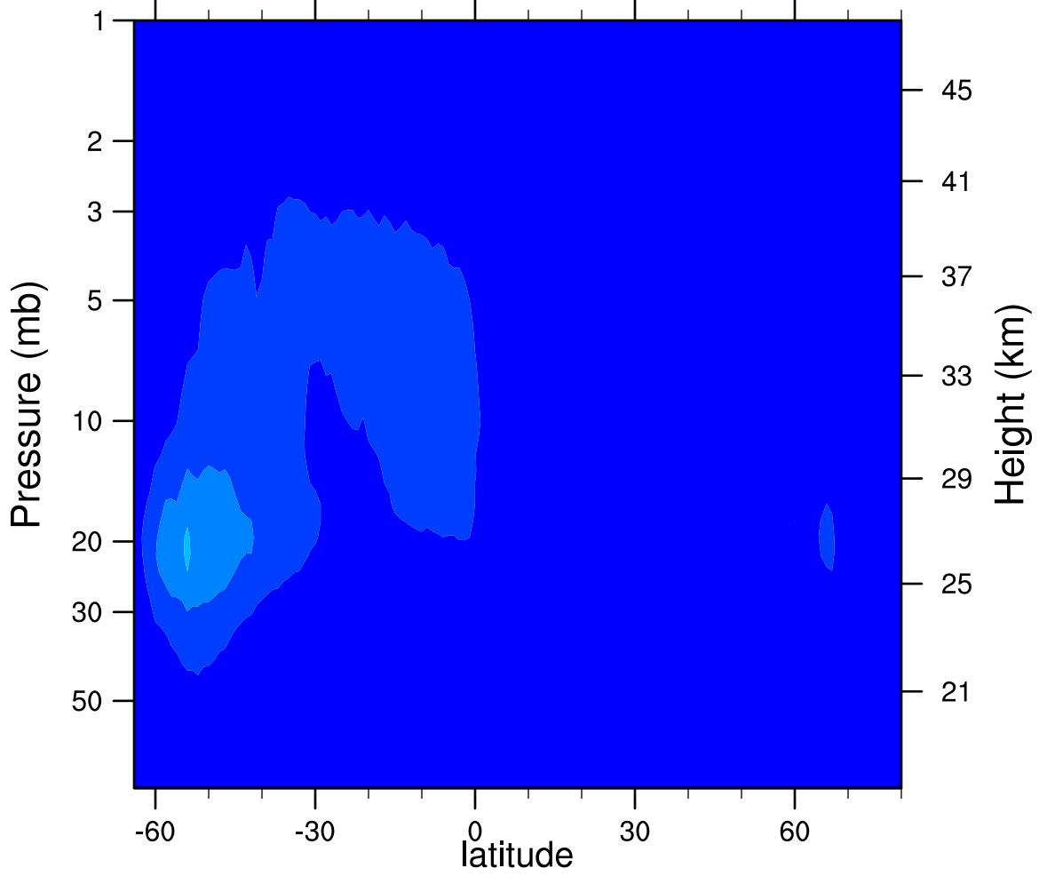
2006d252 N2O5_Ascending (ppbv)
