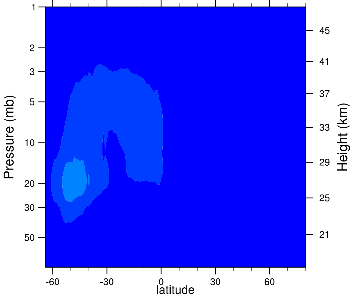
2006d248 N2O5_Ascending (ppbv)
