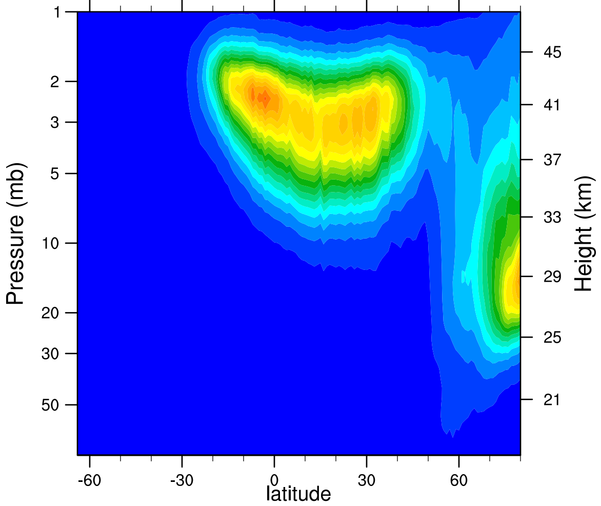
2005d029 N2O5_Ascending (ppbv)
