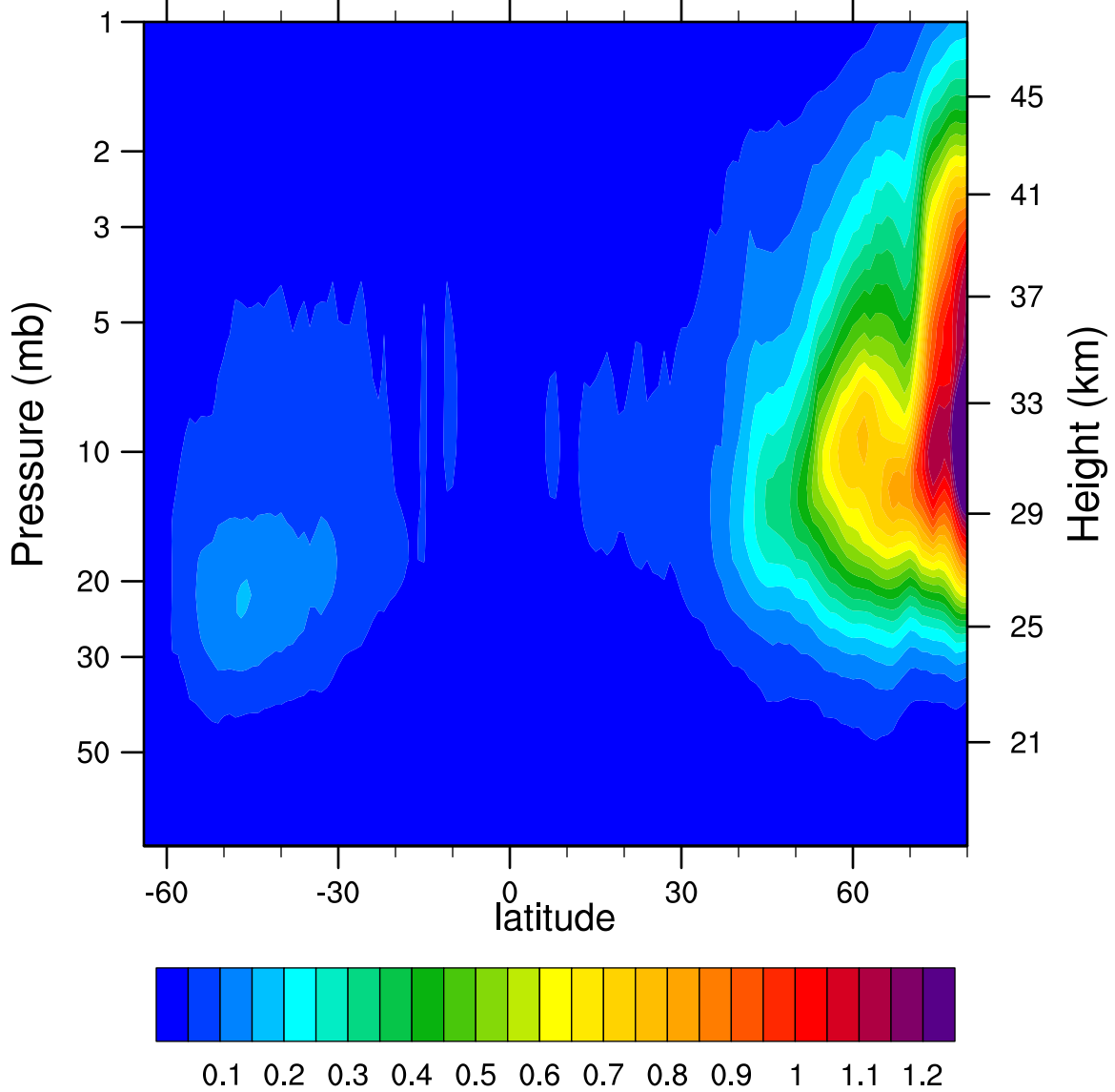
2006d337 N2O5_Ascending (ppbv)
