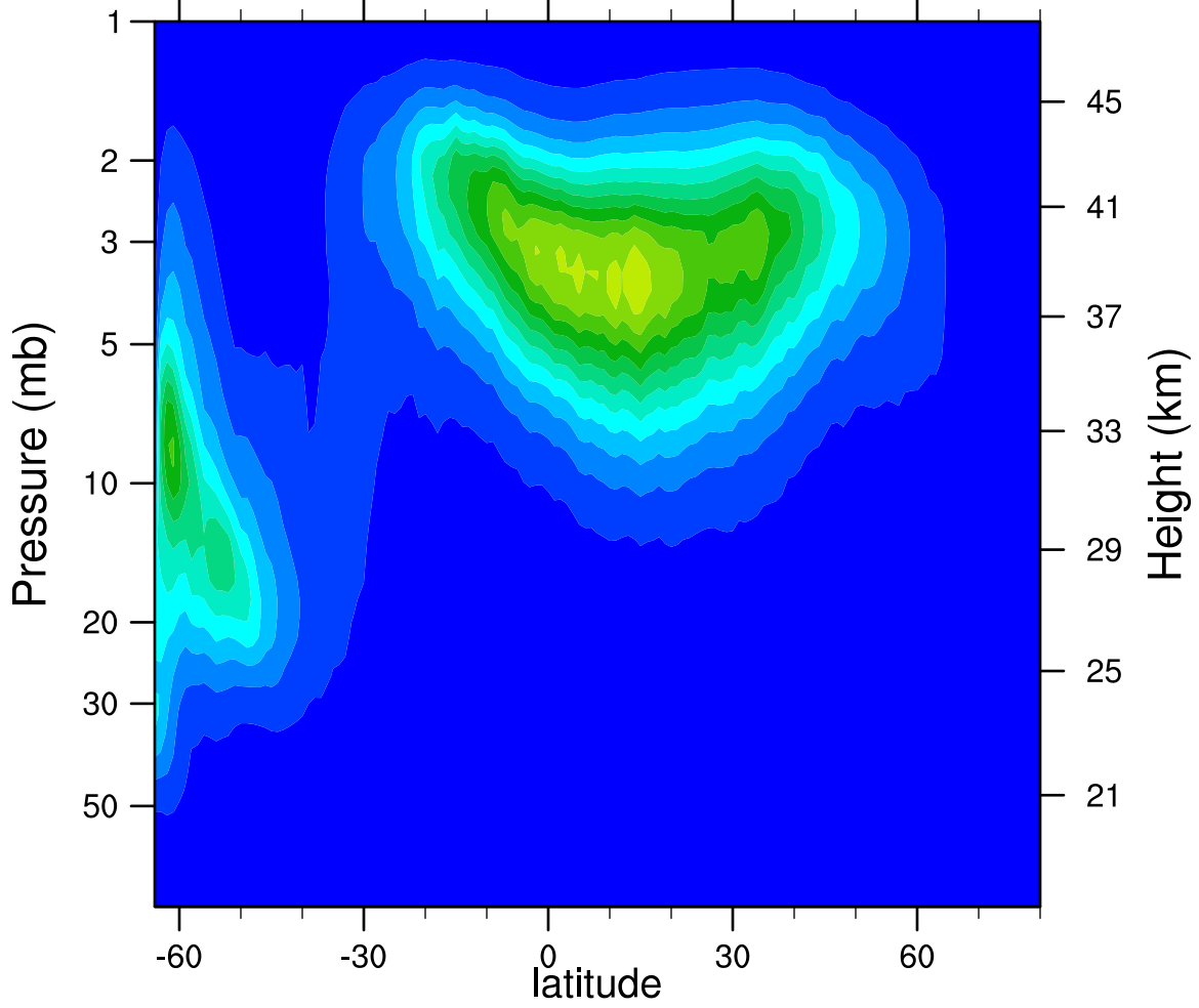
2005d109 N2O5_Ascending (ppbv)
