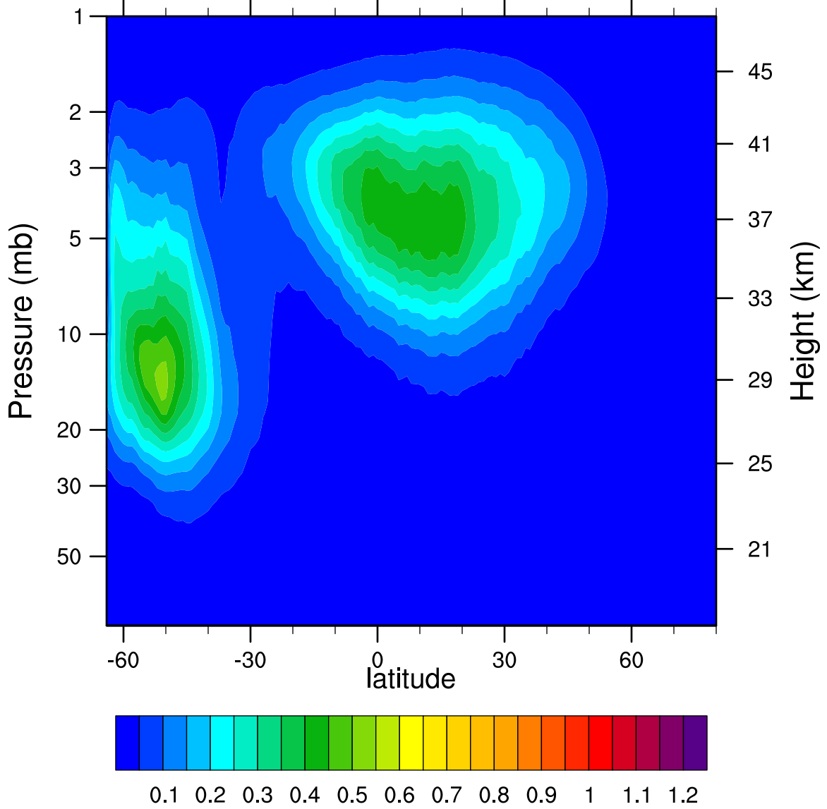
2005d164 N2O5_Ascending (ppbv)
