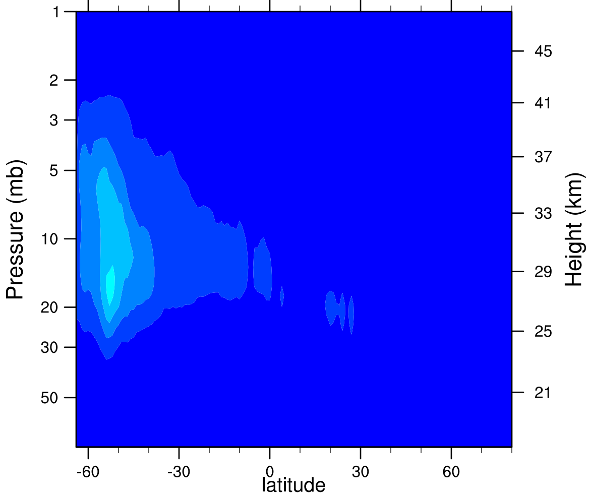
2007d191 N2O5_Ascending (ppbv)
