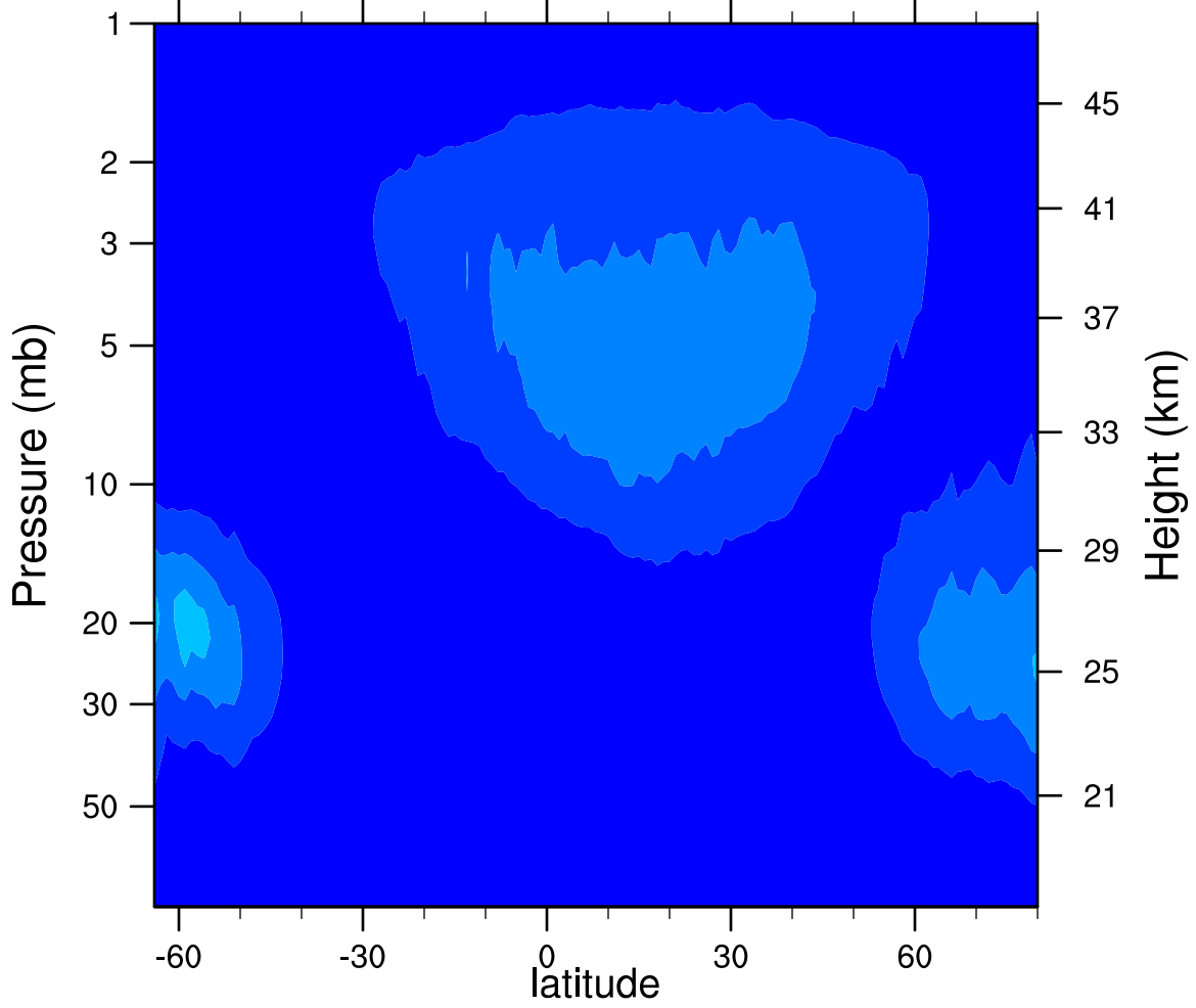
2005d271 N2O5_Ascending (ppbv)
