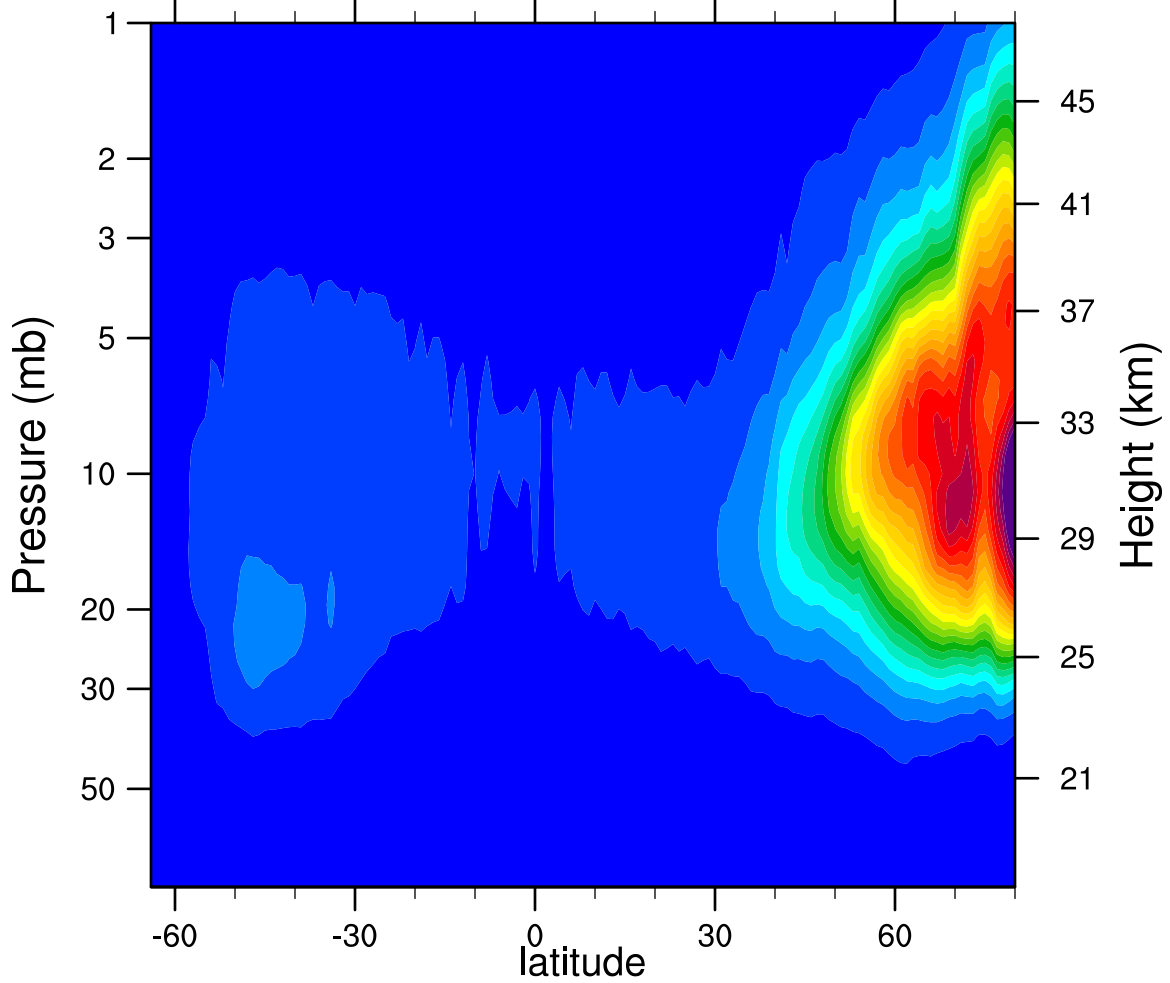
2006d345 N2O5_Ascending (ppbv)
