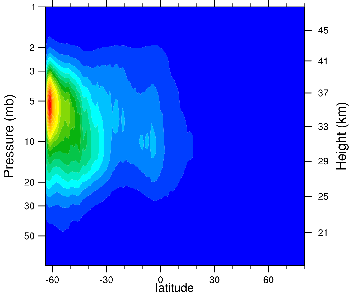
2006d159 N2O5_Ascending (ppbv)
