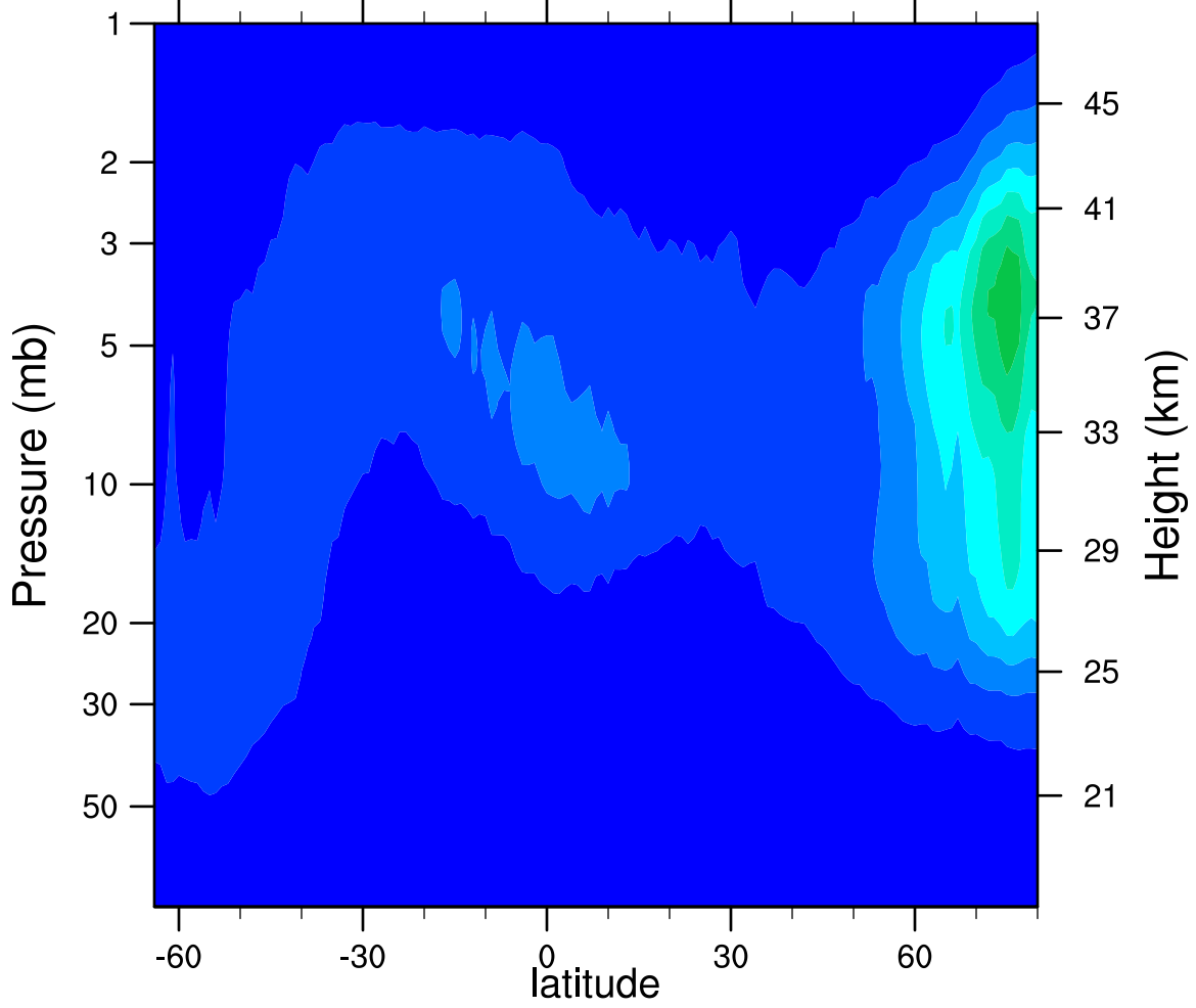
2006d065 N2O5_Ascending (ppbv)
