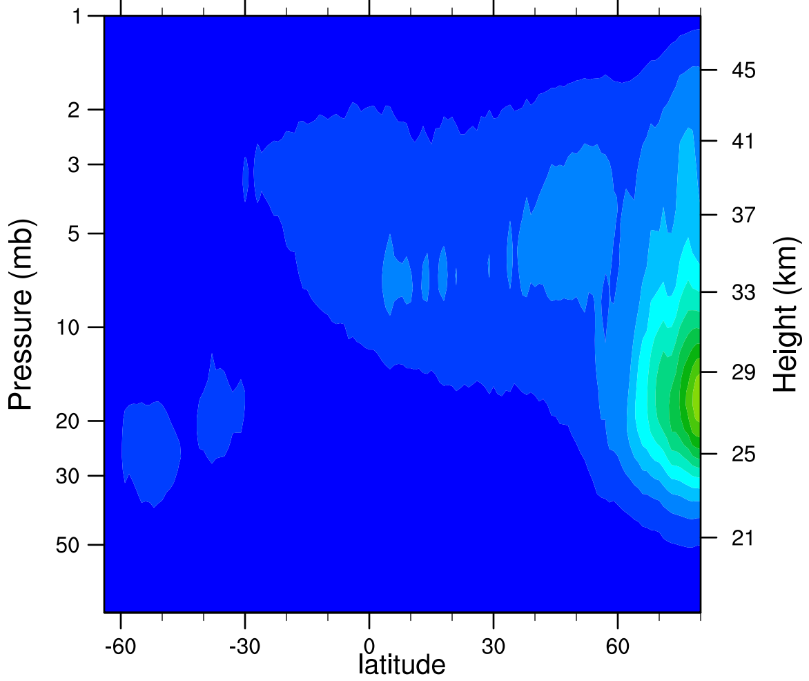
2005d289 N2O5_Ascending (ppbv)
