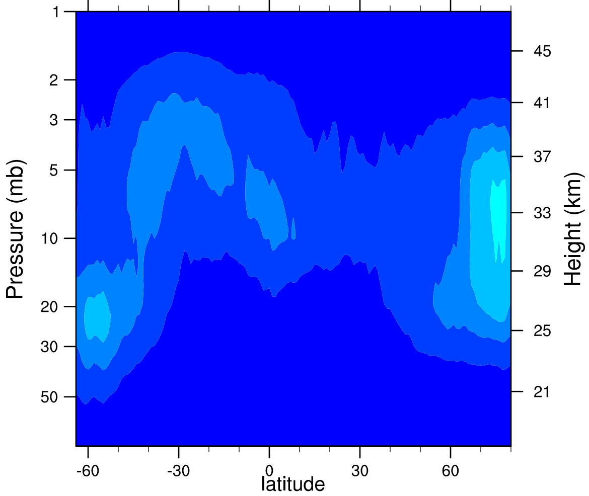
2006d079 N2O5_Ascending (ppbv)
