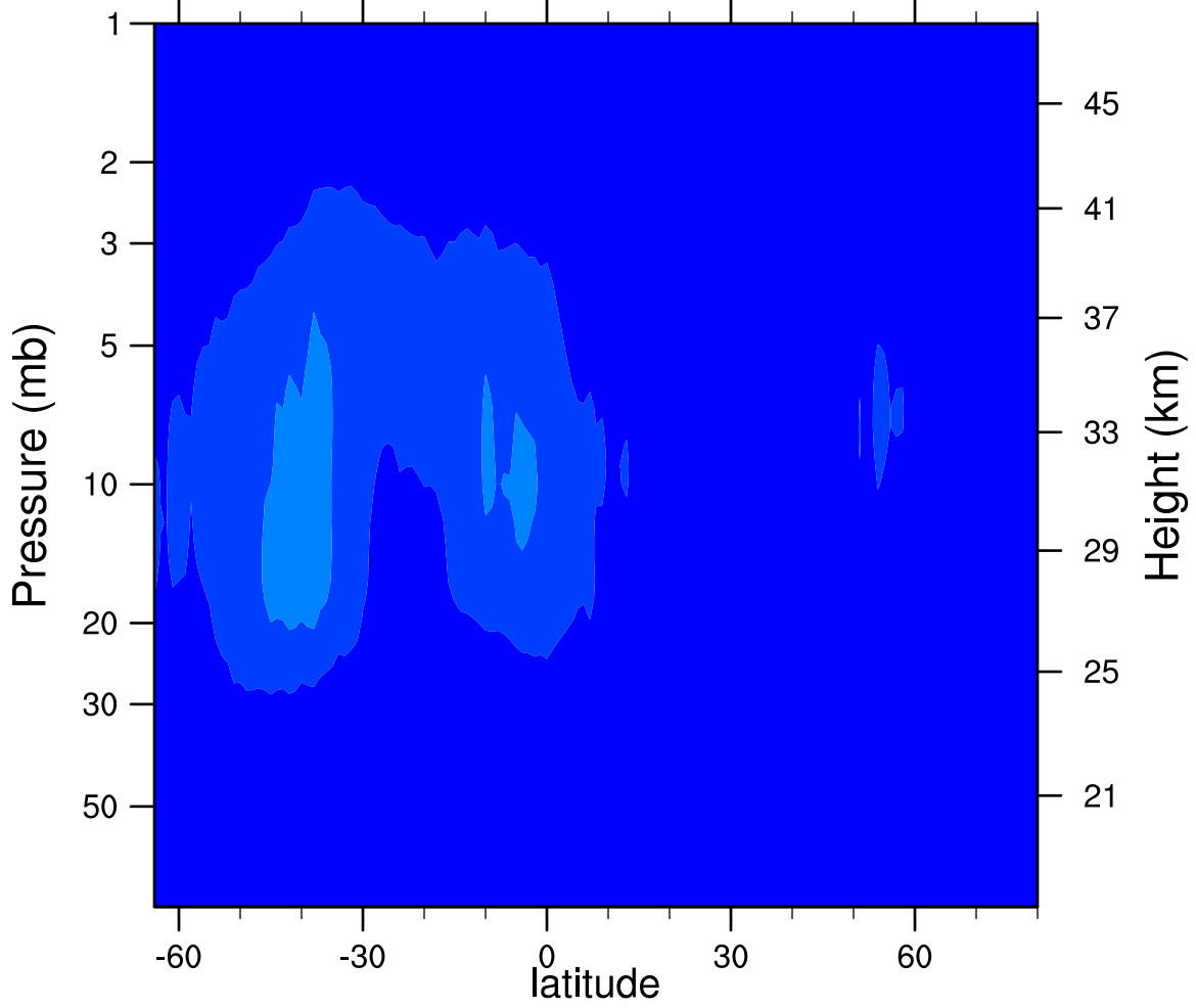
2006d222 N2O5_Ascending (ppbv)
