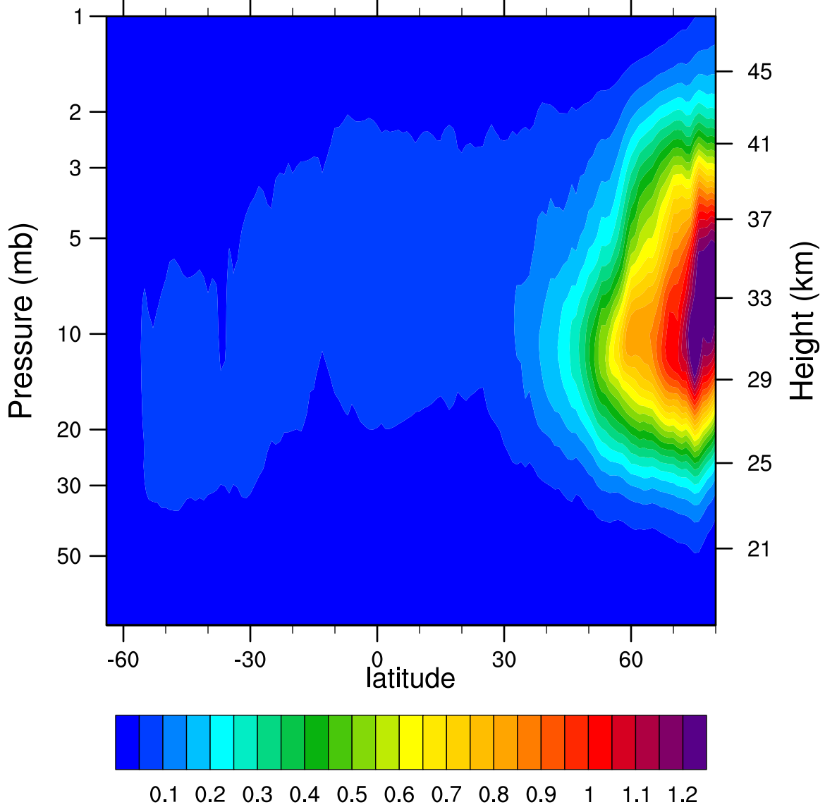
2007d352 N2O5_Ascending (ppbv)
