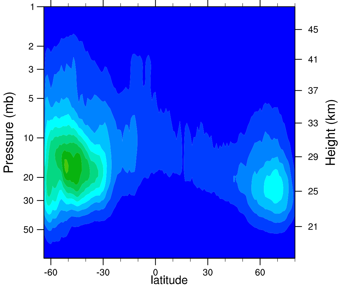
2007d251 N2O5_Ascending (ppbv)
