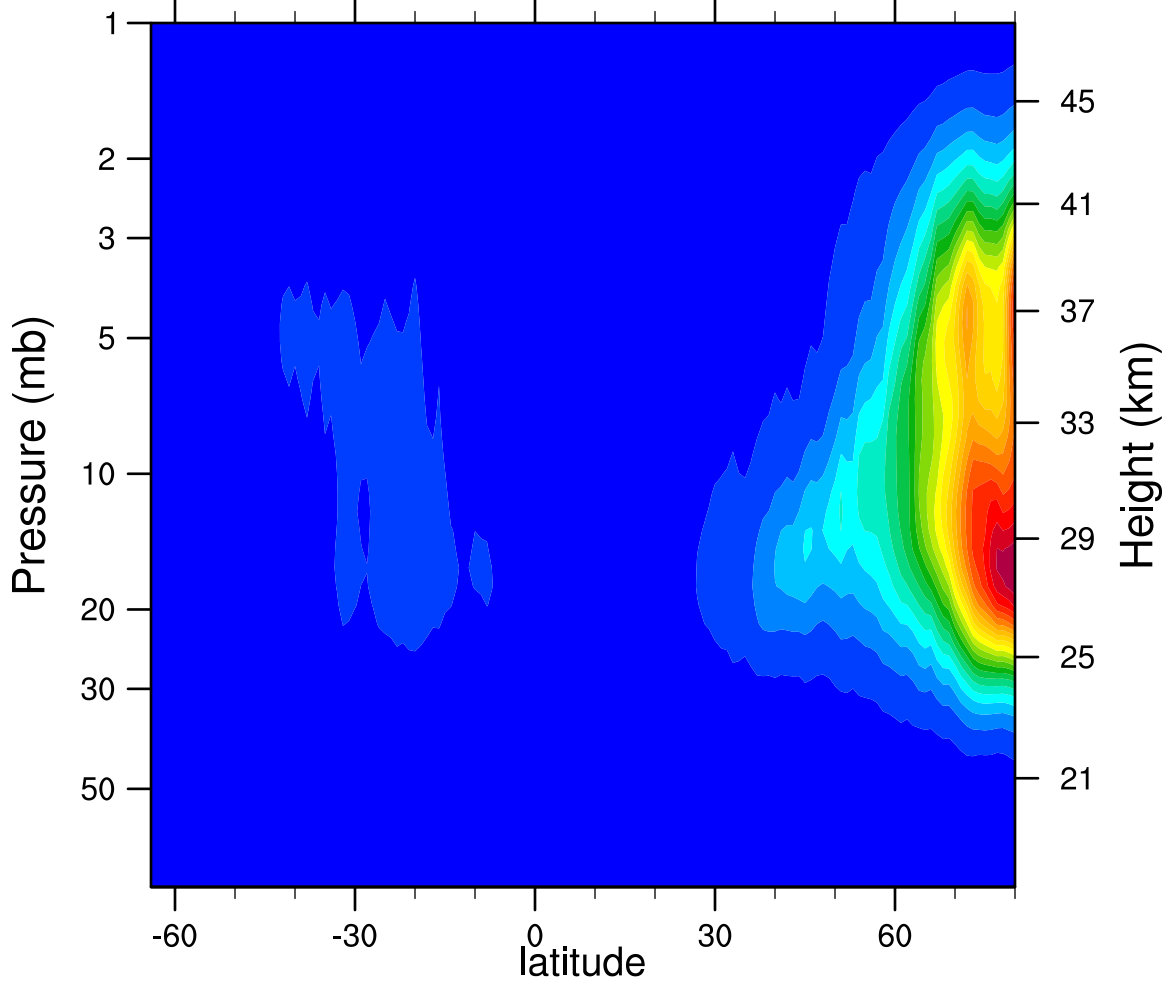
2006d308 N2O5_Ascending (ppbv)
