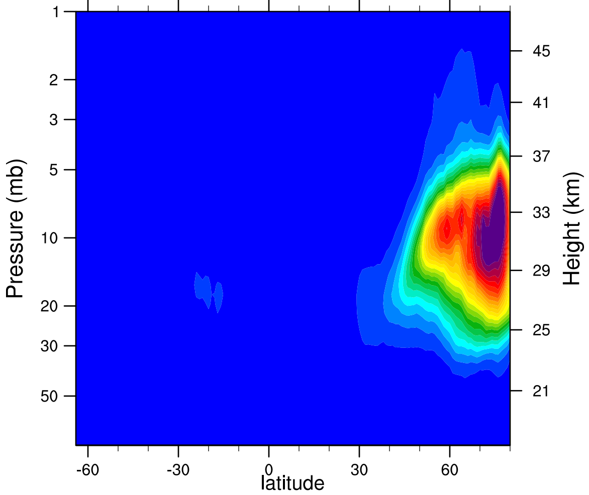
2006d365 N2O5_Ascending (ppbv)
