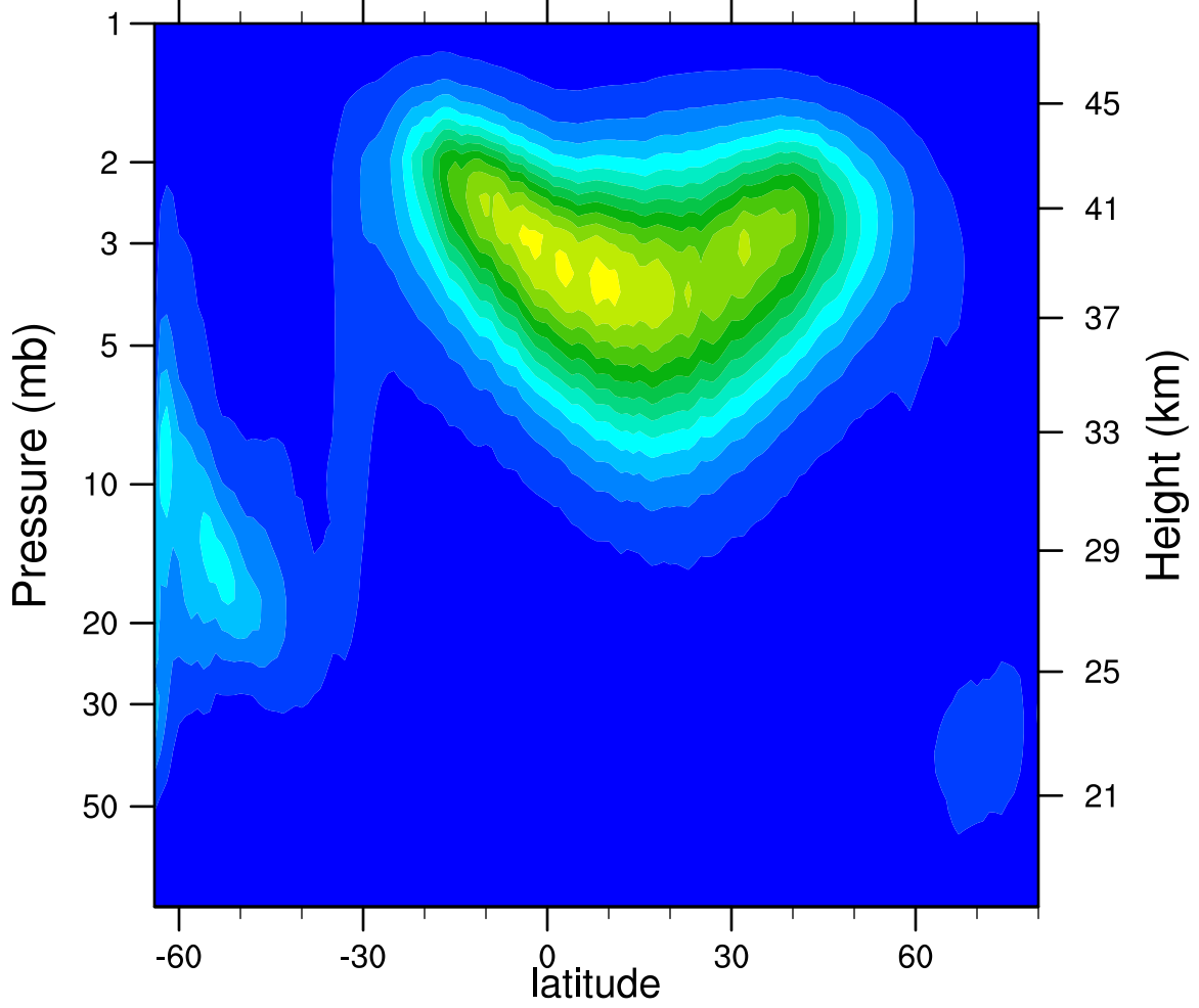
2005d097 N2O5_Ascending (ppbv)
