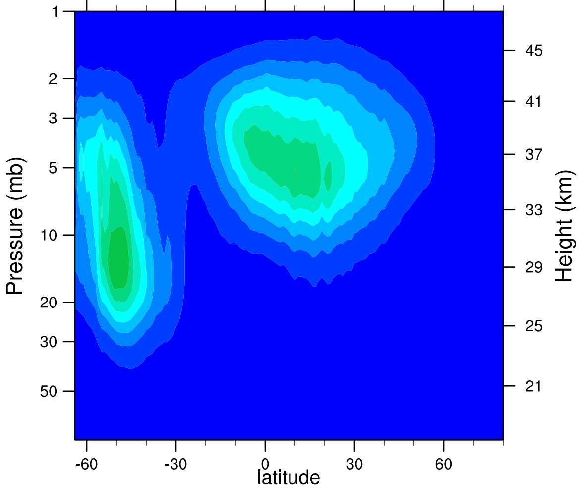
2005d190 N2O5_Ascending (ppbv)
