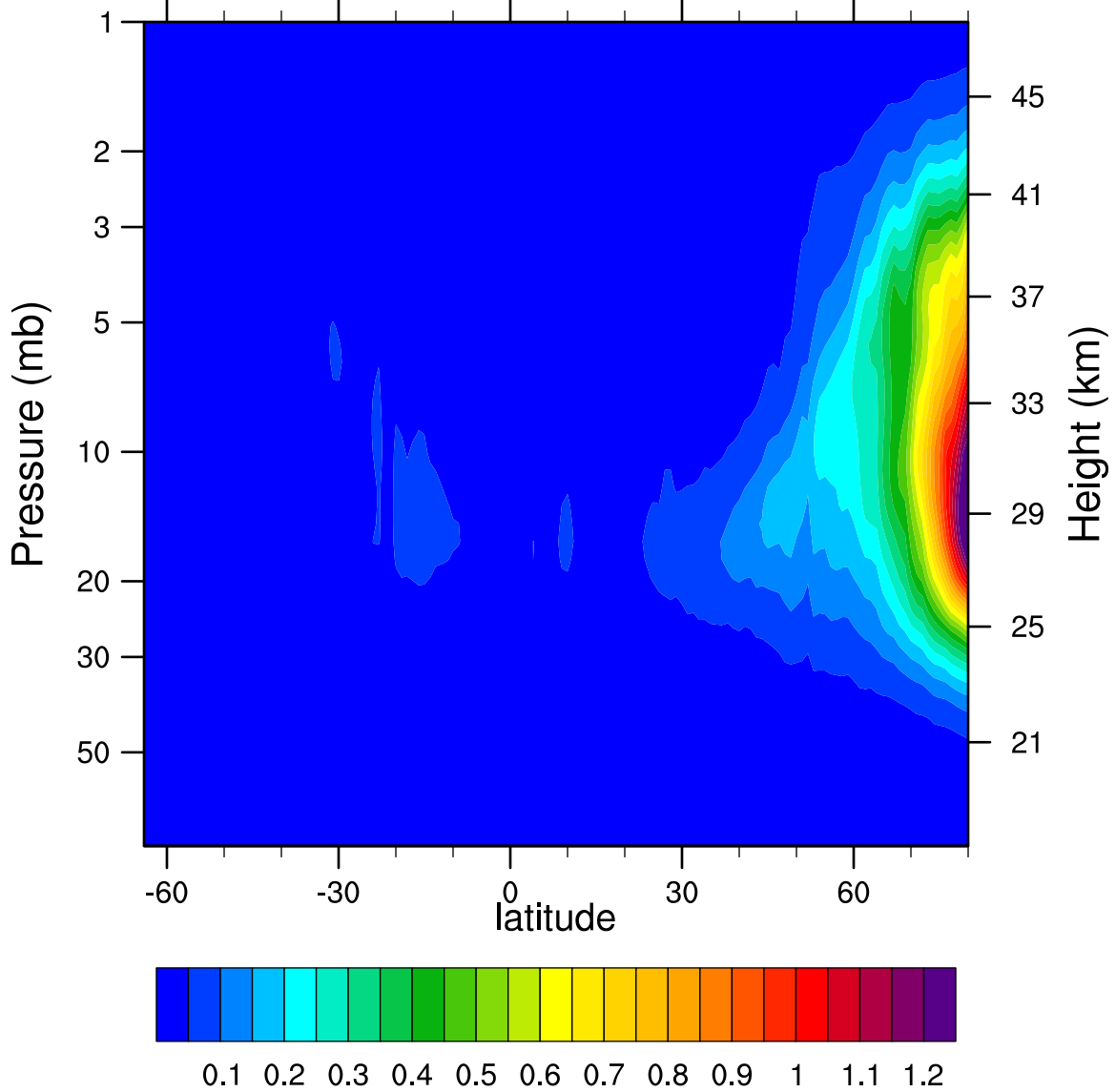
2006d299 N2O5_Ascending (ppbv)
