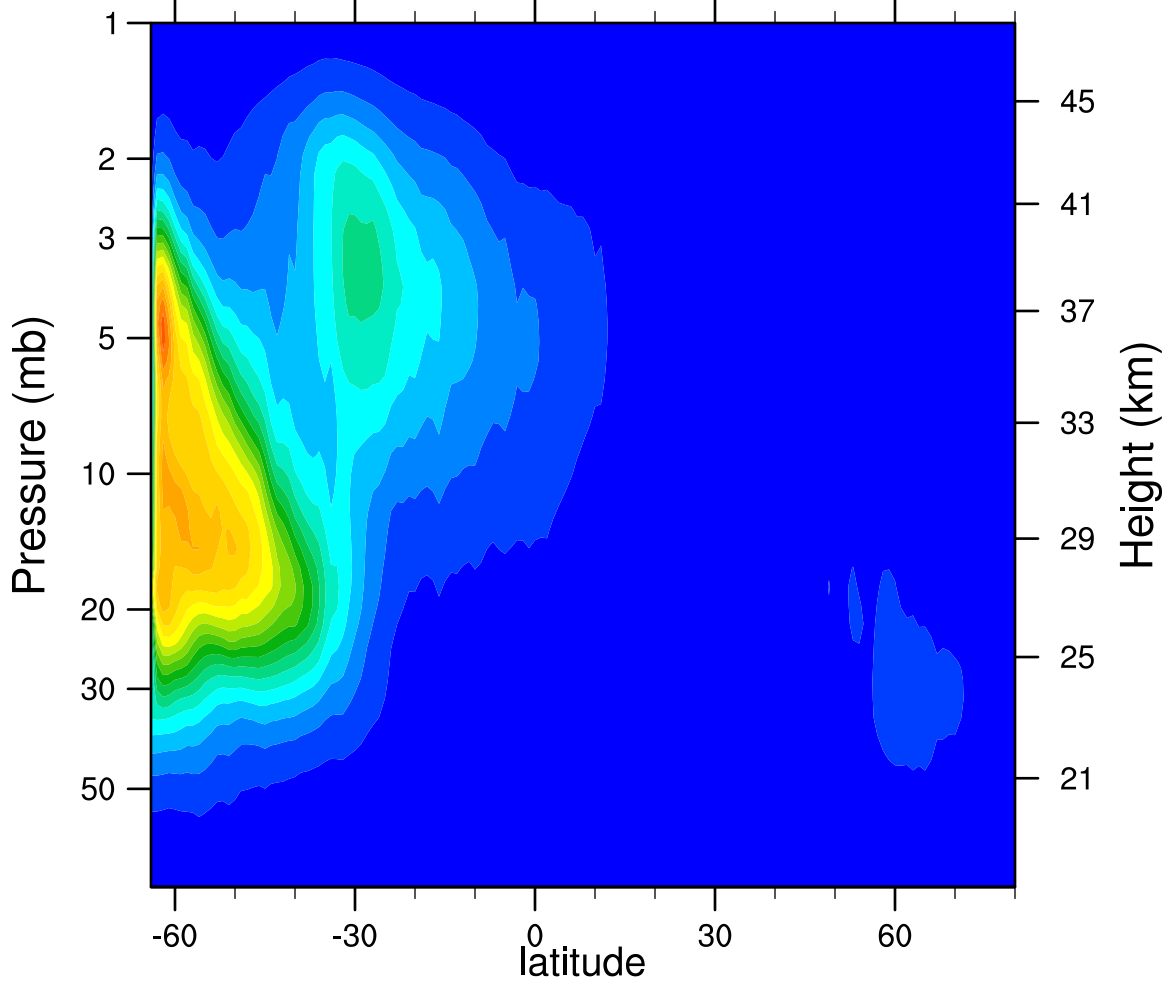
2007d116 N2O5_Ascending (ppbv)
