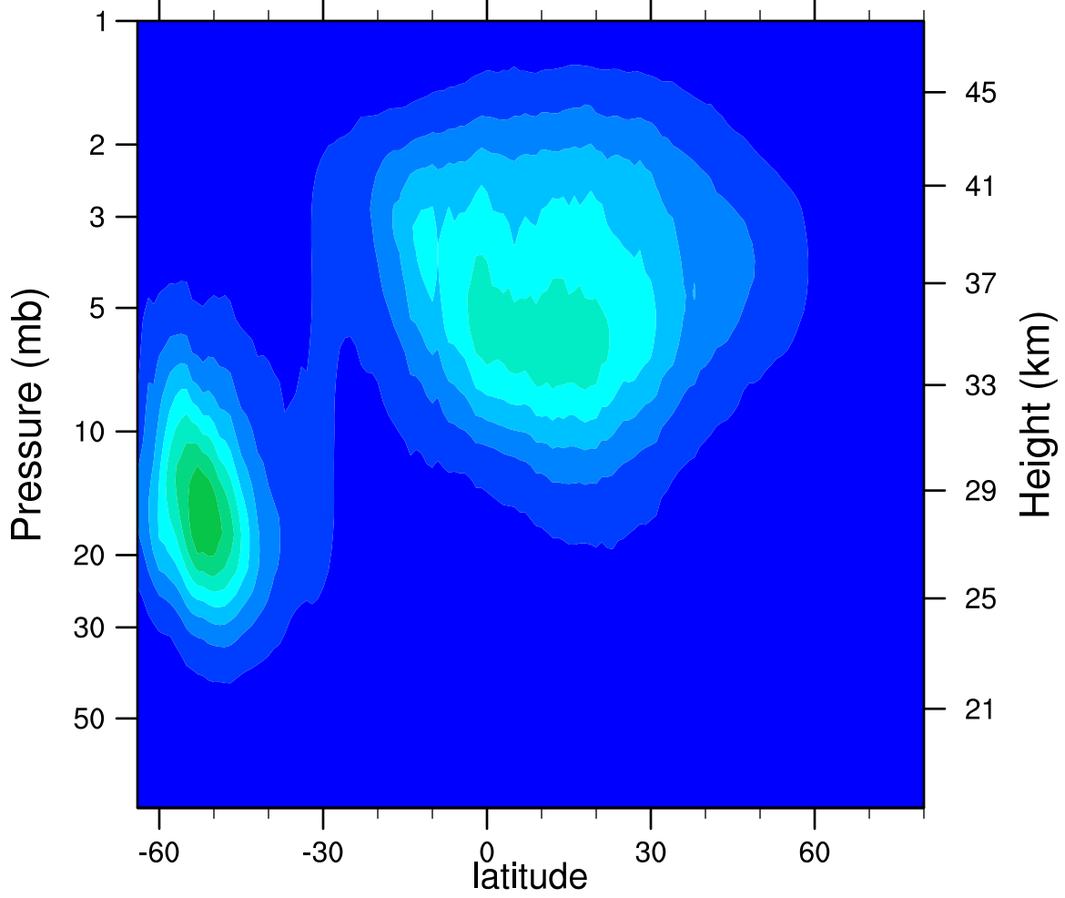
2005d219 N2O5_Ascending (ppbv)
