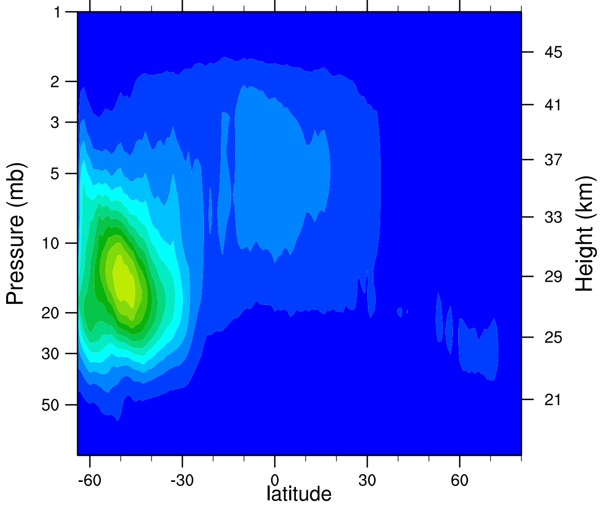
2007d232 N2O5_Ascending (ppbv)
