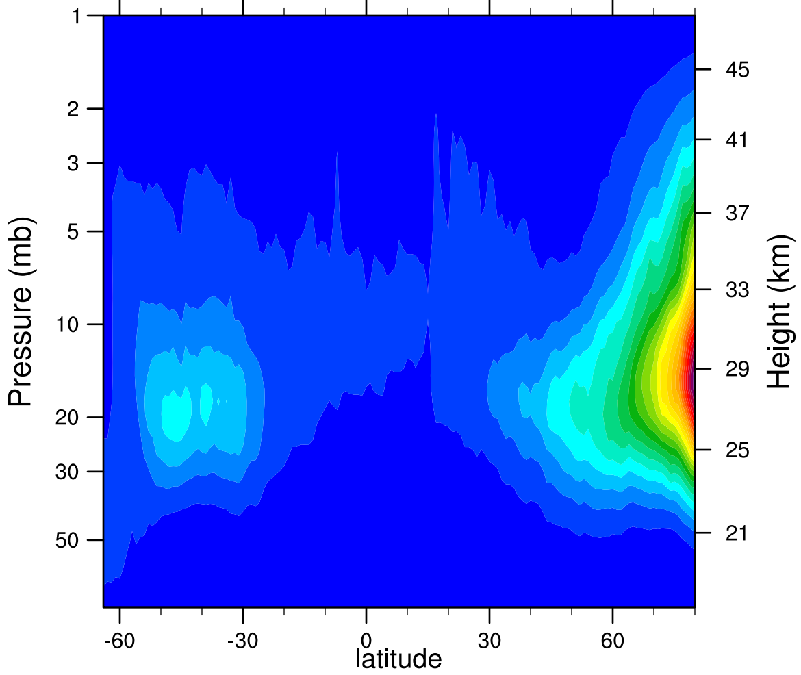
2007d289 N2O5_Ascending (ppbv)
