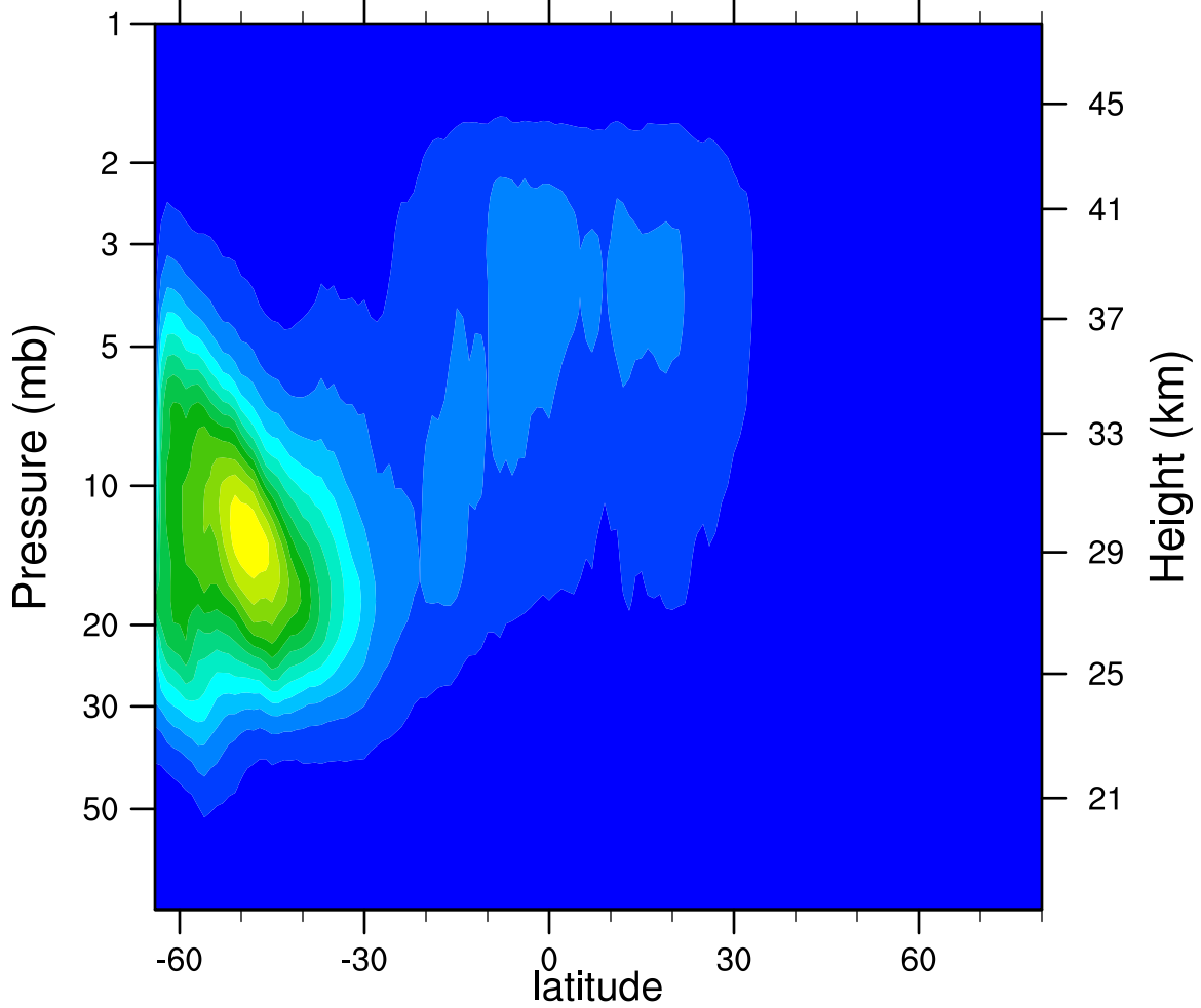
2007d218 N2O5_Ascending (ppbv)
