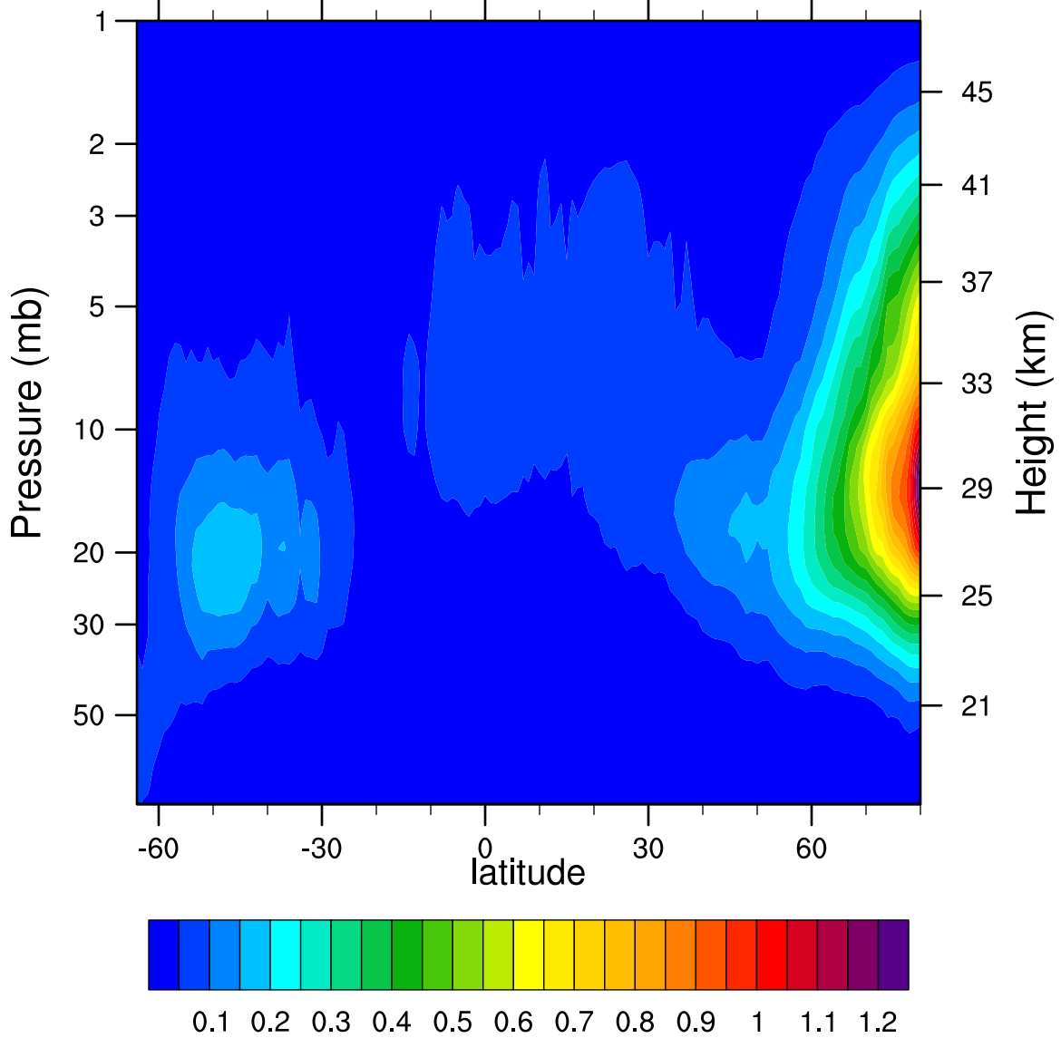
2007d296 N2O5_Ascending (ppbv)
