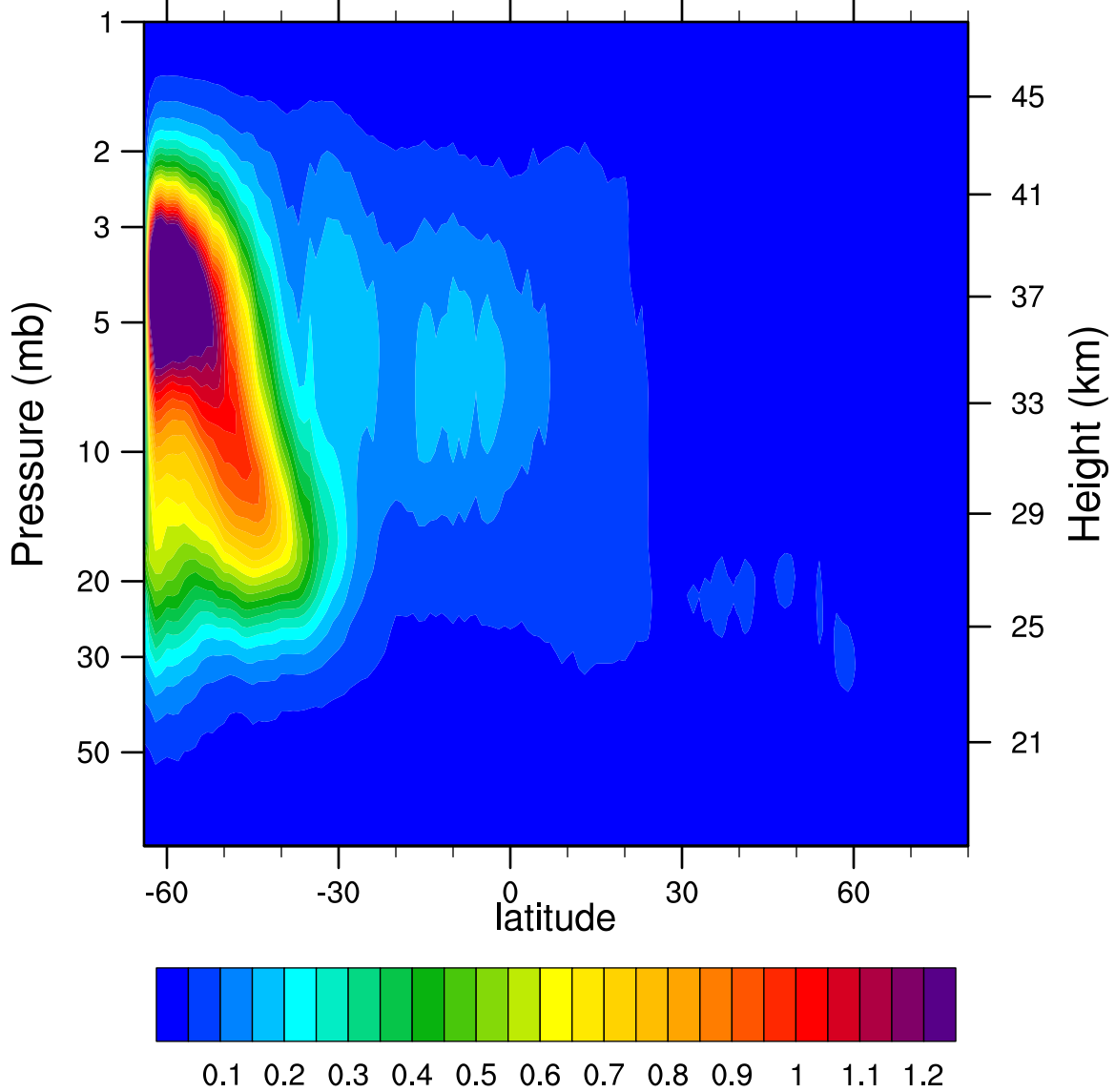
2007d141 N2O5_Ascending (ppbv)
