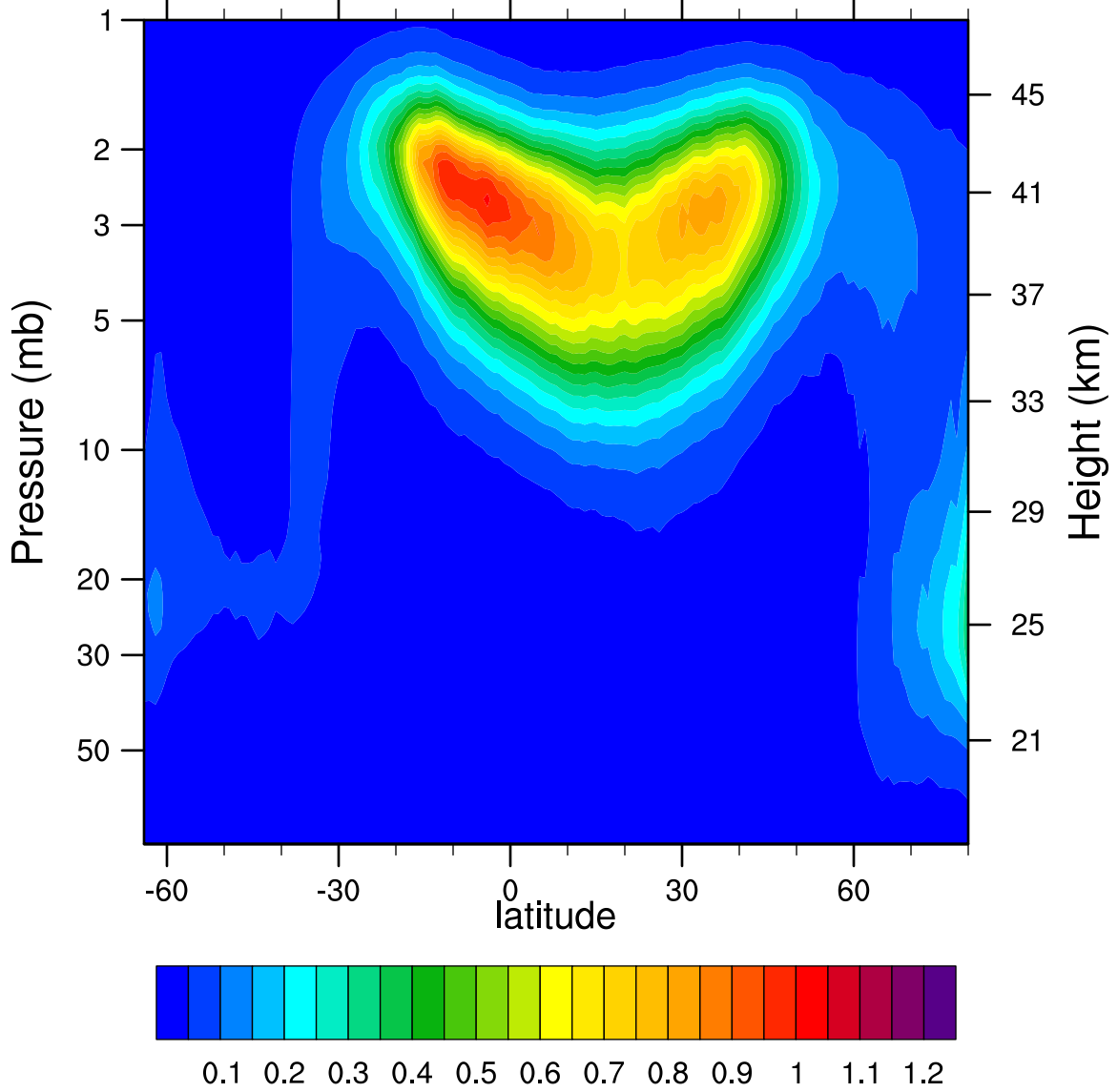
2005d070 N2O5_Ascending (ppbv)
