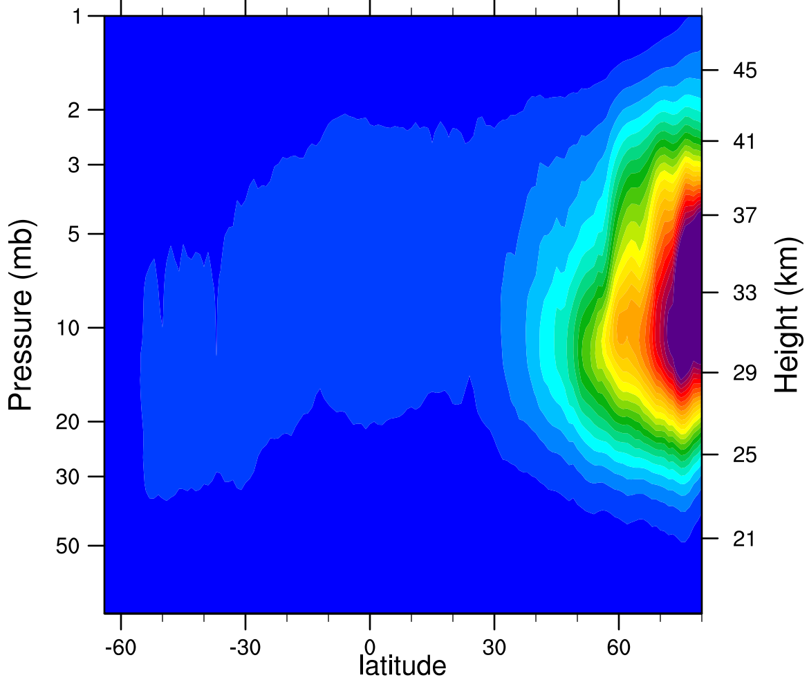
2007d349 N2O5_Ascending (ppbv)
