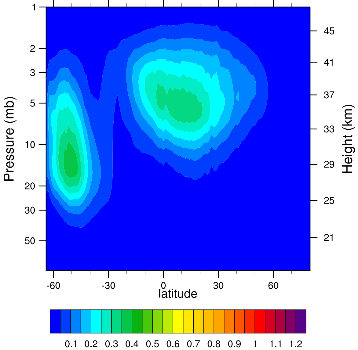
2005d197 N2O5_Ascending (ppbv)
