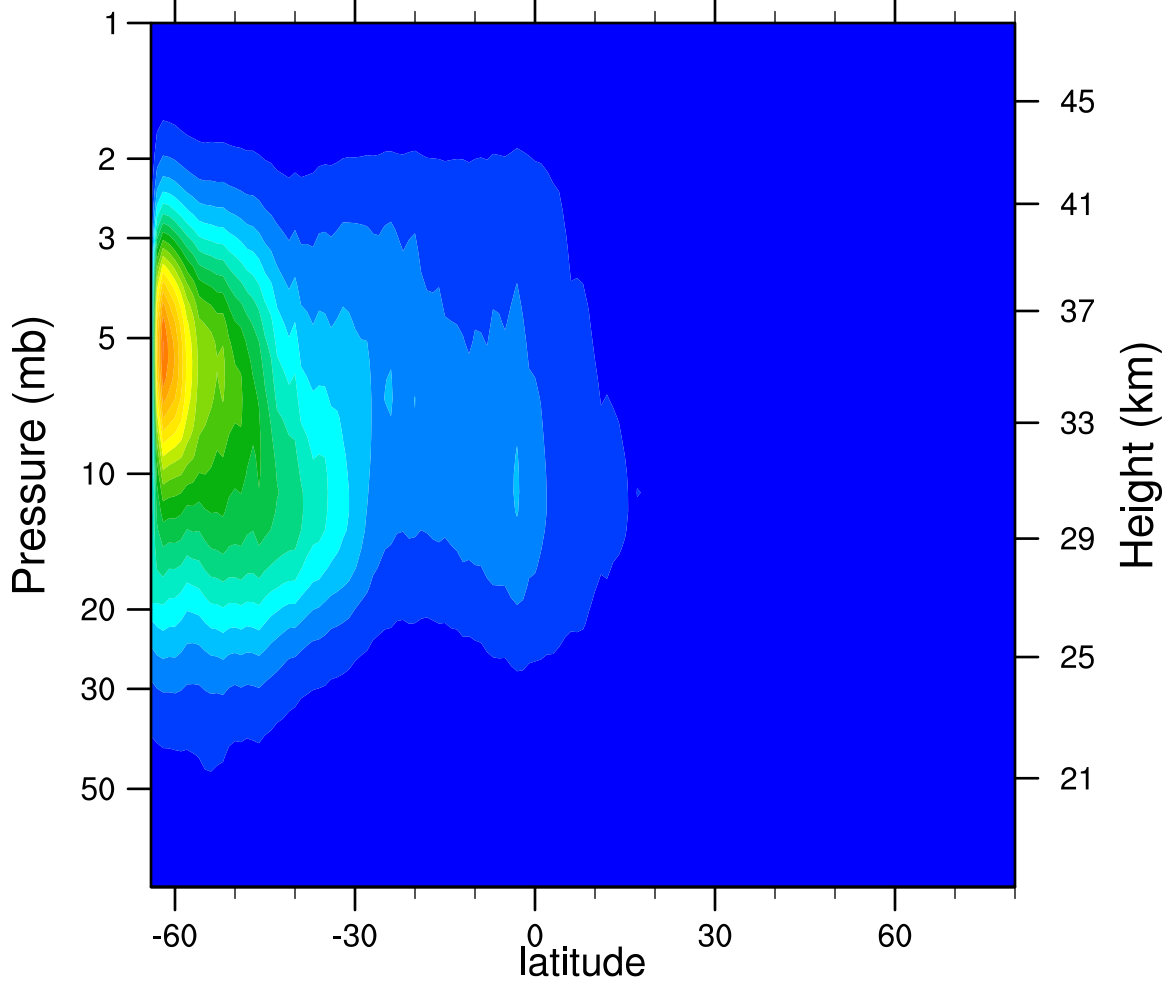
2006d157 N2O5_Ascending (ppbv)
