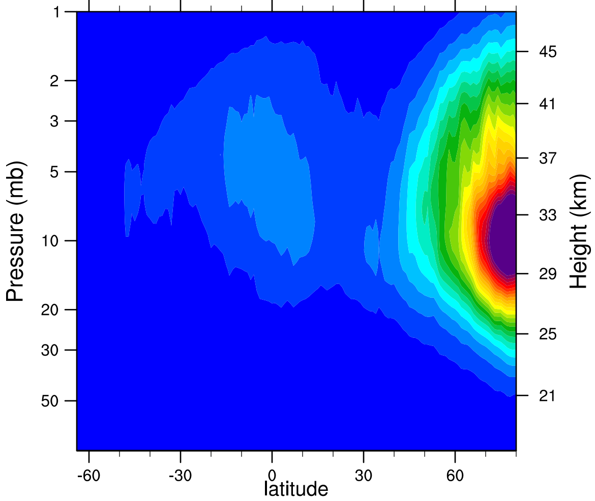
2006d012 N2O5_Ascending (ppbv)
