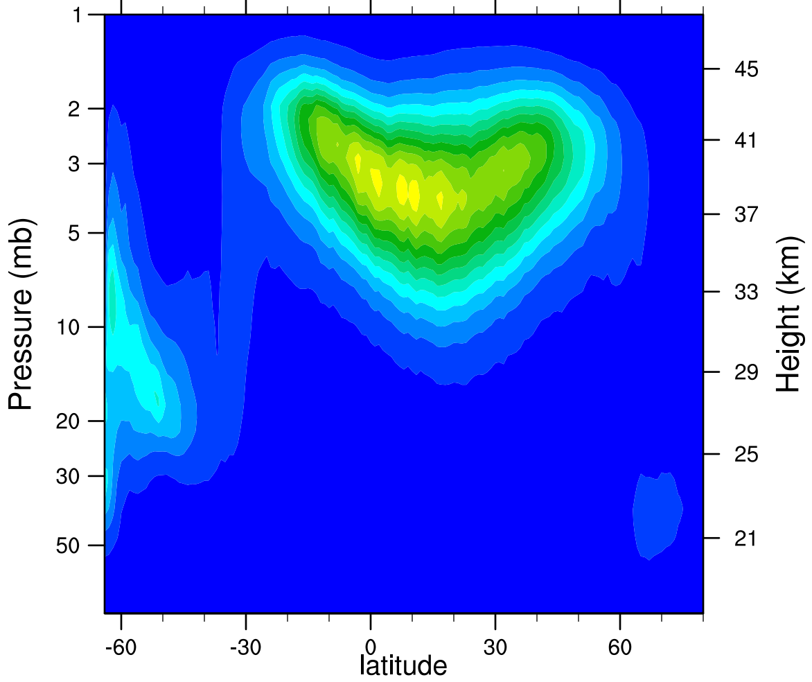
2005d100 N2O5_Ascending (ppbv)
