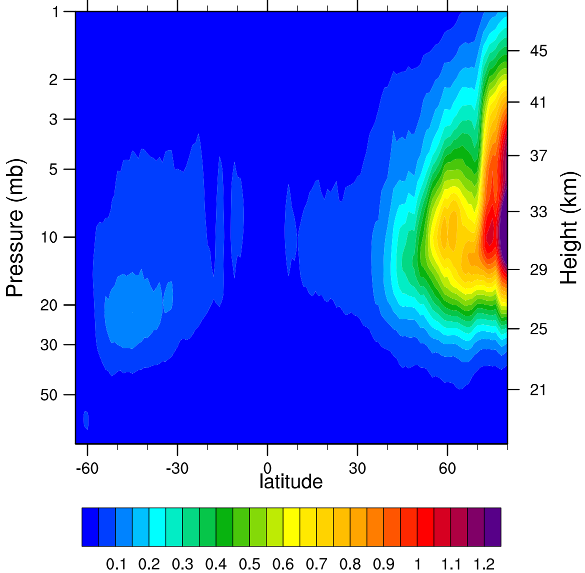
2006d339 N2O5_Ascending (ppbv)
