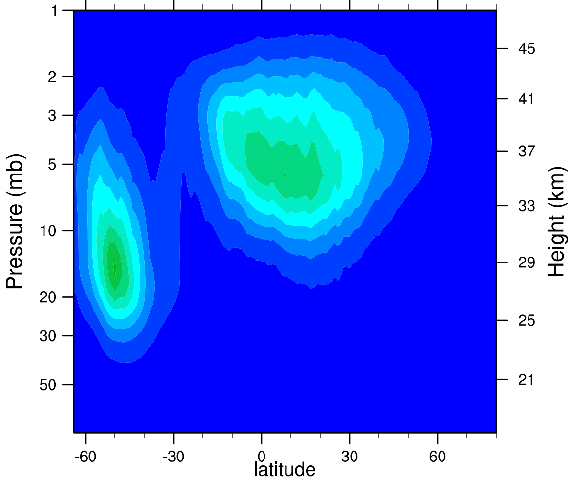
2005d205 N2O5_Ascending (ppbv)
