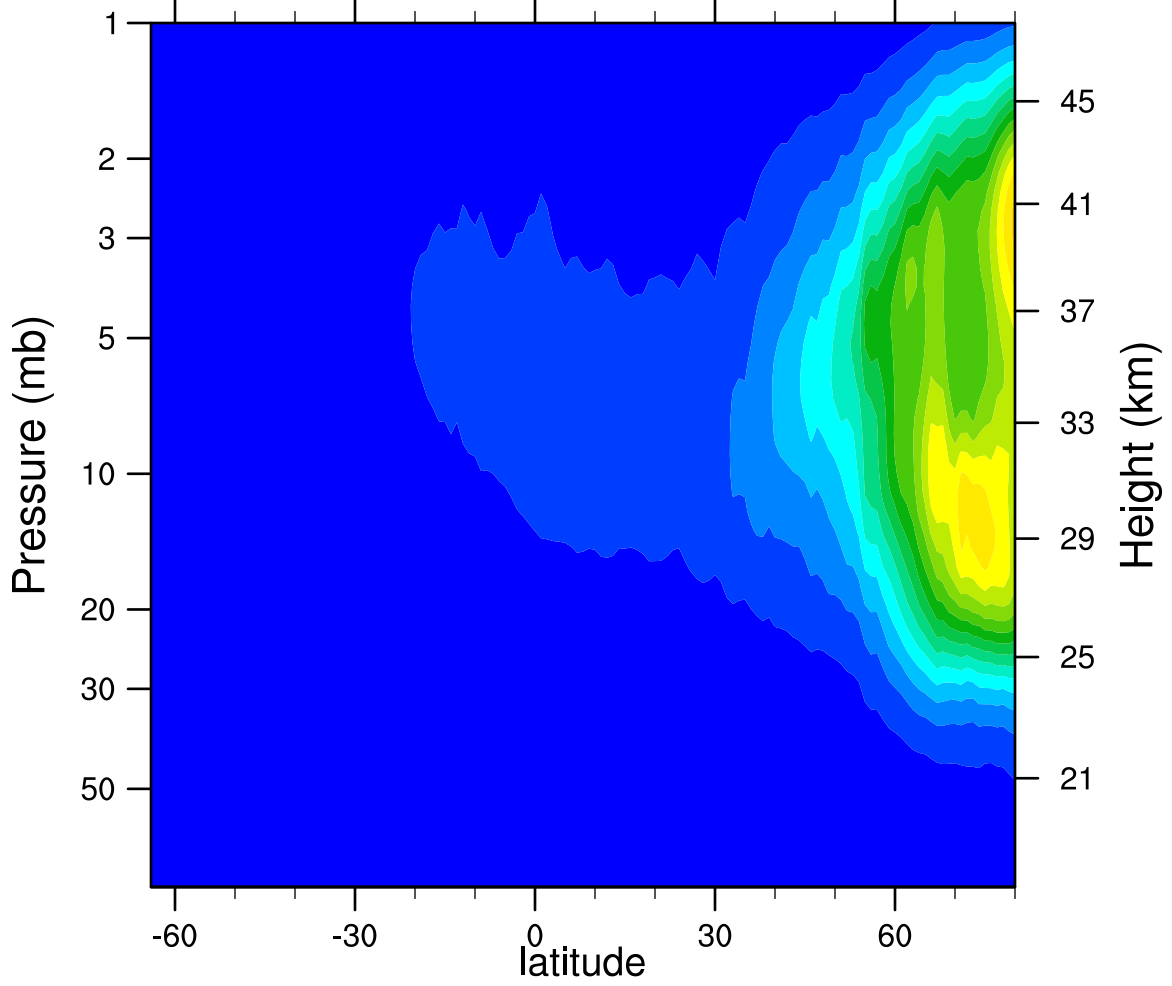
2005d317 N2O5_Ascending (ppbv)
