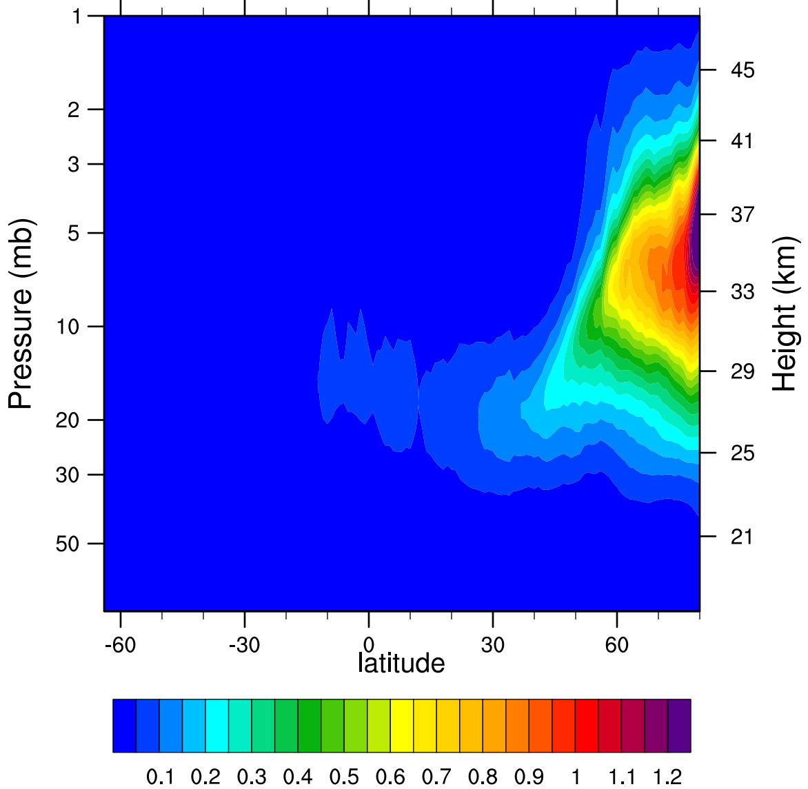
2007d034 N2O5_Ascending (ppbv)
