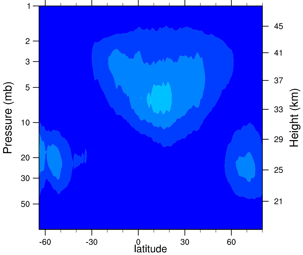
2005d264 N2O5_Ascending (ppbv)
