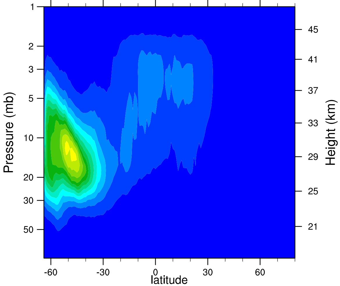
2007d217 N2O5_Ascending (ppbv)
