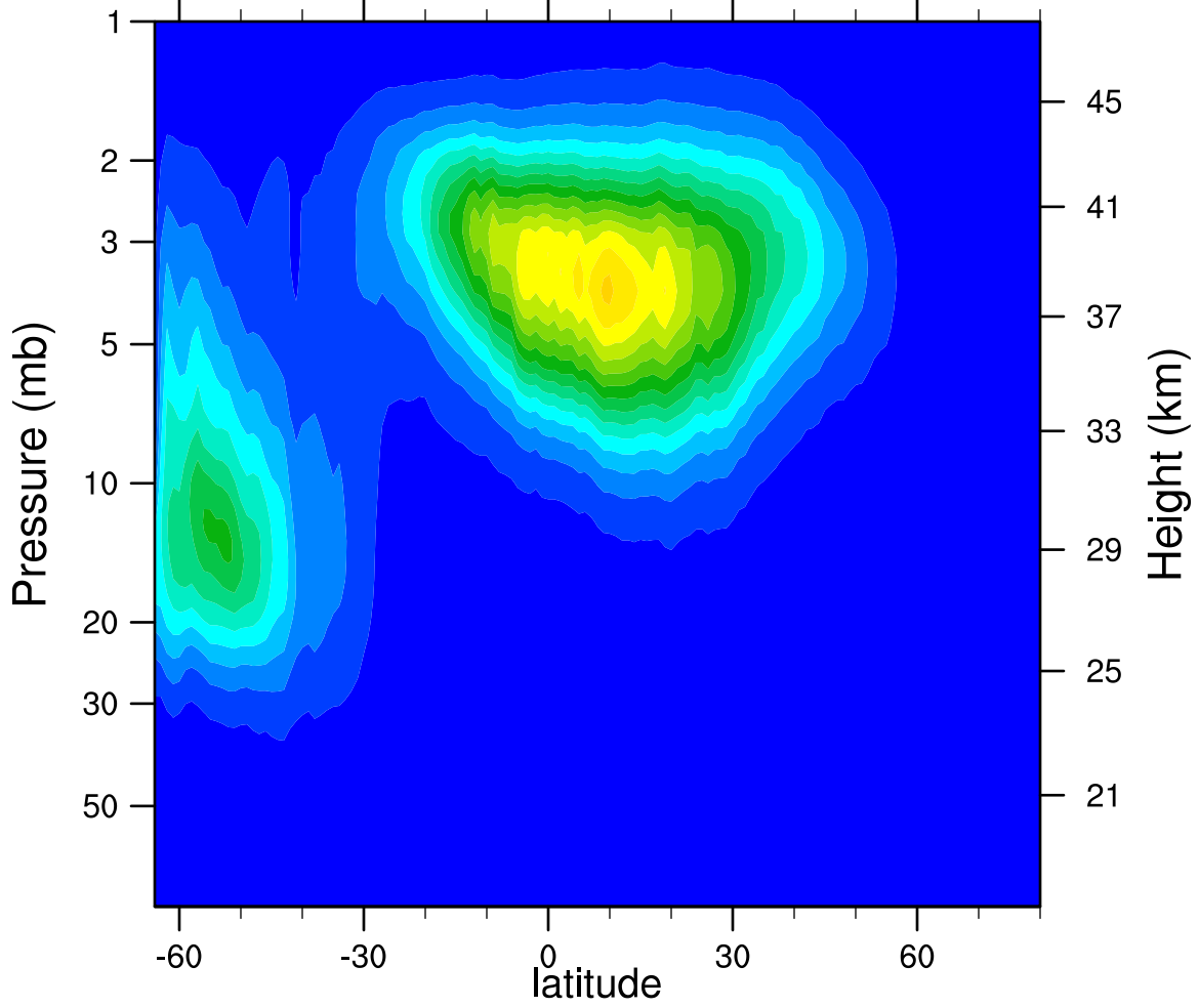
2005d145 N2O5_Ascending (ppbv)
