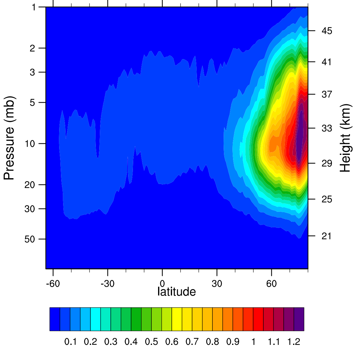
2007d354 N2O5_Ascending (ppbv)
