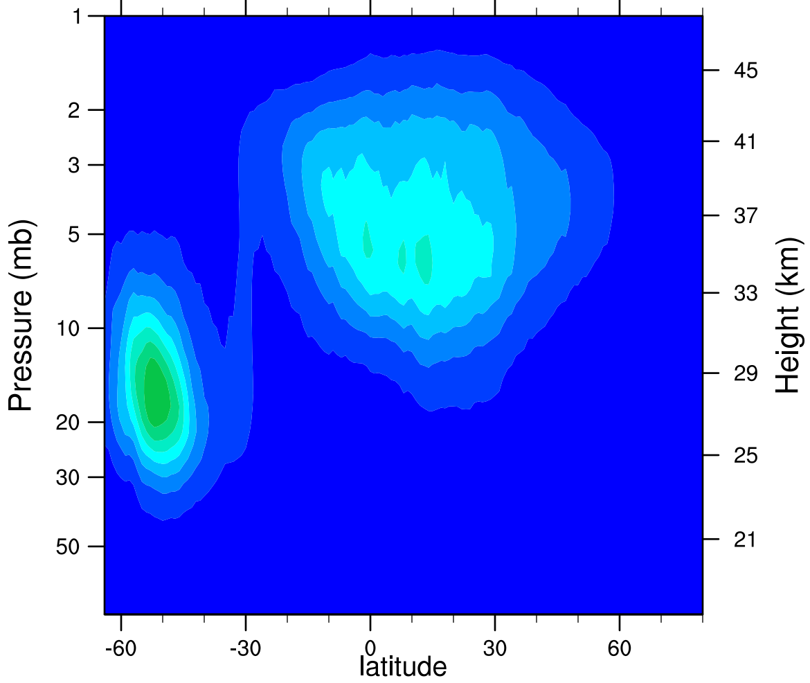
2005d222 N2O5_Ascending (ppbv)
