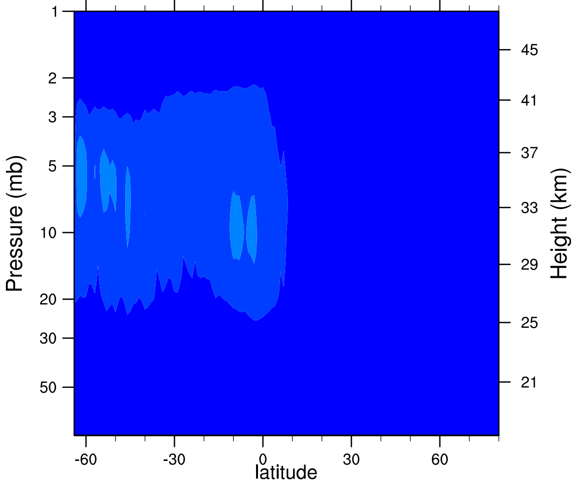
2006d178 N2O5_Ascending (ppbv)
