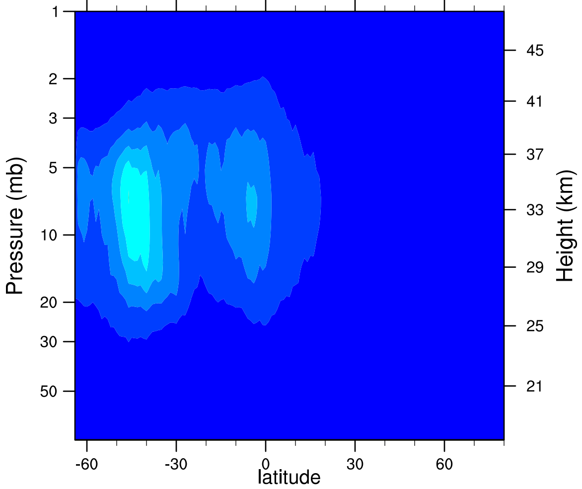
2006d195 N2O5_Ascending (ppbv)
