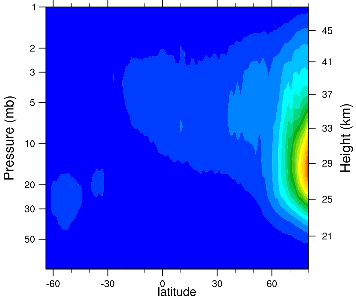
2005d296 N2O5_Ascending (ppbv)
