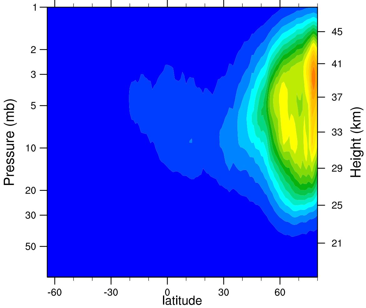
2005d326 N2O5_Ascending (ppbv)
