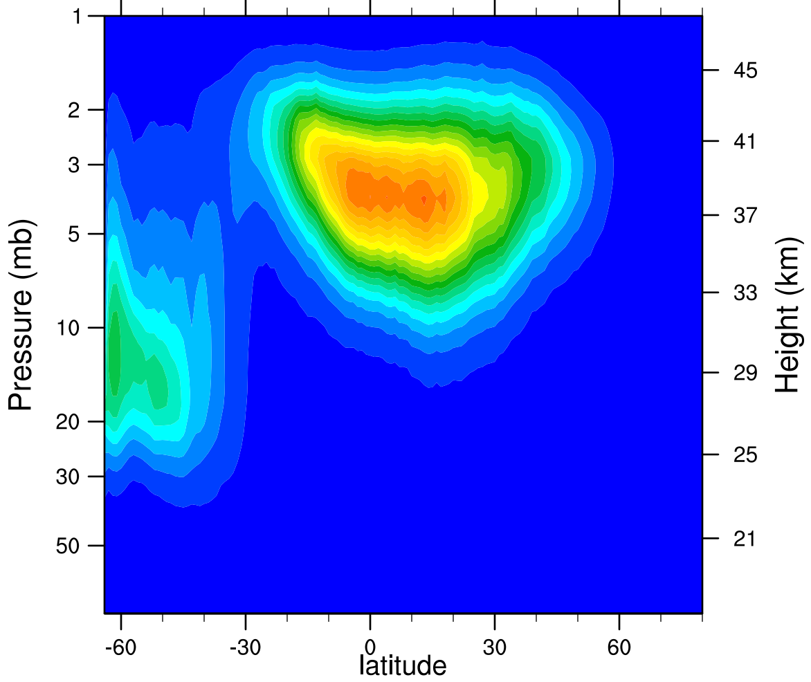
2005d126 N2O5_Ascending (ppbv)
