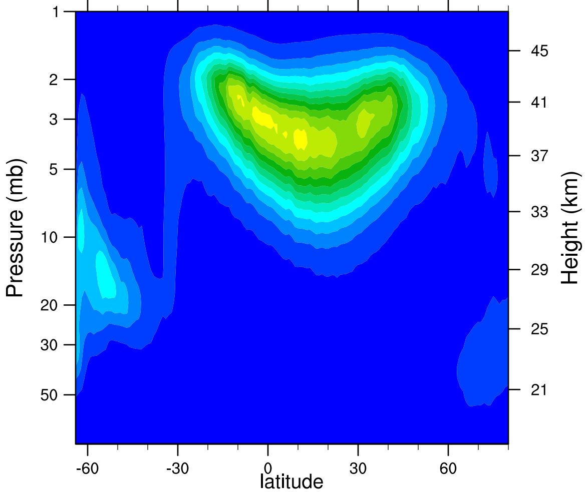
2005d094 N2O5_Ascending (ppbv)
