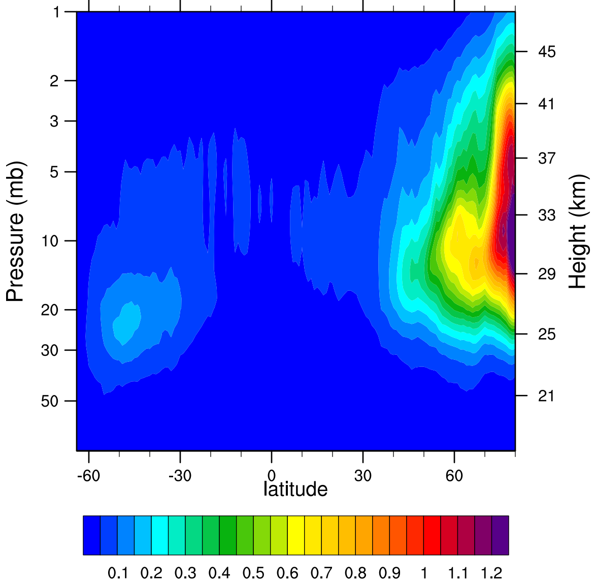
2006d335 N2O5_Ascending (ppbv)
