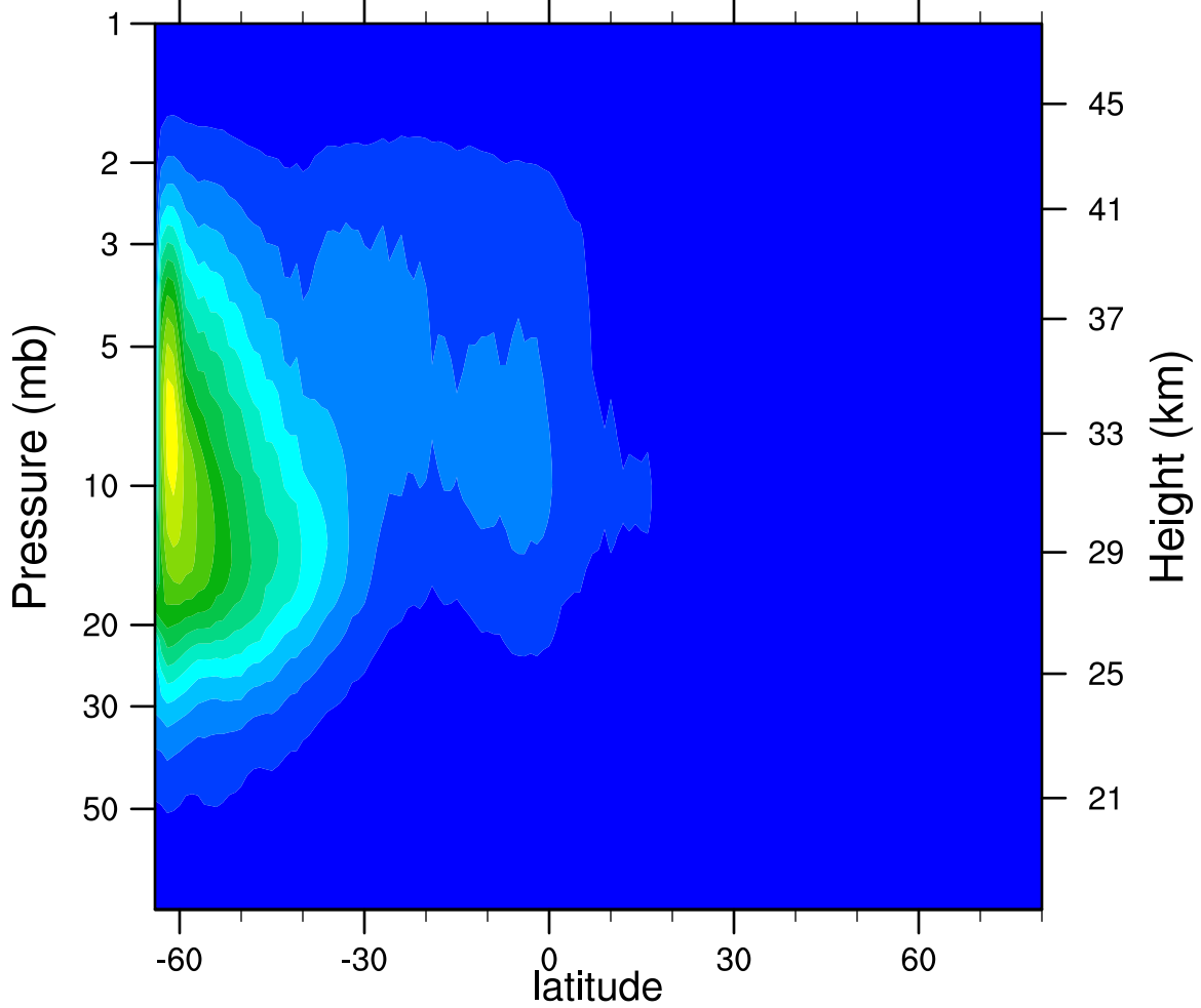
2006d131 N2O5_Ascending (ppbv)
