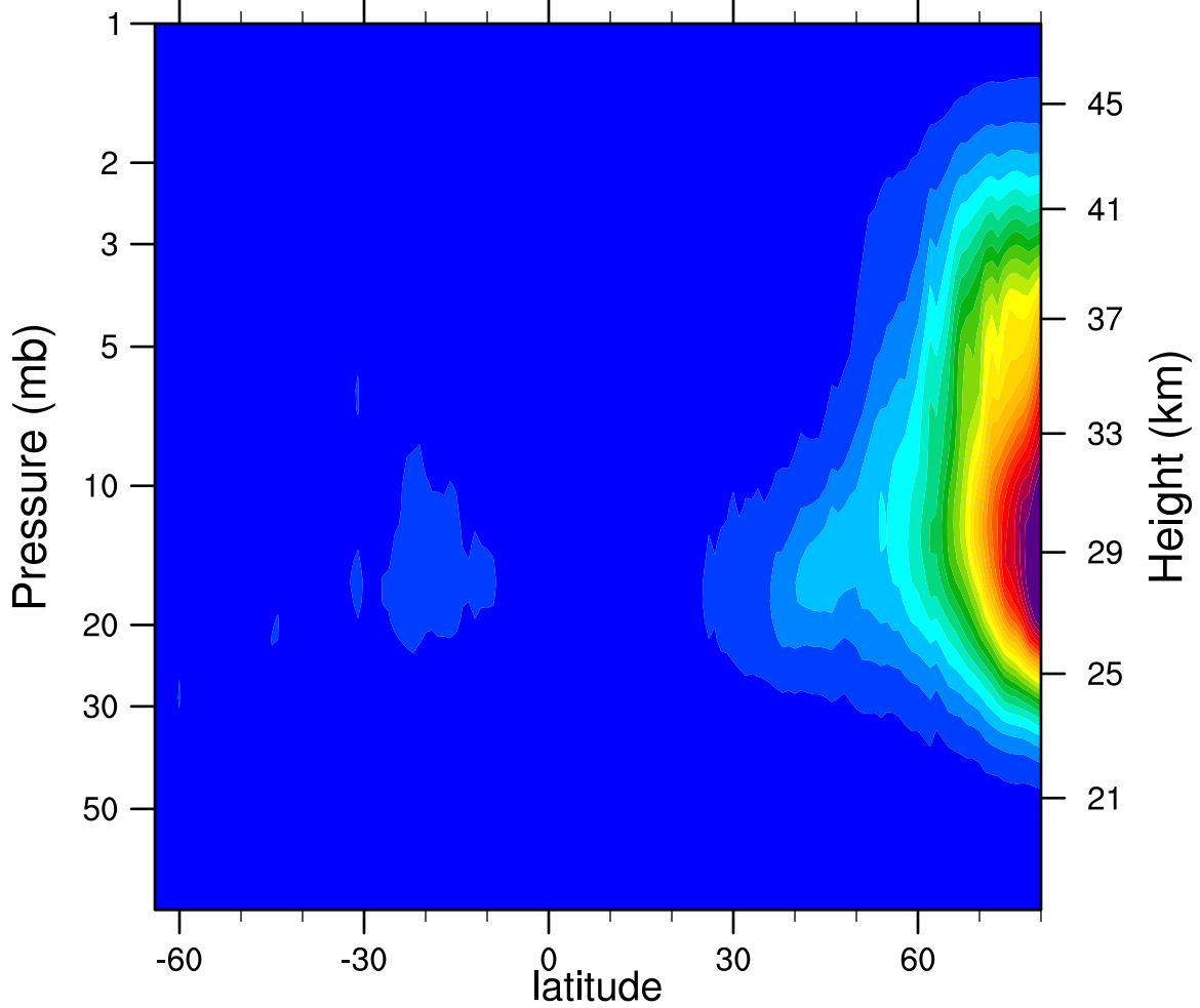
2006d305 N2O5_Ascending (ppbv)
