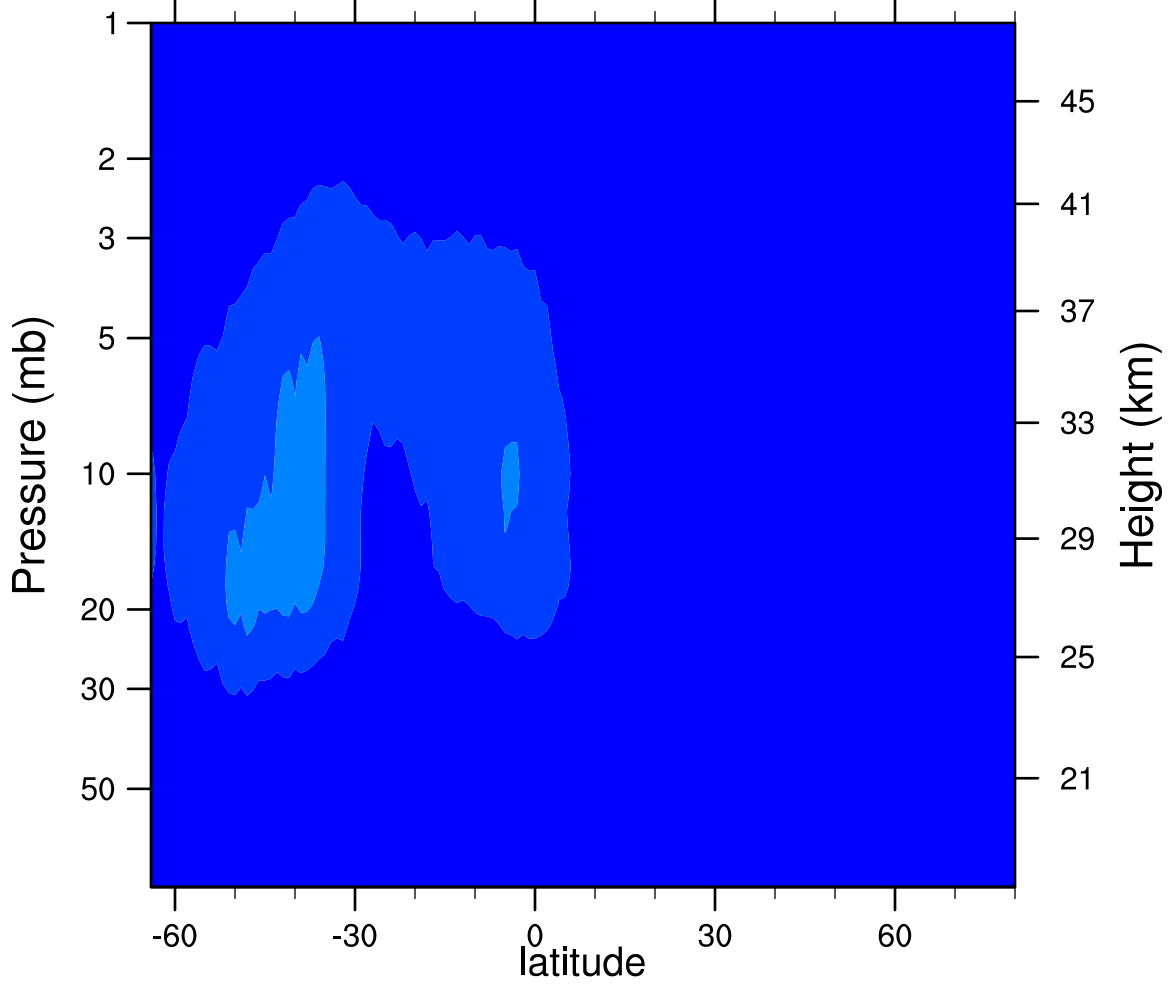
2006d225 N2O5_Ascending (ppbv)
