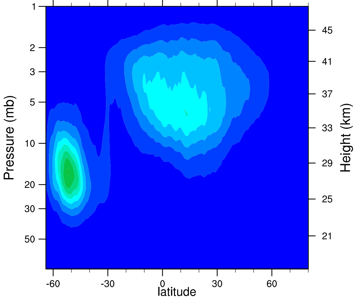
2005d224 N2O5_Ascending (ppbv)
