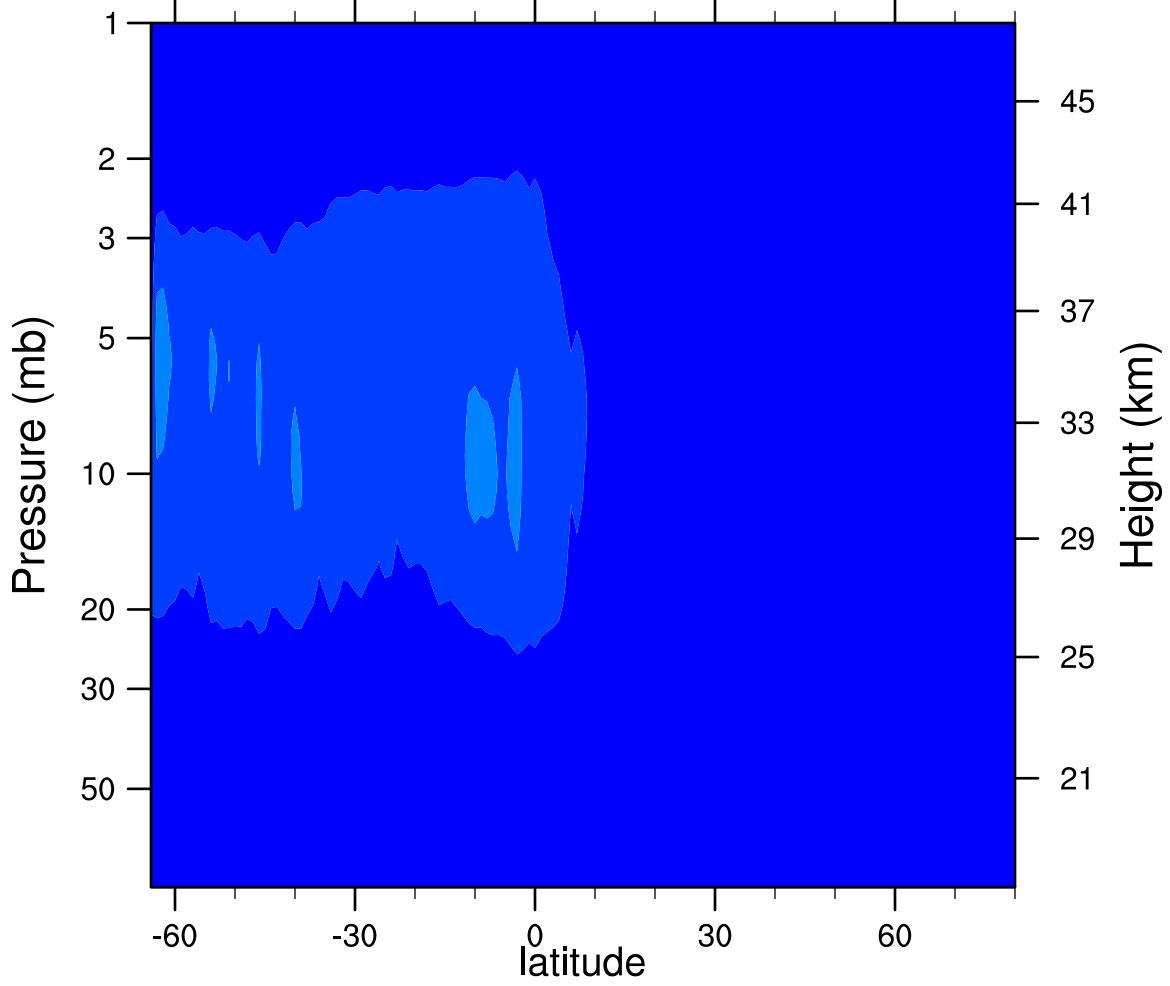
2006d179 N2O5_Ascending (ppbv)
