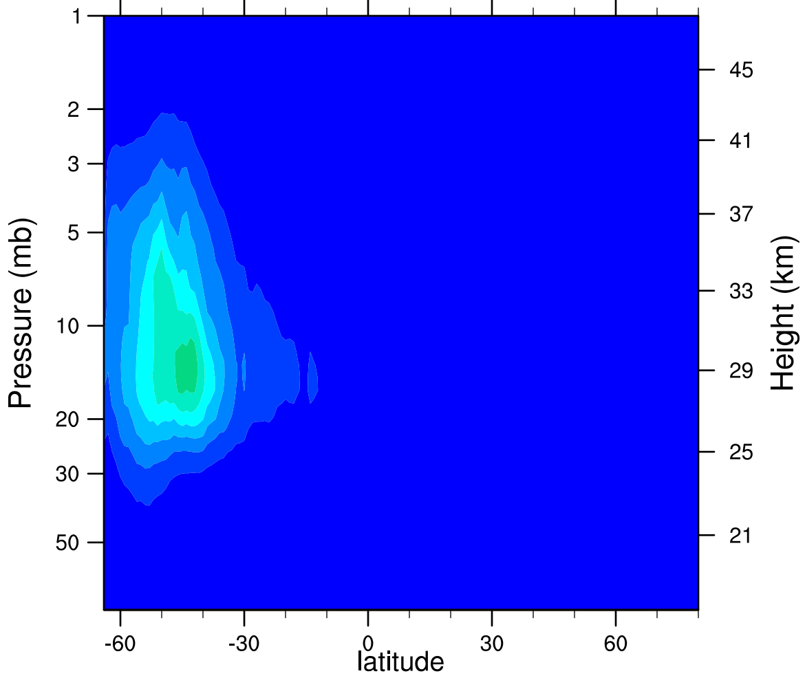
2007d203 N2O5_Ascending (ppbv)
