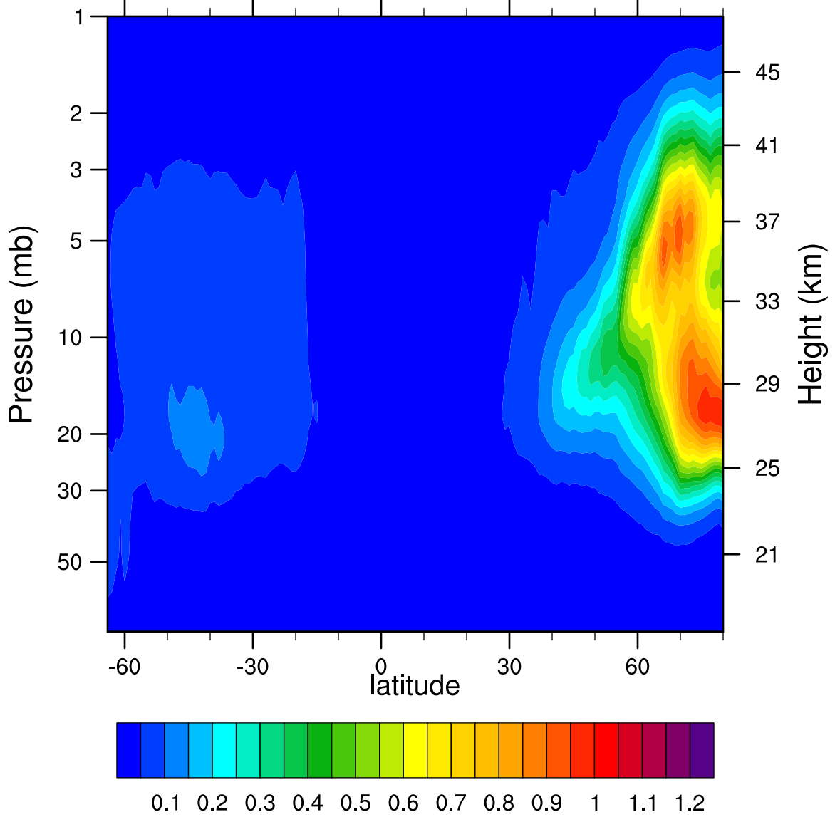
2006d312 N2O5_Ascending (ppbv)
