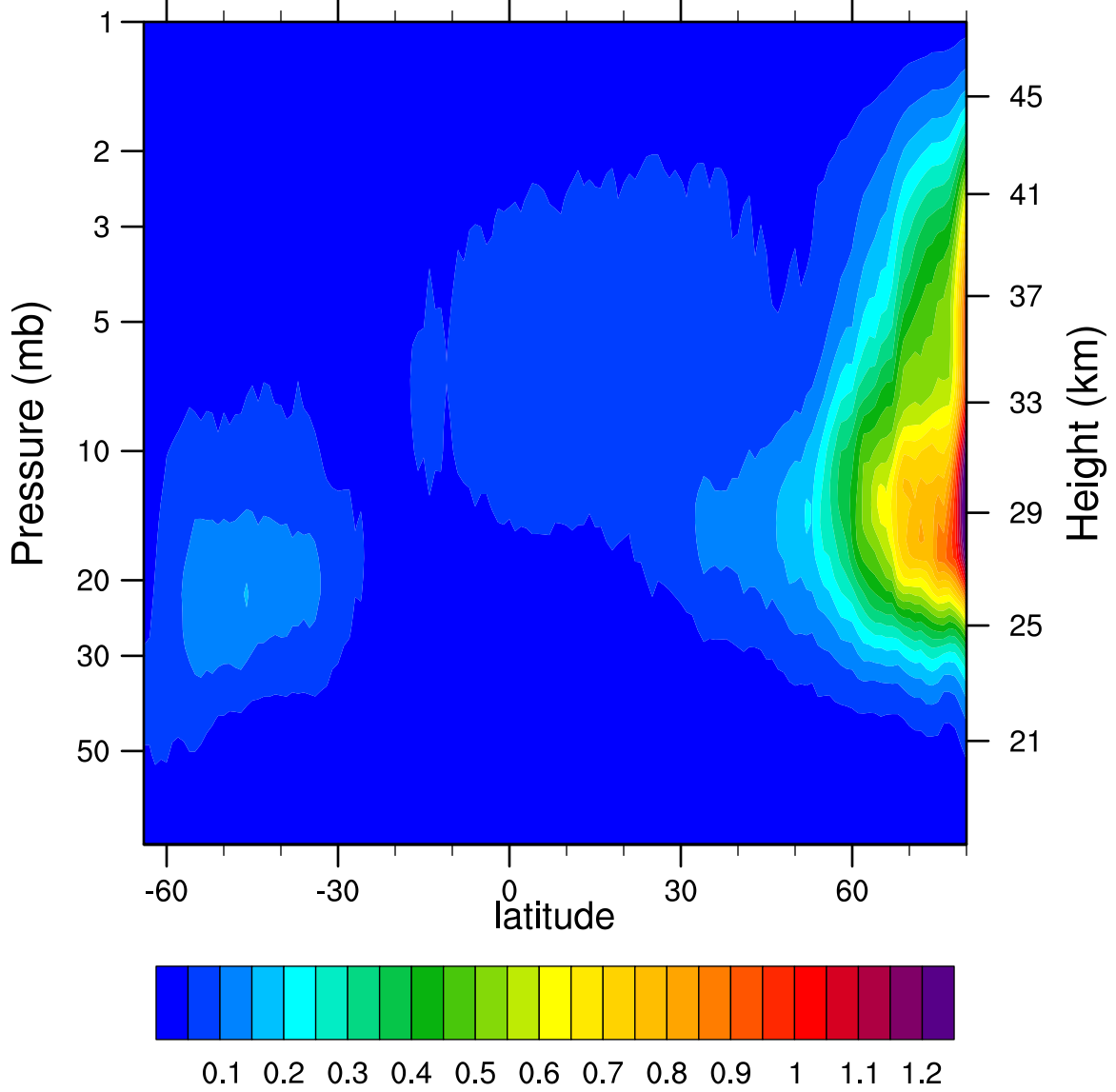
2007d309 N2O5_Ascending (ppbv)
