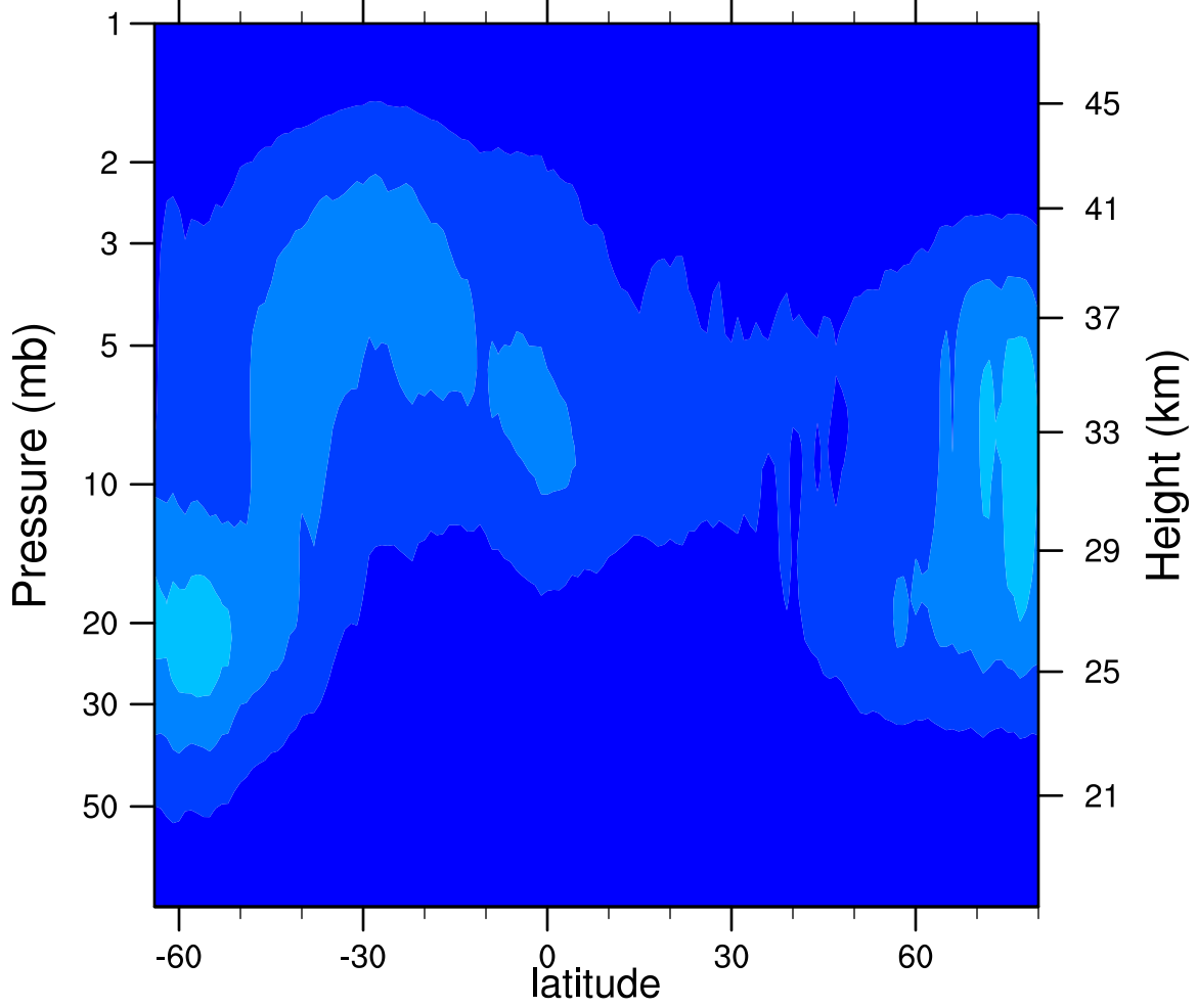
2006d083 N2O5_Ascending (ppbv)
