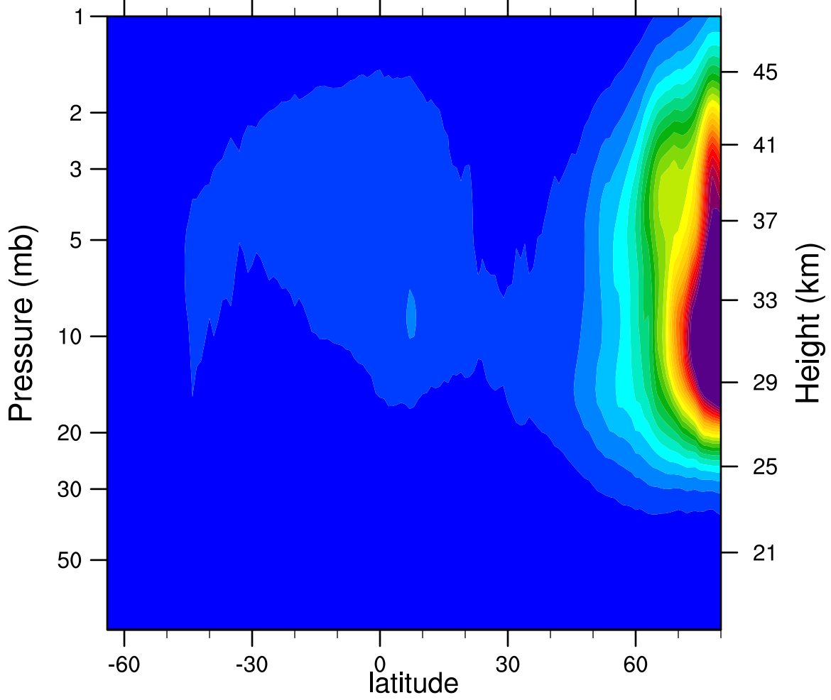
2006d038 N2O5_Ascending (ppbv)
