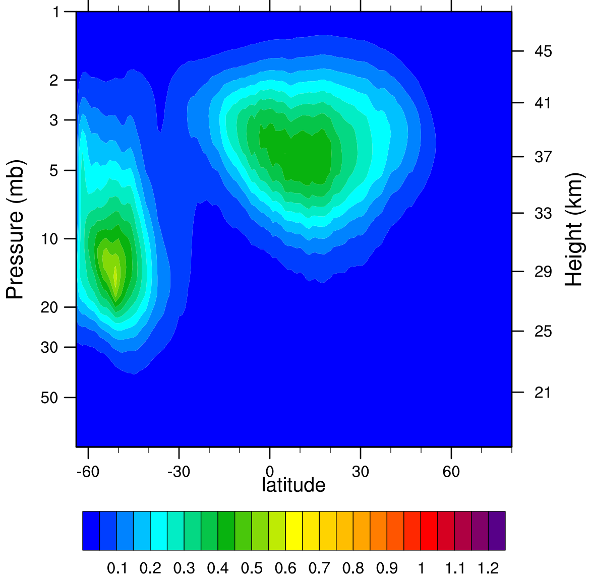
2005d162 N2O5_Ascending (ppbv)
