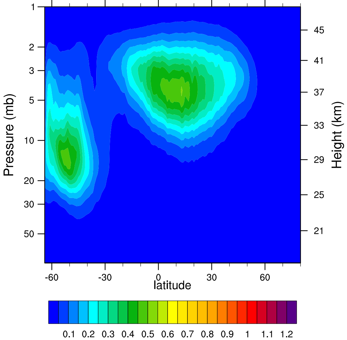
2005d156 N2O5_Ascending (ppbv)
