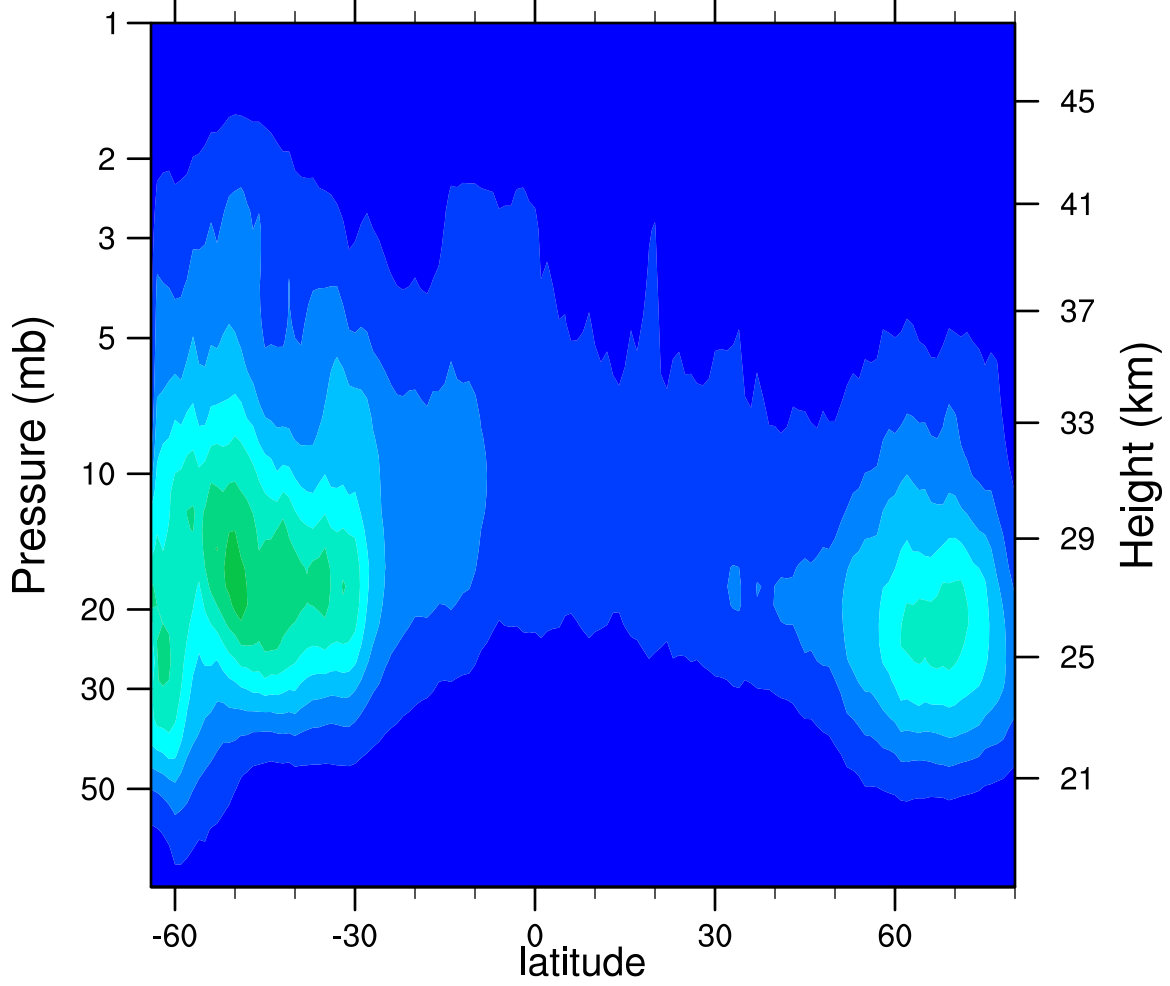
2007d257 N2O5_Ascending (ppbv)
