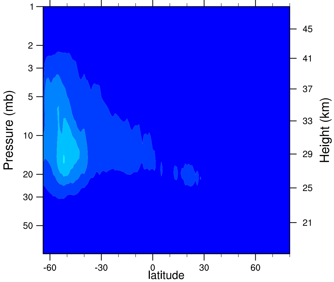
2007d187 N2O5_Ascending (ppbv)
