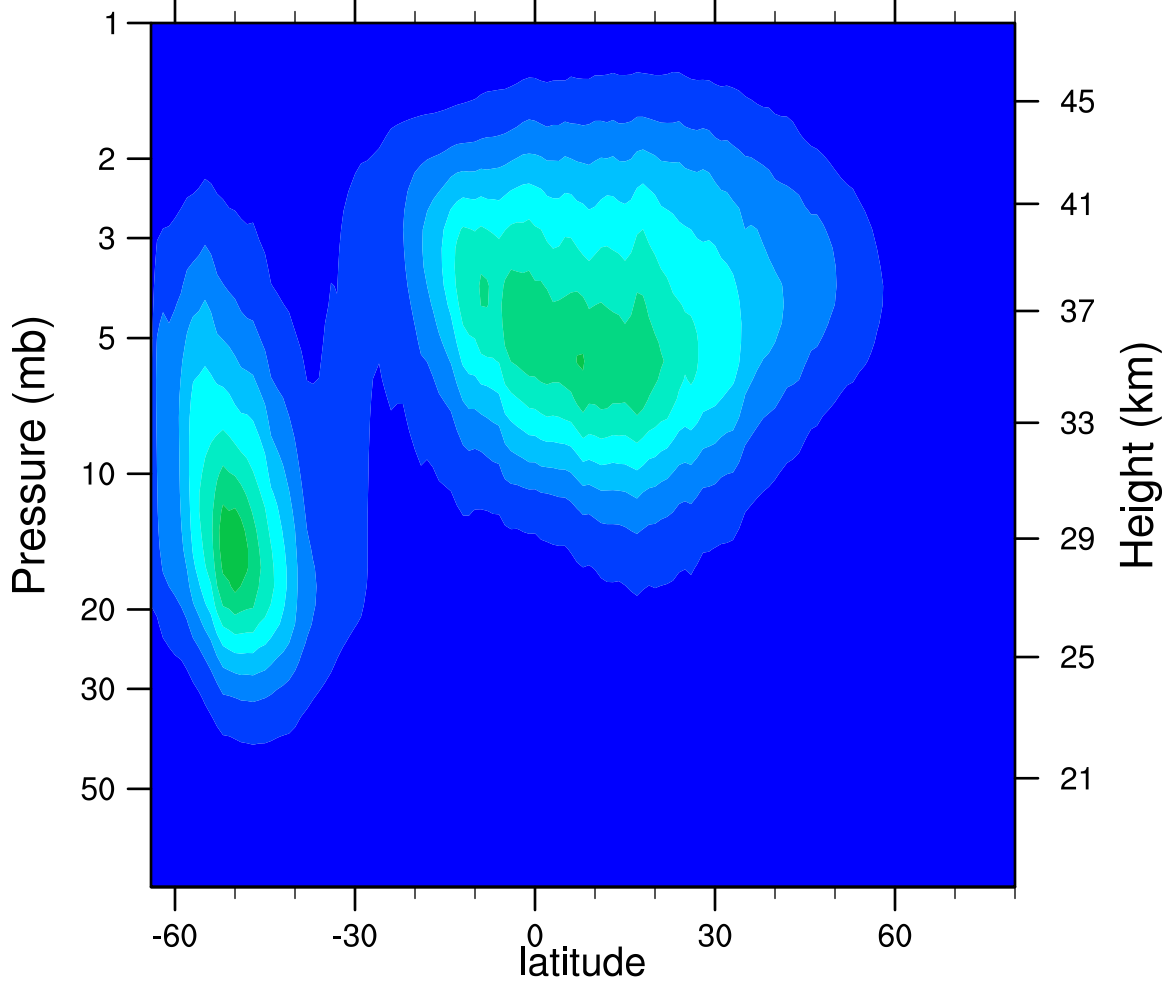
2005d206 N2O5_Ascending (ppbv)
