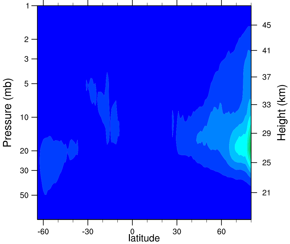
2006d281 N2O5_Ascending (ppbv)
