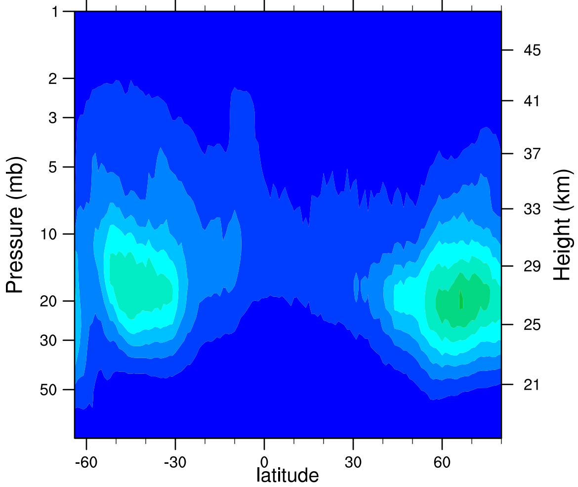
2007d265 N2O5_Ascending (ppbv)
