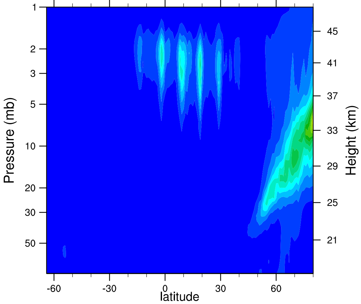
2005d023 N2O5_Ascending (ppbv)
