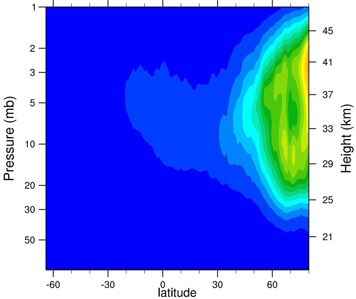
2005d319 N2O5_Ascending (ppbv)
