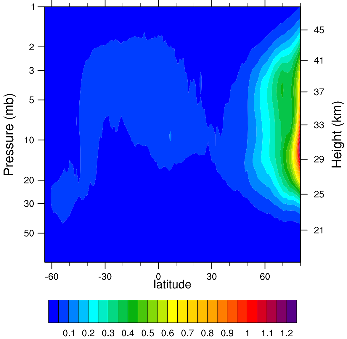
2006d051 N2O5_Ascending (ppbv)
