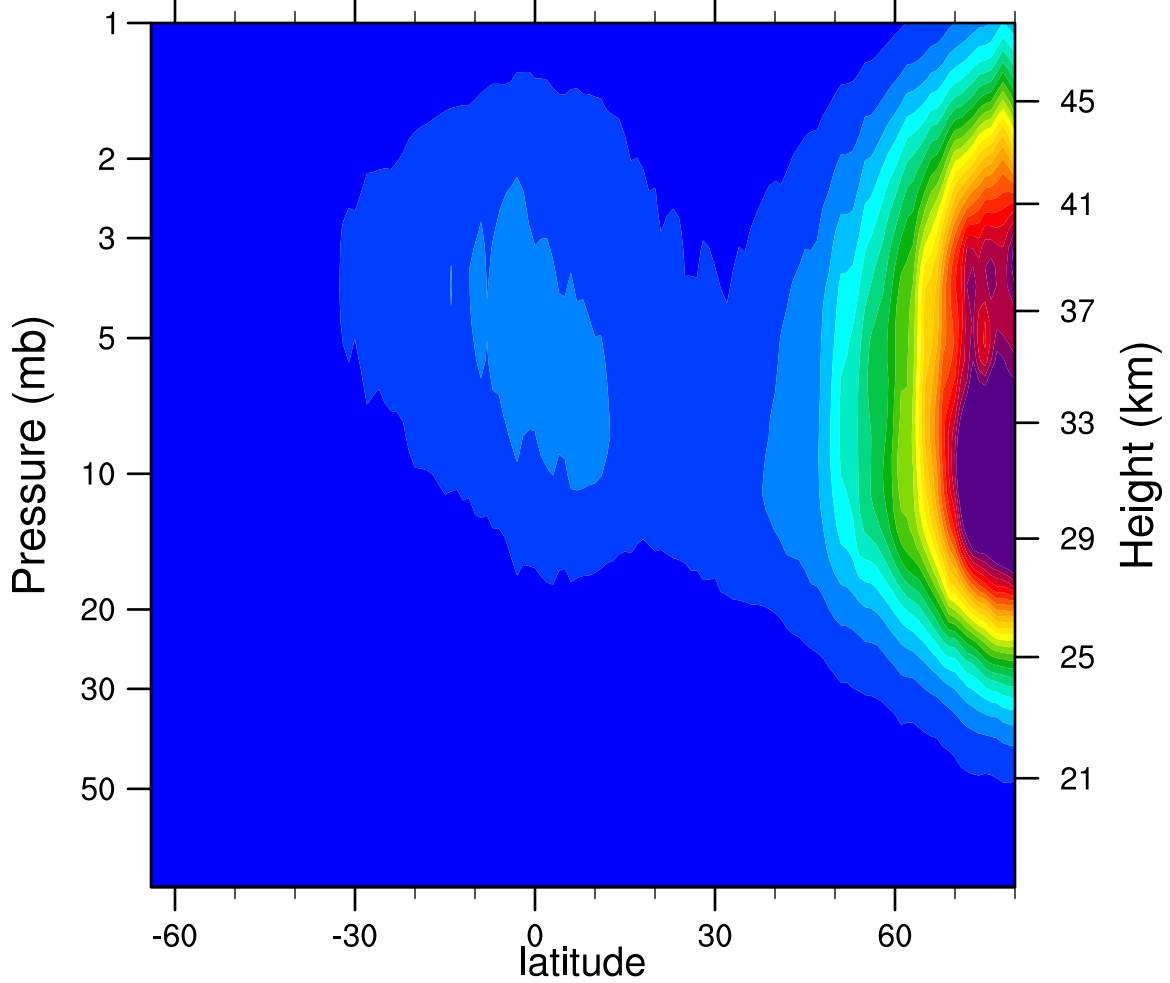
2006d019 N2O5_Ascending (ppbv)
