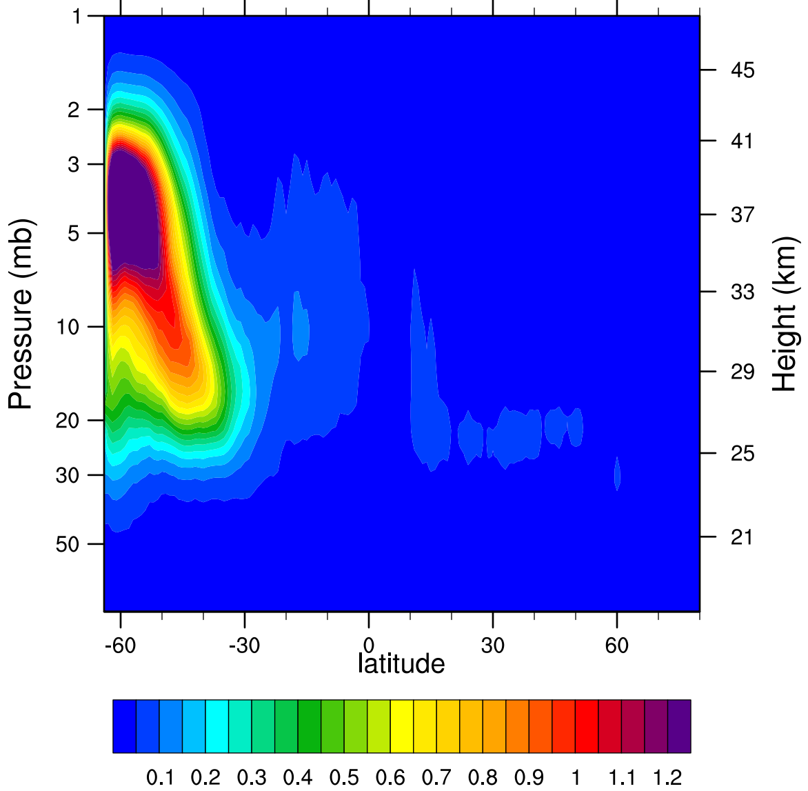
2007d145 N2O5_Ascending (ppbv)
