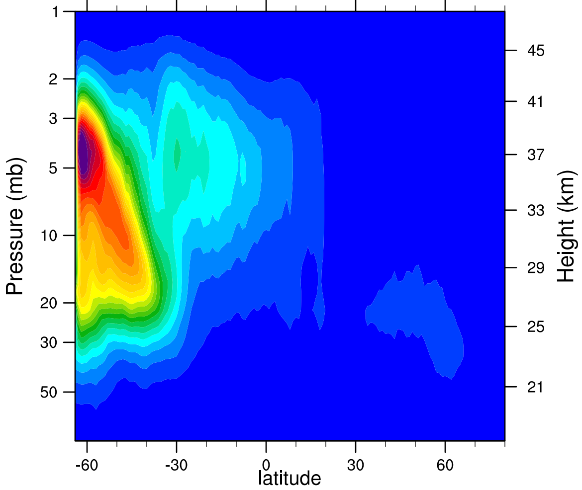
2007d130 N2O5_Ascending (ppbv)
