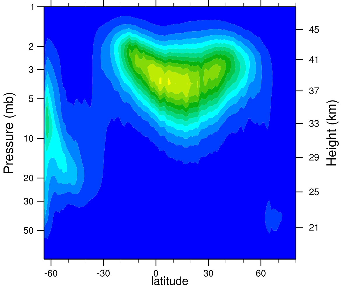
2005d103 N2O5_Ascending (ppbv)
