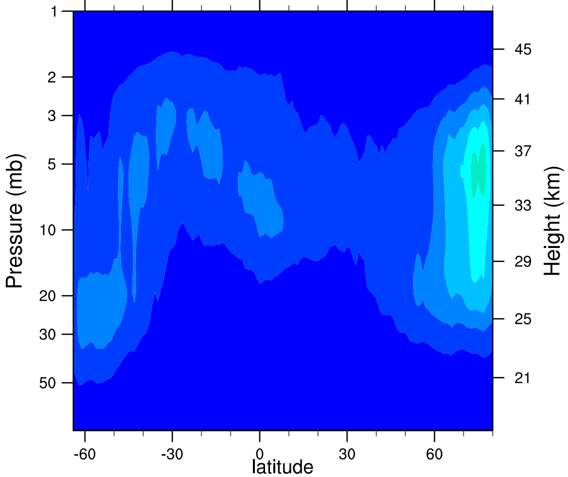
2006d073 N2O5_Ascending (ppbv)
