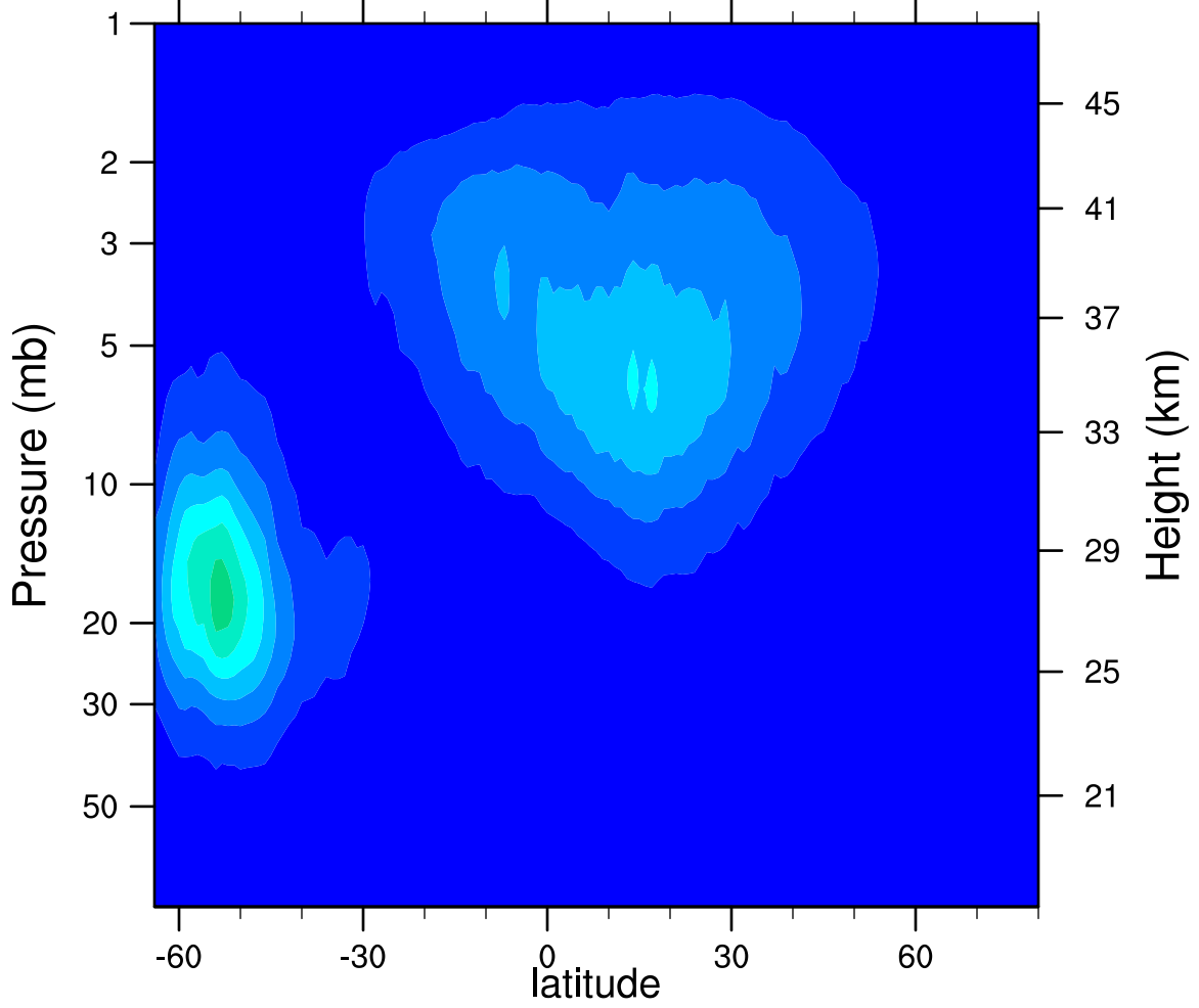
2005d233 N2O5_Ascending (ppbv)
