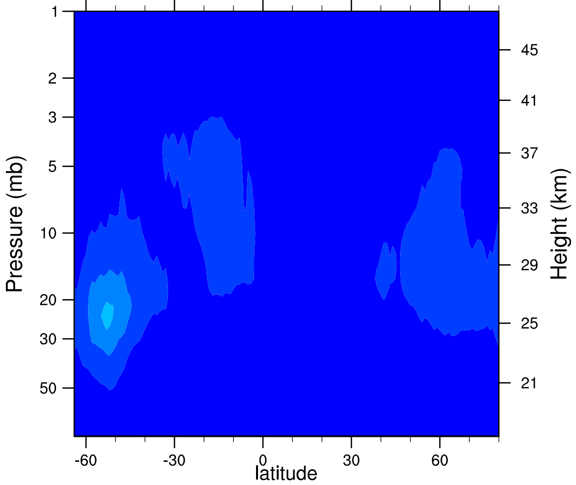
2006d265 N2O5_Ascending (ppbv)
