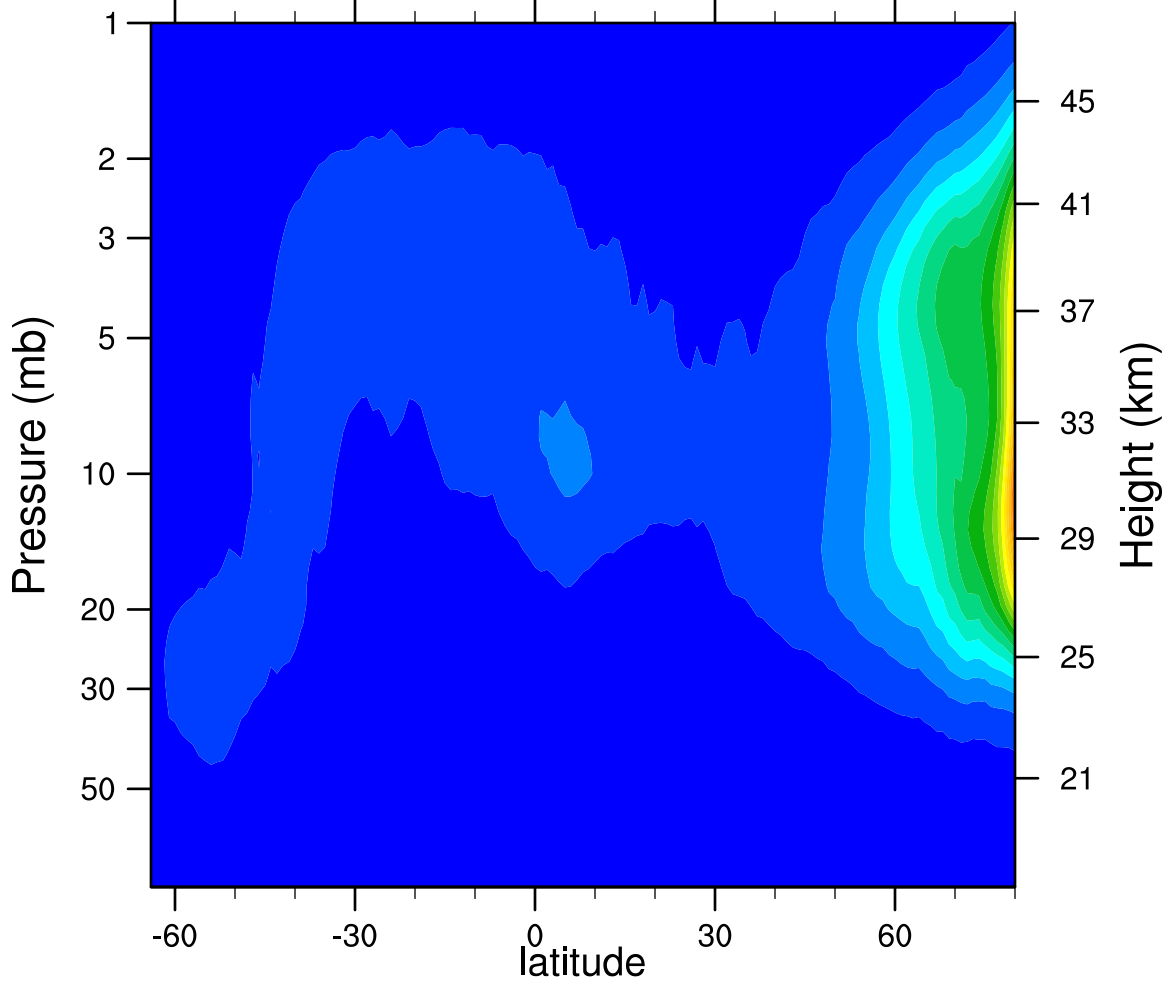
2006d054 N2O5_Ascending (ppbv)
