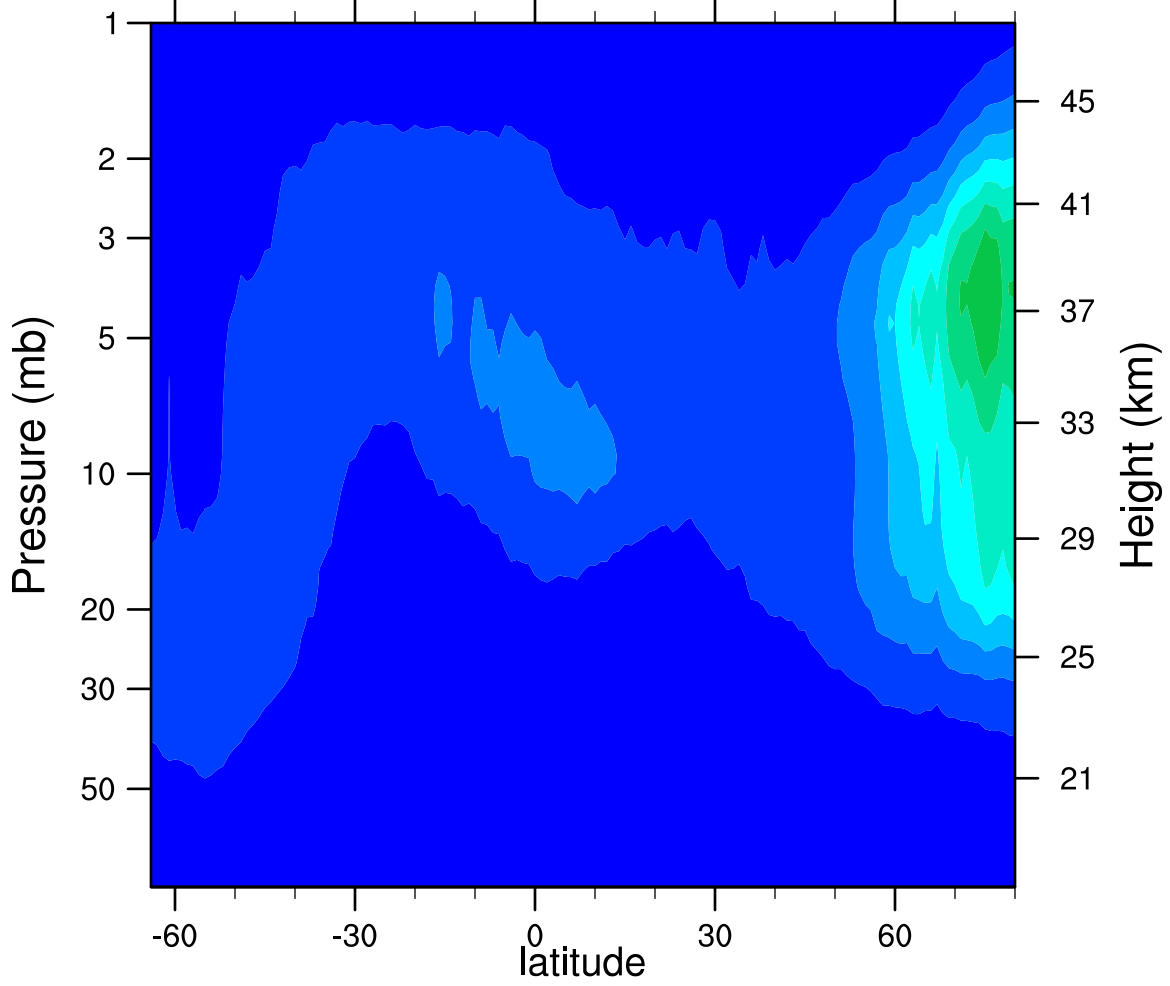
2006d064 N2O5_Ascending (ppbv)
