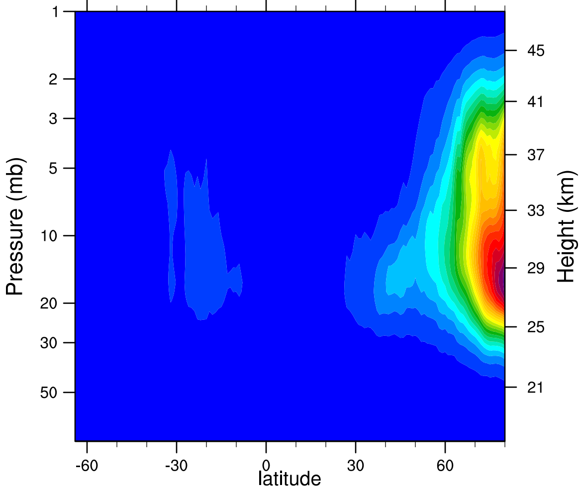
2006d307 N2O5_Ascending (ppbv)
