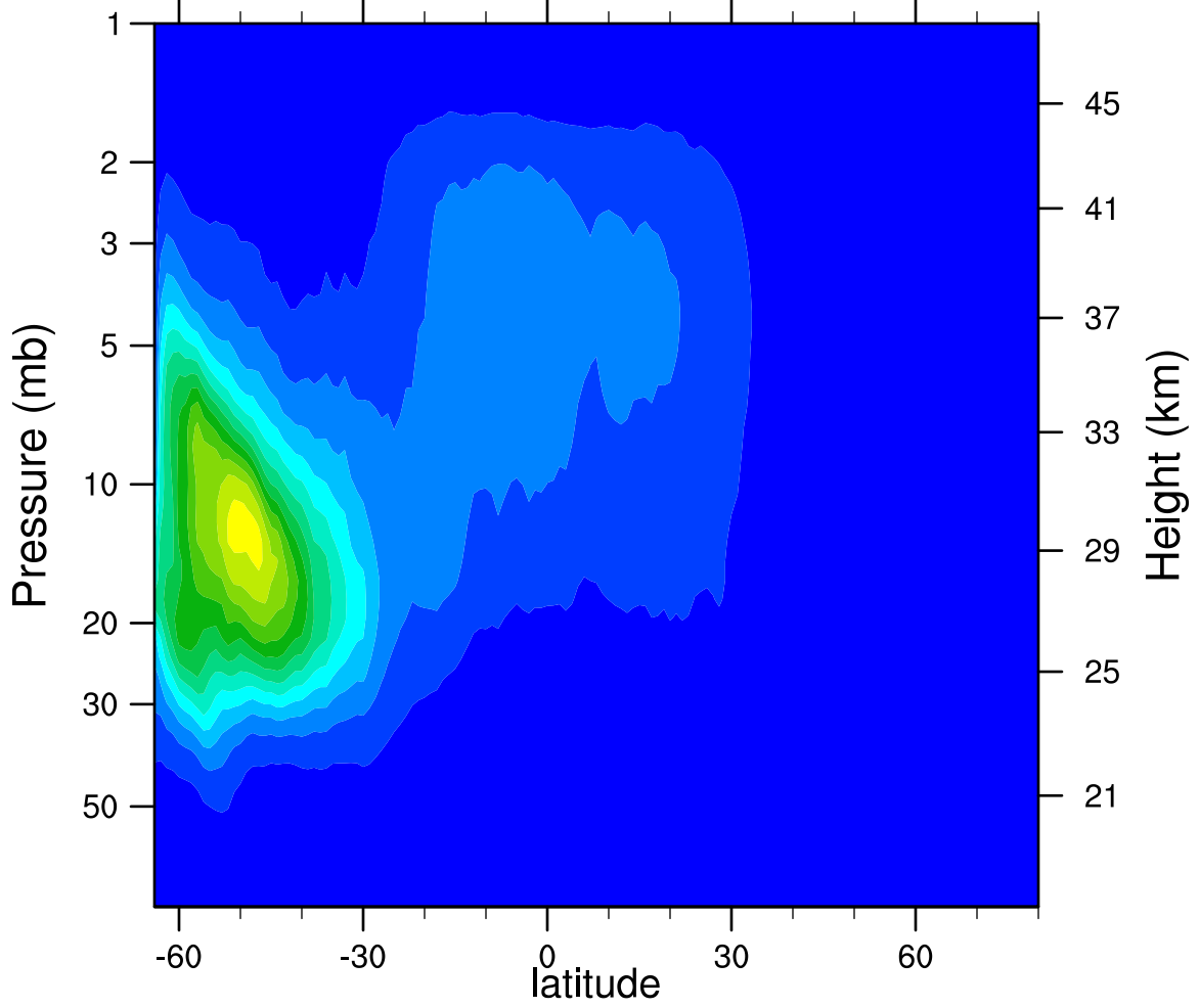
2007d224 N2O5_Ascending (ppbv)
