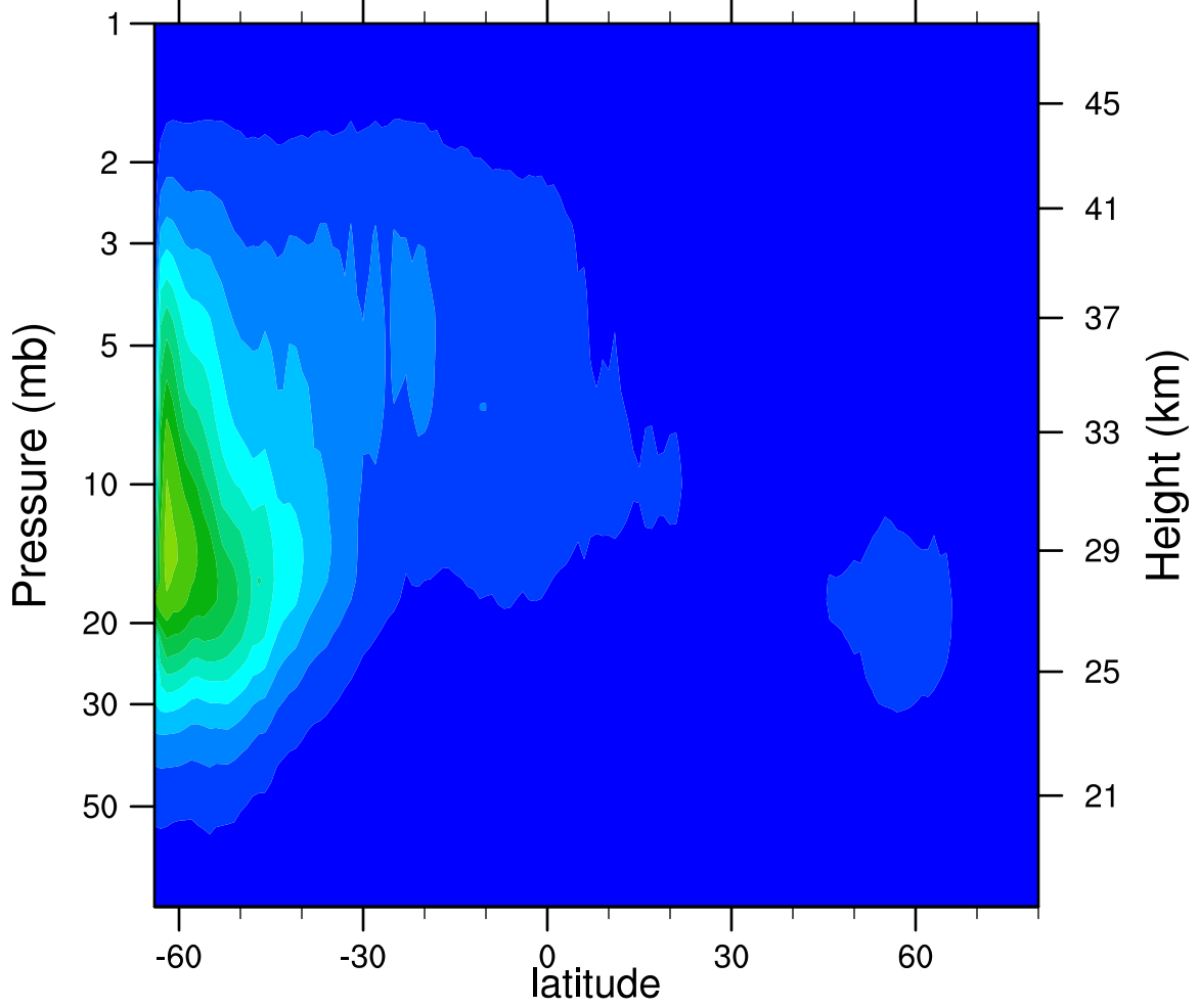
2006d113 N2O5_Ascending (ppbv)
