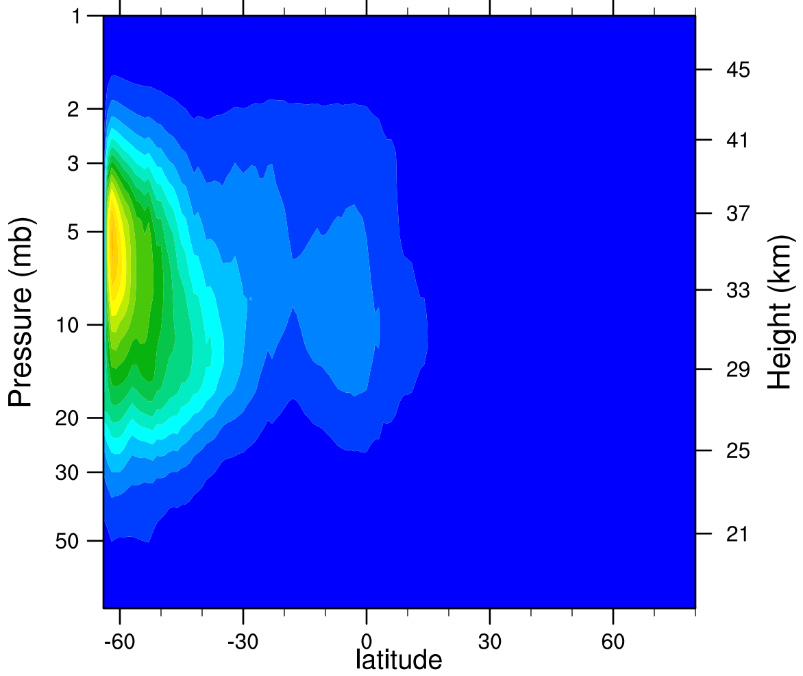
2006d145 N2O5_Ascending (ppbv)
