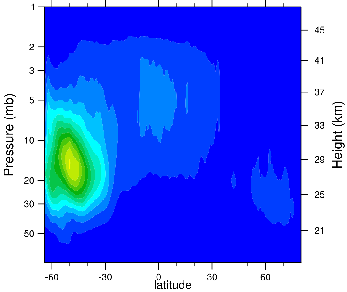
2007d234 N2O5_Ascending (ppbv)
