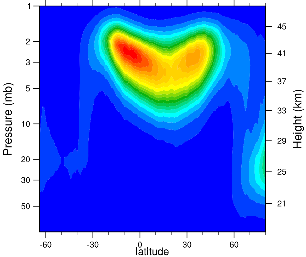
2005d068 N2O5_Ascending (ppbv)
