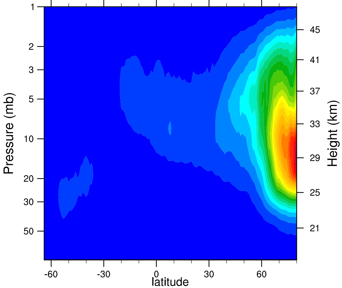
2005d308 N2O5_Ascending (ppbv)
