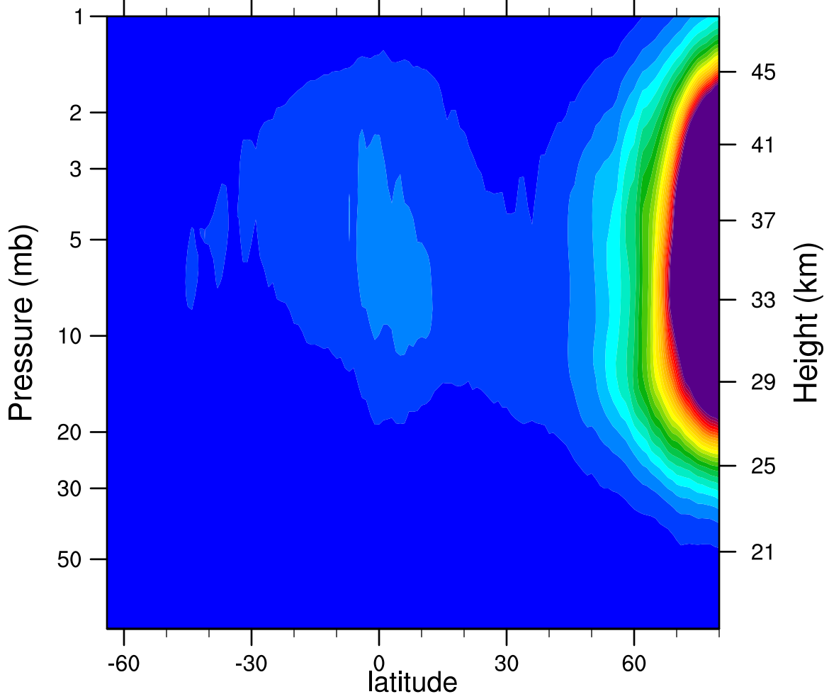
2006d027 N2O5_Ascending (ppbv)
