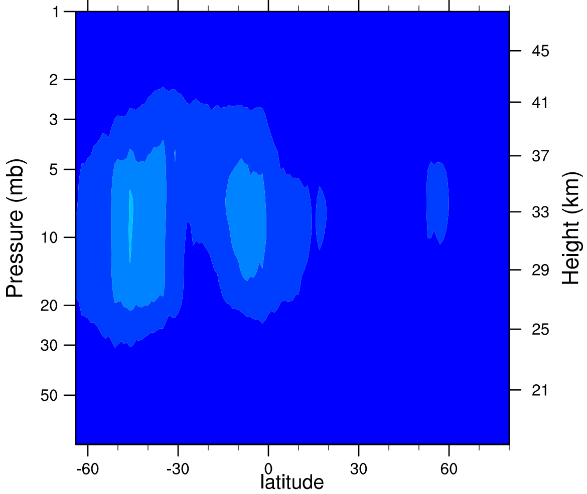
2006d216 N2O5_Ascending (ppbv)
