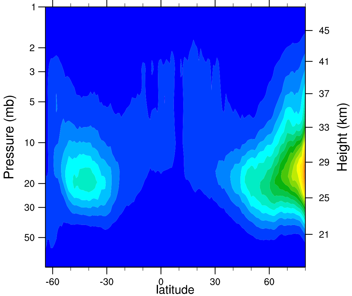
2007d281 N2O5_Ascending (ppbv)
