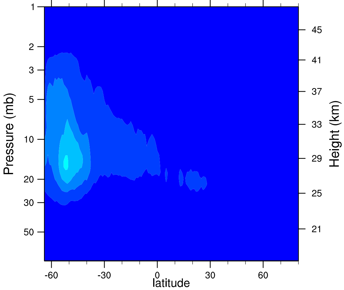
2007d186 N2O5_Ascending (ppbv)
