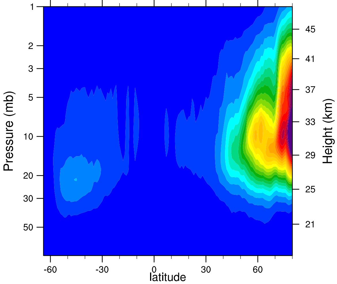
2006d338 N2O5_Ascending (ppbv)
