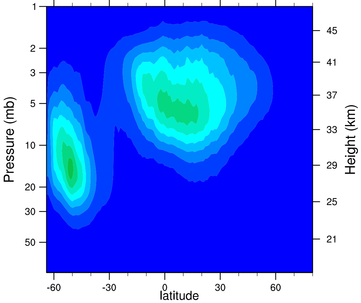
2005d211 N2O5_Ascending (ppbv)
