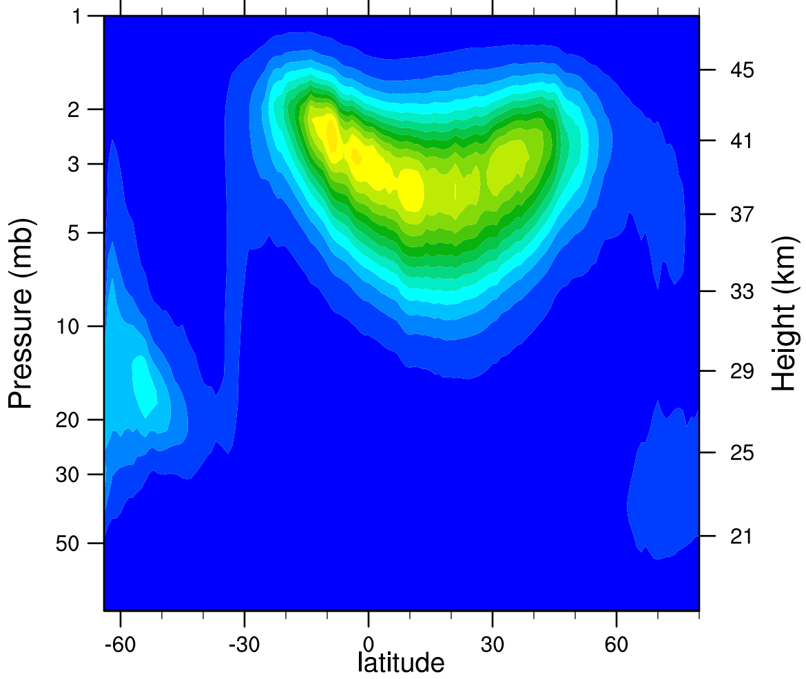
2005d089 N2O5_Ascending (ppbv)
