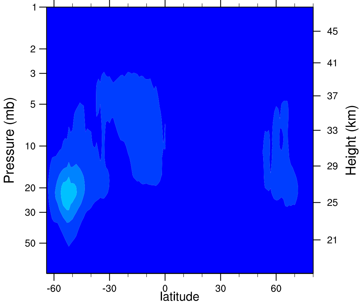
2006d258 N2O5_Ascending (ppbv)
