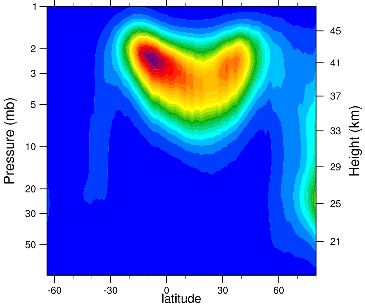
2005d060 N2O5_Ascending (ppbv)
