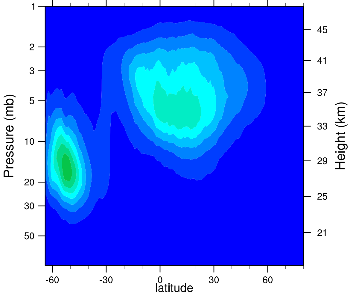
2005d218 N2O5_Ascending (ppbv)
