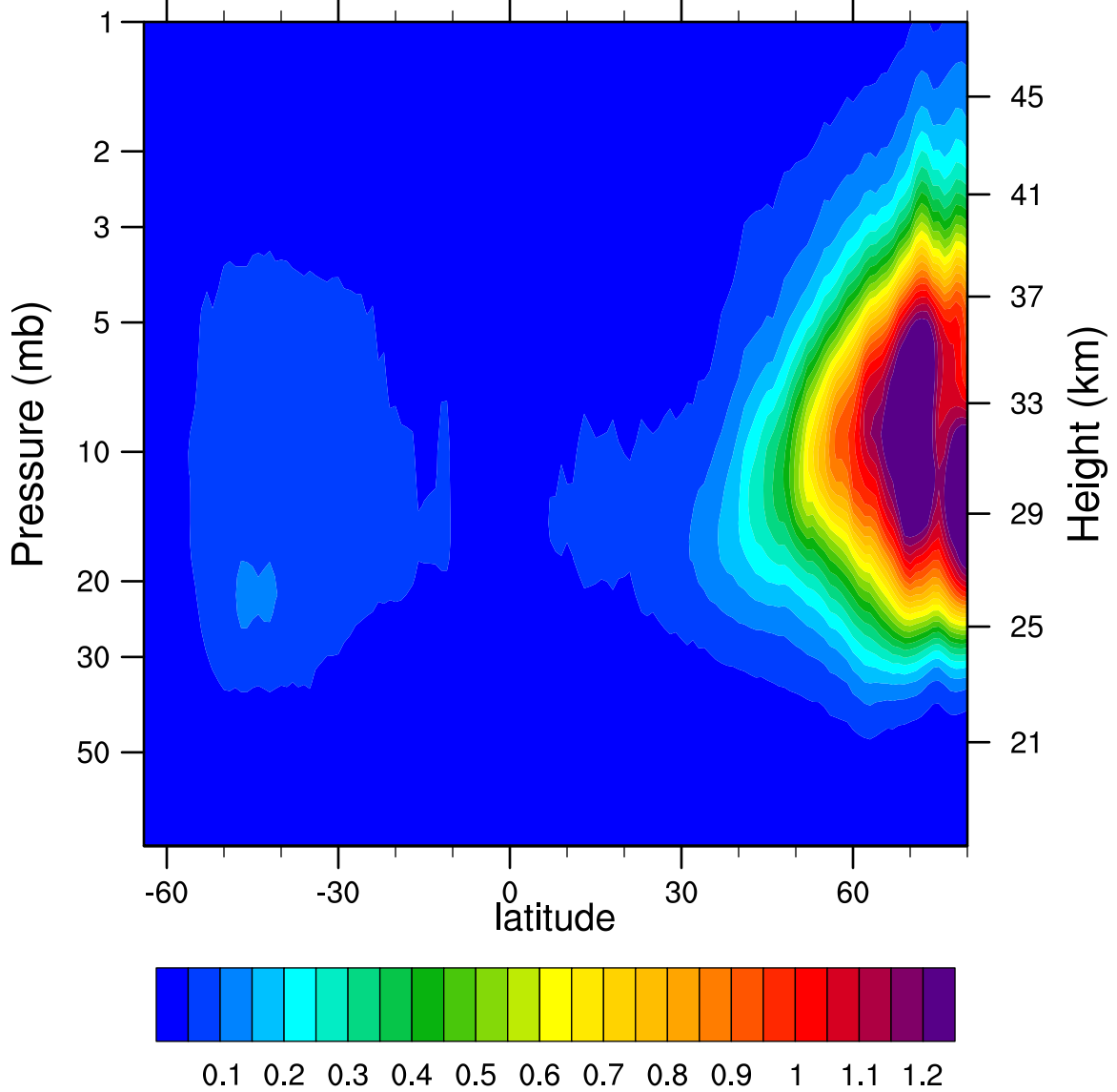
2006d351 N2O5_Ascending (ppbv)
