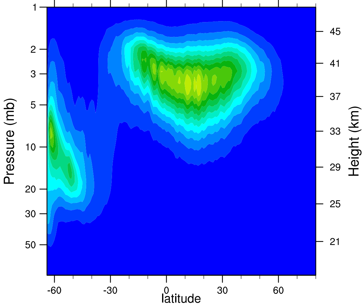
2005d114 N2O5_Ascending (ppbv)
