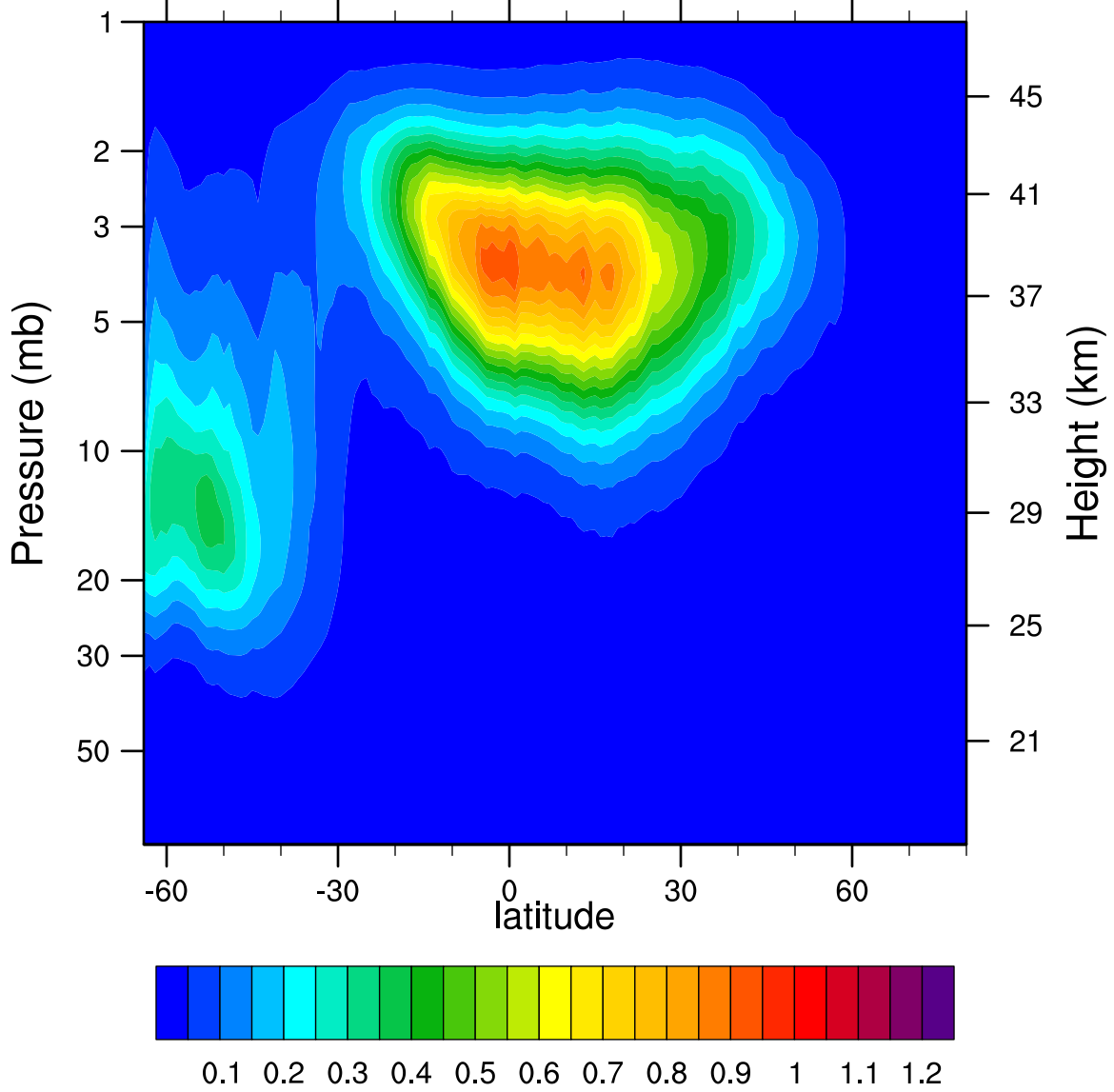
2005d130 N2O5_Ascending (ppbv)
