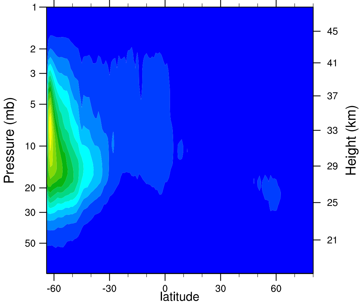
2006d123 N2O5_Ascending (ppbv)
