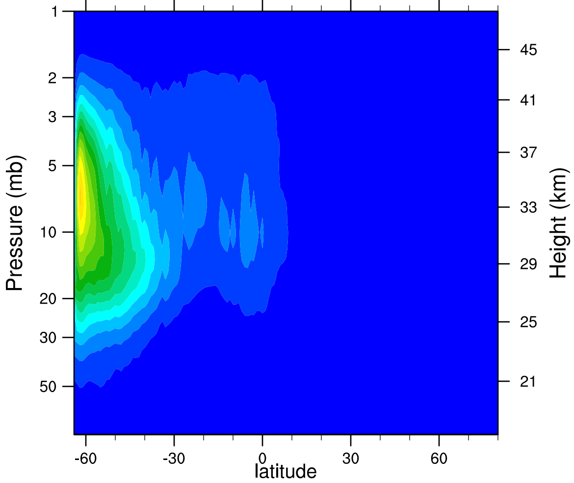
2006d138 N2O5_Ascending (ppbv)
