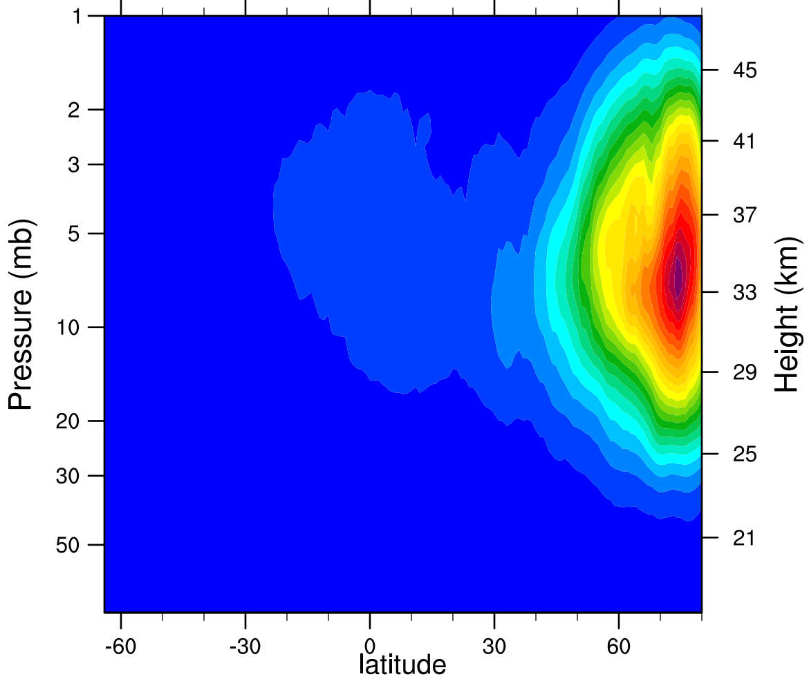
2005d342 N2O5_Ascending (ppbv)
