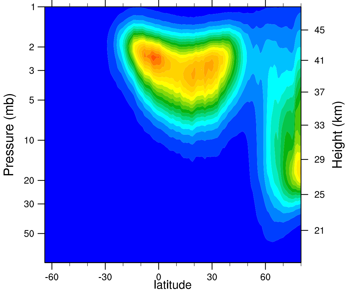
2005d039 N2O5_Ascending (ppbv)
