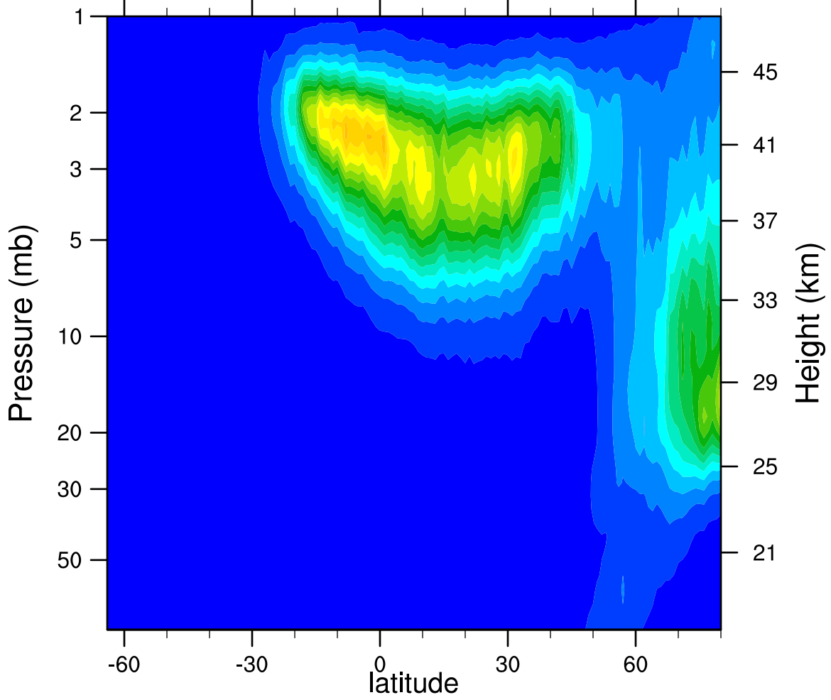
2005d027 N2O5_Ascending (ppbv)
