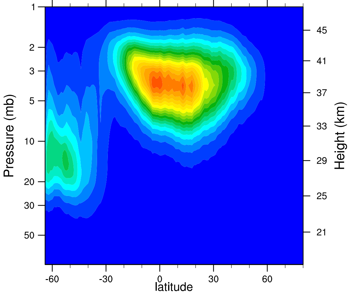
2005d129 N2O5_Ascending (ppbv)
