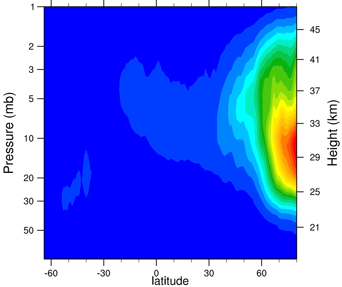
2005d311 N2O5_Ascending (ppbv)
