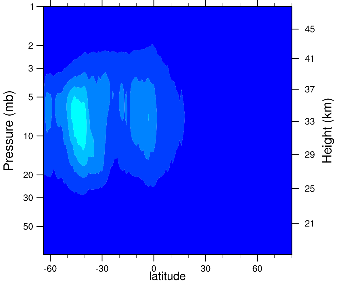
2006d193 N2O5_Ascending (ppbv)
