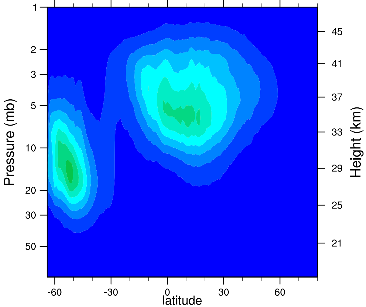
2005d214 N2O5_Ascending (ppbv)
