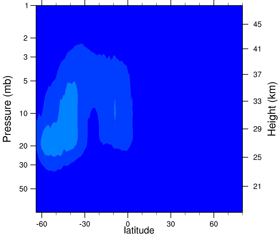
2006d229 N2O5_Ascending (ppbv)
