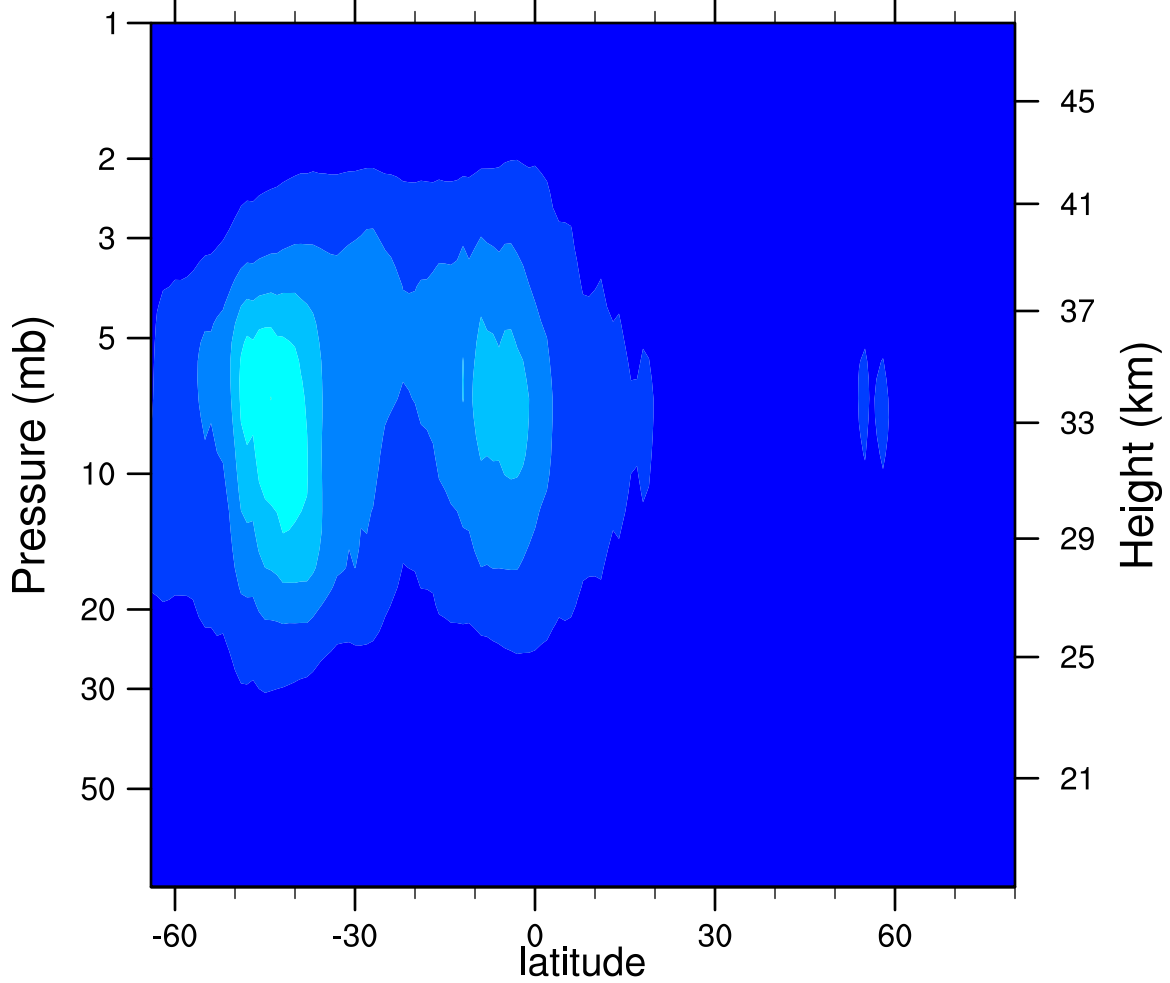
2006d203 N2O5_Ascending (ppbv)
