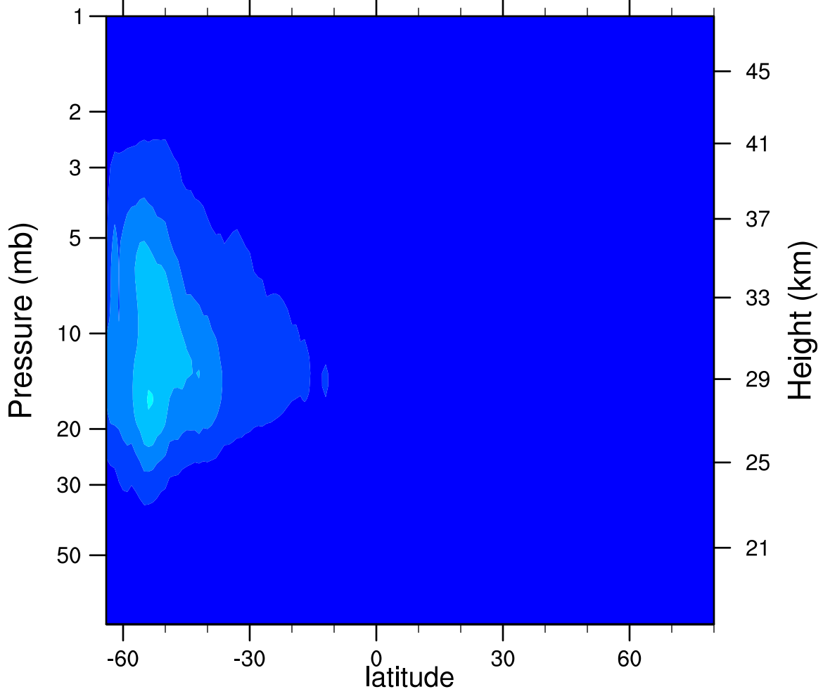
2007d195 N2O5_Ascending (ppbv)
