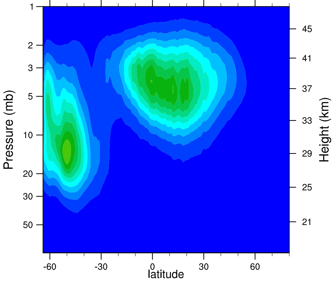
2005d169 N2O5_Ascending (ppbv)
