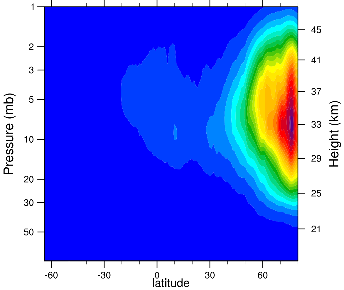
2005d334 N2O5_Ascending (ppbv)
