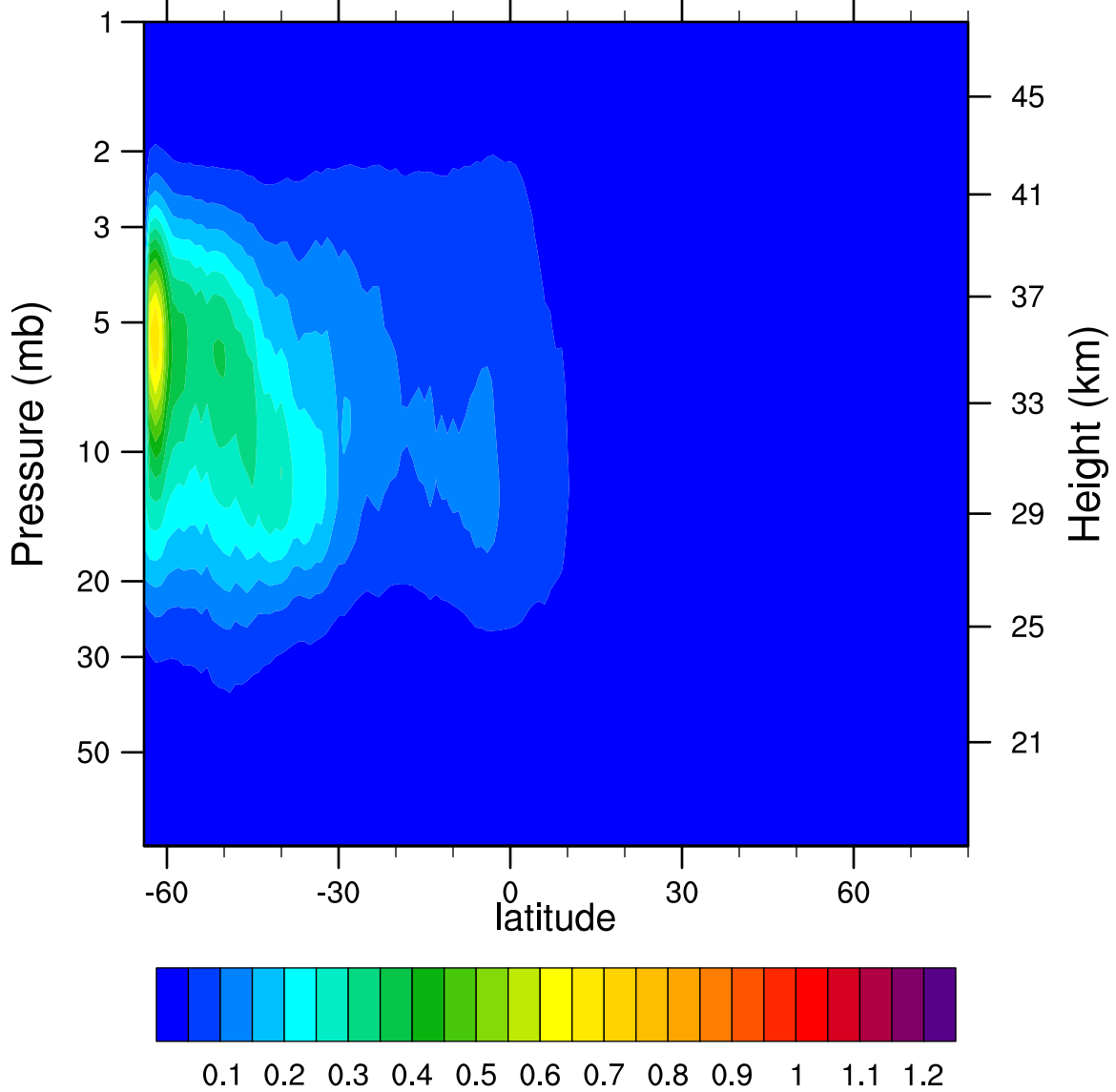
2006d173 N2O5_Ascending (ppbv)
