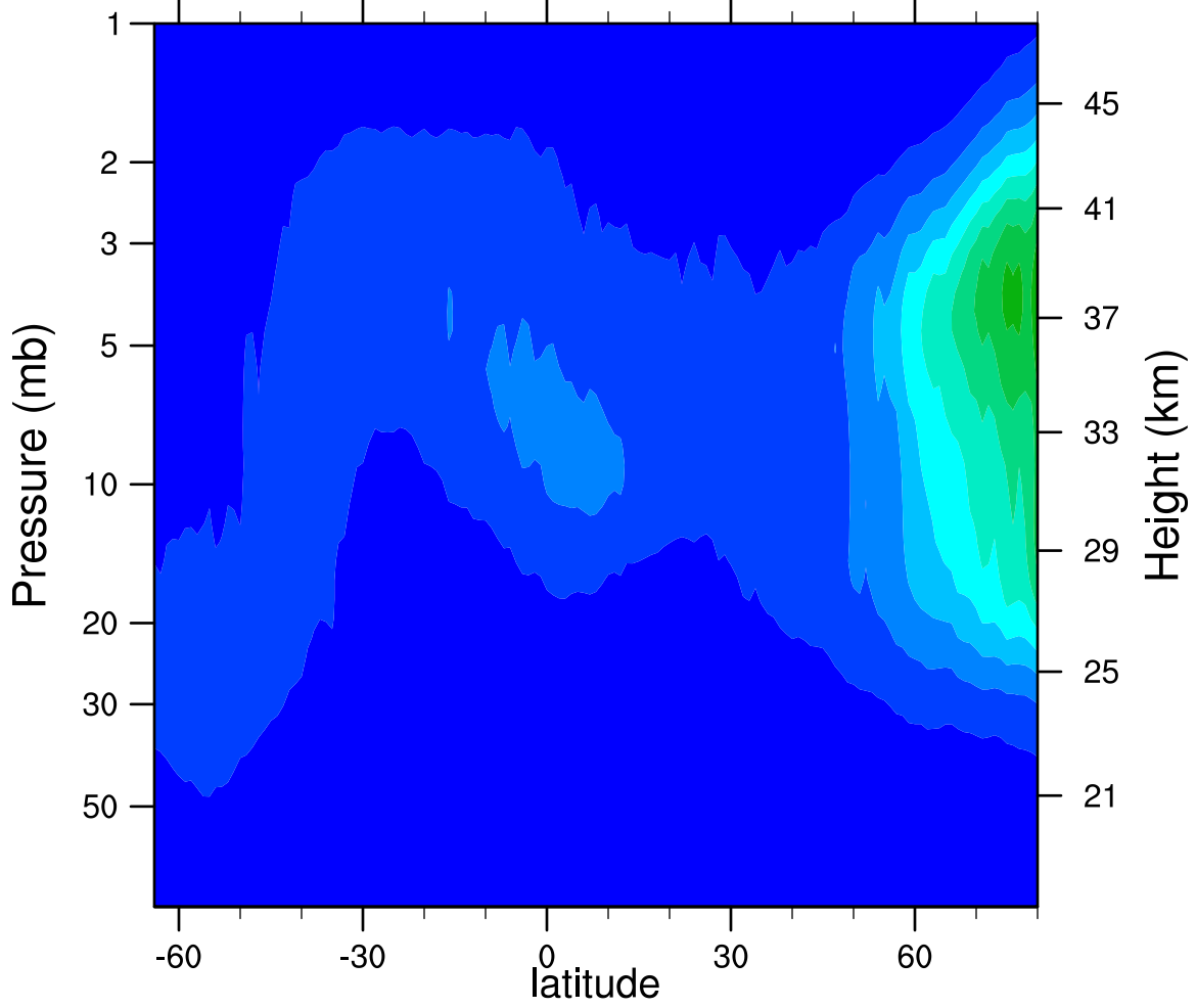
2006d062 N2O5_Ascending (ppbv)
