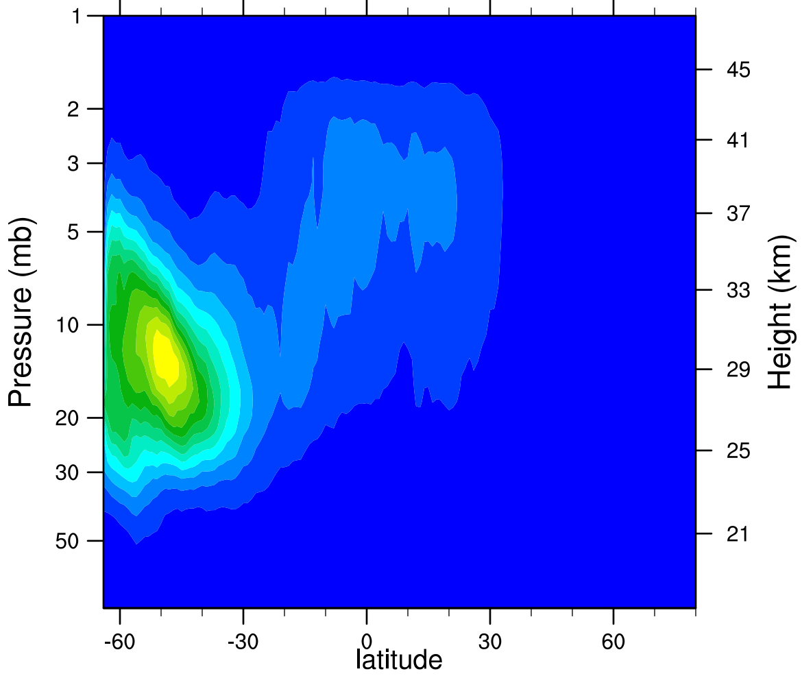
2007d219 N2O5_Ascending (ppbv)
