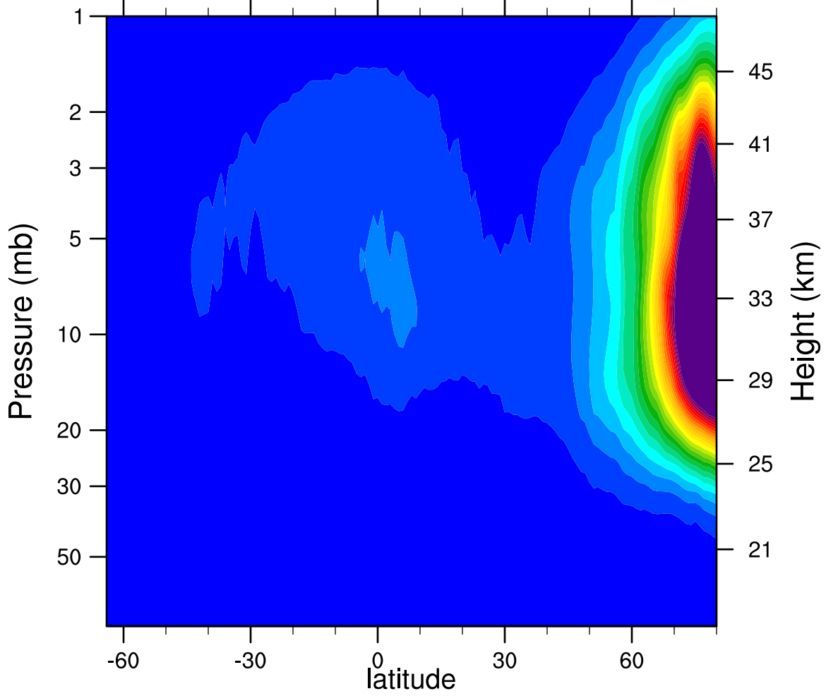
2006d032 N2O5_Ascending (ppbv)
