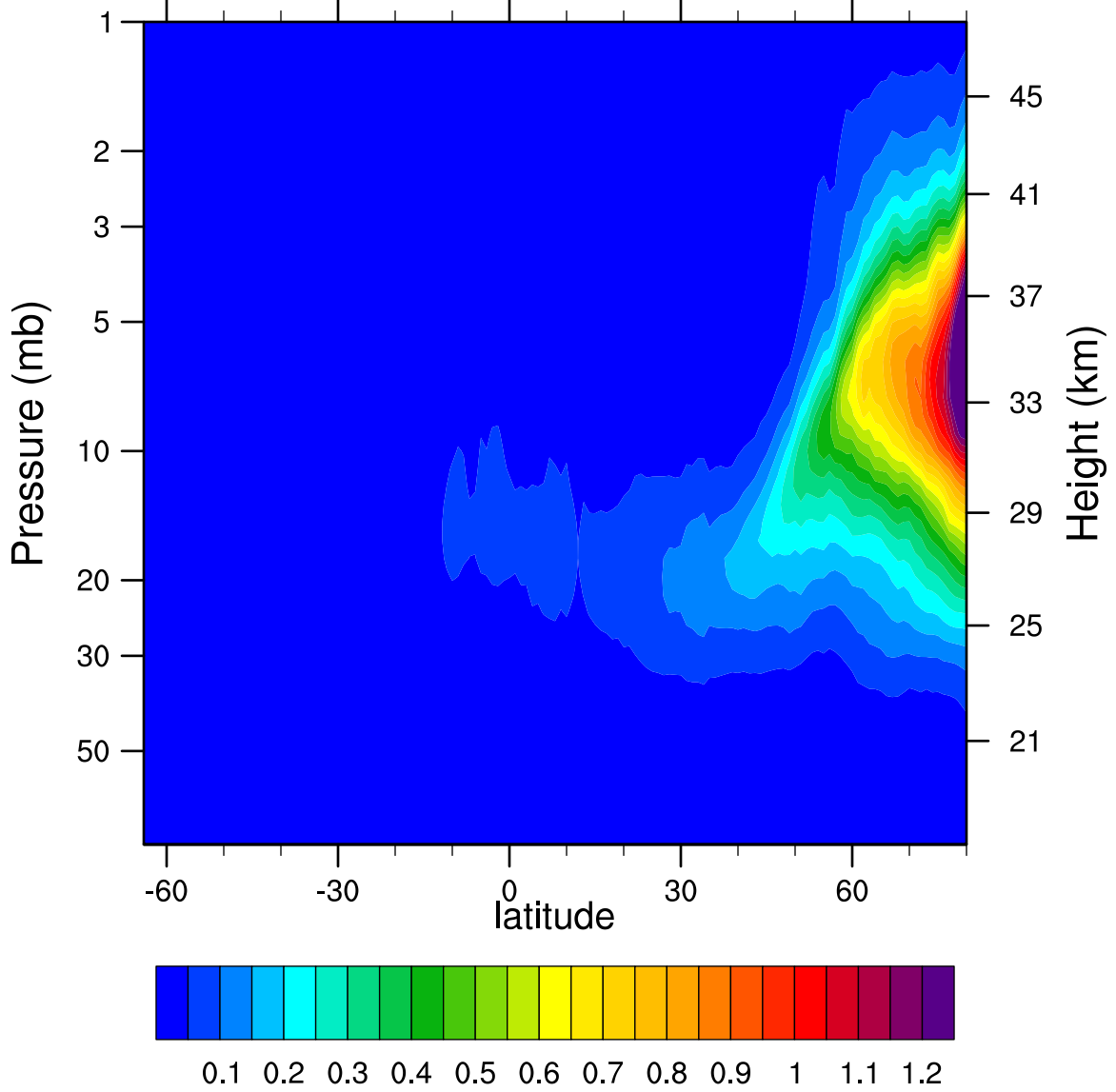
2007d035 N2O5_Ascending (ppbv)
