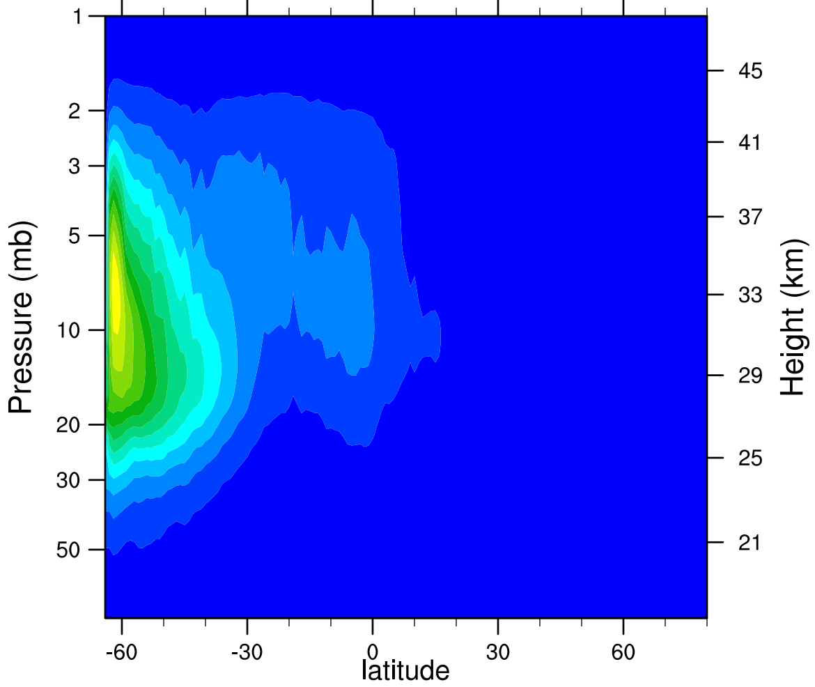
2006d130 N2O5_Ascending (ppbv)
