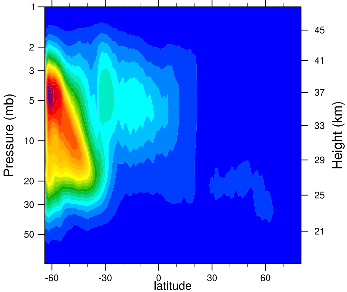
2007d133 N2O5_Ascending (ppbv)
