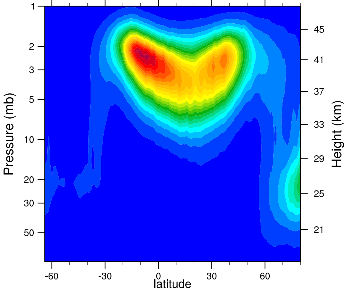
2005d065 N2O5_Ascending (ppbv)
