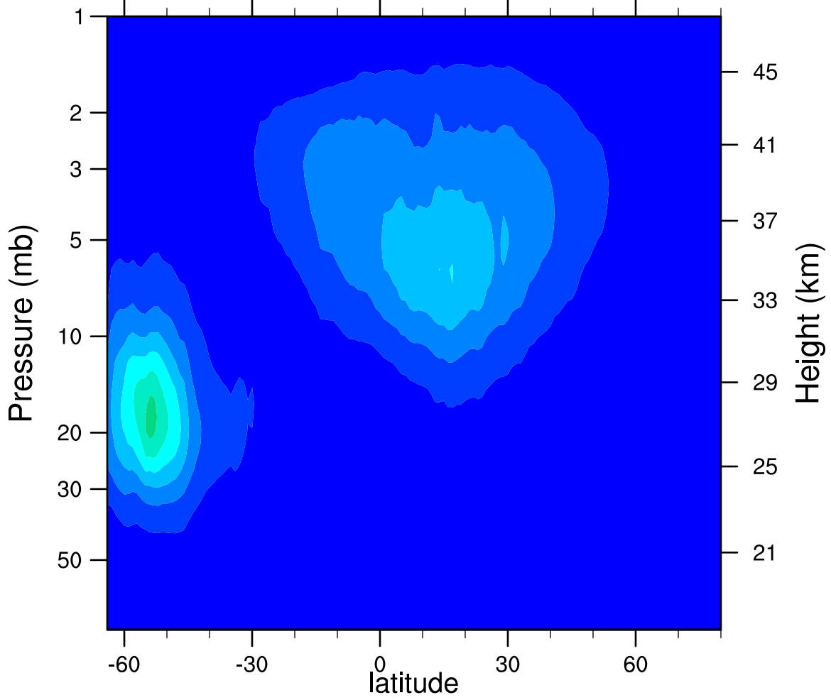
2005d235 N2O5_Ascending (ppbv)
