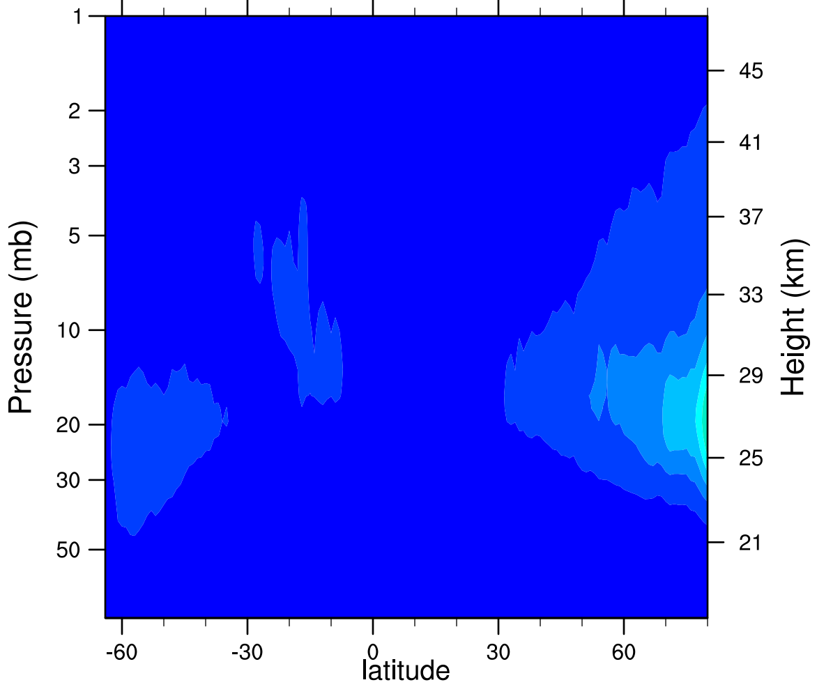
2006d276 N2O5_Ascending (ppbv)
