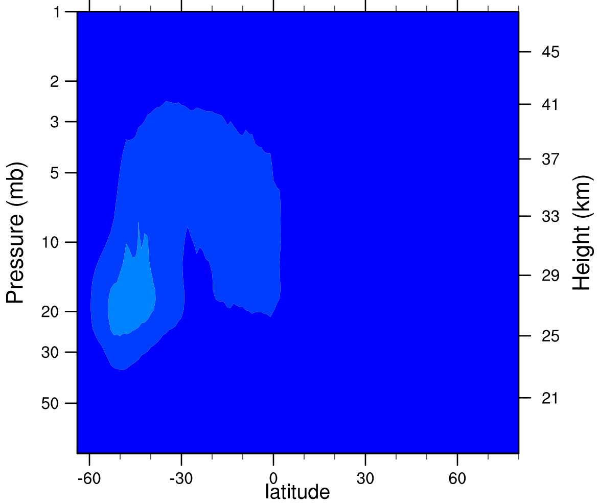
2006d240 N2O5_Ascending (ppbv)
