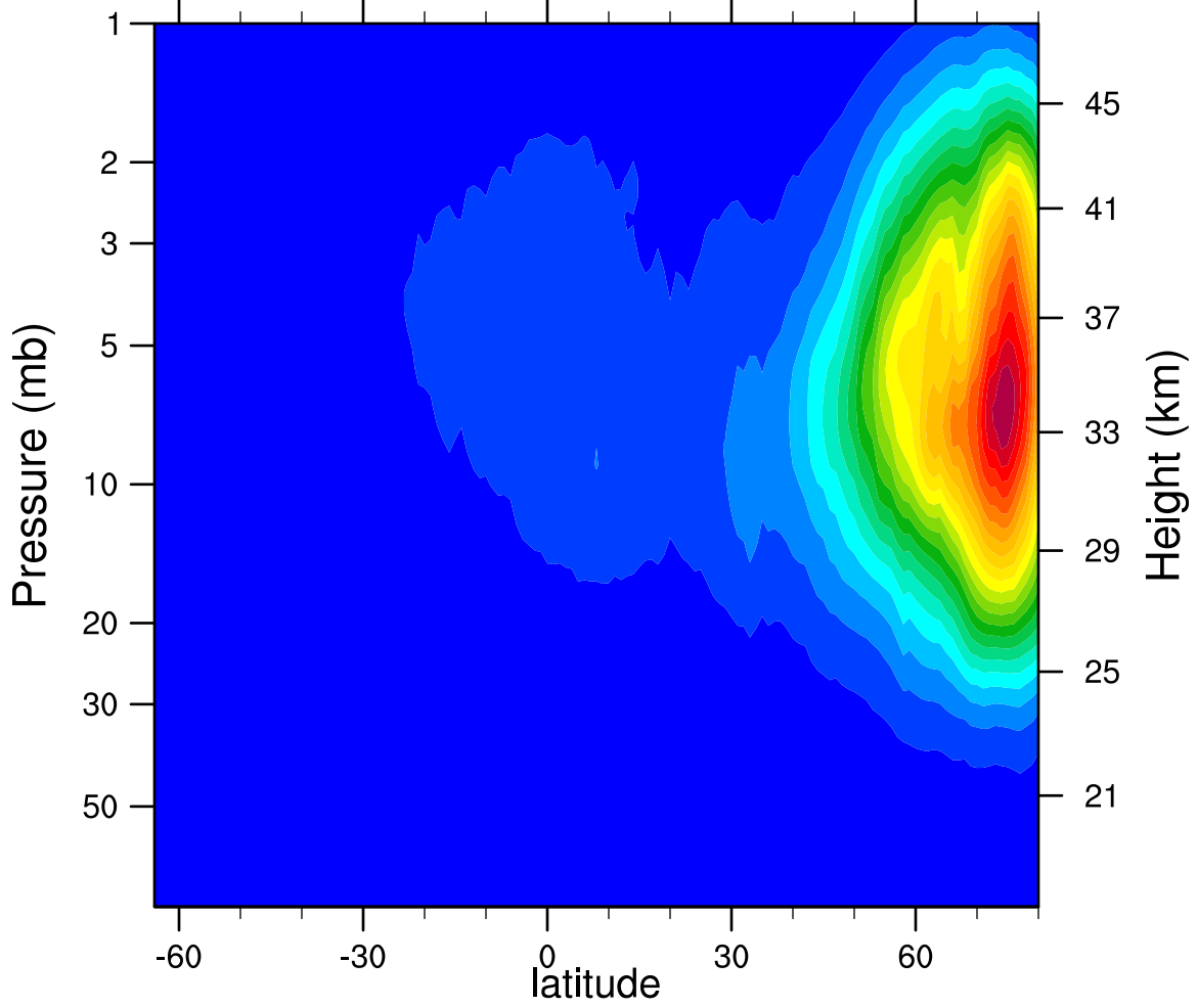
2005d341 N2O5_Ascending (ppbv)
