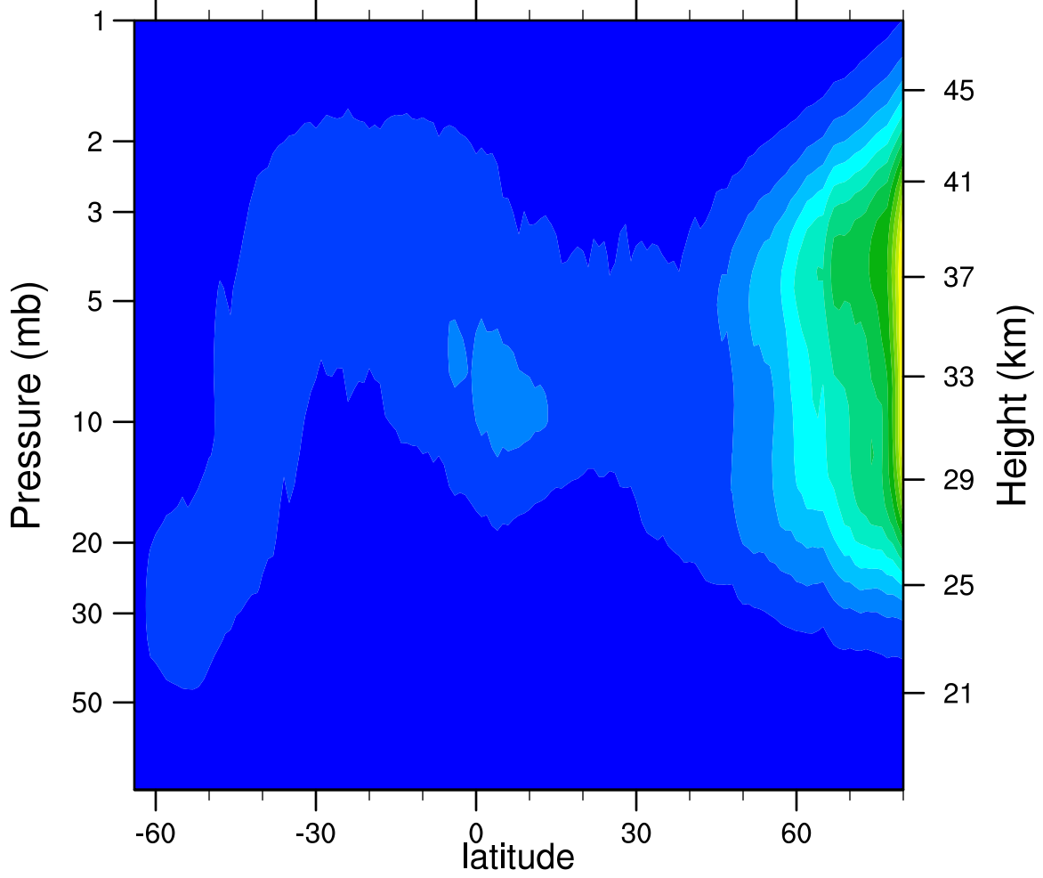
2006d057 N2O5_Ascending (ppbv)
