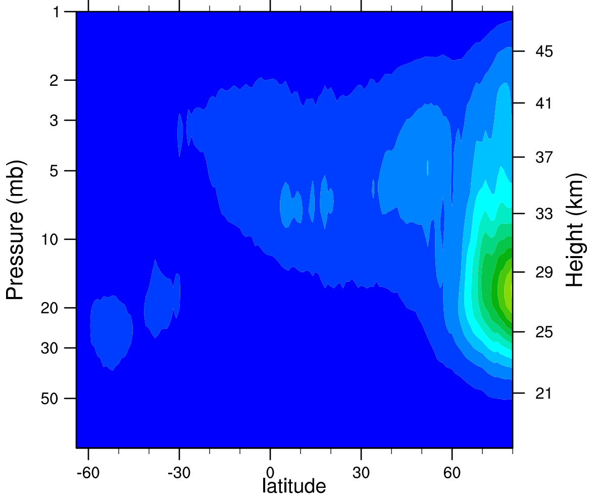
2005d290 N2O5_Ascending (ppbv)
