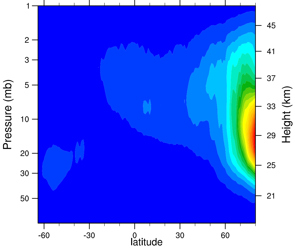
2005d299 N2O5_Ascending (ppbv)
