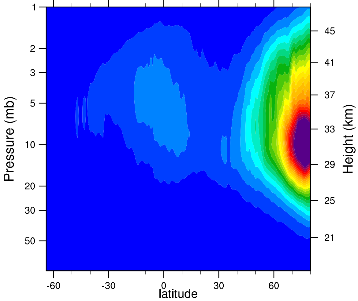
2006d013 N2O5_Ascending (ppbv)
