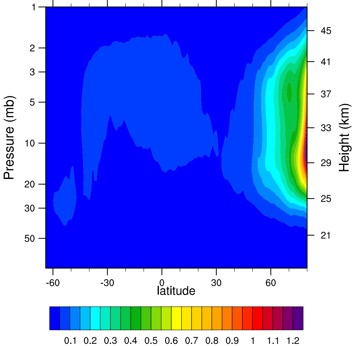
2006d049 N2O5_Ascending (ppbv)
