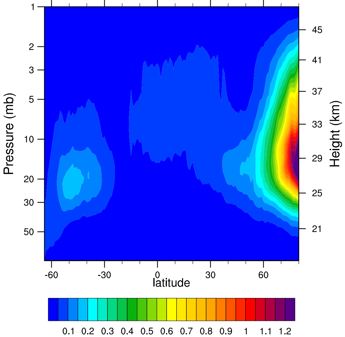
2007d301 N2O5_Ascending (ppbv)
