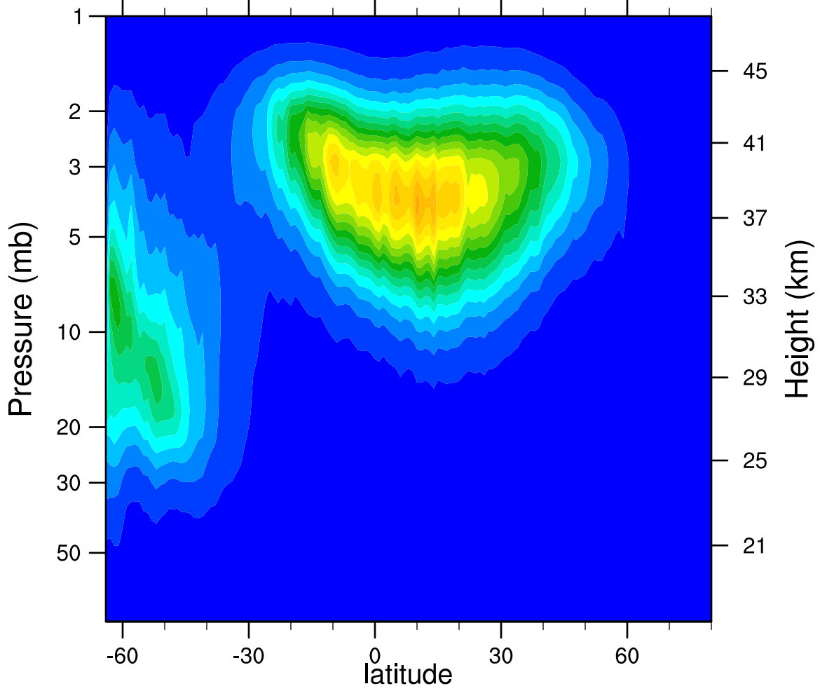
2005d118 N2O5_Ascending (ppbv)
