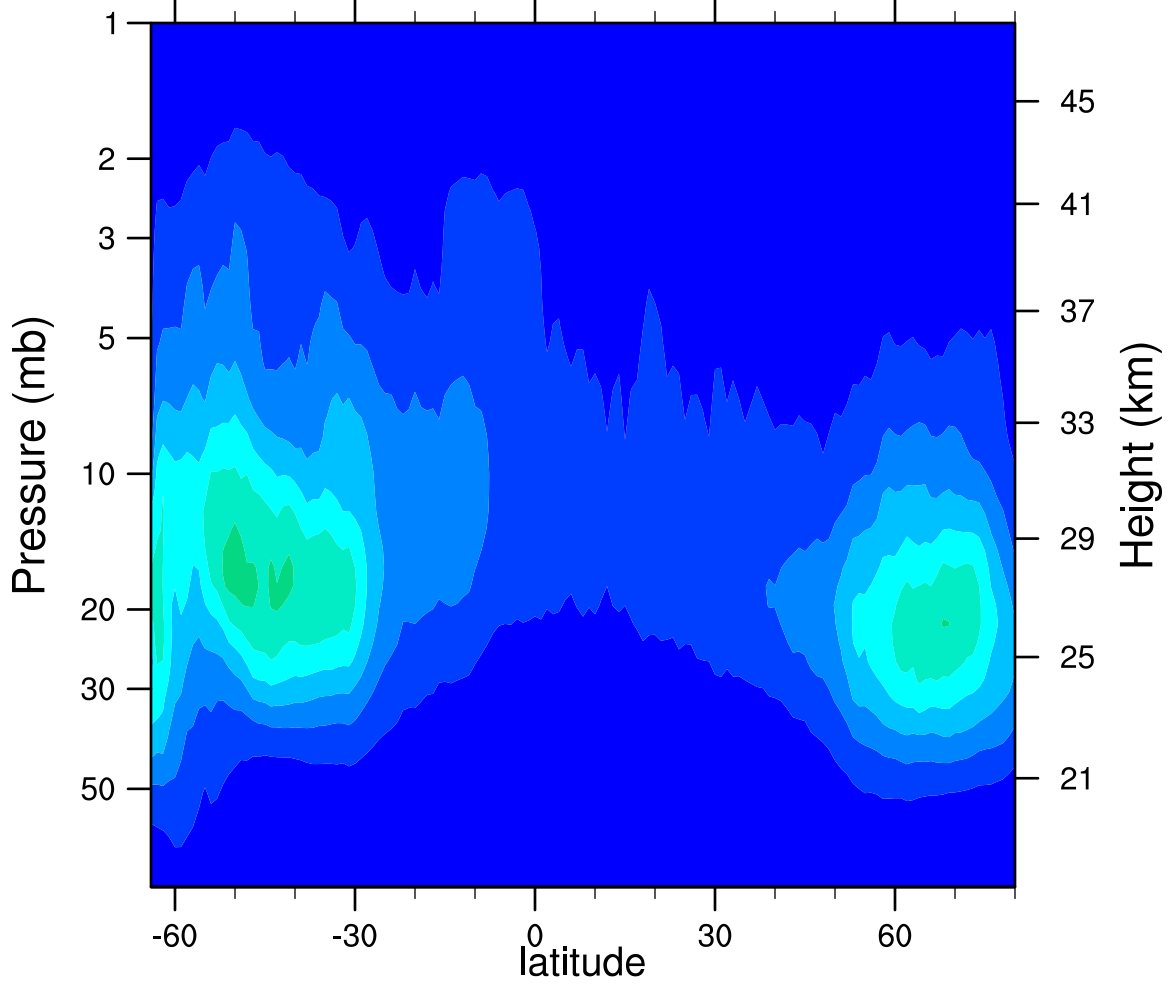
2007d260 N2O5_Ascending (ppbv)
