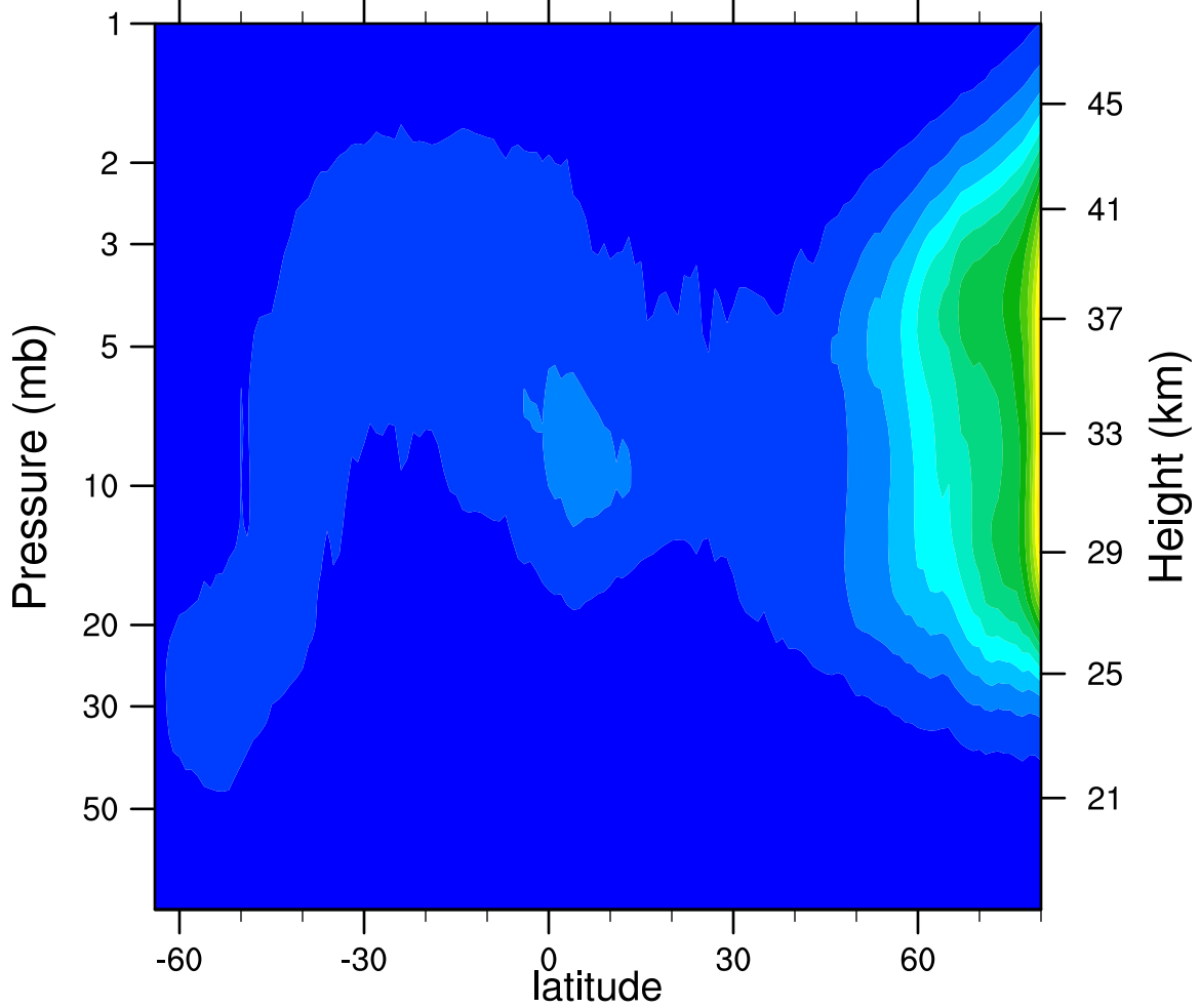
2006d056 N2O5_Ascending (ppbv)
