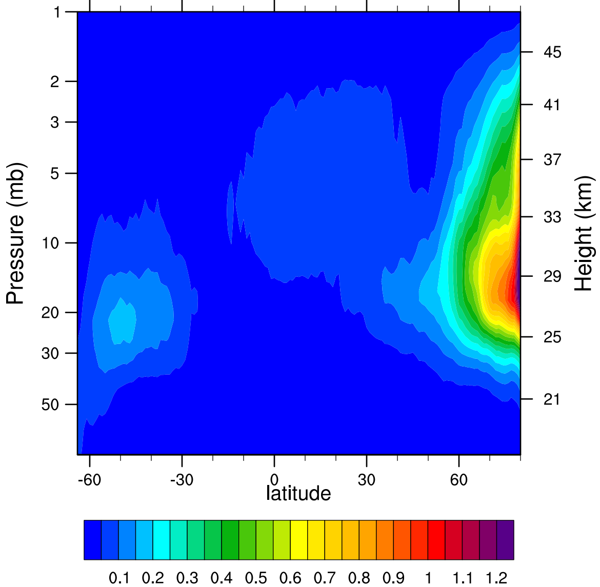
2007d306 N2O5_Ascending (ppbv)
