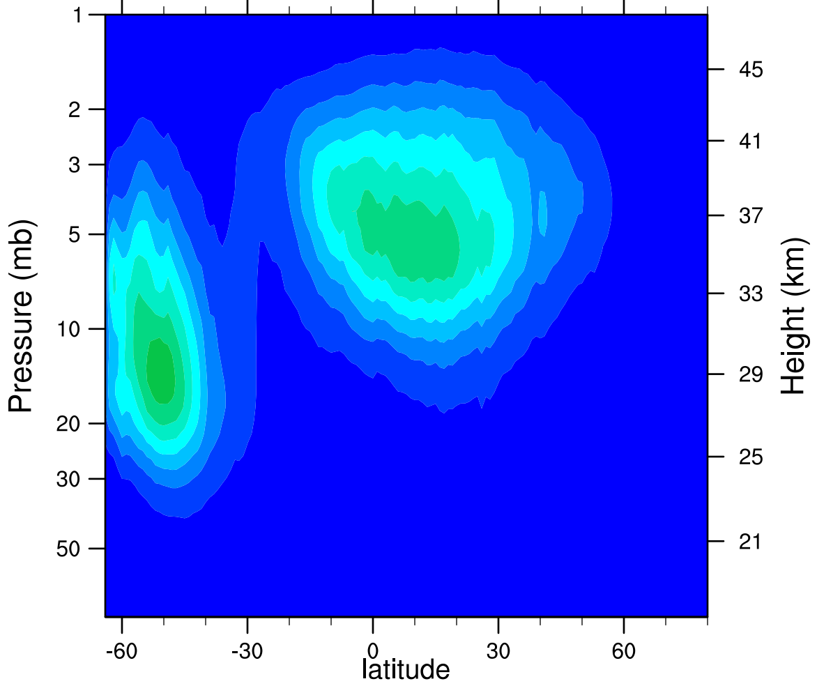
2005d201 N2O5_Ascending (ppbv)
