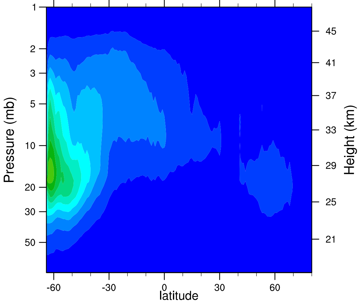
2006d108 N2O5_Ascending (ppbv)
