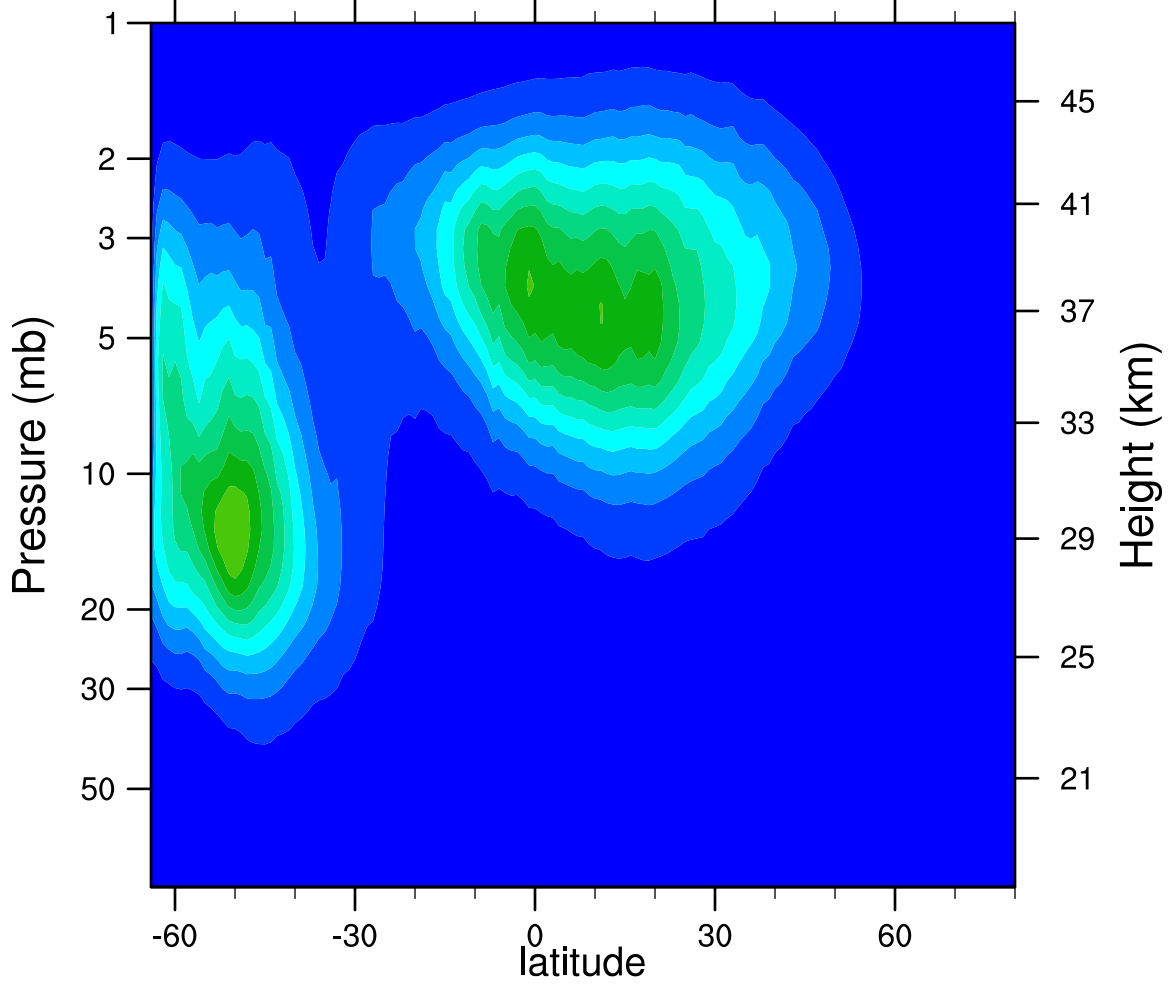
2005d167 N2O5_Ascending (ppbv)
