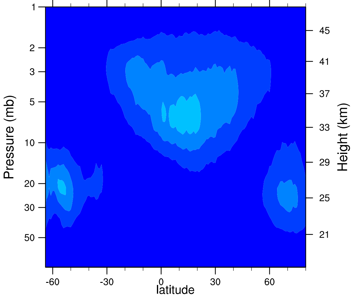
2005d262 N2O5_Ascending (ppbv)
