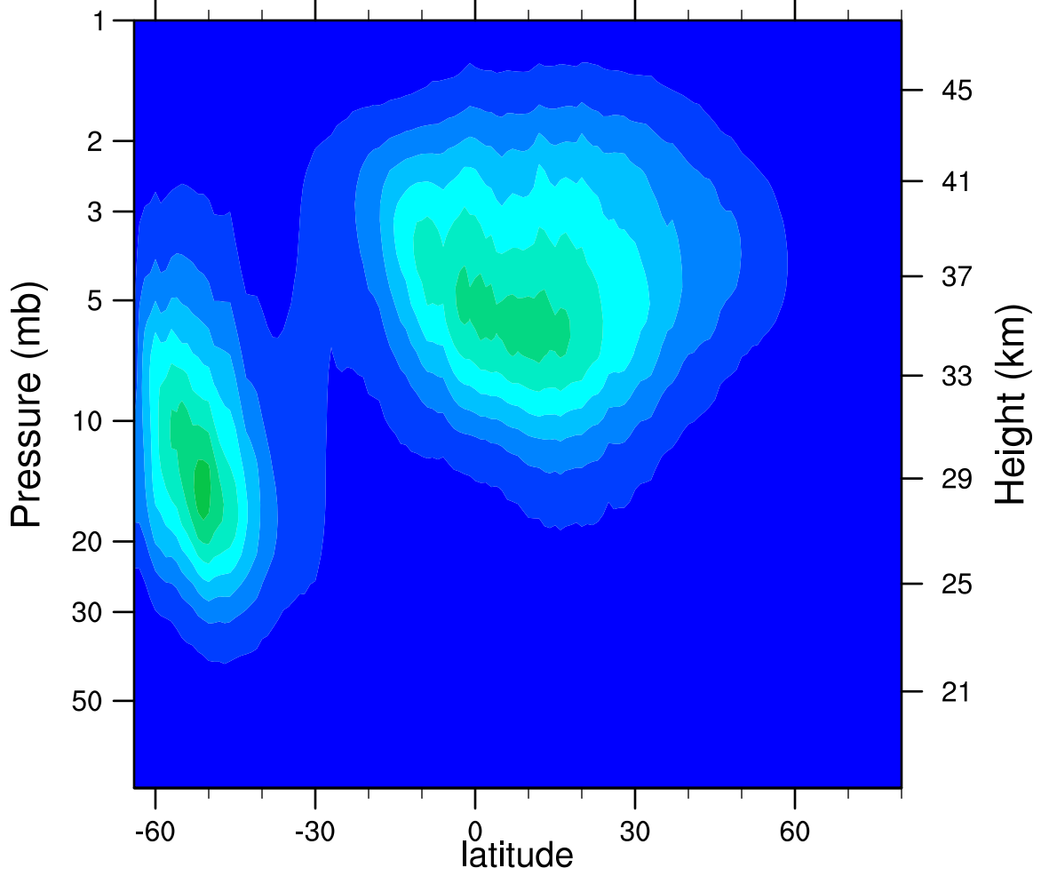
2005d212 N2O5_Ascending (ppbv)
