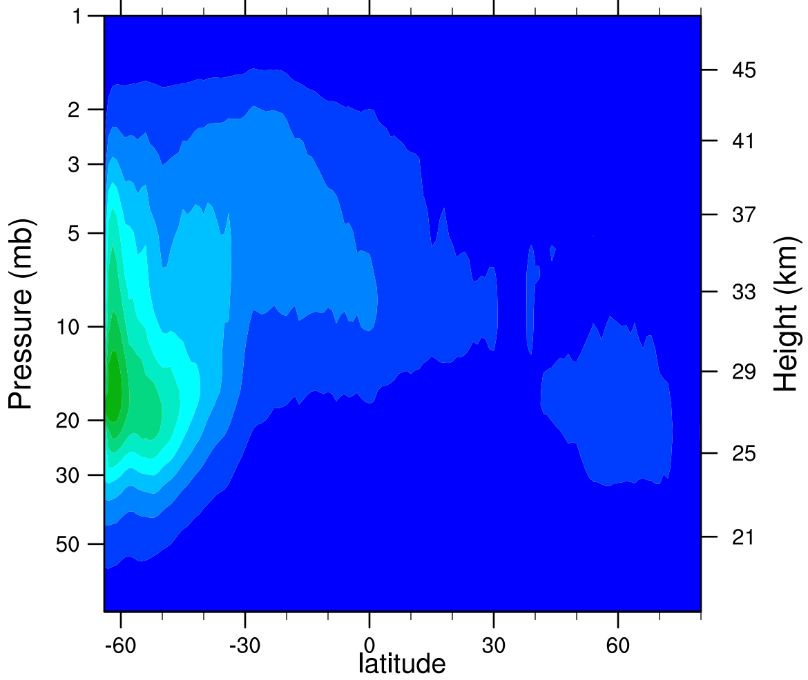
2006d106 N2O5_Ascending (ppbv)
