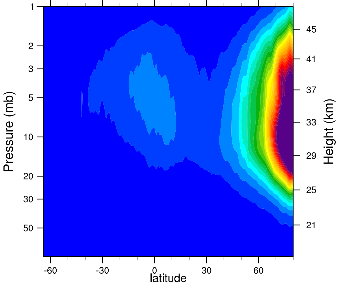
2006d017 N2O5_Ascending (ppbv)
