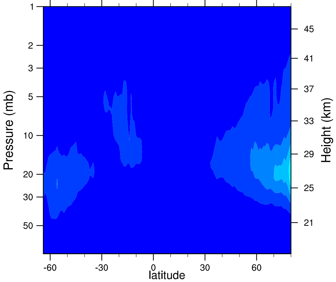
2006d274 N2O5_Ascending (ppbv)
