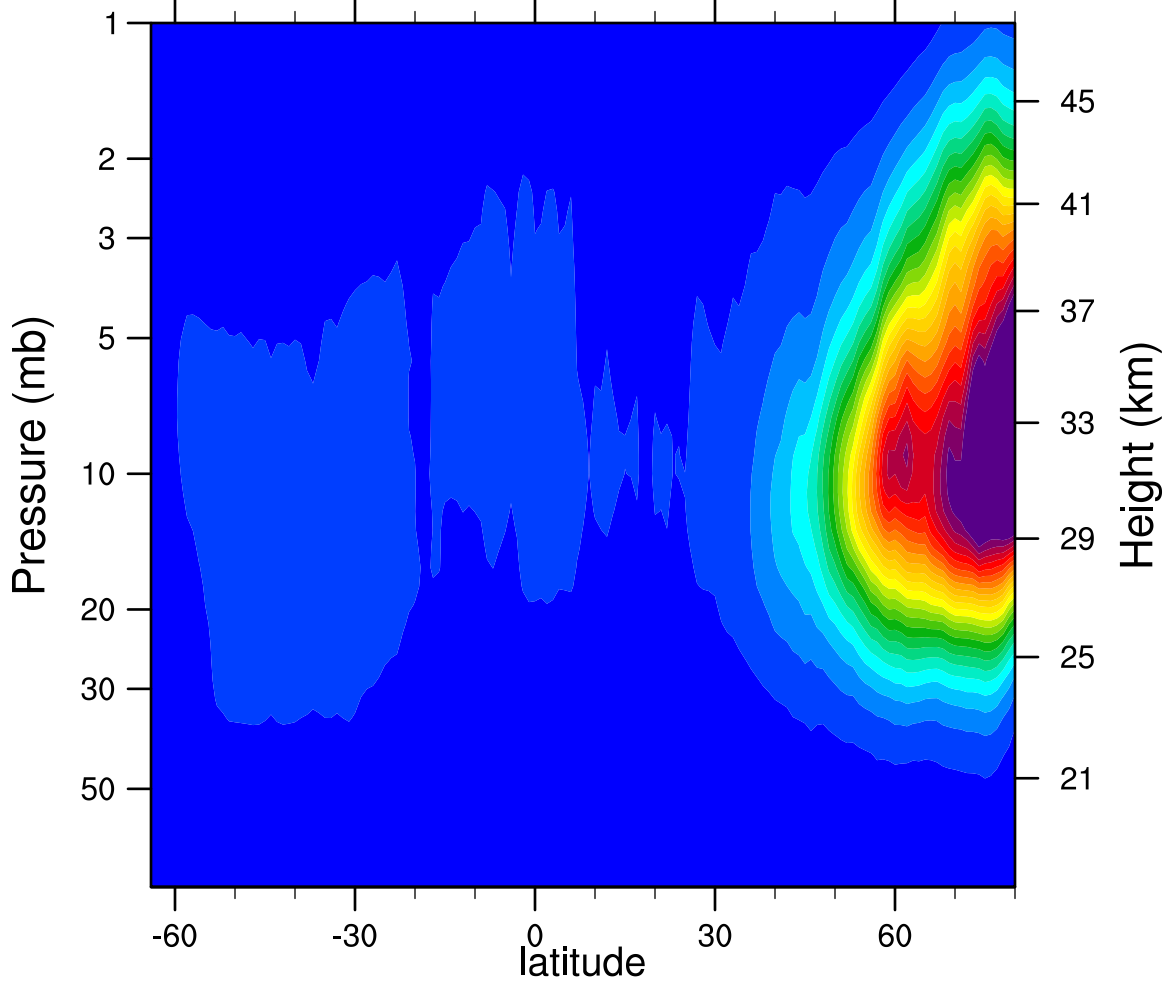
2007d360 N2O5_Ascending (ppbv)
