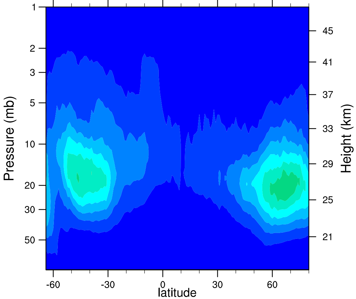
2007d264 N2O5_Ascending (ppbv)
