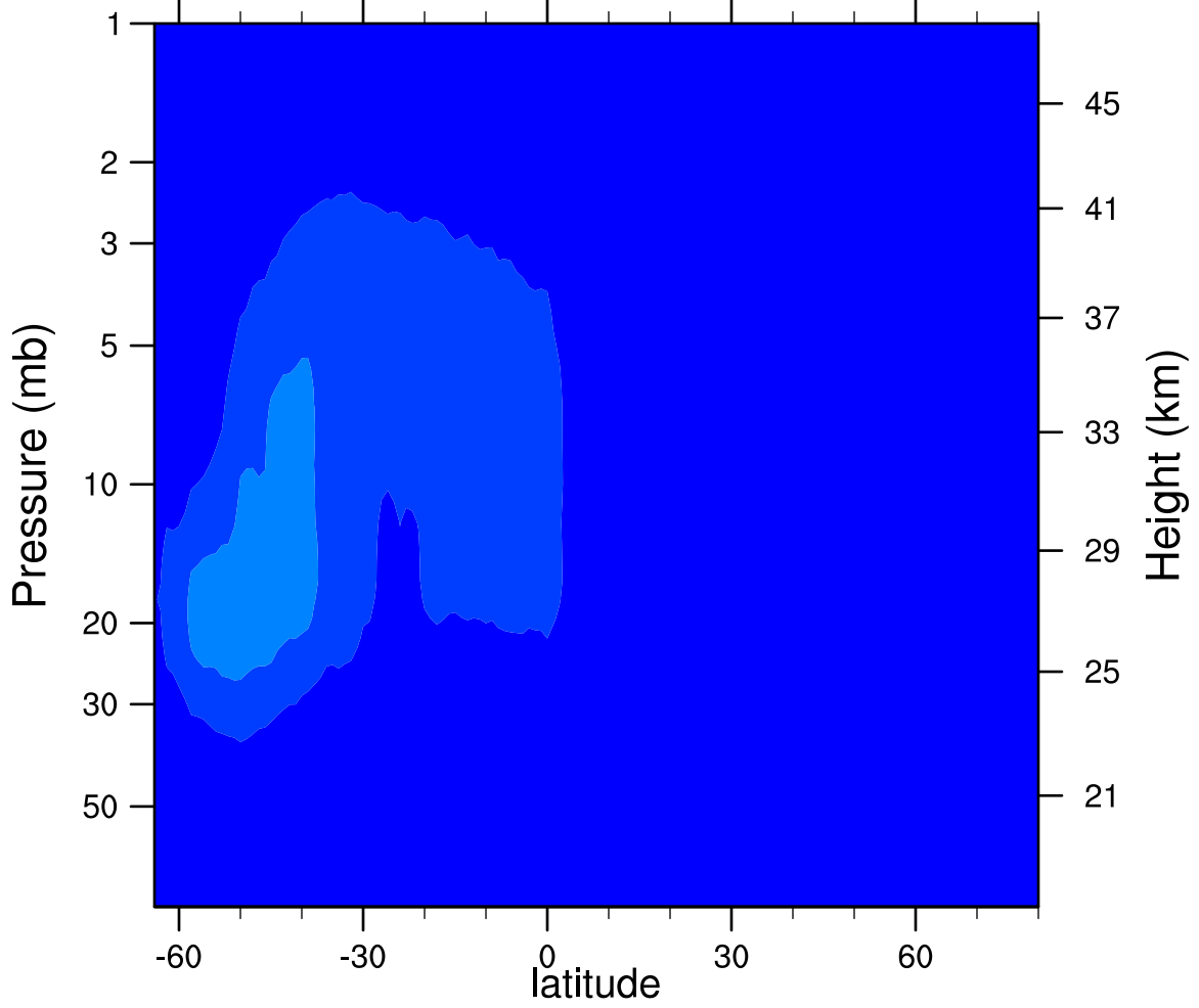
2006d235 N2O5_Ascending (ppbv)
