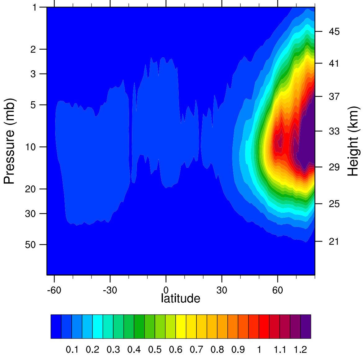
2007d359 N2O5_Ascending (ppbv)
