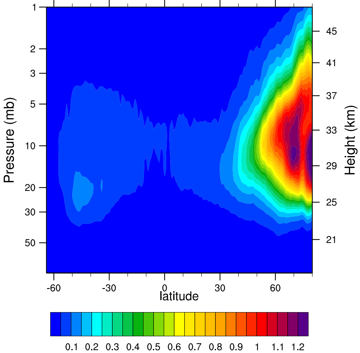
2006d346 N2O5_Ascending (ppbv)
