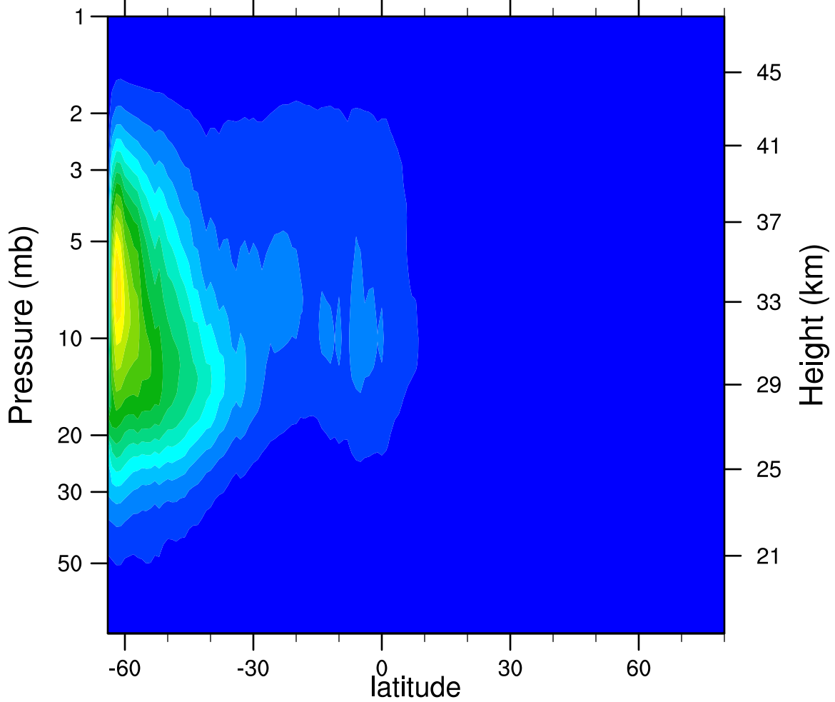
2006d137 N2O5_Ascending (ppbv)
