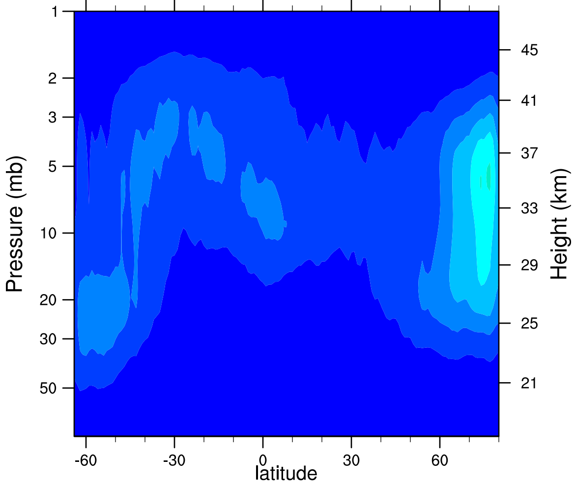
2006d074 N2O5_Ascending (ppbv)
