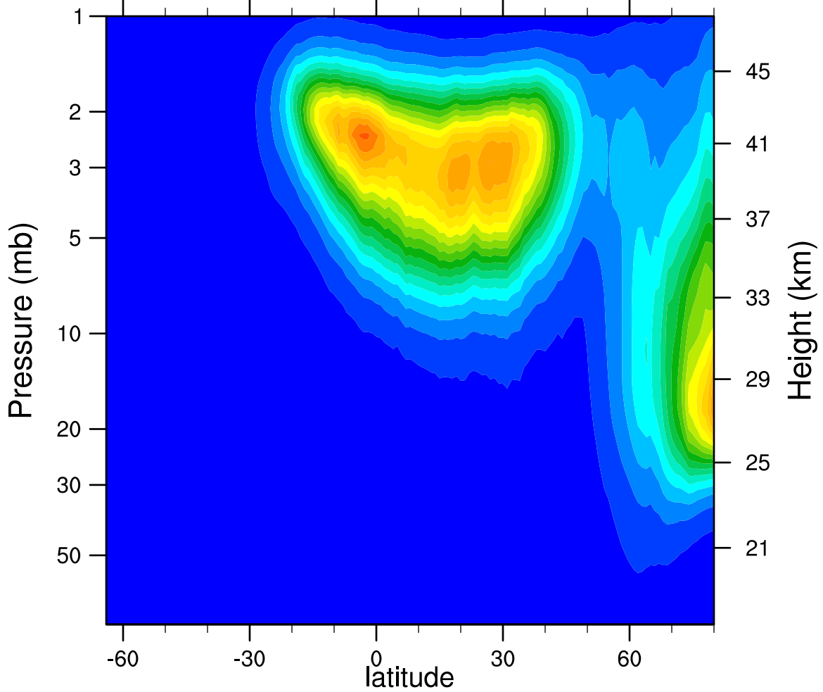
2005d034 N2O5_Ascending (ppbv)
