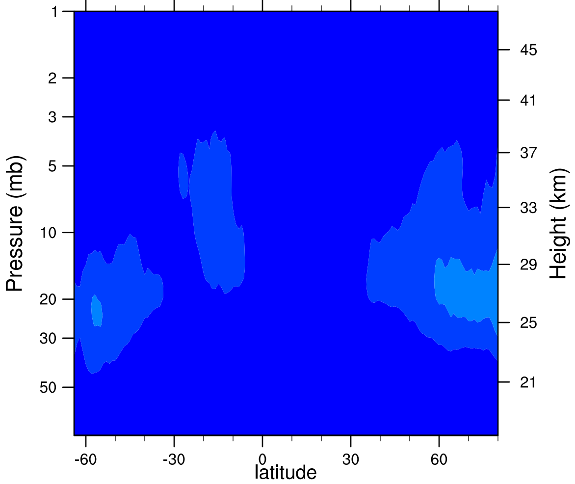
2006d271 N2O5_Ascending (ppbv)
