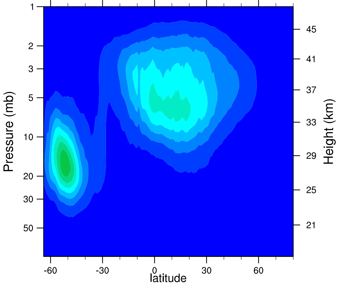
2005d220 N2O5_Ascending (ppbv)
