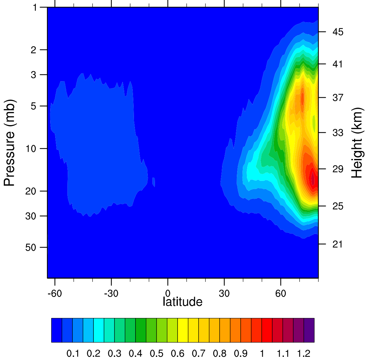
2006d310 N2O5_Ascending (ppbv)
