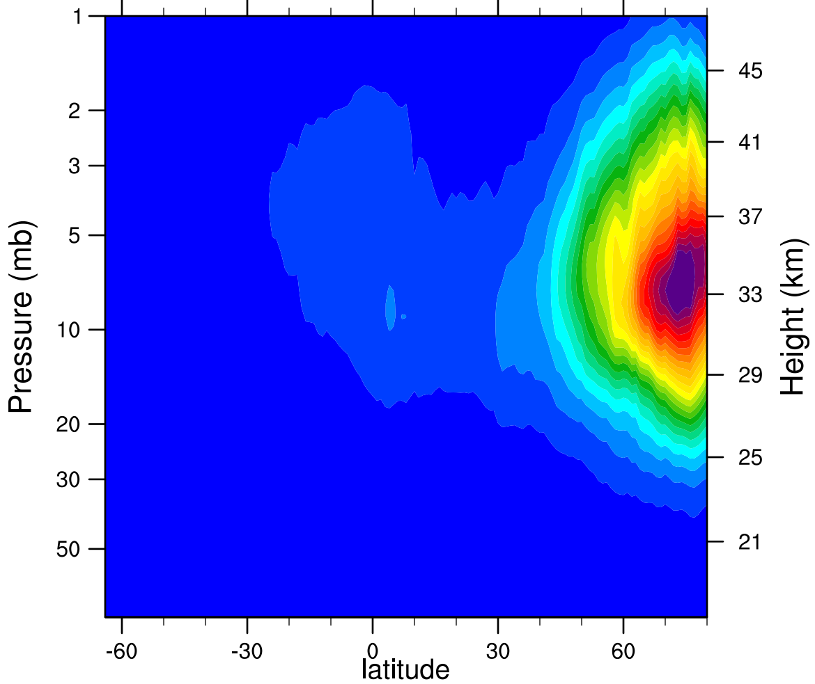
2005d353 N2O5_Ascending (ppbv)
