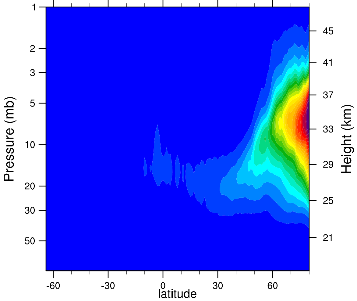
2007d038 N2O5_Ascending (ppbv)
