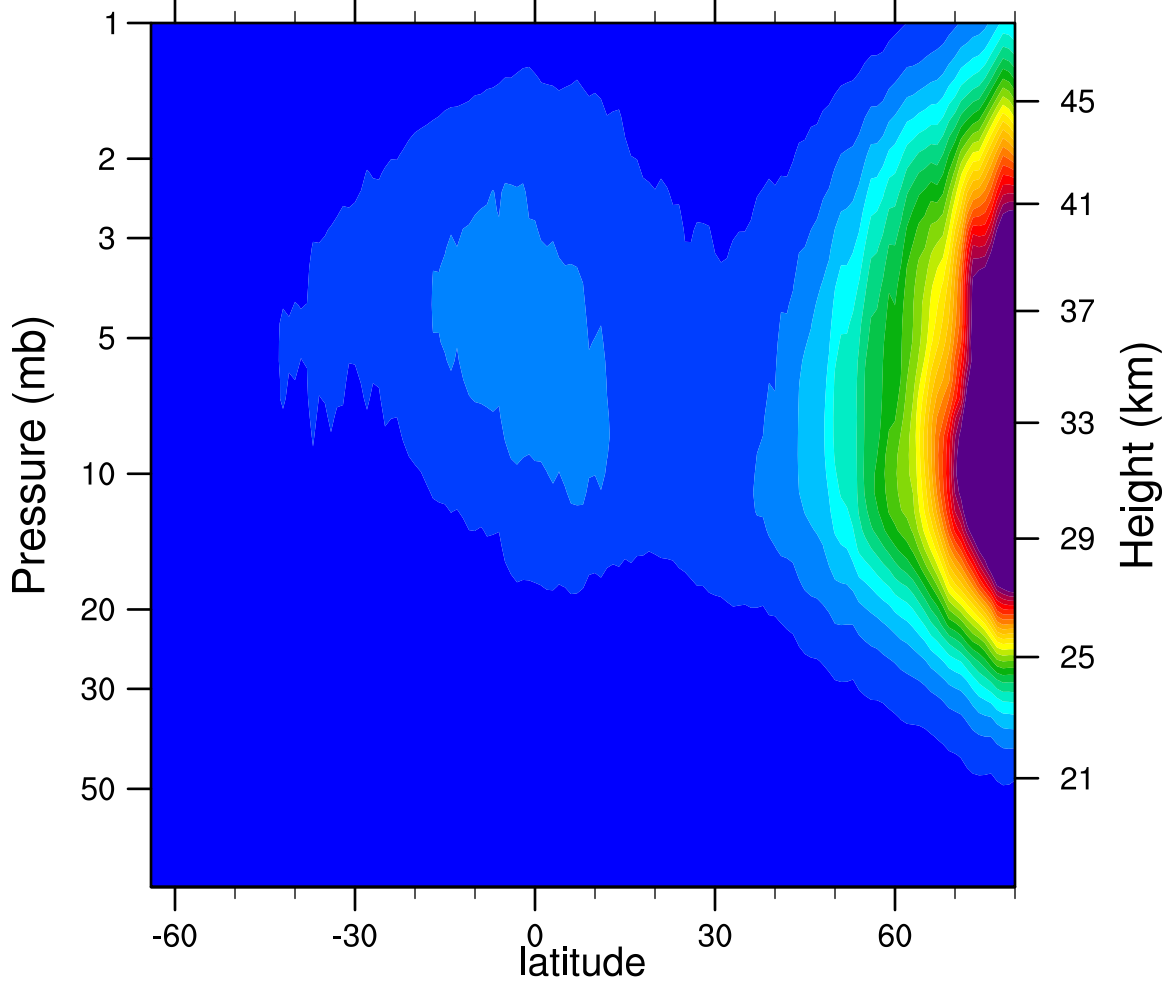
2006d016 N2O5_Ascending (ppbv)
