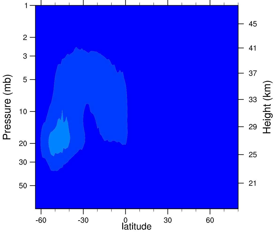
2006d243 N2O5_Ascending (ppbv)
