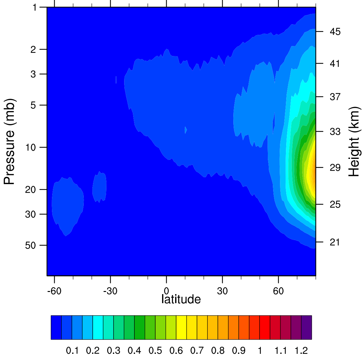
2005d295 N2O5_Ascending (ppbv)
