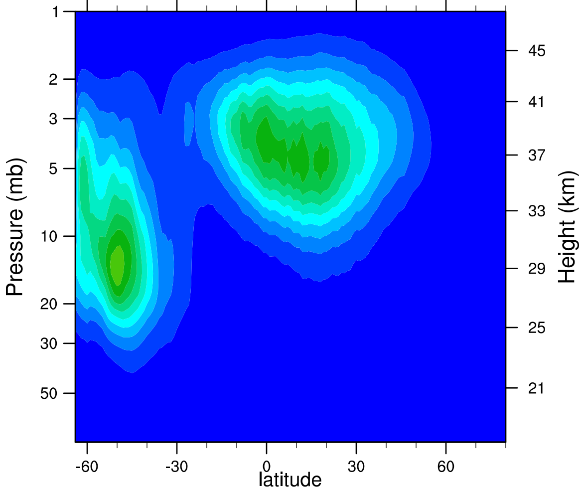
2005d170 N2O5_Ascending (ppbv)
