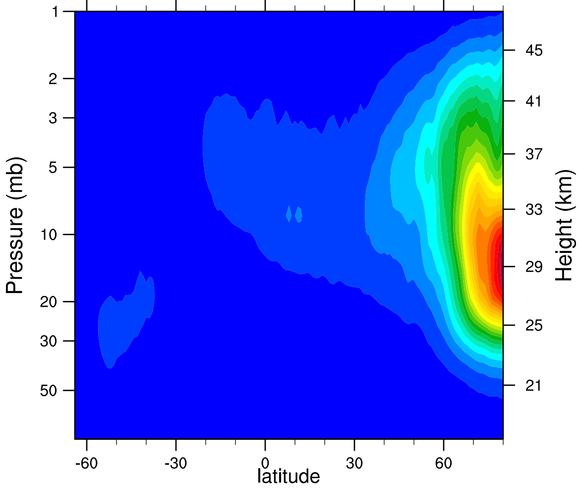
2005d306 N2O5_Ascending (ppbv)
