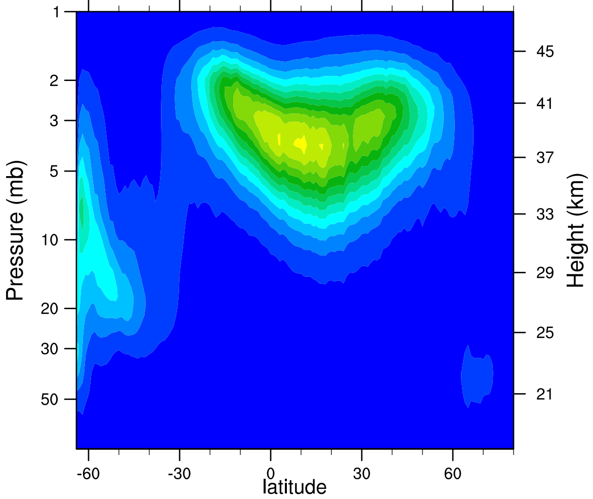
2005d102 N2O5_Ascending (ppbv)
