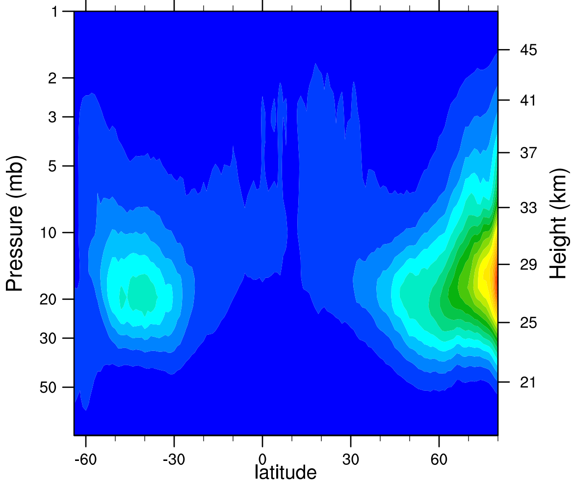
2007d282 N2O5_Ascending (ppbv)
