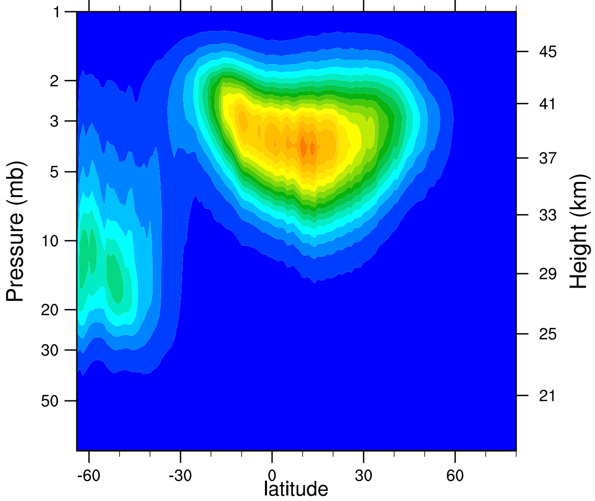
2005d120 N2O5_Ascending (ppbv)
