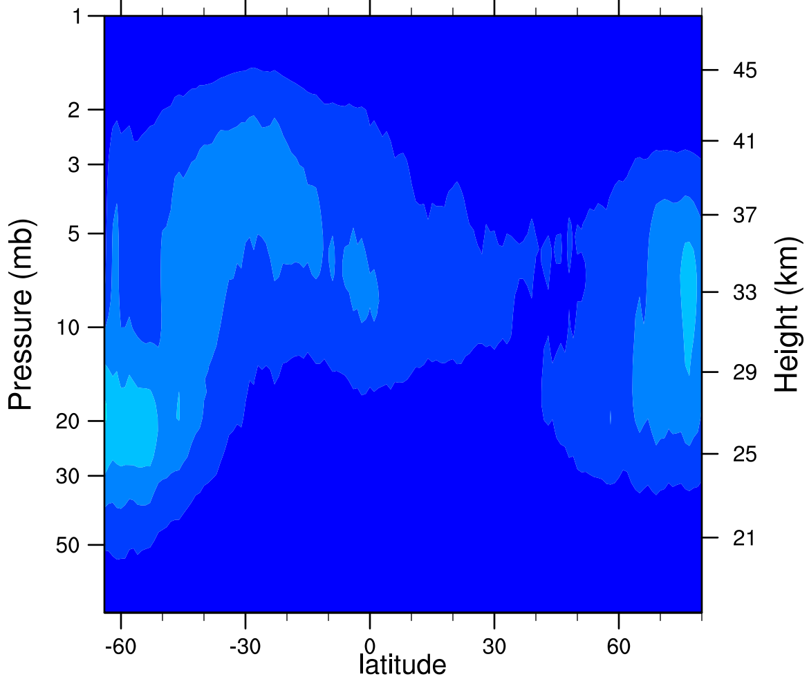
2006d085 N2O5_Ascending (ppbv)
