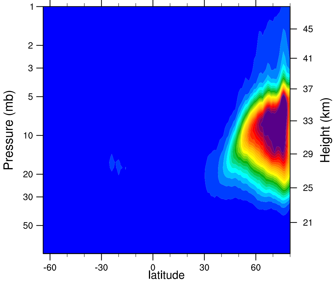
2006d361 N2O5_Ascending (ppbv)
