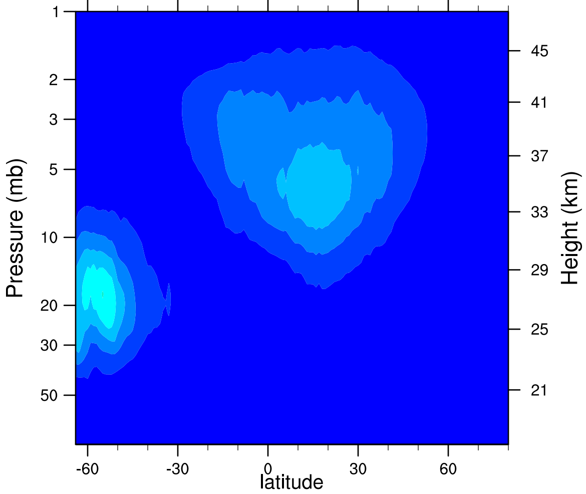
2005d243 N2O5_Ascending (ppbv)
