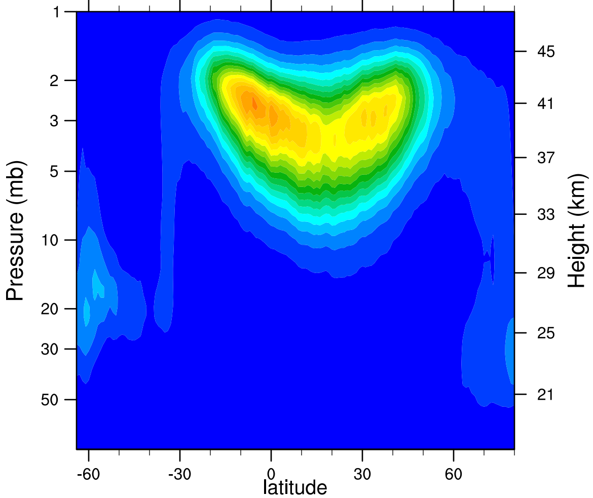
2005d079 N2O5_Ascending (ppbv)
