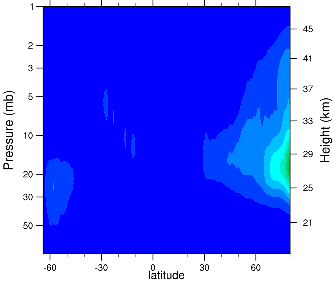
2006d284 N2O5_Ascending (ppbv)
