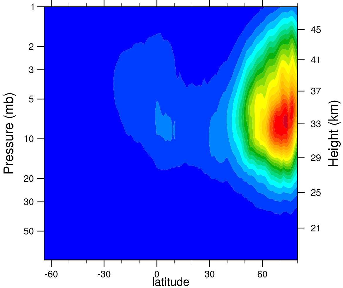
2005d359 N2O5_Ascending (ppbv)
