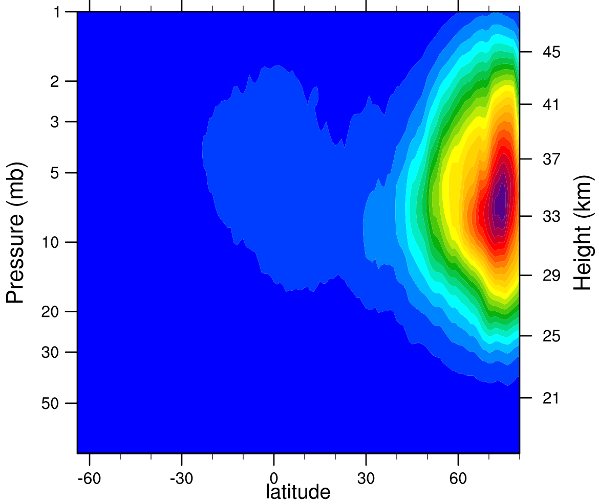
2005d344 N2O5_Ascending (ppbv)
