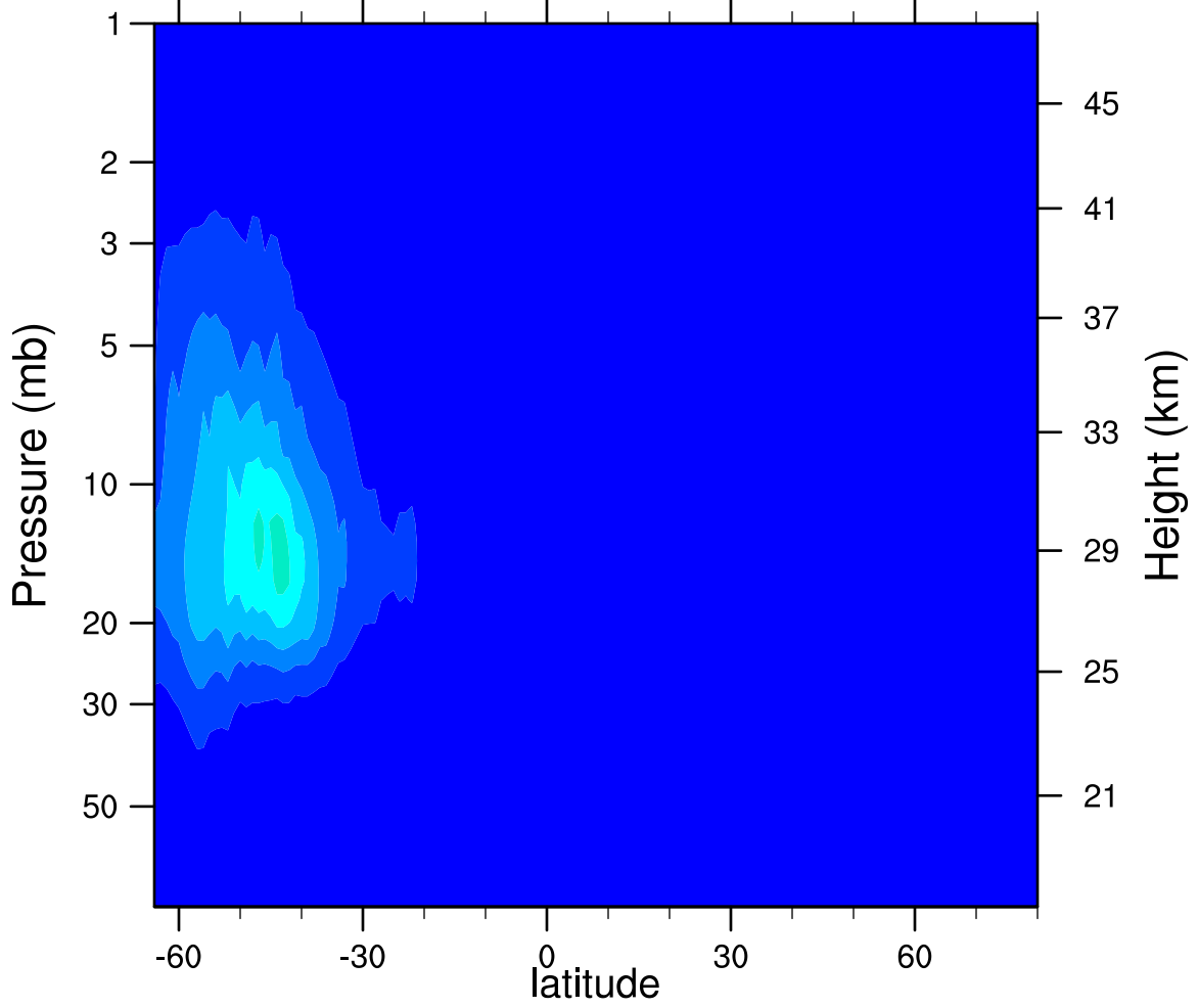
2007d208 N2O5_Ascending (ppbv)
