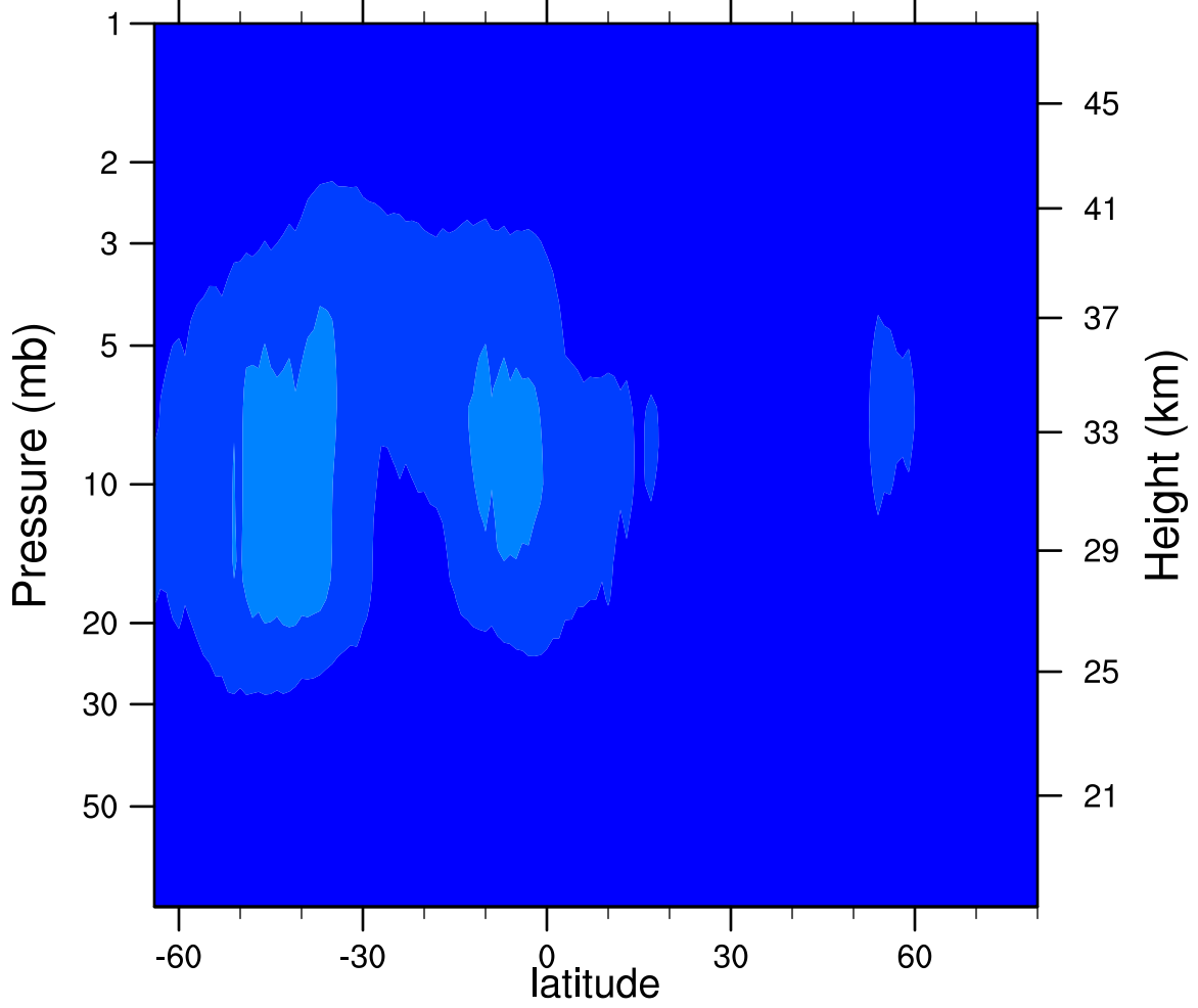
2006d218 N2O5_Ascending (ppbv)
