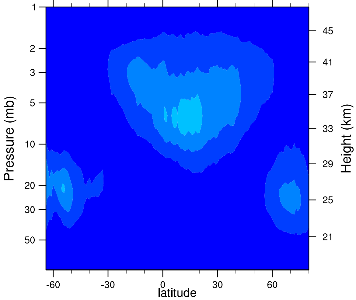
2005d263 N2O5_Ascending (ppbv)
