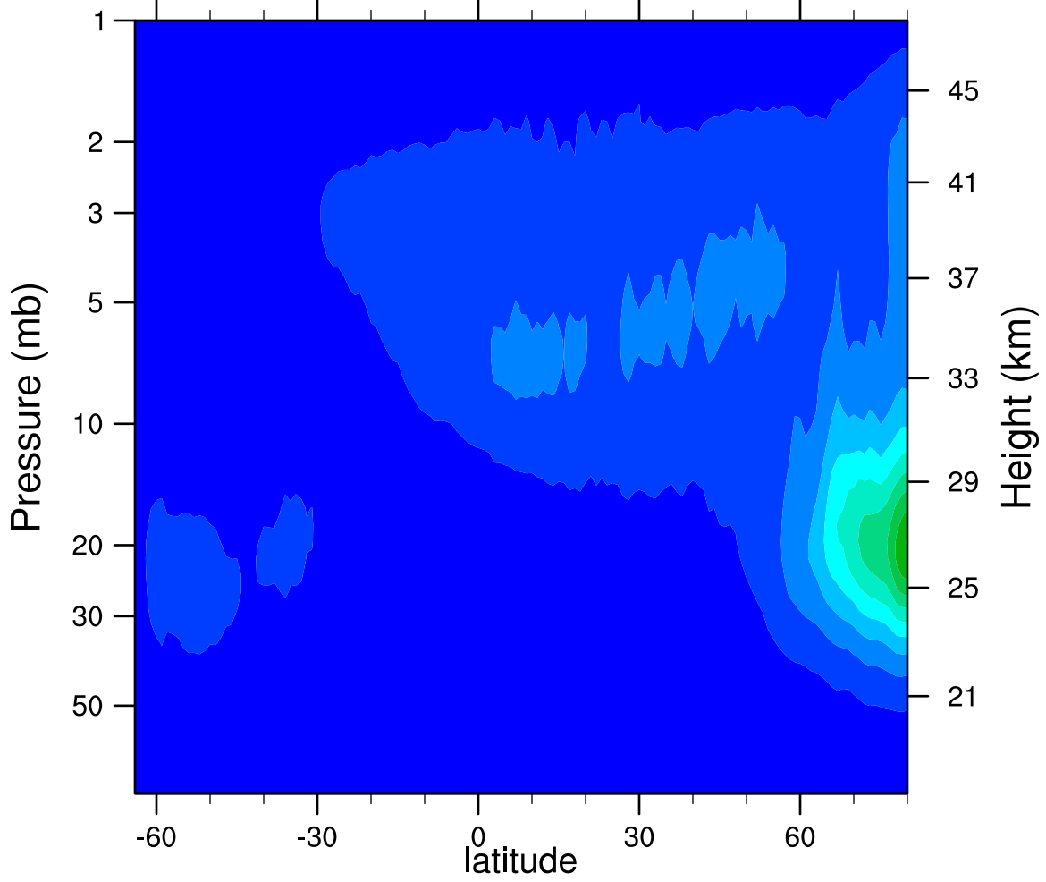
2005d285 N2O5_Ascending (ppbv)
