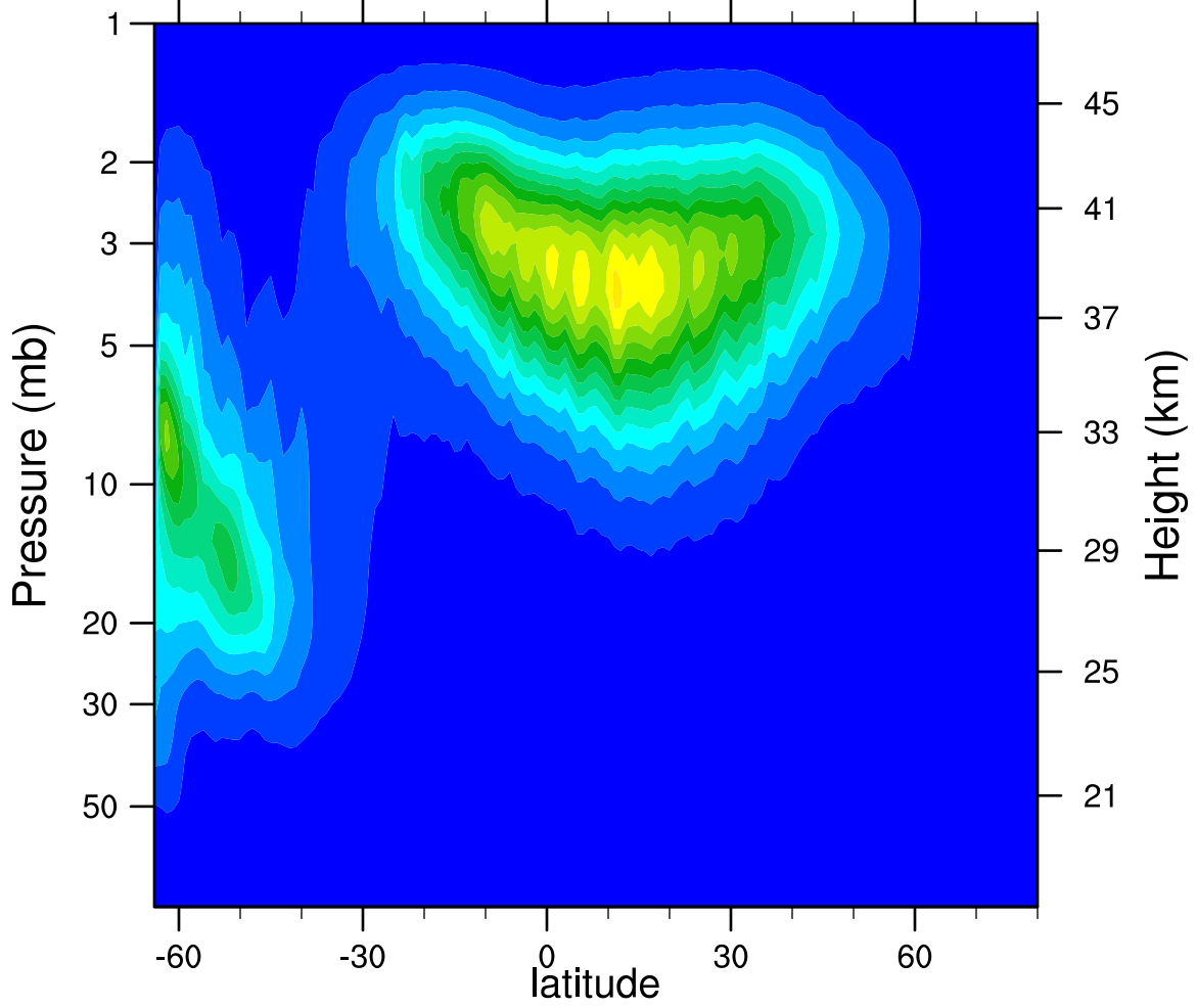
2005d116 N2O5_Ascending (ppbv)
