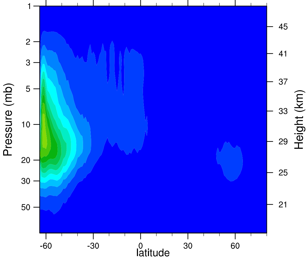
2006d117 N2O5_Ascending (ppbv)
