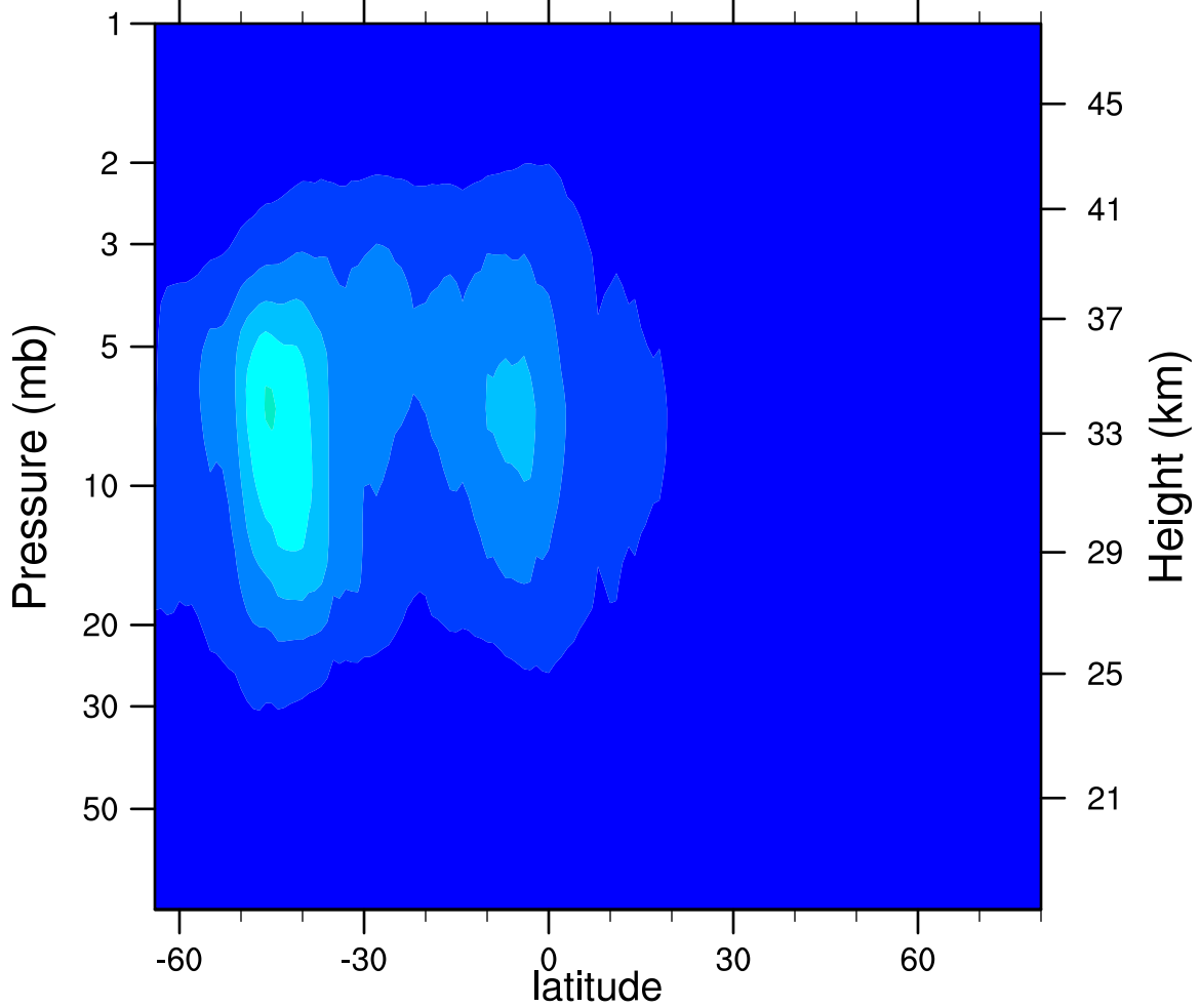
2006d199 N2O5_Ascending (ppbv)
