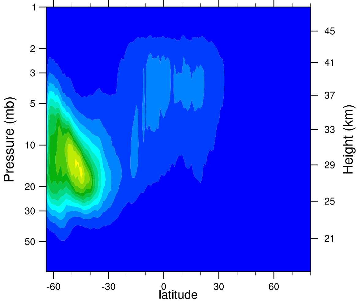
2007d216 N2O5_Ascending (ppbv)
