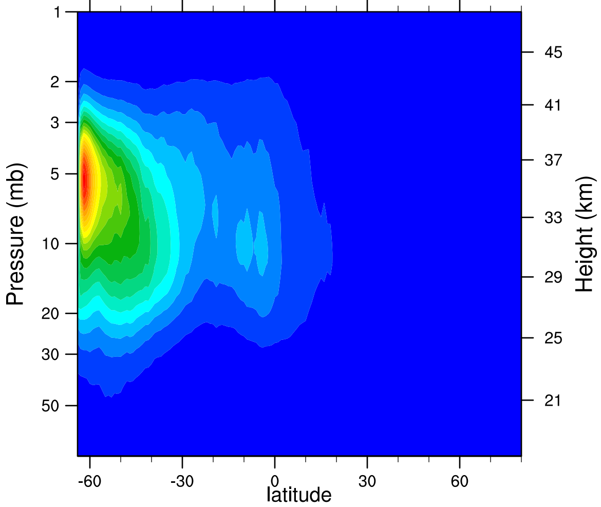
2006d163 N2O5_Ascending (ppbv)
