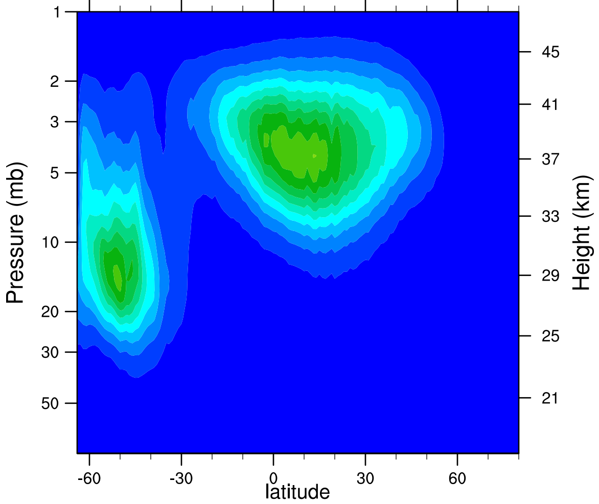
2005d155 N2O5_Ascending (ppbv)
