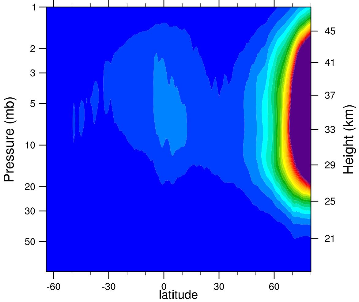
2006d026 N2O5_Ascending (ppbv)
