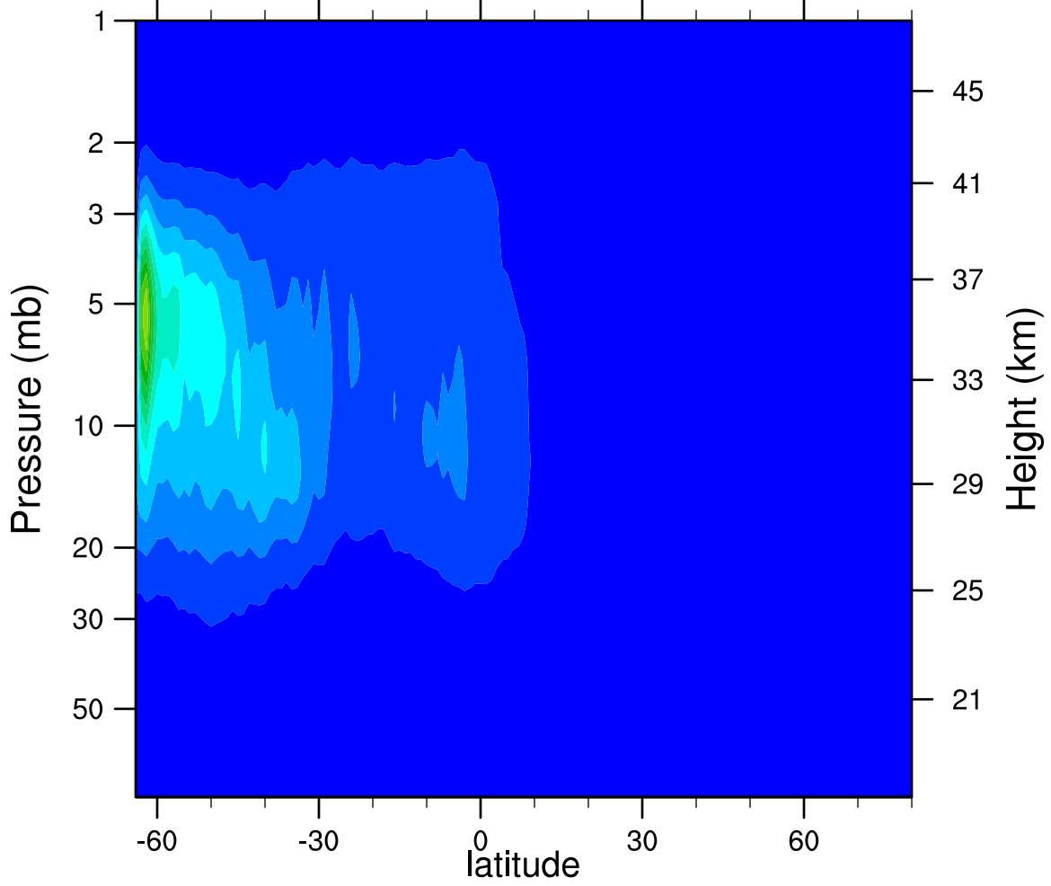
2006d175 N2O5_Ascending (ppbv)
