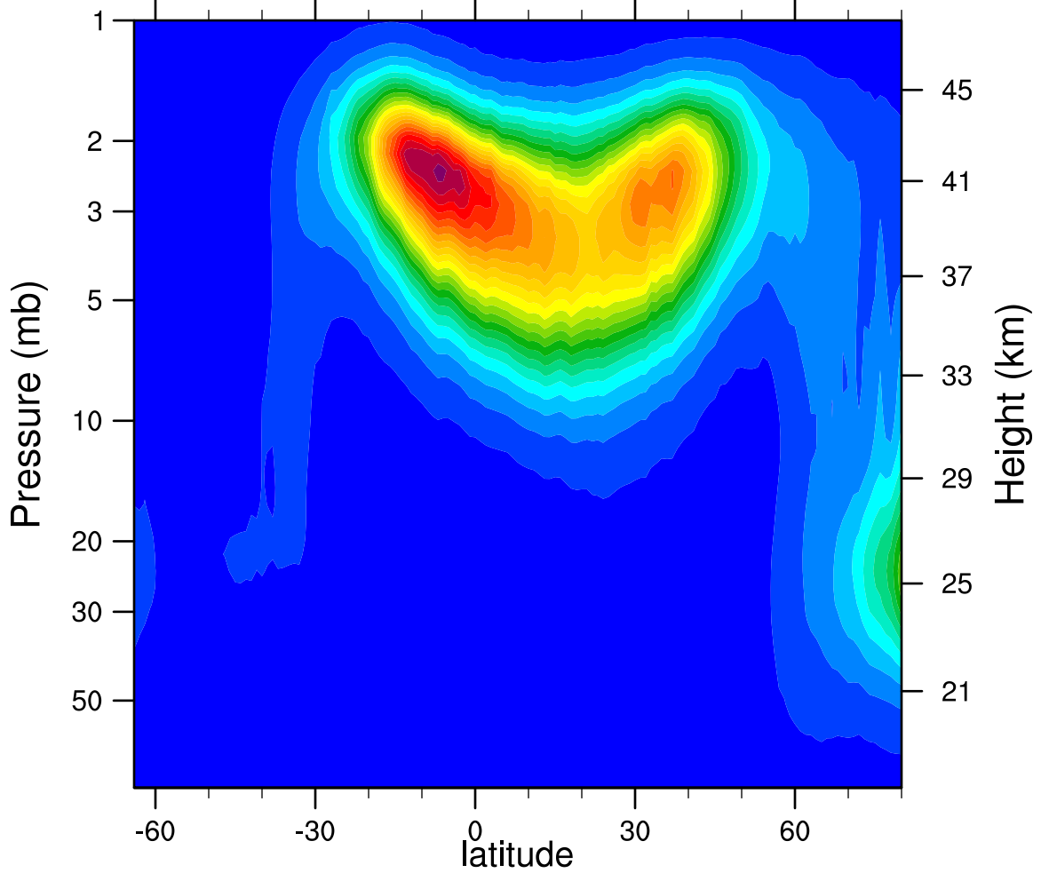
2005d063 N2O5_Ascending (ppbv)
