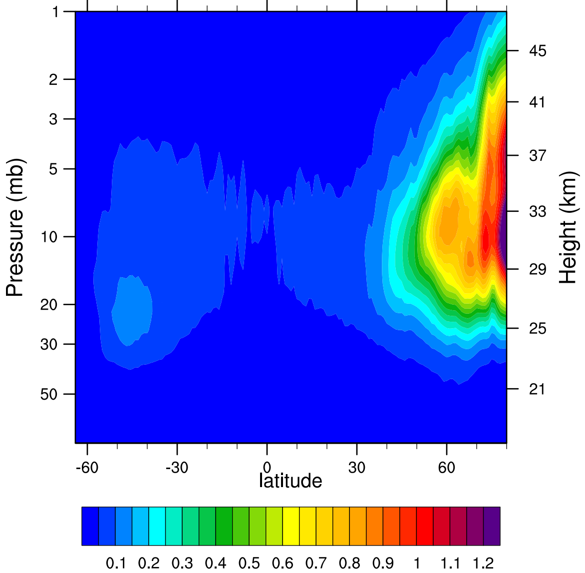
2006d342 N2O5_Ascending (ppbv)
