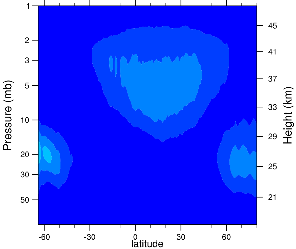
2005d269 N2O5_Ascending (ppbv)
