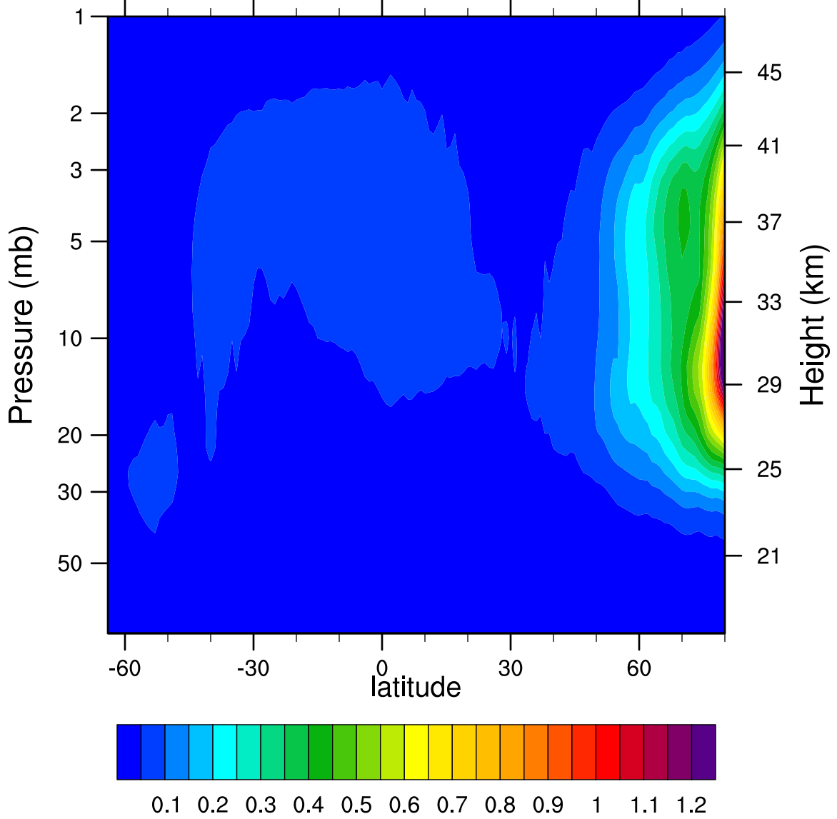
2006d048 N2O5_Ascending (ppbv)
