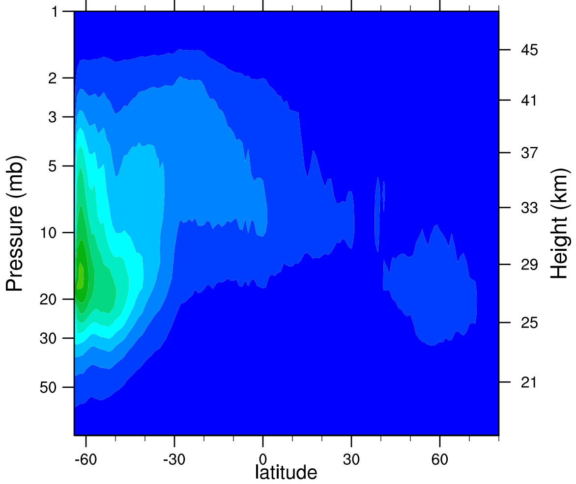
2006d107 N2O5_Ascending (ppbv)
