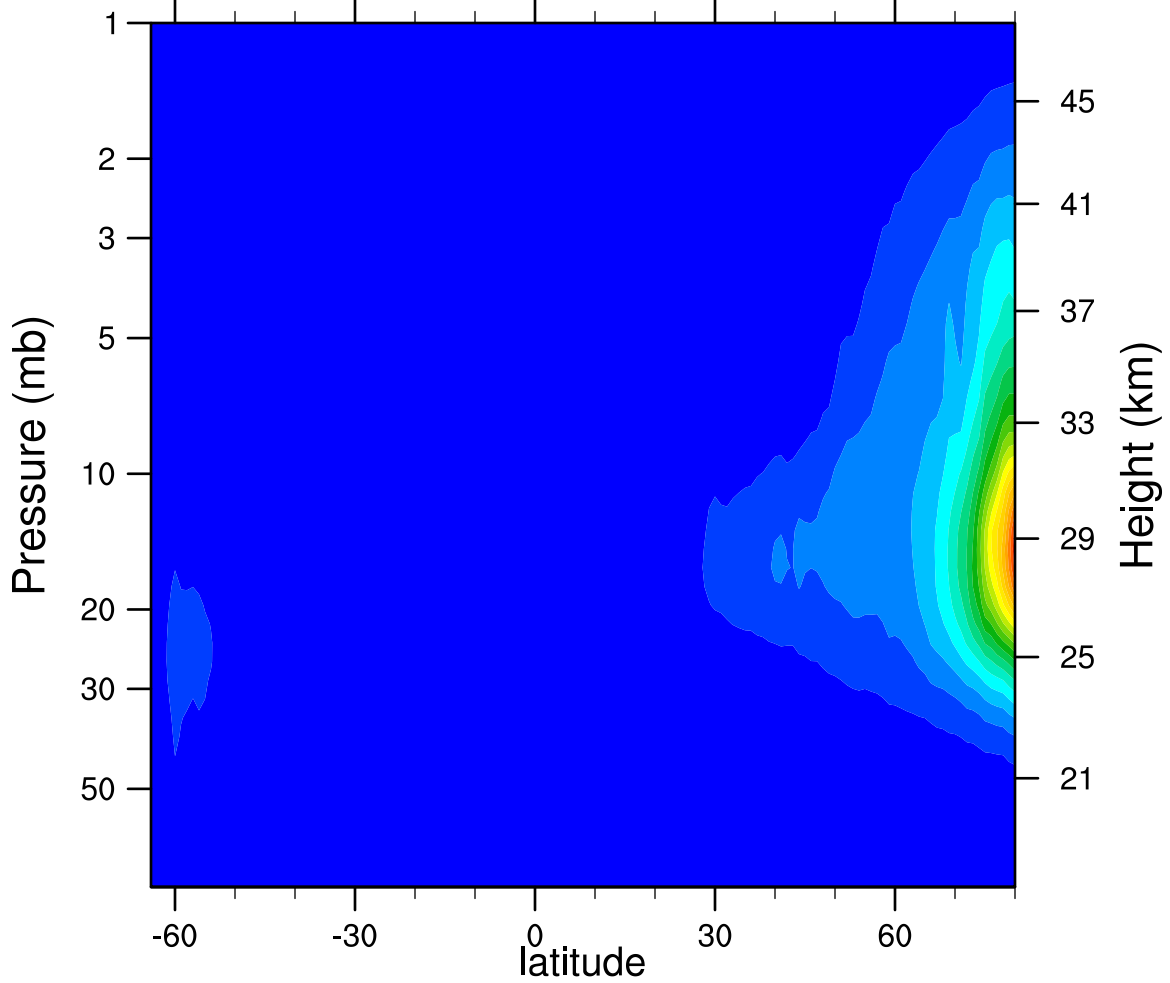
2006d290 N2O5_Ascending (ppbv)
