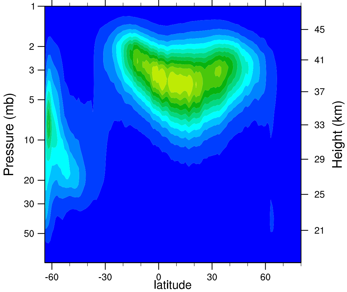
2005d105 N2O5_Ascending (ppbv)
