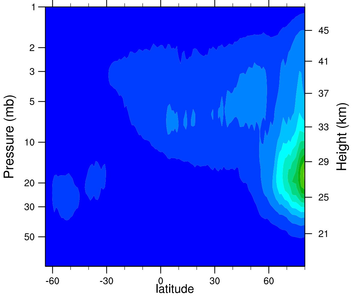
2005d288 N2O5_Ascending (ppbv)
