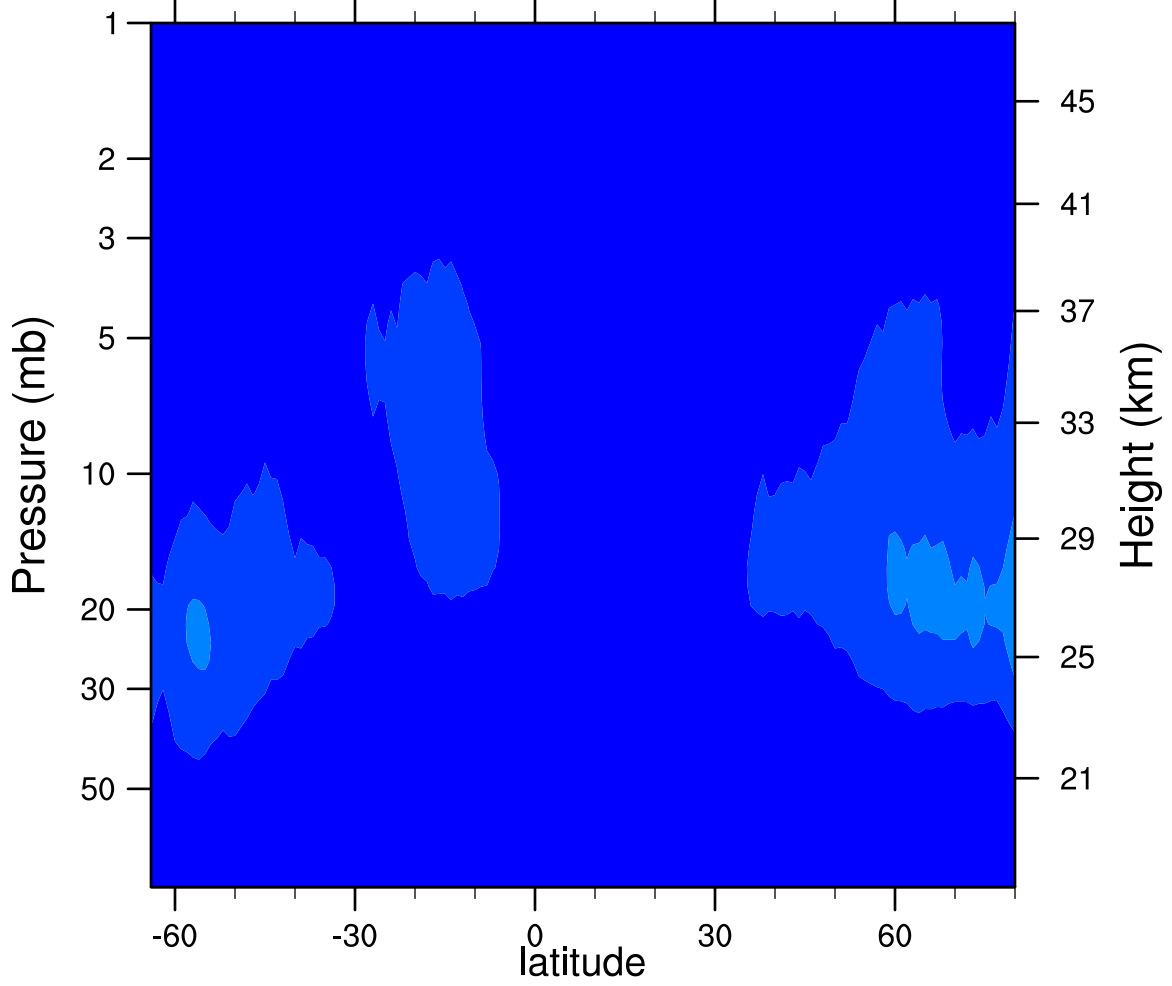
2006d270 N2O5_Ascending (ppbv)
