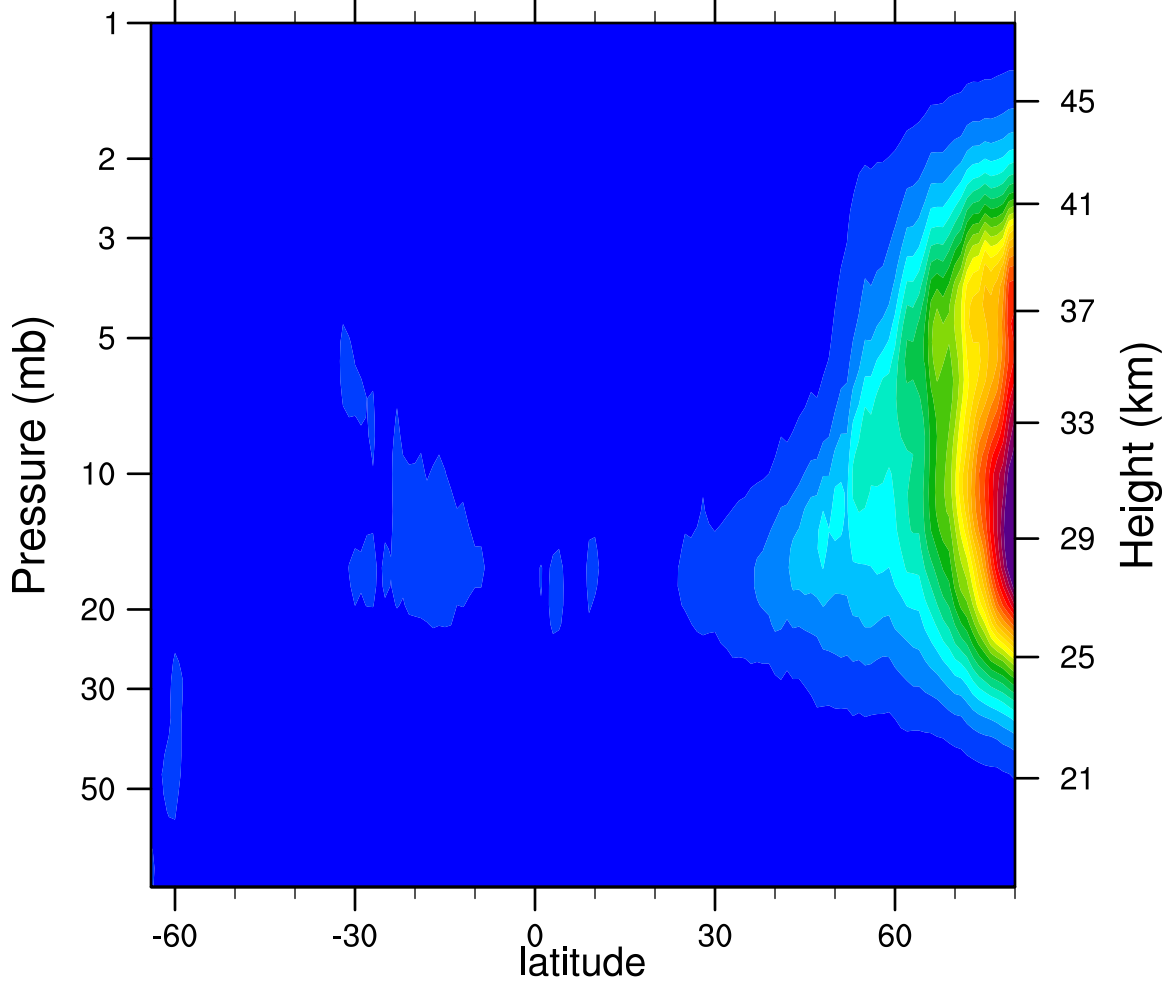
2006d300 N2O5_Ascending (ppbv)
