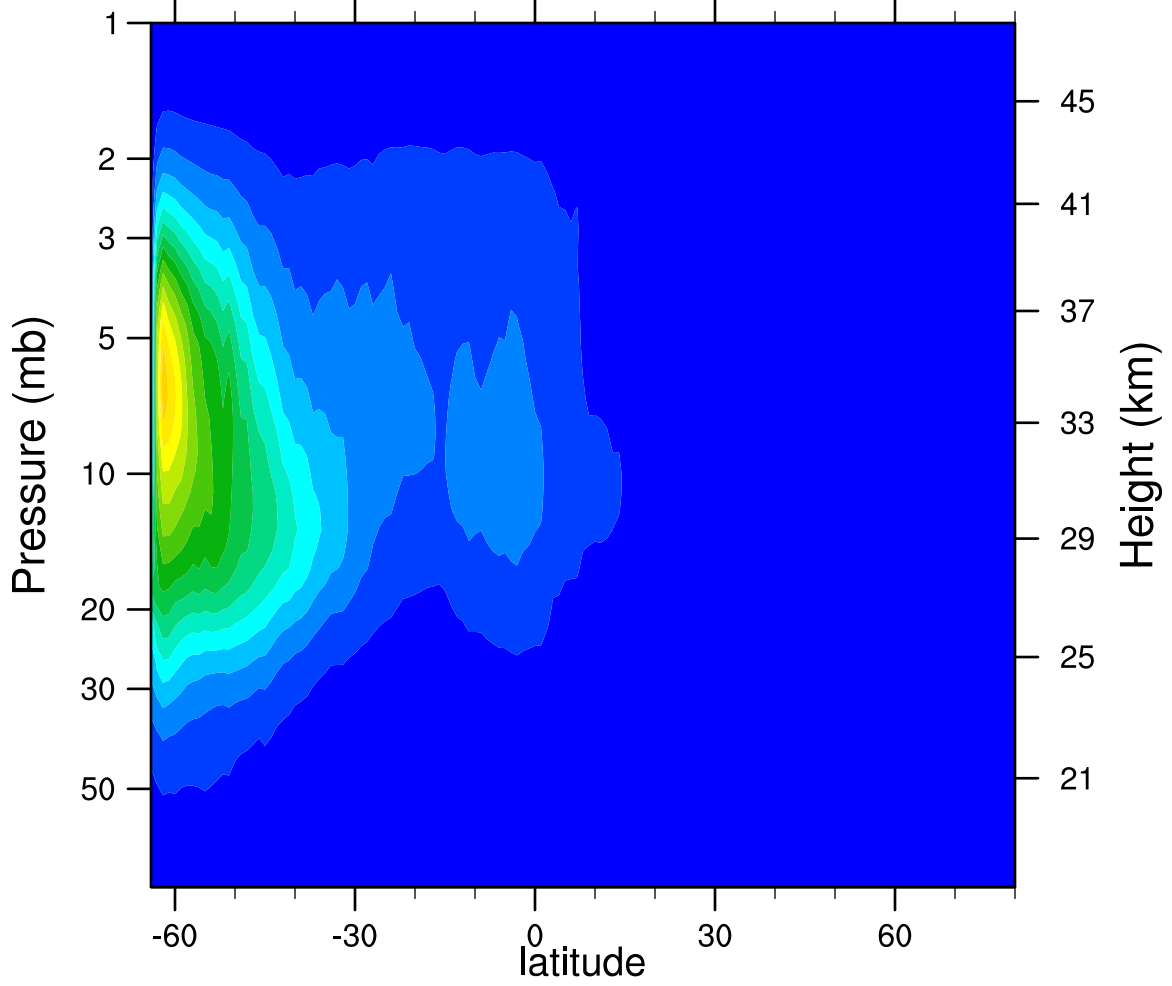
2006d141 N2O5_Ascending (ppbv)
