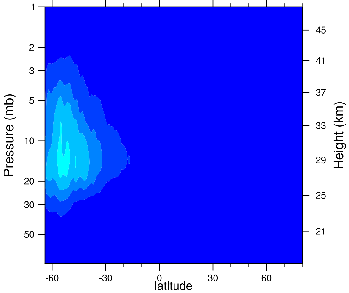
2007d199 N2O5_Ascending (ppbv)
