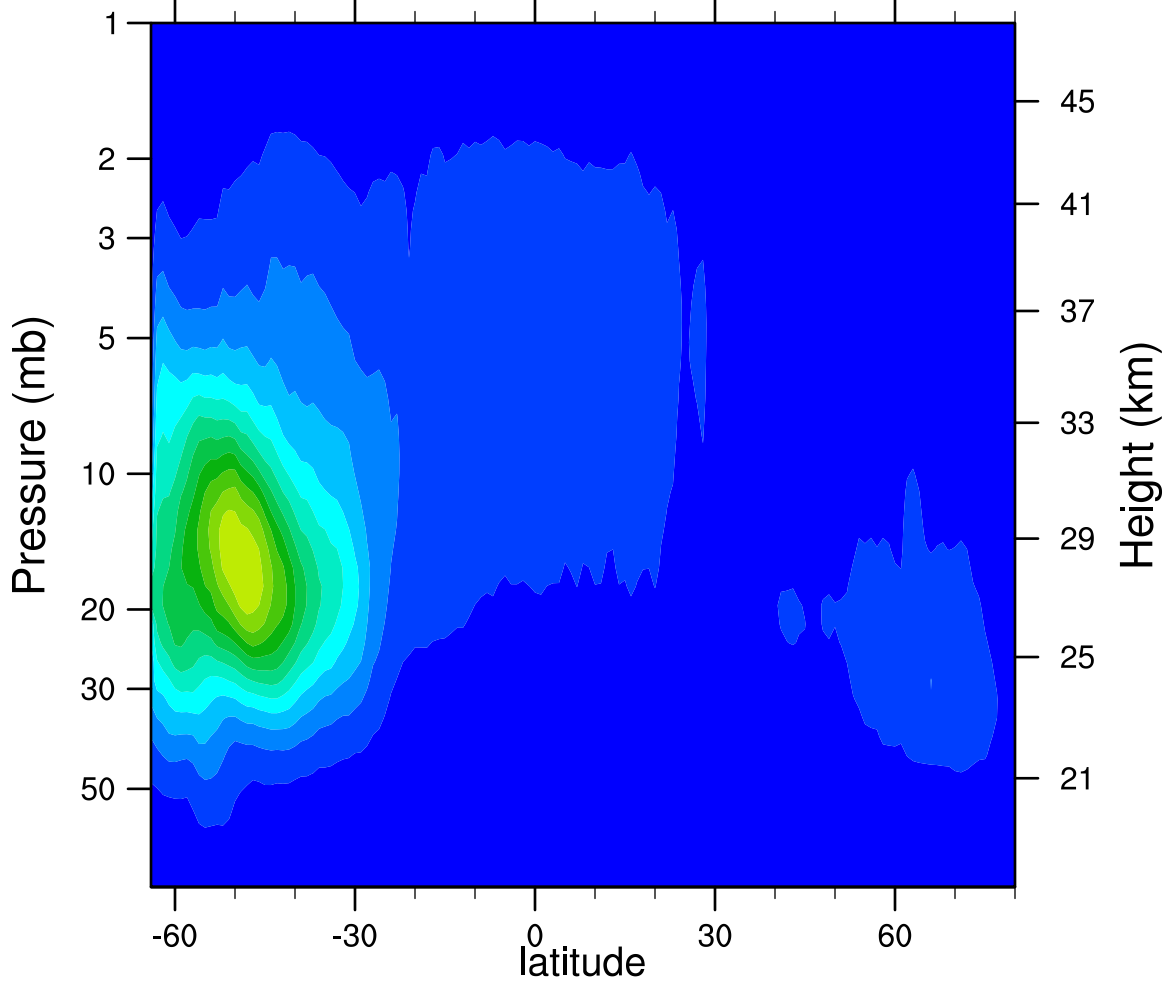
2007d236 N2O5_Ascending (ppbv)
