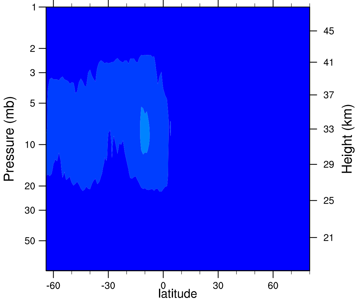
2006d186 N2O5_Ascending (ppbv)
