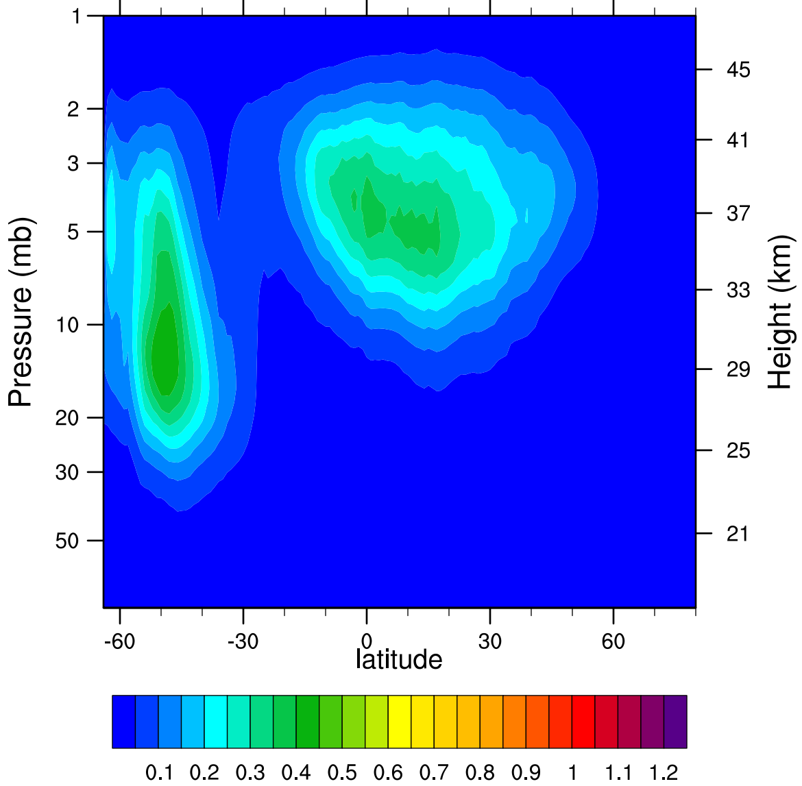
2005d180 N2O5_Ascending (ppbv)
