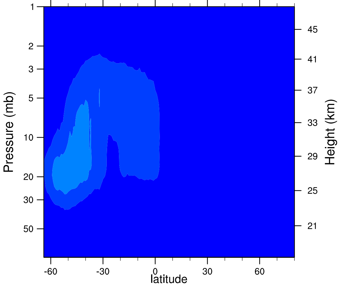
2006d234 N2O5_Ascending (ppbv)
