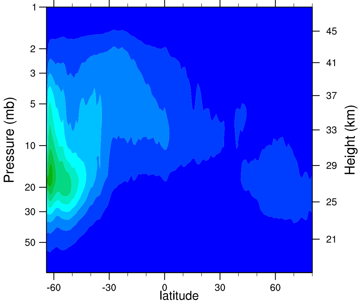
2006d104 N2O5_Ascending (ppbv)
