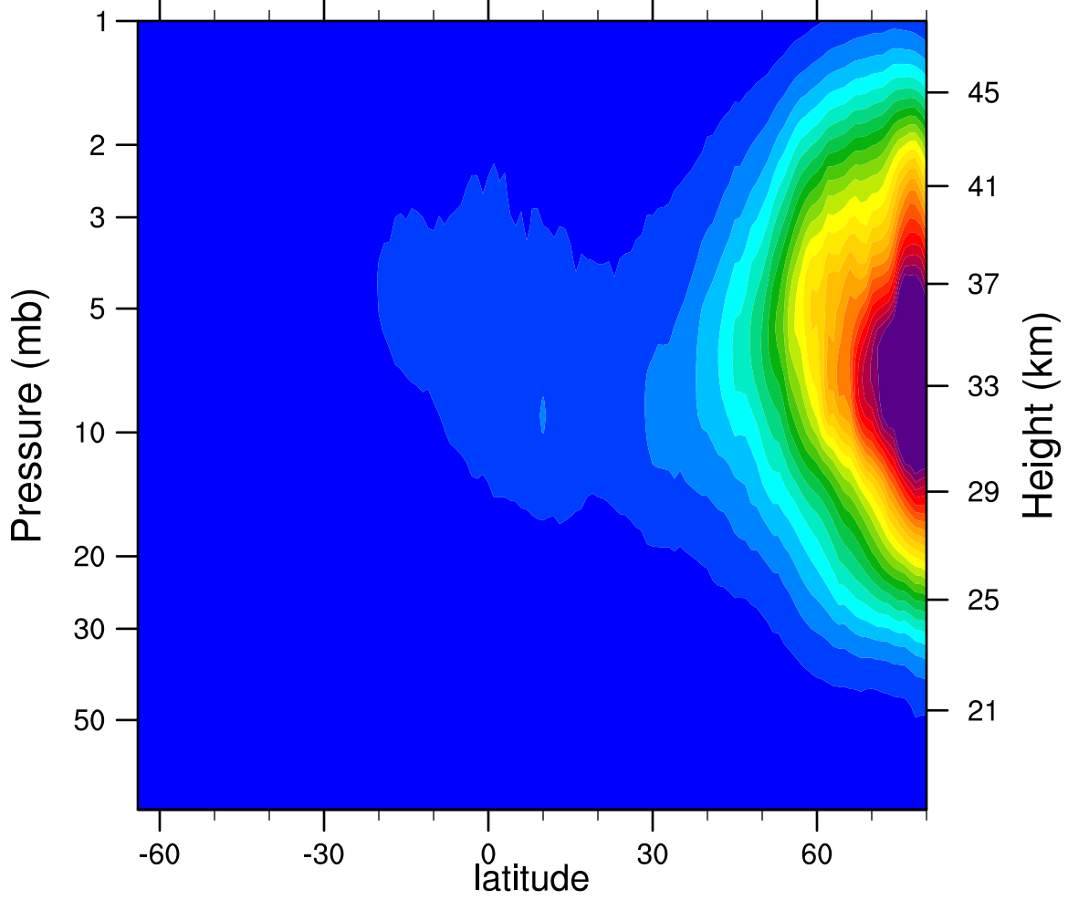
2005d330 N2O5_Ascending (ppbv)
