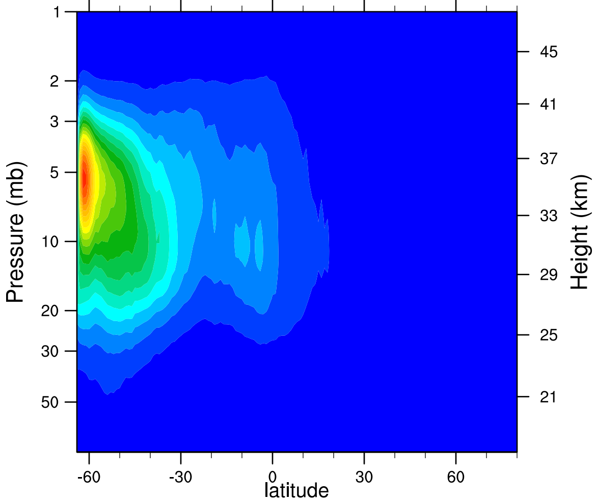
2006d164 N2O5_Ascending (ppbv)
