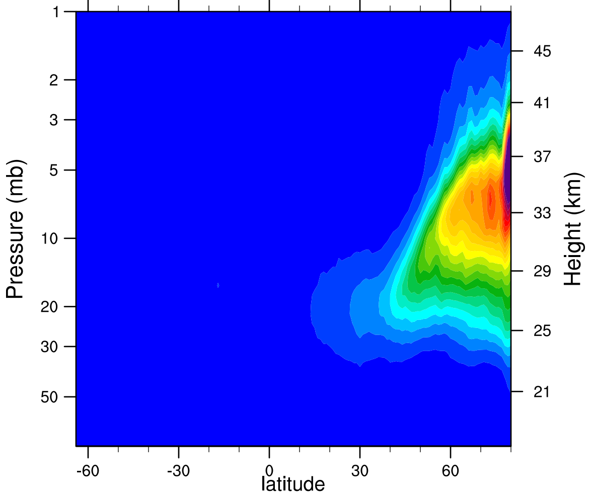
2007d029 N2O5_Ascending (ppbv)
