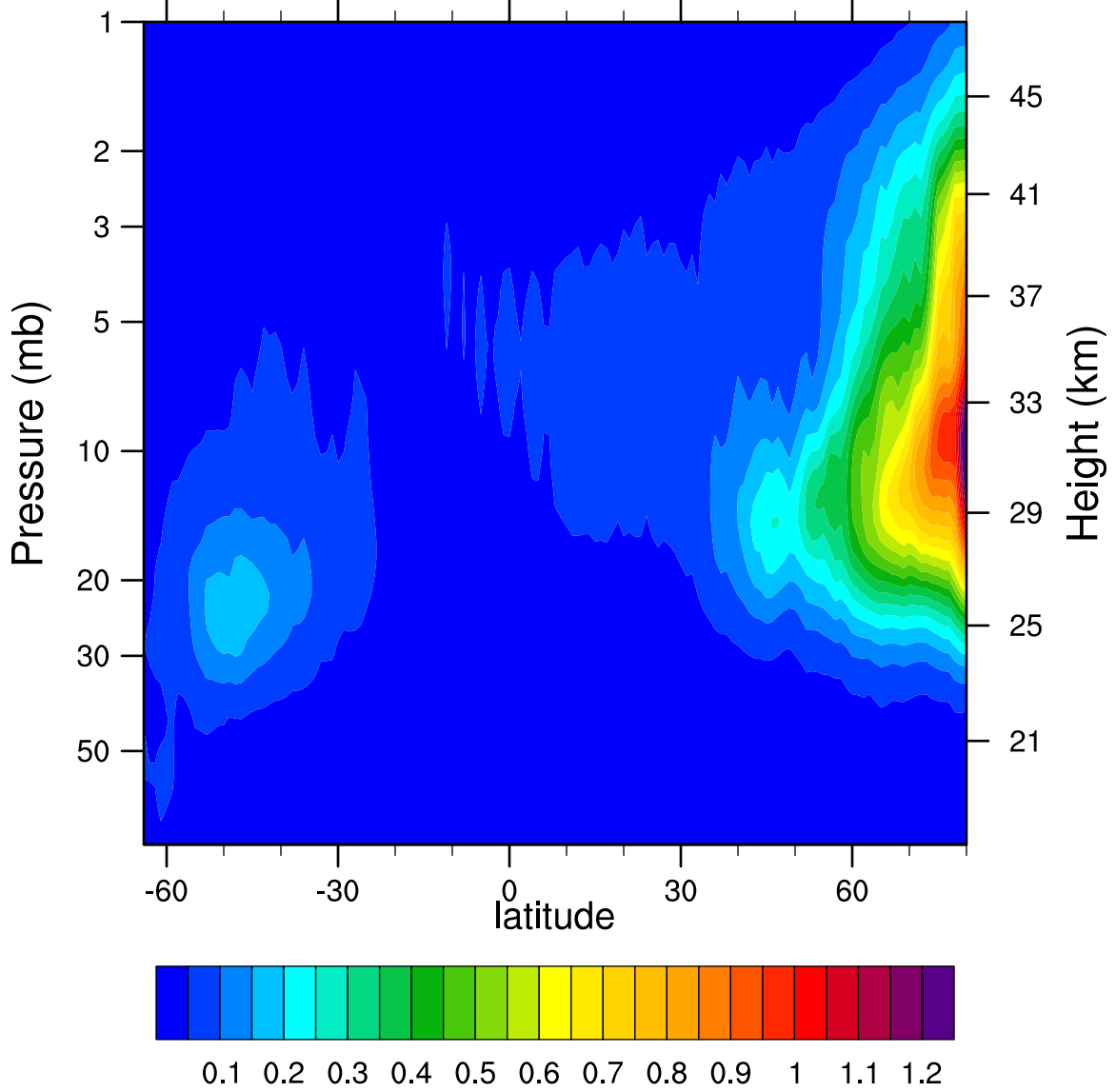
2006d331 N2O5_Ascending (ppbv)
