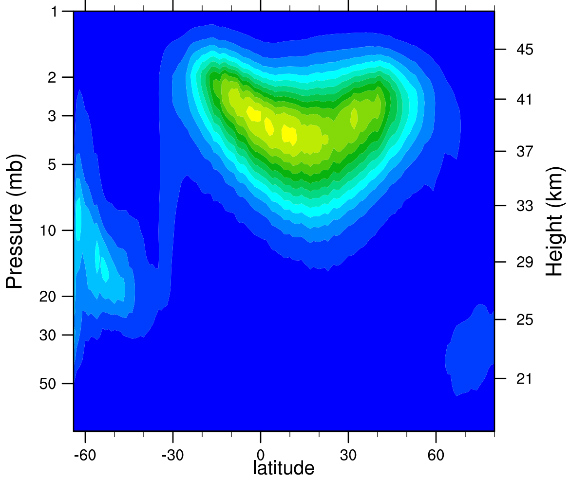
2005d096 N2O5_Ascending (ppbv)
