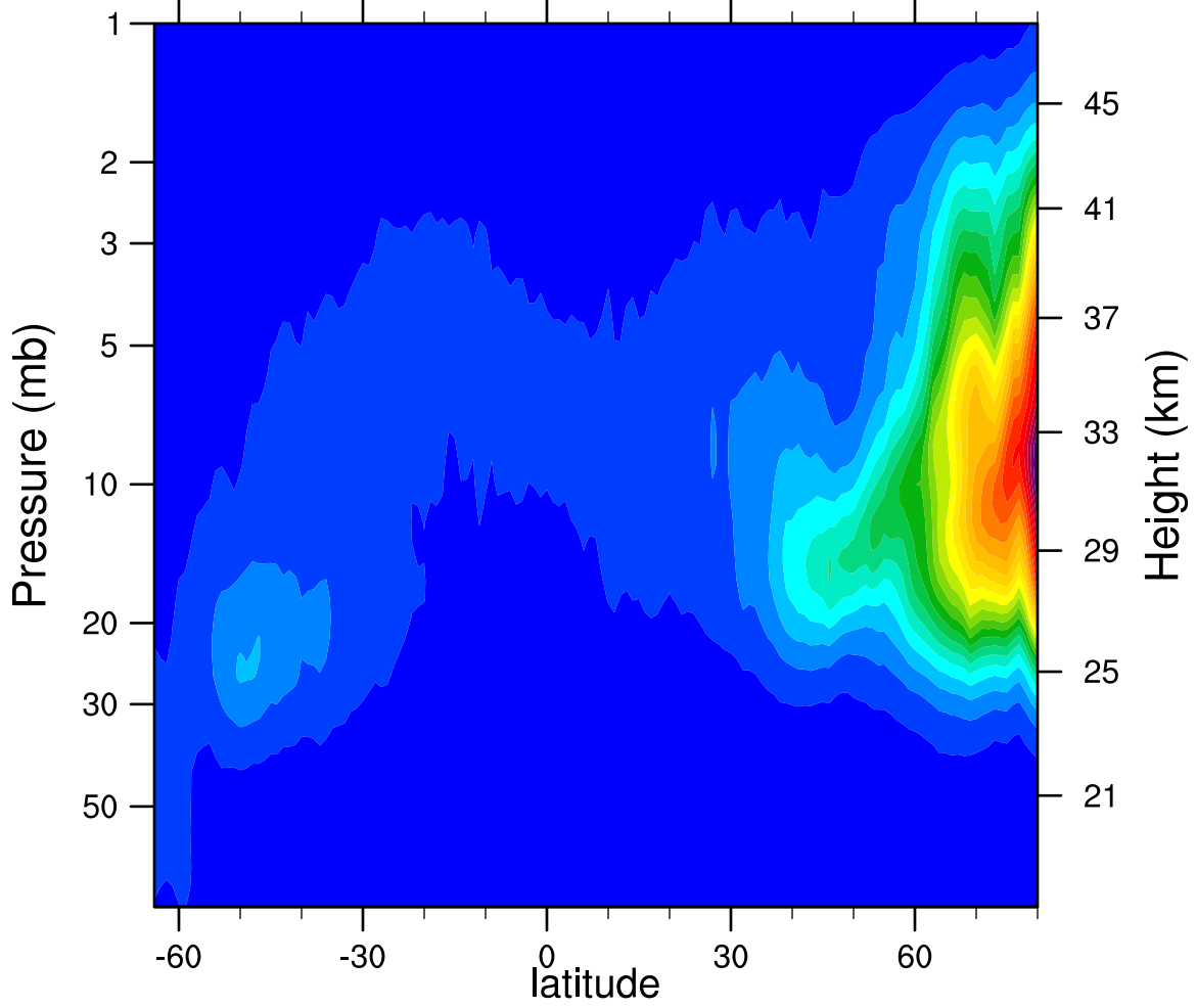
2006d326 N2O5_Ascending (ppbv)
