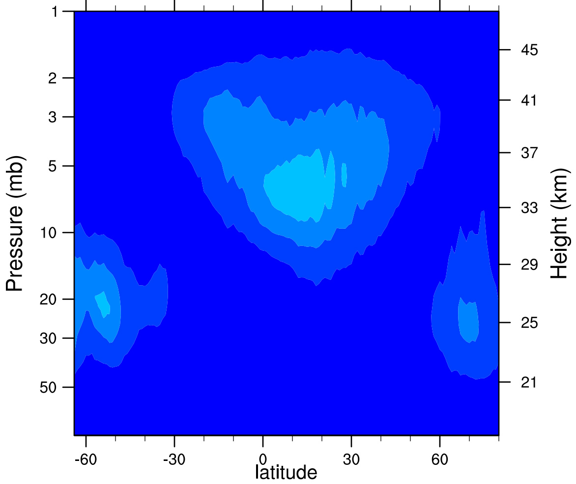
2005d259 N2O5_Ascending (ppbv)
