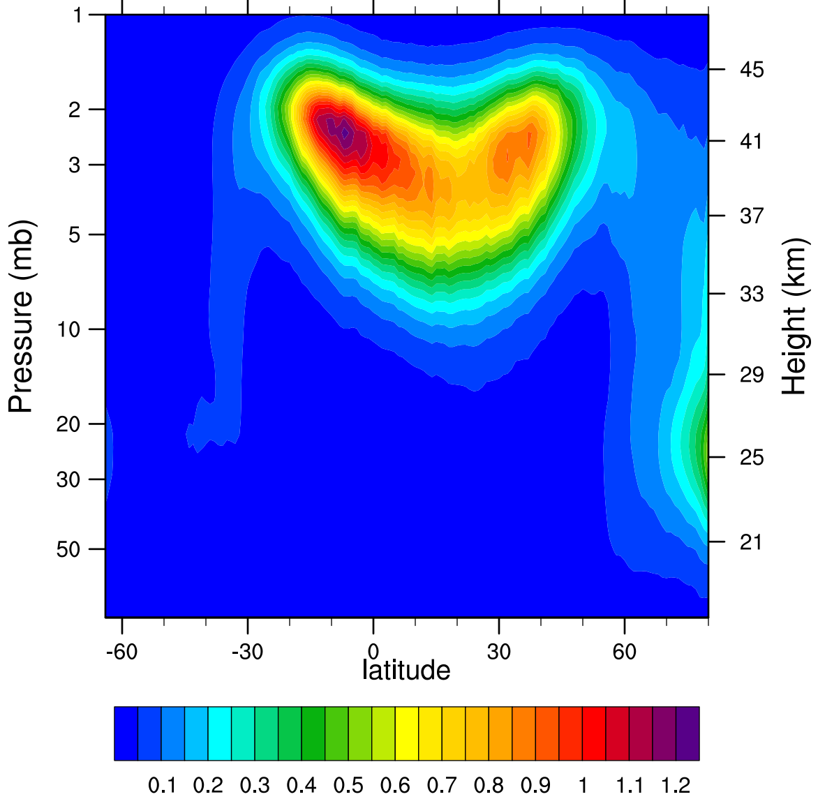
2005d061 N2O5_Ascending (ppbv)
