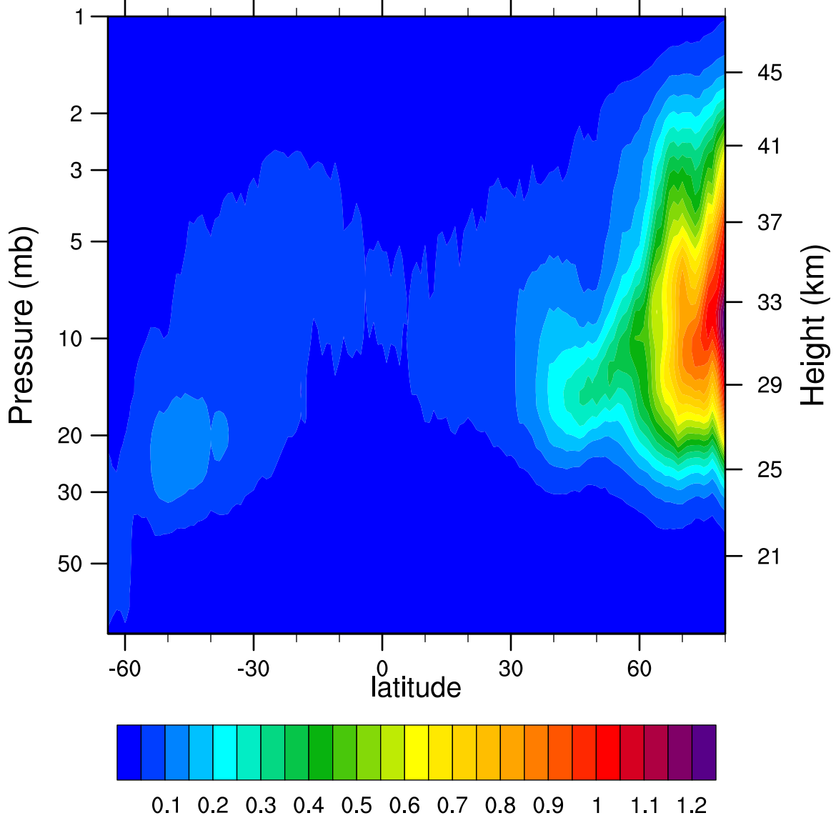
2006d325 N2O5_Ascending (ppbv)
