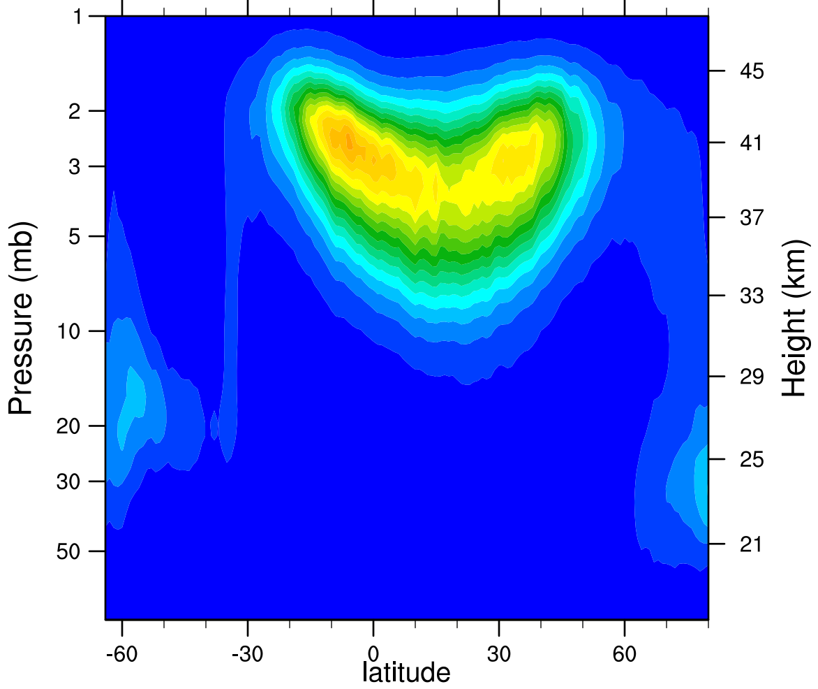
2005d081 N2O5_Ascending (ppbv)
