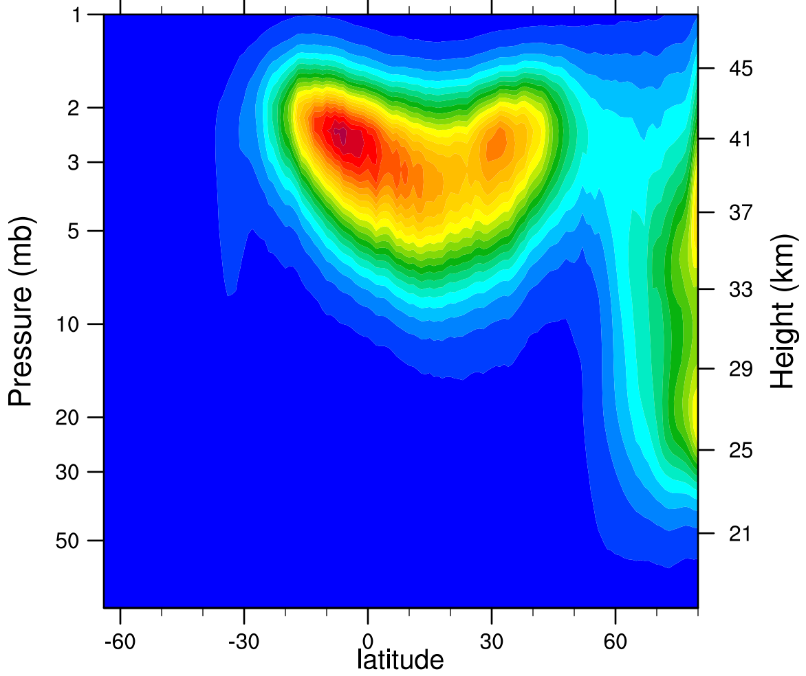
2005d050 N2O5_Ascending (ppbv)
