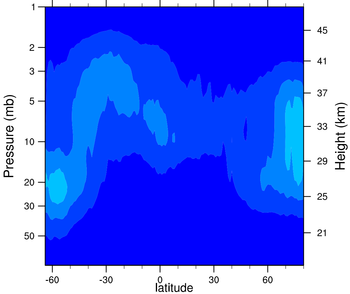
2006d082 N2O5_Ascending (ppbv)
