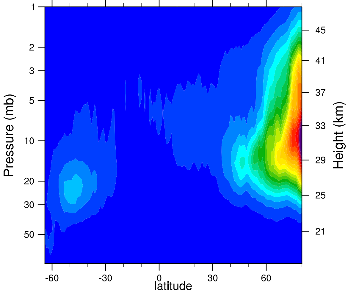
2006d332 N2O5_Ascending (ppbv)
