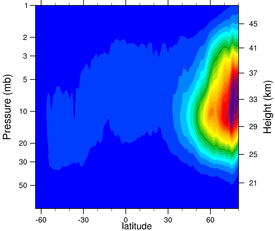
2007d353 N2O5_Ascending (ppbv)
