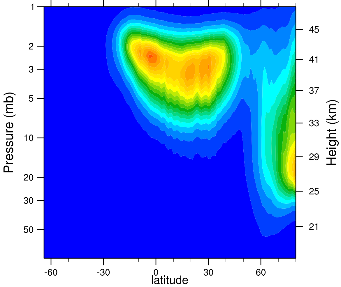
2005d036 N2O5_Ascending (ppbv)
