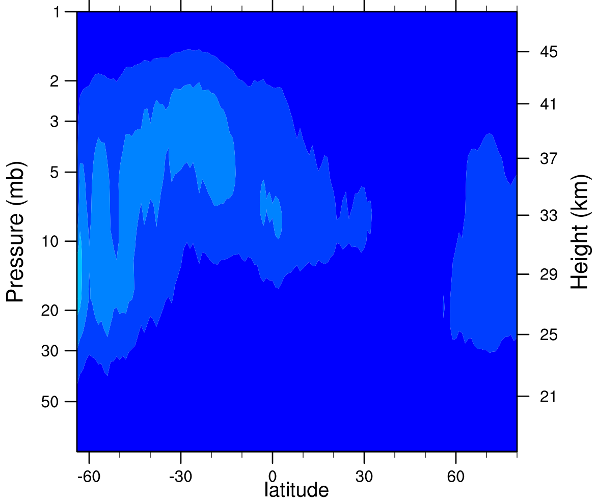
2006d094 N2O5_Ascending (ppbv)
