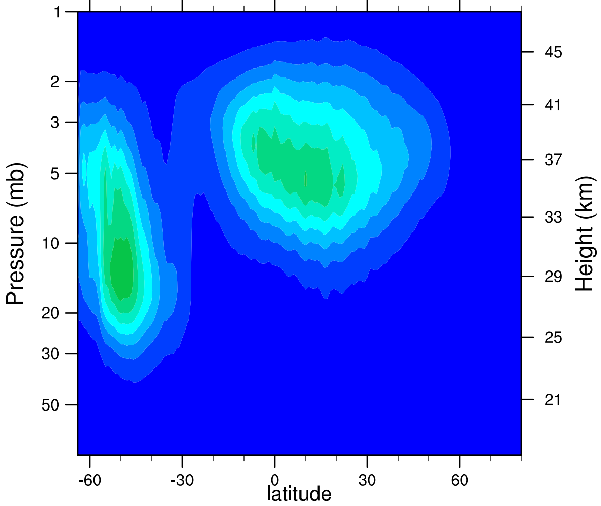
2005d191 N2O5_Ascending (ppbv)
