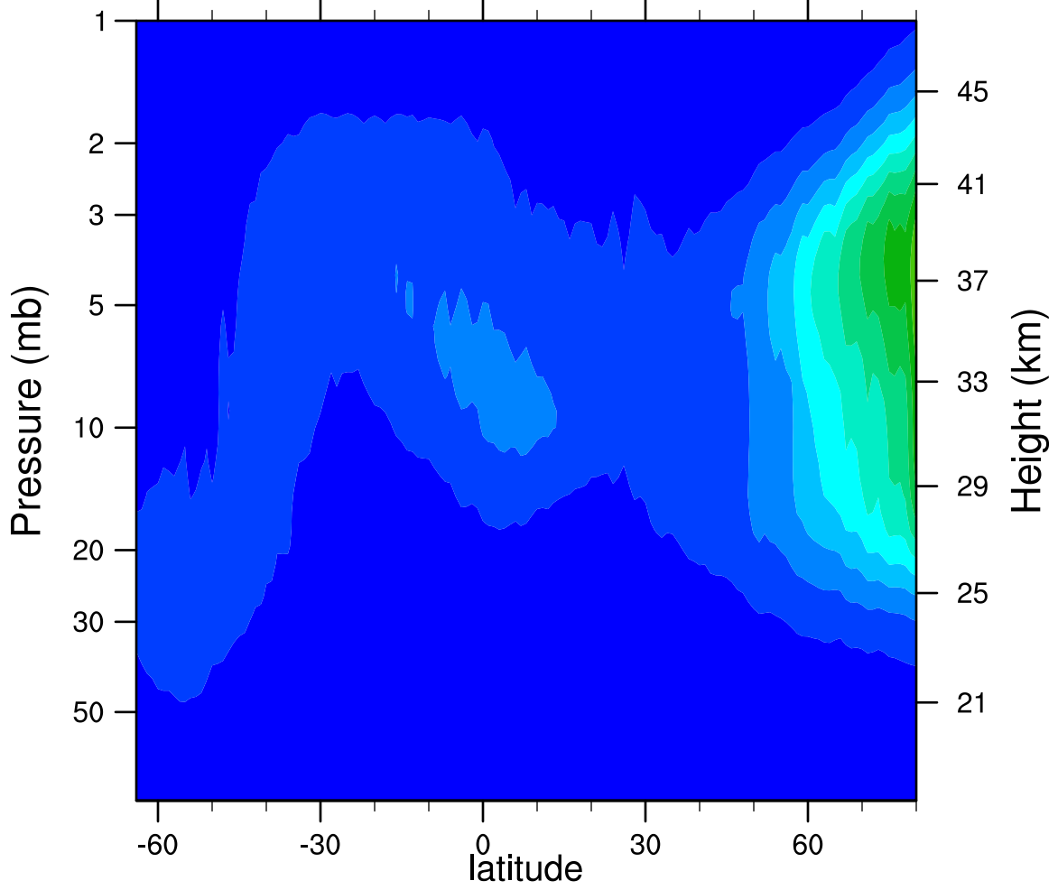
2006d061 N2O5_Ascending (ppbv)
