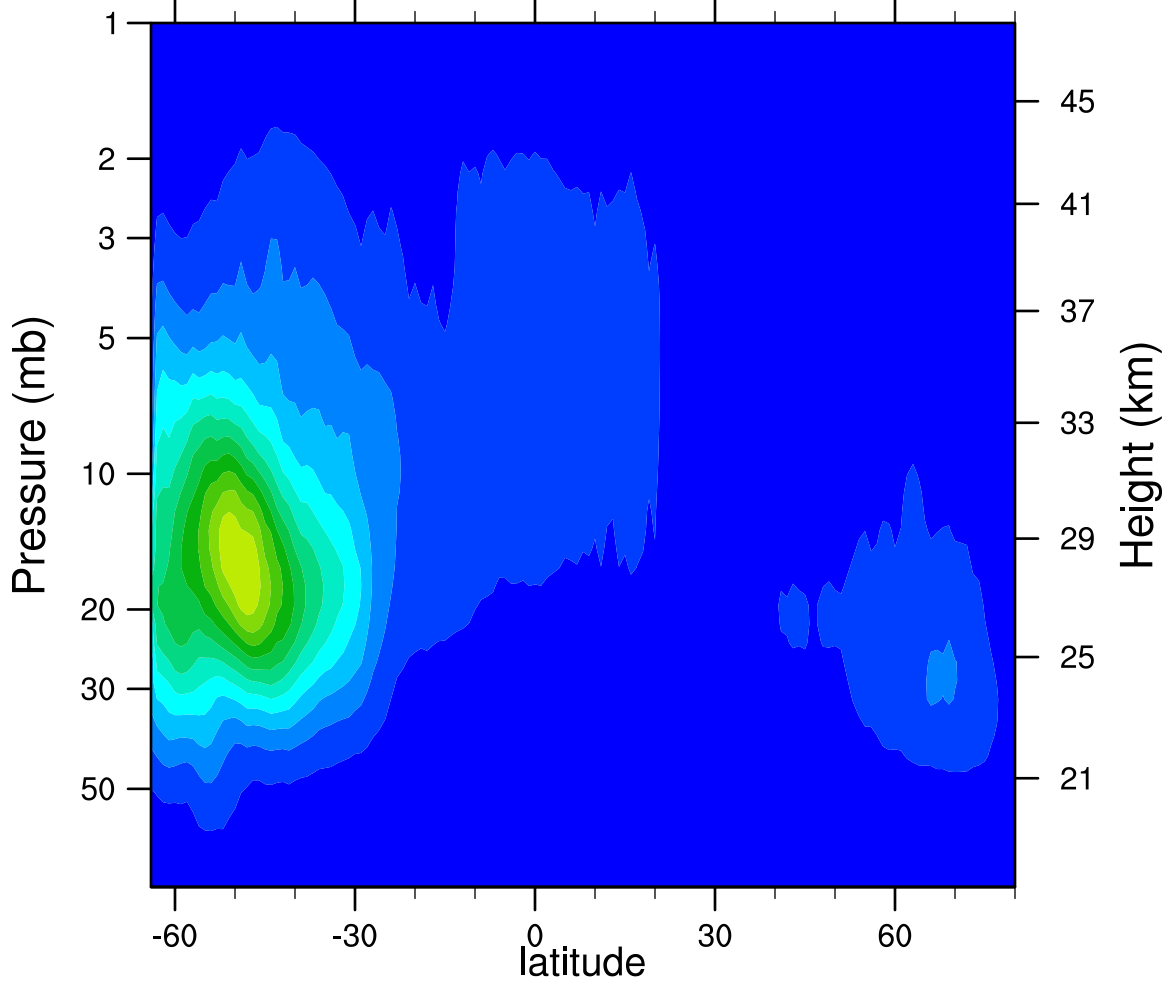
2007d237 N2O5_Ascending (ppbv)
