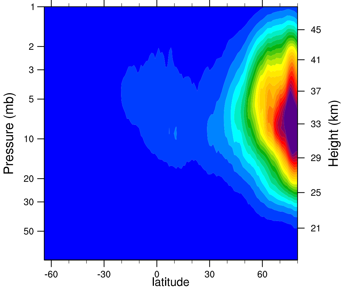
2005d332 N2O5_Ascending (ppbv)
