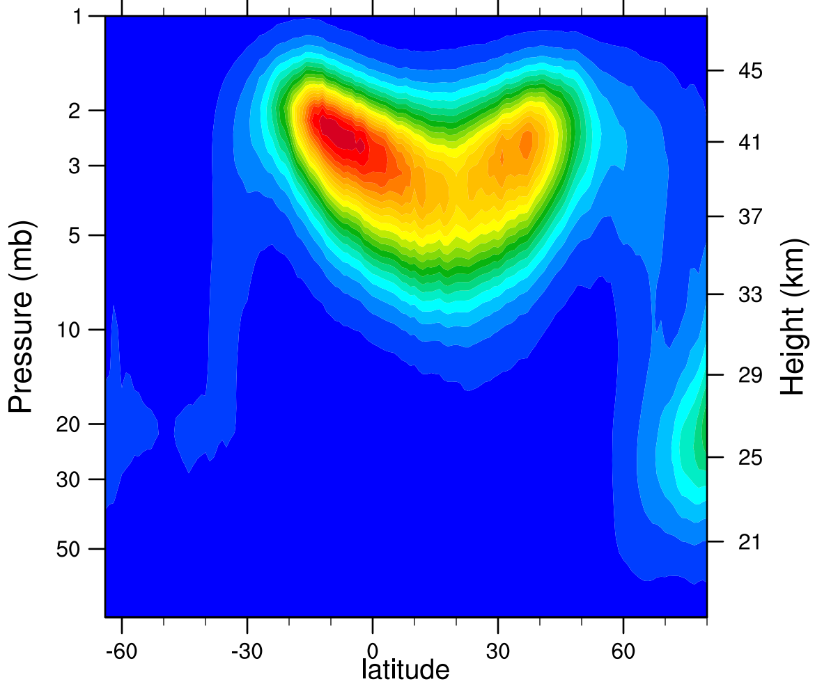
2005d066 N2O5_Ascending (ppbv)
