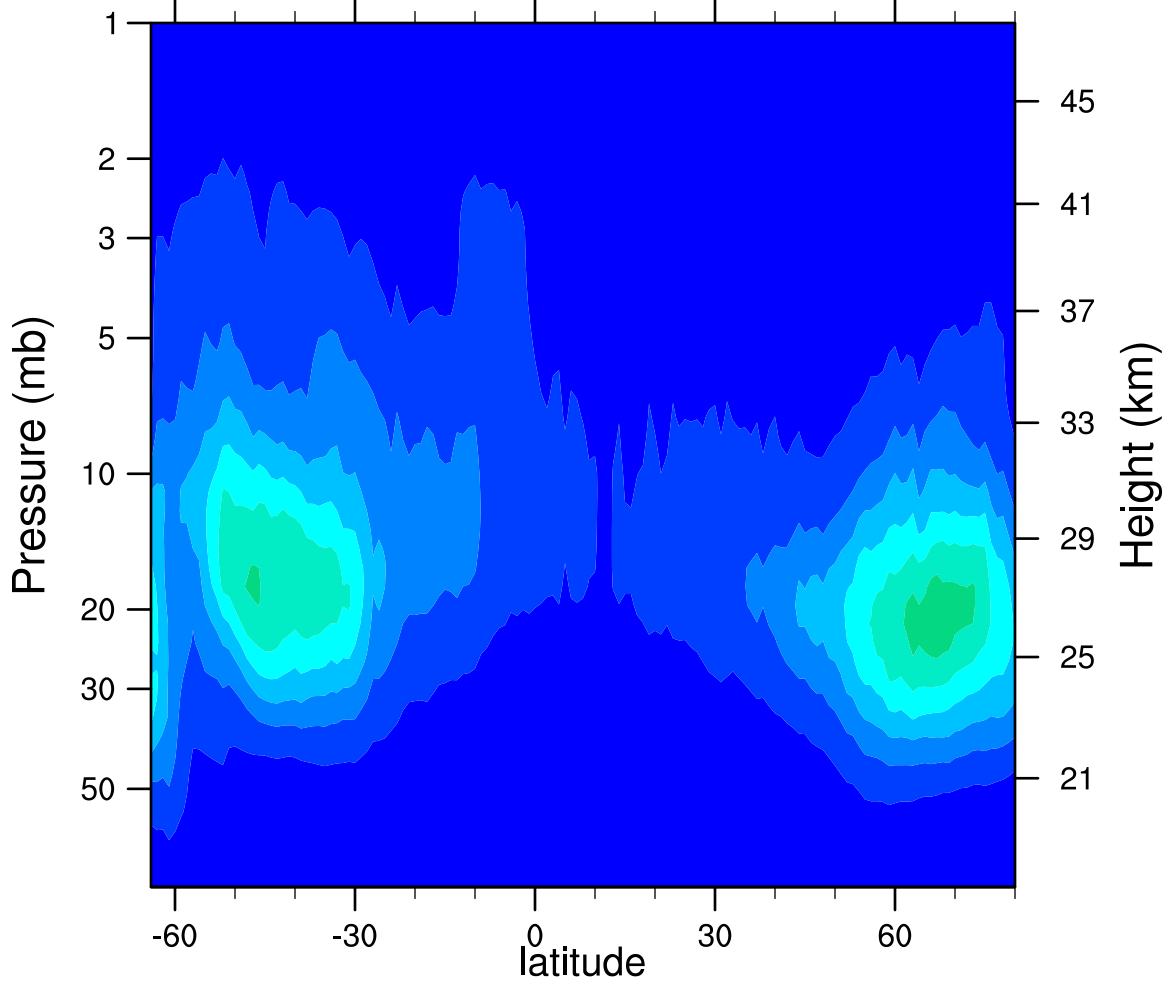
2007d263 N2O5_Ascending (ppbv)
