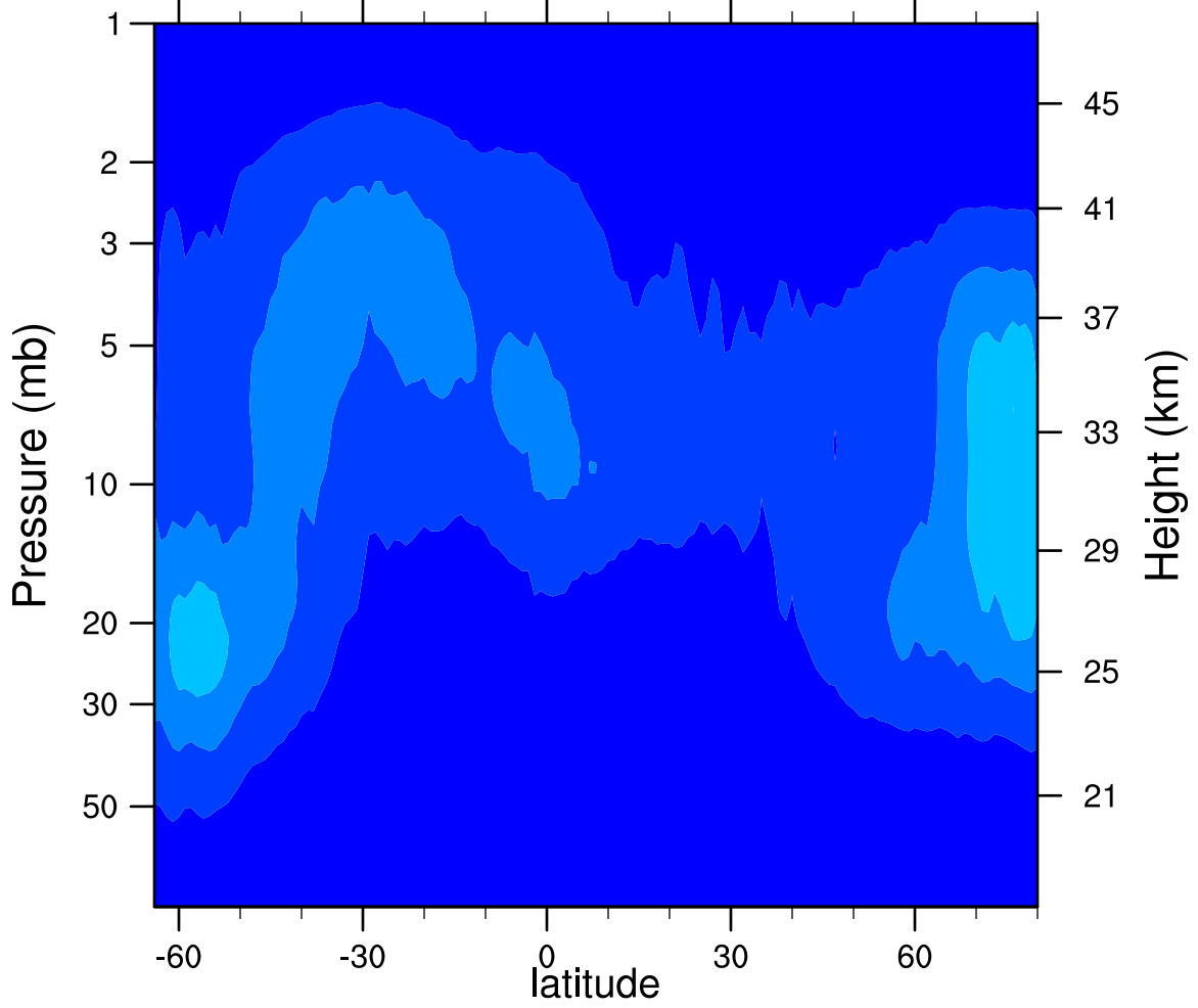
2006d081 N2O5_Ascending (ppbv)
