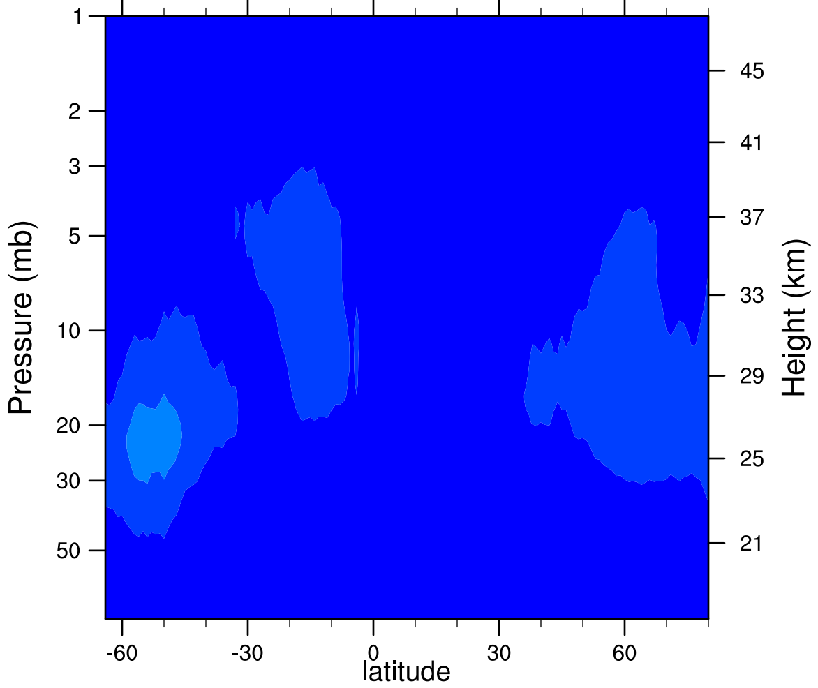
2006d267 N2O5_Ascending (ppbv)
