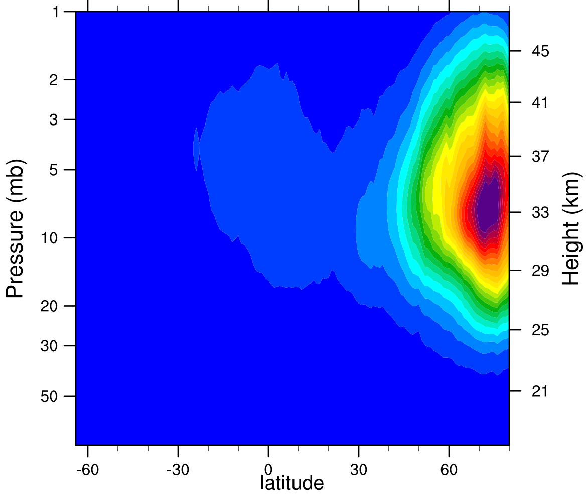
2005d348 N2O5_Ascending (ppbv)
