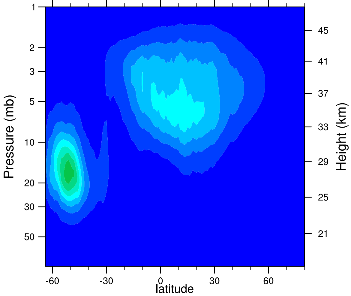
2005d226 N2O5_Ascending (ppbv)
