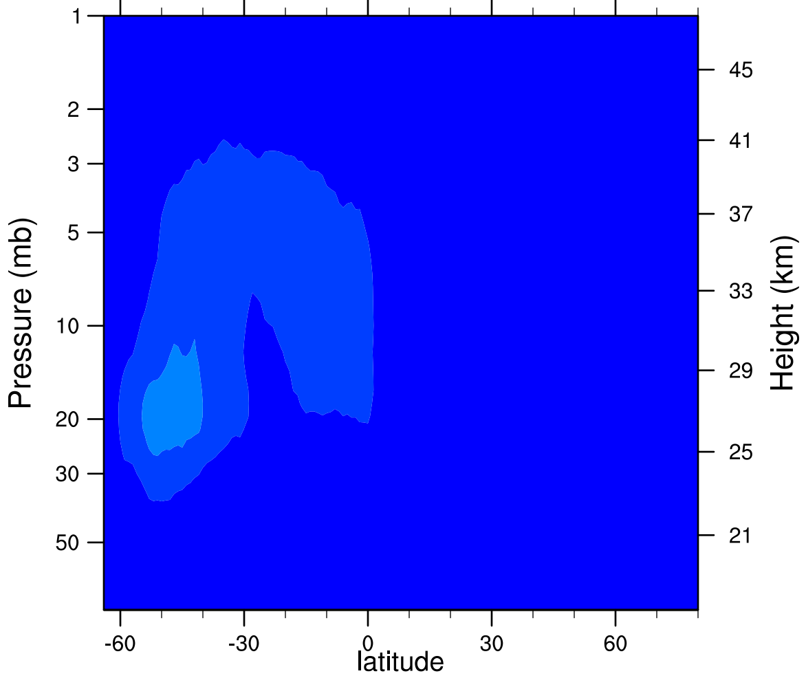
2006d244 N2O5_Ascending (ppbv)
