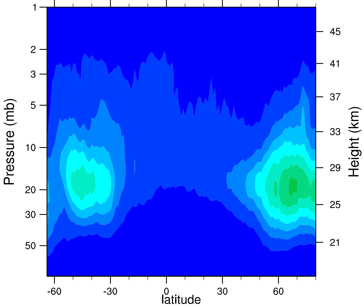
2007d269 N2O5_Ascending (ppbv)
