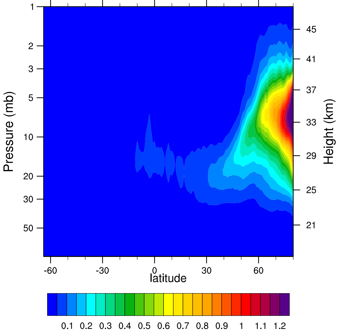
2007d037 N2O5_Ascending (ppbv)
