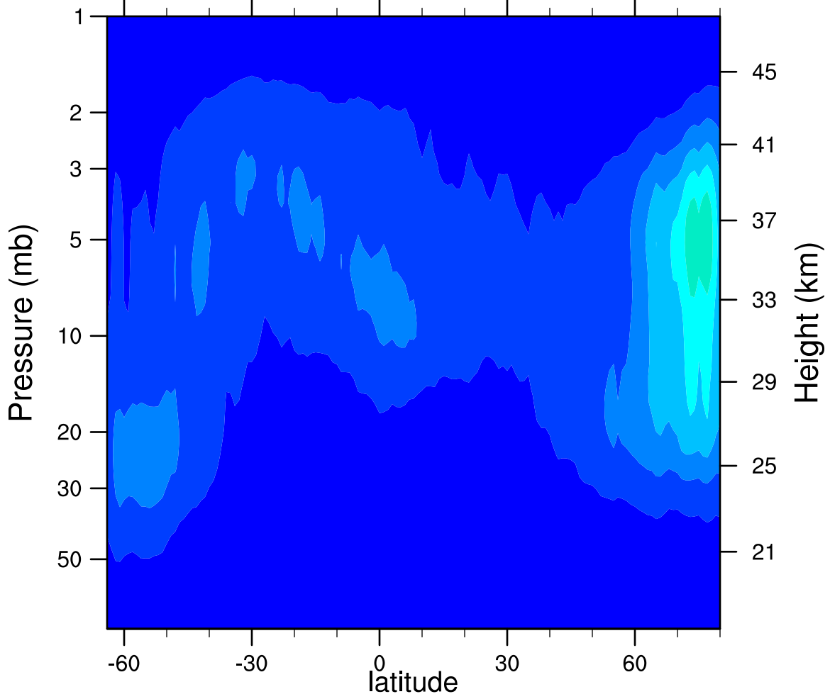
2006d072 N2O5_Ascending (ppbv)
