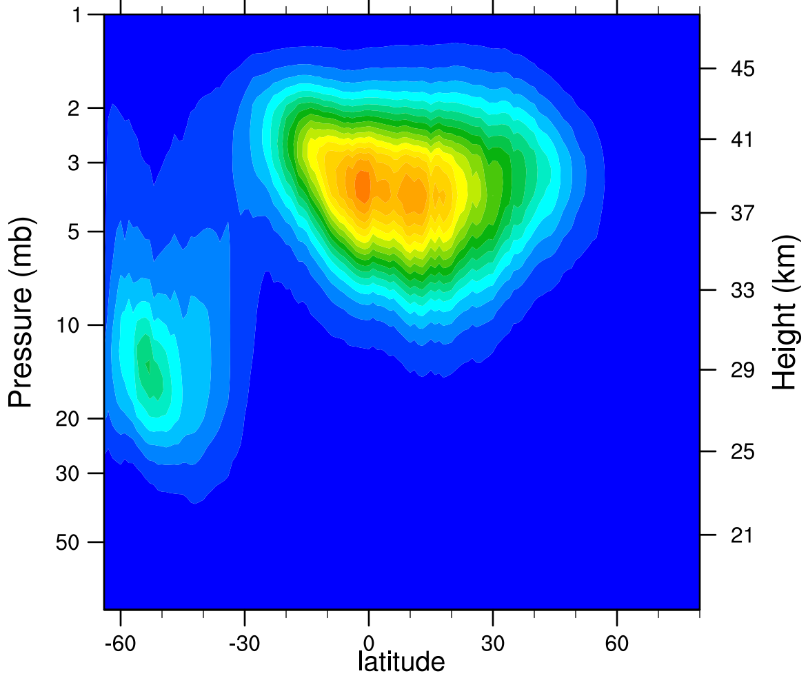
2005d137 N2O5_Ascending (ppbv)
