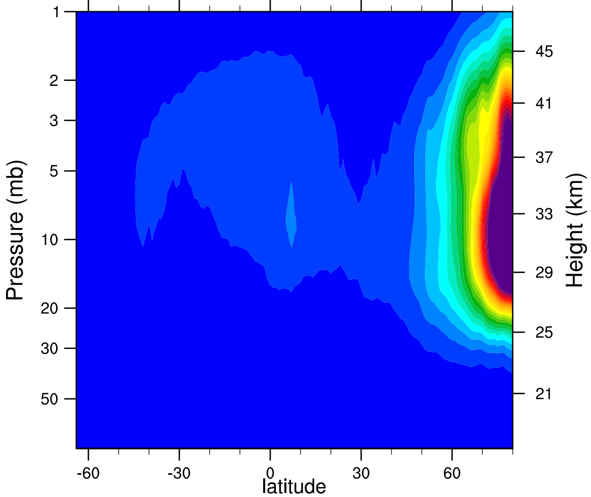
2006d036 N2O5_Ascending (ppbv)
