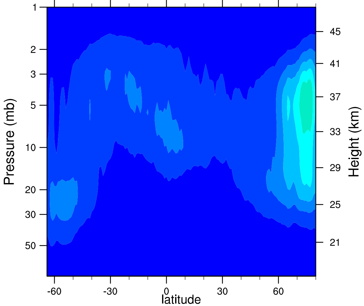
2006d071 N2O5_Ascending (ppbv)
