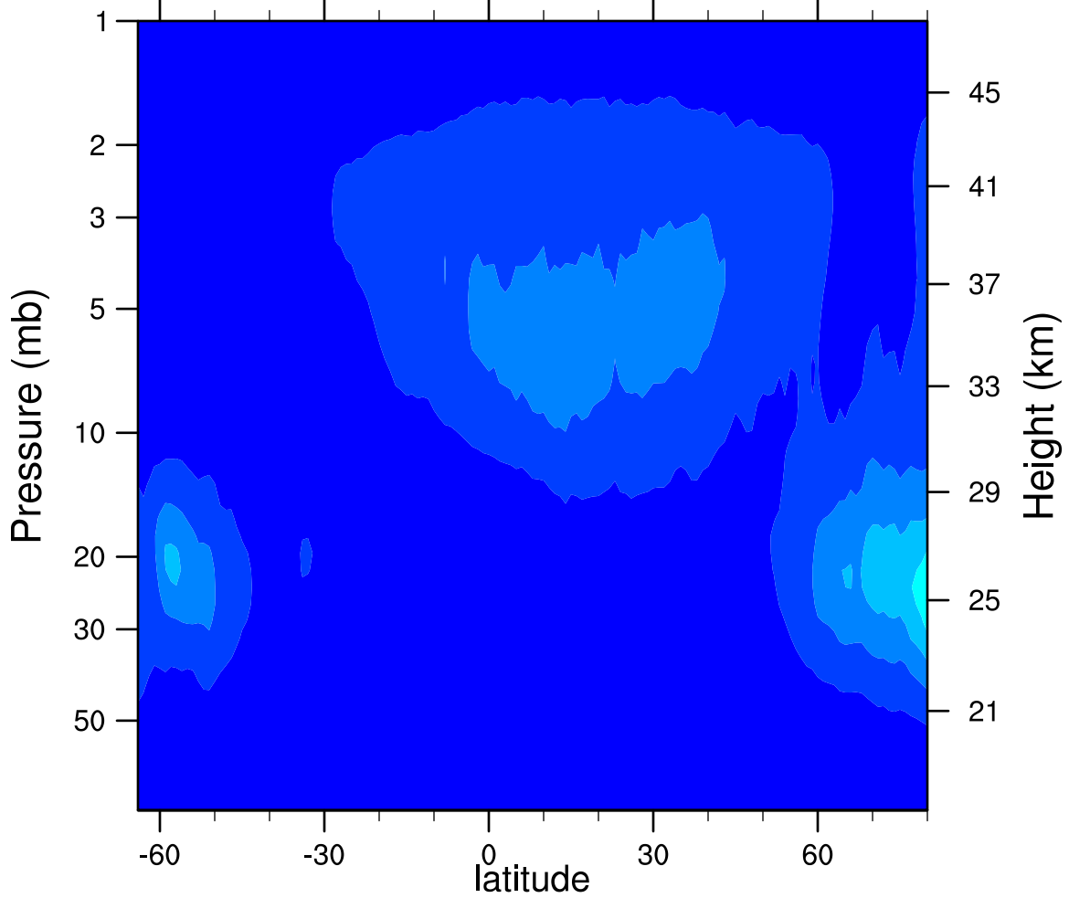
2005d274 N2O5_Ascending (ppbv)
