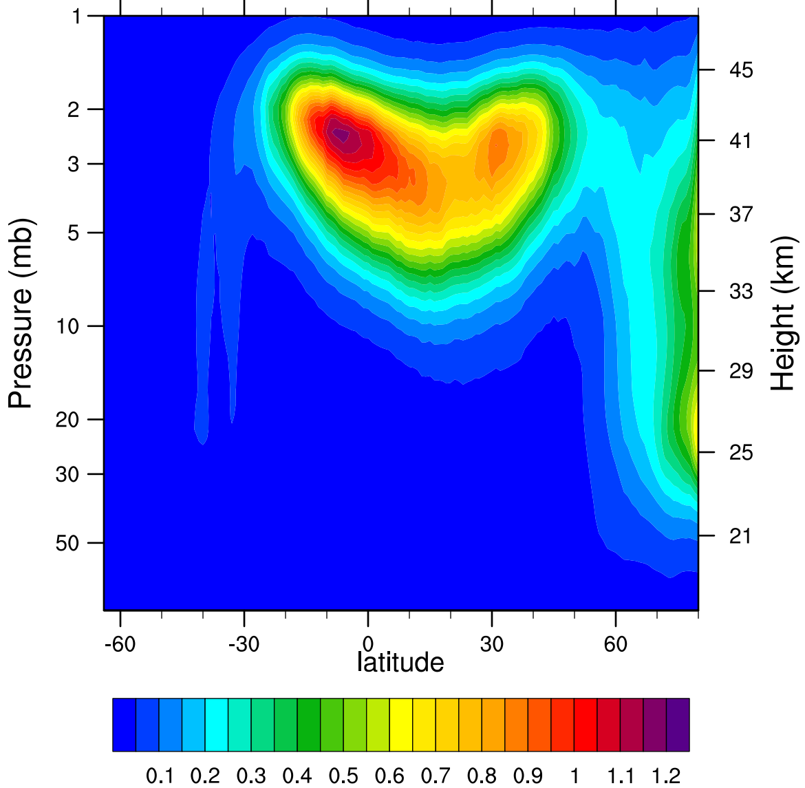
2005d052 N2O5_Ascending (ppbv)
