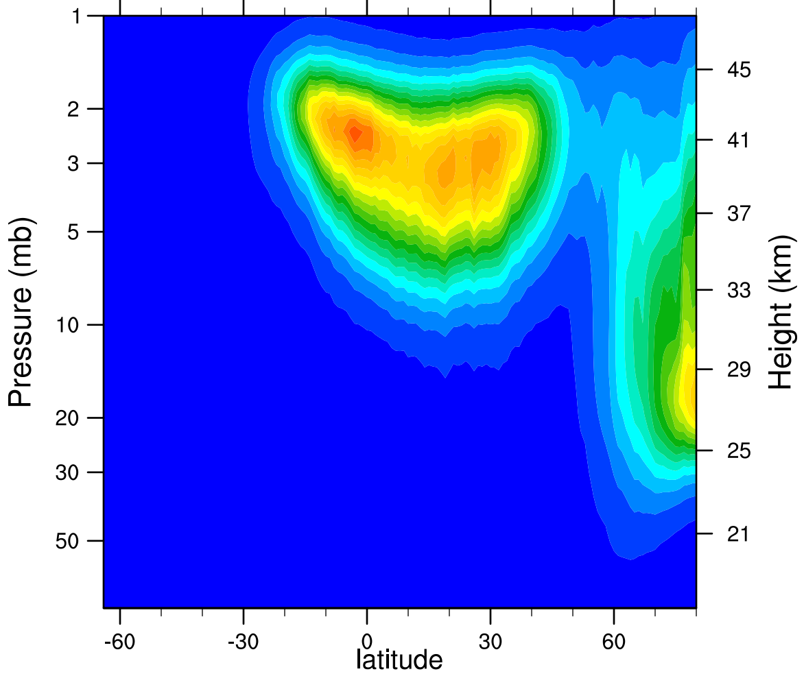
2005d038 N2O5_Ascending (ppbv)
