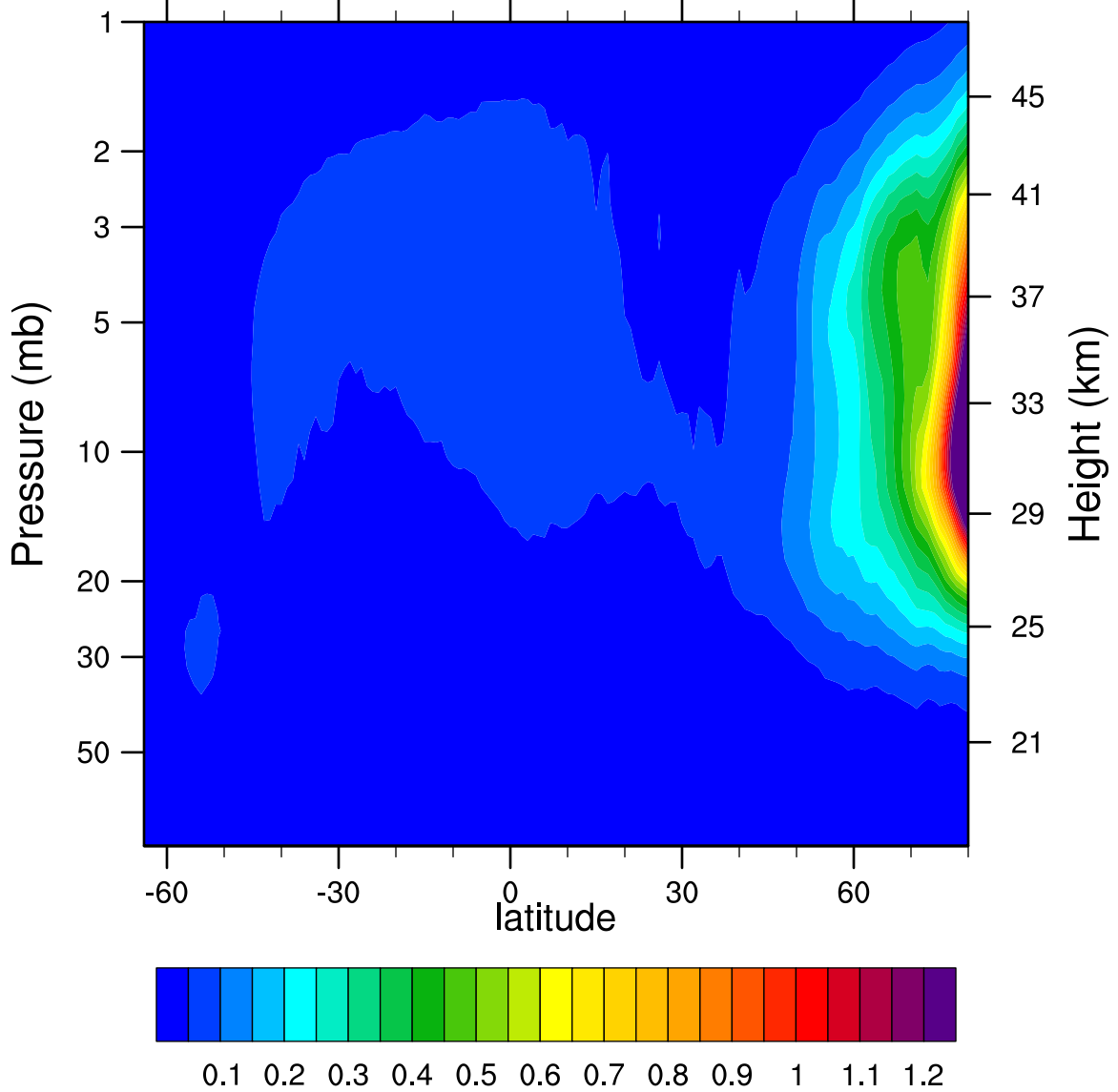
2006d044 N2O5_Ascending (ppbv)
