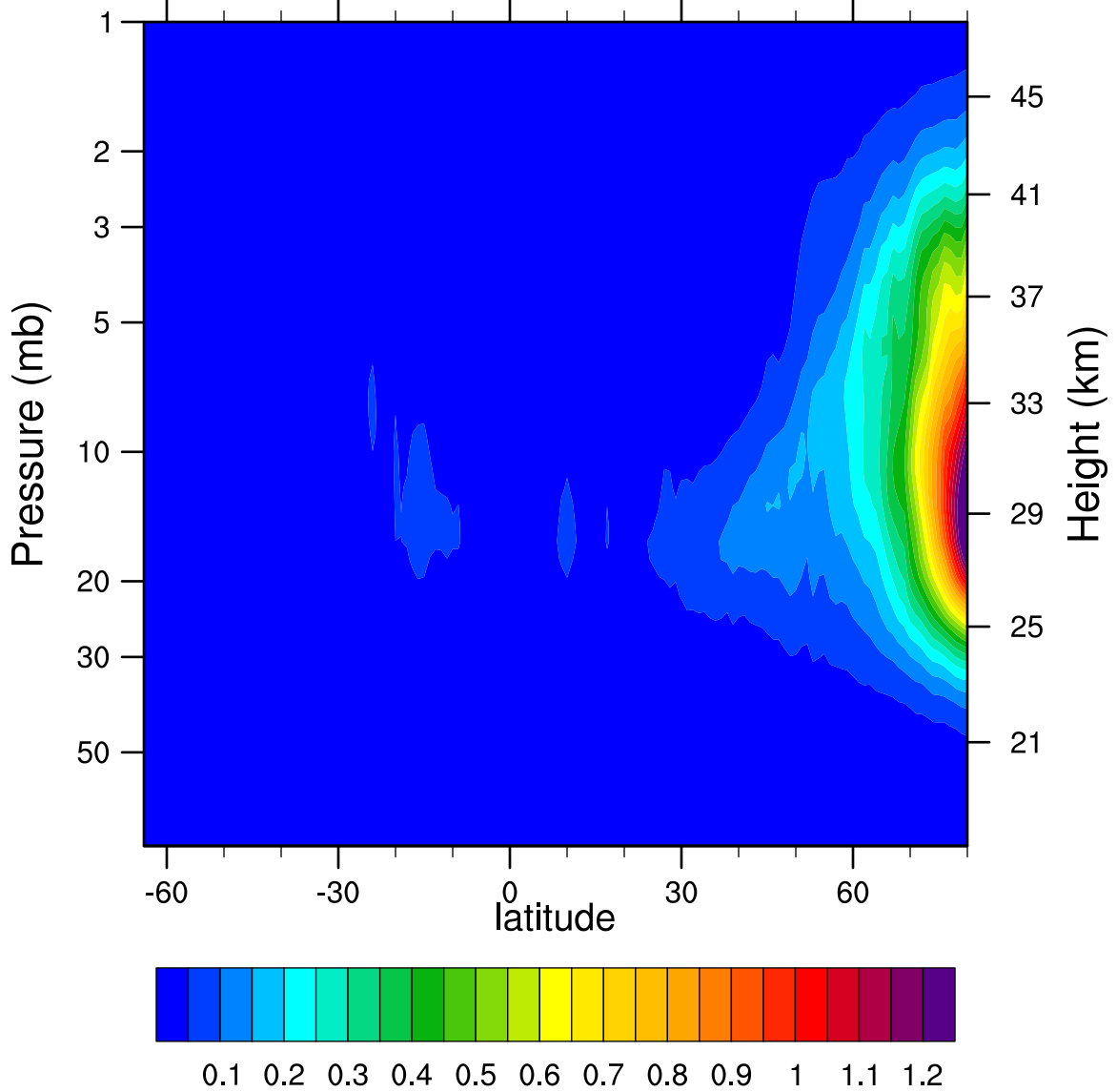
2006d298 N2O5_Ascending (ppbv)
