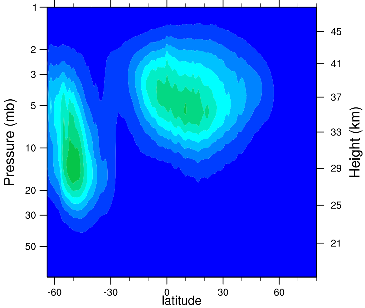
2005d192 N2O5_Ascending (ppbv)
