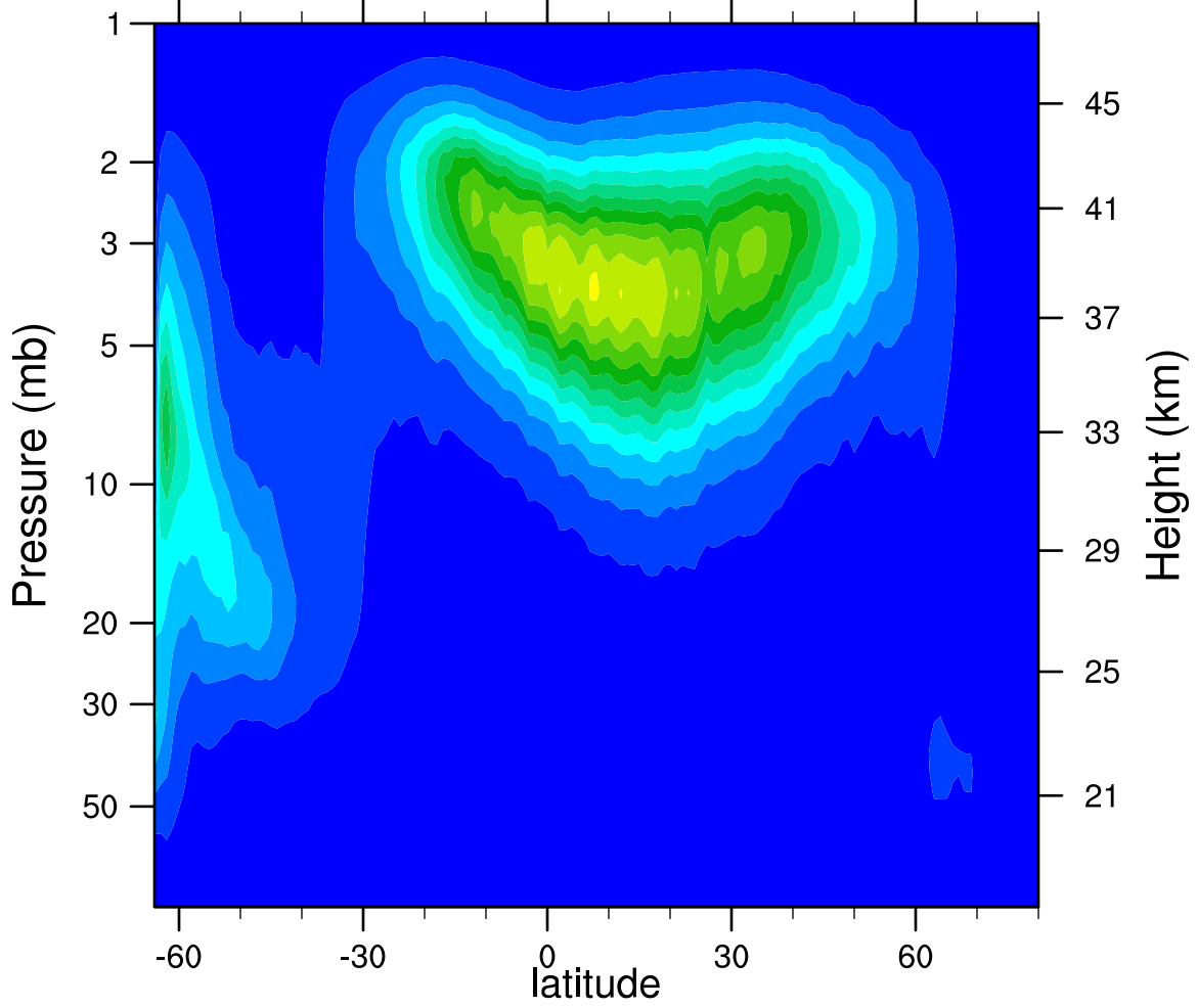
2005d104 N2O5_Ascending (ppbv)
