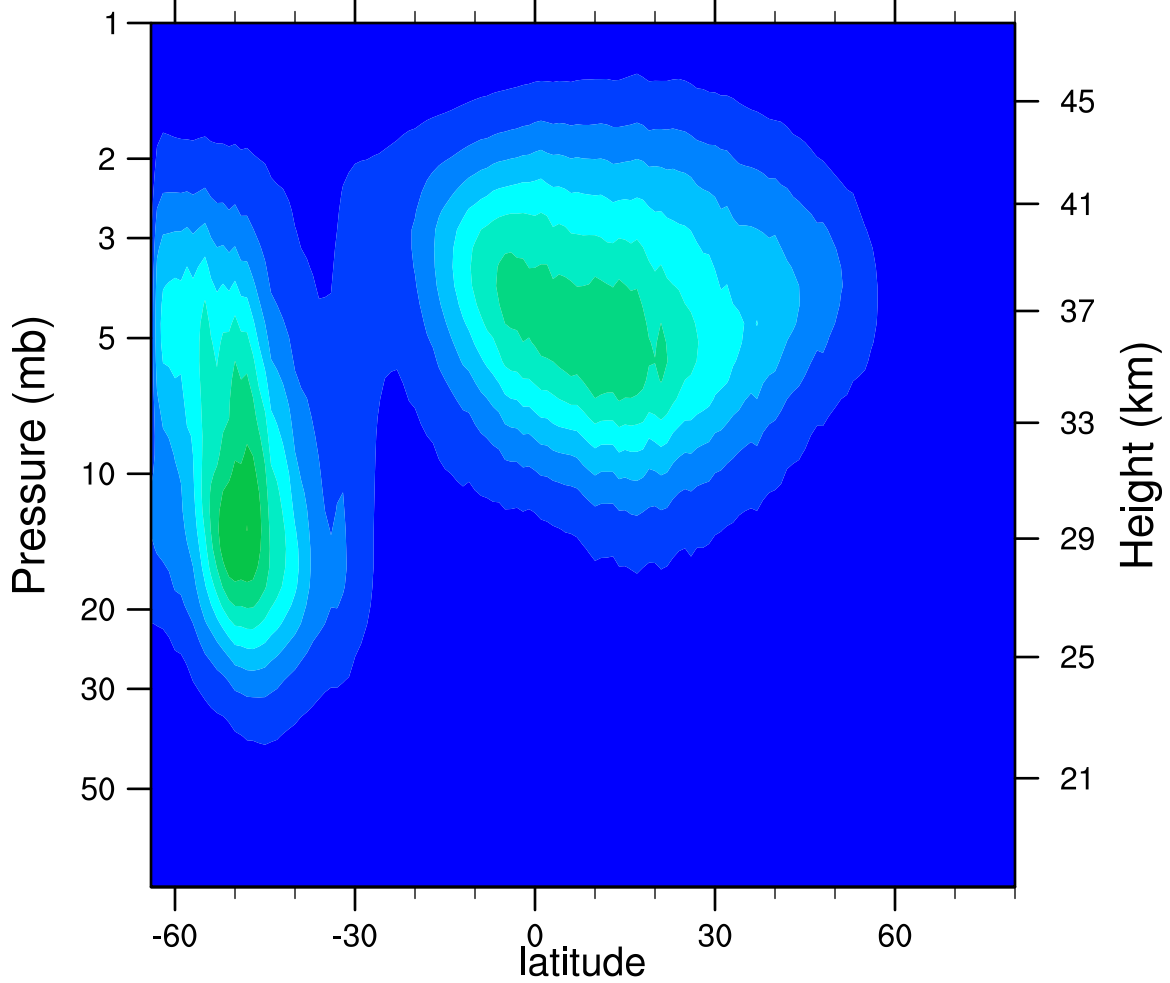
2005d189 N2O5_Ascending (ppbv)
