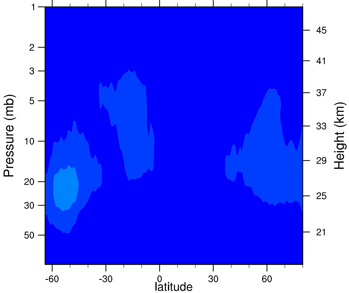
2006d266 N2O5_Ascending (ppbv)
