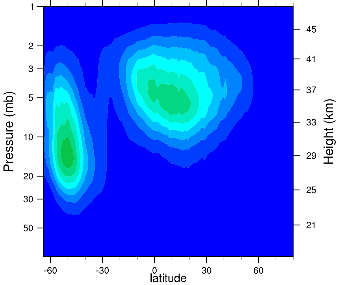
2005d195 N2O5_Ascending (ppbv)
