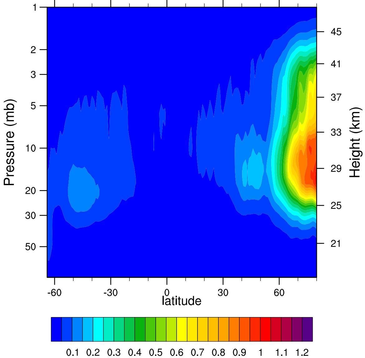
2006d317 N2O5_Ascending (ppbv)
