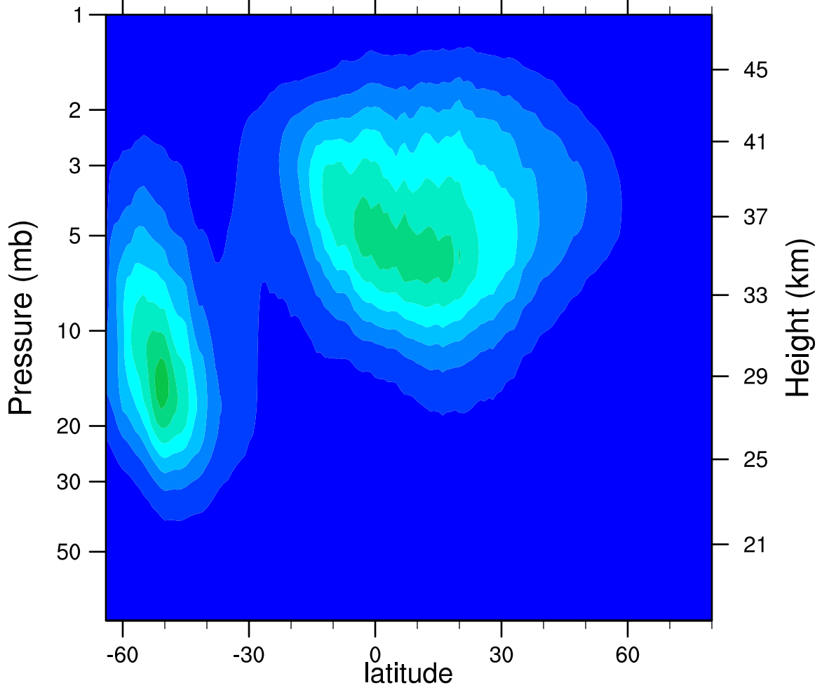
2005d210 N2O5_Ascending (ppbv)
