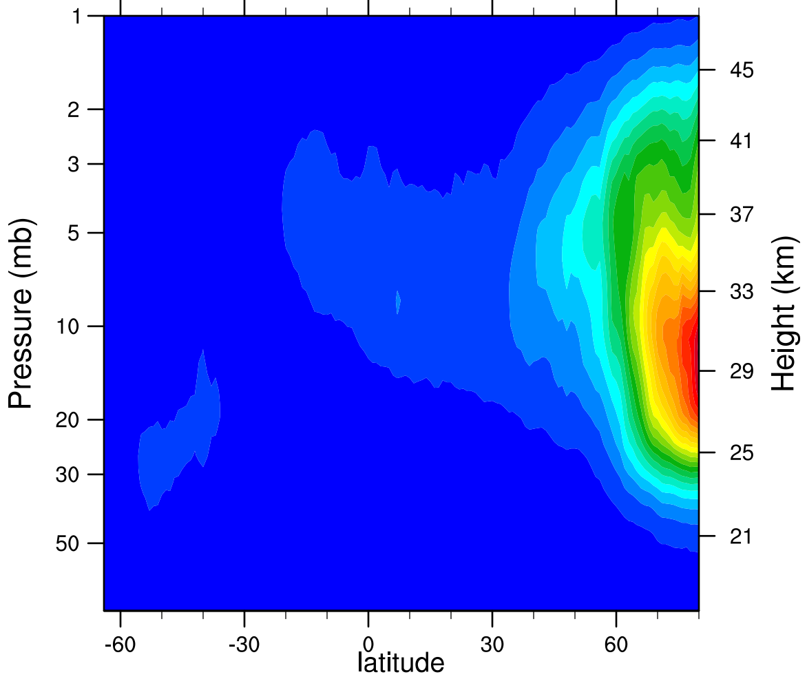
2005d309 N2O5_Ascending (ppbv)
