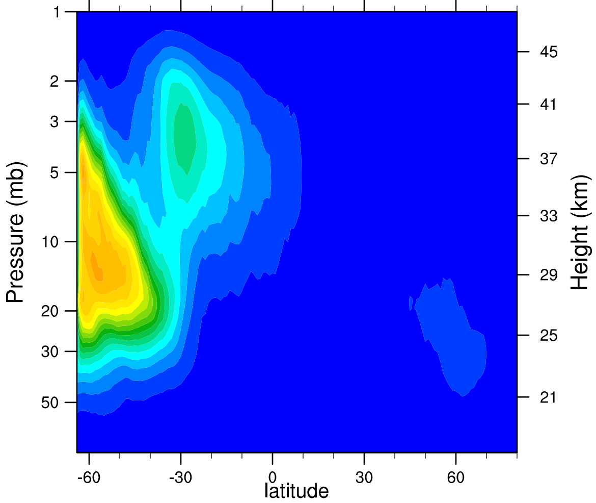
2007d119 N2O5_Ascending (ppbv)
