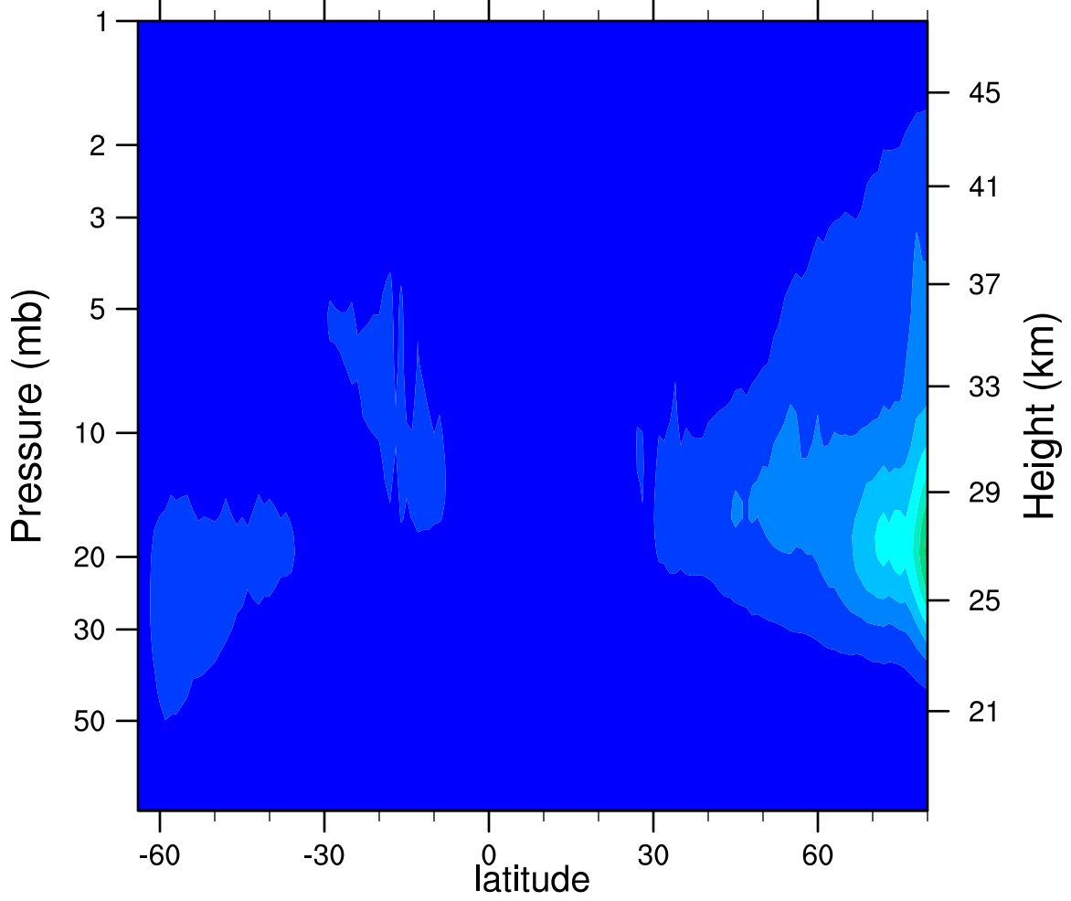
2006d279 N2O5_Ascending (ppbv)
