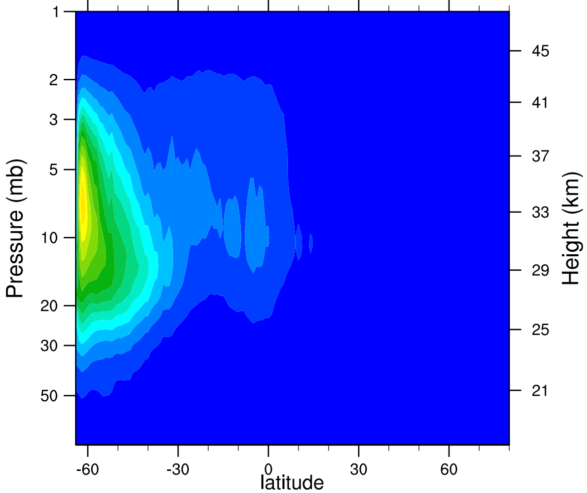
2006d136 N2O5_Ascending (ppbv)
