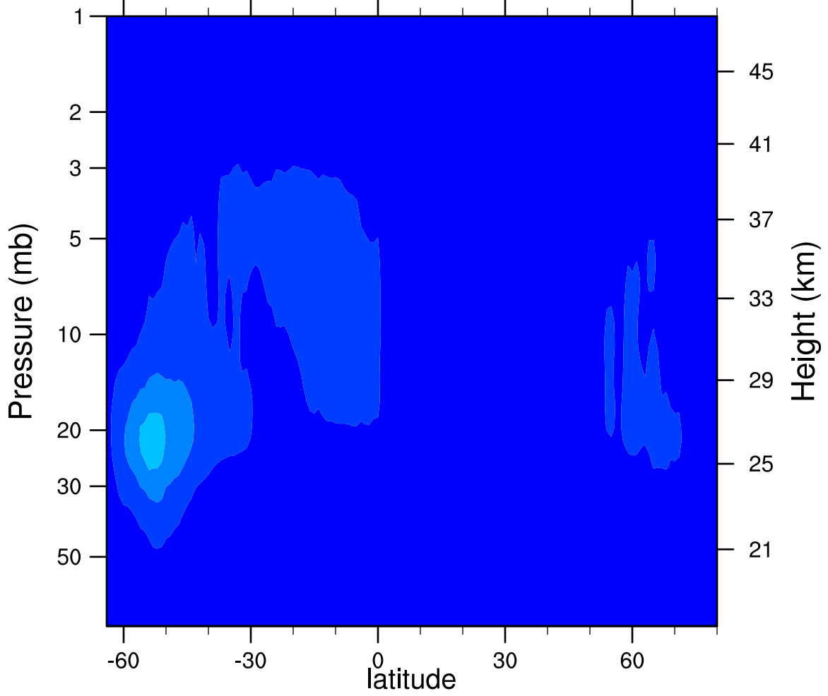
2006d256 N2O5_Ascending (ppbv)
