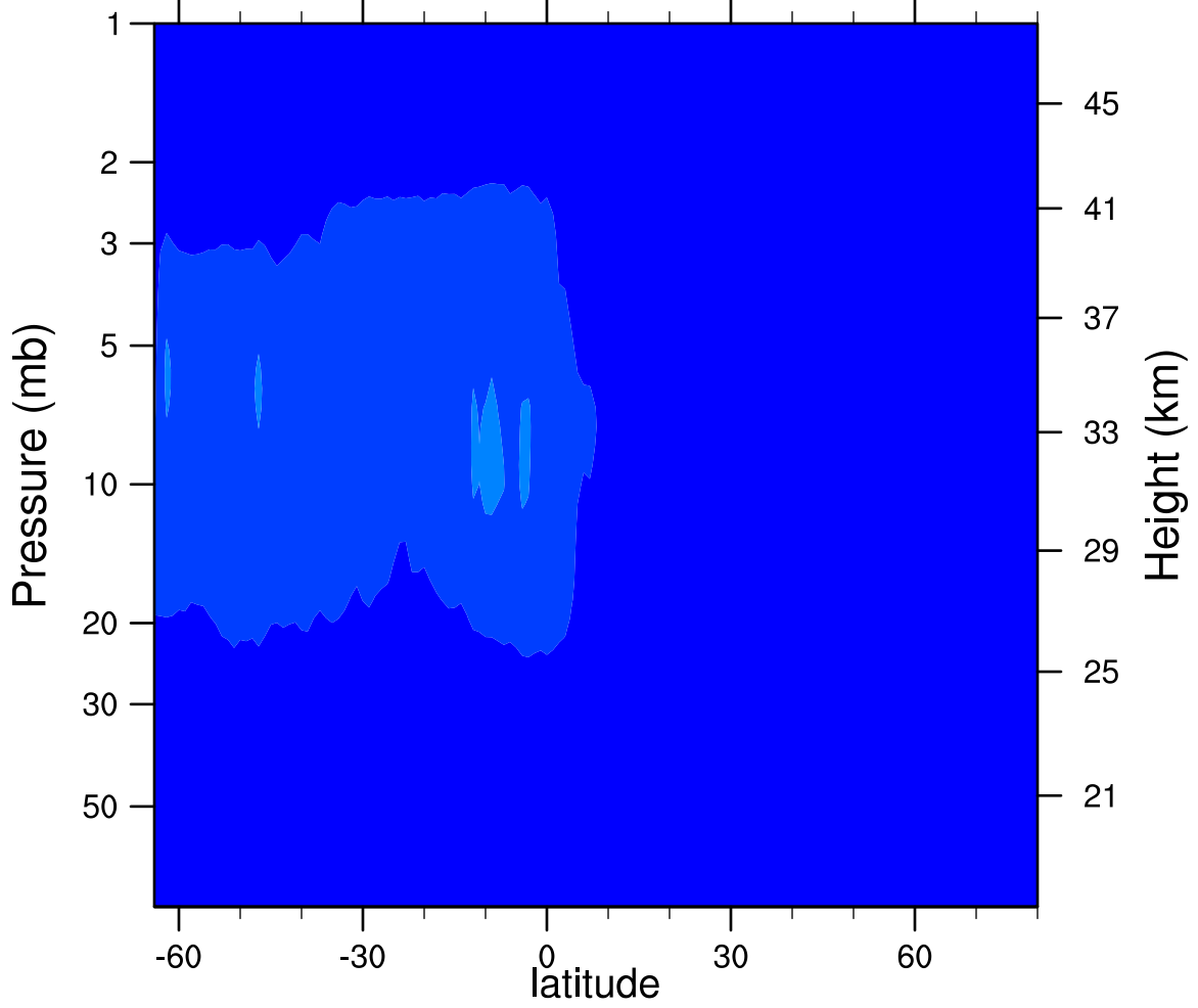
2006d182 N2O5_Ascending (ppbv)
