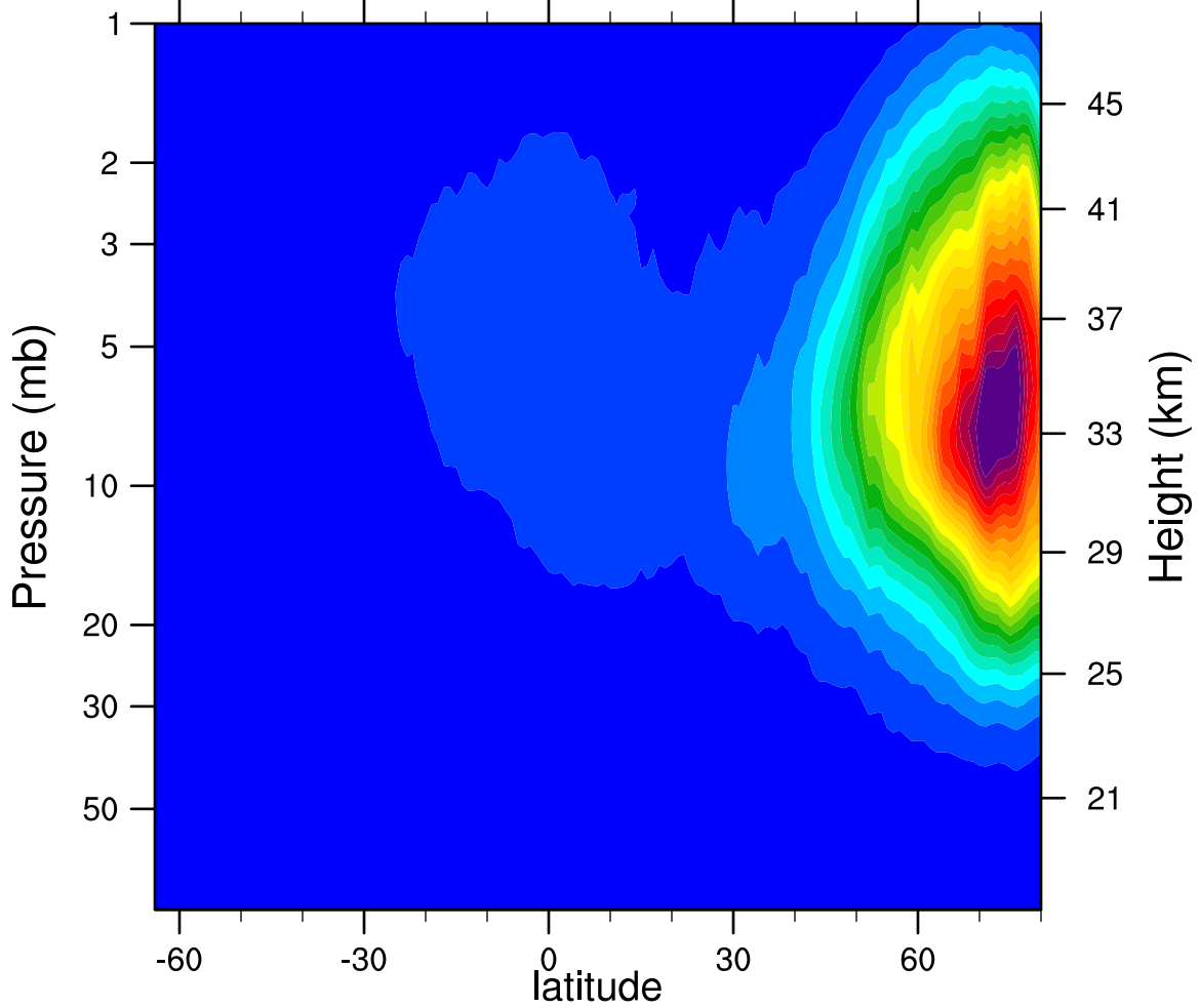
2005d346 N2O5_Ascending (ppbv)
