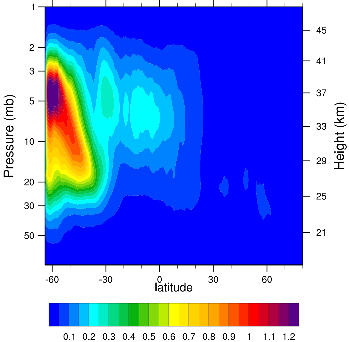
2007d138 N2O5_Ascending (ppbv)
