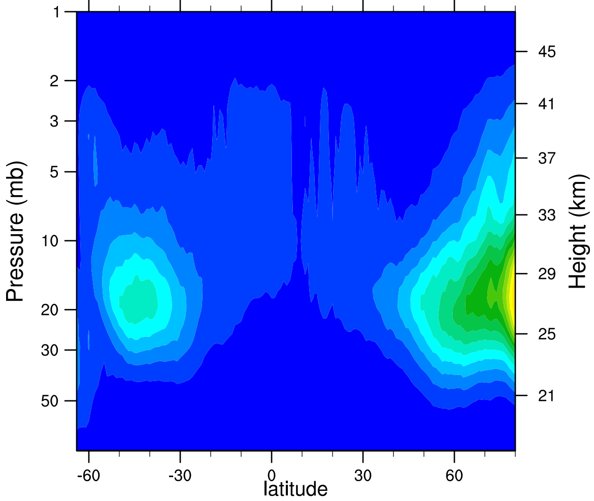
2007d277 N2O5_Ascending (ppbv)
