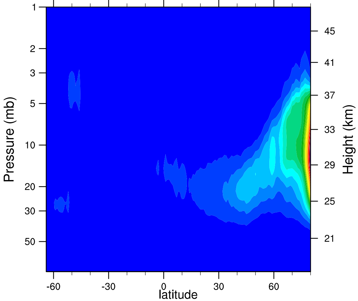
2007d056 N2O5_Ascending (ppbv)
