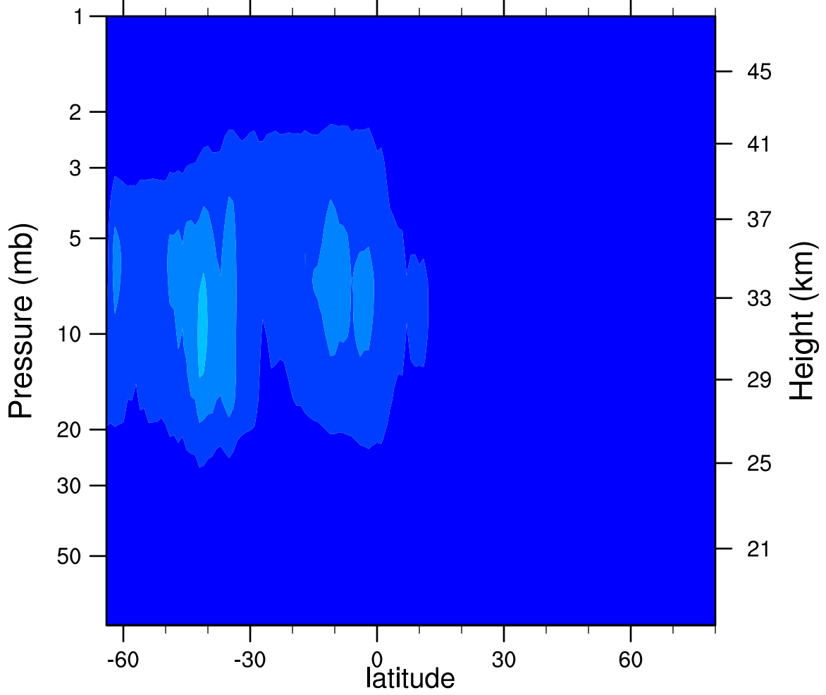
2006d189 N2O5_Ascending (ppbv)
