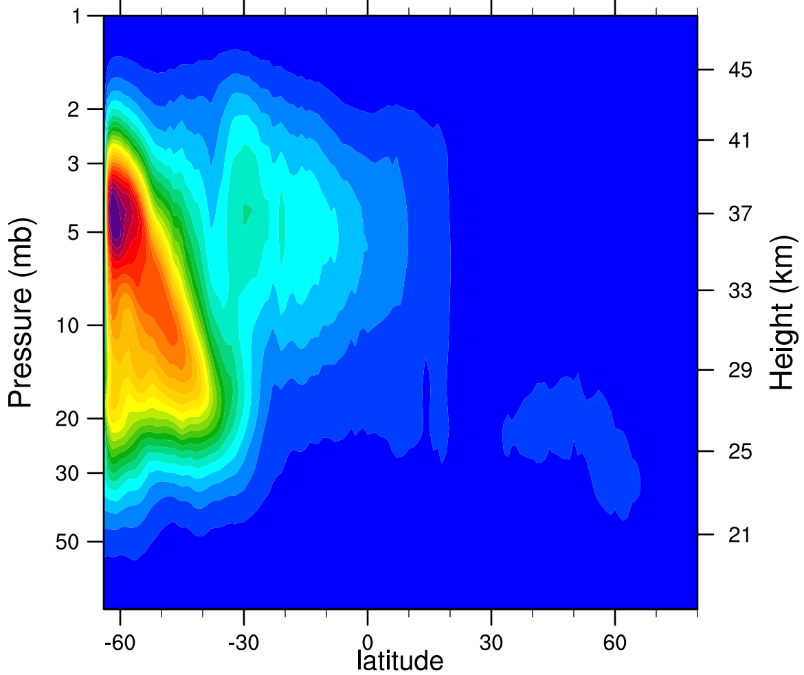
2007d131 N2O5_Ascending (ppbv)
