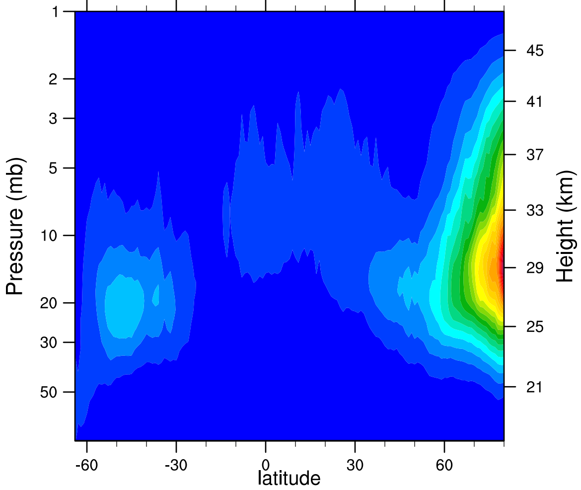
2007d295 N2O5_Ascending (ppbv)
