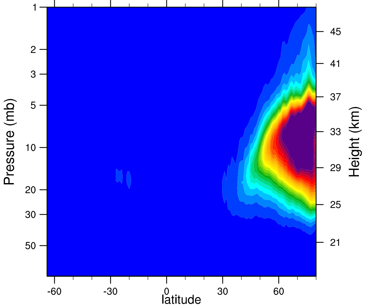
2006d359 N2O5_Ascending (ppbv)
