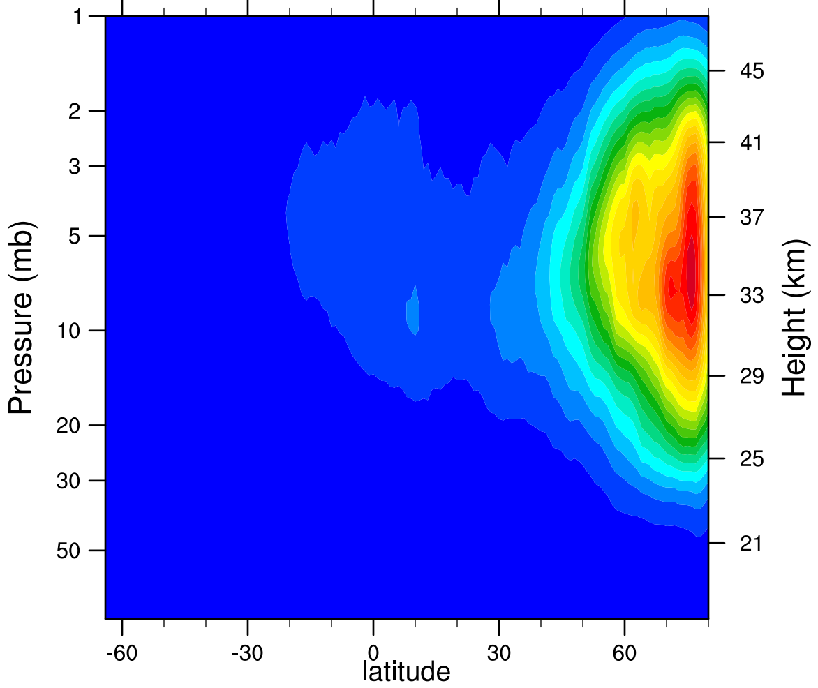
2005d336 N2O5_Ascending (ppbv)
