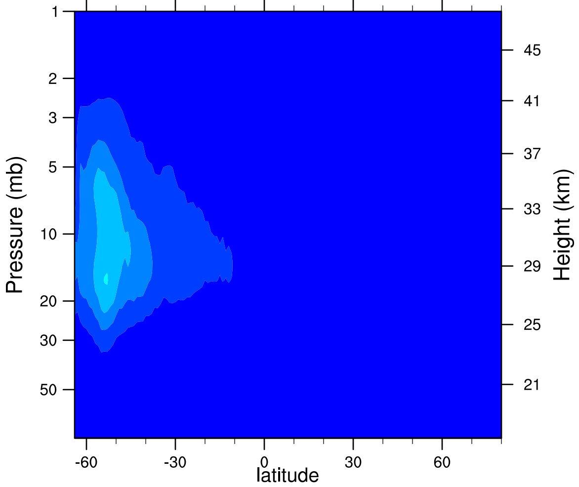
2007d194 N2O5_Ascending (ppbv)
