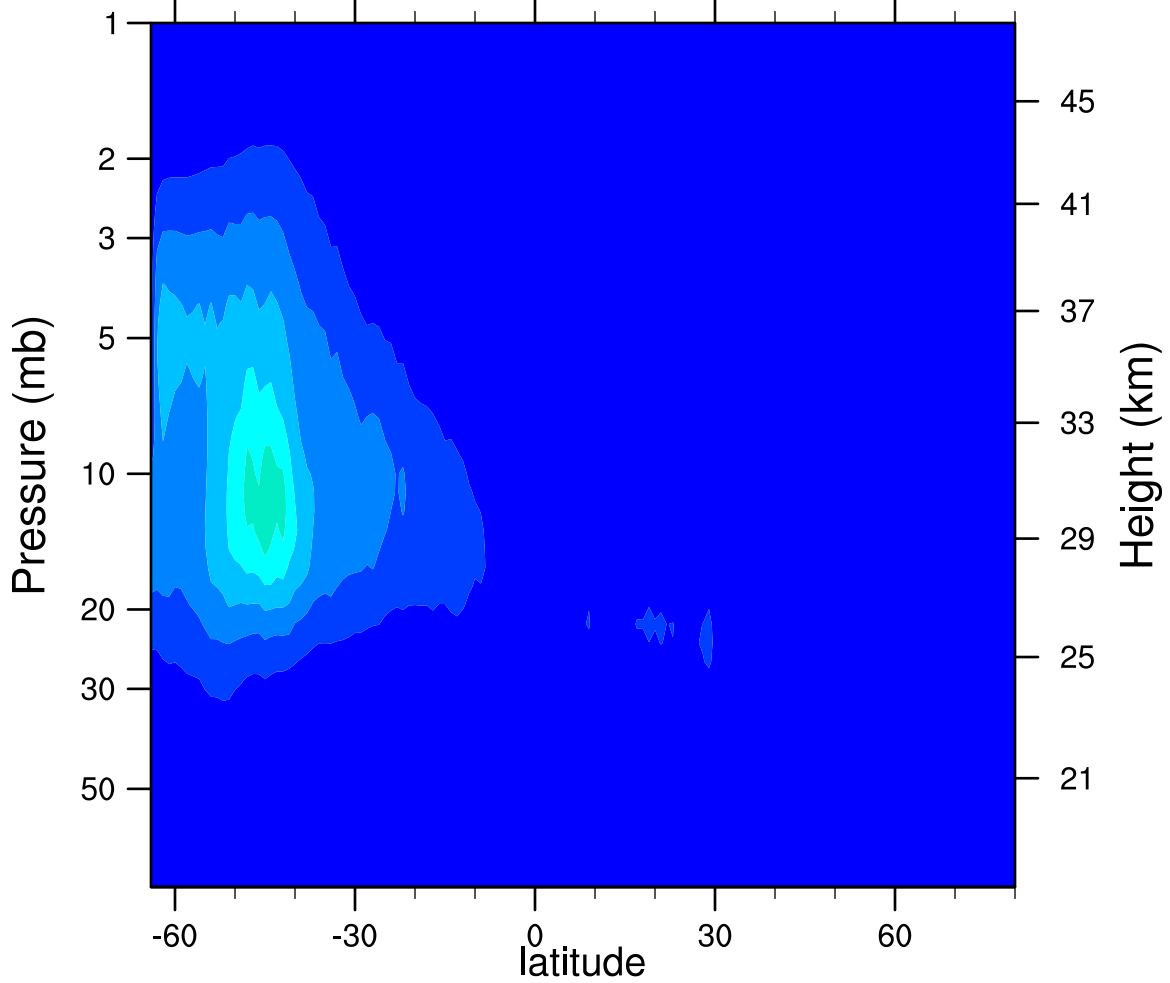
2007d177 N2O5_Ascending (ppbv)
