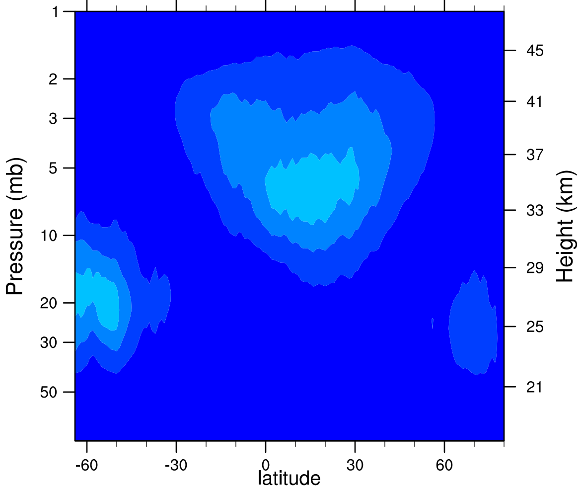
2005d253 N2O5_Ascending (ppbv)
