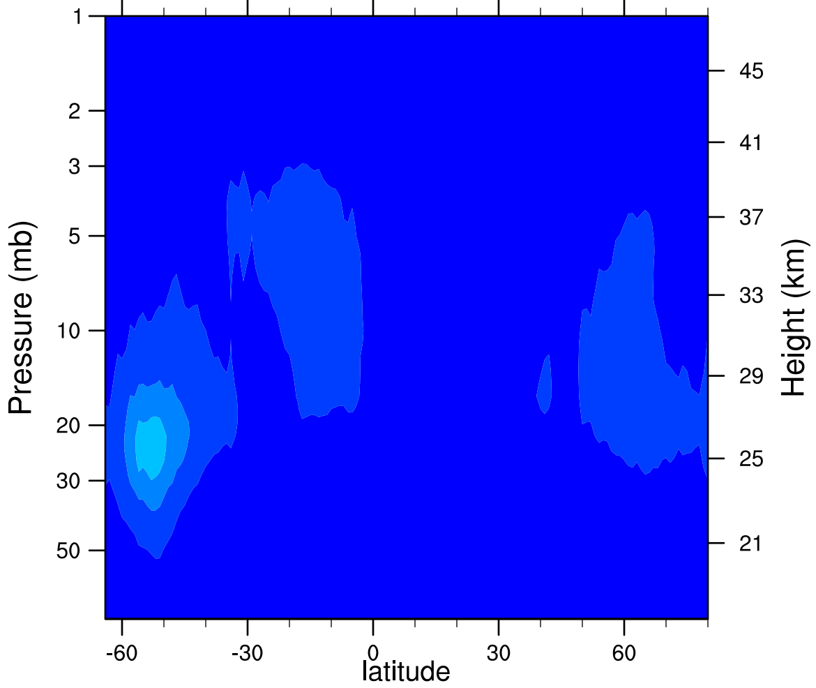
2006d263 N2O5_Ascending (ppbv)
