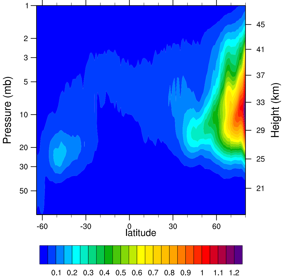
2006d328 N2O5_Ascending (ppbv)
