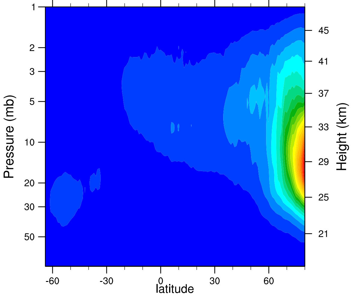
2005d298 N2O5_Ascending (ppbv)
