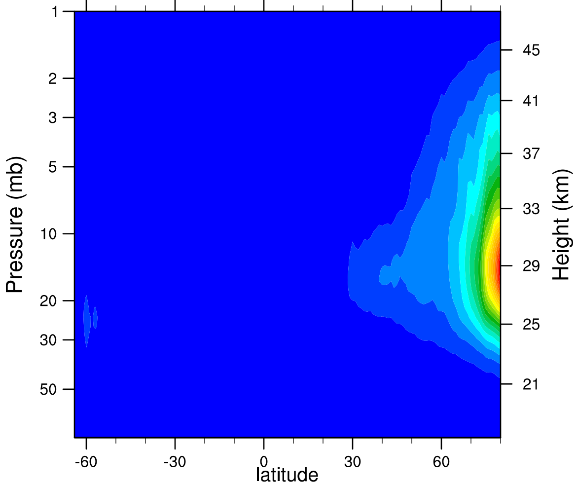
2006d291 N2O5_Ascending (ppbv)
