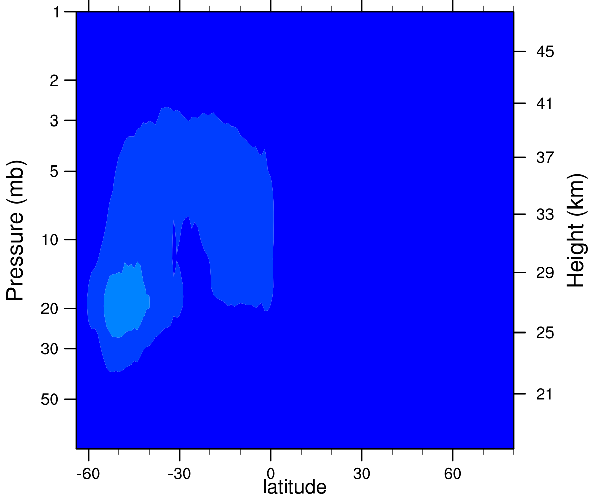
2006d247 N2O5_Ascending (ppbv)
