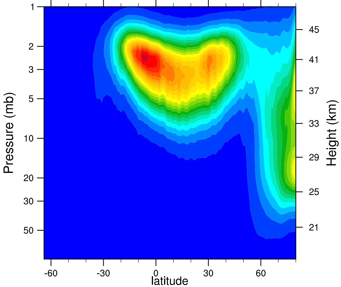
2005d048 N2O5_Ascending (ppbv)
