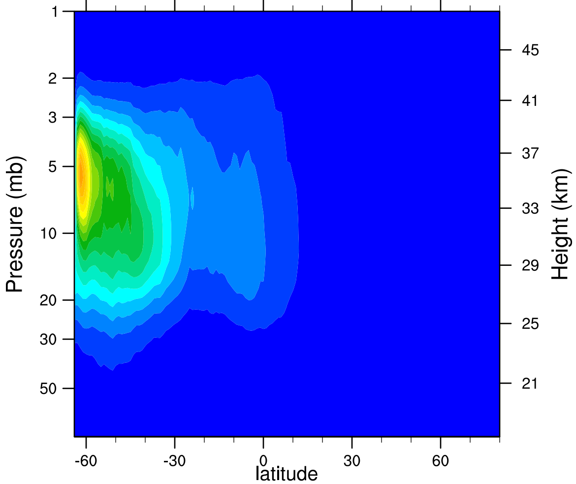
2006d168 N2O5_Ascending (ppbv)
