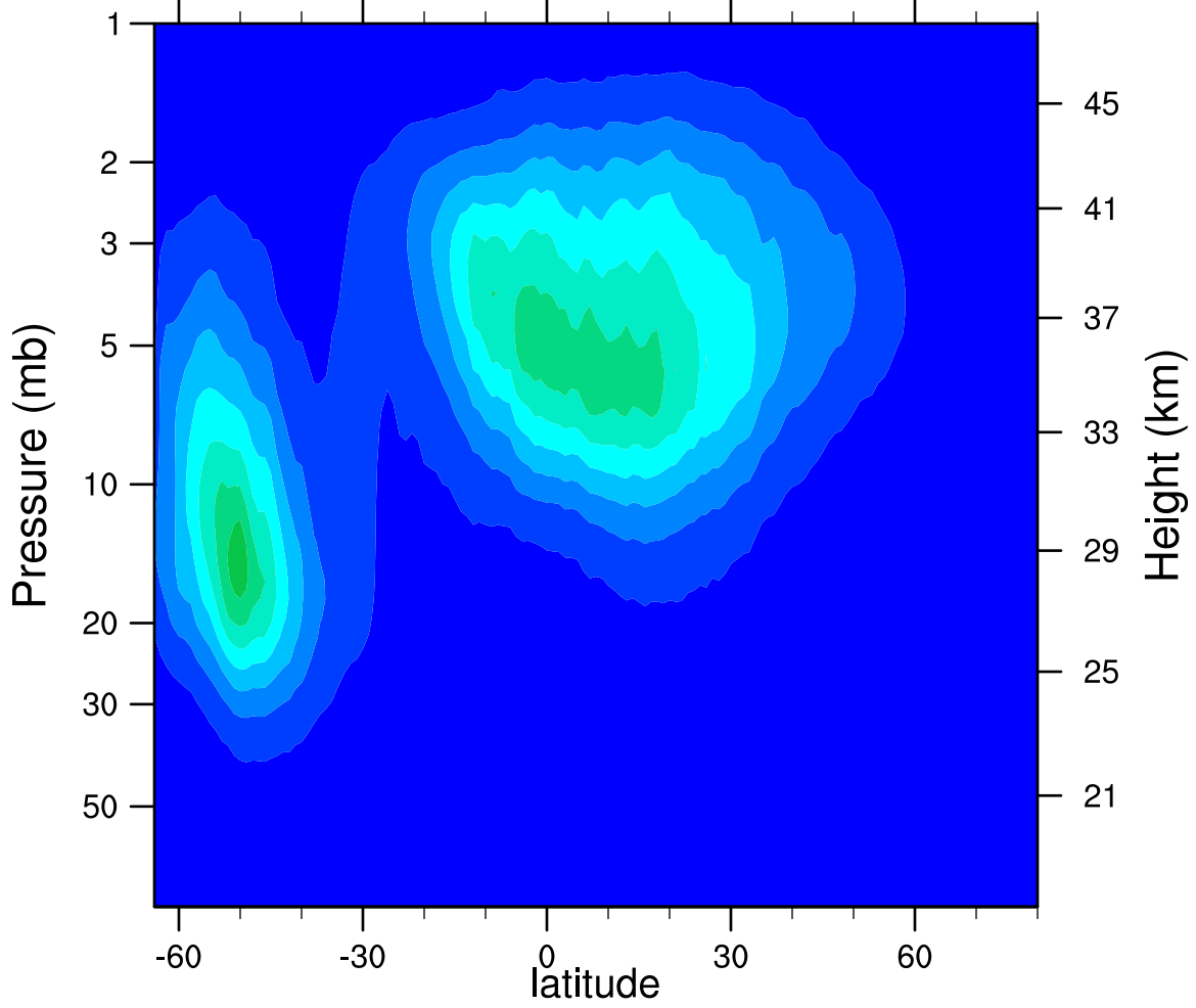
2005d209 N2O5_Ascending (ppbv)
