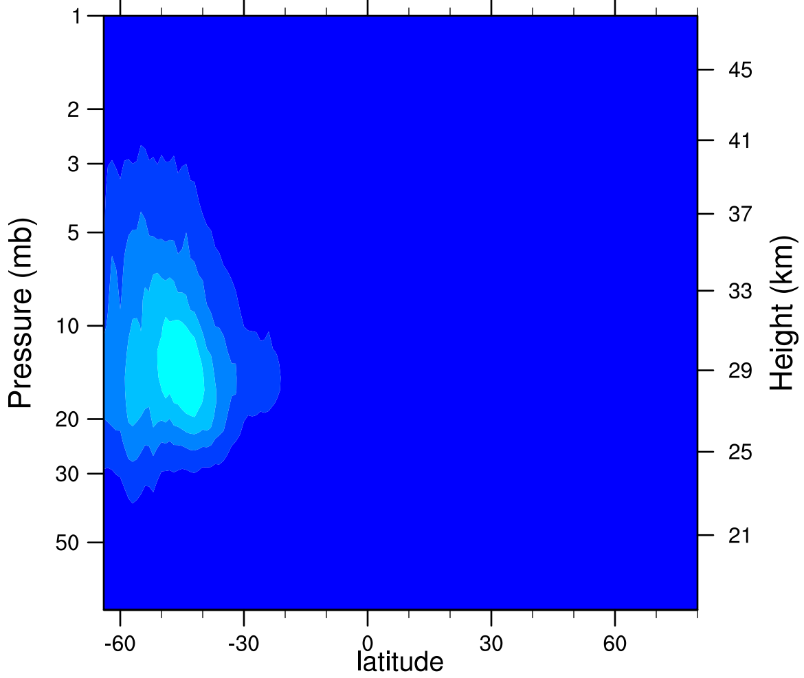
2007d209 N2O5_Ascending (ppbv)
