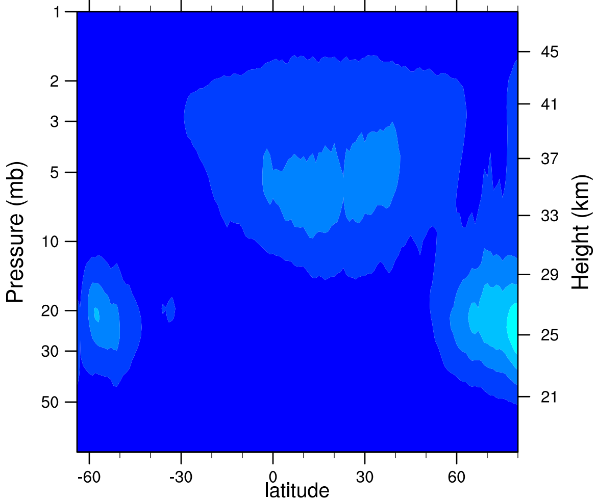
2005d275 N2O5_Ascending (ppbv)
