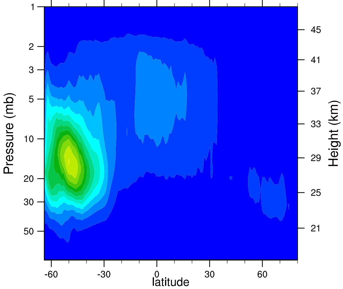
2007d233 N2O5_Ascending (ppbv)
