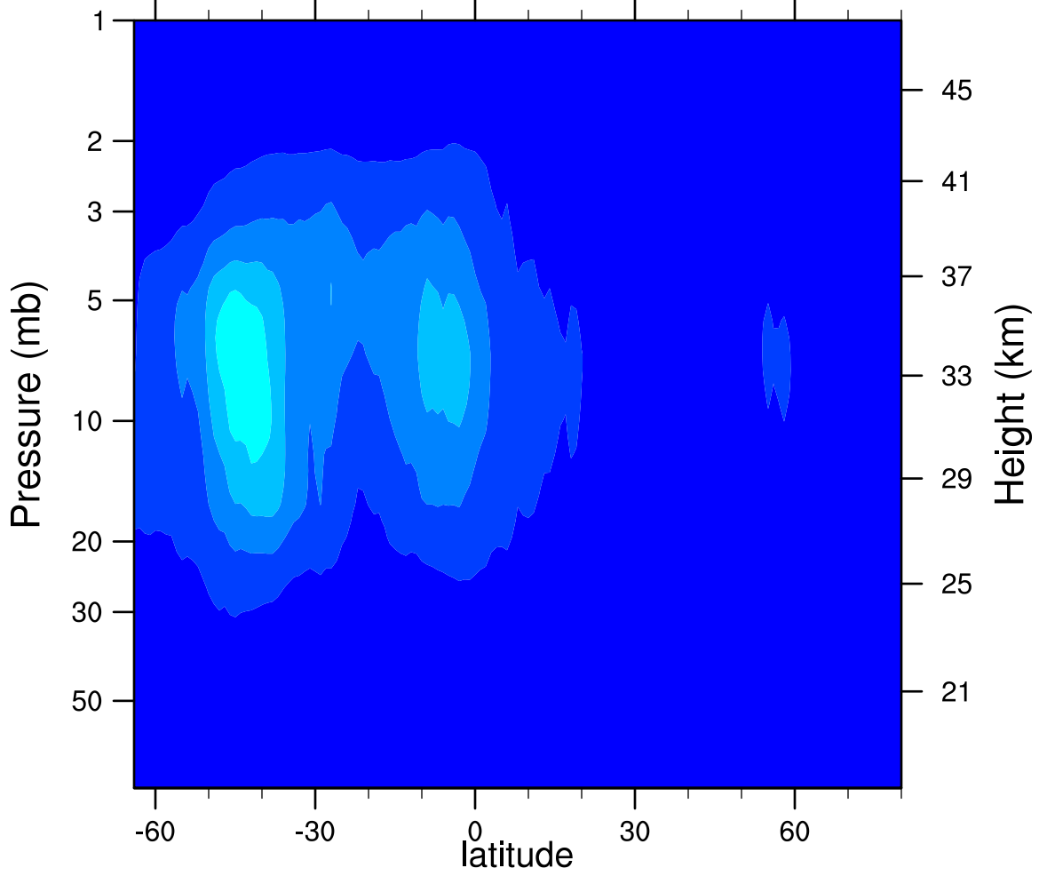
2006d204 N2O5_Ascending (ppbv)
