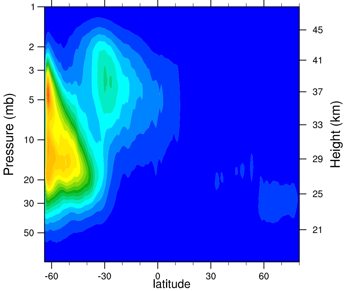
2007d113 N2O5_Ascending (ppbv)
