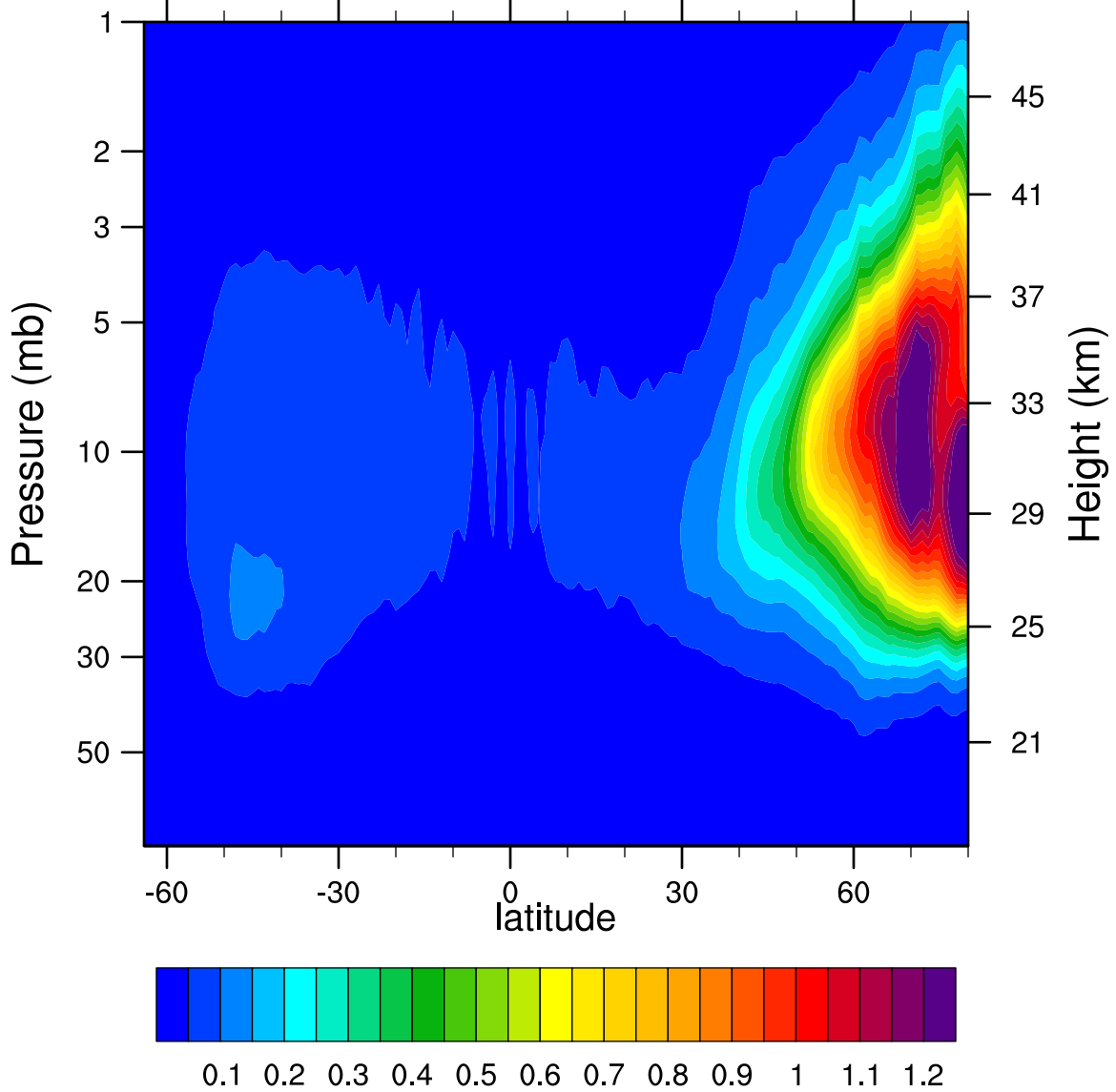
2006d348 N2O5_Ascending (ppbv)
