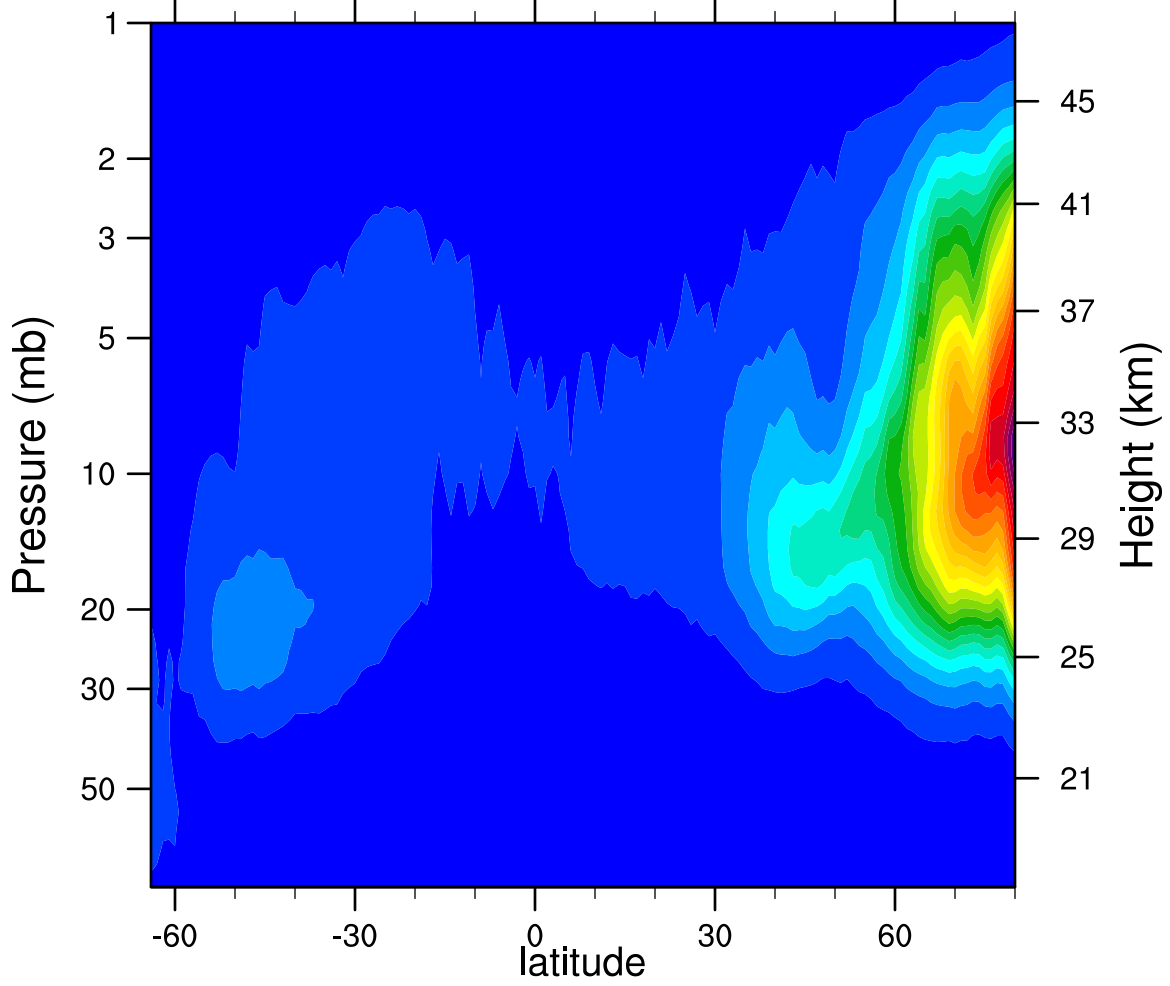
2006d324 N2O5_Ascending (ppbv)
