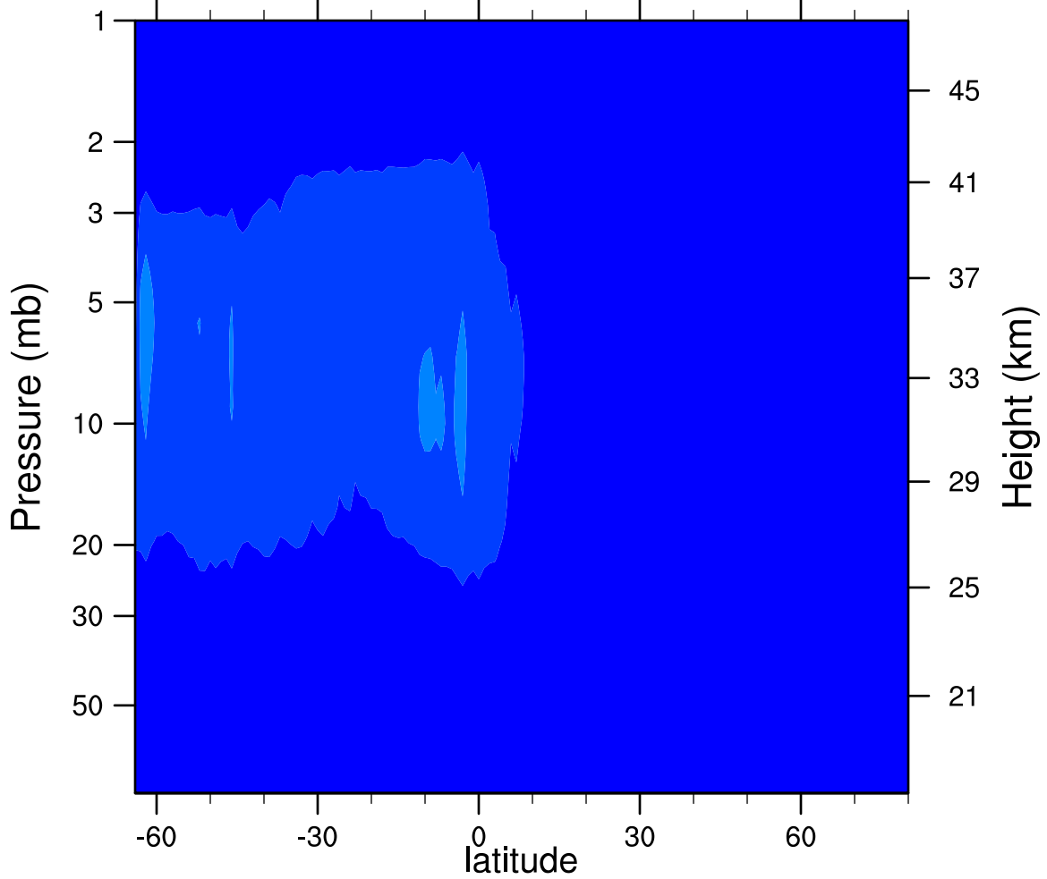
2006d180 N2O5_Ascending (ppbv)
