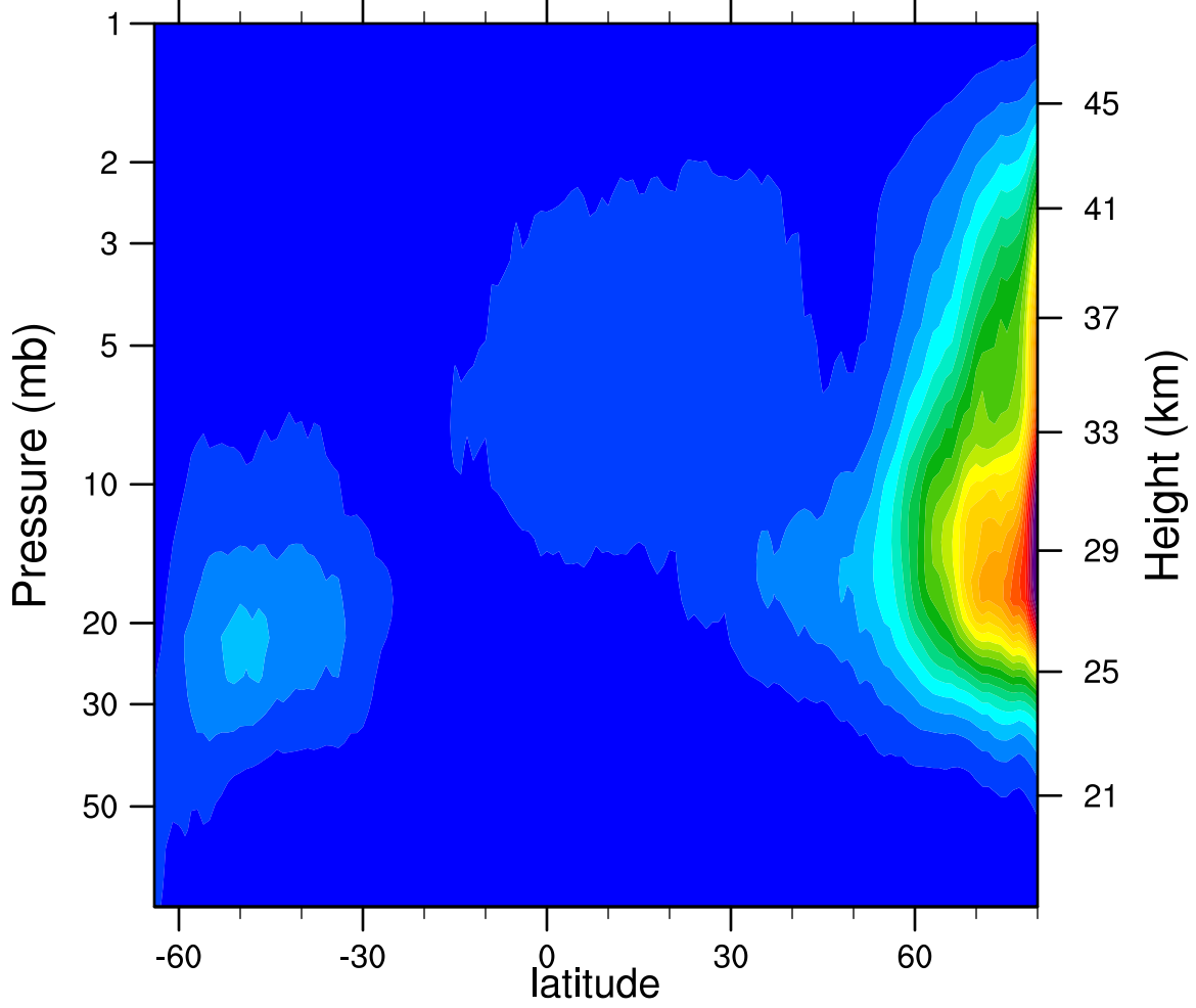
2007d307 N2O5_Ascending (ppbv)
