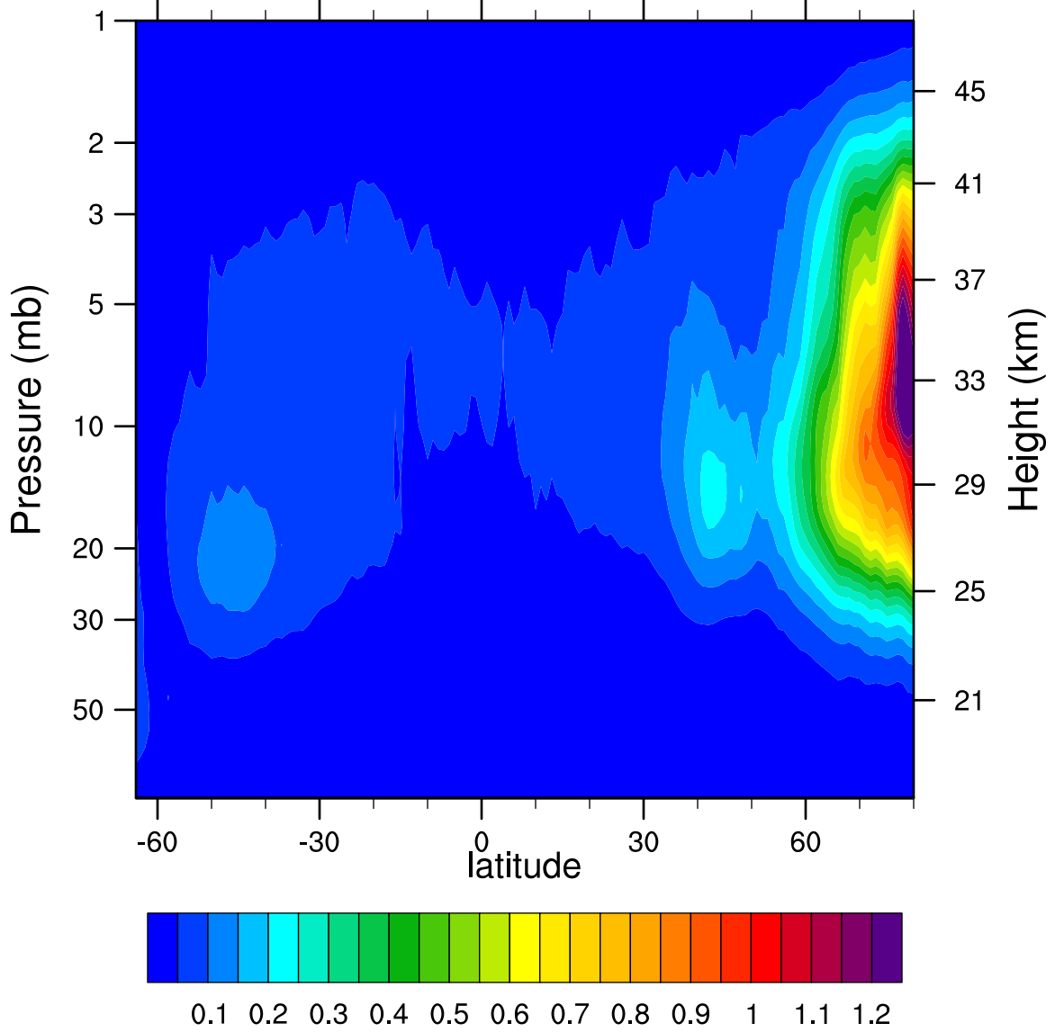
2006d320 N2O5_Ascending (ppbv)
