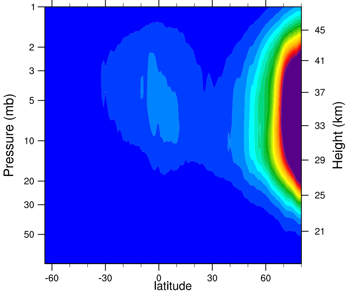
2006d022 N2O5_Ascending (ppbv)
