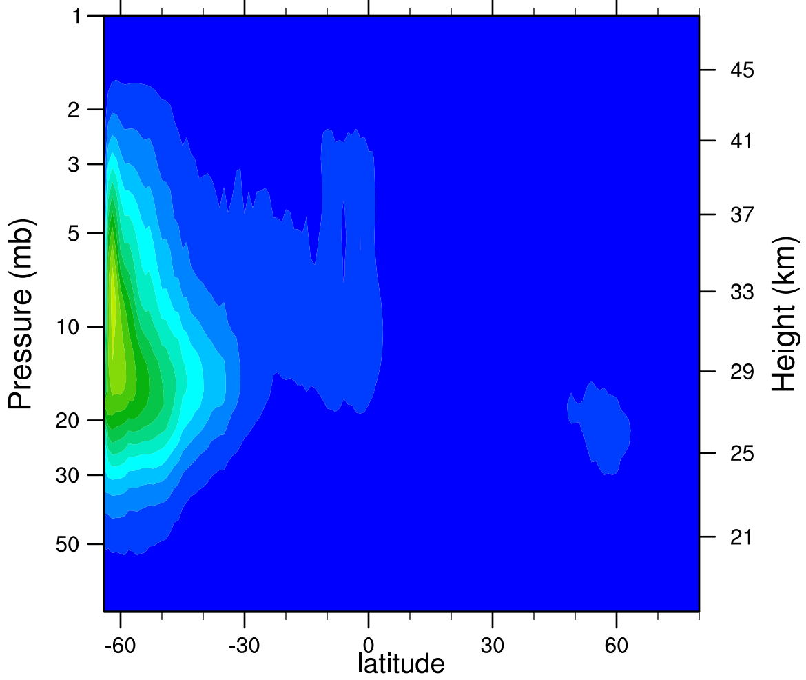
2006d121 N2O5_Ascending (ppbv)
