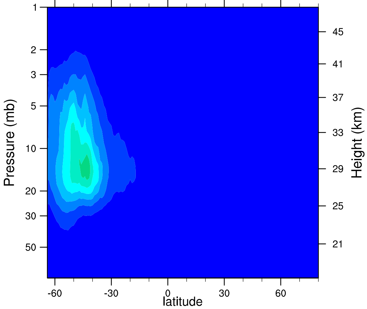
2007d204 N2O5_Ascending (ppbv)
