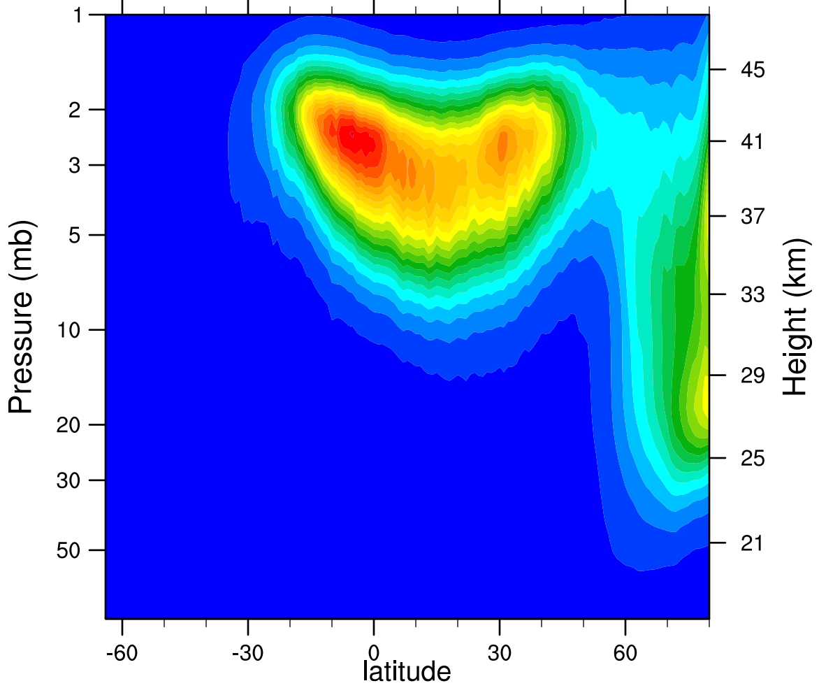
2005d047 N2O5_Ascending (ppbv)
