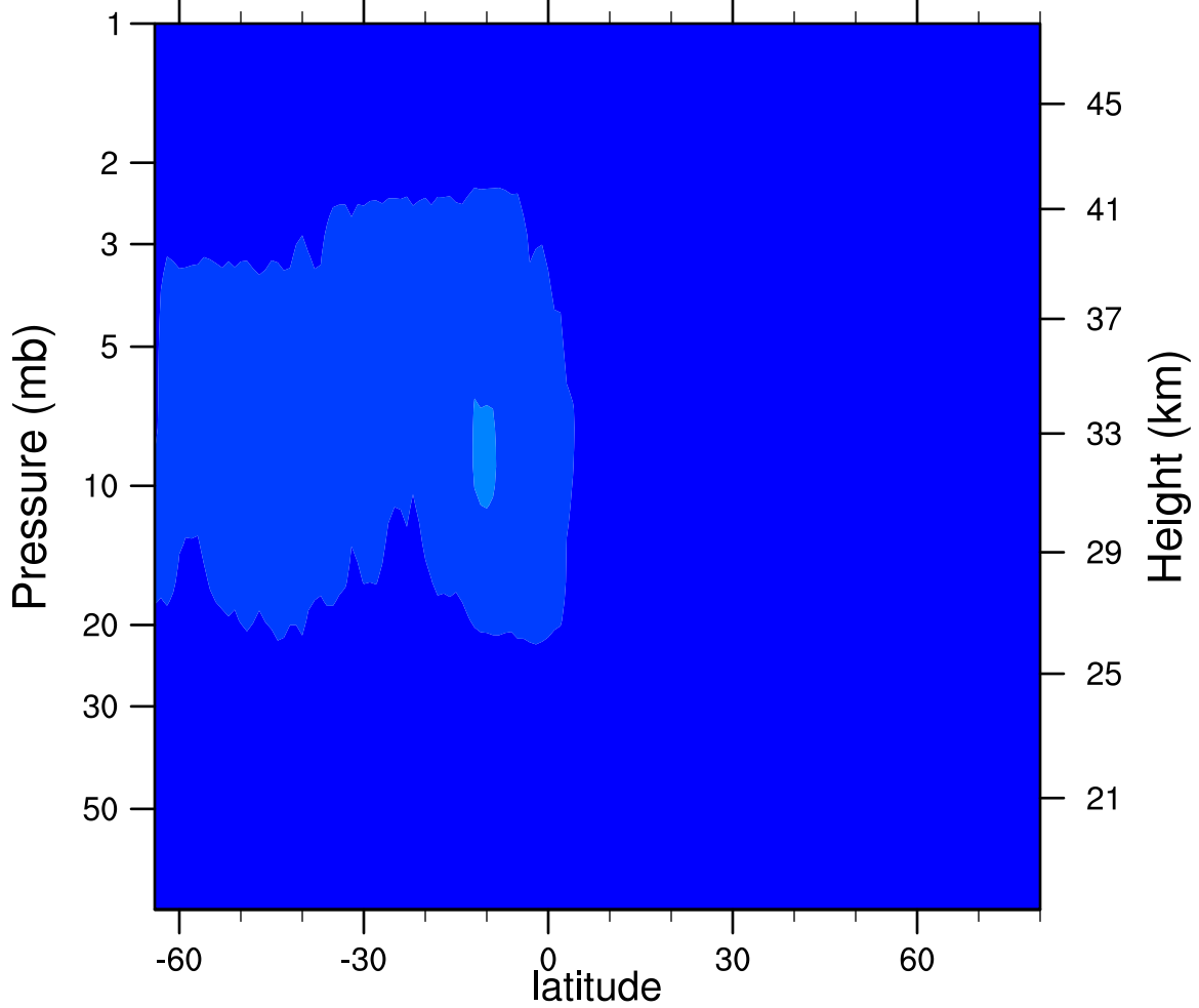
2006d185 N2O5_Ascending (ppbv)
