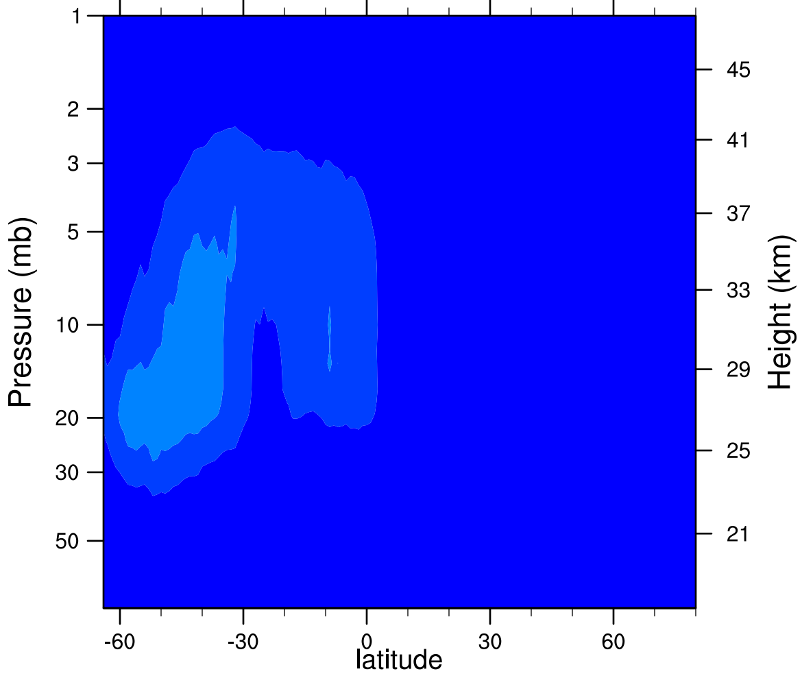
2006d232 N2O5_Ascending (ppbv)
