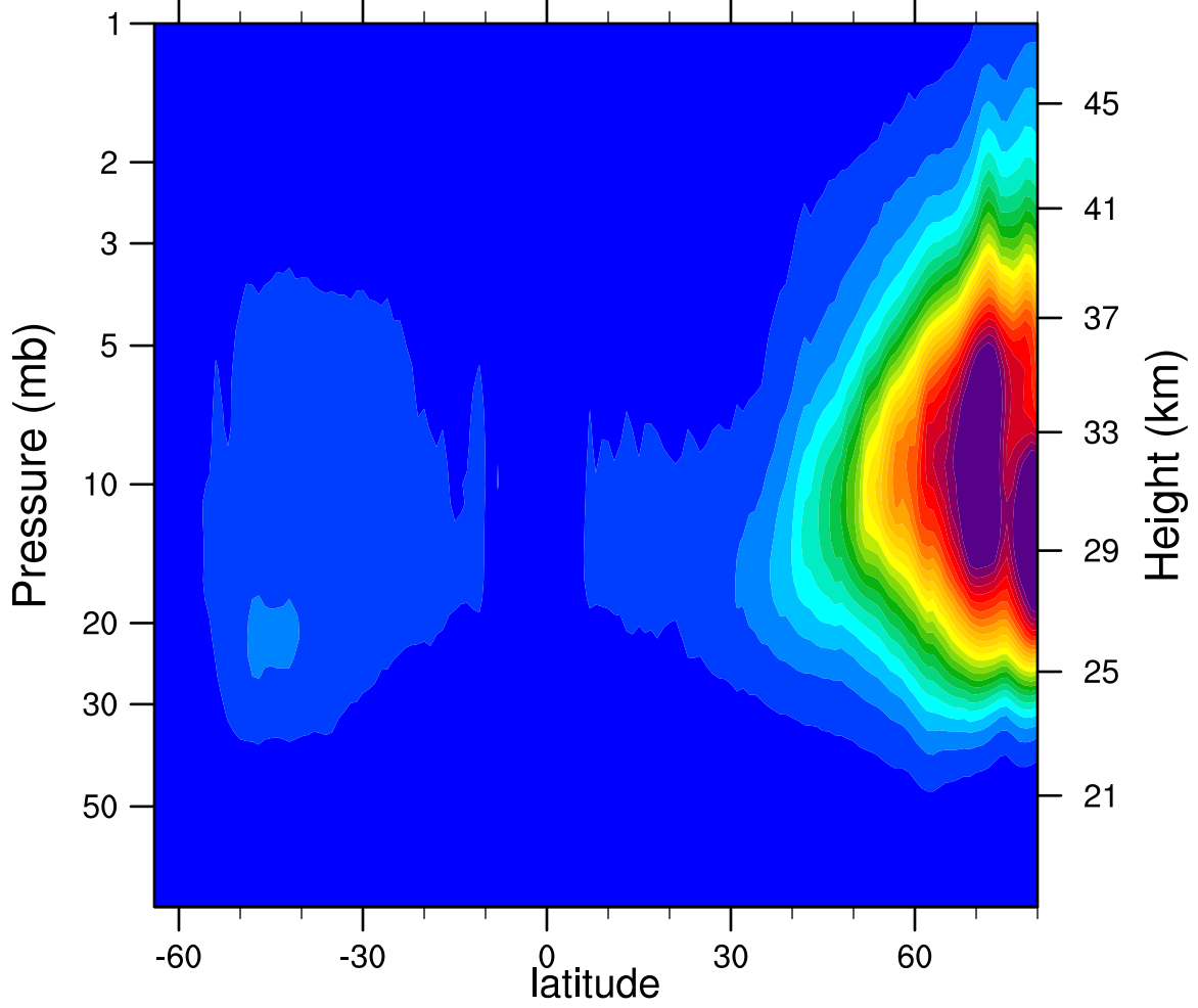
2006d350 N2O5_Ascending (ppbv)
