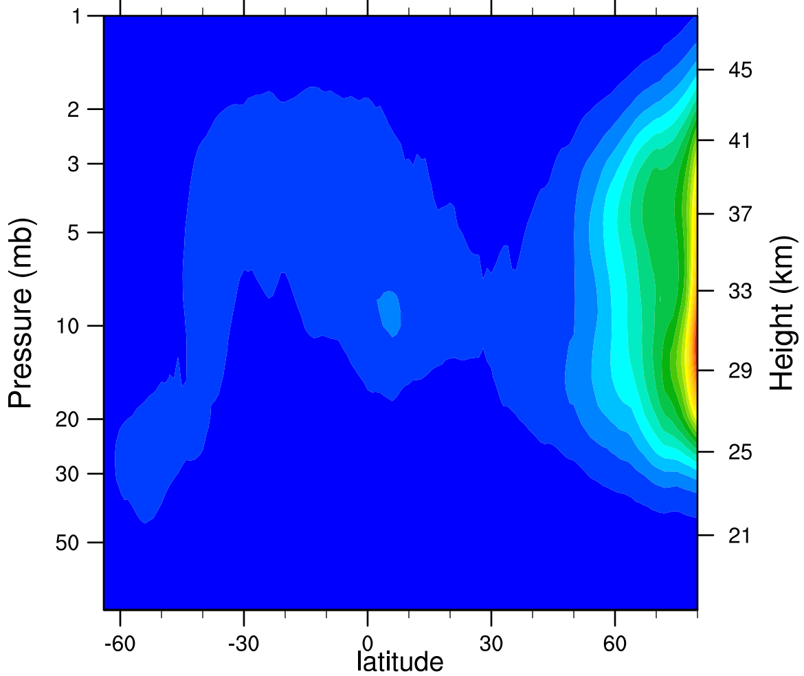
2006d053 N2O5_Ascending (ppbv)
