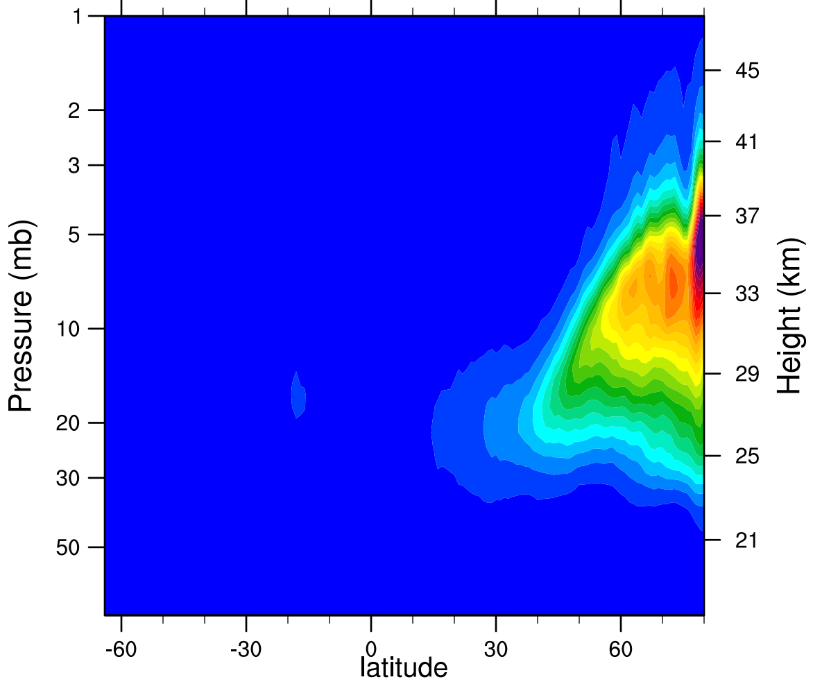
2007d027 N2O5_Ascending (ppbv)
