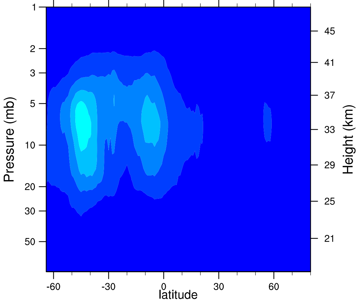
2006d207 N2O5_Ascending (ppbv)
