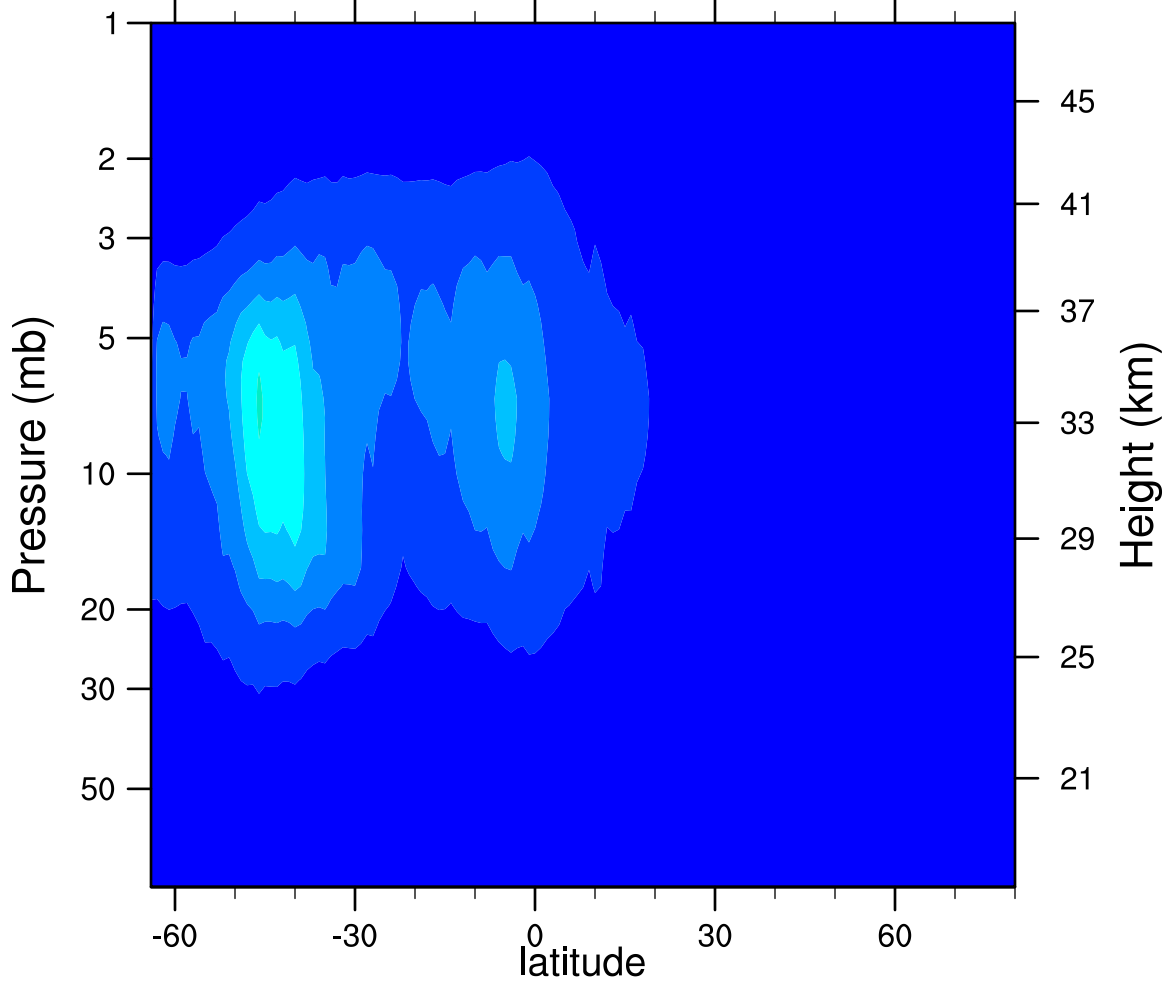
2006d196 N2O5_Ascending (ppbv)
