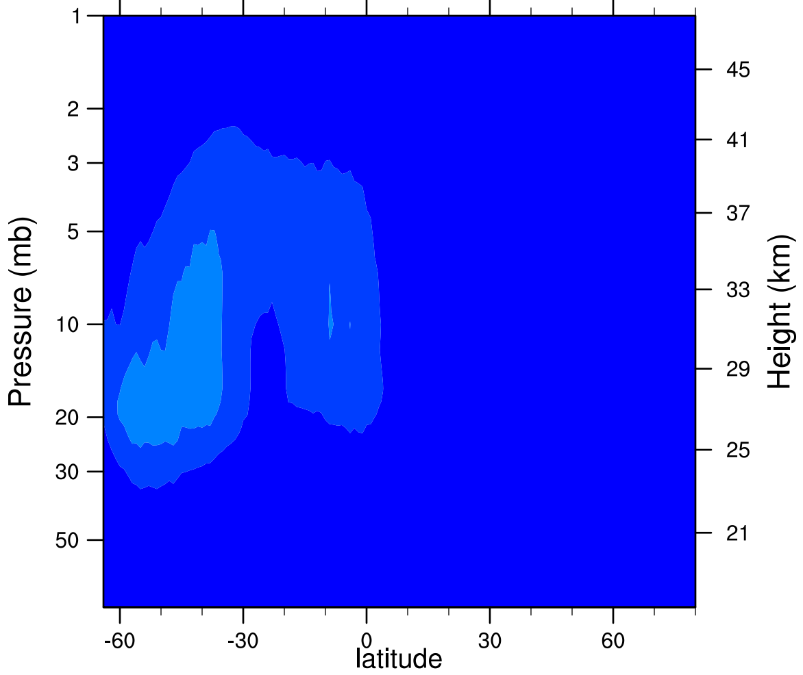
2006d228 N2O5_Ascending (ppbv)
