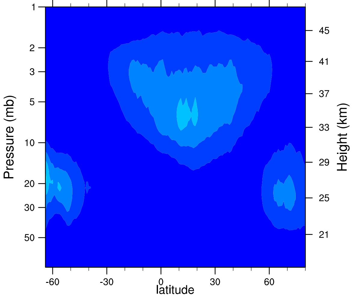
2005d266 N2O5_Ascending (ppbv)
