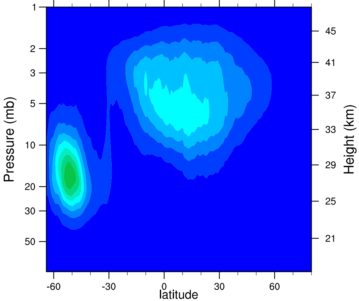
2005d225 N2O5_Ascending (ppbv)
