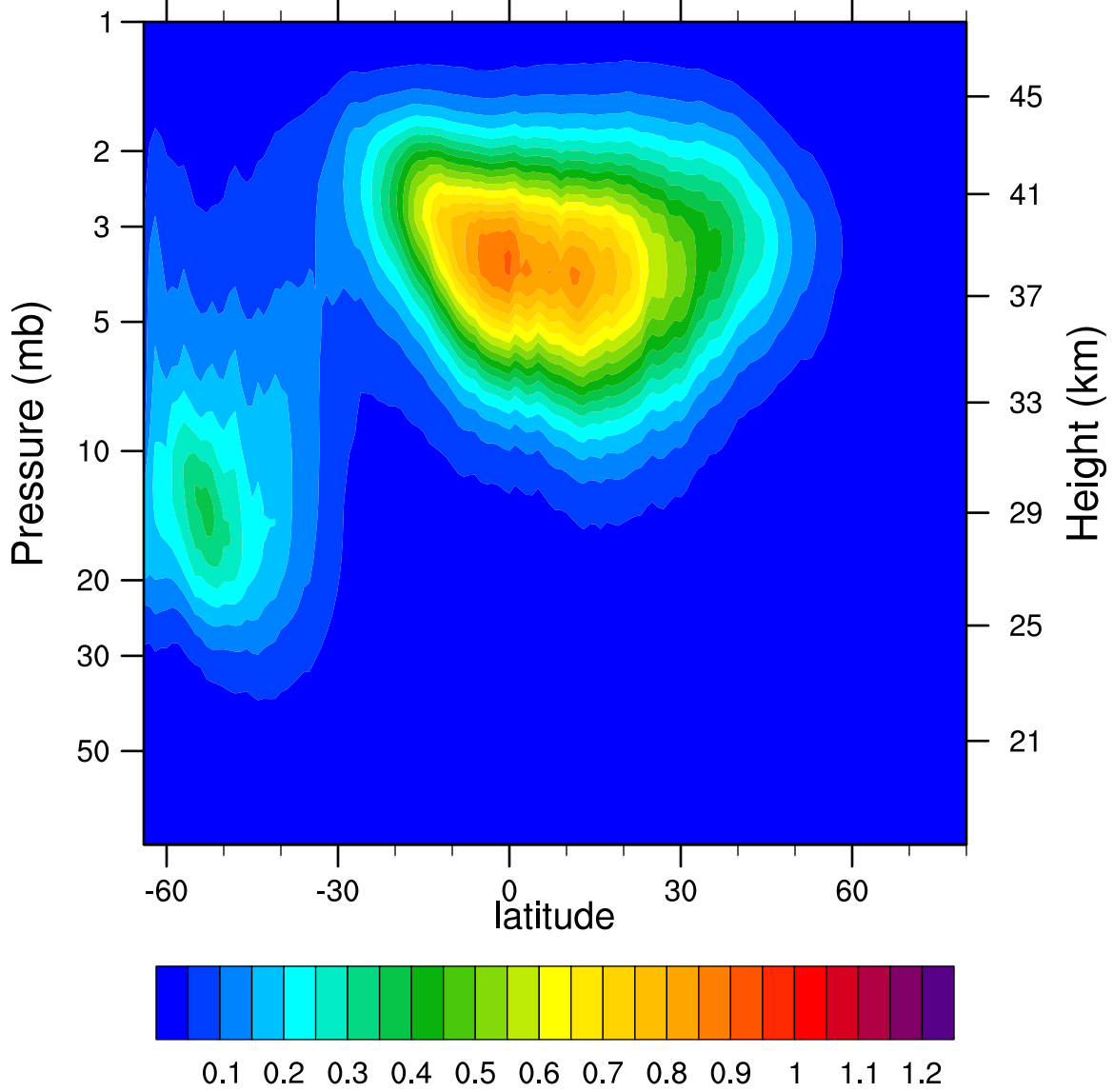
2005d134 N2O5_Ascending (ppbv)
