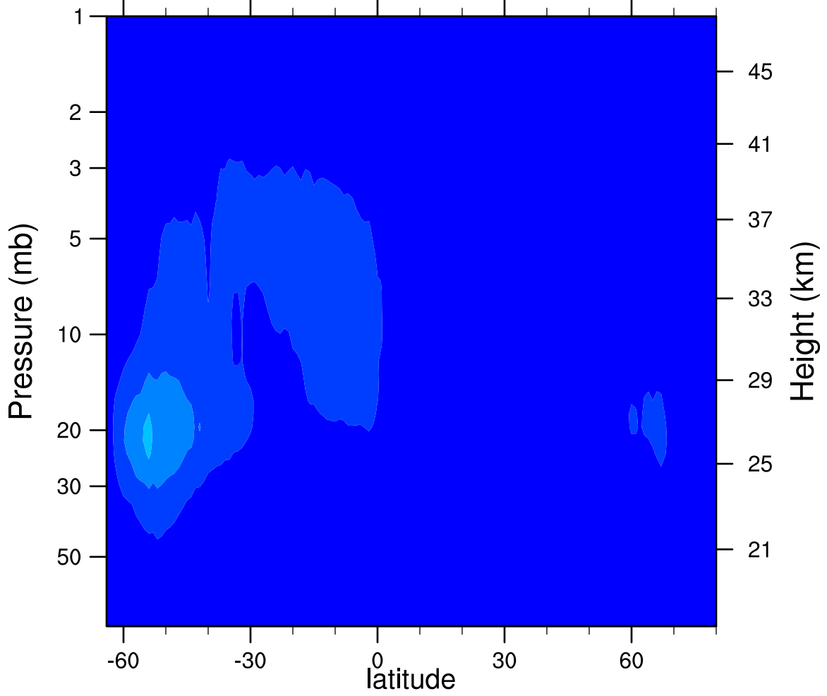
2006d253 N2O5_Ascending (ppbv)
