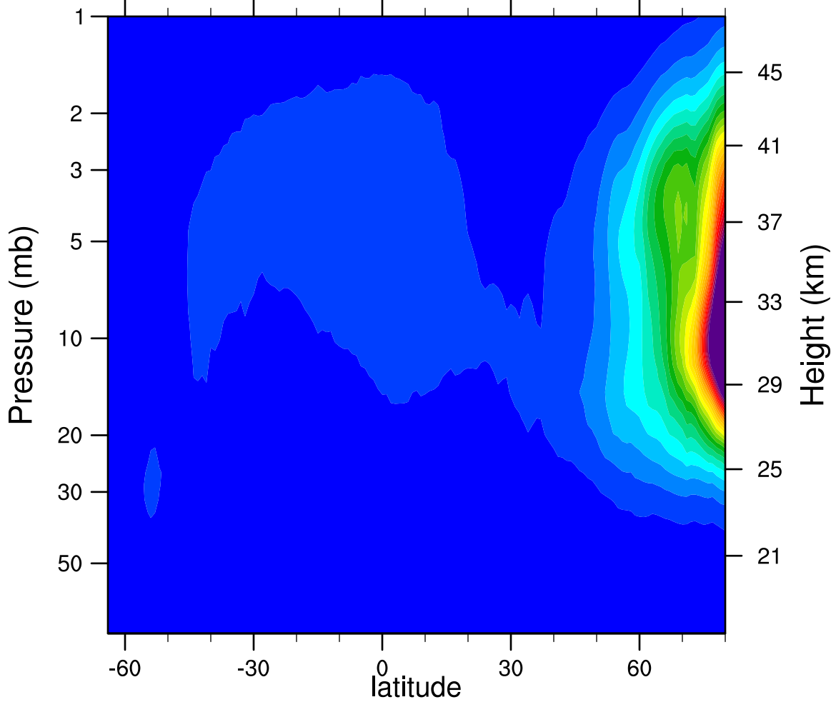
2006d043 N2O5_Ascending (ppbv)
