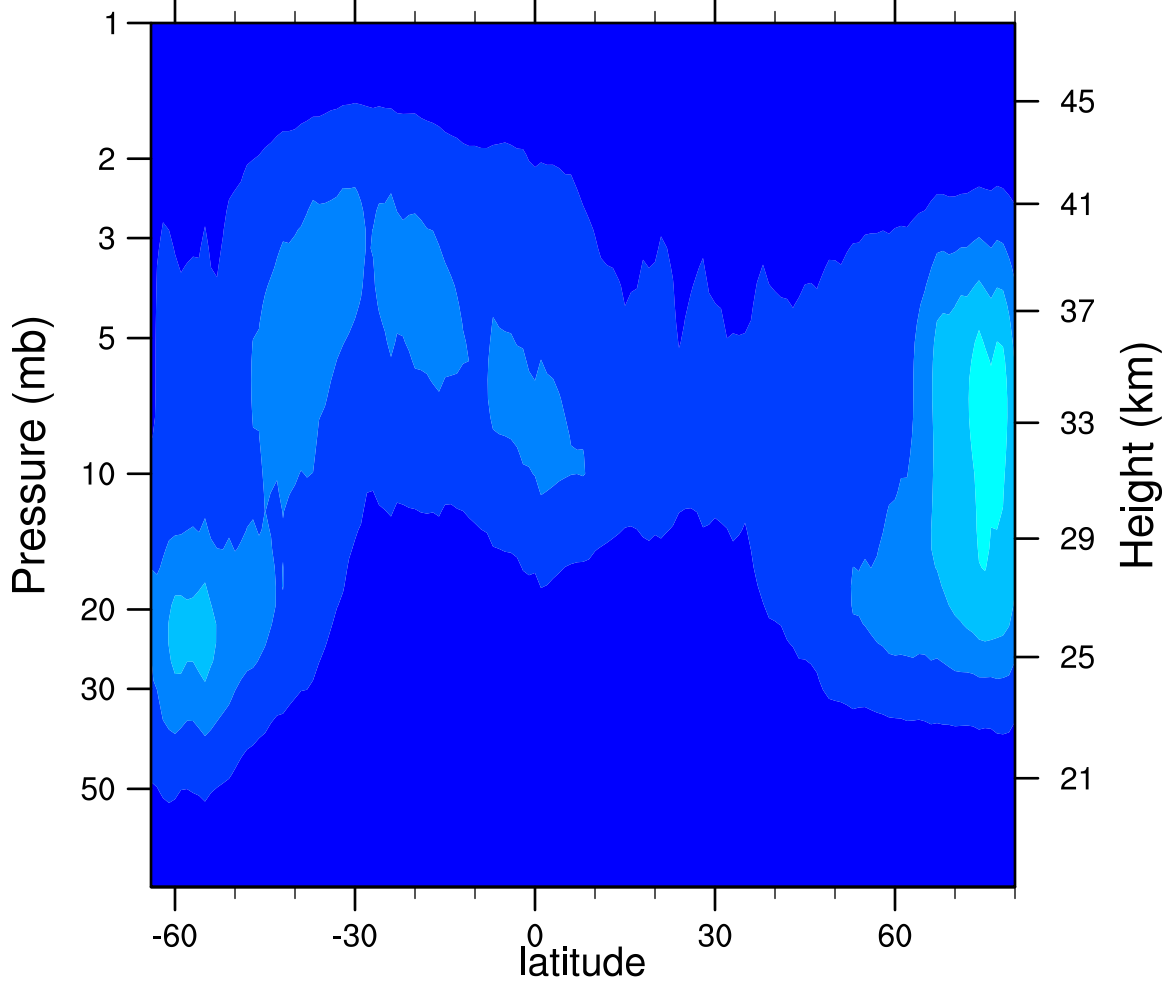
2006d078 N2O5_Ascending (ppbv)
