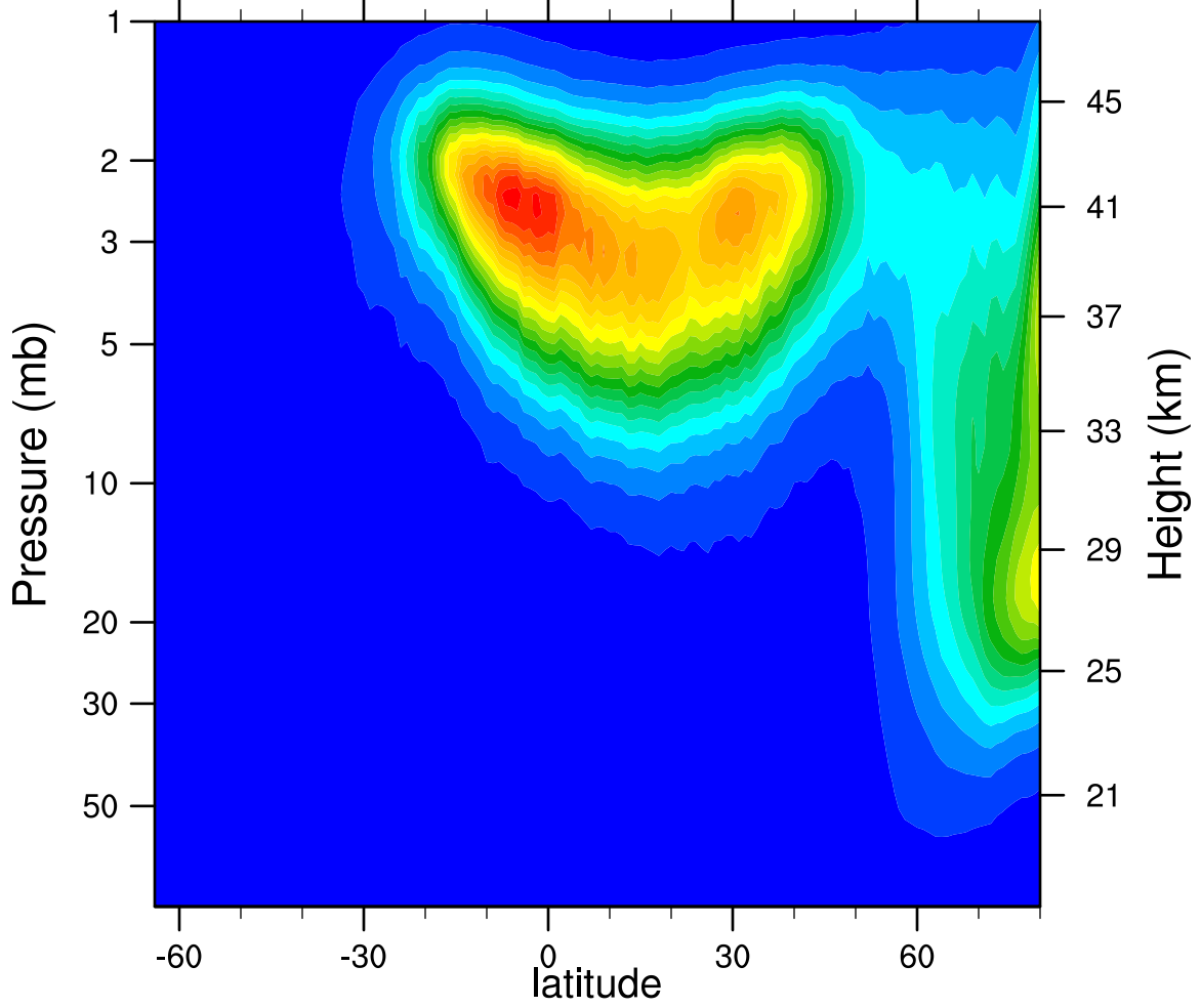
2005d046 N2O5_Ascending (ppbv)
