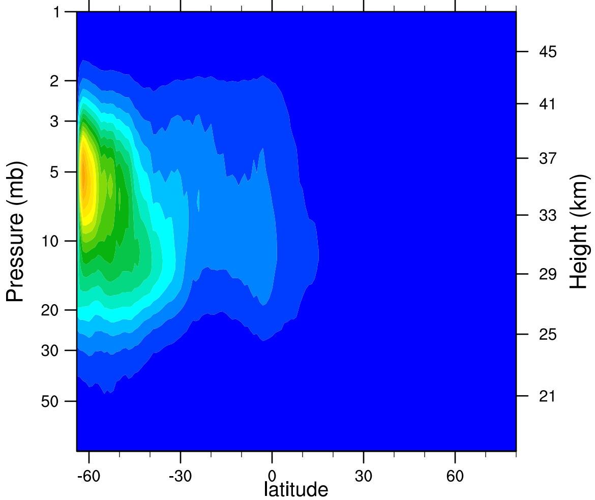
2006d155 N2O5_Ascending (ppbv)
