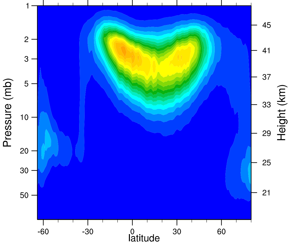
2005d080 N2O5_Ascending (ppbv)
