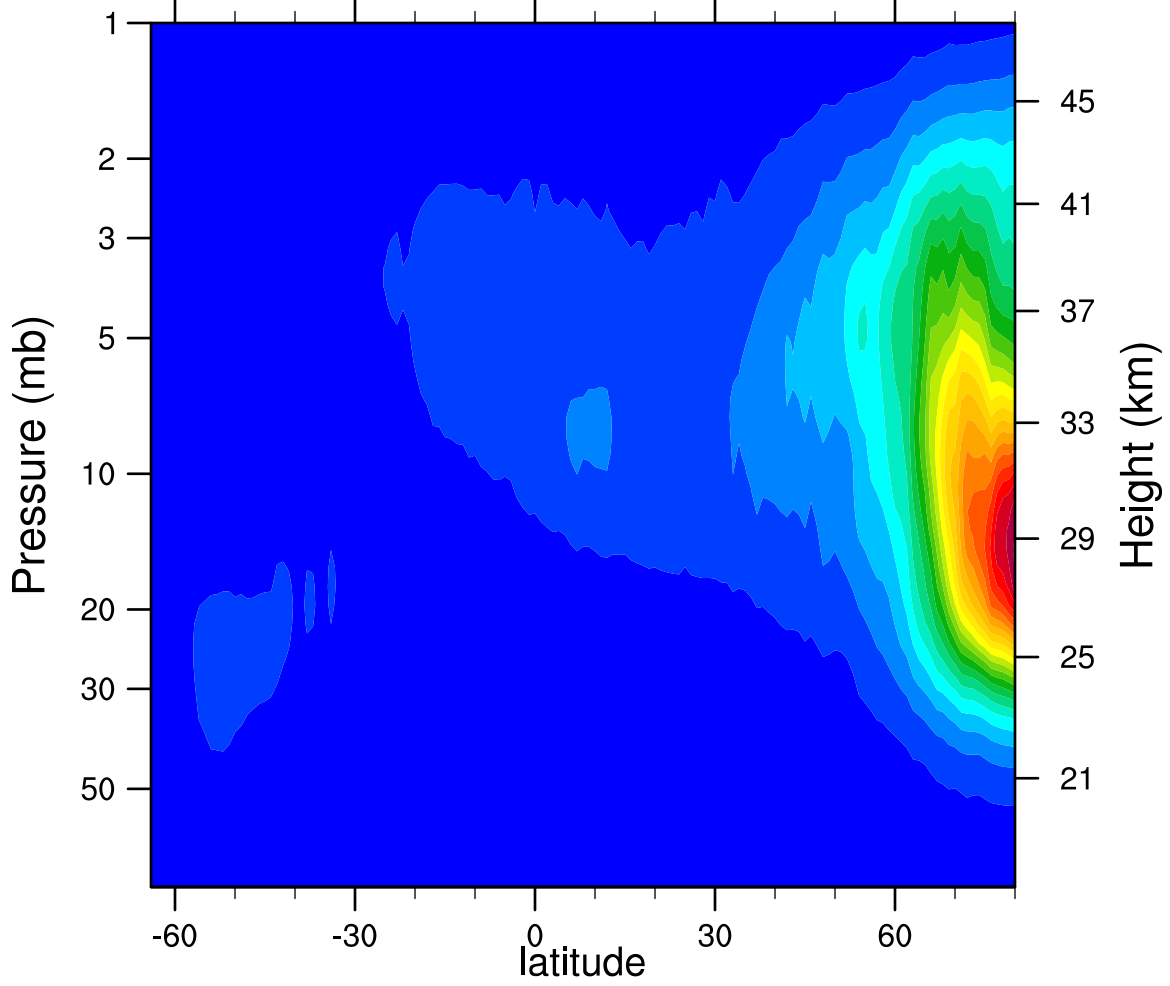
2005d303 N2O5_Ascending (ppbv)
