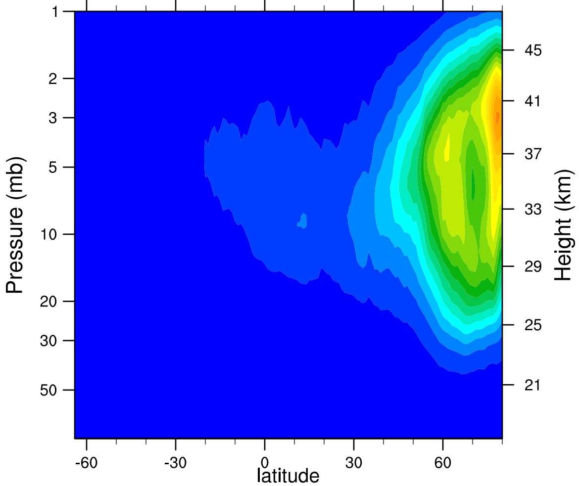
2005d325 N2O5_Ascending (ppbv)
