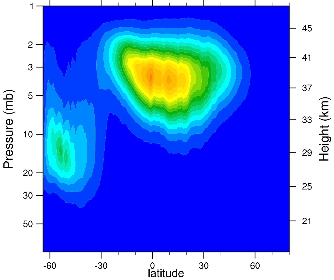
2005d138 N2O5_Ascending (ppbv)
