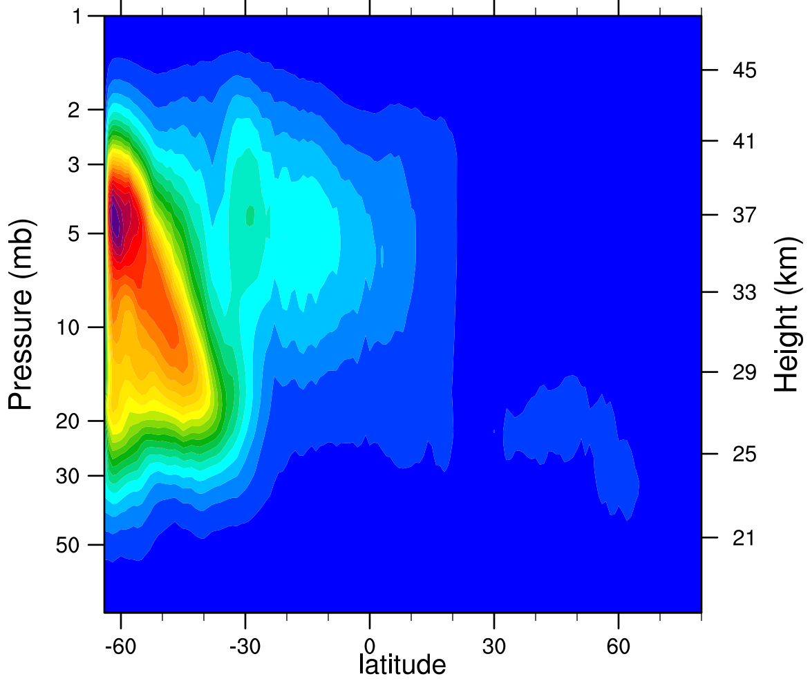
2007d132 N2O5_Ascending (ppbv)
