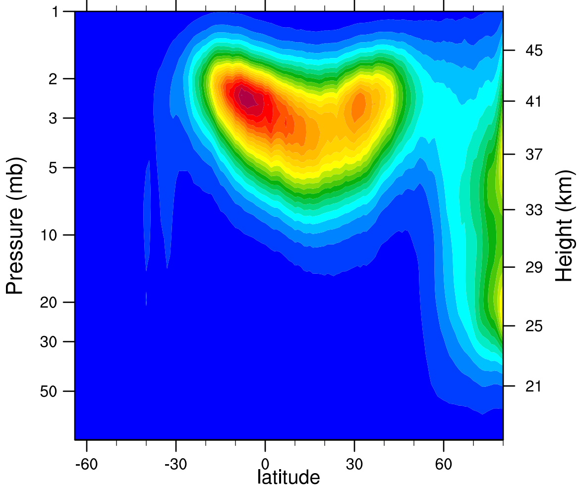
2005d051 N2O5_Ascending (ppbv)
