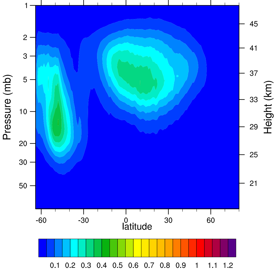
2005d188 N2O5_Ascending (ppbv)
