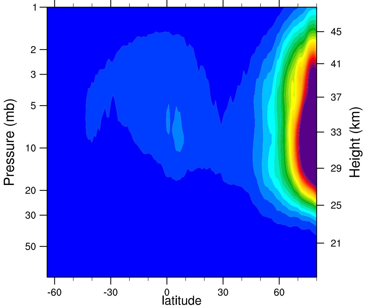
2006d034 N2O5_Ascending (ppbv)
