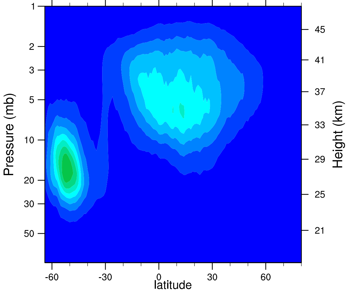
2005d223 N2O5_Ascending (ppbv)
