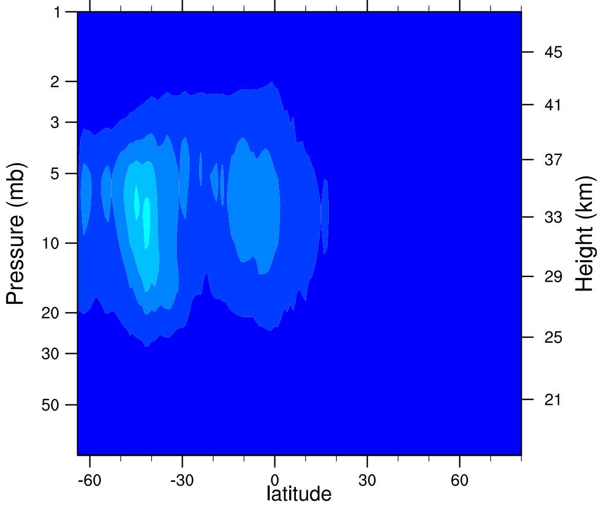
2006d191 N2O5_Ascending (ppbv)
