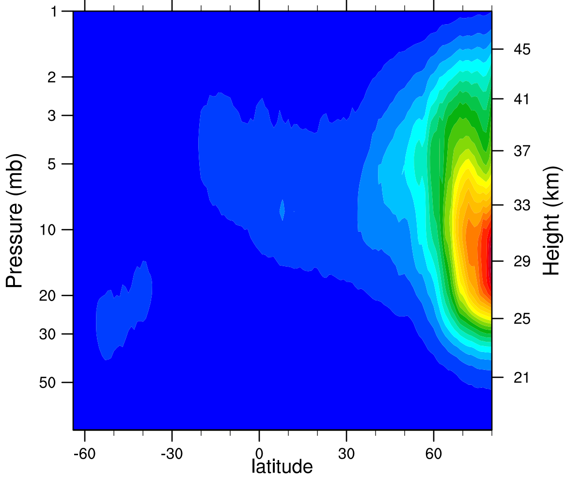
2005d307 N2O5_Ascending (ppbv)
