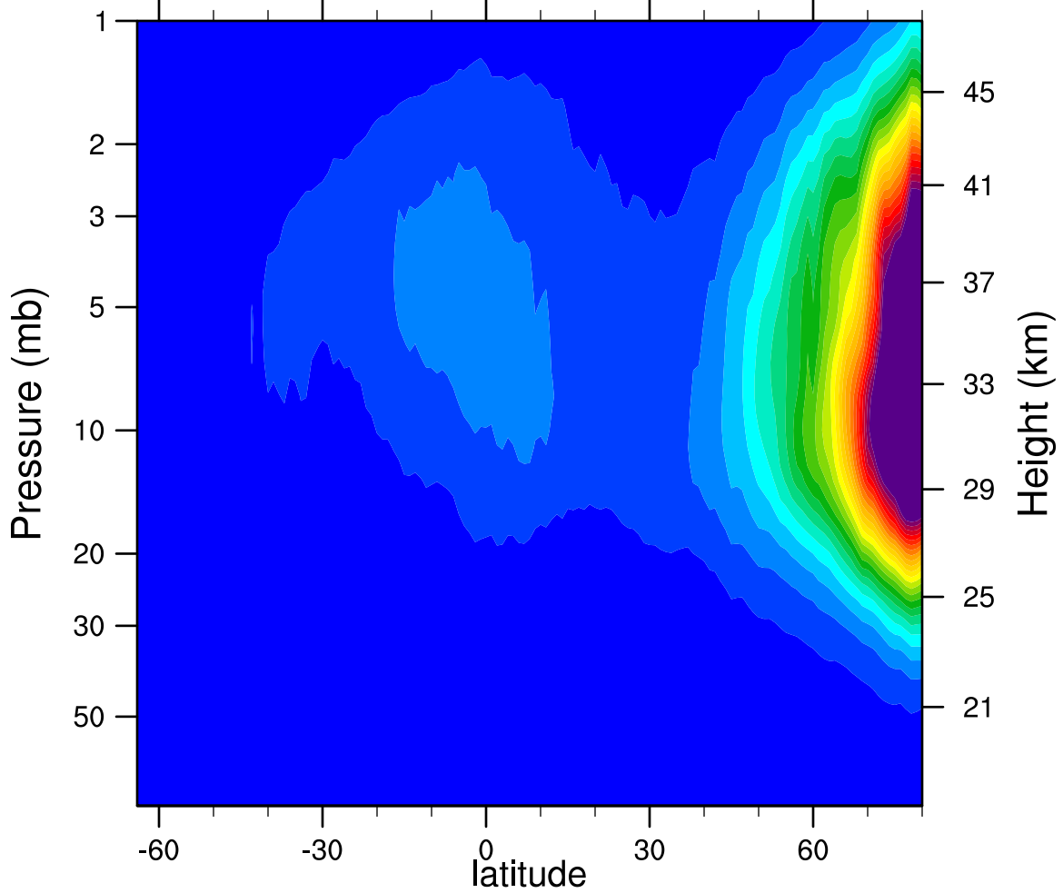
2006d015 N2O5_Ascending (ppbv)
