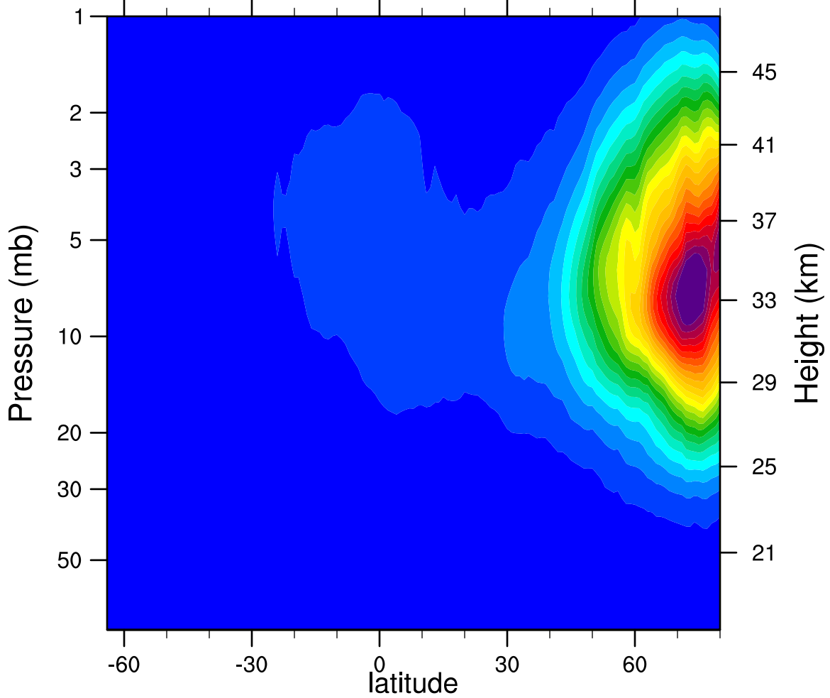
2005d350 N2O5_Ascending (ppbv)
