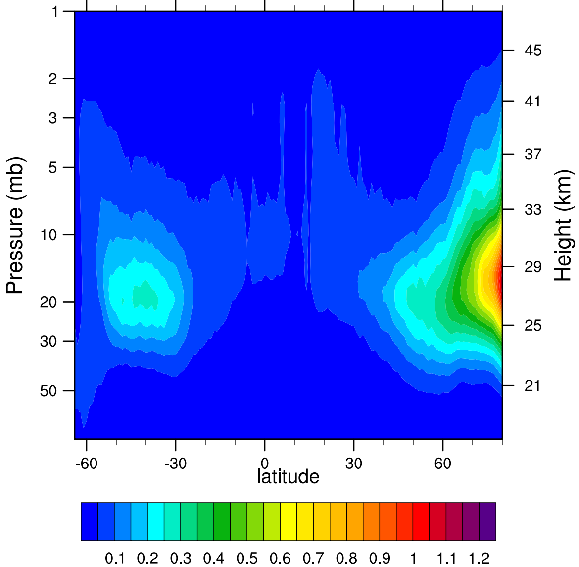
2007d284 N2O5_Ascending (ppbv)
