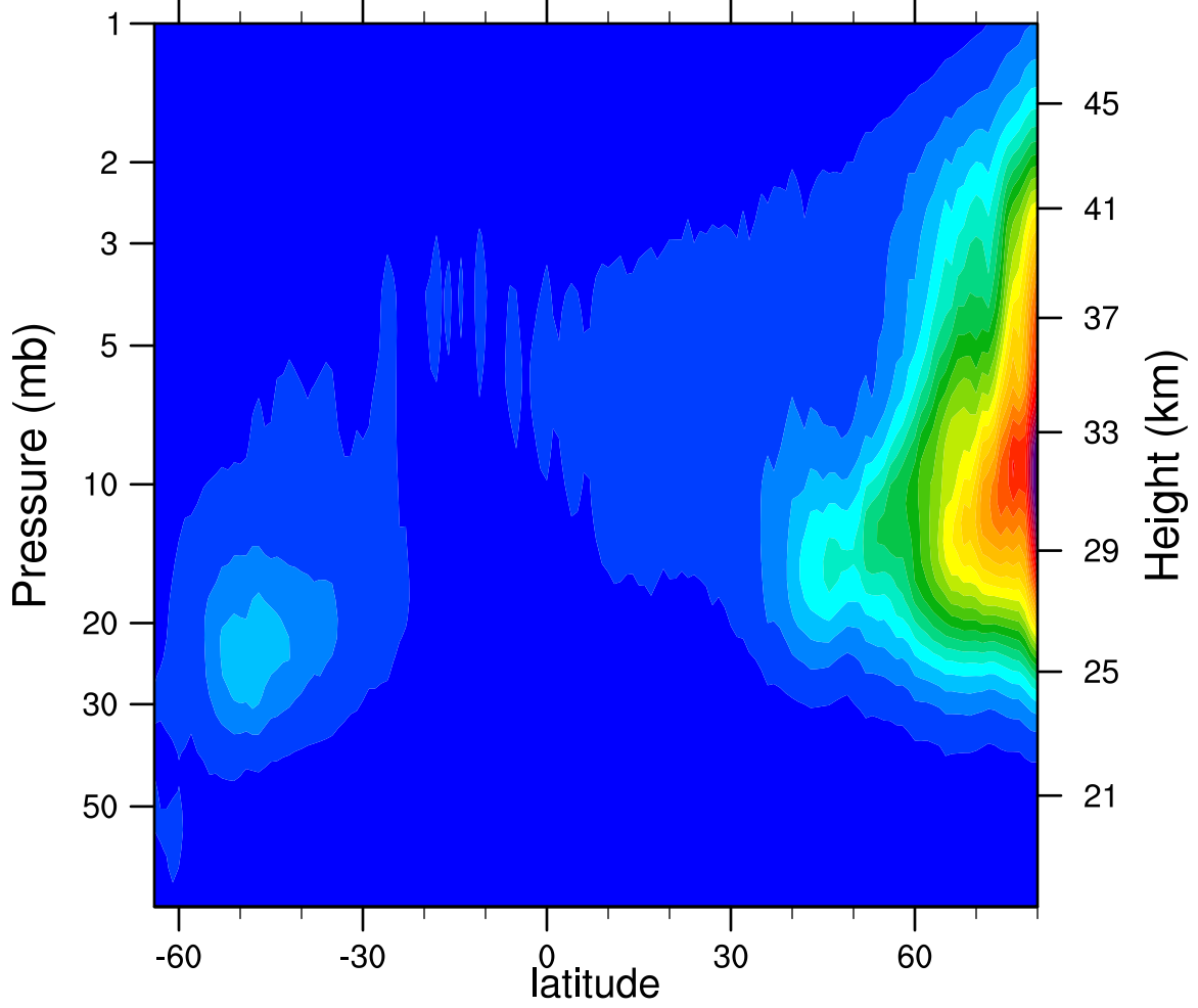
2006d330 N2O5_Ascending (ppbv)
