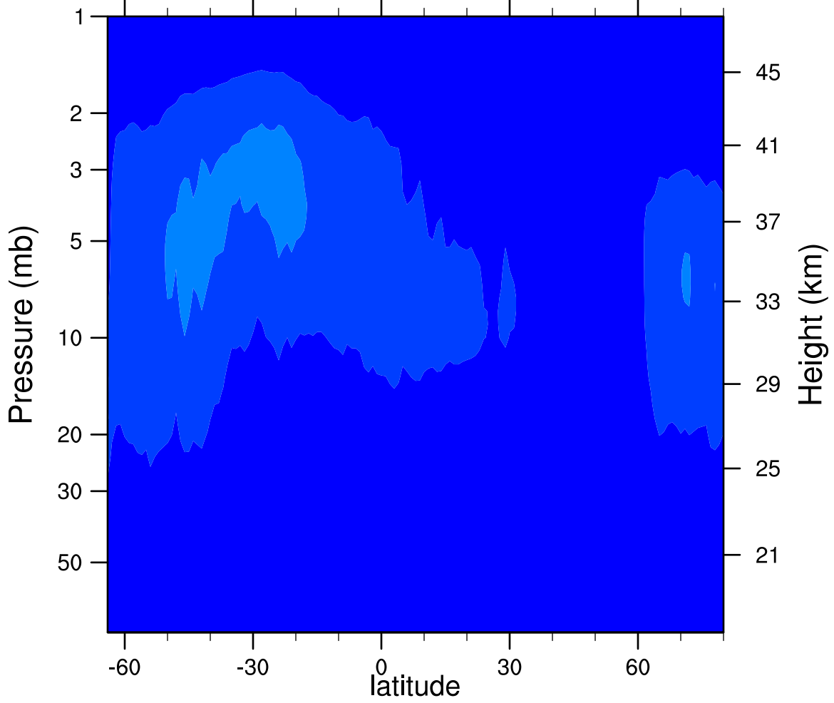
2006d089 N2O5_Ascending (ppbv)
