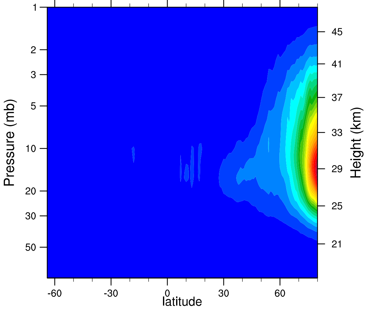
2006d294 N2O5_Ascending (ppbv)
