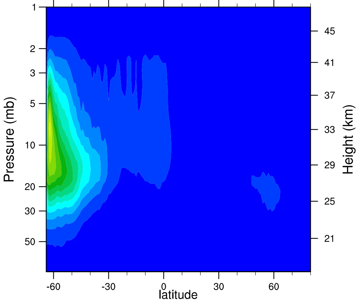
2006d122 N2O5_Ascending (ppbv)
