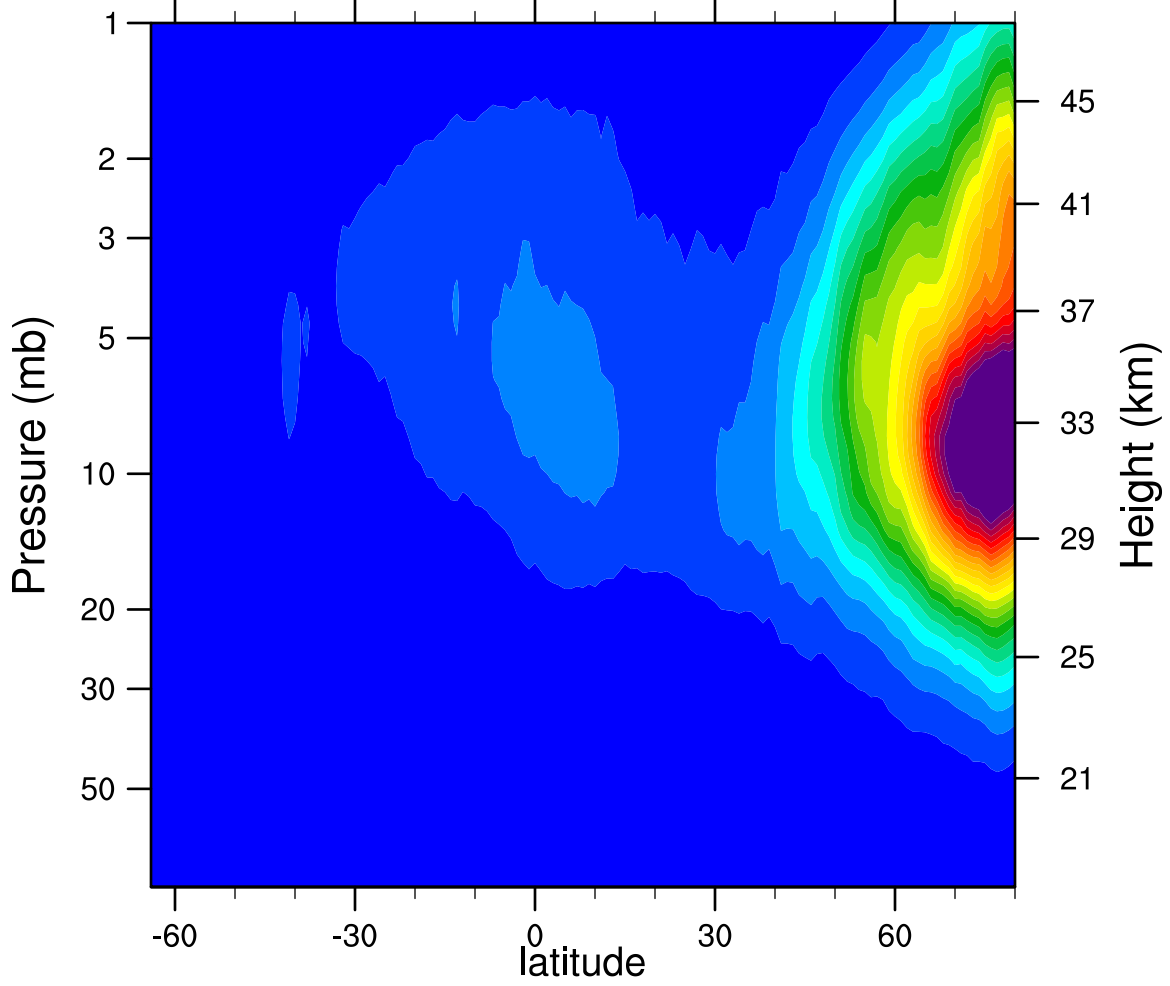
2006d006 N2O5_Ascending (ppbv)
