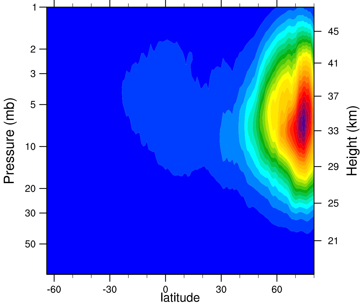
2005d343 N2O5_Ascending (ppbv)
