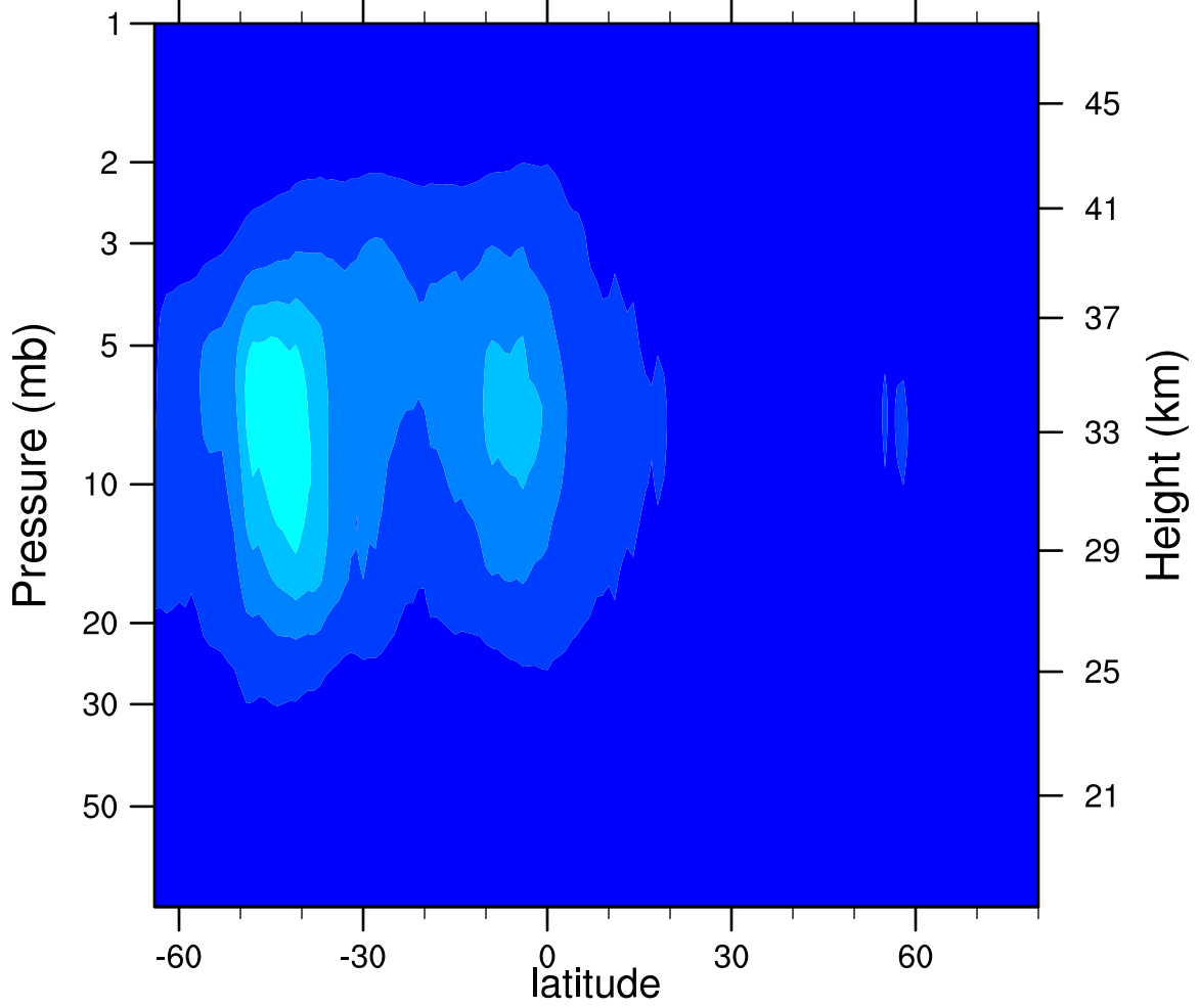
2006d201 N2O5_Ascending (ppbv)
