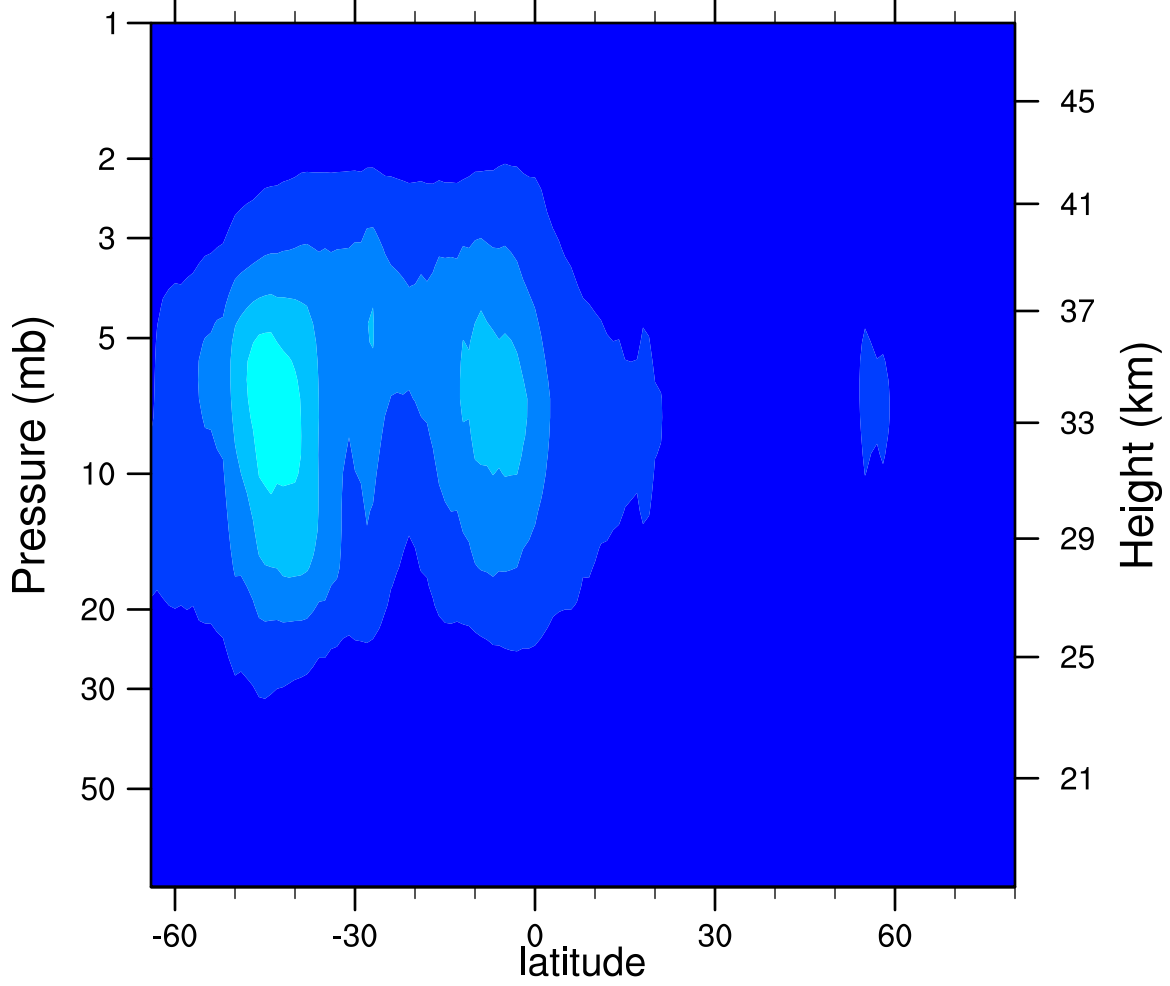
2006d206 N2O5_Ascending (ppbv)
