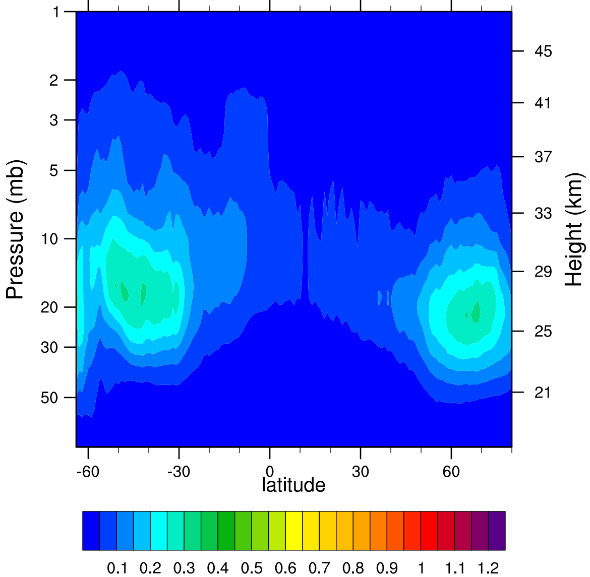
2007d261 N2O5_Ascending (ppbv)
