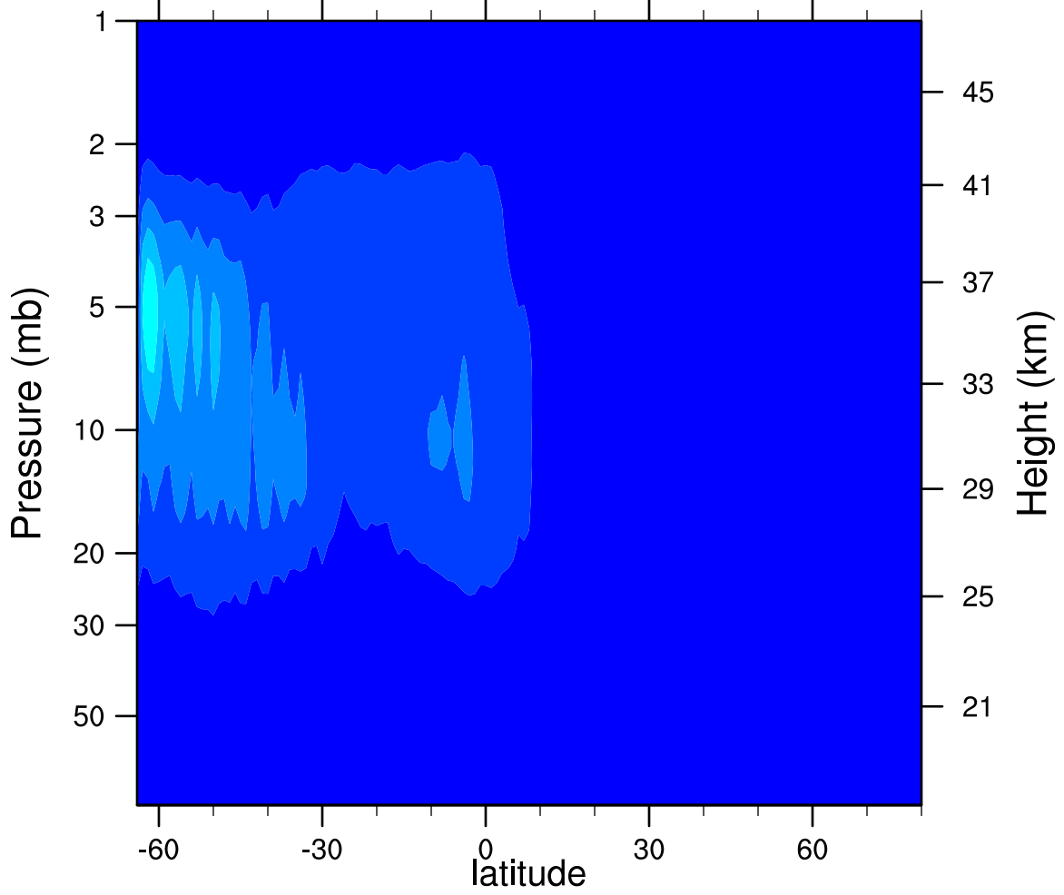
2006d176 N2O5_Ascending (ppbv)
