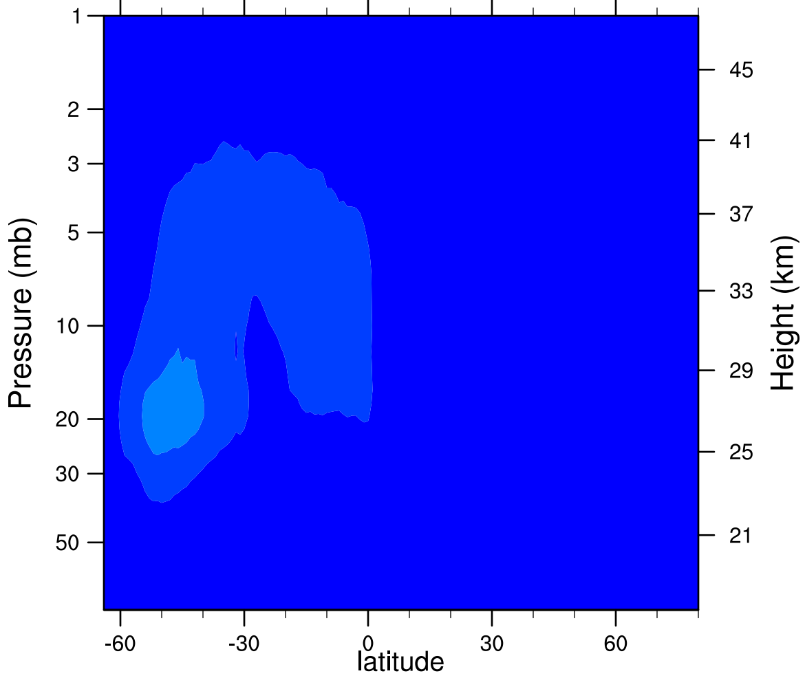
2006d245 N2O5_Ascending (ppbv)
