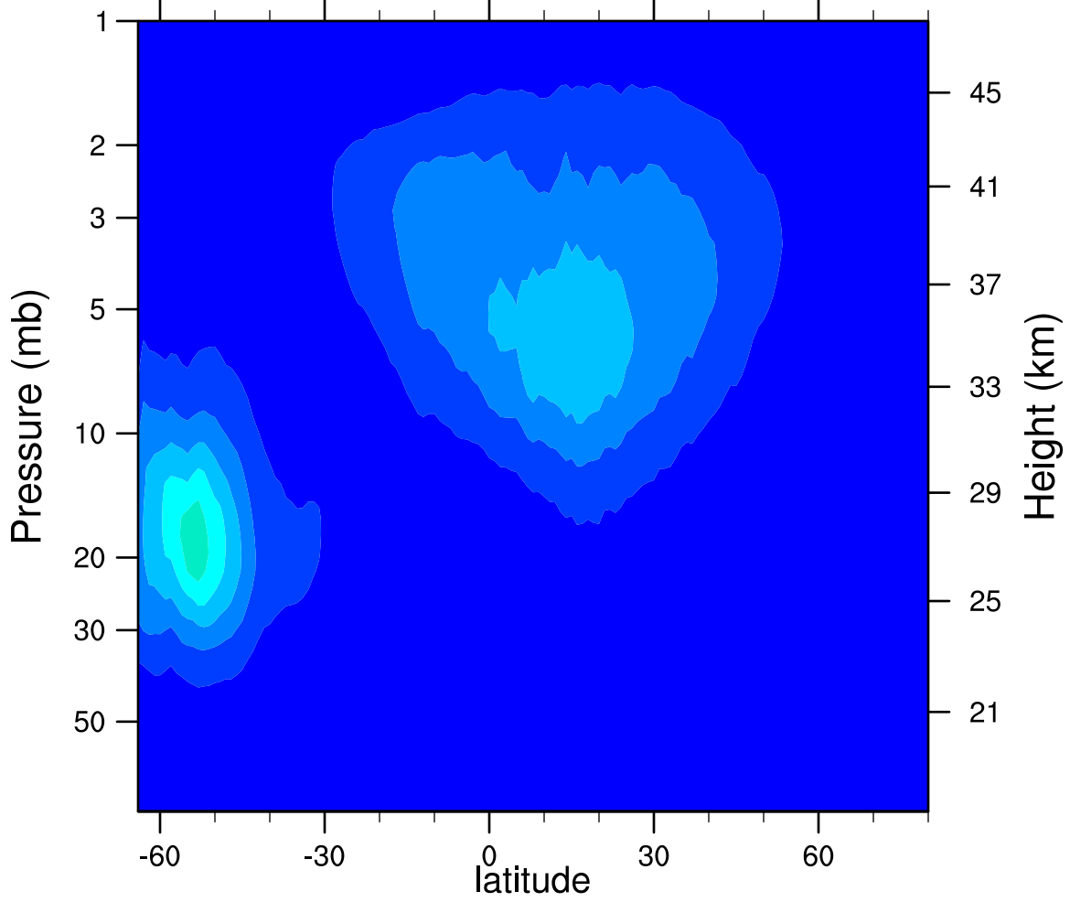
2005d237 N2O5_Ascending (ppbv)
