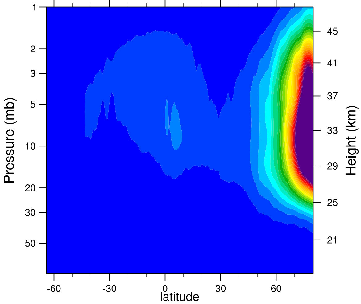
2006d033 N2O5_Ascending (ppbv)
