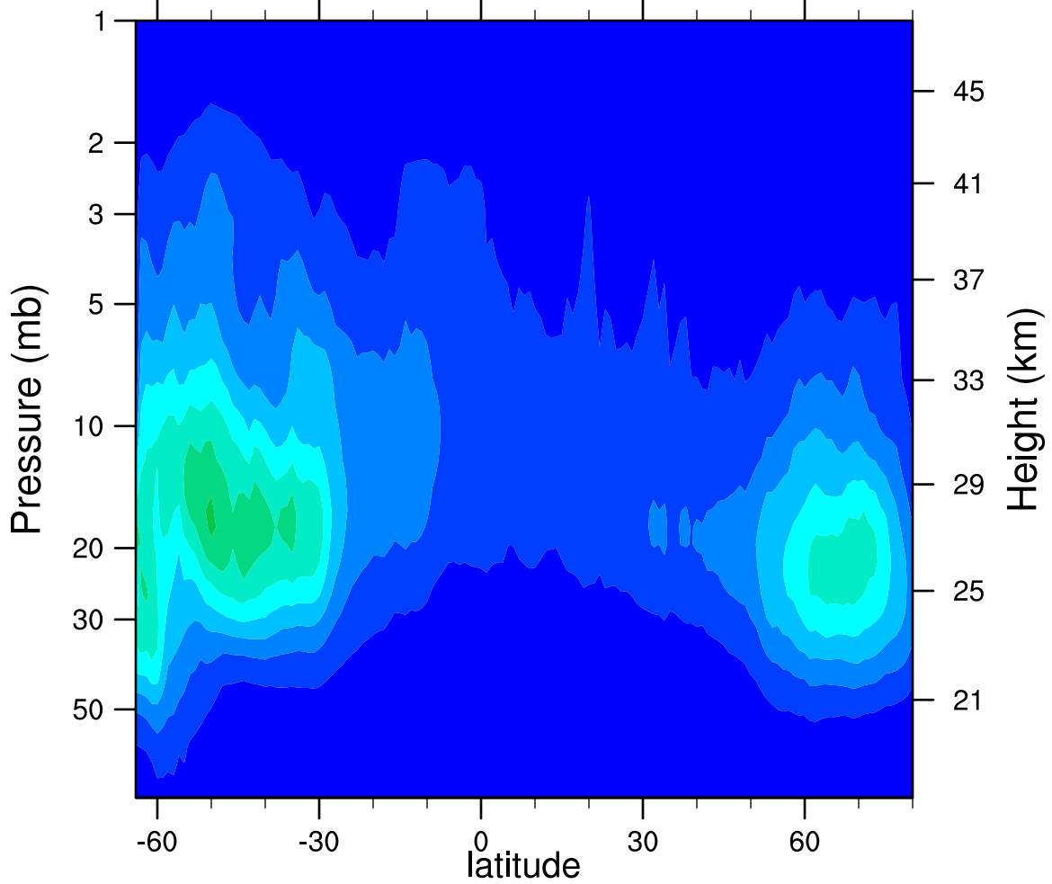
2007d258 N2O5_Ascending (ppbv)
