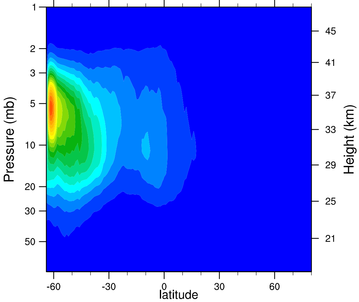
2006d165 N2O5_Ascending (ppbv)
