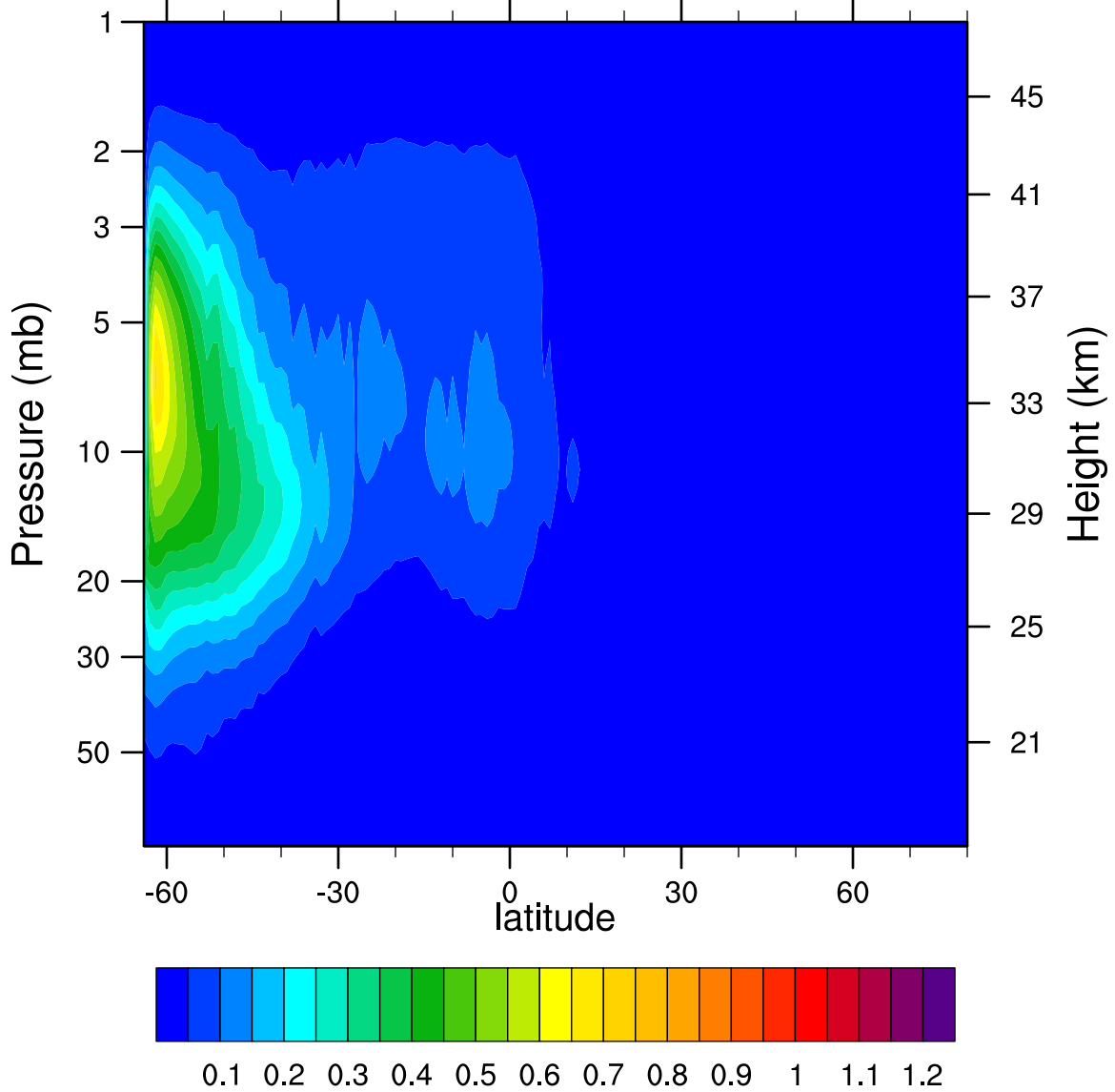
2006d139 N2O5_Ascending (ppbv)
