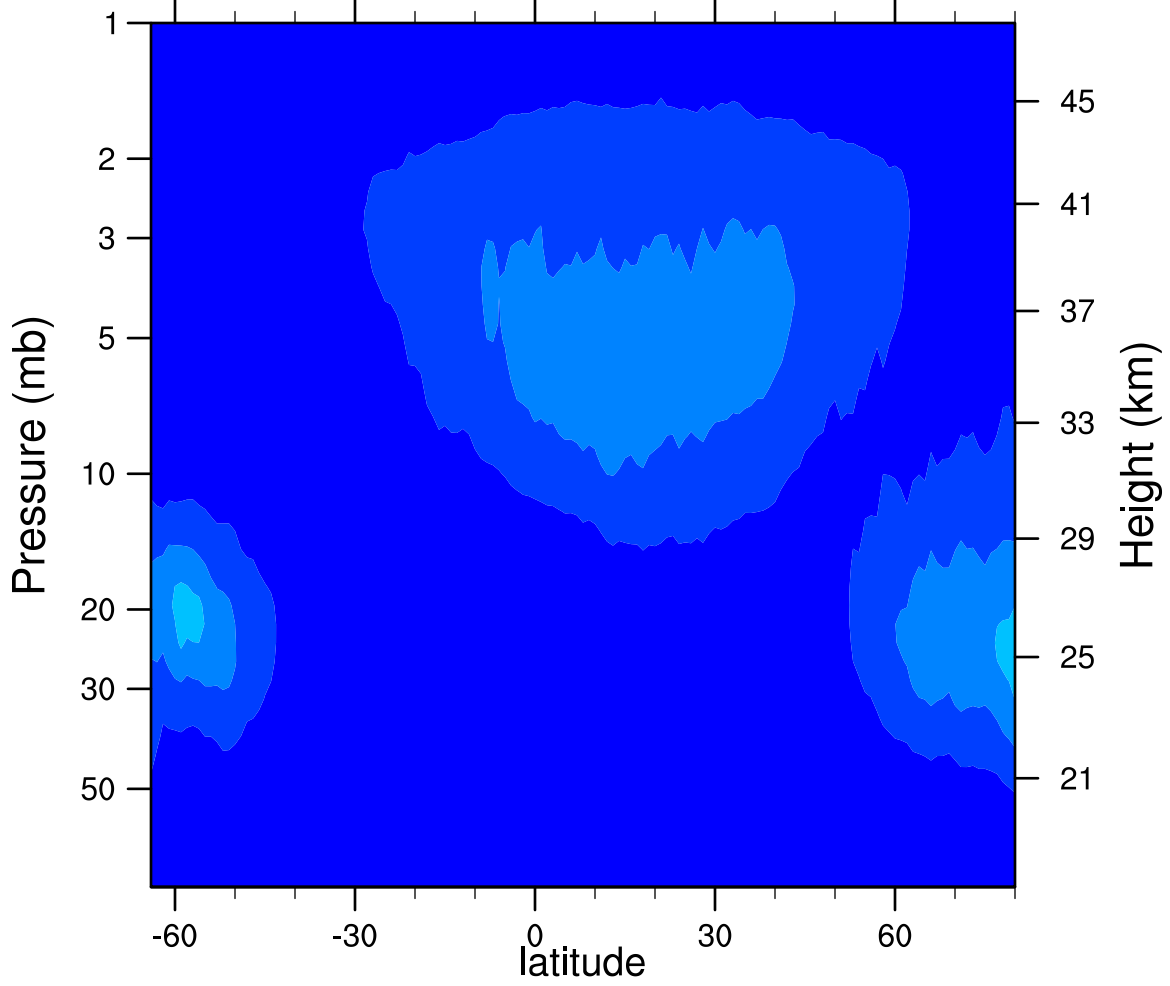
2005d272 N2O5_Ascending (ppbv)
