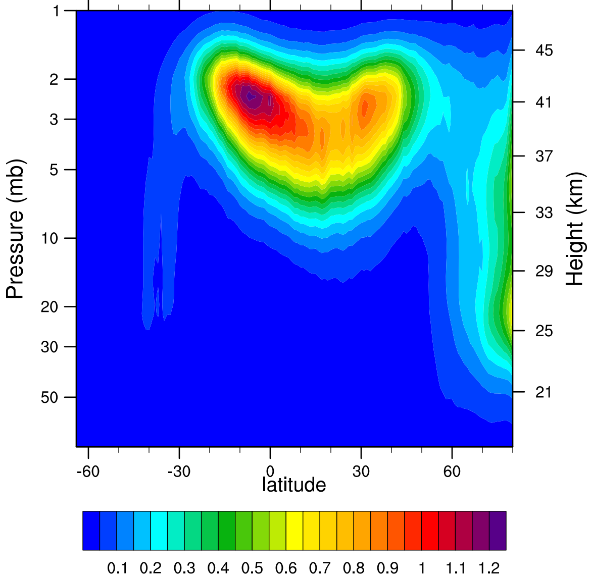
2005d054 N2O5_Ascending (ppbv)
