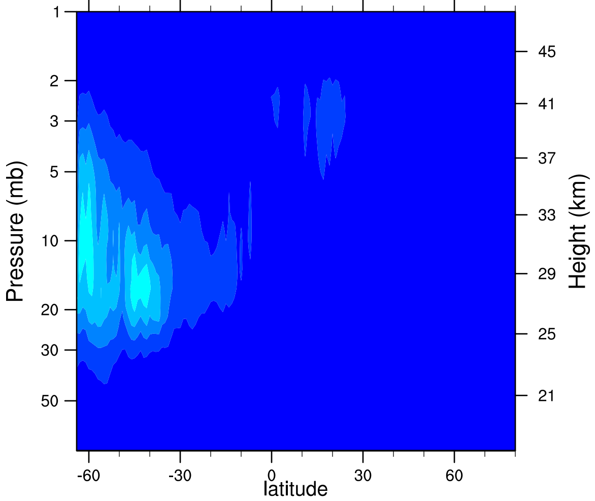
2007d212 N2O5_Ascending (ppbv)
