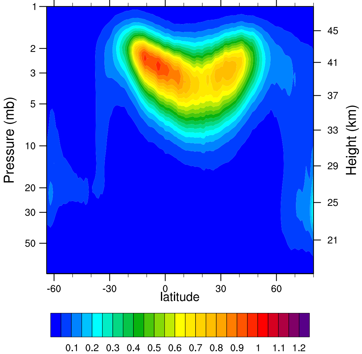
2005d073 N2O5_Ascending (ppbv)
