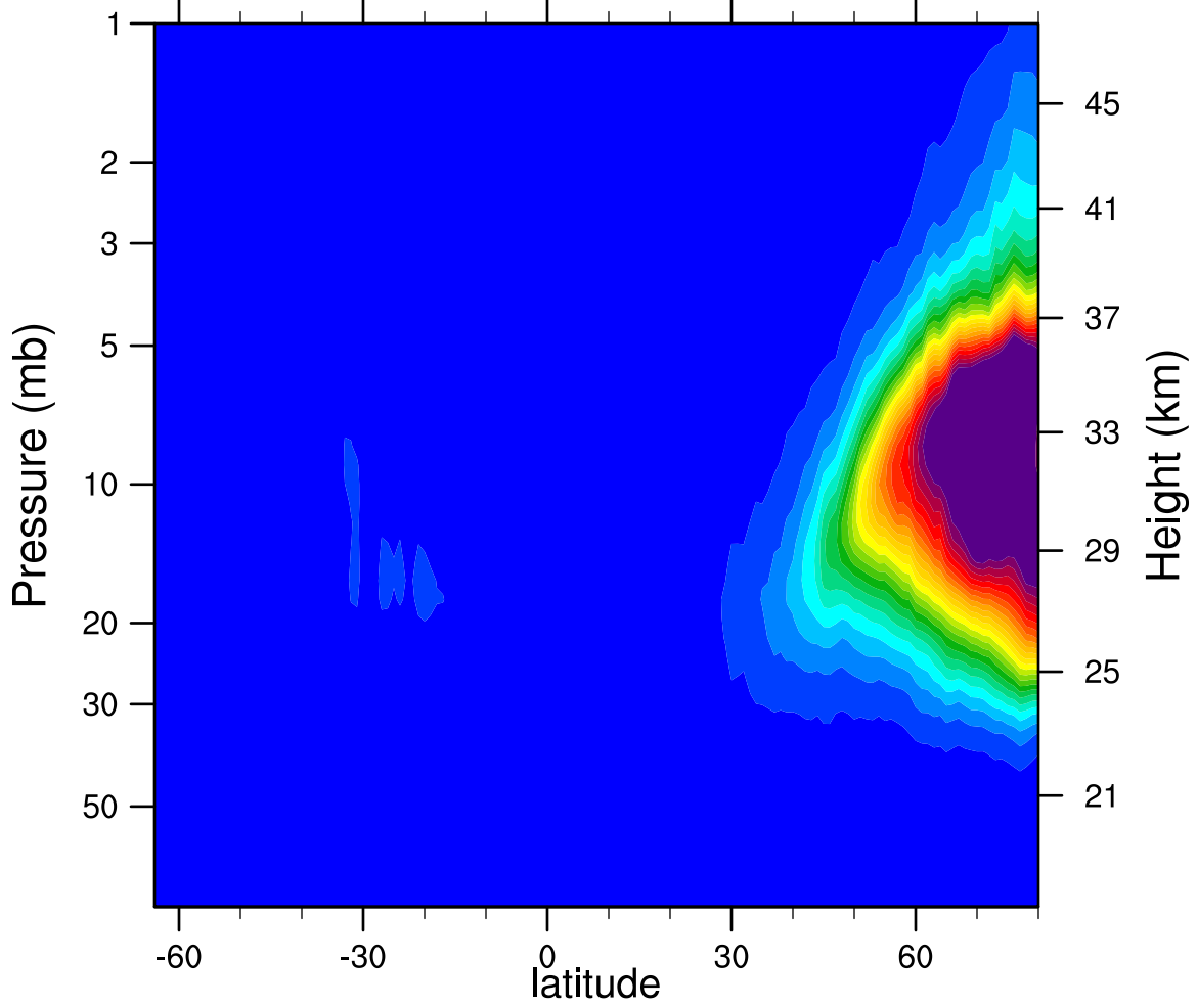
2006d358 N2O5_Ascending (ppbv)
