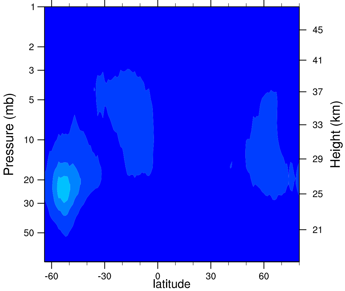
2006d262 N2O5_Ascending (ppbv)
