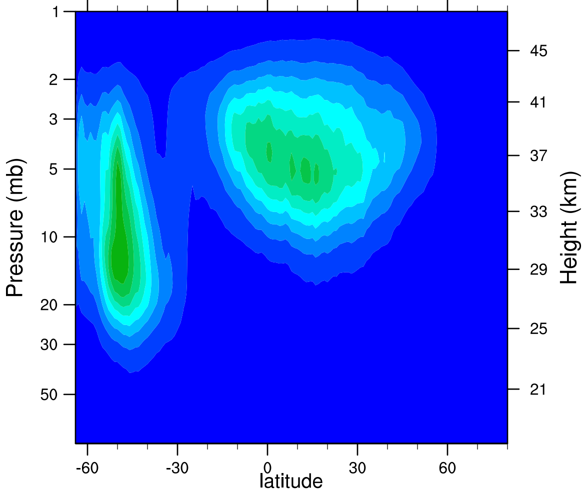
2005d182 N2O5_Ascending (ppbv)
