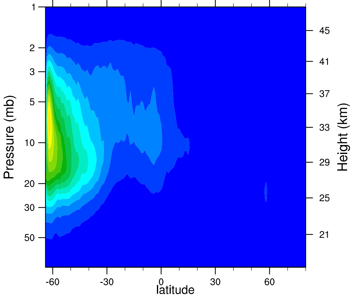
2006d128 N2O5_Ascending (ppbv)
