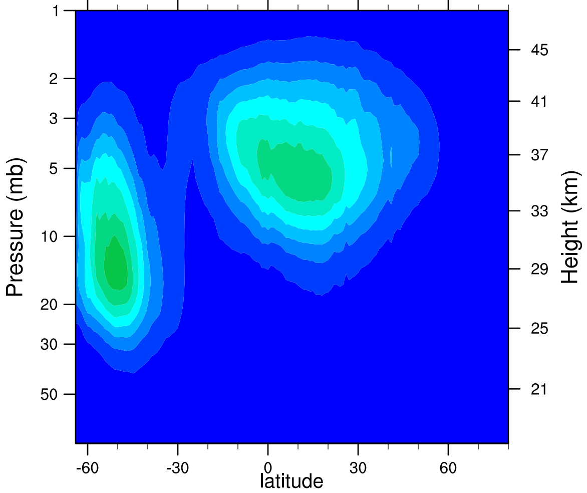
2005d198 N2O5_Ascending (ppbv)
