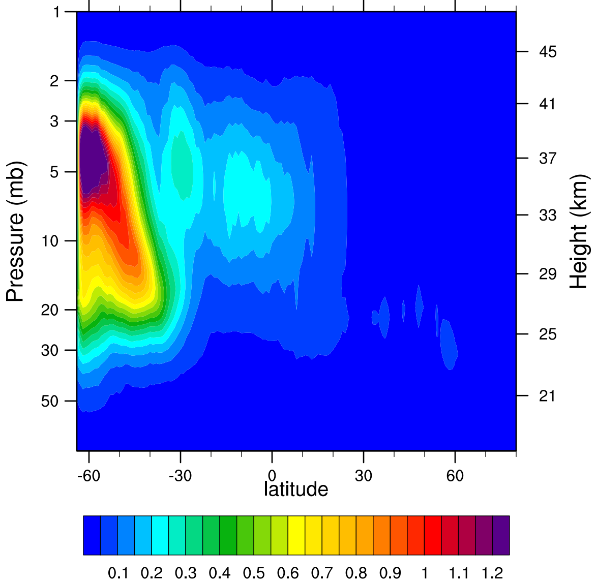
2007d139 N2O5_Ascending (ppbv)
