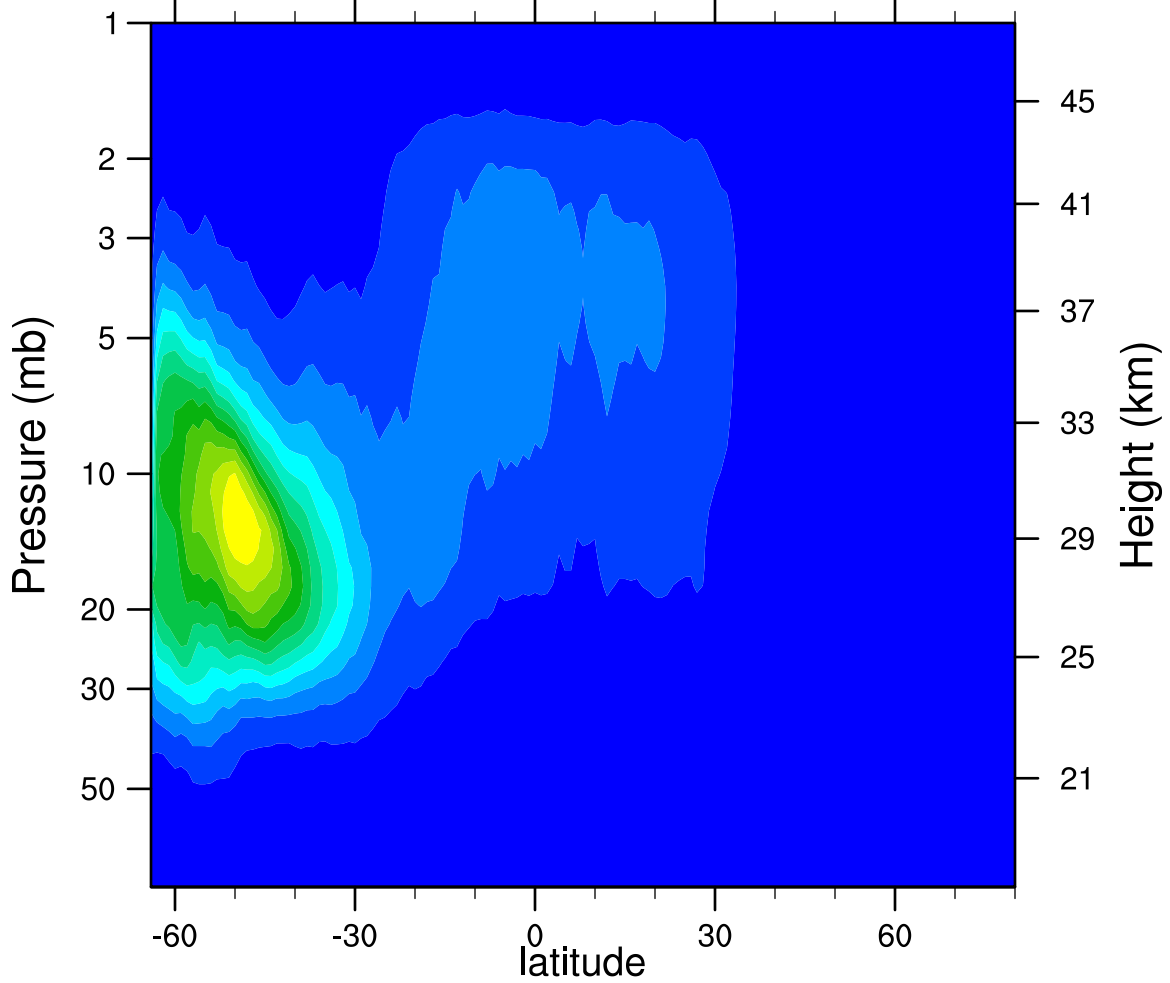
2007d221 N2O5_Ascending (ppbv)
