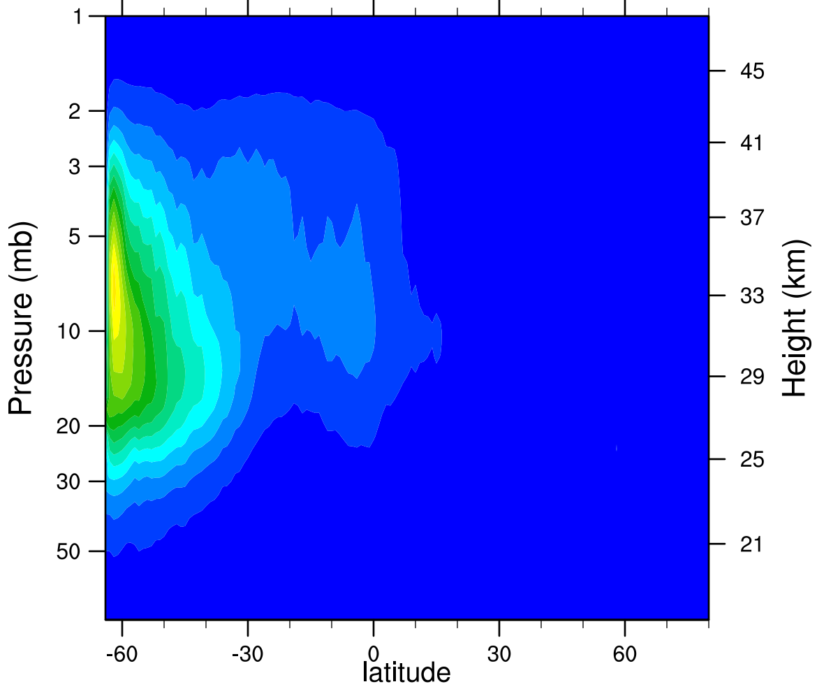
2006d129 N2O5_Ascending (ppbv)
