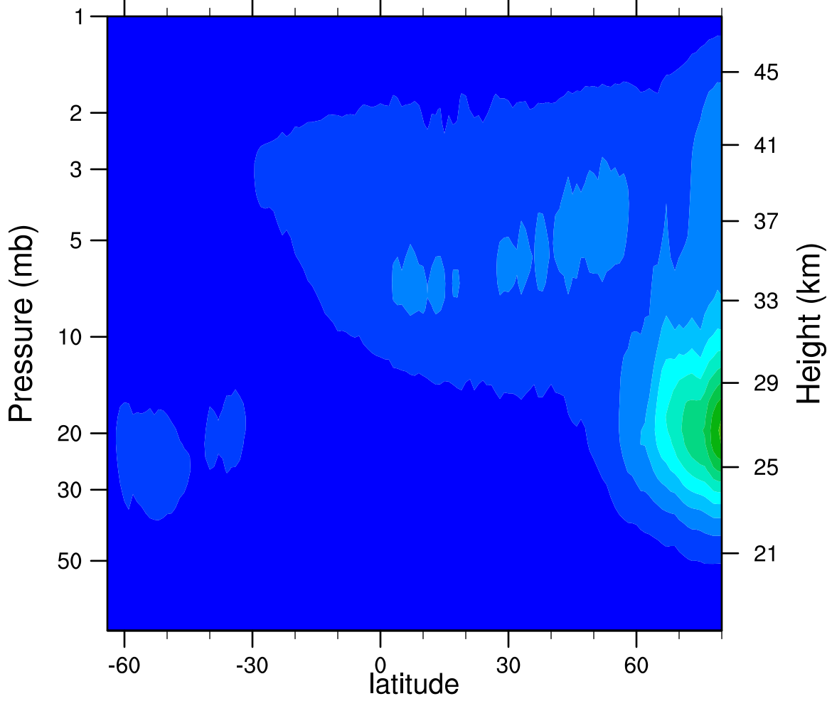
2005d286 N2O5_Ascending (ppbv)
