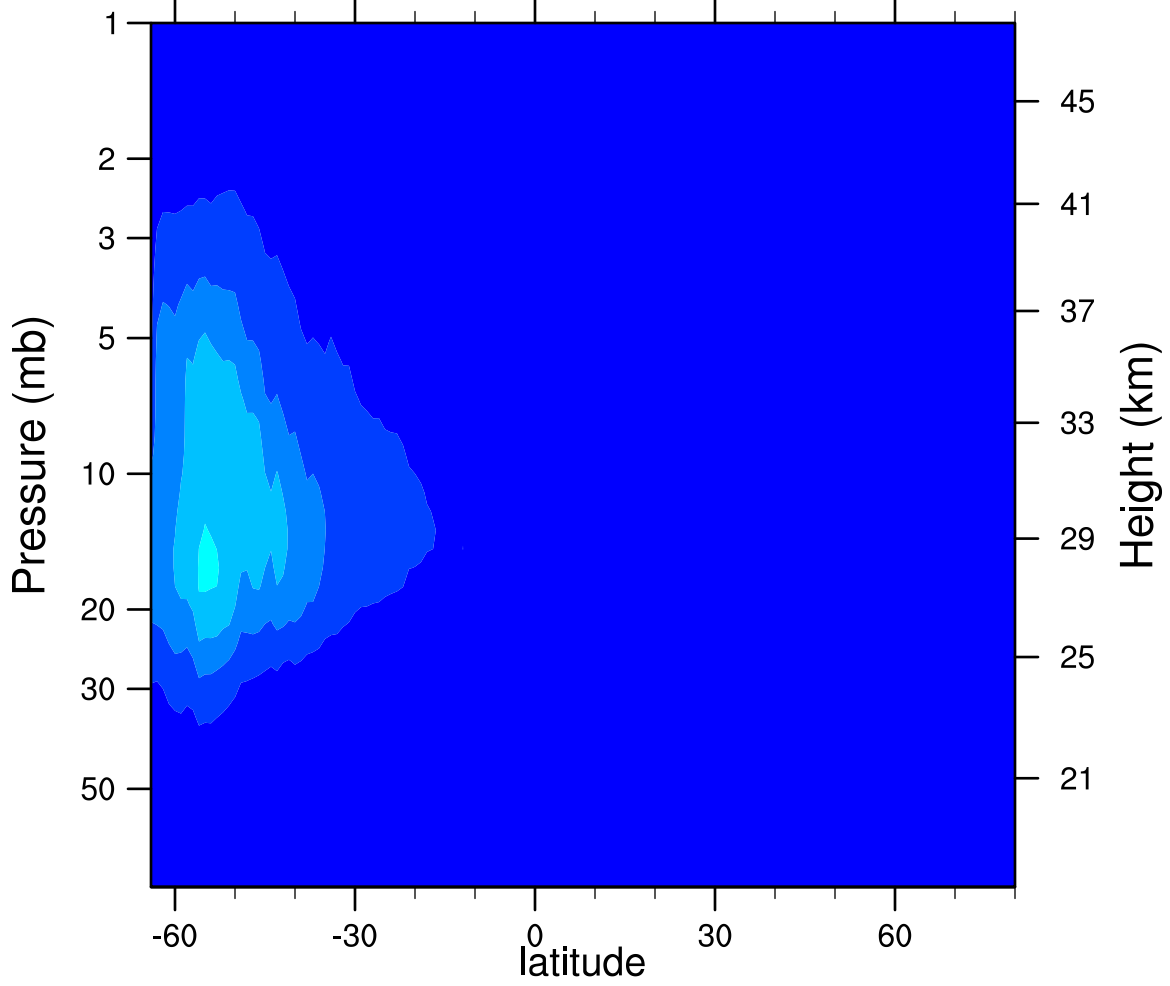
2007d197 N2O5_Ascending (ppbv)
