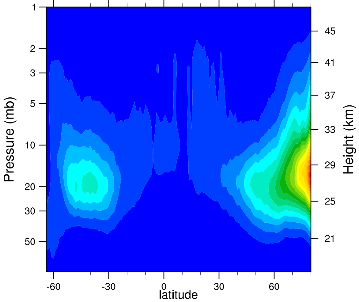
2007d283 N2O5_Ascending (ppbv)
