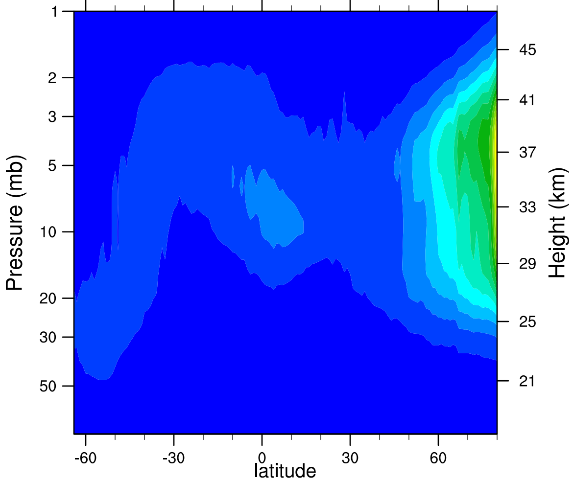
2006d059 N2O5_Ascending (ppbv)
