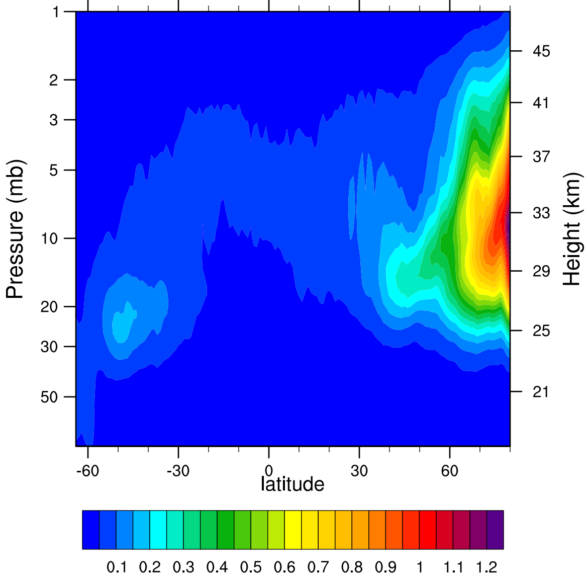
2006d327 N2O5_Ascending (ppbv)
