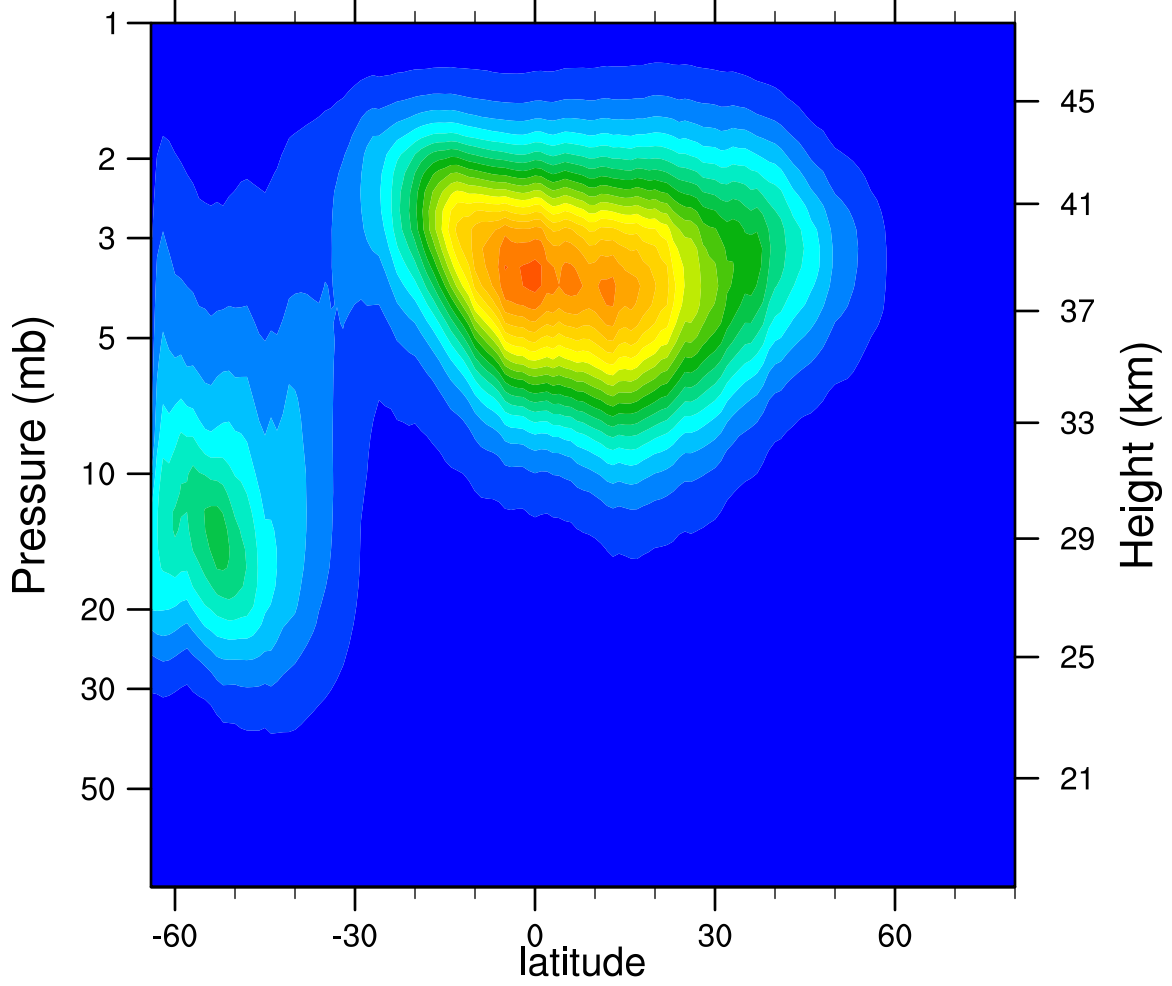
2005d132 N2O5_Ascending (ppbv)
