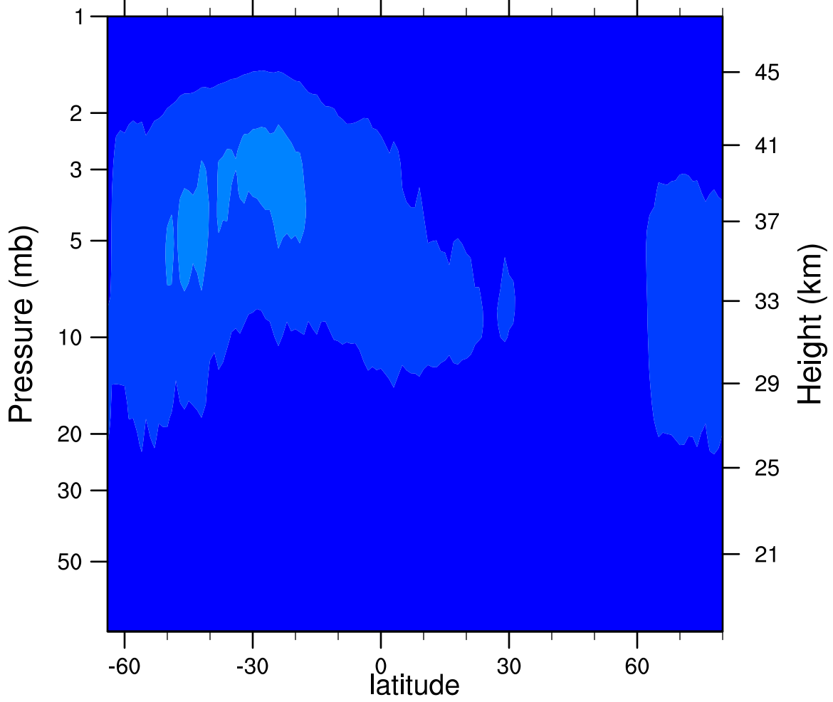
2006d090 N2O5_Ascending (ppbv)
