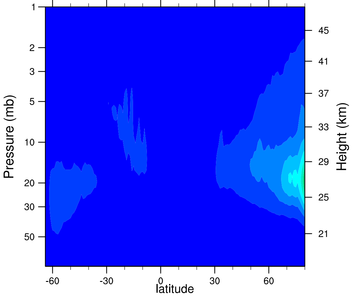
2006d278 N2O5_Ascending (ppbv)
