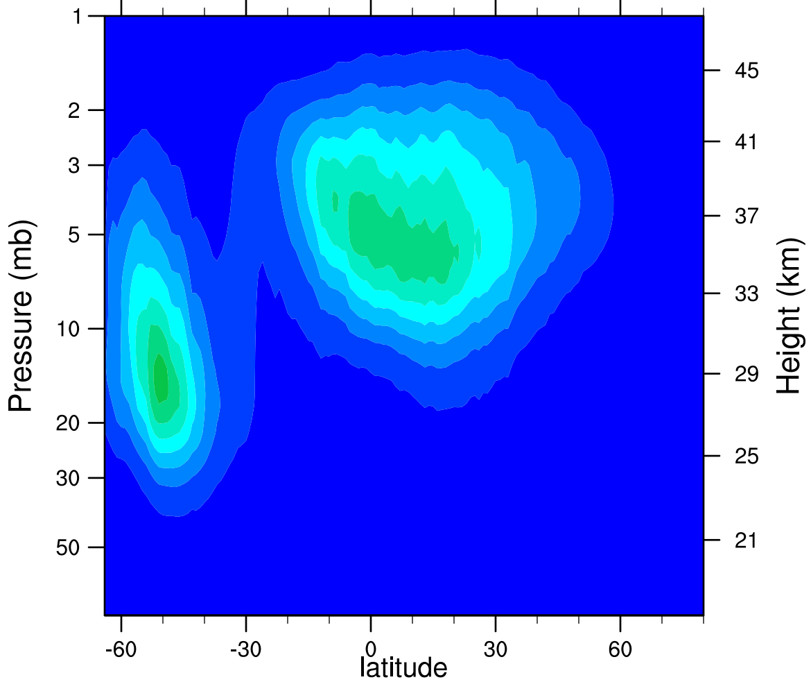
2005d208 N2O5_Ascending (ppbv)
