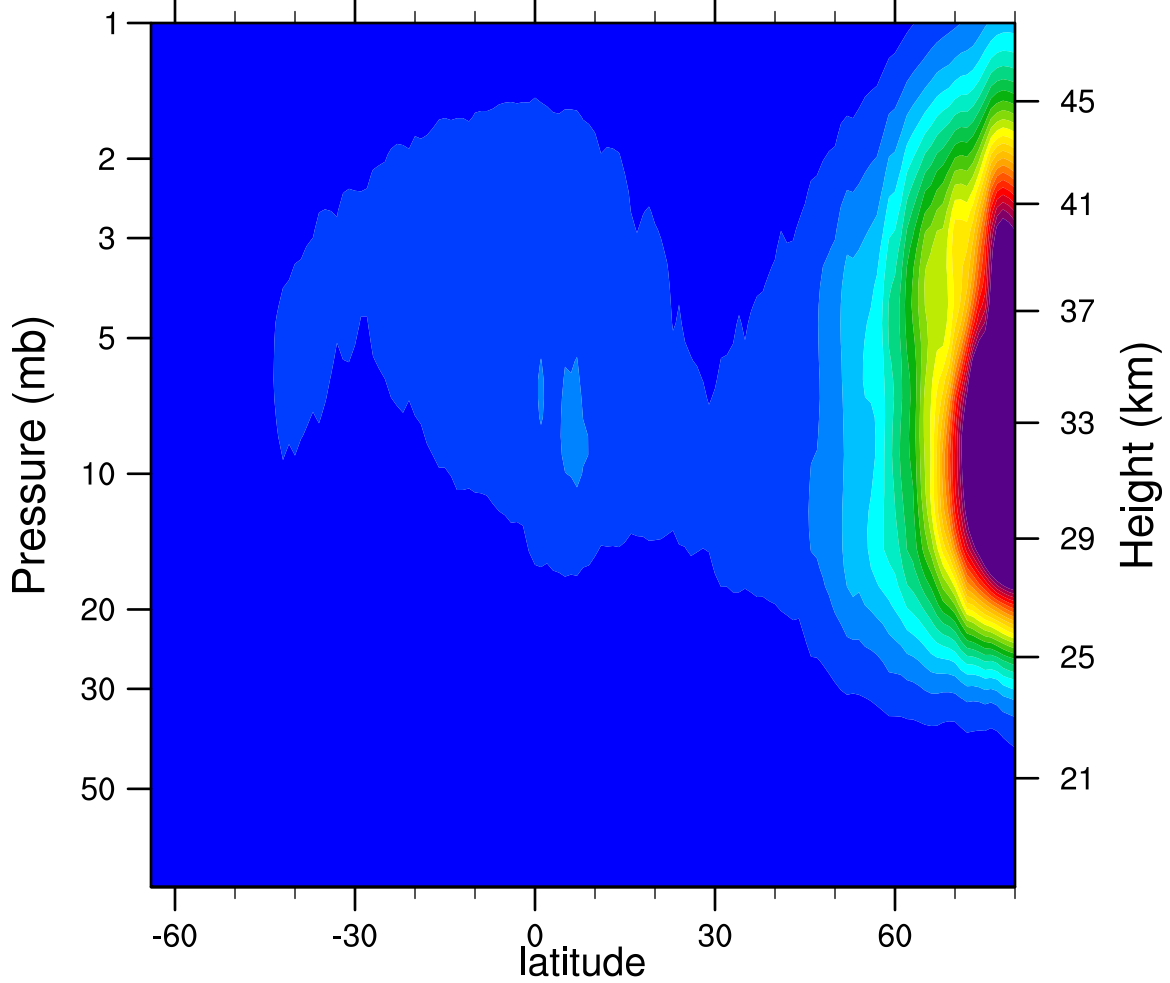
2006d035 N2O5_Ascending (ppbv)
