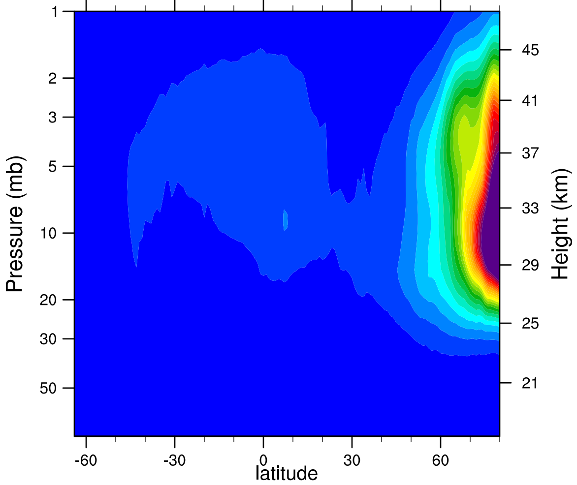
2006d039 N2O5_Ascending (ppbv)
