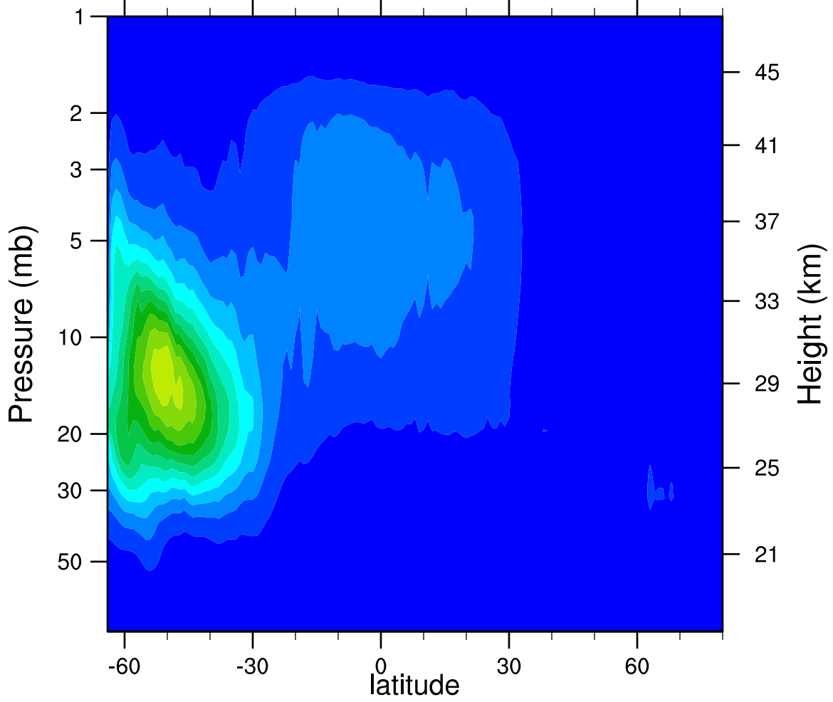
2007d229 N2O5_Ascending (ppbv)
