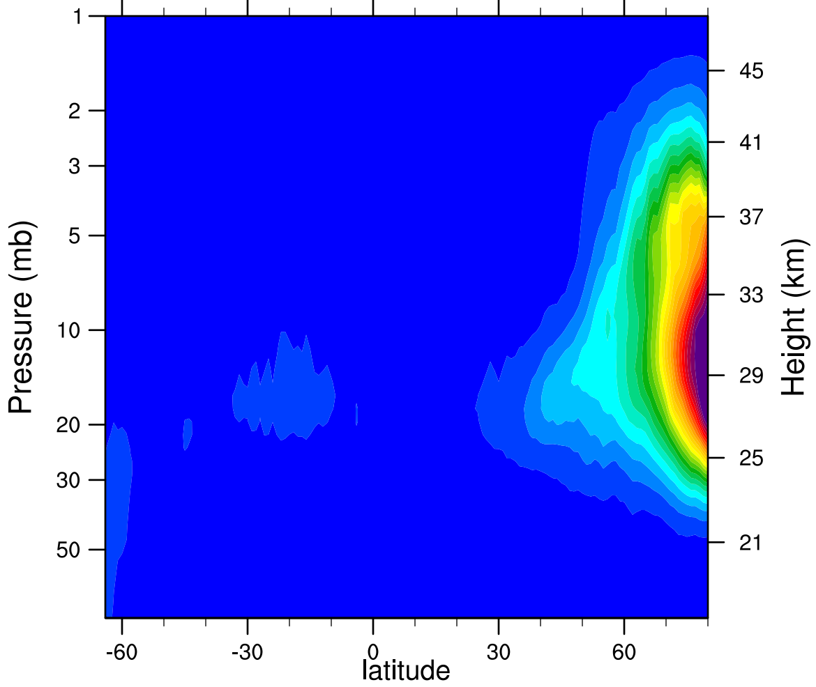
2006d303 N2O5_Ascending (ppbv)
