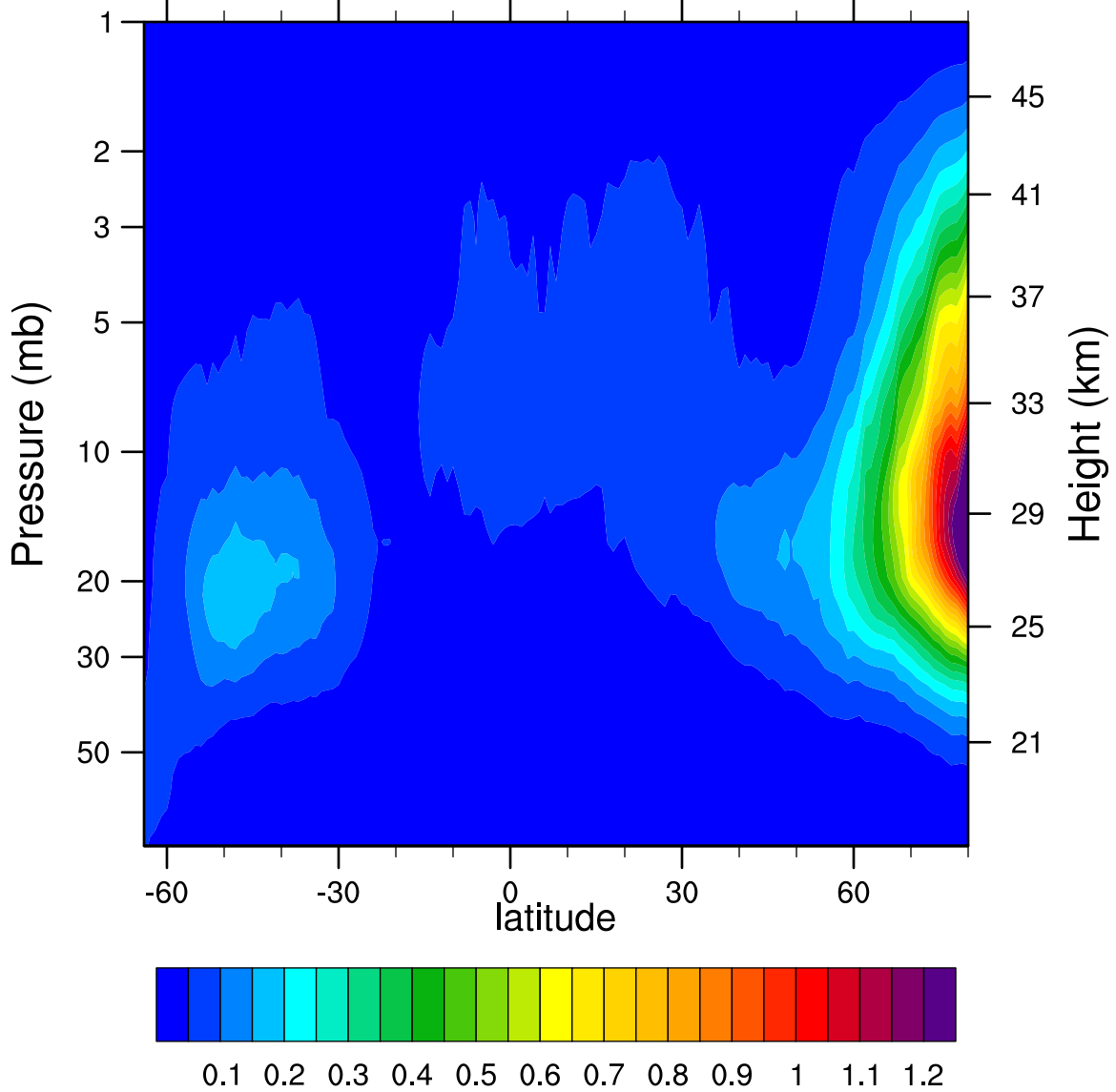
2007d299 N2O5_Ascending (ppbv)
