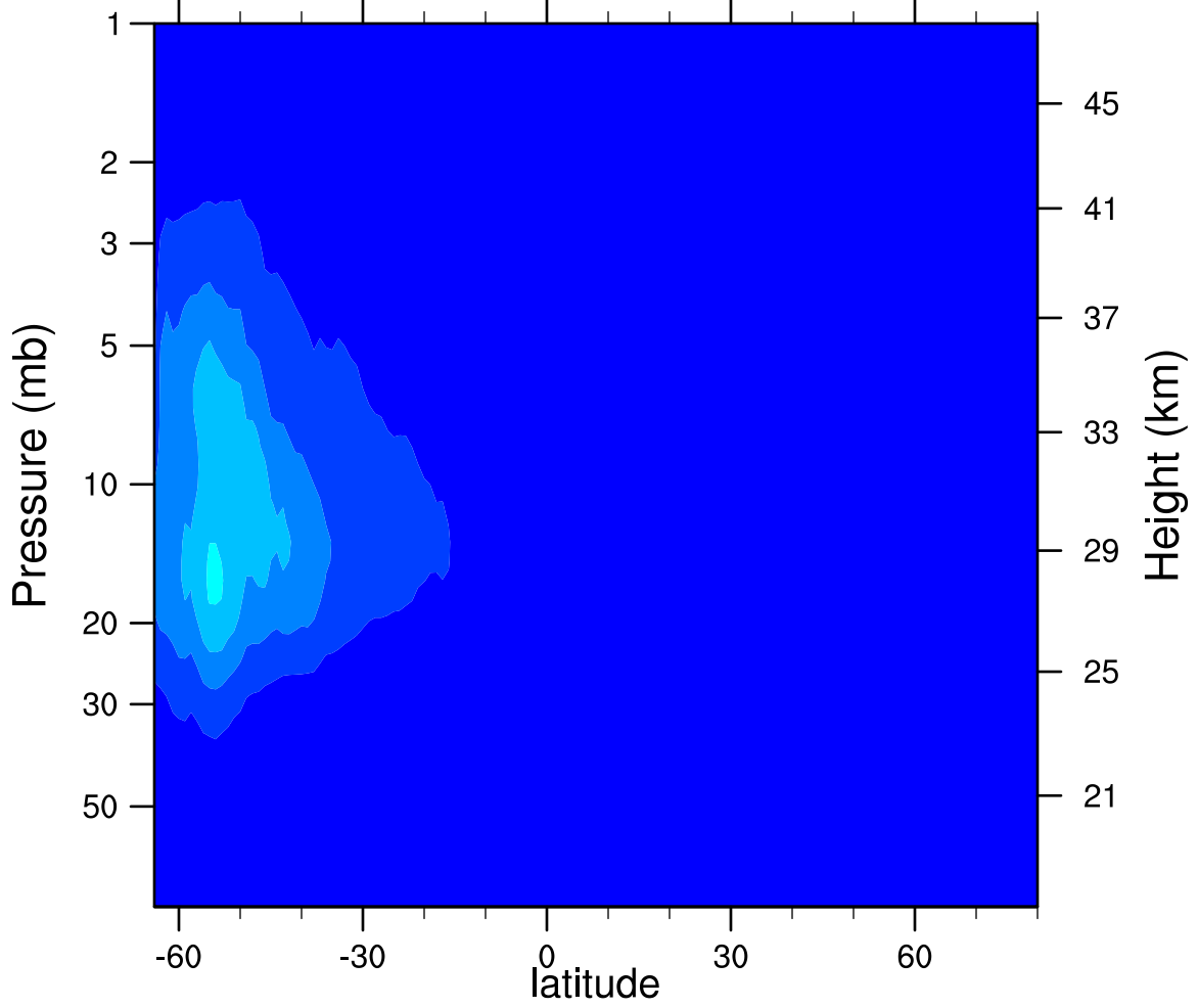
2007d196 N2O5_Ascending (ppbv)
