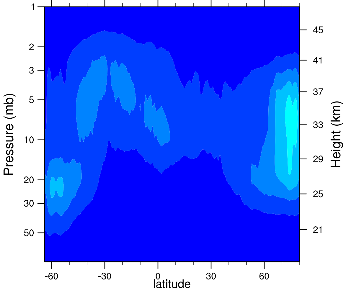
2006d077 N2O5_Ascending (ppbv)
