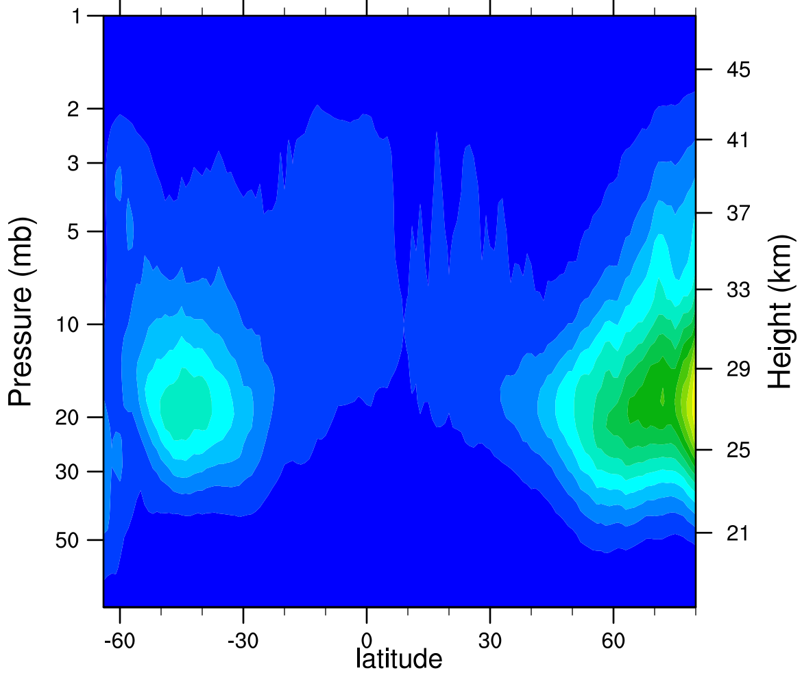
2007d276 N2O5_Ascending (ppbv)
