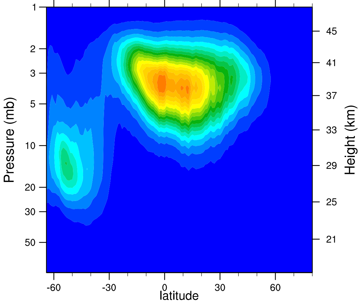
2005d136 N2O5_Ascending (ppbv)
