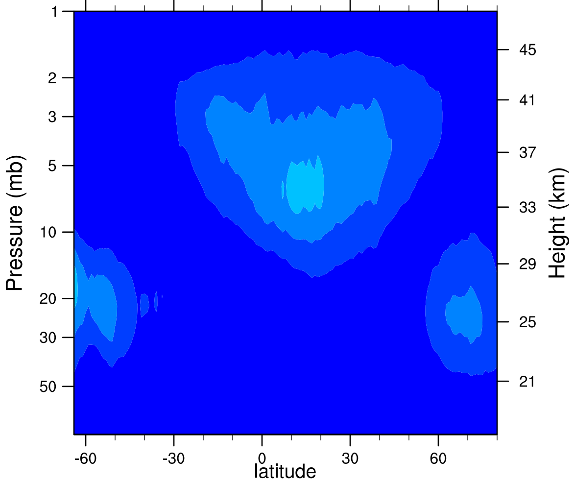
2005d265 N2O5_Ascending (ppbv)
