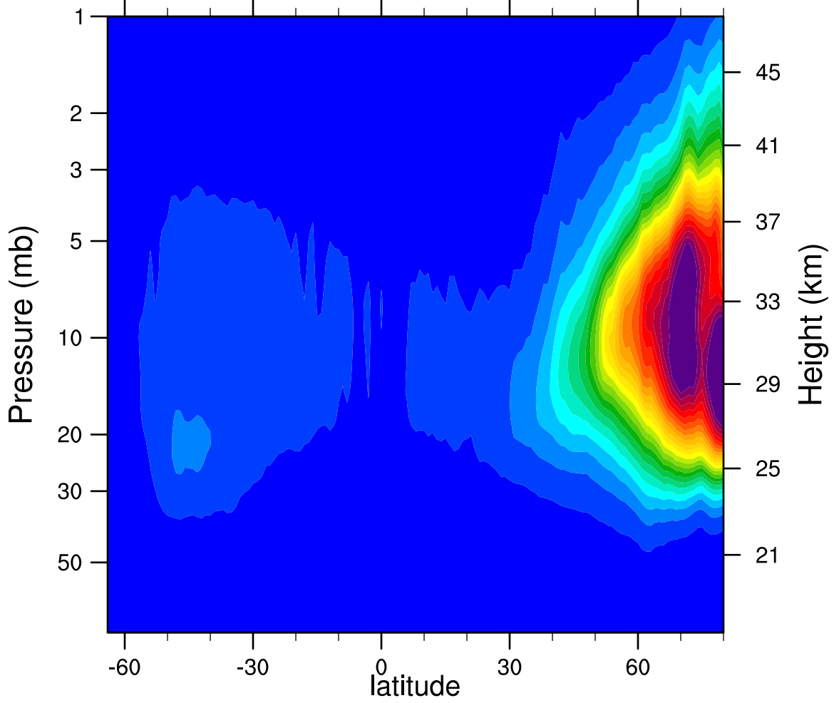
2006d349 N2O5_Ascending (ppbv)
