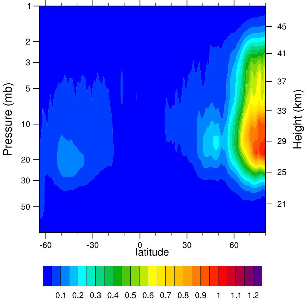
2006d316 N2O5_Ascending (ppbv)
