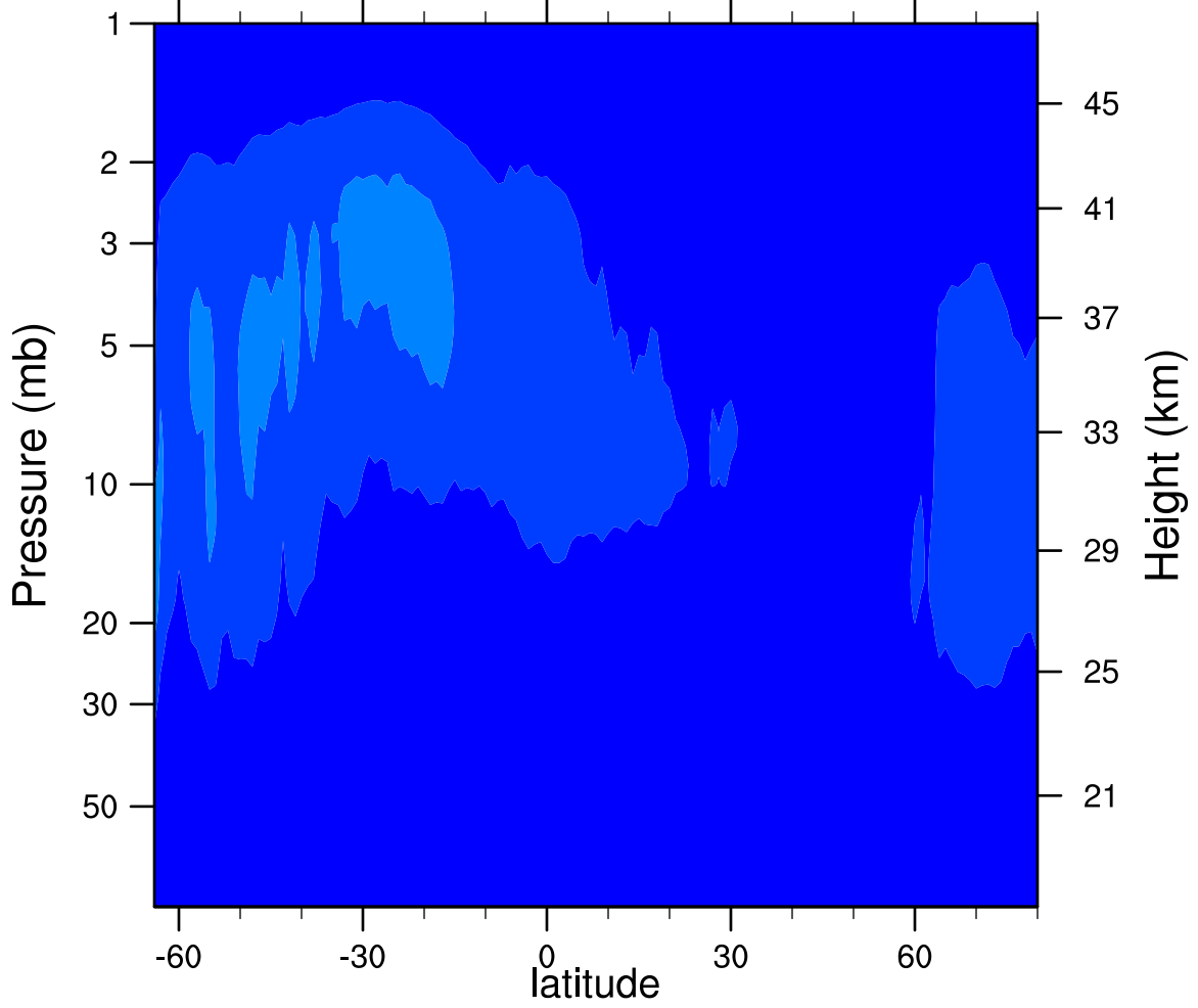
2006d093 N2O5_Ascending (ppbv)
