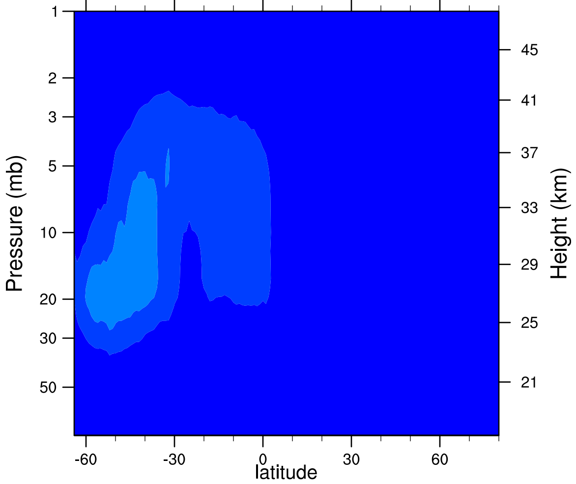
2006d233 N2O5_Ascending (ppbv)
