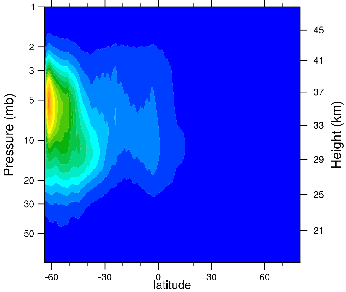
2006d151 N2O5_Ascending (ppbv)
