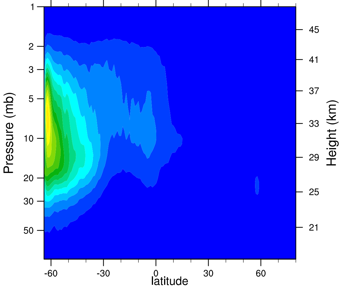
2006d127 N2O5_Ascending (ppbv)
