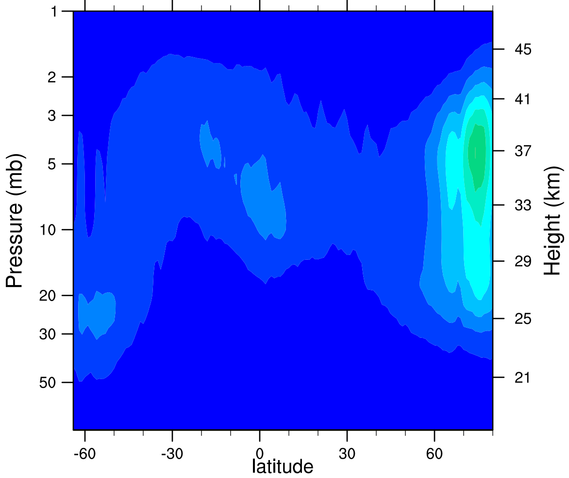
2006d069 N2O5_Ascending (ppbv)
