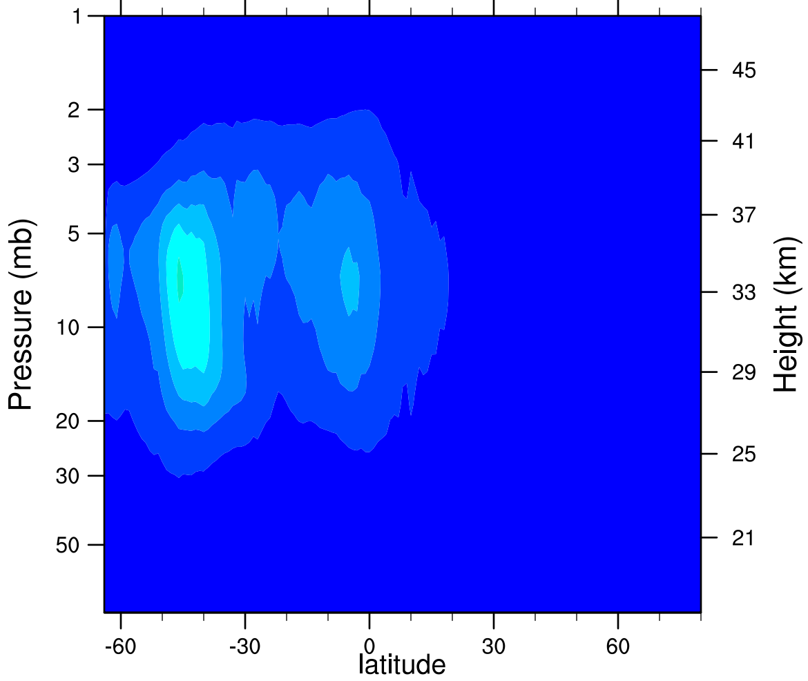
2006d197 N2O5_Ascending (ppbv)
