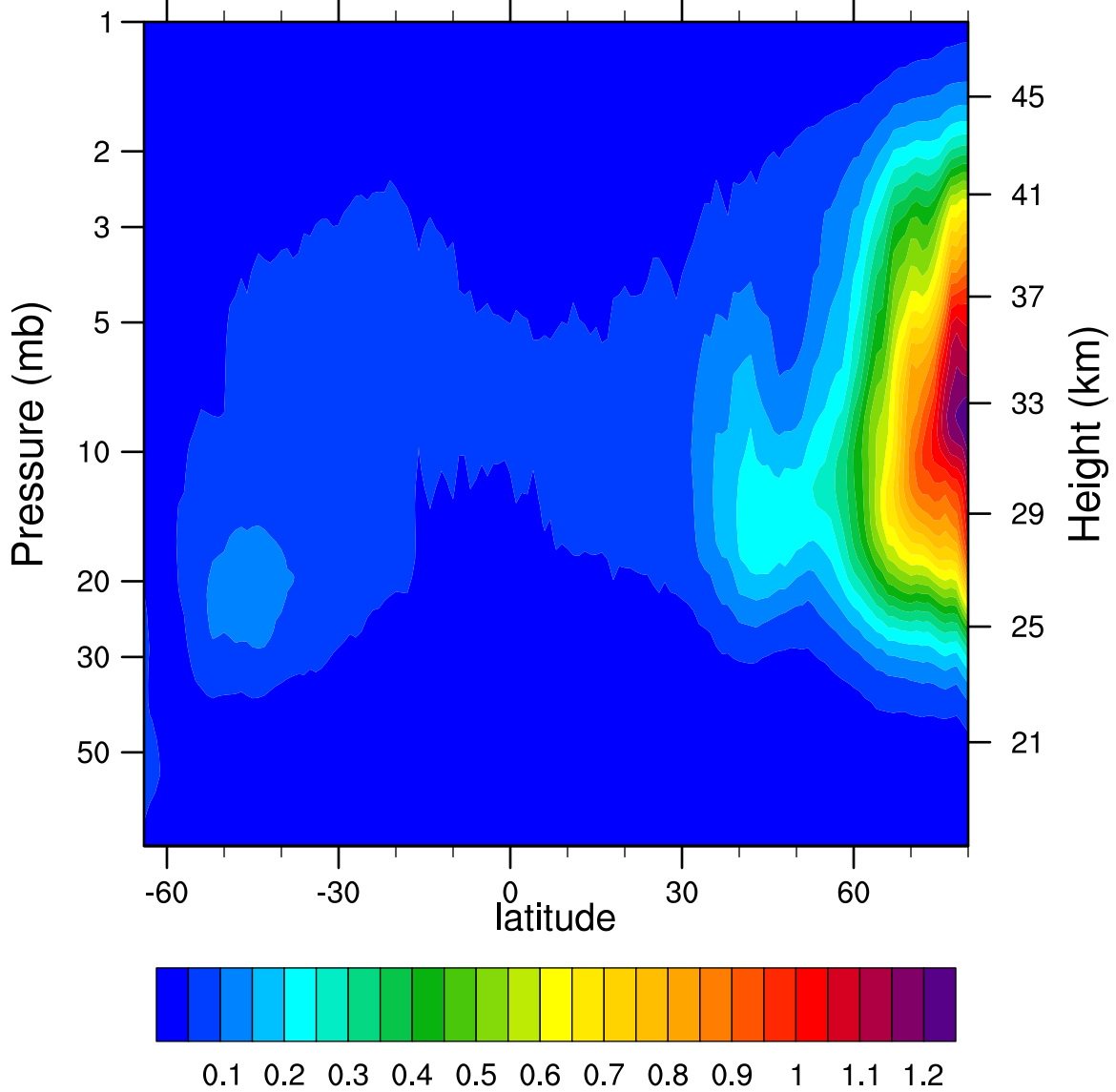
2006d322 N2O5_Ascending (ppbv)
