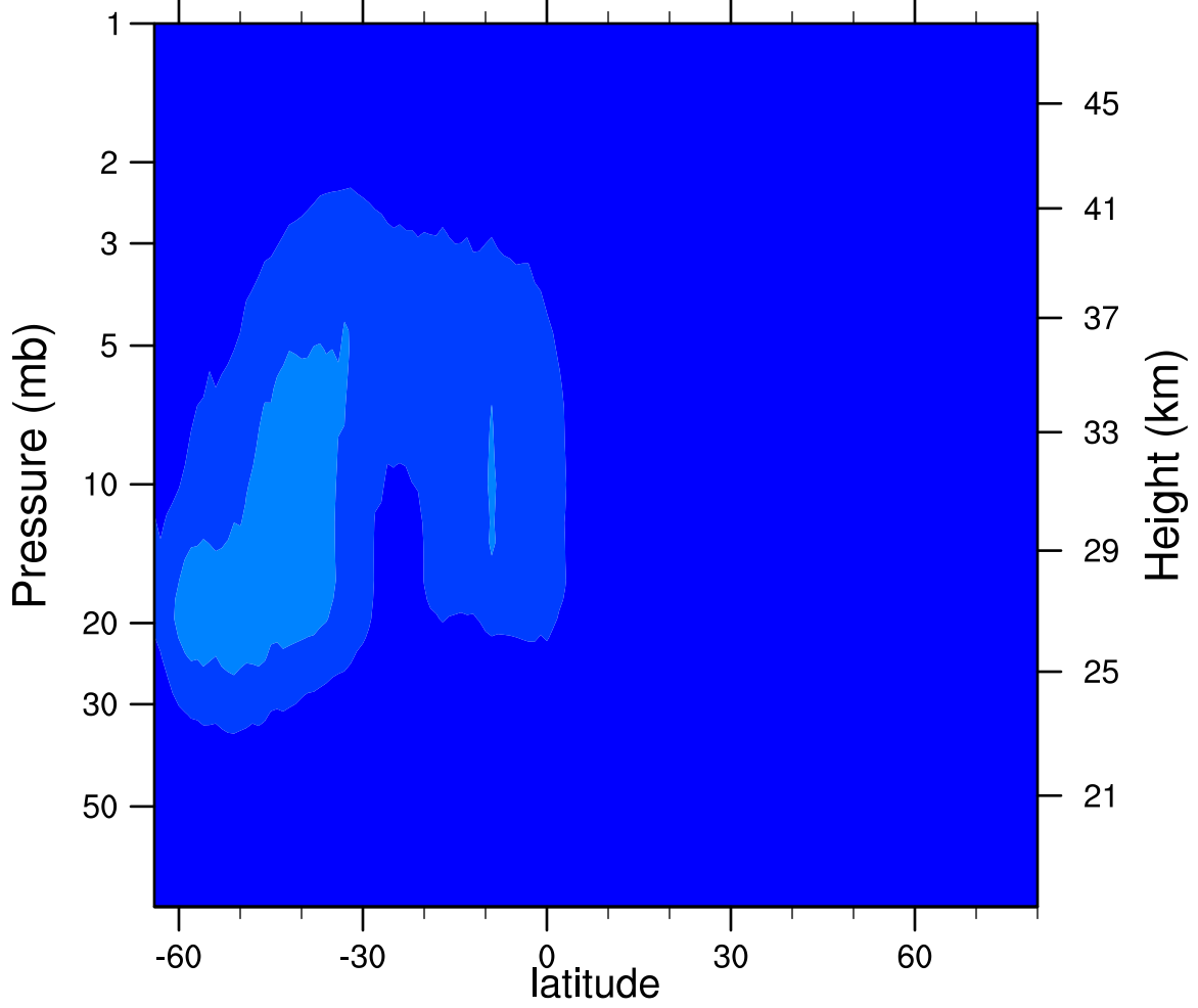
2006d230 N2O5_Ascending (ppbv)
