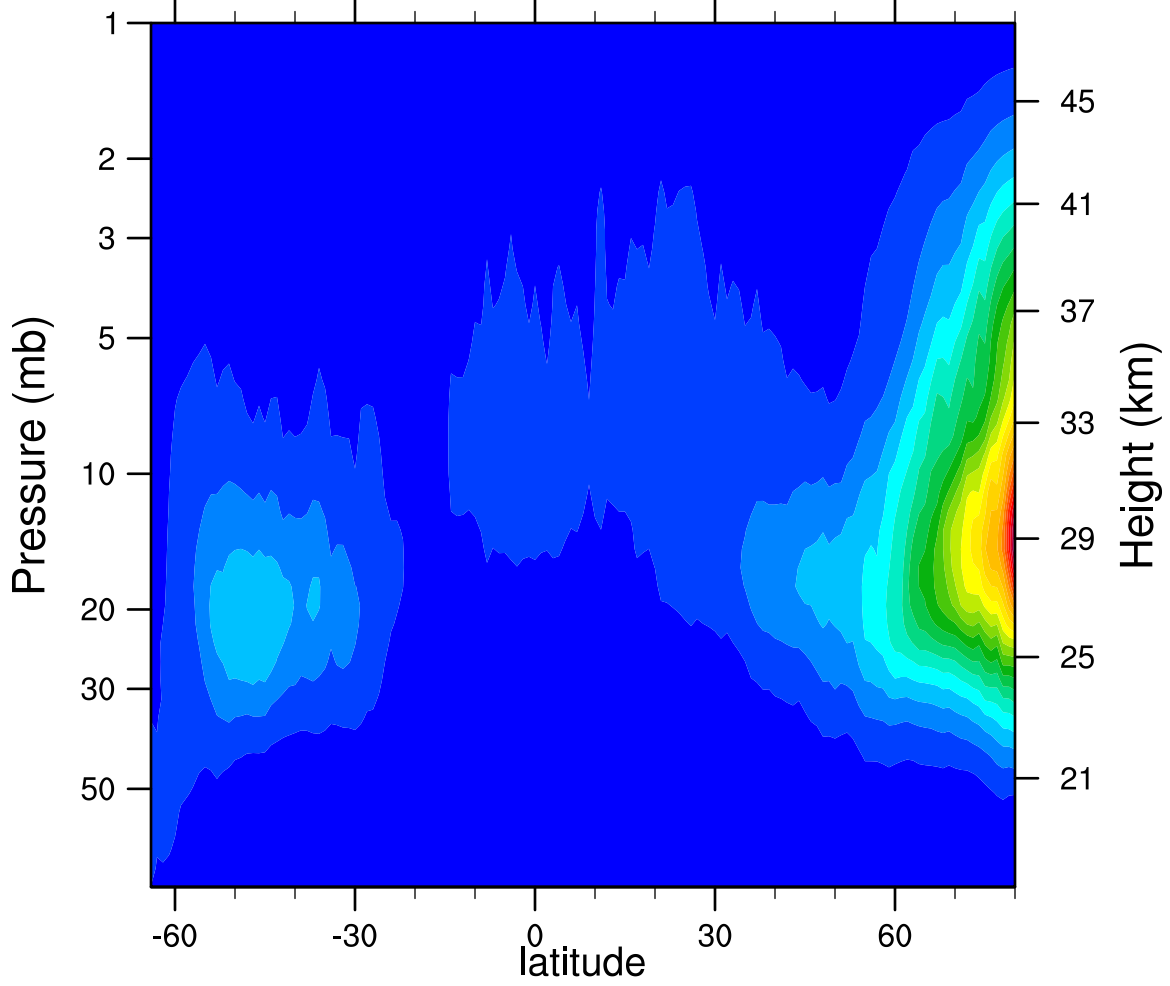
2007d294 N2O5_Ascending (ppbv)
