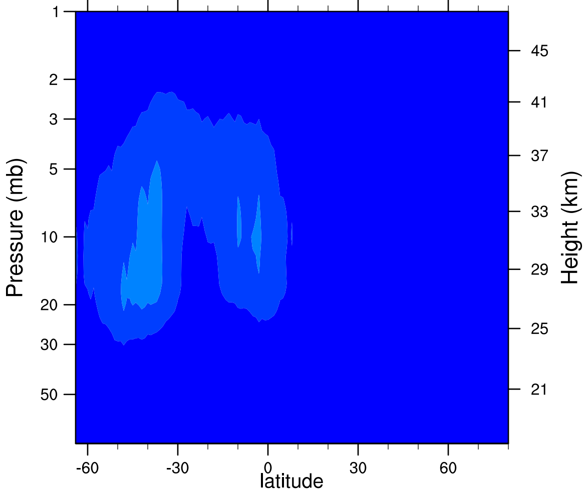
2006d224 N2O5_Ascending (ppbv)
