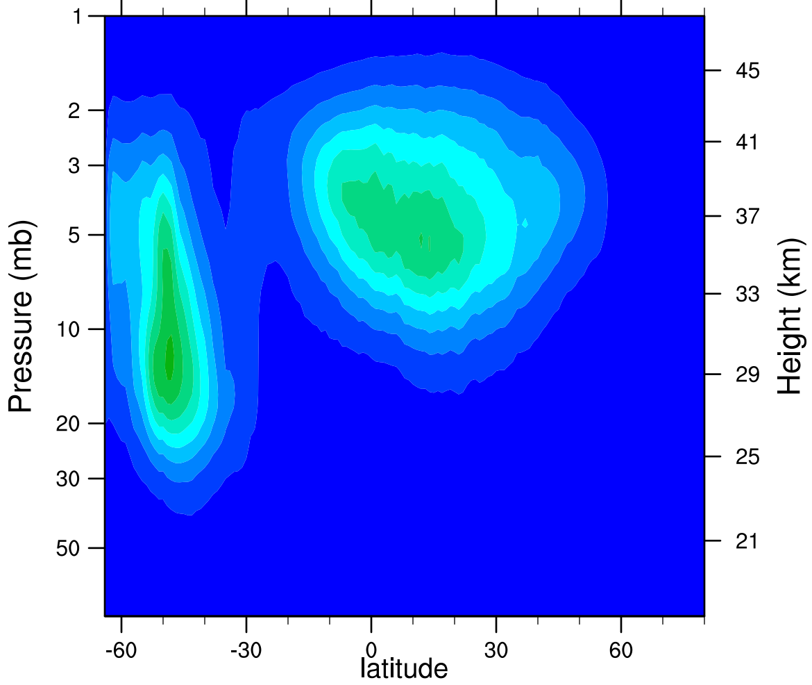
2005d186 N2O5_Ascending (ppbv)
