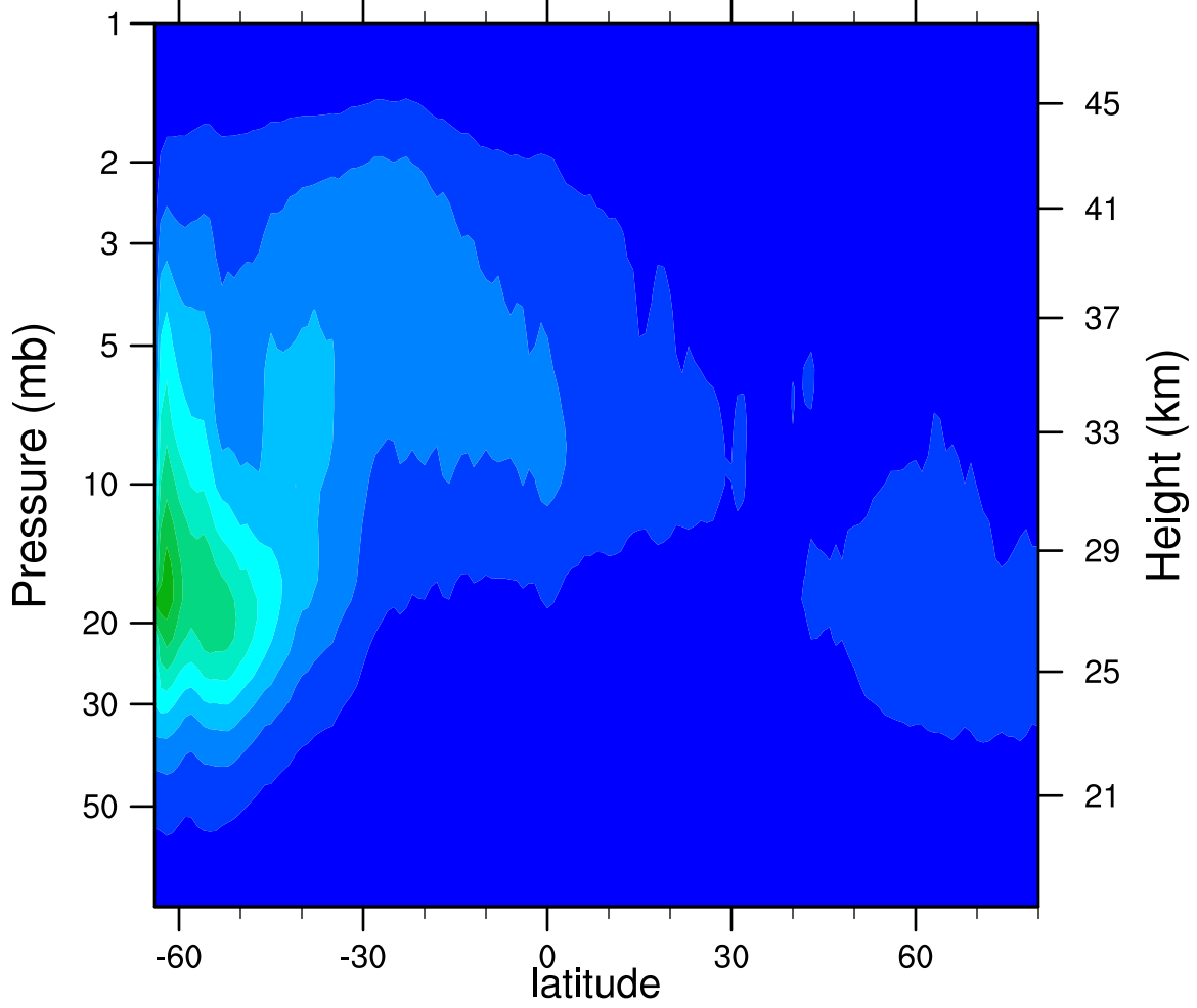
2006d102 N2O5_Ascending (ppbv)
