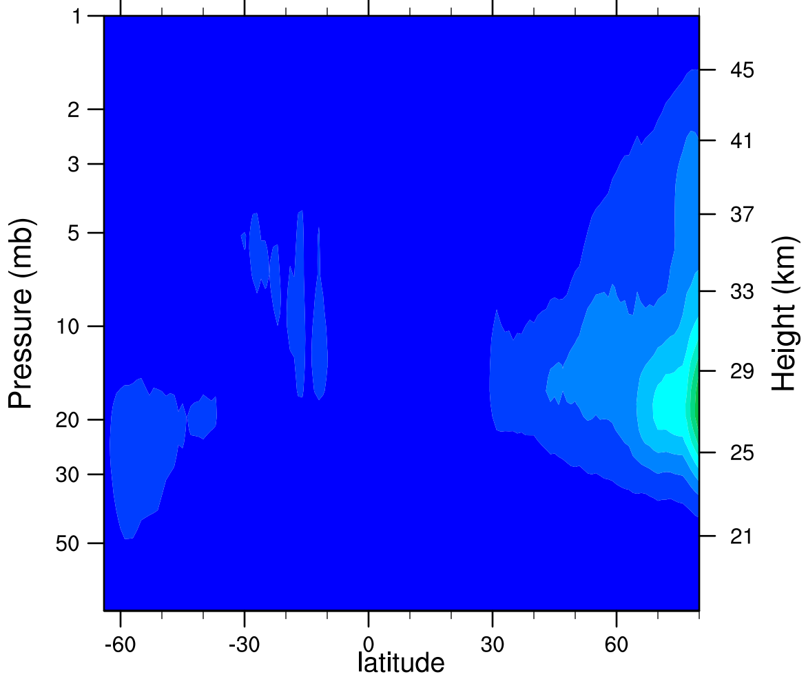
2006d282 N2O5_Ascending (ppbv)
