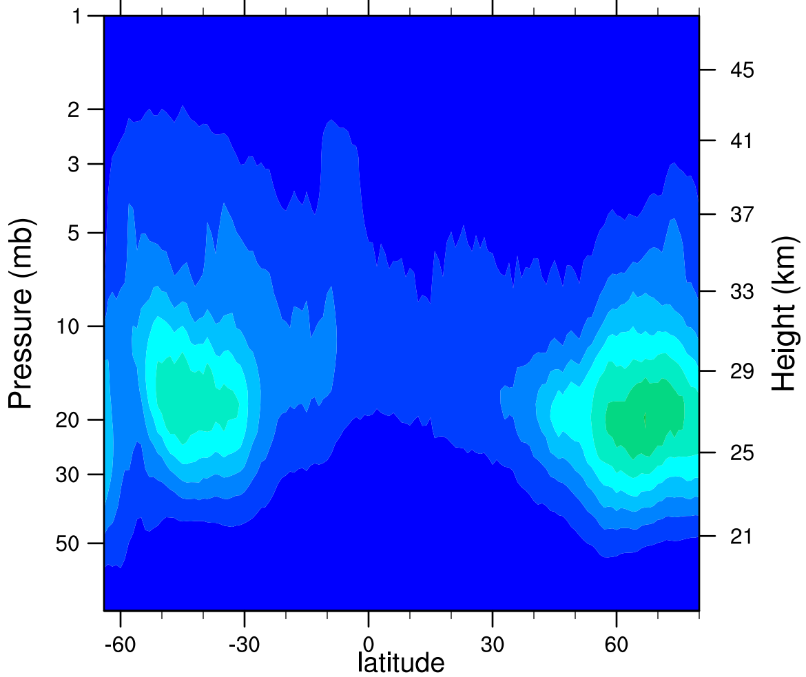
2007d266 N2O5_Ascending (ppbv)
