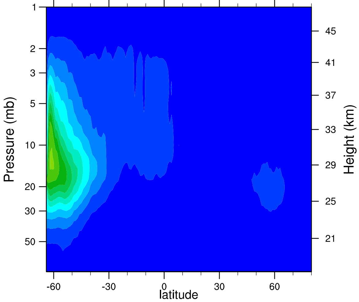
2006d116 N2O5_Ascending (ppbv)
