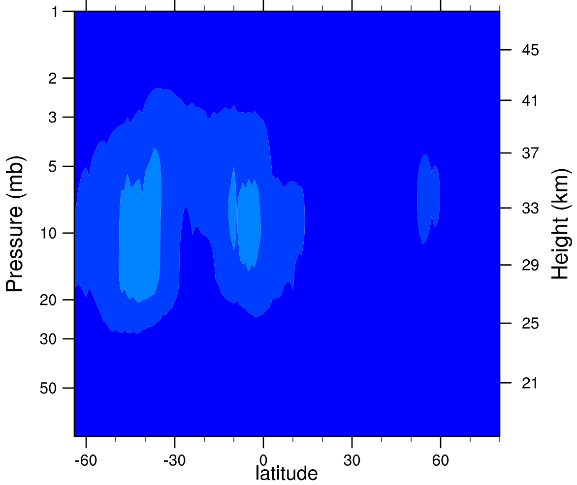
2006d219 N2O5_Ascending (ppbv)
