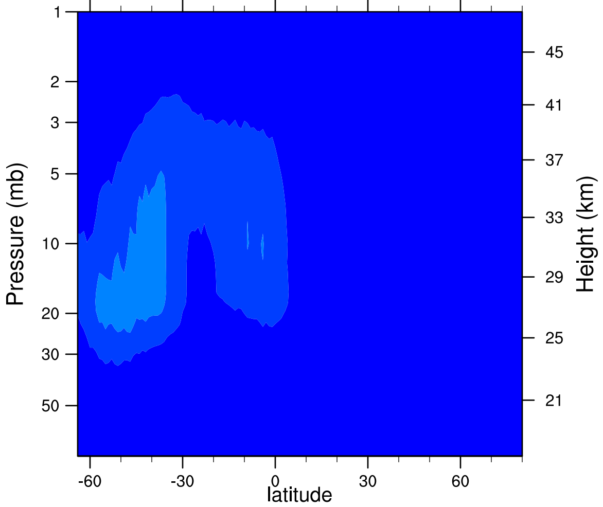
2006d227 N2O5_Ascending (ppbv)
