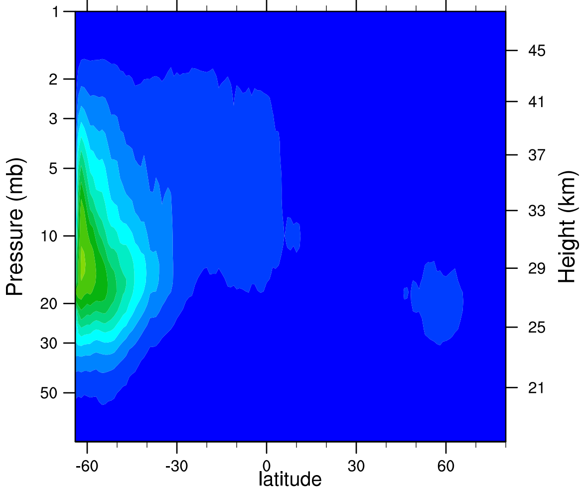
2006d115 N2O5_Ascending (ppbv)
