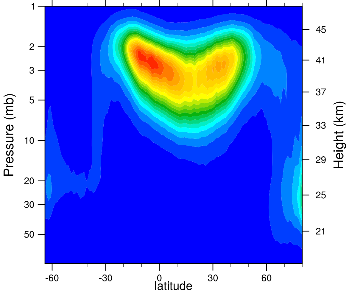
2005d071 N2O5_Ascending (ppbv)
