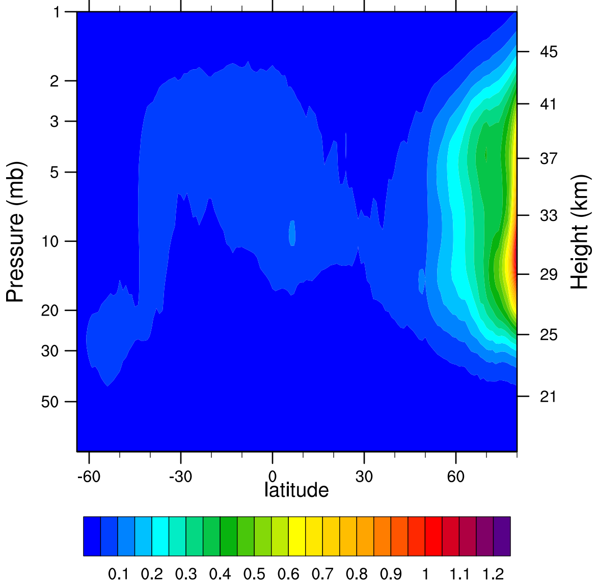
2006d052 N2O5_Ascending (ppbv)
