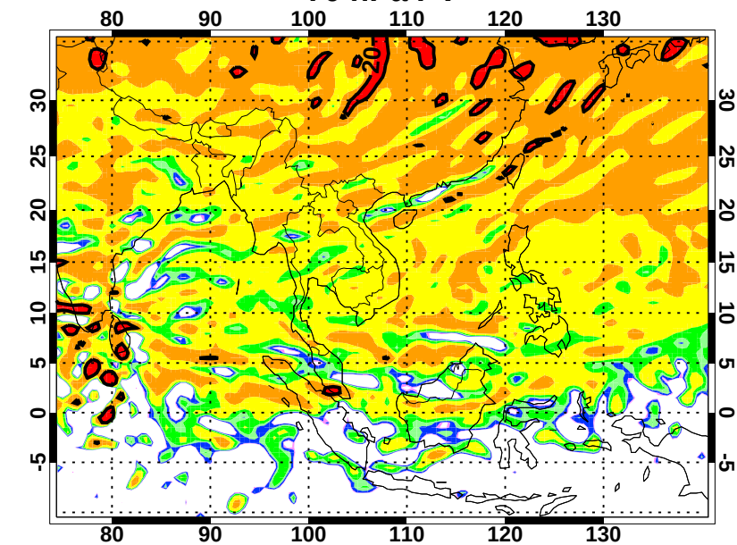
150 hPa PV
