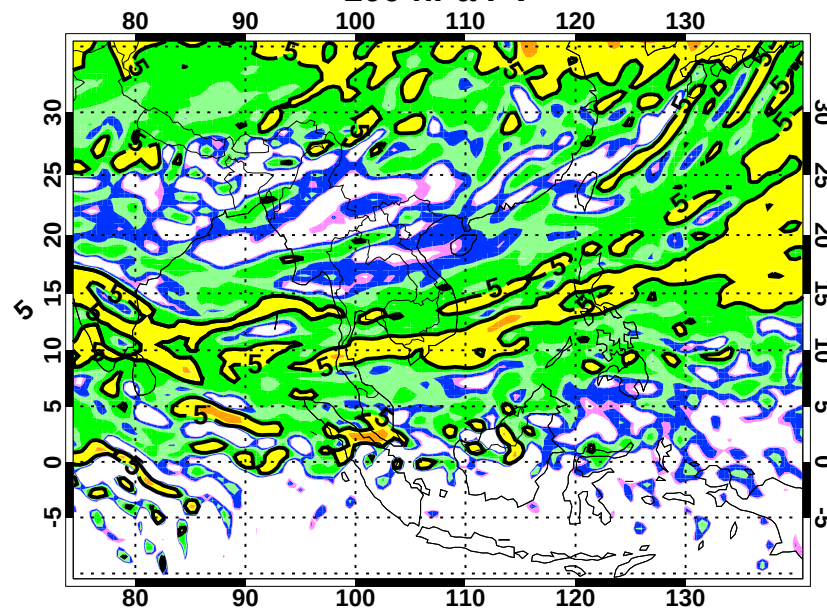
200 hPa PV
