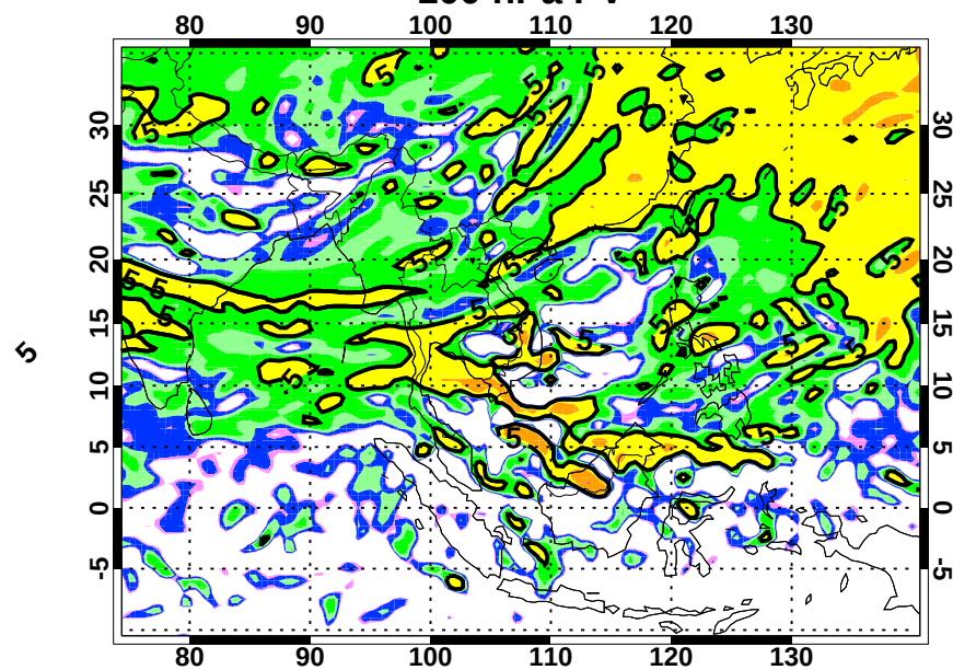
200 hPa PV
