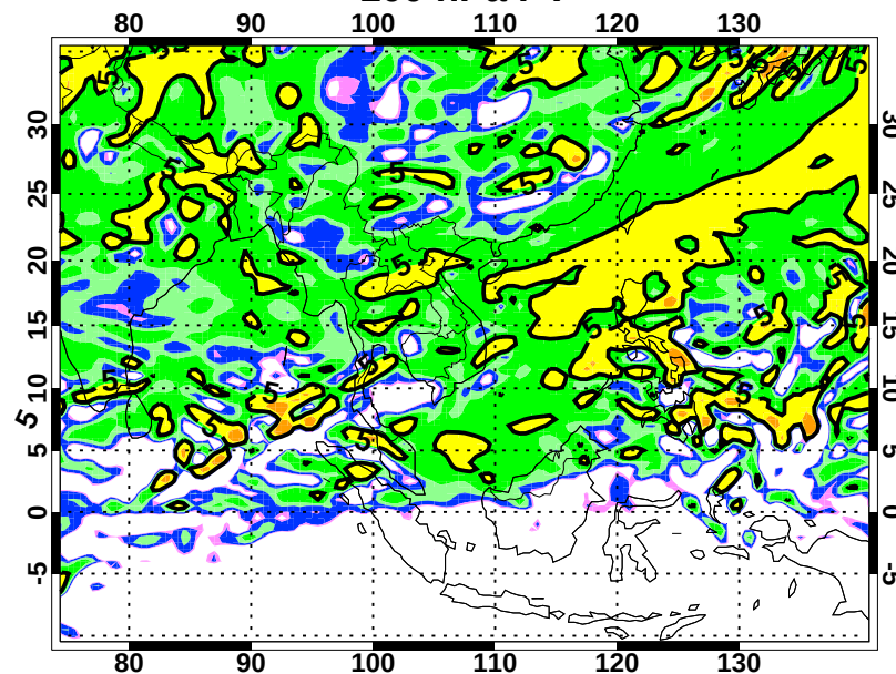
100 hPa PV
