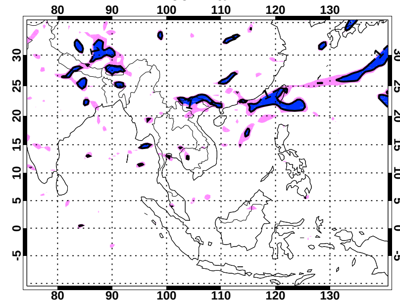
200 hPa PV
