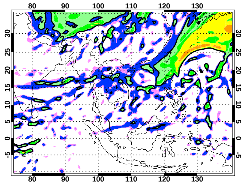
150 hPa PV
