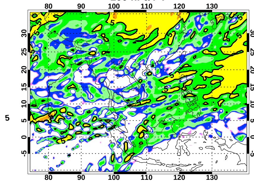
200 hPa PV
