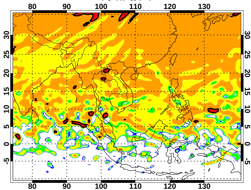
70 hPa PV
