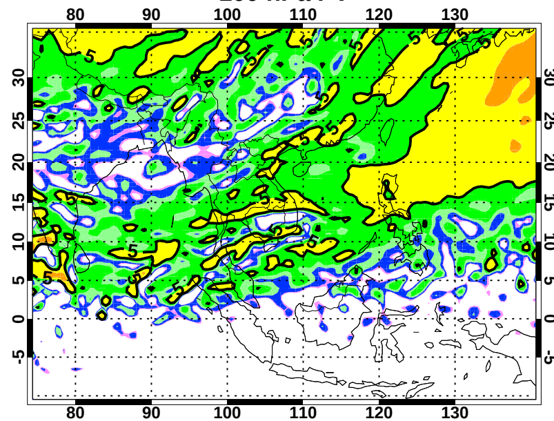
100 hPa PV
