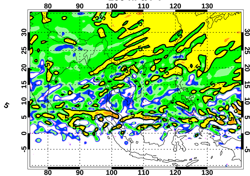
200 hPa PV
